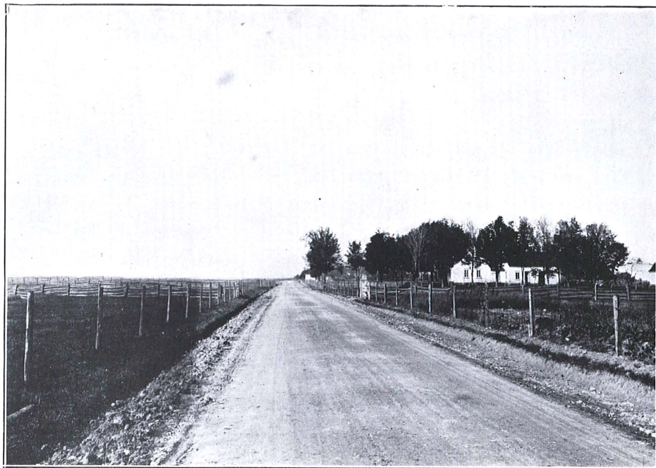
Paroisse Ste-Croix, Lotbinière.—Route Lévis-St-Lambert.—Macadam construit en 1923
