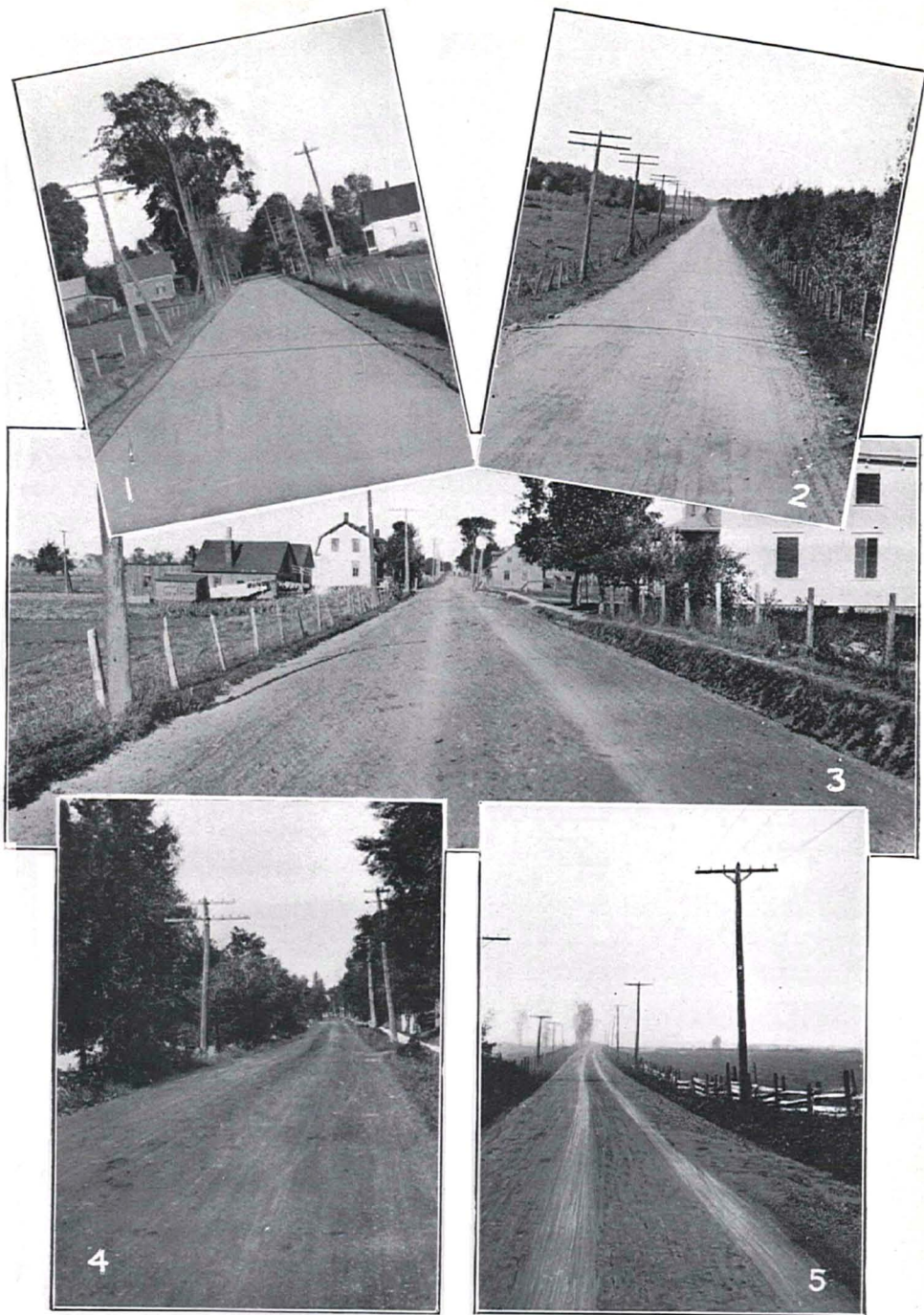
1.—Mariville, route Montréal-Sherbrooke, rue Chambly, béton. 2.—Paroisse Rougemont, route Montréal-Sherbrooke, gravelage. 3.—St-Jean-Baptiste, Rouville; chemin sud de la rivière, gravelage. 4.—Village St-Hilaire, Rouville; chemin du bord de l'eau gravelage arrosé d'huile. 5.—Wendover et Simpson, Richmond, route Drummondville Annville; gravelage.
