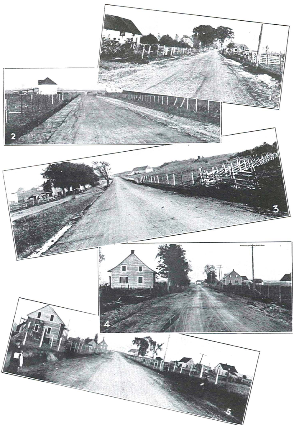
Route Lévis-Saint-Lambert.—1.—Lotbinière, est, macadam en construction; 2.—St-Croix, macadam en construction; 3.—St-Nicolas; macadam terminé en 1923; 4.—Gentilly, ouest du village, macadam en construction; 5.—Gentilly, est du village, macadam terminé en 1923.
