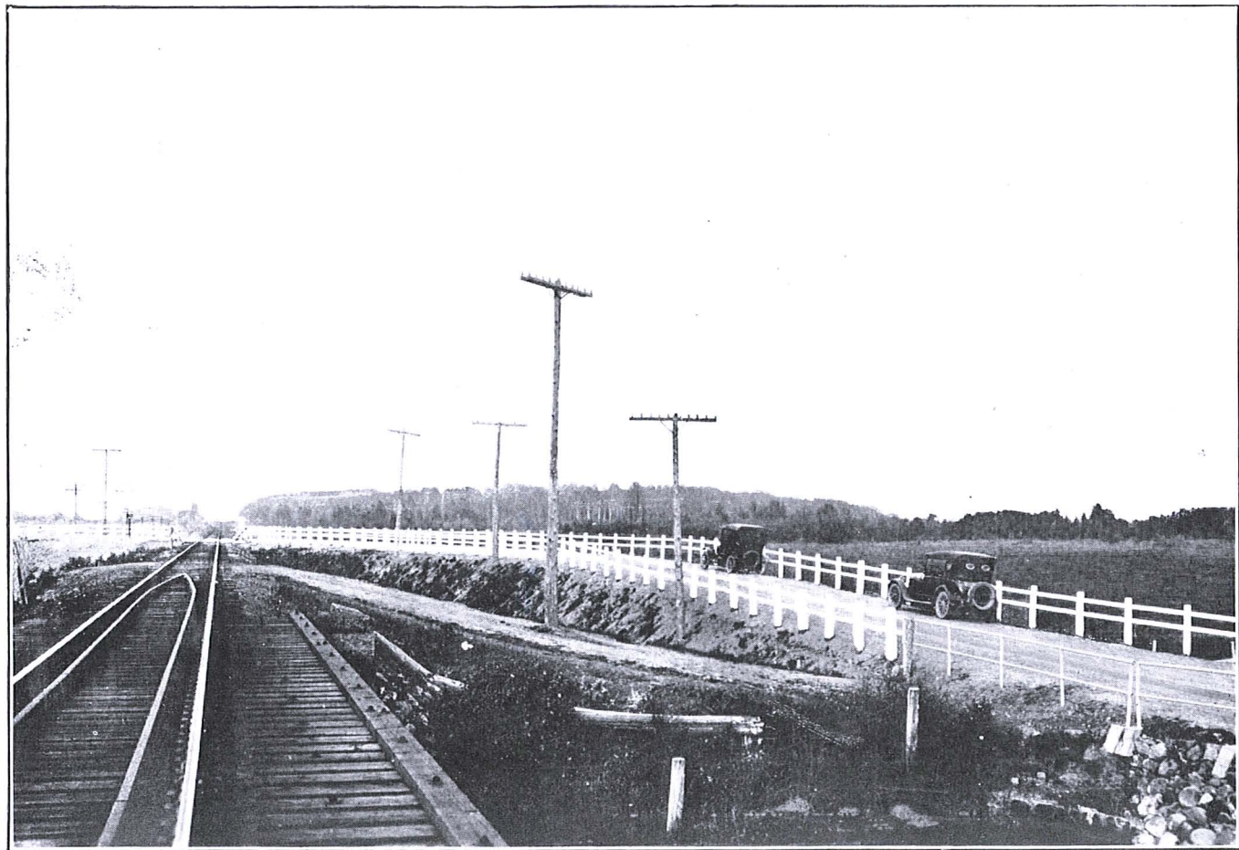
Canton Stanford, Arthabaska.—Route Lévis-Sherbrooke.—Traverse à niveau sur le Grand-Tronc.
