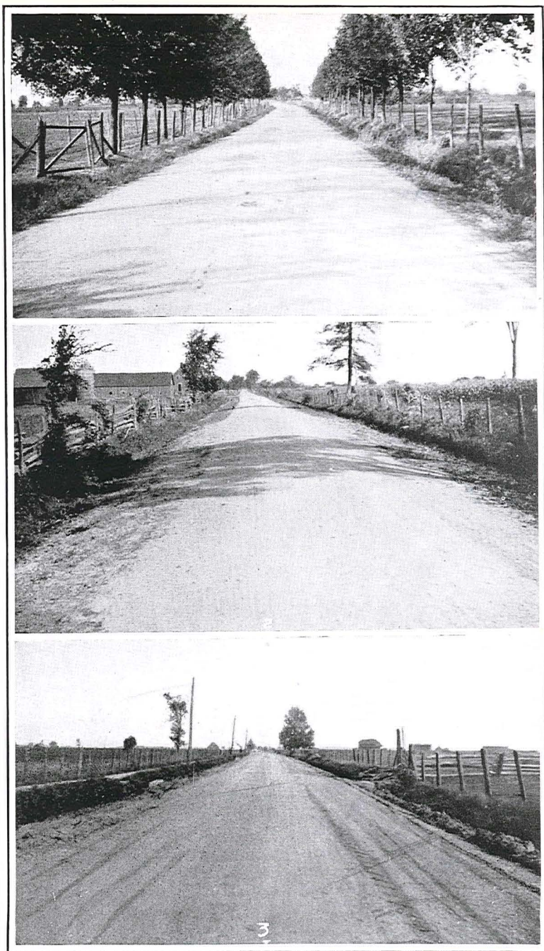
De haut en bas 1. Laprairie, paroisse, comté de Laprairie, macadam bitumineux fait en 1921 ; 2. Napierville, paroisse, comté de Napierville, macadam fait en 1921 ; 3. Ste-Marguerite, comté de St-Jean, macadam fait en 1921.
