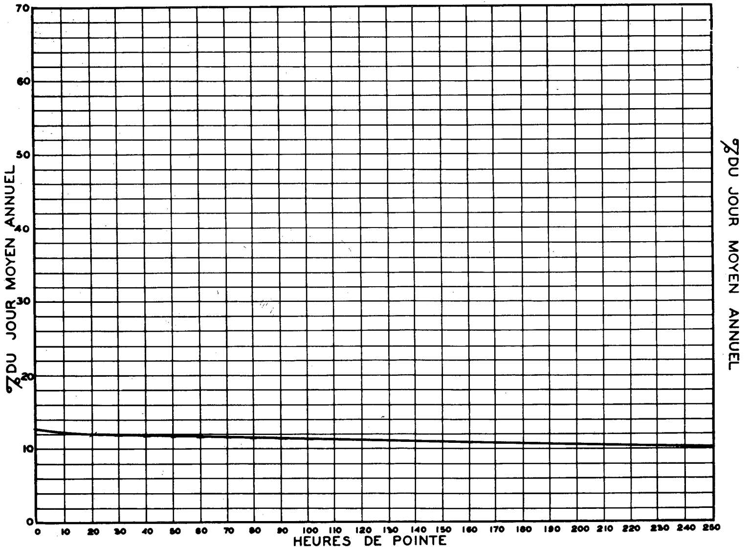
RELATION ENTRE LES HEURES DE POINTE ET LE JOUR MOYEN ANNUEL STATION: ST-ROMUALD (VOIE SUD) ROUTE N° 2-1-4
