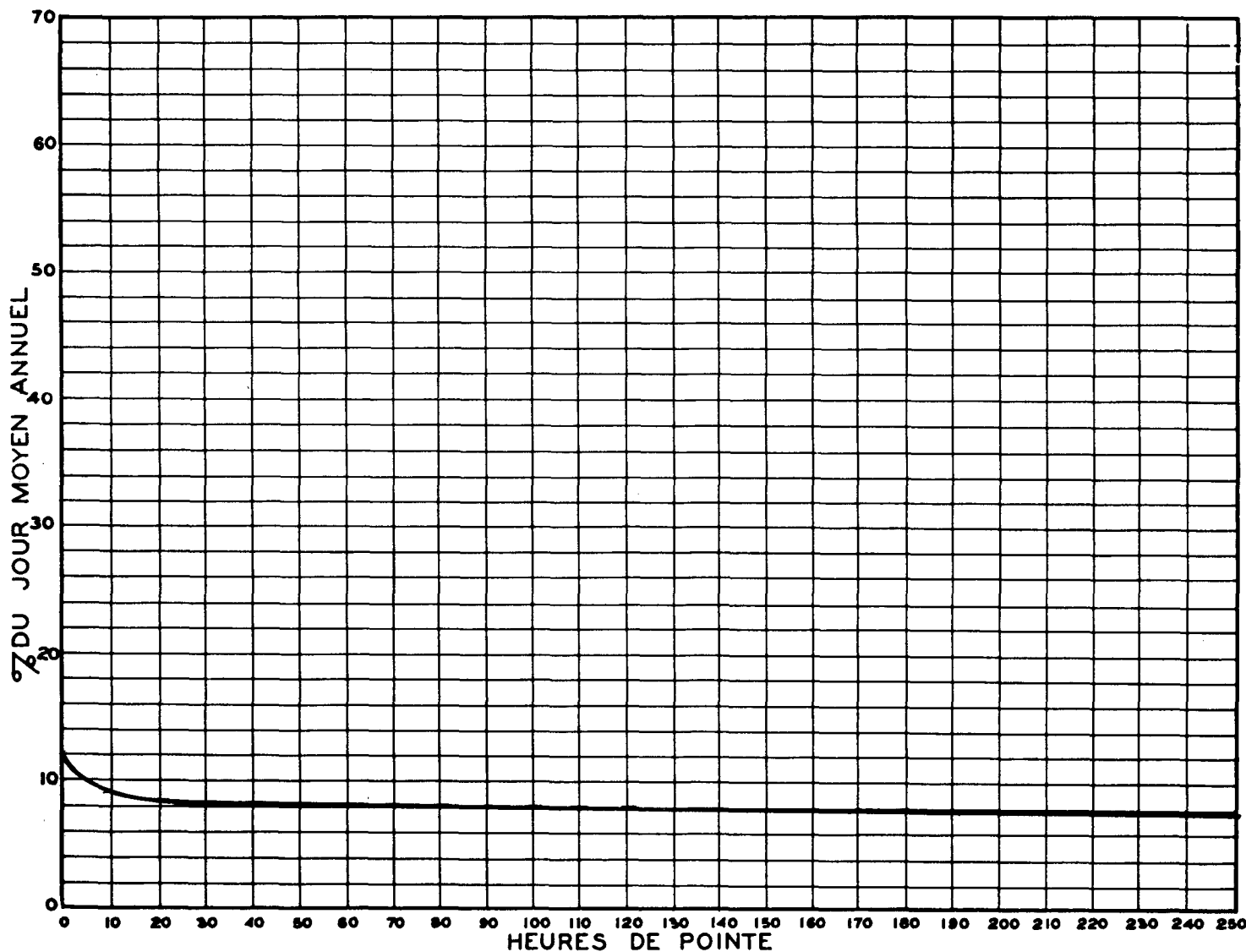
RELATION ENTRE LES HEURES DE POINTE ET LE JOUR MOYEN ANNUEL STATION: LAVAL (2 VOIES) ROUTE N°11-4-81
