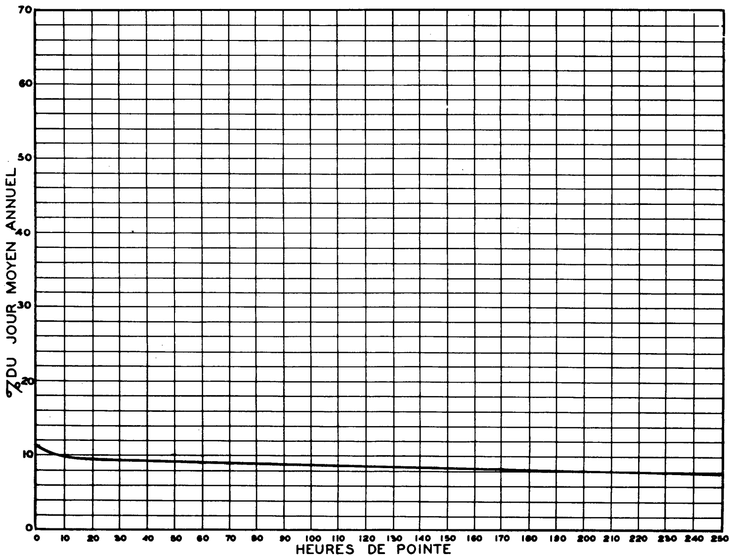
RELATION ENTRE LES HEURES DE POINTE ET LE JOUR MOYEN ANNUEL STATION: ROSEMERE ROUTE N° 11-5-62
