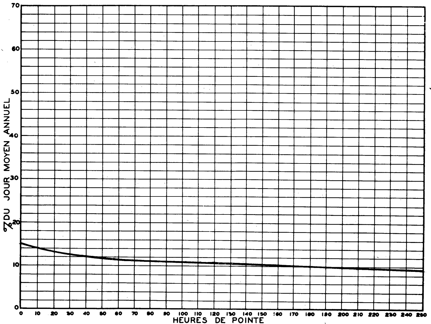
RELATION ENTRE LES HEURES DE POINTE ET LE JOUR MOYEN ANNUEL STATION: CADILLAC ROUTE N° 59-6-52
