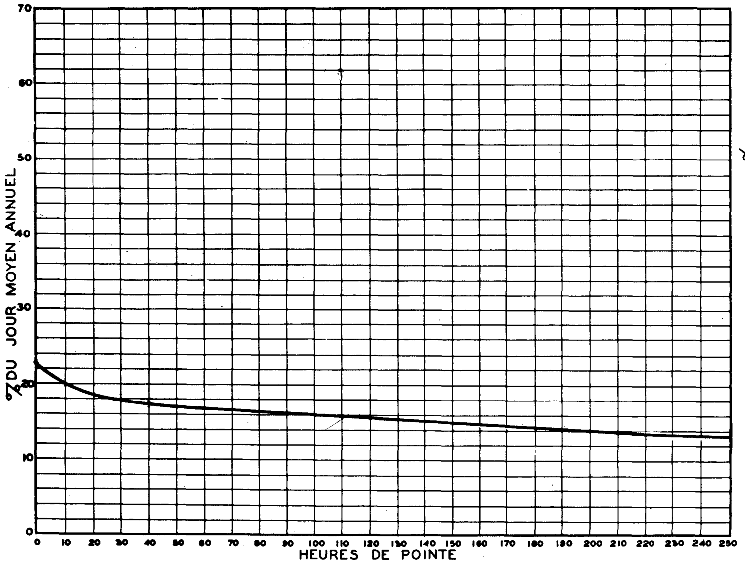
RELATION ENTRE LES HEURES DE POINTE ET LE JOUR MOYEN ANNUEL STATION: POINTE FORTUNE ROUTE N° 40-4-52
