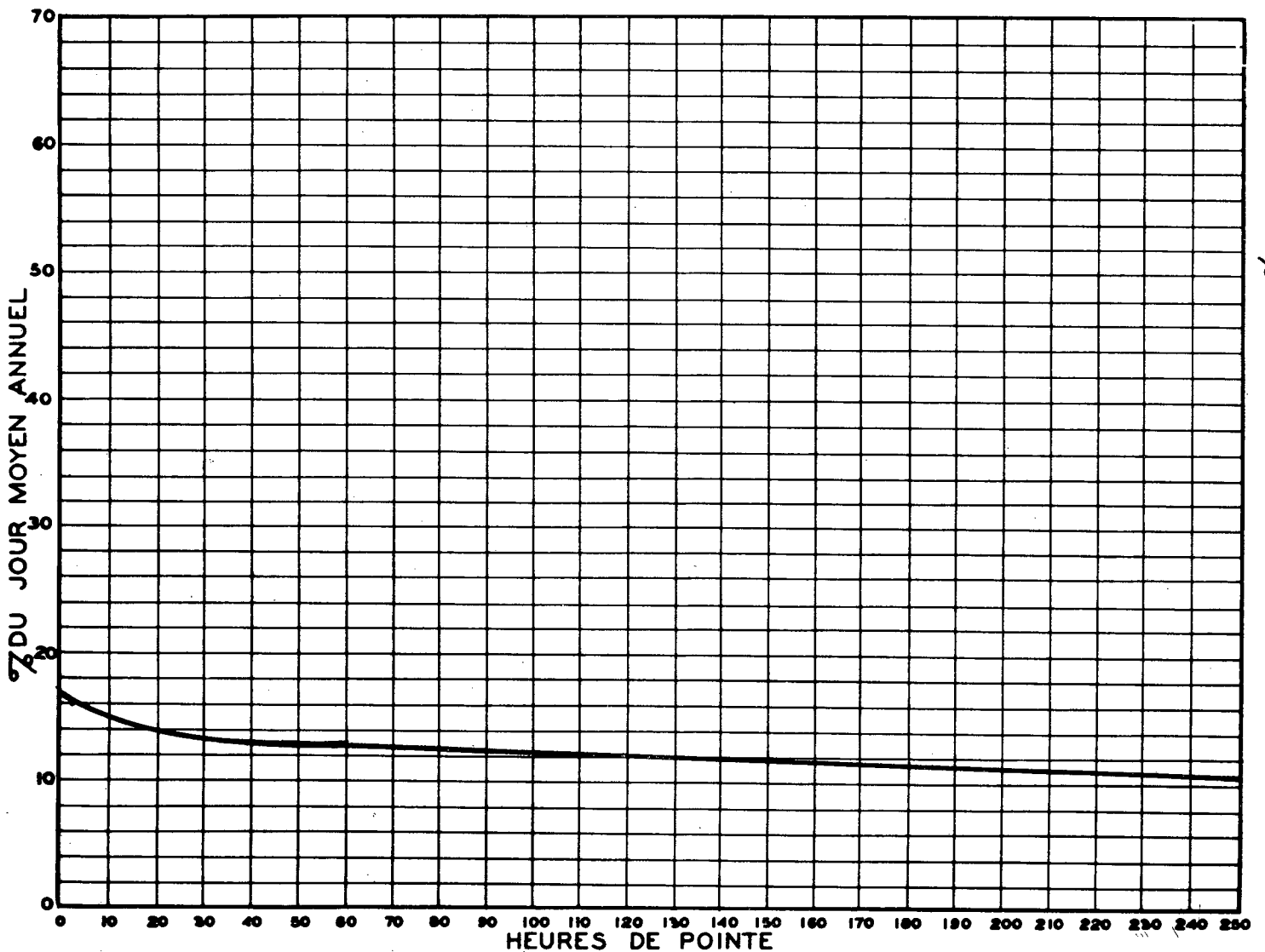
RELATION ENTRE LES HEURES DE POINTE ET LE JOUR MOYEN ANNUEL STATION: ST-HENRI-DE-TAILLON ROUTE N o 55-7-2
