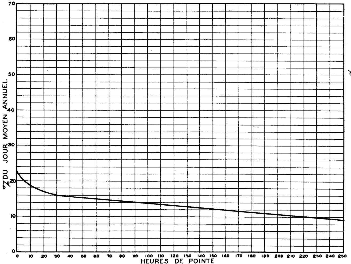
RELATION ENTRE LES HEURES DE POINTE ET LE JOUR MOYEN ANNUEL STATION: NOTRE-DAME-DES-LAURENTIDES ROUTE N° 54-1-17
