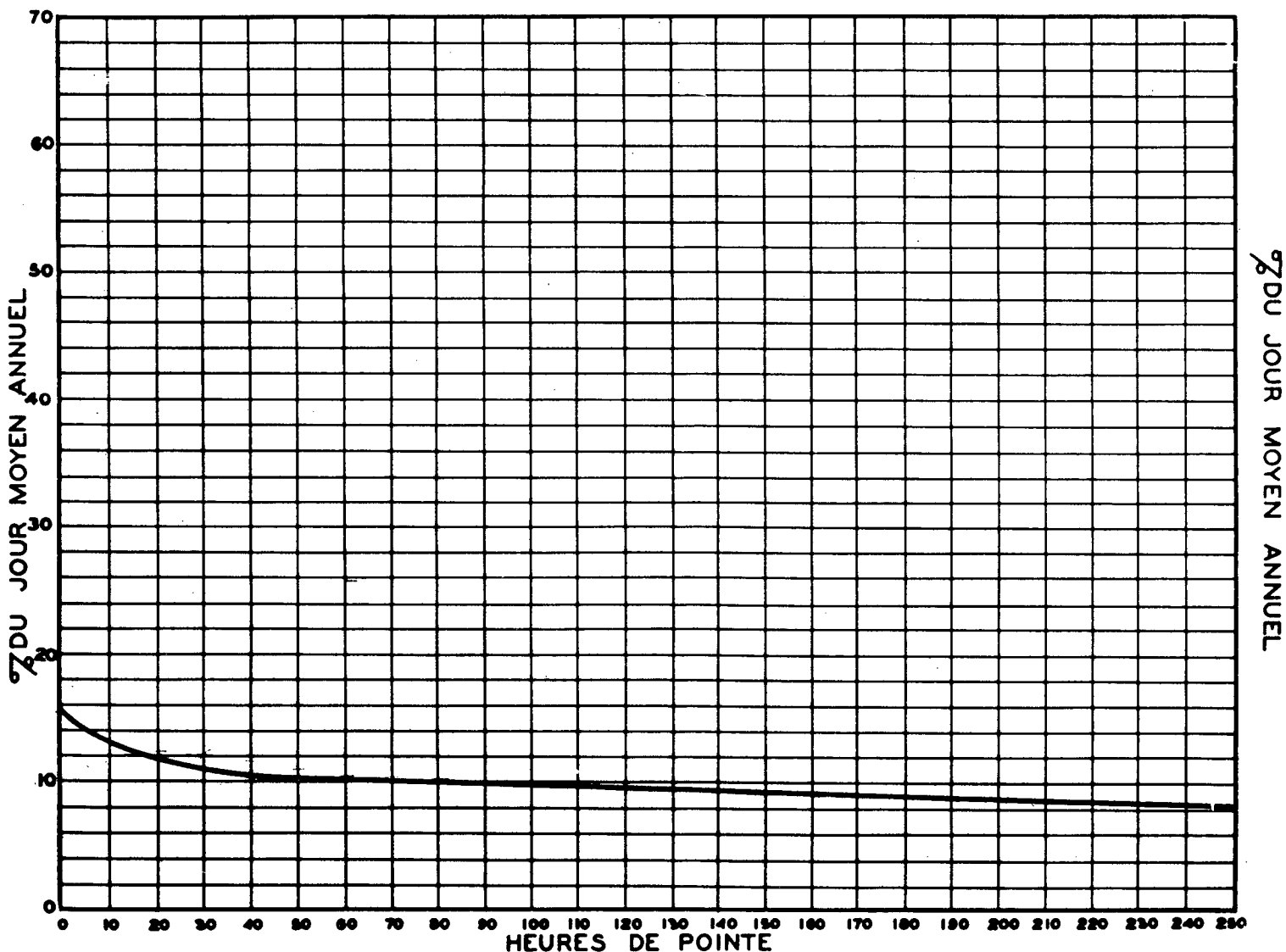
RELATION ENTRE LES HEURES DE POINTE ET LE JOUR MOYEN ANNUEL STATION: LAUZON ROUTE N° 2-1-17
