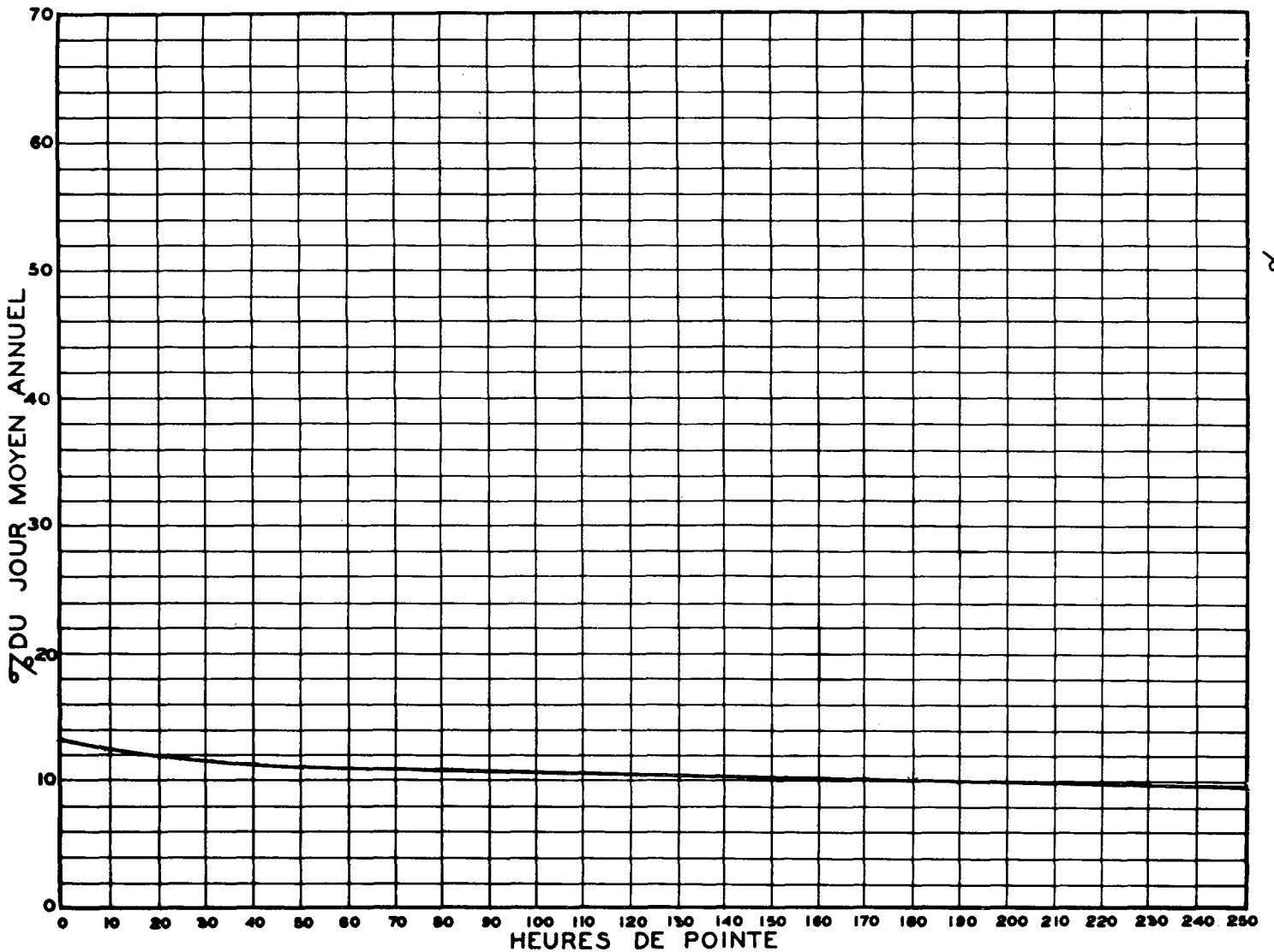
RELATION ENTRE LES HEURES DE POINTE ET LE JOUR MOYEN ANNUEL — STATION: ST-NICOLAS (2 VOIES) ROUTE N° RS-1-99
