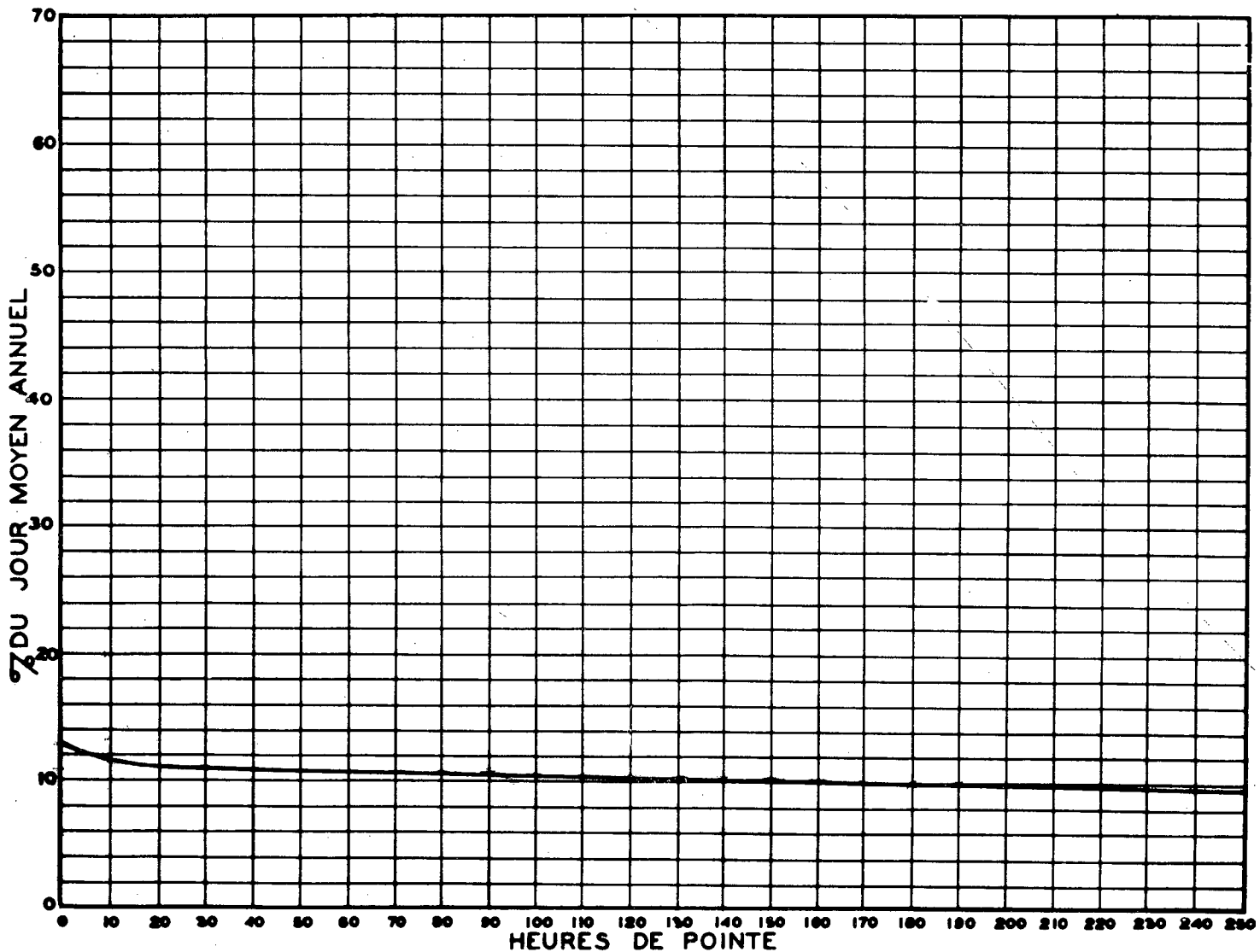
RELATION ENTRE LES HEURES DE POINTE ET LE JOUR MOYEN ANNUEL — STATION: SILLERY ROUTE N° RS-1-69
