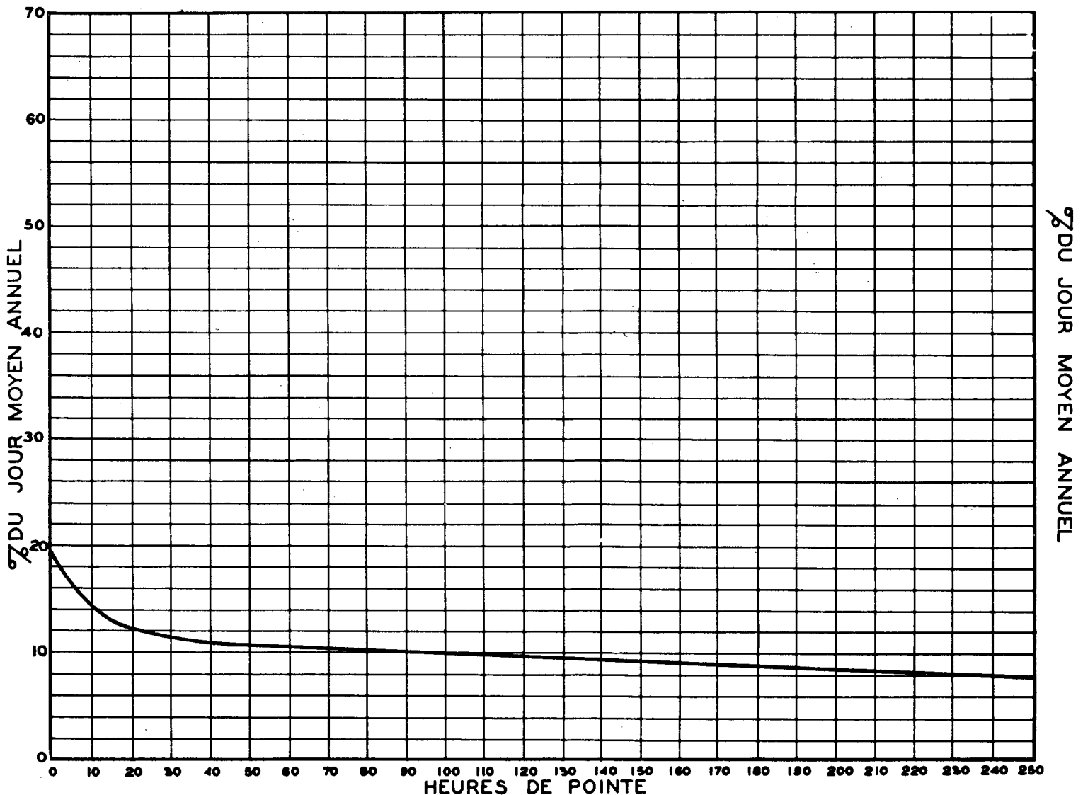
RELATION ENTRE LES HEURES DE POINTE ET LE JOUR MOYEN ANNUEL STATION: ST-REDEMPTEUR ROUTE N° 5-1-5
