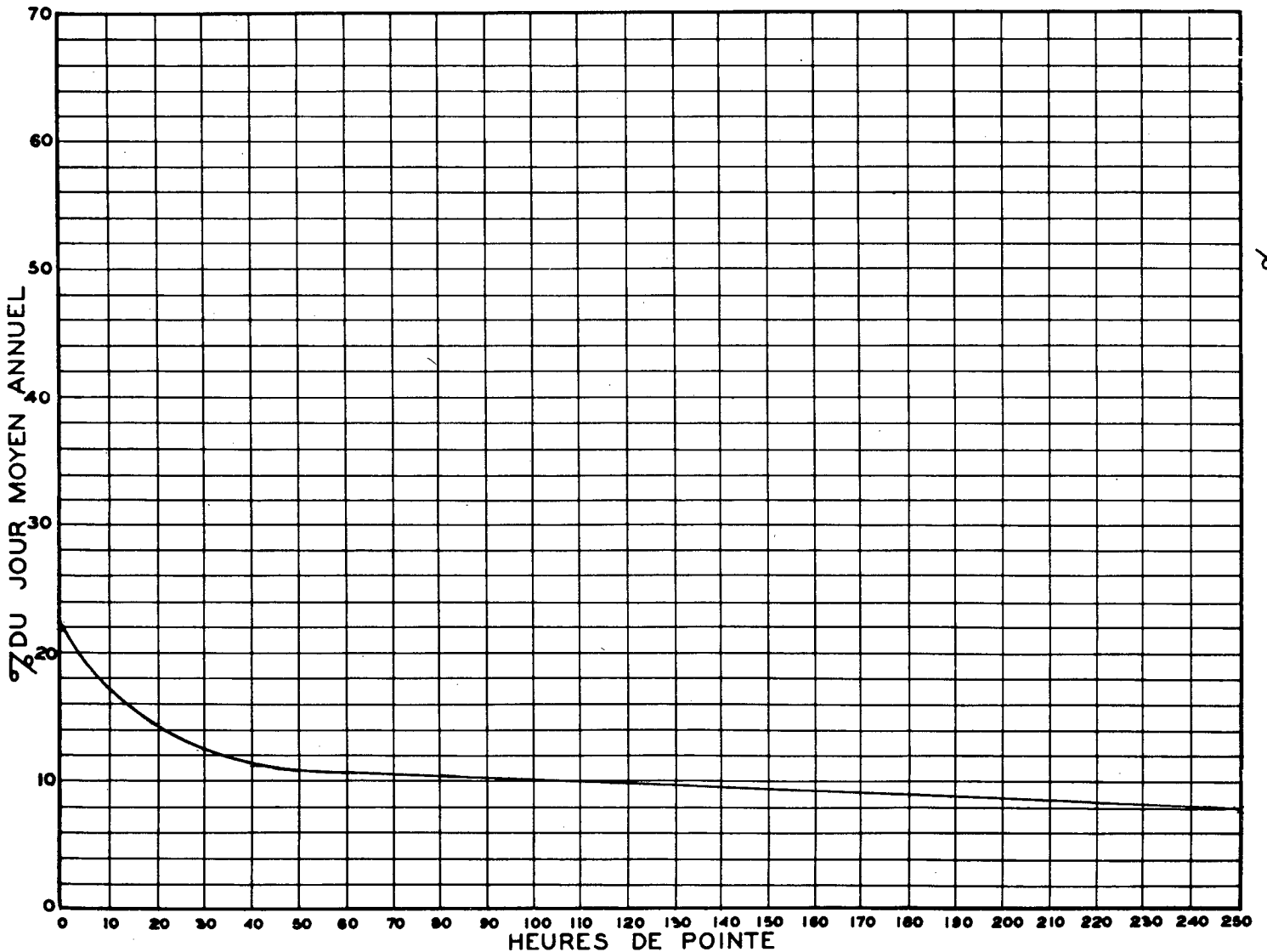
RELATION ENTRE LES HEURES DE POINTE ET LE JOUR MOYEN ANNUEL — STATION: CHARLESBOURG (VOIE EST) ROUTE N° 54-1-1
