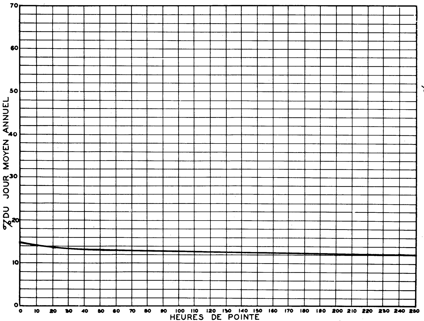
RELATION ENTRE LES HEURES DE POINTE ET LE JOUR MOYEN ANNUEL — STATION: LONGUEUIL (VOIE SUD) ROUTE N° 9-9-80
