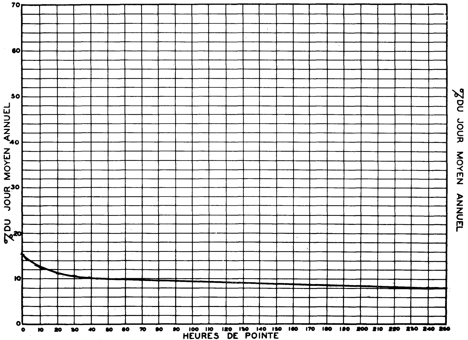
RELATION ENTRE LES HEURES DE POINTE ET LE JOUR MOYEN ANNUEL STATION: ST-JEAN-CHRYSOSTOME ROUTE N° RS-1-74
