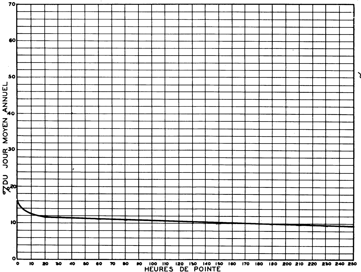
RELATION ENTRE LES HEURES DE POINTE ET LE JOUR MOYEN ANNUEL STATION: NOTRE-DAME-DE-LA-PROVIDENCE ROUTE N° 23-3-16
