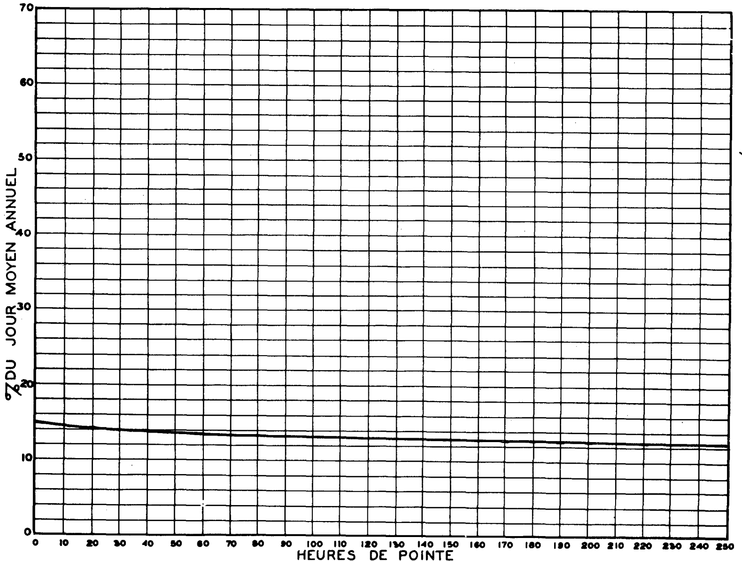
RELATION ENTRE LES HEURES DE POINTE ET LE JOUR MOYEN ANNUEL STATION: LONGUEUIL (VOIE NORD) ROUTE N° 9-9-80
