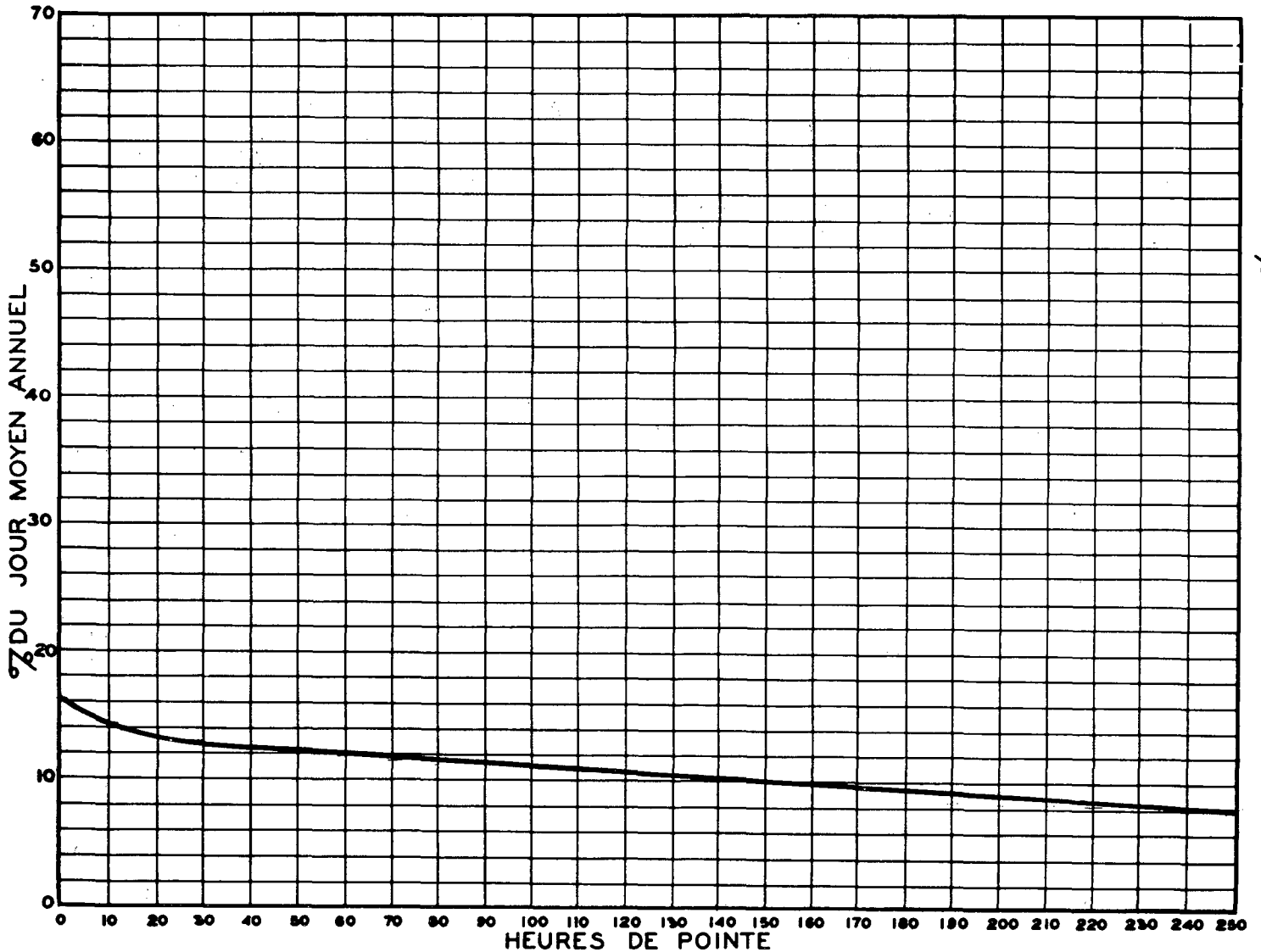
RELATION ENTRE LES HEURES DE POINTE ET LE JOUR MOYEN ANNUEL STATION: COURVILLE ROUTE N° 15-1-4
