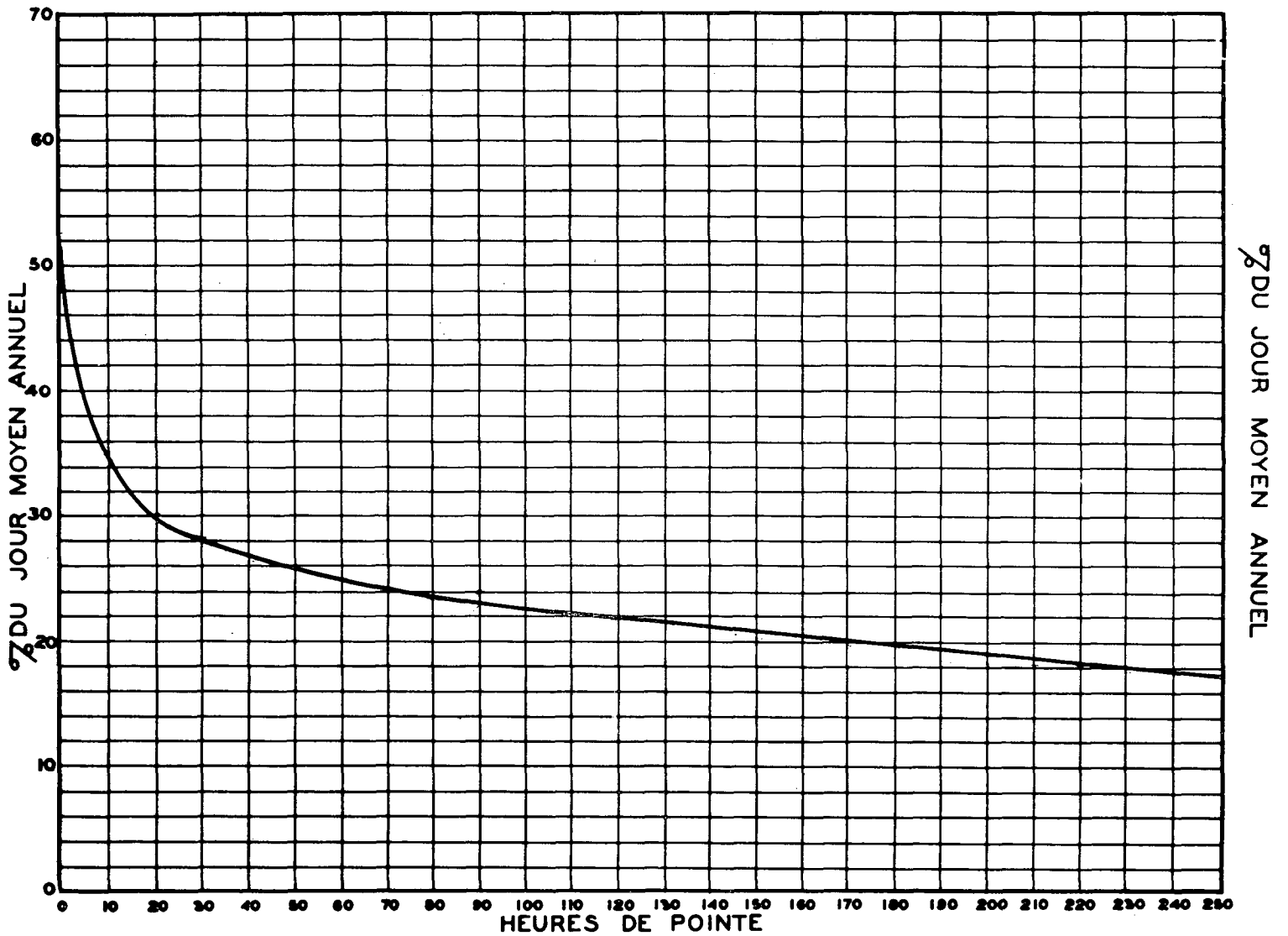
RELATION ENTRE LES HEURES DE POINTE ET LE JOUR MOYEN ANNUEL — STATION: VILLEROY ROUTE N° RS-3-3
