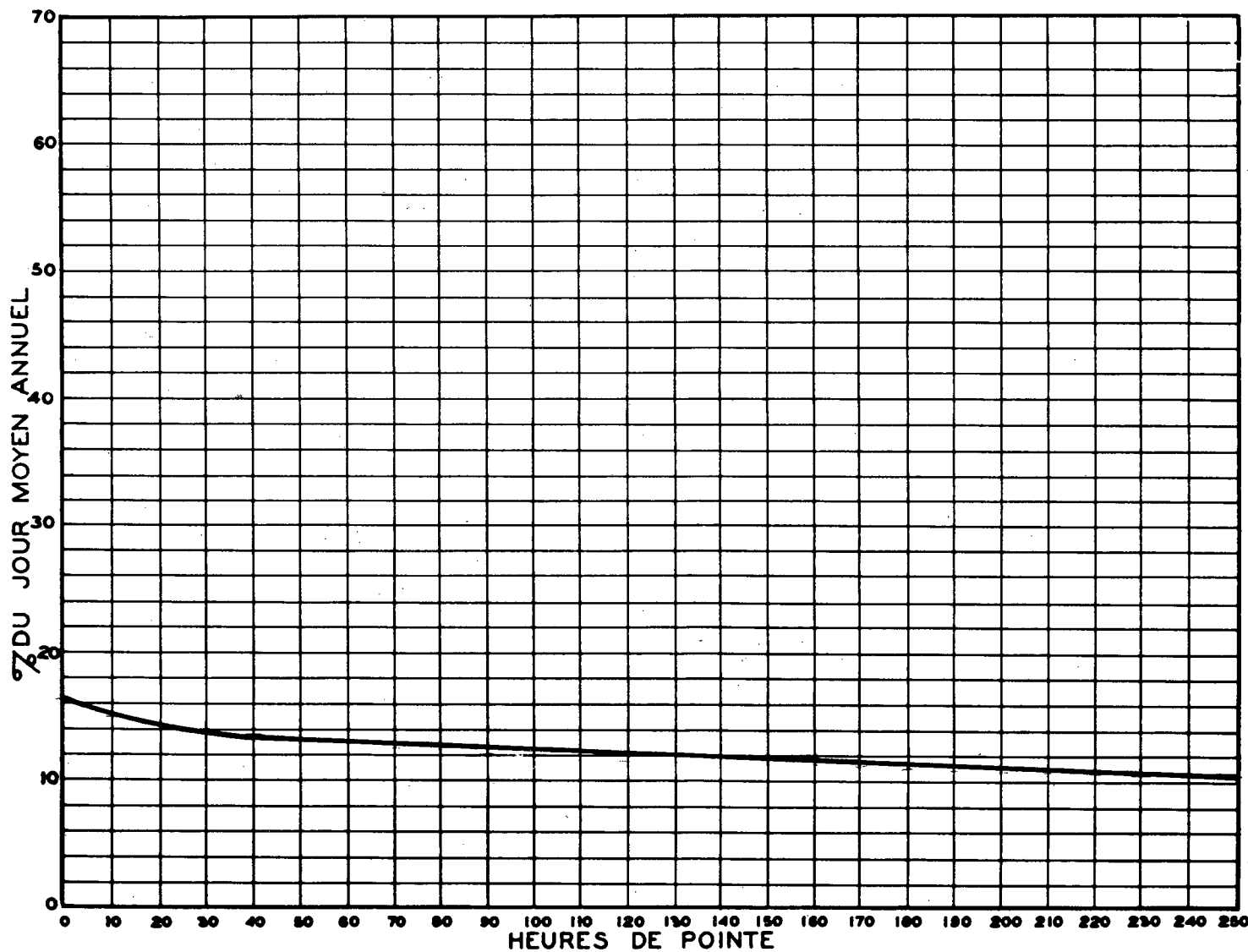
RELATION ENTRE LES HEURES DE POINTE ET LE JOUR MOYEN ANNUEL STATION: ST-ISIDORE ROUTE N° 23-1-16
