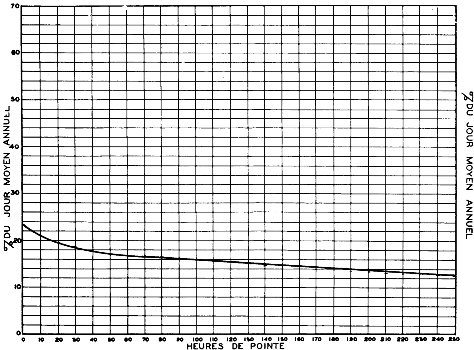
RELATION ENTRE LES HEURES DE POINTE ET LE JOUR MOYEN ANNUEL STATION: ST-BLAISE ROUTE N° 9-9-88
