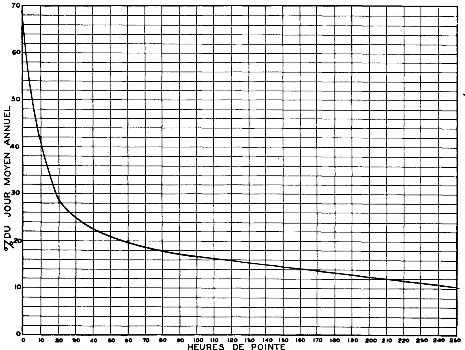
RELATION ENTRE LES HEURES DE POINTE ET LE JOUR MOYEN ANNUEL STATION: CHARLESBOURG (VOIE OUEST) ROUTE N° 54-1-1
