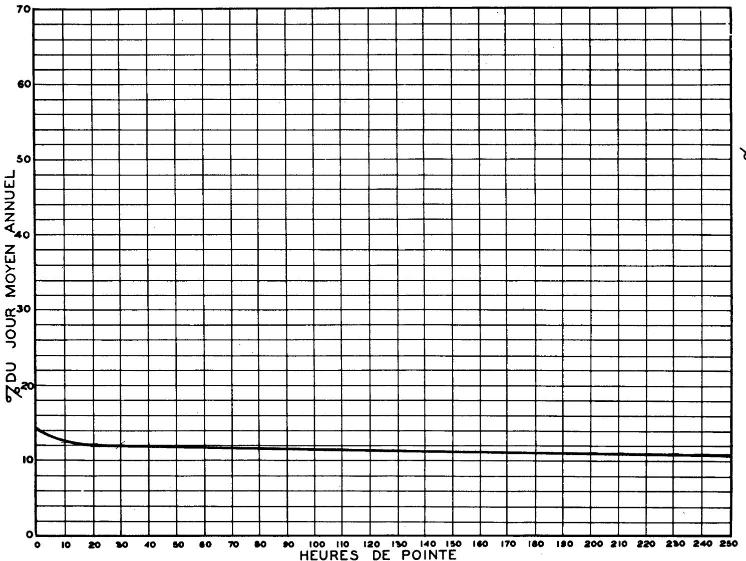
RELATION ENTRE LES HEURES DE POINTE ET LE JOUR MOYEN ANNUEL STATION: LAVAL (VOIE EST) ROUTE N° 11-4-81
