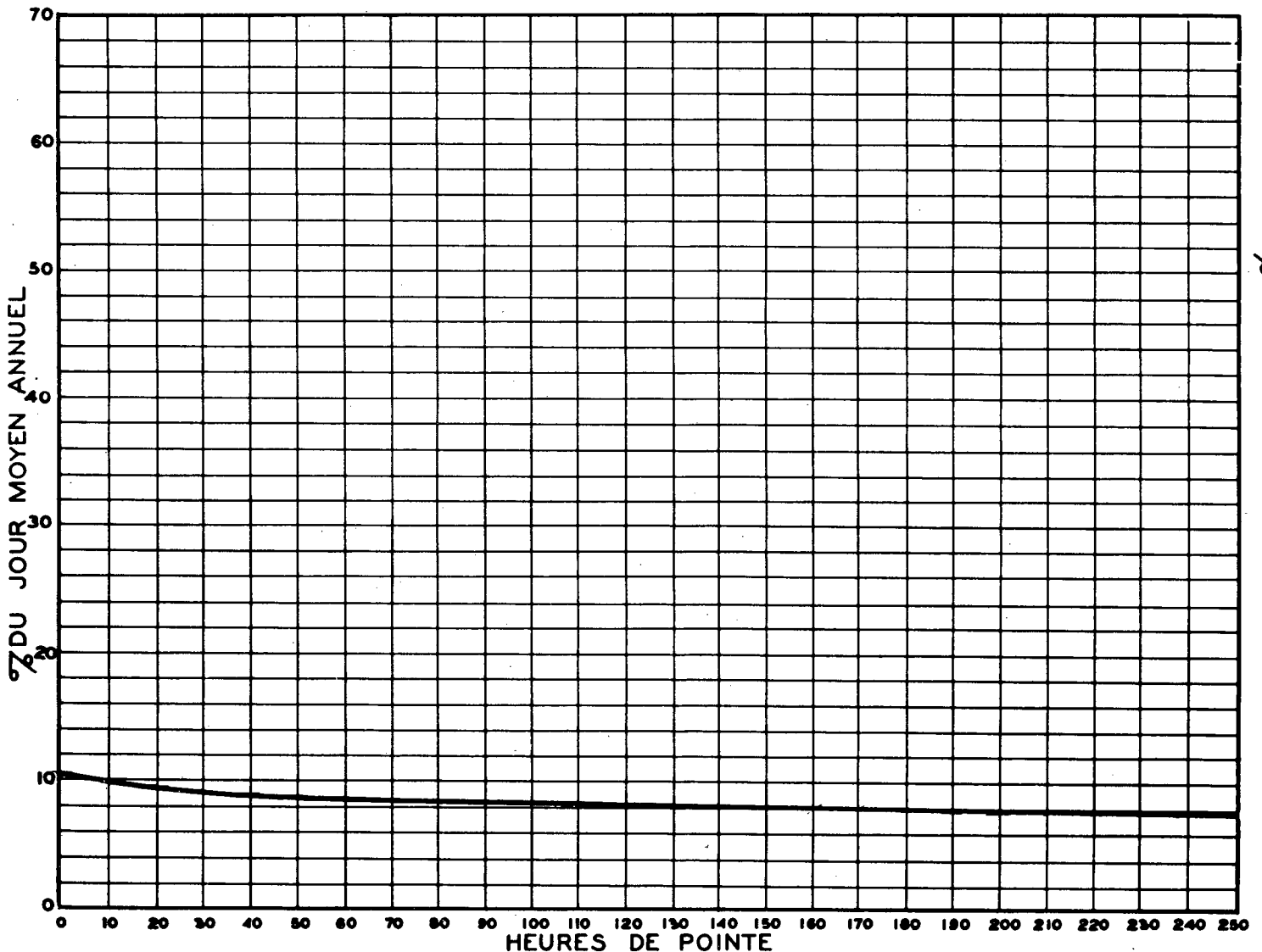
RELATION ENTRE LES HEURES DE POINTE ET LE JOUR MOYEN ANNUEL STATION: LEVIS ROUTE N° 23-1-17
