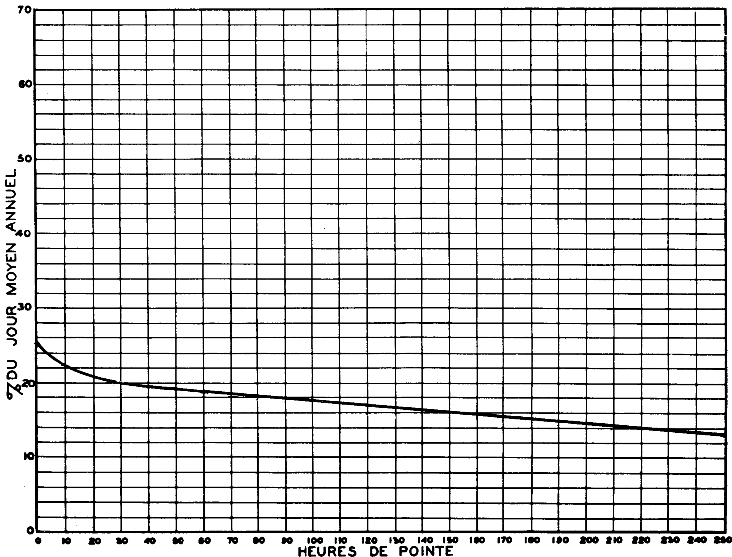
RELATION ENTRE LES HEURES DE POINTE ET LE JOUR MOYEN ANNUEL STATION: ST-JOACHIM ROUTE N° 15-1-13
