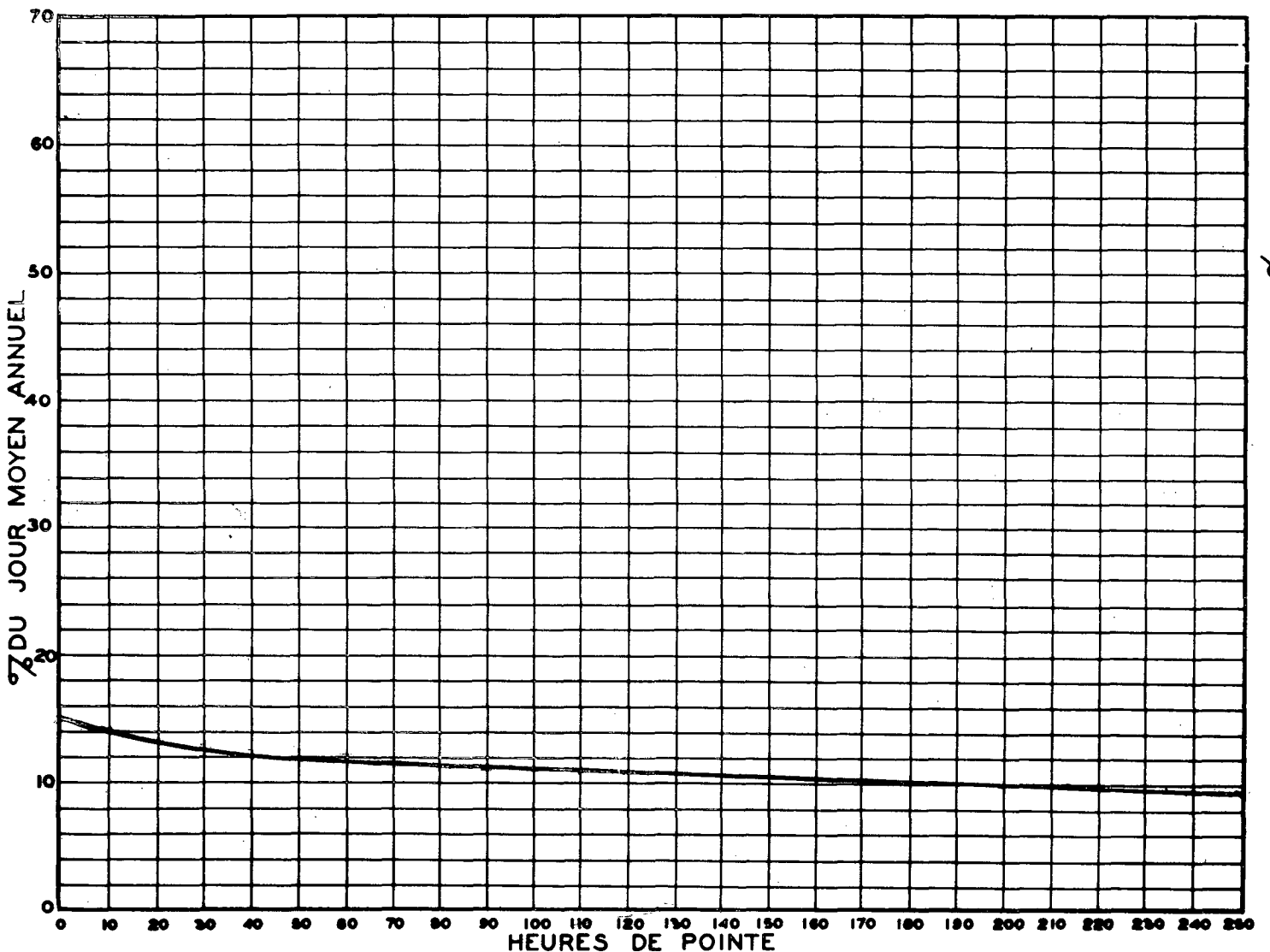
RELATION ENTRE LES HEURES DE POINTE ET LE JOUR MOYEN ANNUEL — STATION: ST-NICOLAS (VOIE EST) ROUTE N° RS-1-99
