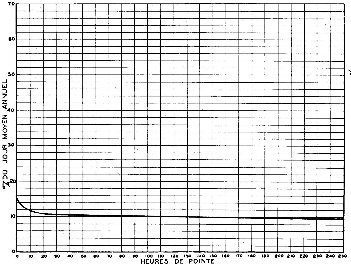
RELATION ENTRE LES HEURES DE POINTE ET LE JOUR MOYEN ANNUEL STATION: TERREBONNE ROUTE N° 18-4-70
