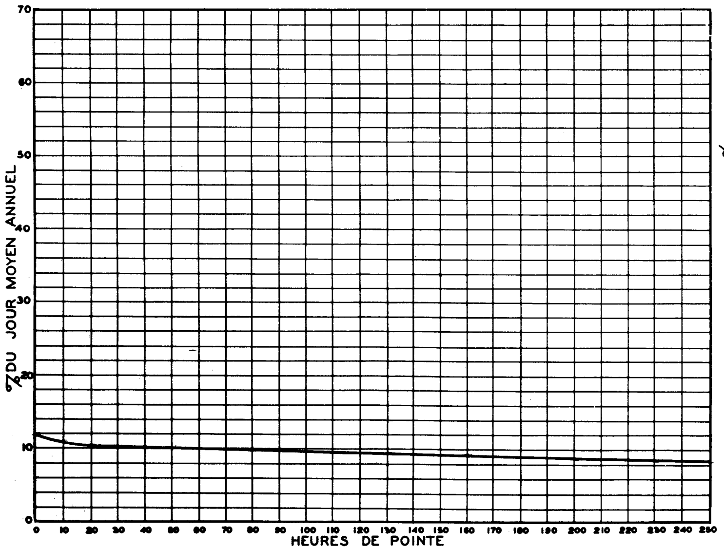
RELATION ENTRE LES HEURES DE POINTE ET LE JOUR MOYEN ANNUEL — STATION: ST-ROMUALD (VOIE NORD) ROUTE N° 2-1-4
