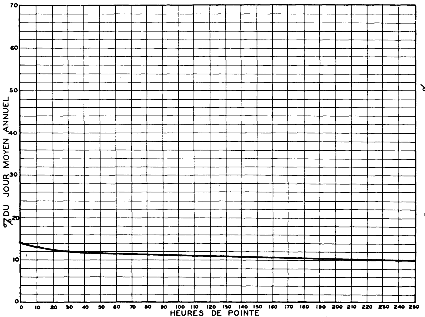
RELATION ENTRE LES HEURES DE POINTE ET LE JOUR MOYEN ANNUEL STATION: ST-ROMUALD ROUTE N° 20-1-1
