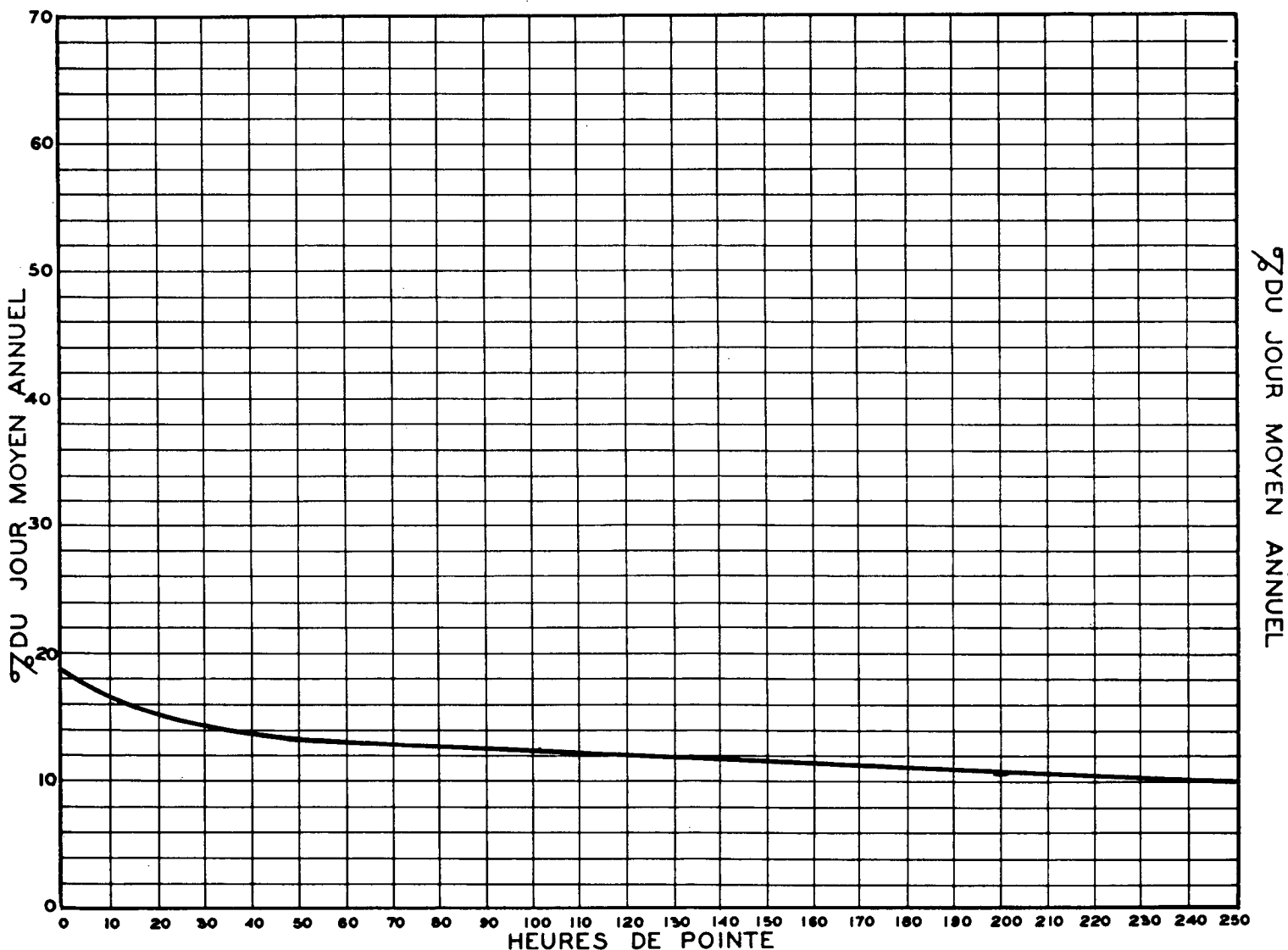
RELATION ENTRE LES HEURES DE POINTE ET LE JOUR MOYEN ANNUEL STATION: MERCIER ROUTE N° 4-9-61
