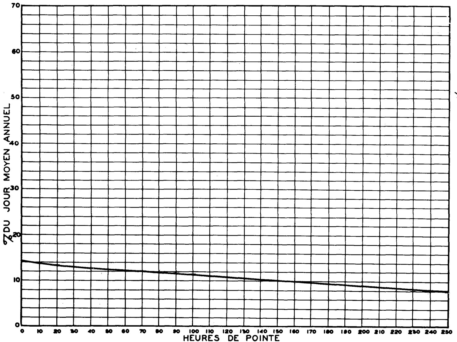
RELATION ENTRE LES HEURES DE POINTE ET LE JOUR MOYEN ANNUEL STATION: DORVAL (VOIE SUD) ROUTE N° 20-4-54
