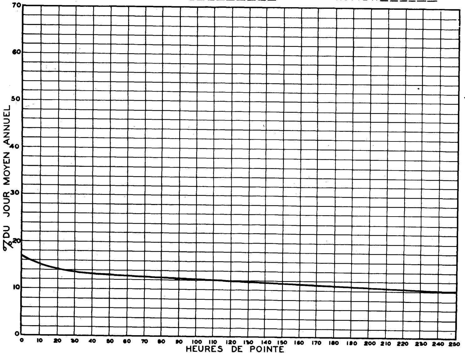
RELATION ENTRE LES HEURES DE POINTE ET LE JOUR MOYEN ANNUEL STATION: ST-PATRICE ROUTE N° 10-2-2
