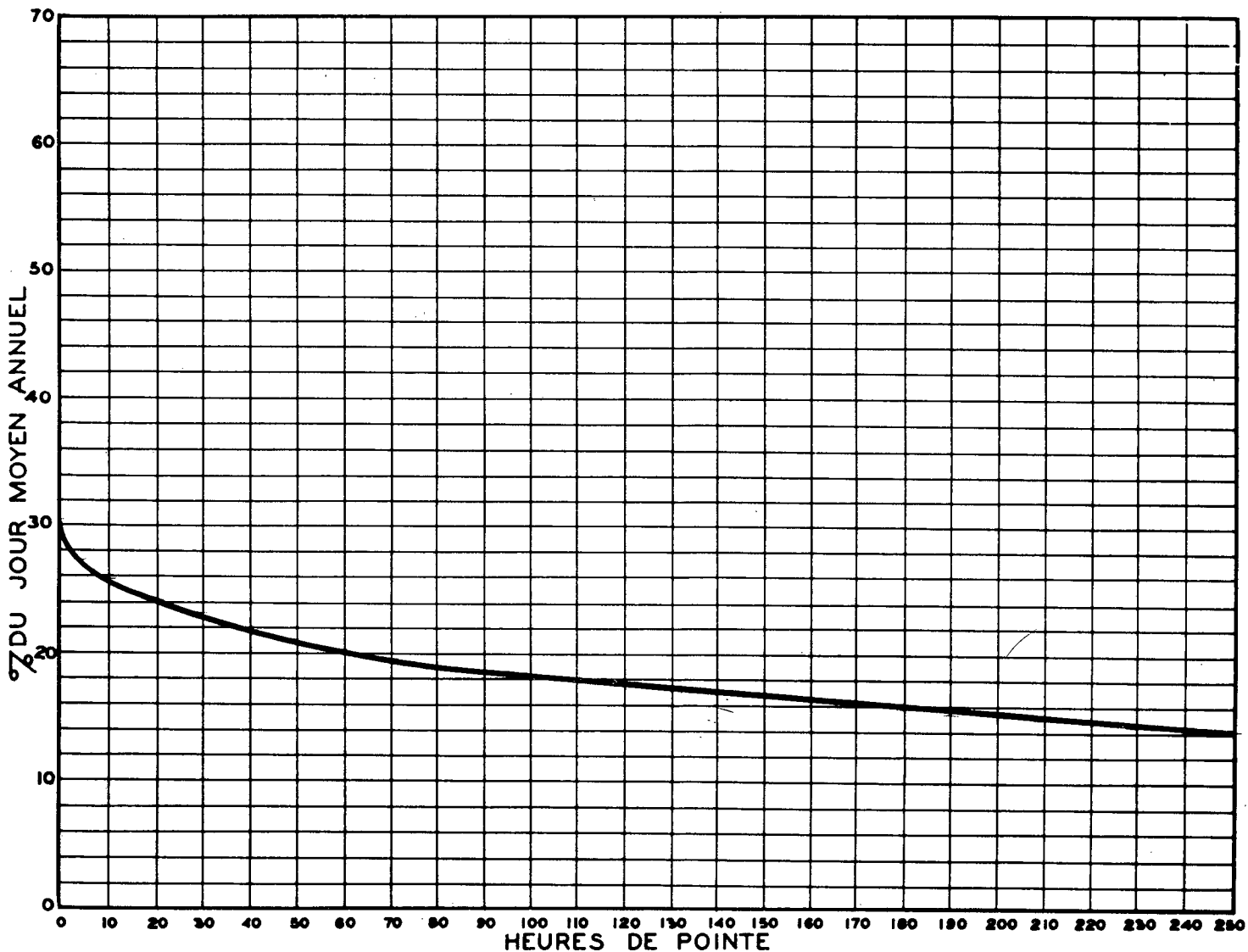
RELATION ENTRE LES HEURES DE POINTE ET LE JOUR MOYEN ANNUEL STATION: GRANDES-PILES ROUTE N° 19-10-14
