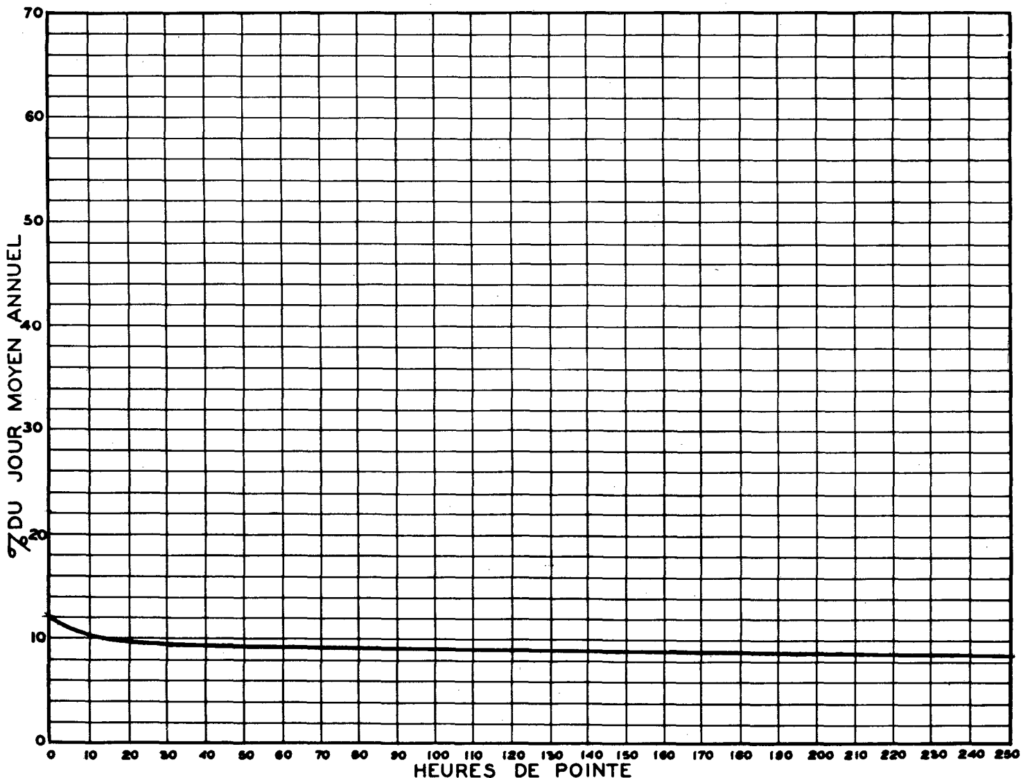
RELATION ENTRE LES HEURES DE POINTE ET LE JOUR MOYEN ANNUEL STATION: ST-LÉONARD ROUTE N° 40-4-86
