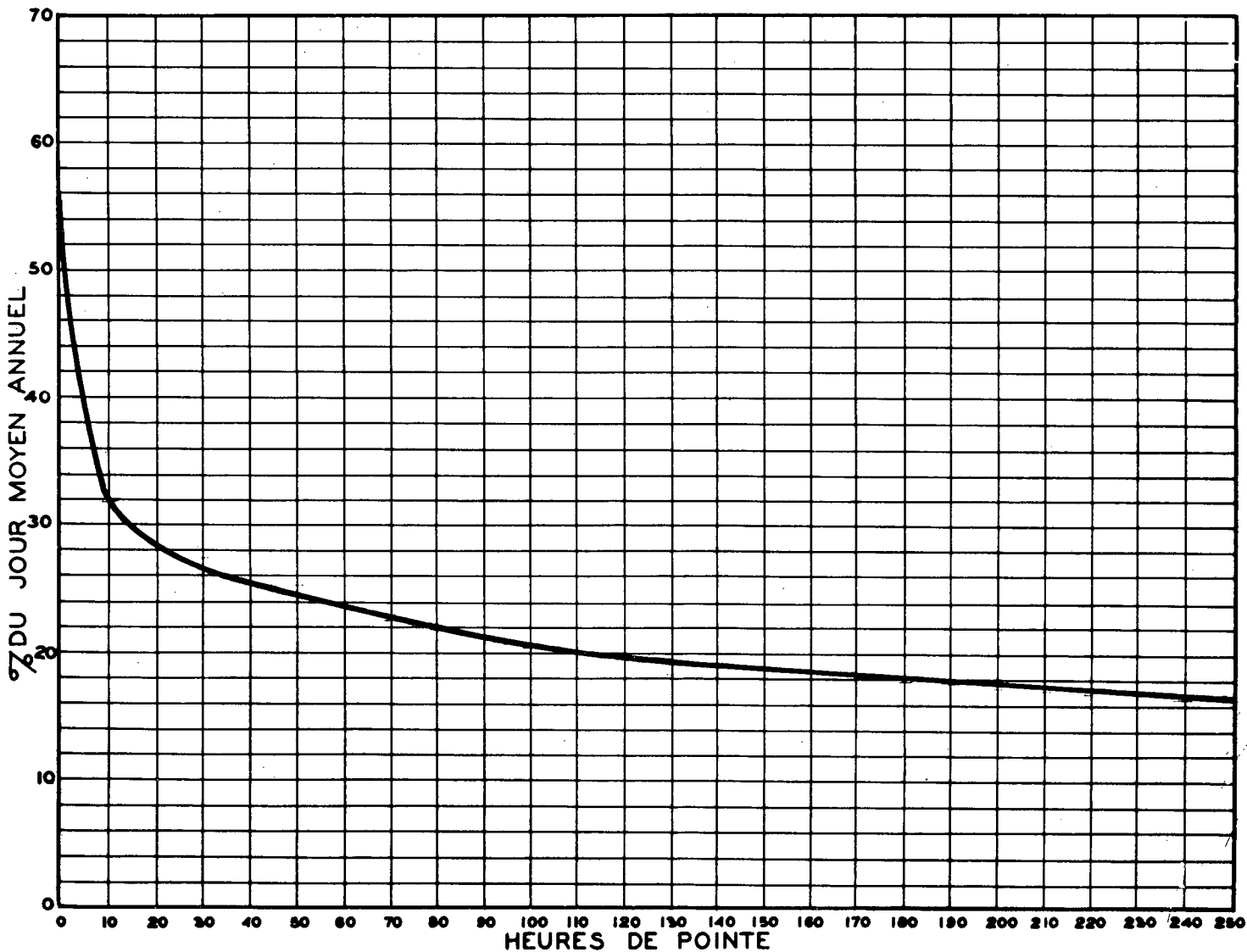
RELATION ENTRE LES HEURES DE POINTE ET LE JOUR MOYEN ANNUEL STATION: ST-JEAN-BOSCO ROUTE N° 19-10-4
