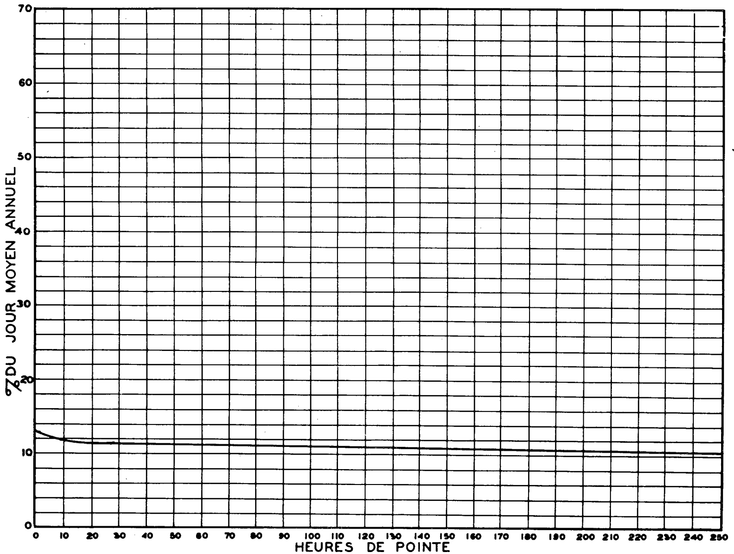
RELATION ENTRE LES HEURES DE POINTE ET LE JOUR MOYEN ANNUEL — STATION: MONTREAL - PONT PAPINEAU (2 VOIES) ROUTE N° R-S 4-4
