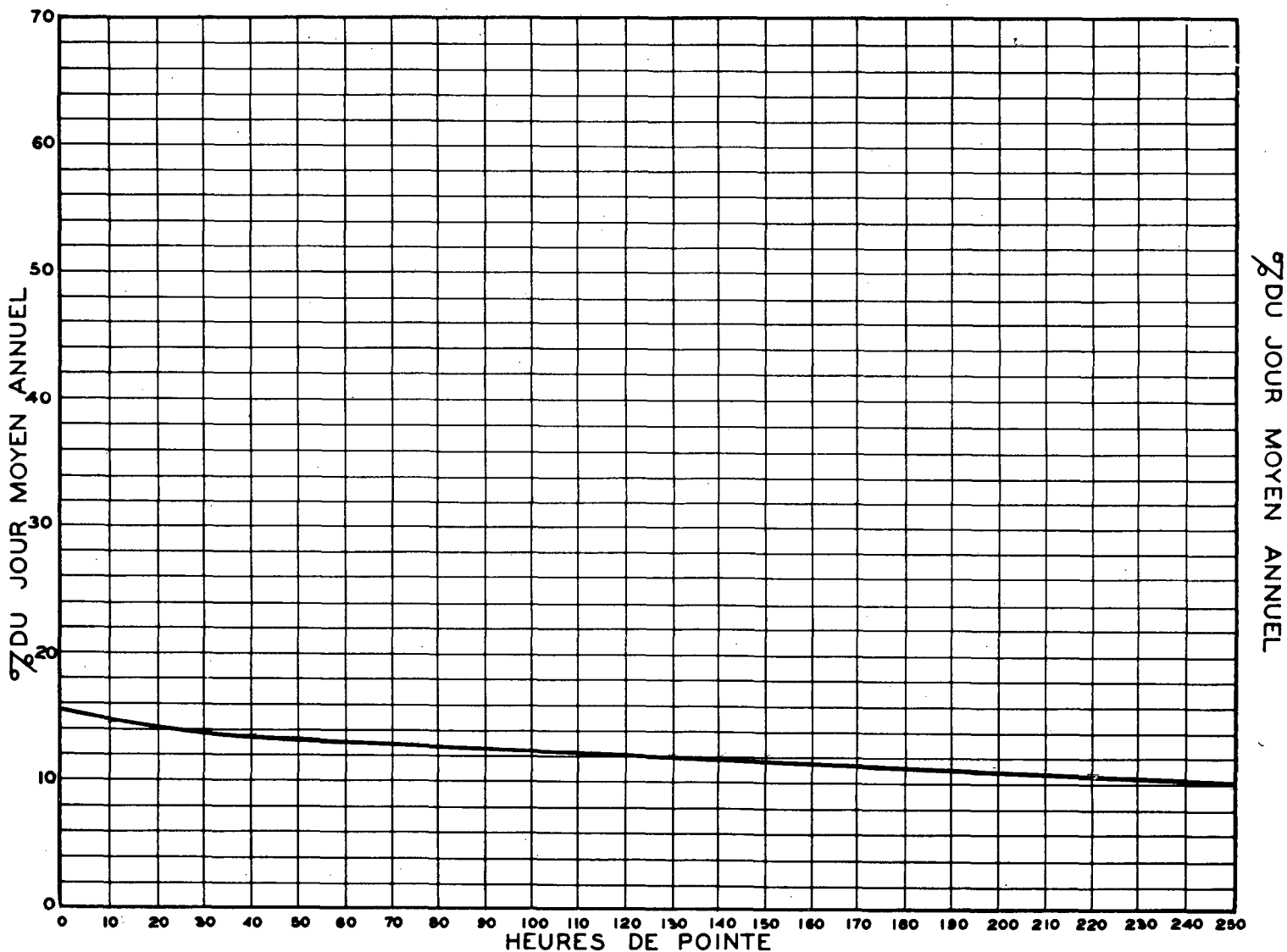
RELATION ENTRE LES HEURES DE POINTE ET LE JOUR MOYEN ANNUEL STATION: POINTE-AUX-TREMBLES (VOIE EST) ROUTE N° 2-4-85
