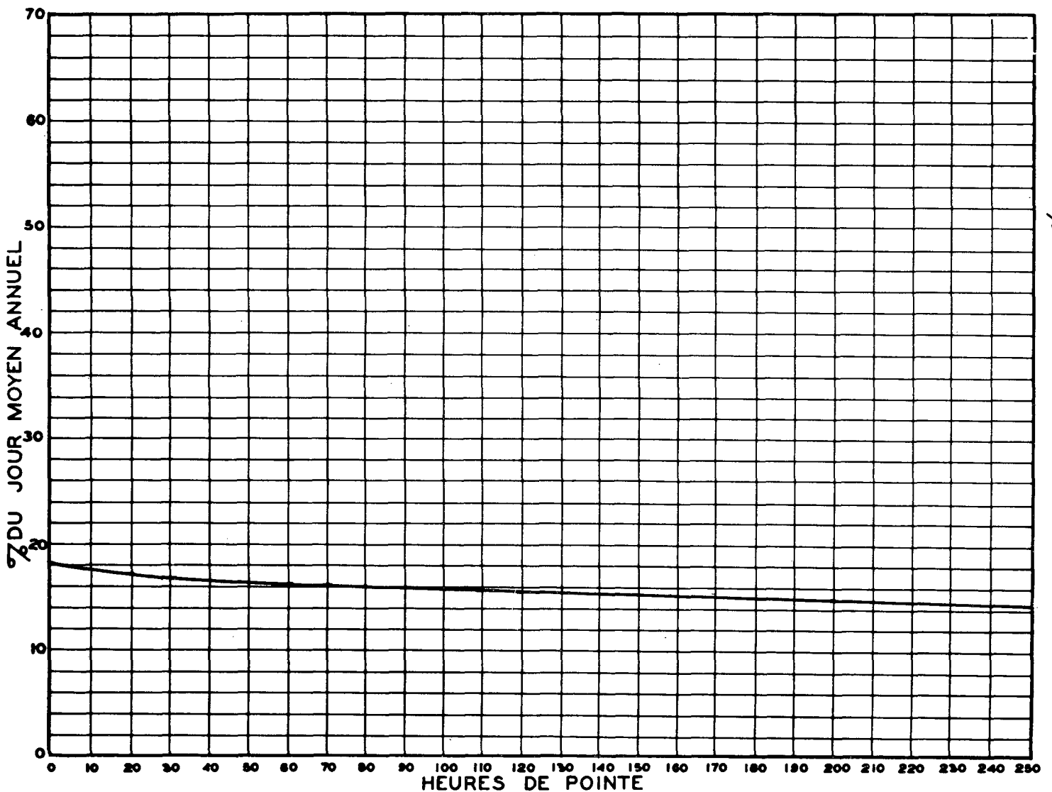
RELATION ENTRE LES HEURES DE POINTE ET LE JOUR MOYEN ANNUEL — STATION: MONTREAL - PONT PAPINEAU (VOIE OUEST) ROUTE N° RS-4-4
