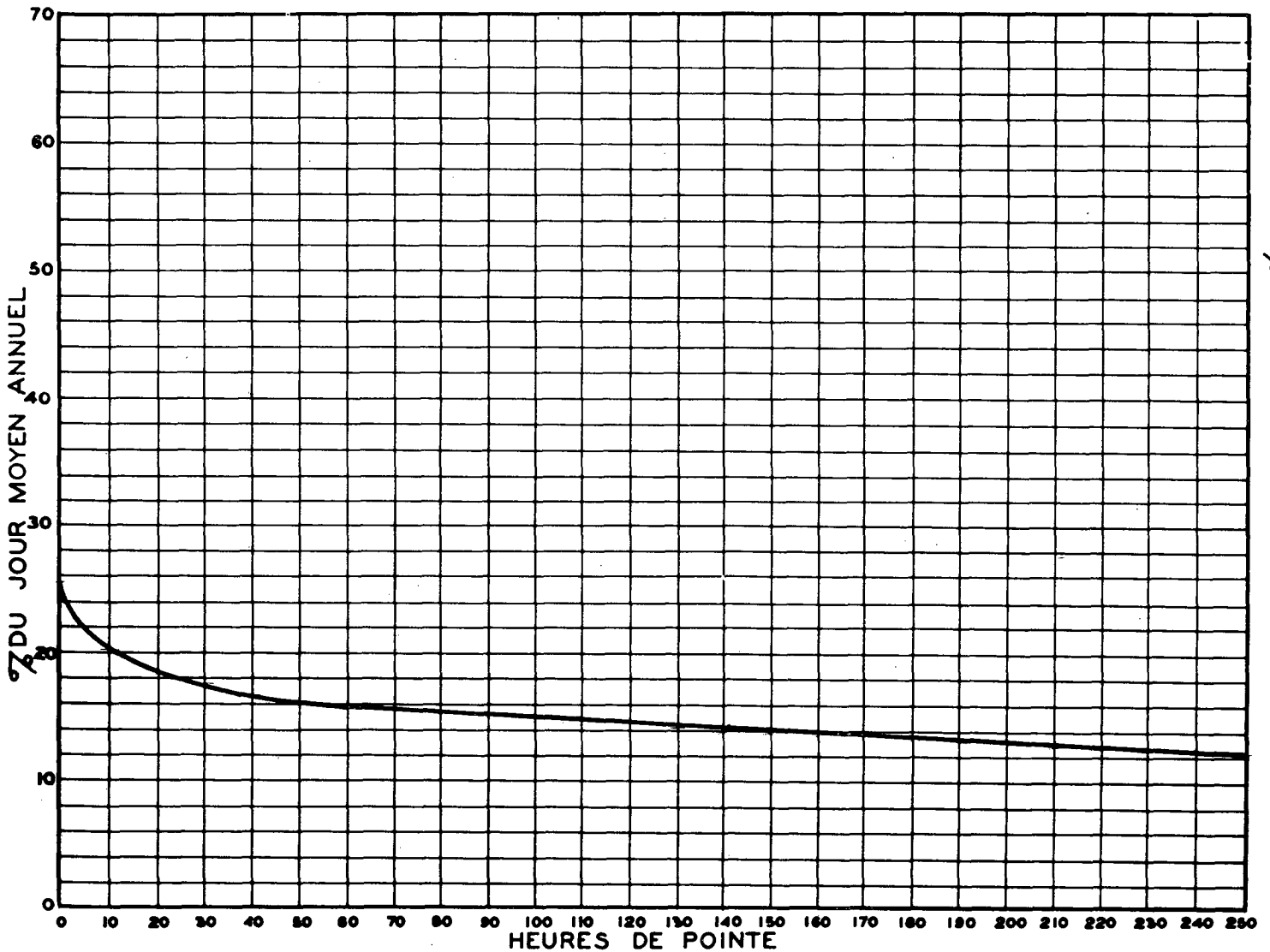
RELATION ENTRE LES HEURES DE POINTE ET LE JOUR MOYEN ANNUEL STATION: ST-LEONARD ROUTE N° 20-8-1
