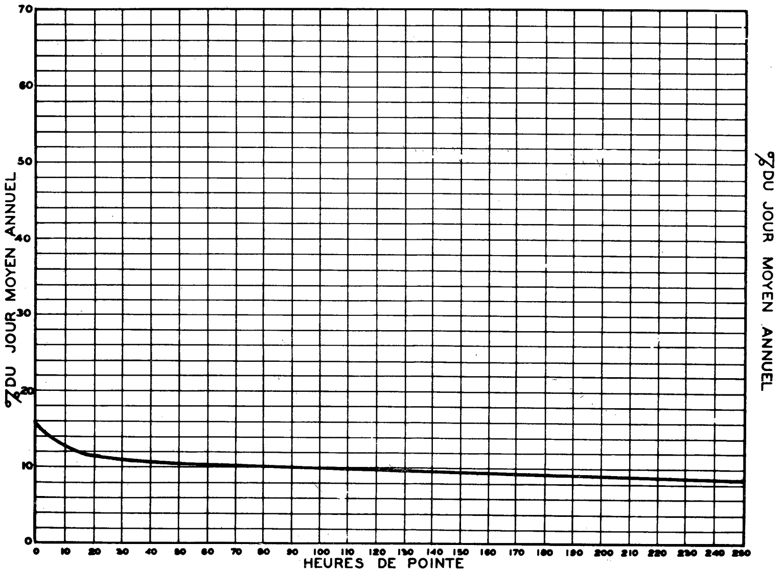
RELATION ENTRE LES HEURES DE POINTE ET LE JOUR MOYEN ANNUEL STATION: Ancienne-Lorette ROUTE N° RS-1-1
