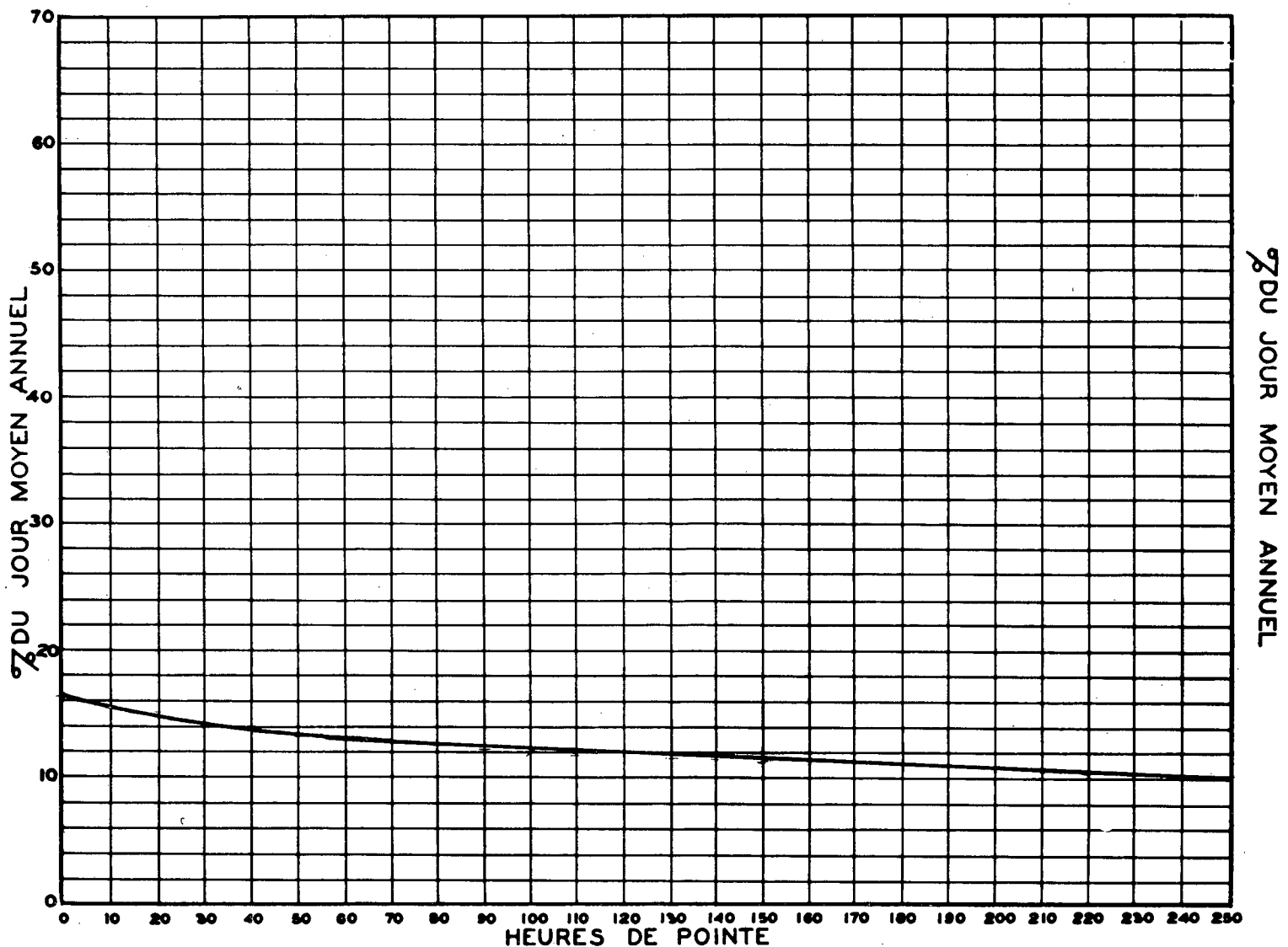
RELATION ENTRE LES HEURES DE POINTE ET LE JOUR MOYEN ANNUEL — STATION: ST-GREGOIRE ROUTE N° RS-8-15
