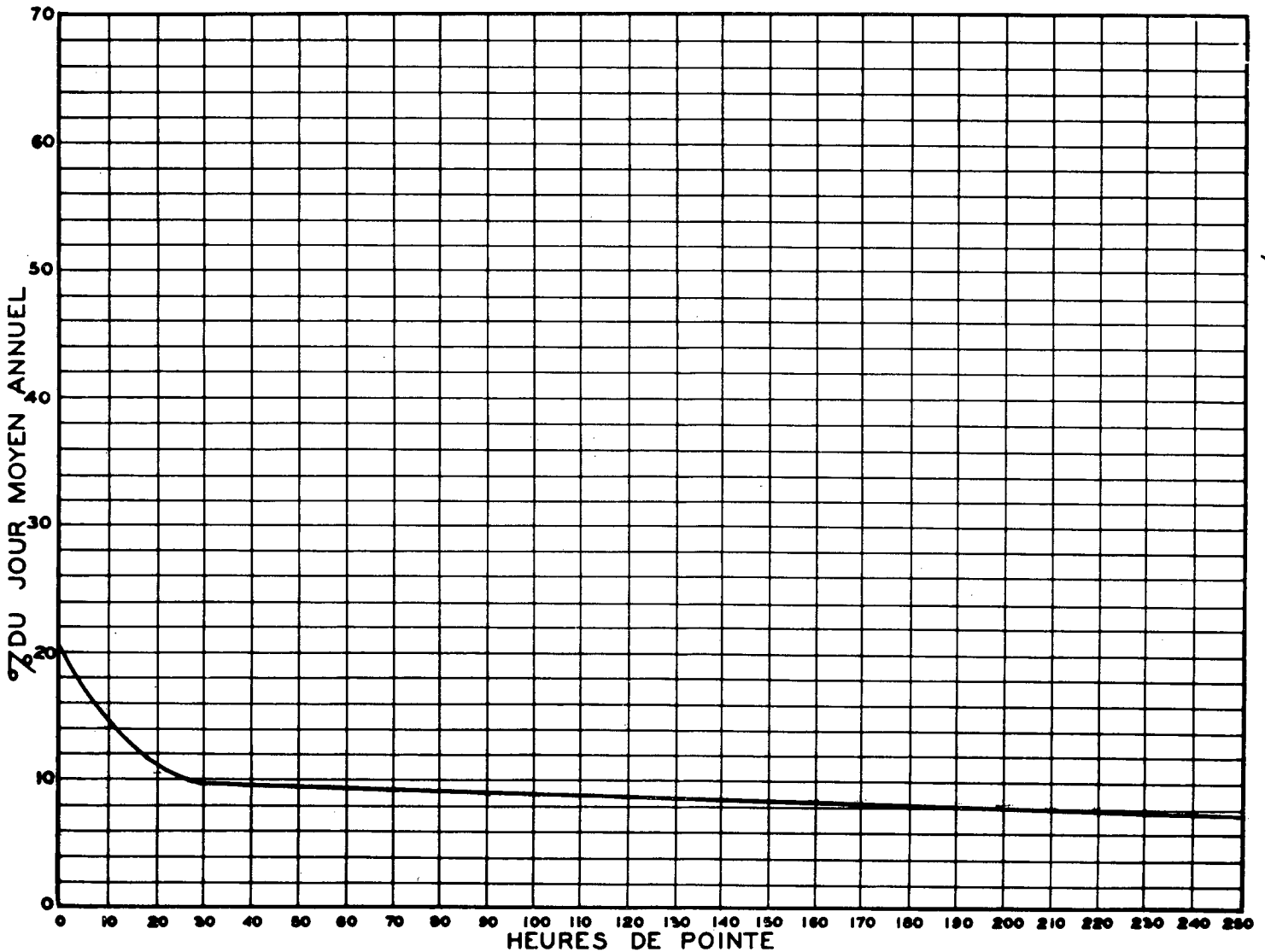
RELATION ENTRE LES HEURES DE POINTE ET LE JOUR MOYEN ANNUEL STATION: CHARNY ROUTE N° RS-1-73
