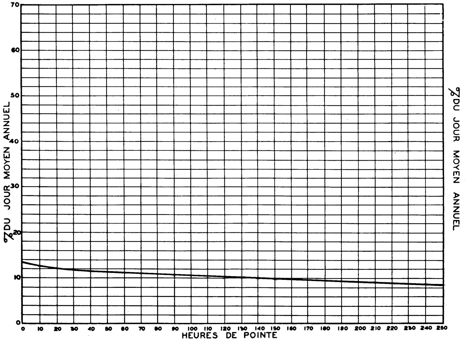
RELATION ENTRE LES HEURES DE POINTE ET LE JOUR MOYEN ANNUEL STATION: ANCIENNE-LORETTE (2 VOIES) ROUTE N° 2-1-7
