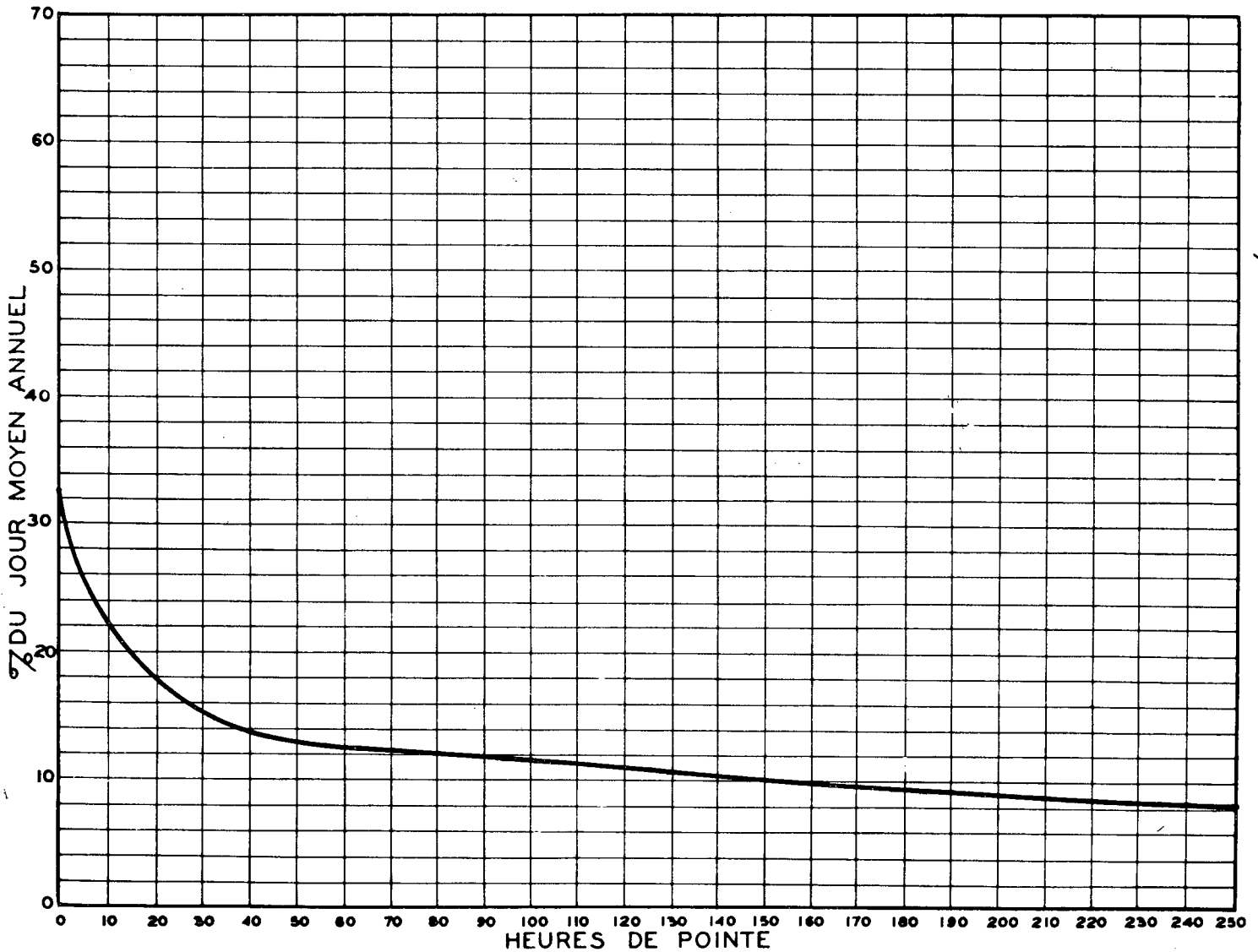
RELATION ENTRE LES HEURES DE POINTE ET LE JOUR MOYEN ANNUEL STATION: CHARLESBOURG (2 VOIES) ROUTE N° 54-1-1
