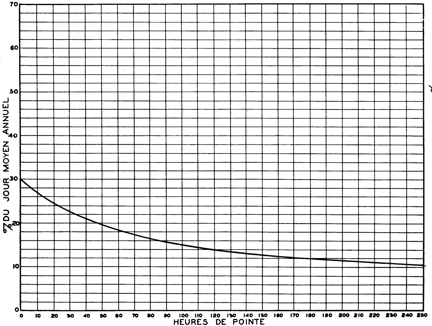
RELATION ENTRE LES HEURES DE POINTE ET LE JOUR MOYEN ANNUEL STATION: ST-MARC ROUTE N° 47-9-51
