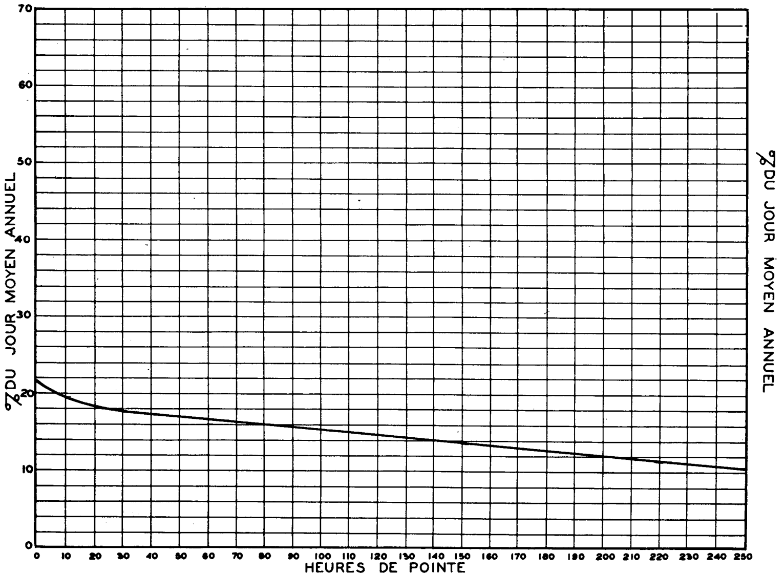
RELATION ENTRE LES HEURES DE POINTE ET LE JOUR MOYEN ANNUEL STATION: ROUEMONT ROUTE N° 1-8-80
