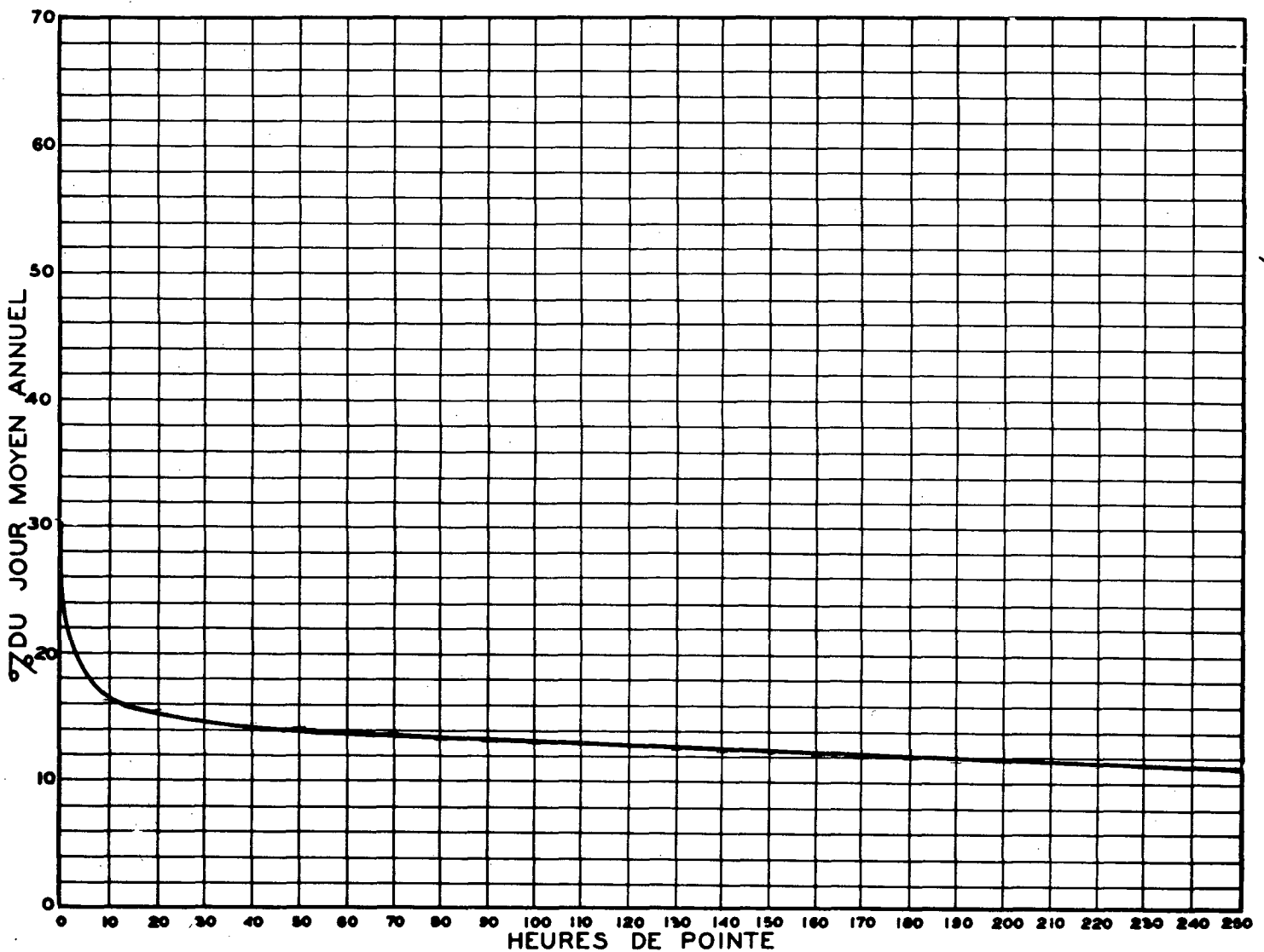
RELATION ENTRE LES HEURES DE POINTE ET LE JOUR MOYEN ANNUEL STATION: TERREBONNE ROUTE N° 25-4-51
