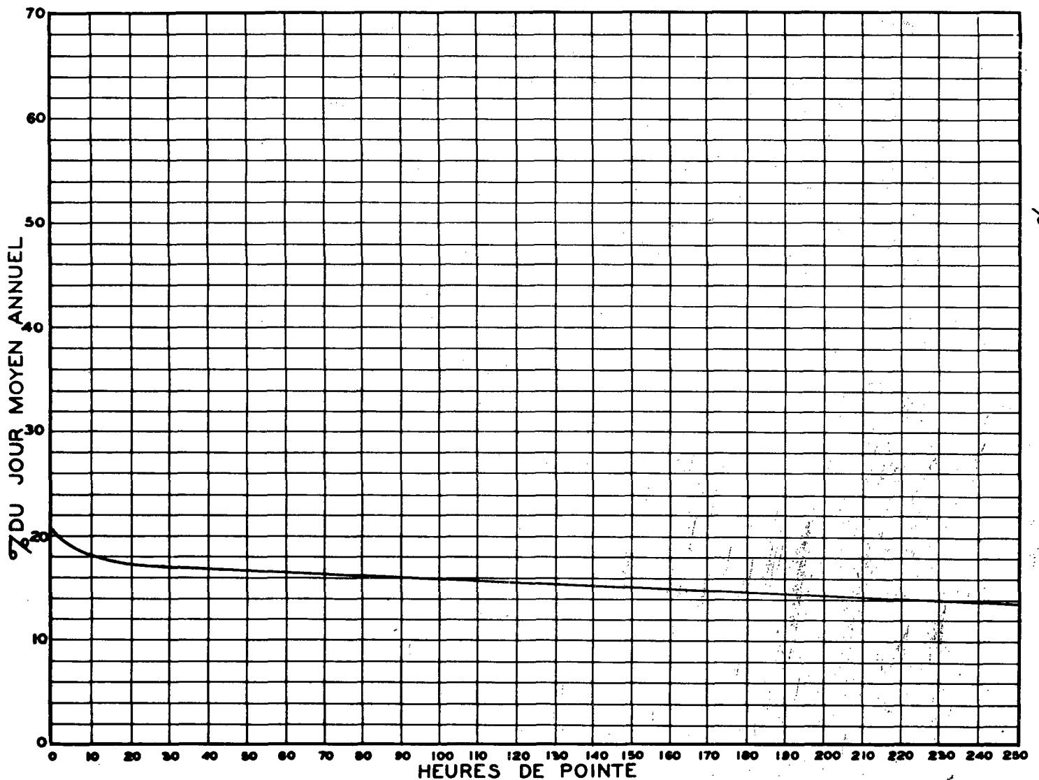
RELATION ENTRE LES HEURES DE POINTE ET LE JOUR MOYEN ANNUEL — STATION: MONTREAL - PONT PAPINEAU (VOIE EST) ROUTE N° R-S 4-4
