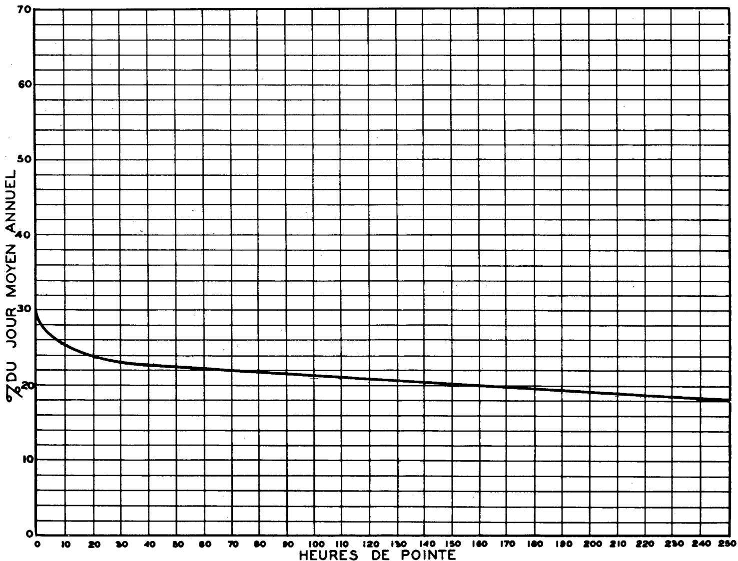
RELATION ENTRE LES HEURES DE POINTE ET LE JOUR MOYEN ANNUEL STATION: ARMSTRONG ROUTE N° 23-3-19
