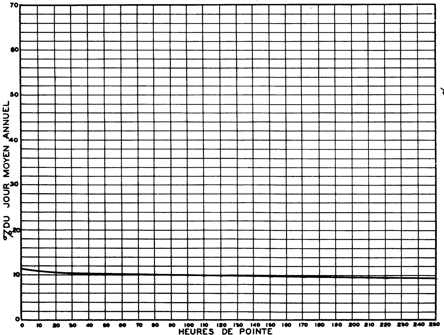
RELATION ENTRE LES HEURES DE POINTE ET LE JOUR MOYEN ANNUEL STATION: ST-ROMUALD (2 VOIES) ROUTE N° 2-1-4
