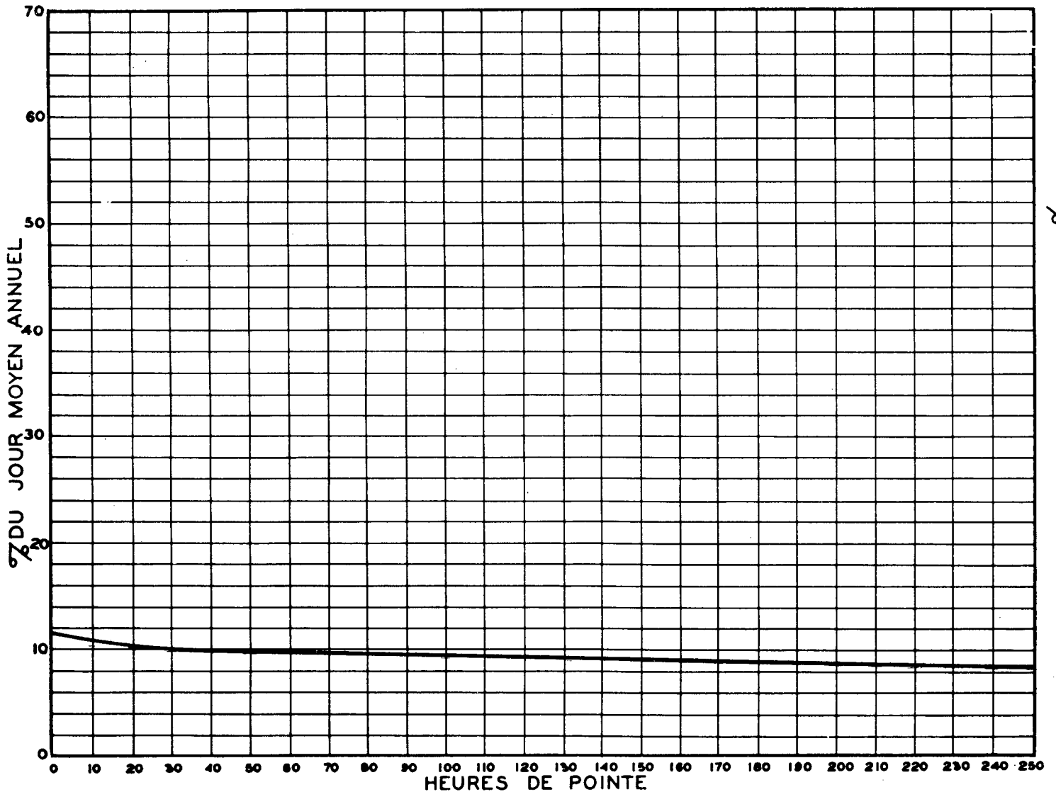
RELATION ENTRE LES HEURES DE POINTE ET LE JOUR MOYEN ANNUEL STATION: POINTE-AUX-TREMBLES (2 VOIES) ROUTE N° 2-4-85
