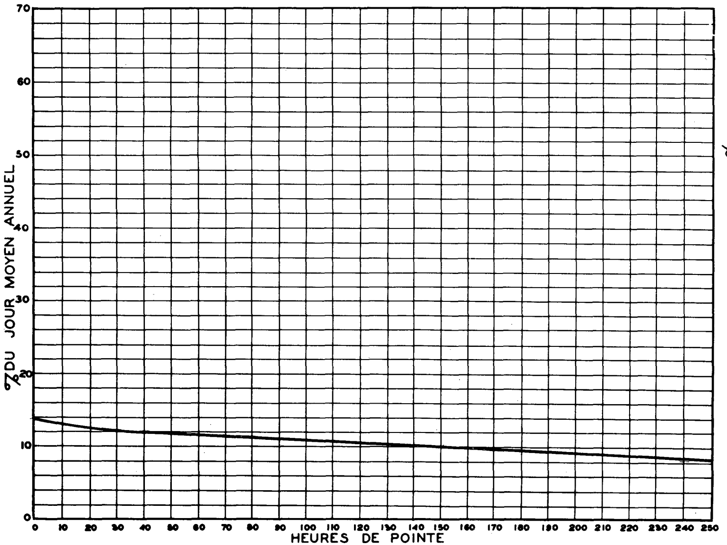
RELATION ENTRE LES HEURES DE POINTE ET LE JOUR MOYEN ANNUEL STATION: DORVAL (VOIE NORD) ROUTE N° 20-4-54
