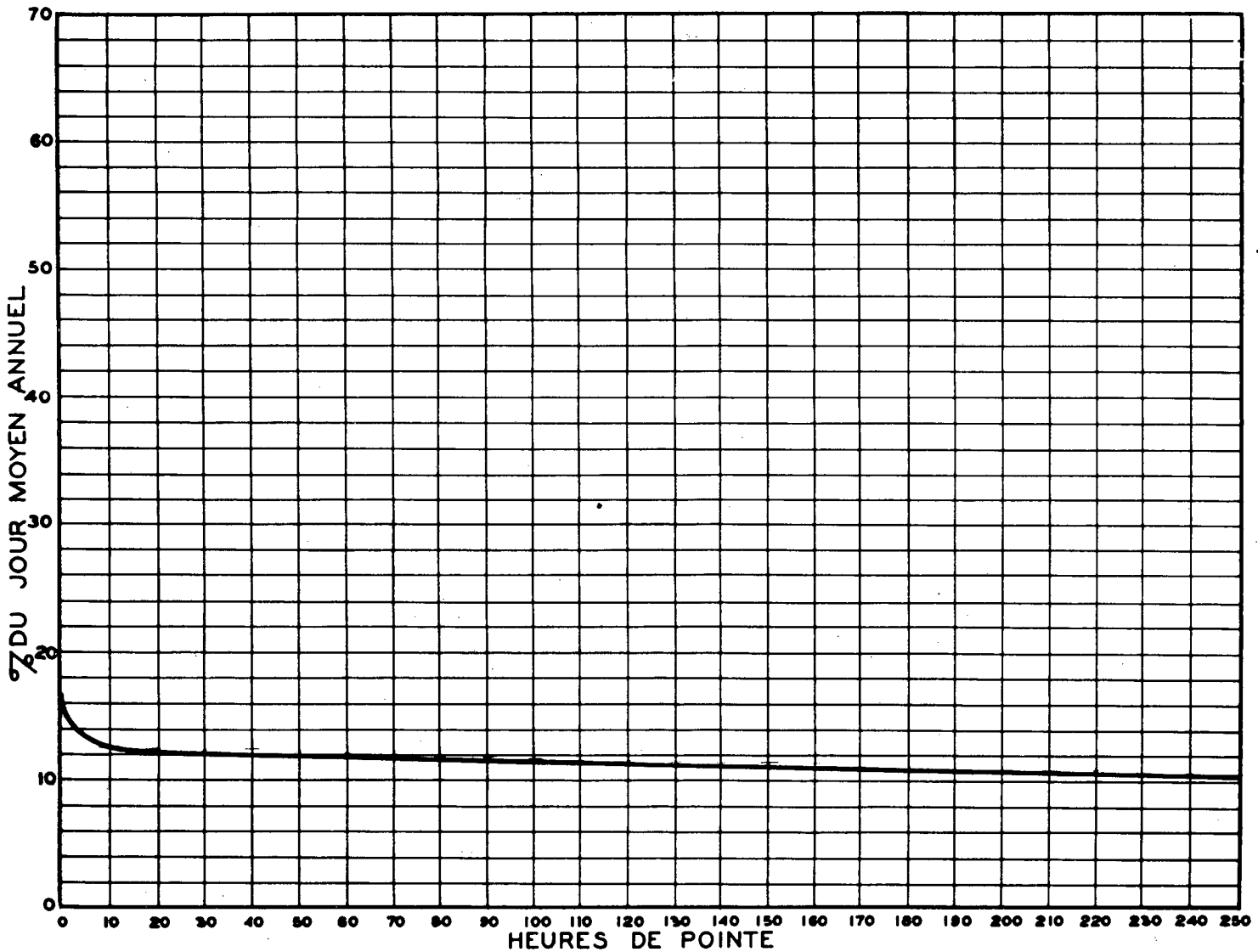
RELATION ENTRE LES HEURES DE POINTE ET LE JOUR MOYEN ANNUEL STATION: LAVAL (VOIE EST) ROUTE N° 11-4-80
