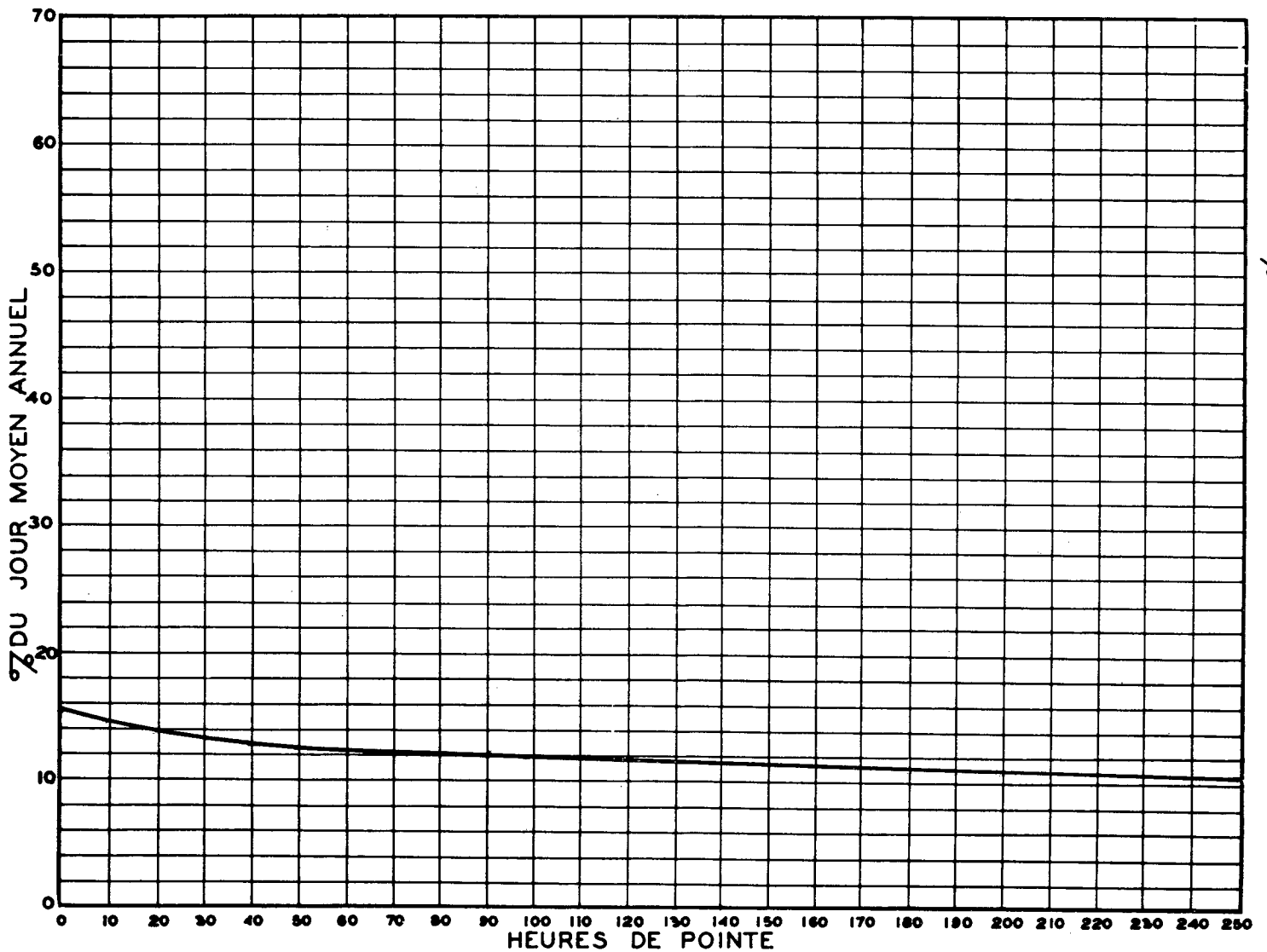
RELATION ENTRE LES HEURES DE POINTE ET LE JOUR MOYEN ANNUEL STATION: ST-NICOLAS (VOIE OUEST) ROUTE N° RS-1-99
