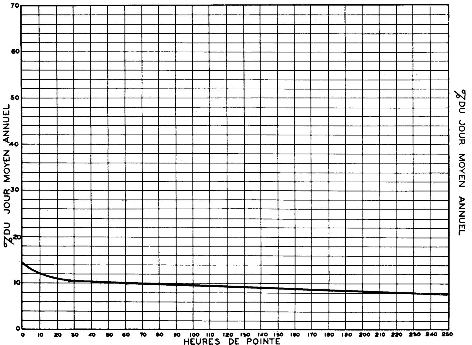
RELATION ENTRE LES HEURES DE POINTE ET LE JOUR MOYEN ANNUEL STATION: ST-NICOLAS ROUTE N° 3-1-2
