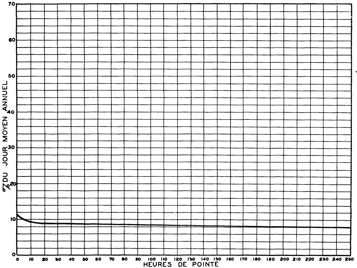
RELATION ENTRE LES HEURES DE POINTE ET LE JOUR MOYEN ANNUEL STATION: LAVAL (2 VOIES) ROUTE N° 11-4-80
