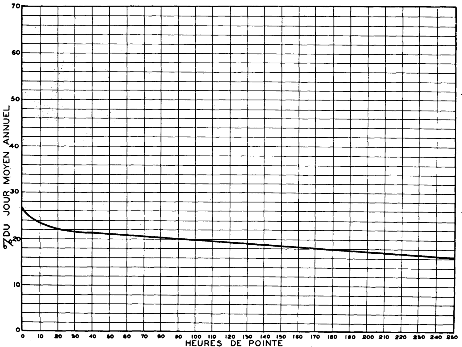
RELATION ENTRE LES HEURES DE POINTE ET LE JOUR MOYEN ANNUEL — STATION: LACOLLE ROUTE N° 15-9-86
