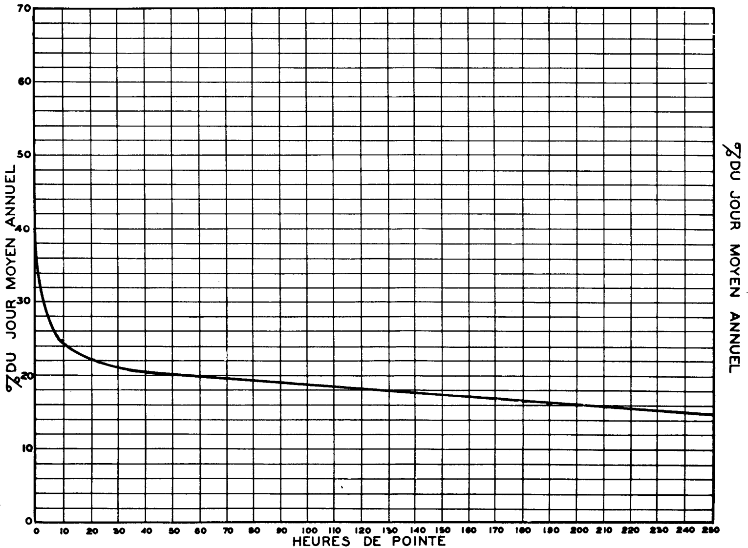
RELATION ENTRE LES HEURES DE POINTE ET LE JOUR MOYEN ANNUEL STATION: ST-ARMAND ROUTE N° 7-9-74
