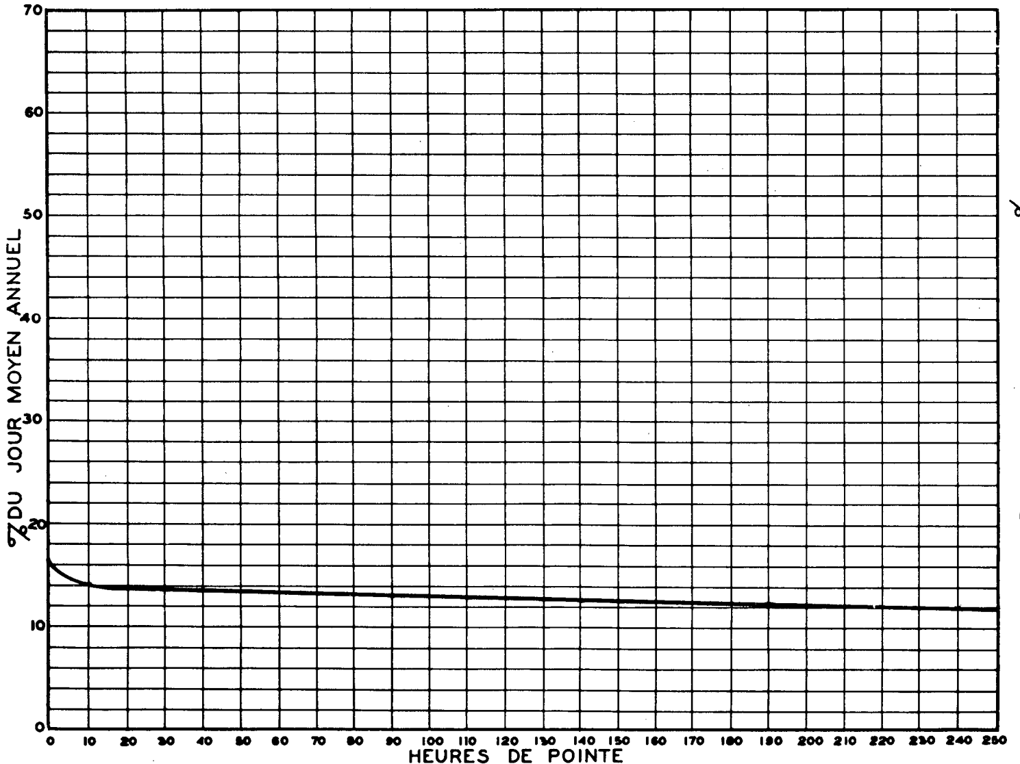
RELATION ENTRE LES HEURES DE POINTE ET LE JOUR MOYEN ANNUEL STATION: ILE-PERROT (VOIE NORD) ROUTE N° 2-4-54
