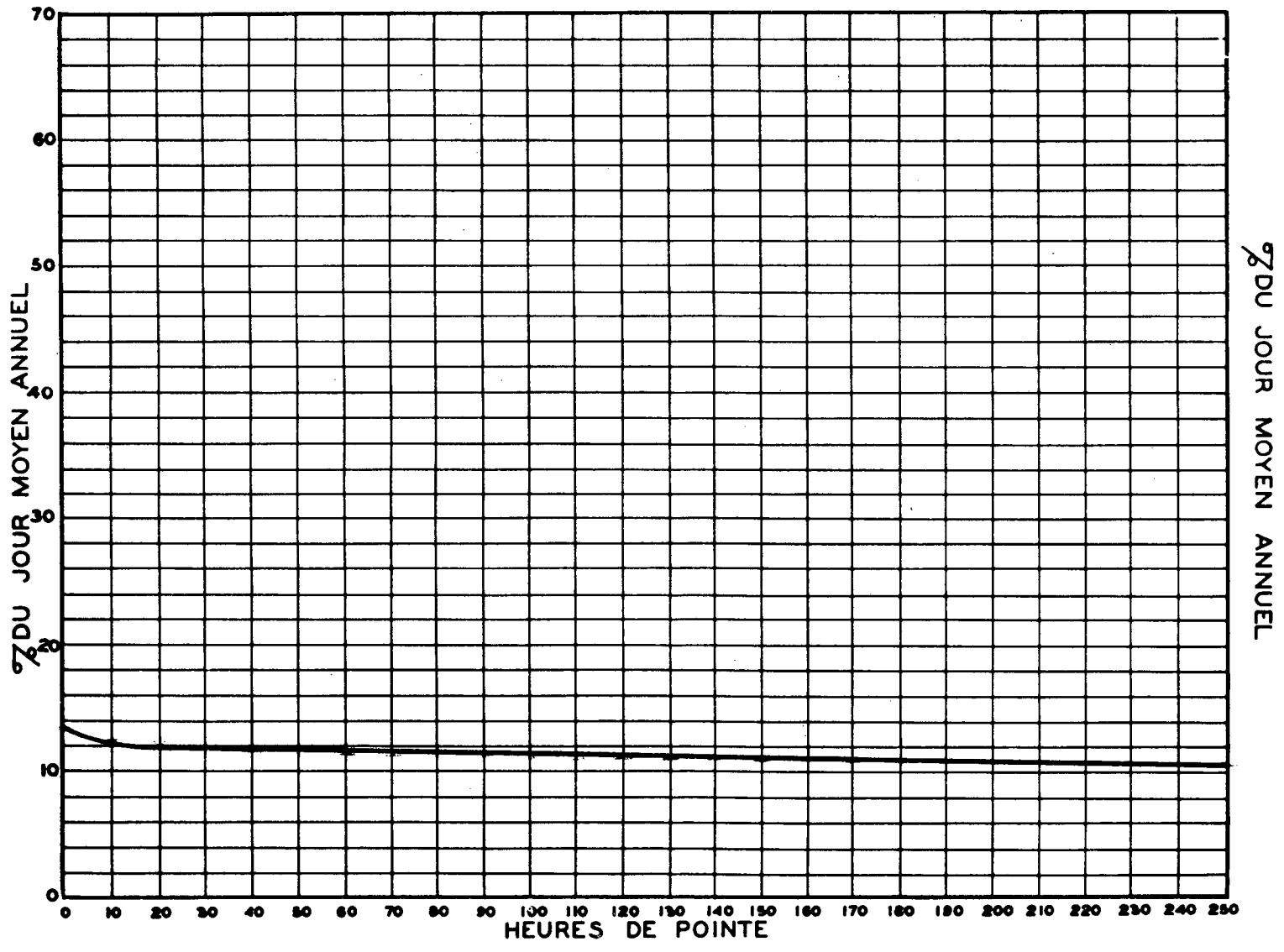
RELATION ENTRE LES HEURES DE POINTE ET LE JOUR MOYEN ANNUEL STATION: JACQUES-CARTIER ROUTE N° 3-20-9-65
