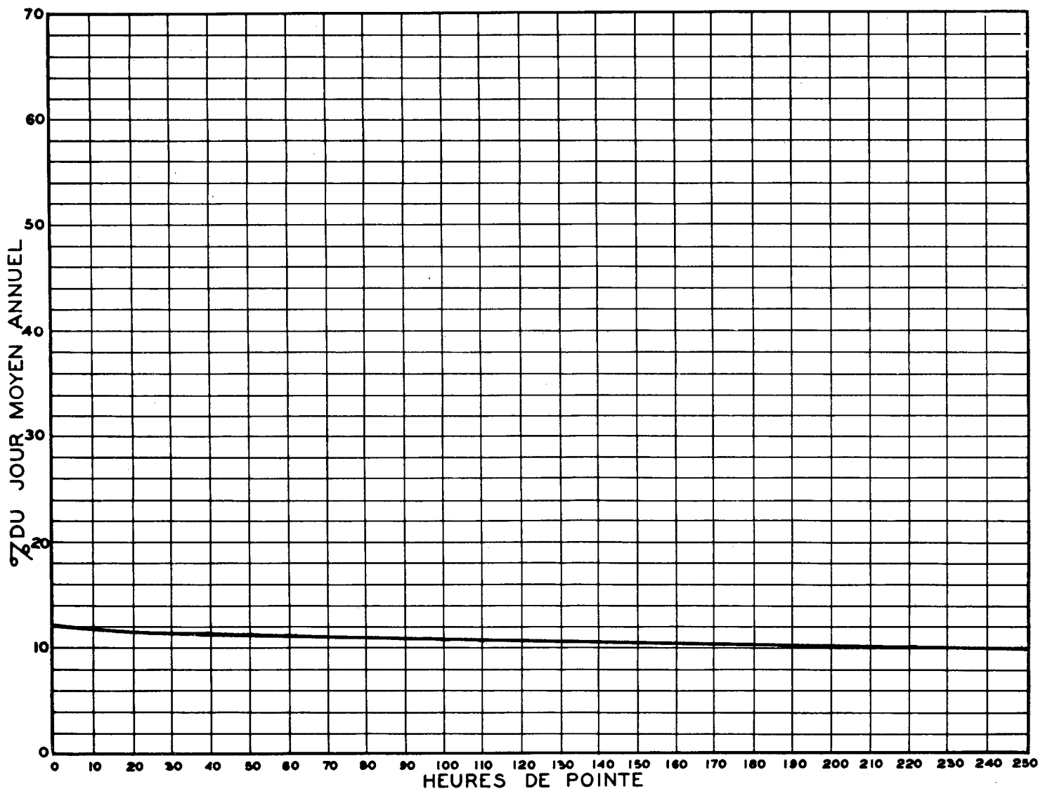
RELATION ENTRE LES HEURES DE POINTE ET LE JOUR MOYEN ANNUEL STATION: HULL ROUTE N° 11-5-71
