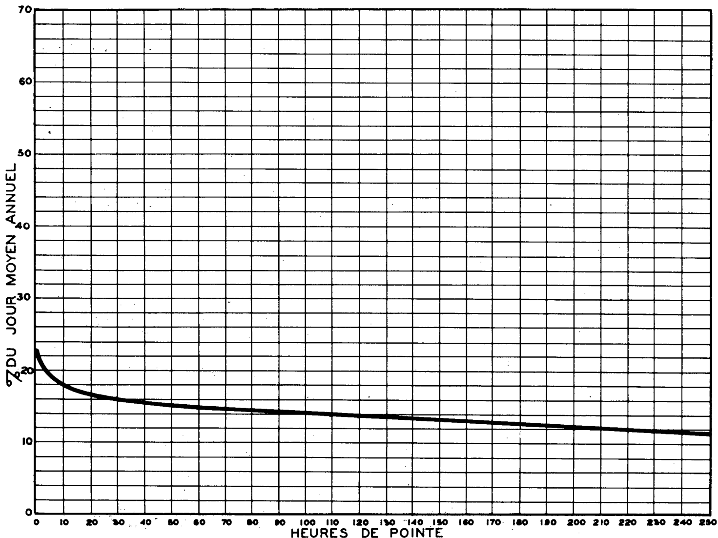
RELATION ENTRE LES HEURES DE POINTE ET LE JOUR MOYEN ANNUEL STATION: VAUDREUIL ROUTE N° 40-4-89 (NORD)
