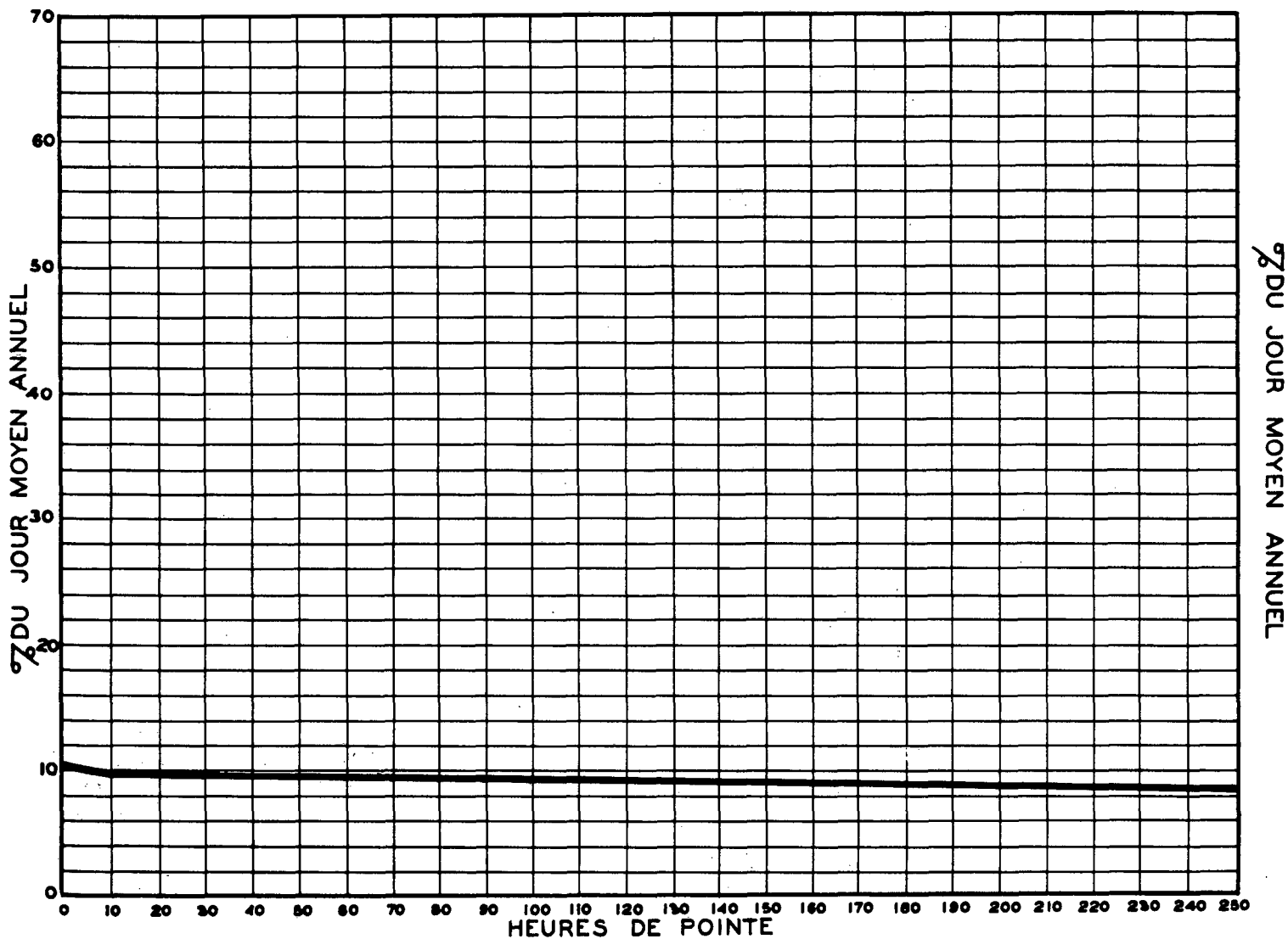
RELATION ENTRE LES HEURES DE POINTE ET LE JOUR MOYEN ANNUEL — STATION: LONGUEUIL PONT JACQUES CARTIER ROUTE N° 9-9-80 (2 VOIES)
