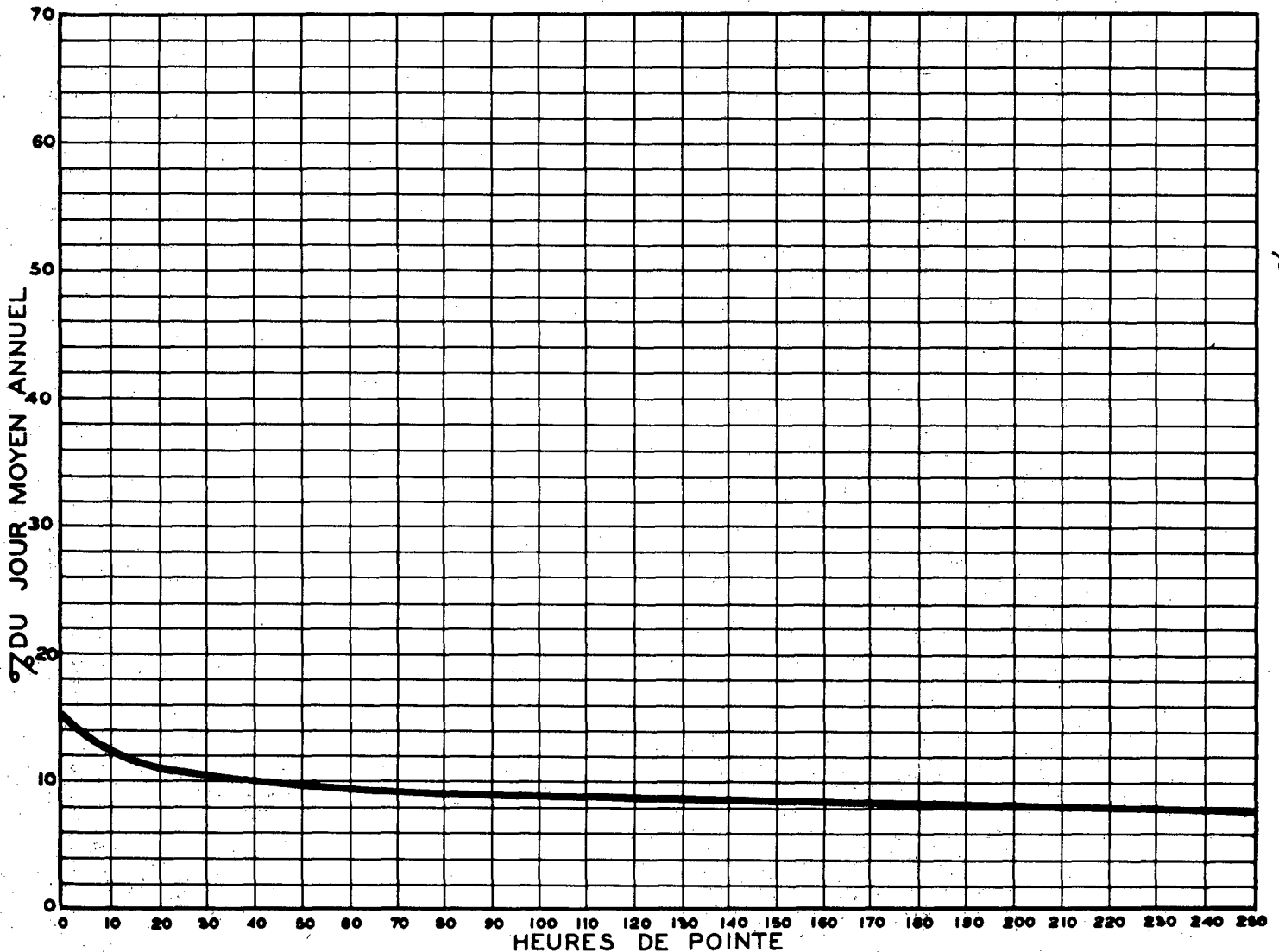
RELATION ENTRE LES HEURES DE POINTE ET LE JOUR MOYEN ANNUEL STATION: ST-NICEPHORE ROUTE N° 22-8-2
