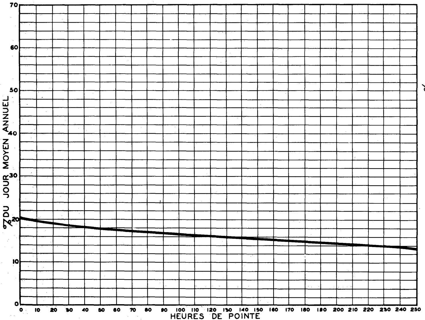
RELATION ENTRE LES HEURES DE POINTE ET LE JOUR MOYEN ANNUEL — STATION: MONTREAL (PONT PAPINEAU) EST ROUTE N° R-S-404
