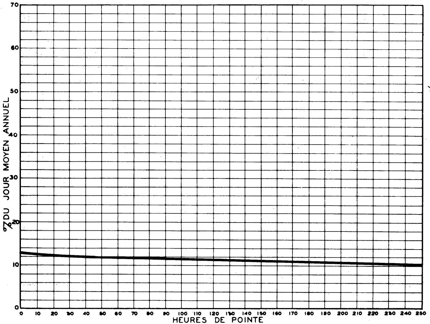
RELATION ENTRE LES HEURES DE POINTE ET LE JOUR MOYEN ANNUEL — STATION: MONTREAL (PONT PAPINEAU) 2 VOIES ROUTE N° R-S-404
