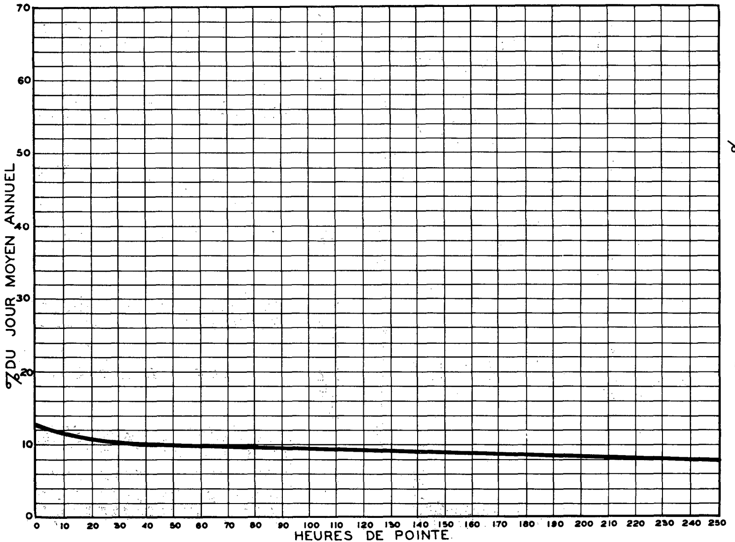
RELATION ENTRE LES HEURES DE POINTE ET LE JOUR MOYEN ANNUEL STATION: LENNOXVILLE ROUTE N° 28-3-3
