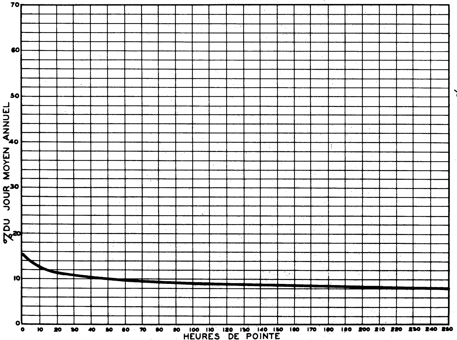
RELATION ENTRE LES HEURES DE POINTE ET LE JOUR MOYEN ANNUEL STATION: LENNOXVILLE ROUTE N° 22-3-3
