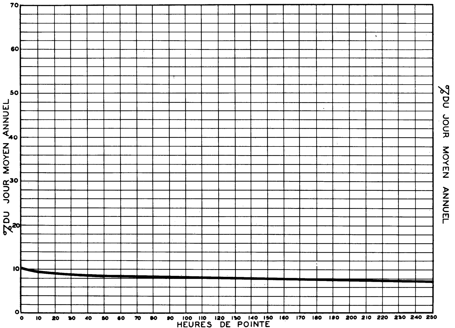
RELATION ENTRE LES HEURES DE POINTE ET LE JOUR MOYEN ANNUEL — 314 STATION: SHERBROOKE ROUTE N° 5-22-3-12 (2 VOIES)
