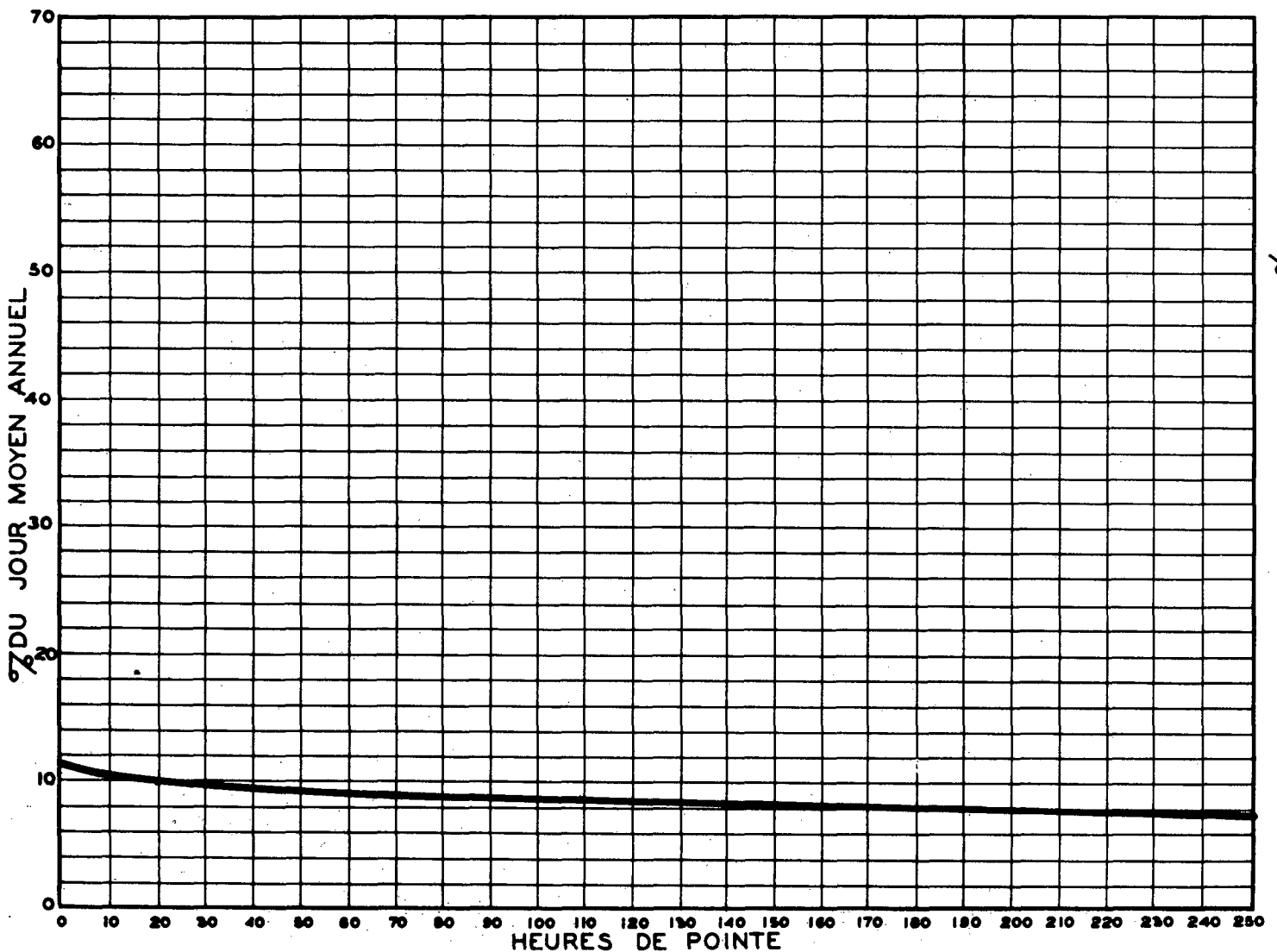
RELATION ENTRE LES HEURES DE POINTE ET LE JOUR MOYEN ANNUEL STATION: ST-HENRI ROUTE N° 23-1-1
