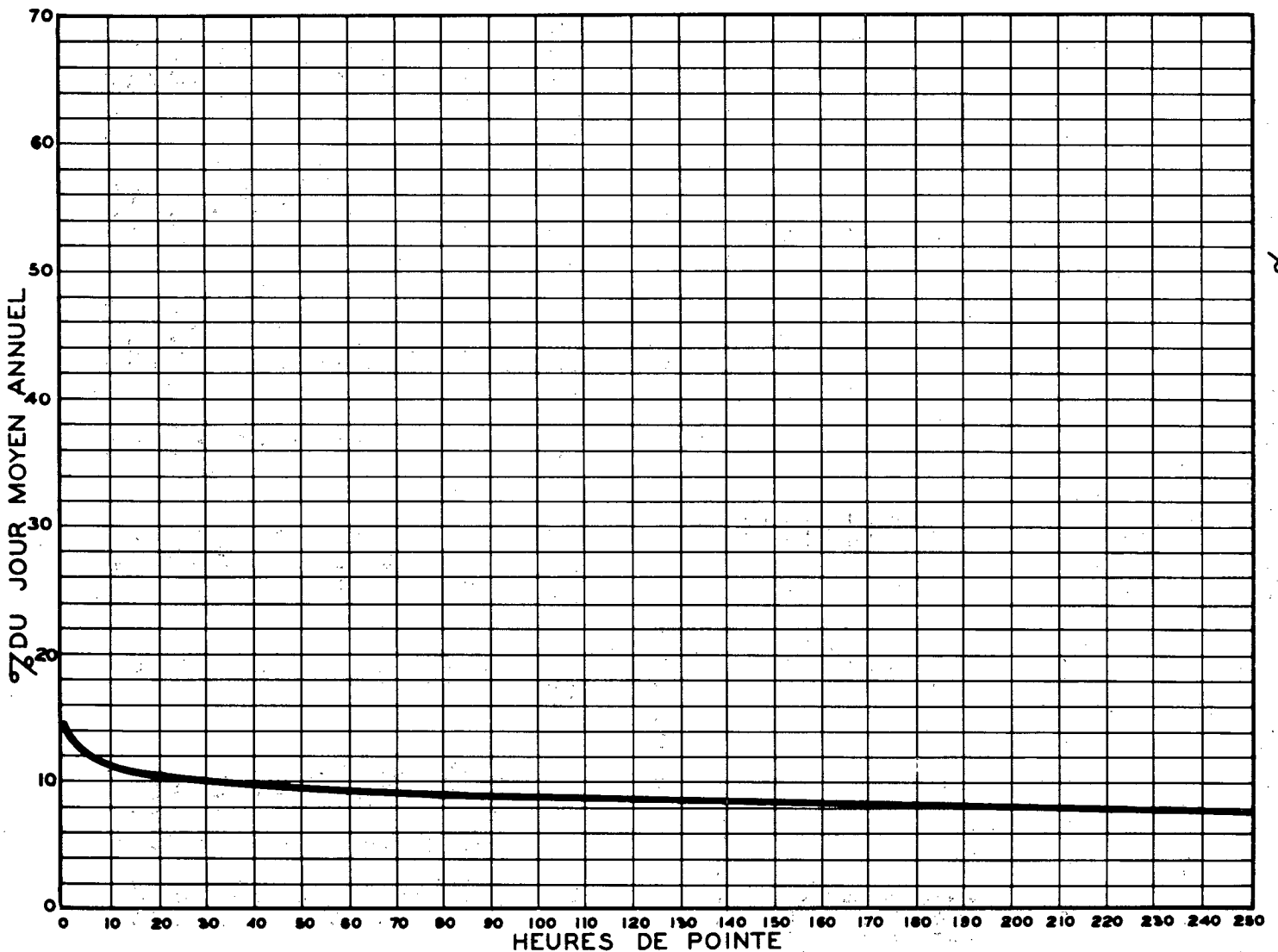
RELATION ENTRE LES HEURES DE POINTE ET LE JOUR MOYEN ANNUEL STATION: STE-MARIE ROUTE N° 23-3-2
