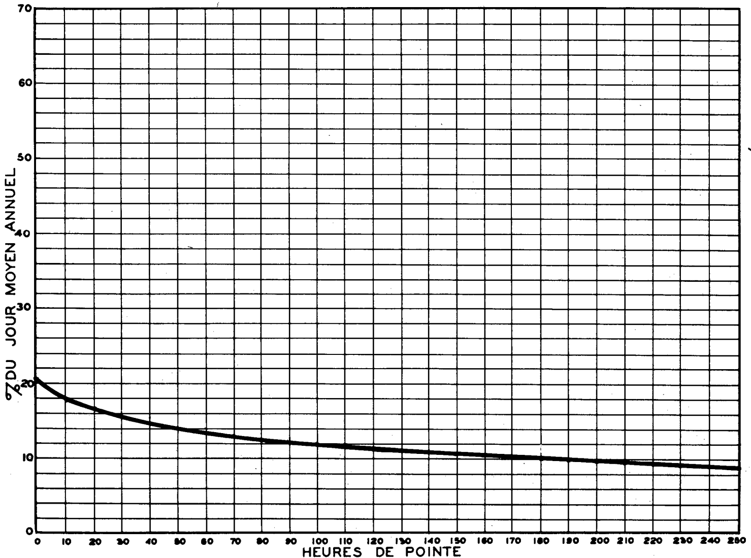
RELATION ENTRE LES HEURES DE POINTE ET LE JOUR MOYEN ANNUEL STATION: ANCIENNE-LORETTE ROUTE N° 2-1-7 (SUD)
