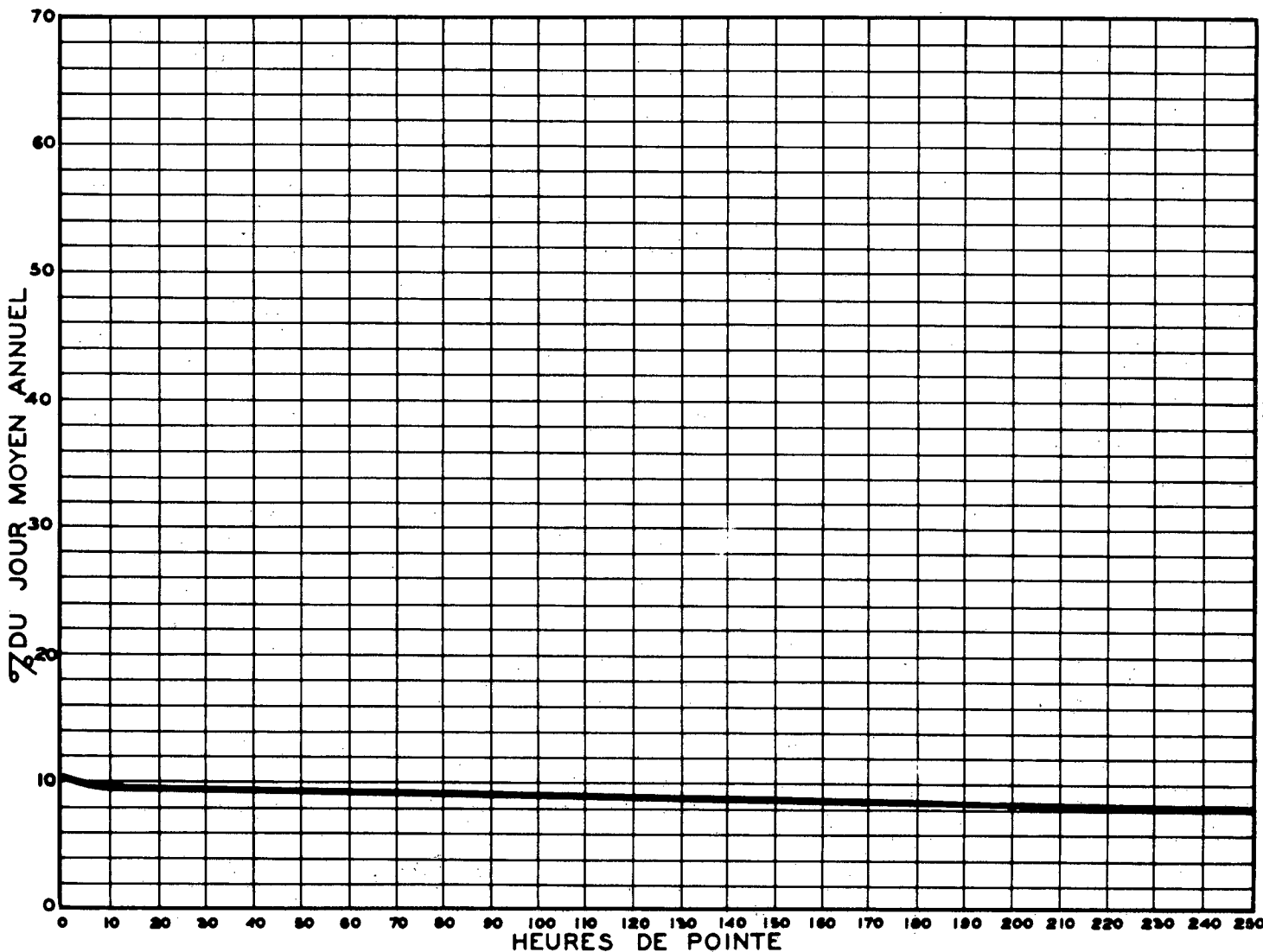
RELATION ENTRE LES HEURES DE POINTE ET LE JOUR MOYEN ANNUEL — STATION: ST-ROMUALD ROUTE N° 2-1-4 (2 VOIES)
