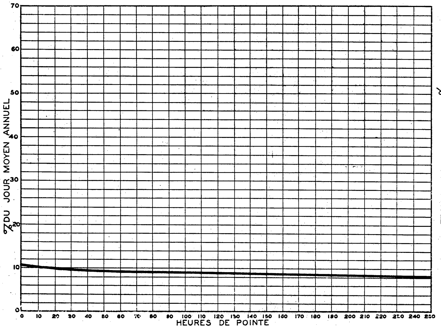
RELATION ENTRE LES HEURES DE POINTE ET LE JOUR MOYEN ANNUEL — STATION: ST-LAURENT ROUTE N° 40-4-87 (NORD)
