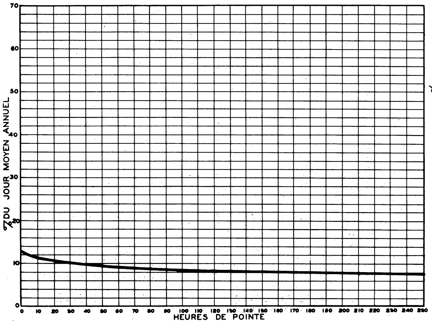
RELATION ENTRE LES HEURES DE POINTE ET LE JOUR MOYEN ANNUEL STATION: SHERBROOKE ROUTE N° 1-3-11
