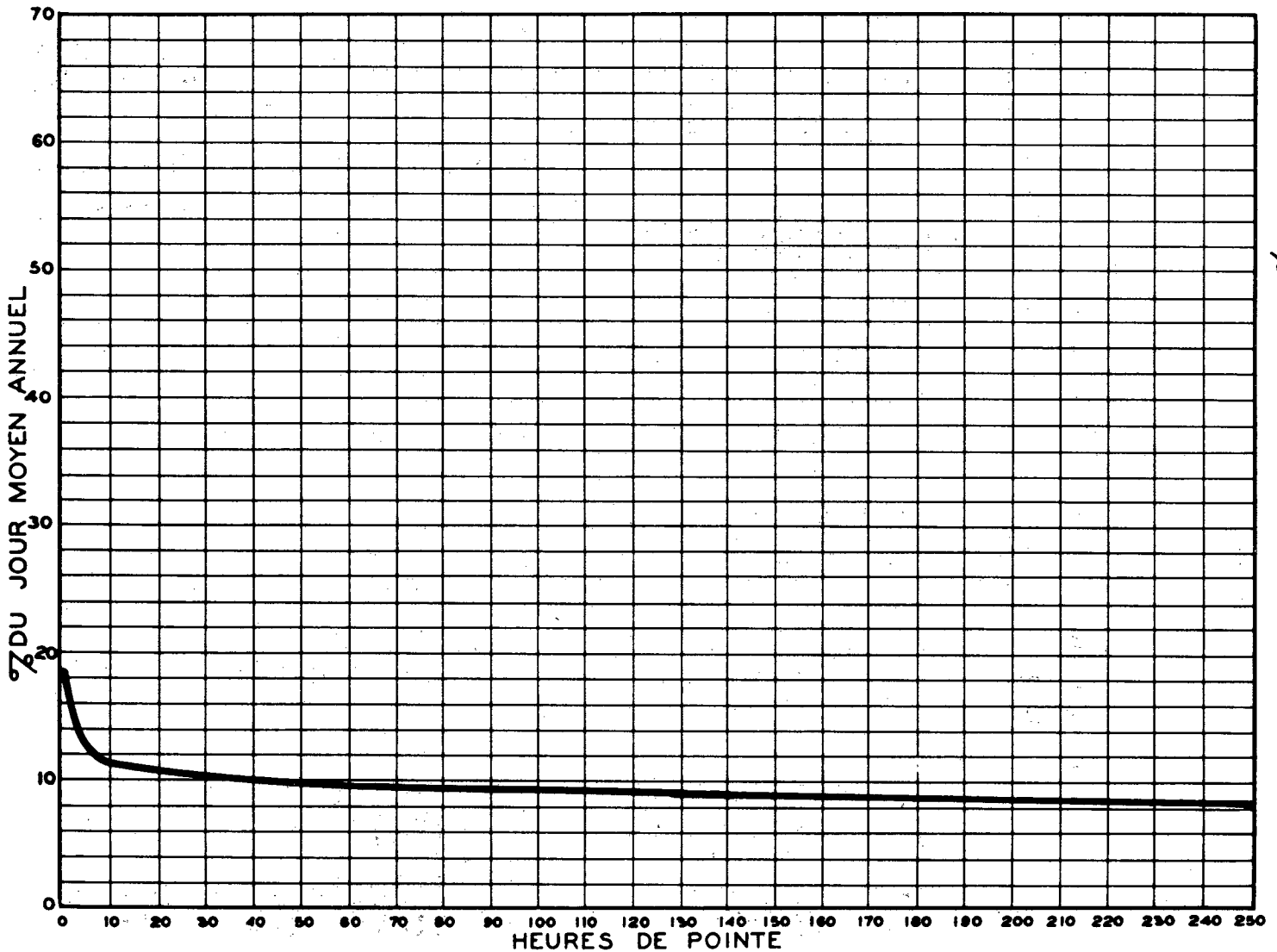
RELATION ENTRE LES HEURES DE POINTE ET LE JOUR MOYEN ANNUEL STATION: LAVAL ROUTE N° S-4-55
