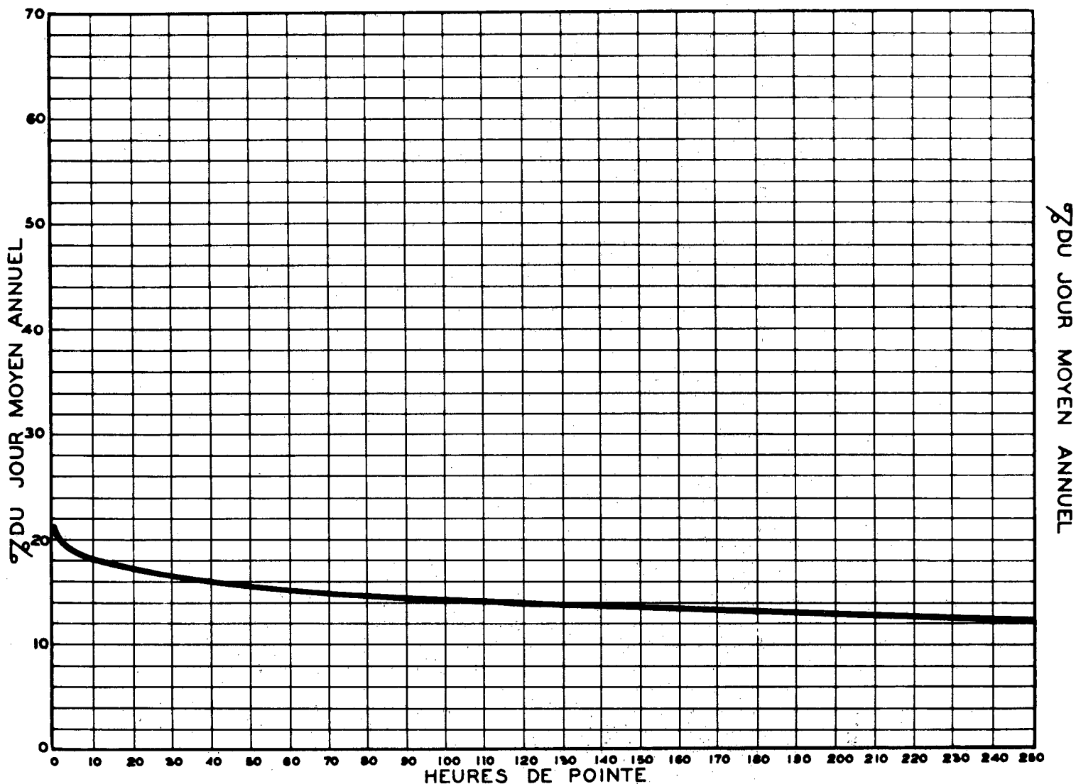
RELATION ENTRE LES HEURES DE POINTE ET LE JOUR MOYEN ANNUEL STATION: ST-PATRICE ROUTE N° 10-1-1
