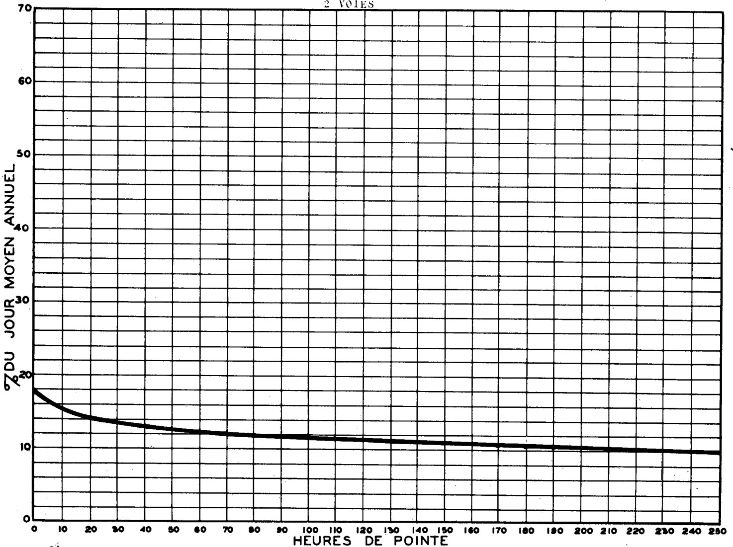
RELATION ENTRE LES HEURES DE POINTE ET LE JOUR MOYEN ANNUEL — STATION: ST-GREGOIRE (PONT DE TROIS-RIVIERES) ROUTE N° R-S-815 2 VOIES
