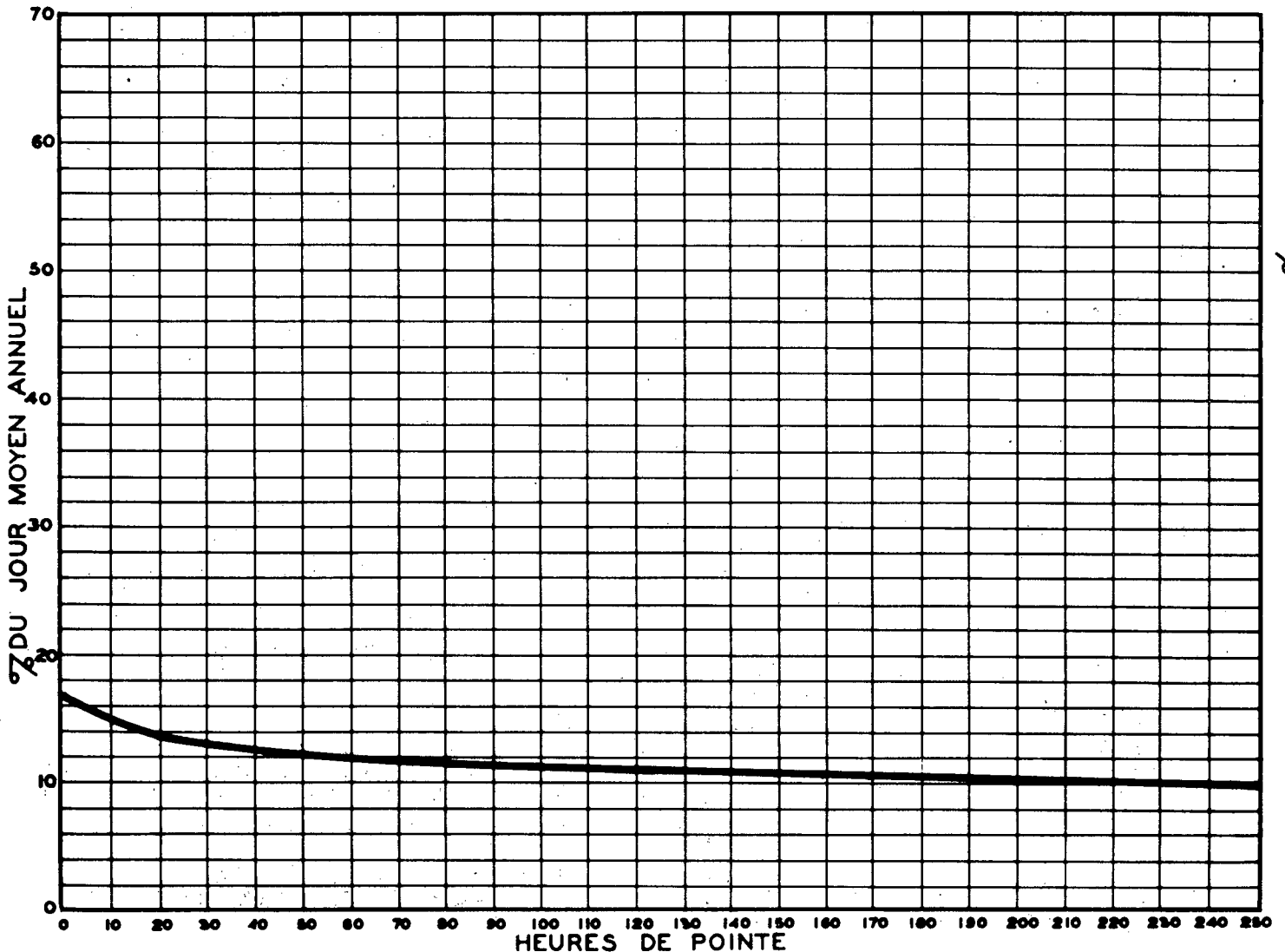
RELATION ENTRE LES HEURES DE POINTE ET LE JOUR MOYEN ANNUEL — STATION: MAGOG ROUTE N° 1-3-3 (SUD)
