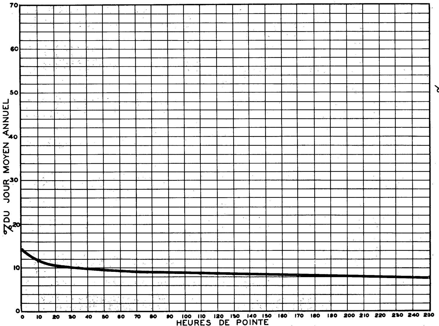
RELATION ENTRE LES HEURES DE POINTE ET LE JOUR MOYEN ANNUEL STATION: ST-JOSEPH ROUTE N° 23-3-4
