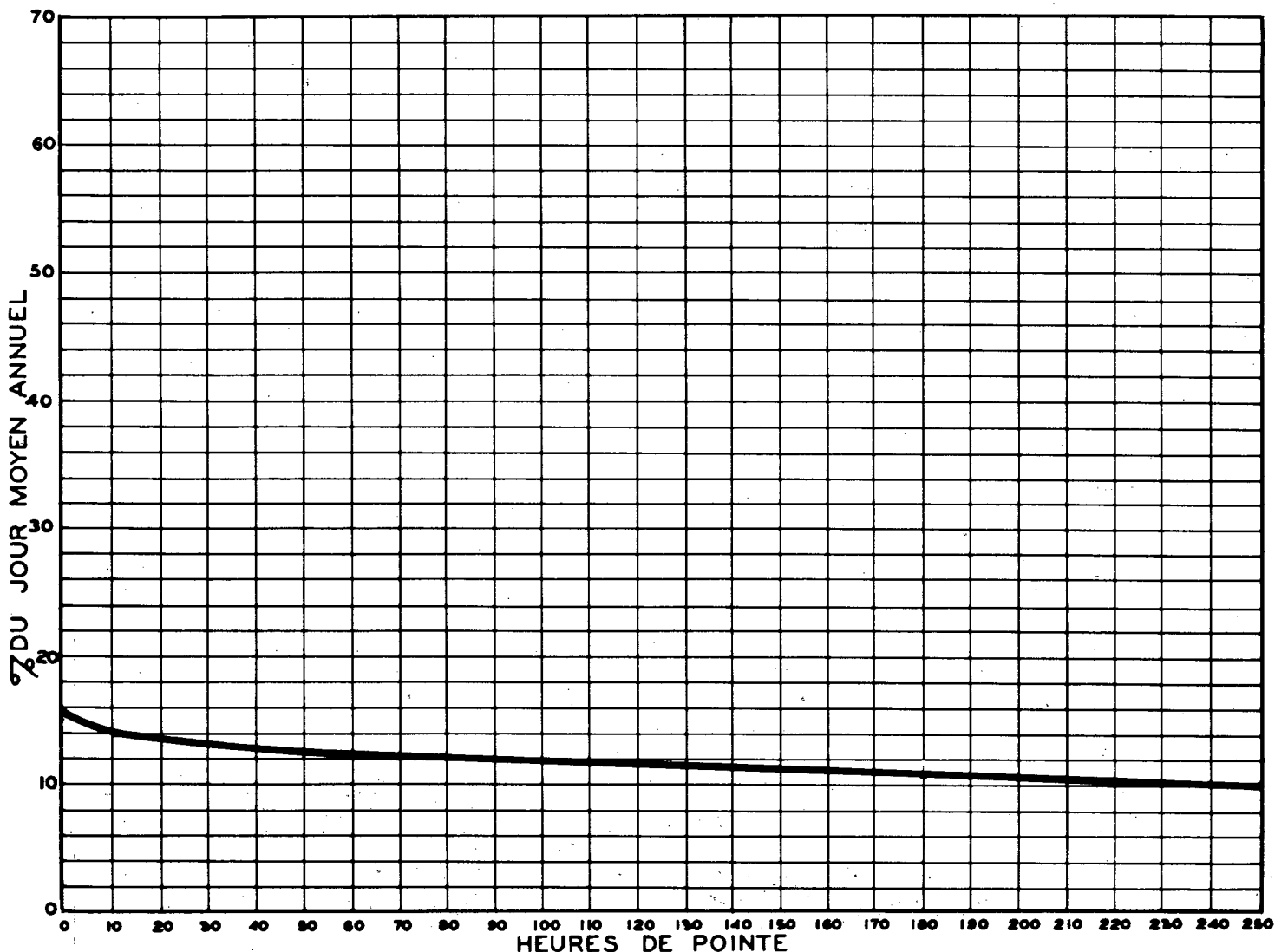
RELATION ENTRE LES HEURES DE POINTE ET LE JOUR MOYEN ANNUEL — STATION: MAGOG ROUTE N° 1-3-3 (2 VOIES)
