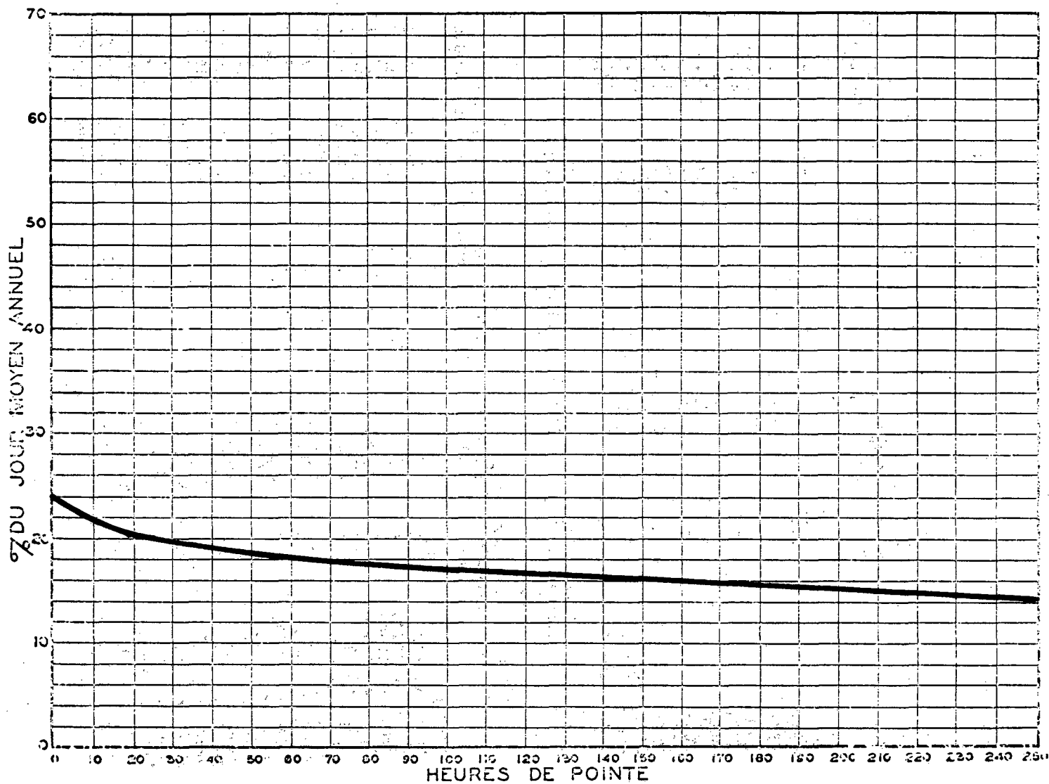
RELATION ENTRE LES HEURES DE POINTE ET LE JOUR MOYEN ANNUEL — STATION: STE-AGATHE ROUTE N° 30-4-51
