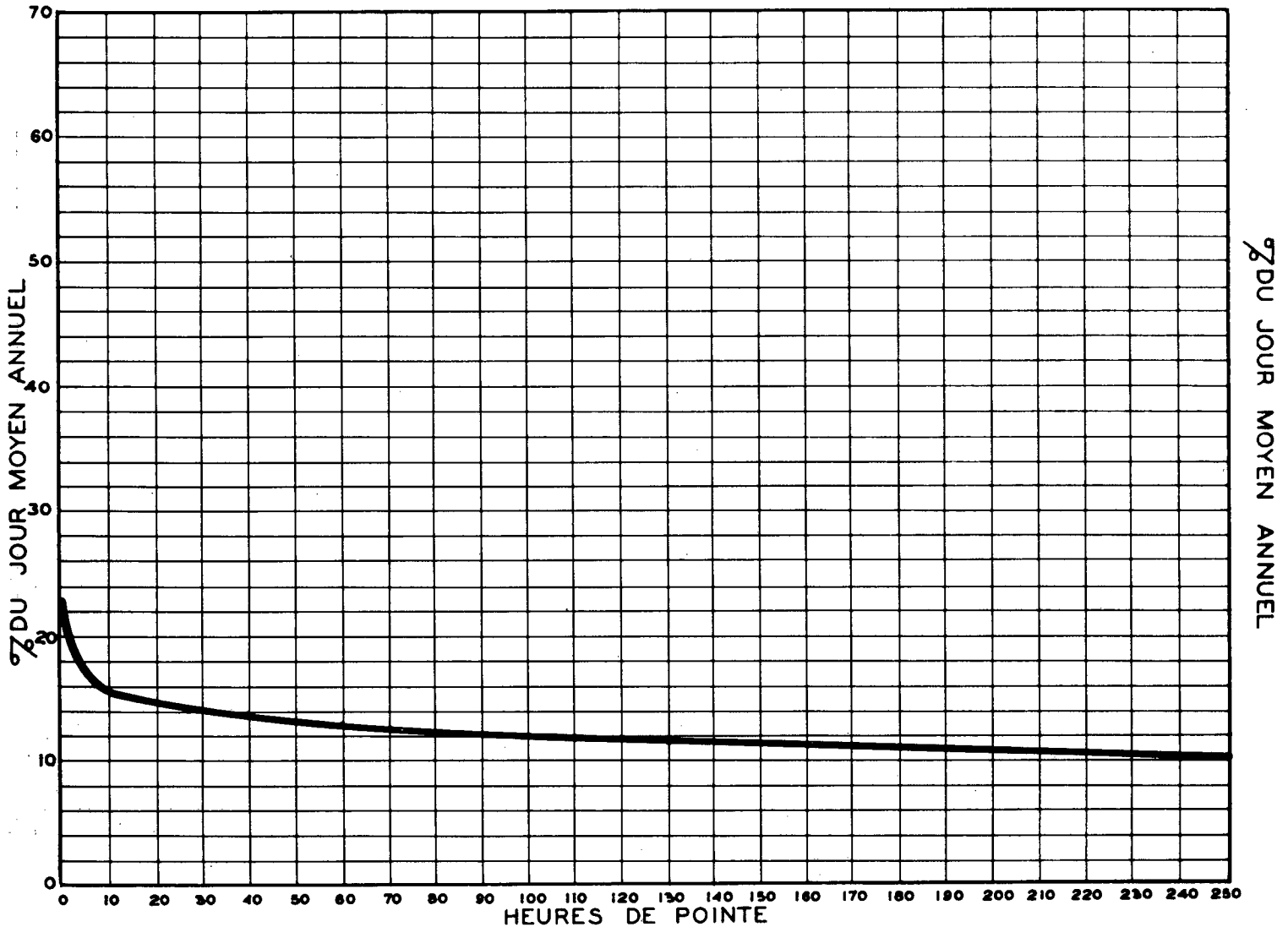
RELATION ENTRE LES HEURES DE POINTE ET LE JOUR MOYEN ANNUEL STATION: ST-GREGOIRE (PONT DE TROIS-RIVIERES) EST ROUTE N° R-S-S15
