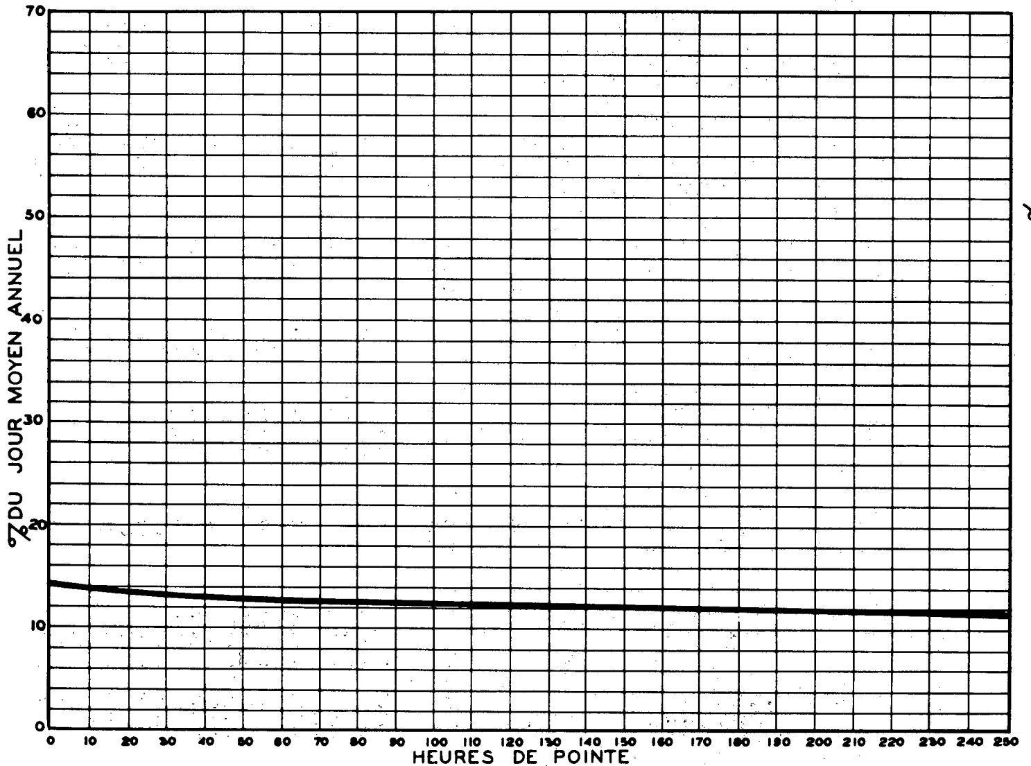
RELATION ENTRE LES HEURES DE POINTE ET LE JOUR MOYEN ANNUEL — STATION: LONGUEUIL PONT JACQUES CARTIER ROUTE N° 9-9-80 (SUD)
