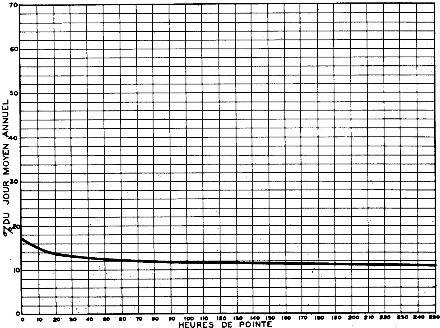
RELATION ENTRE LES HEURES DE POINTE ET LE JOUR MOYEN ANNUEL — STATION: ST-LAMBERT ROUTE N° 3-20-9-60
