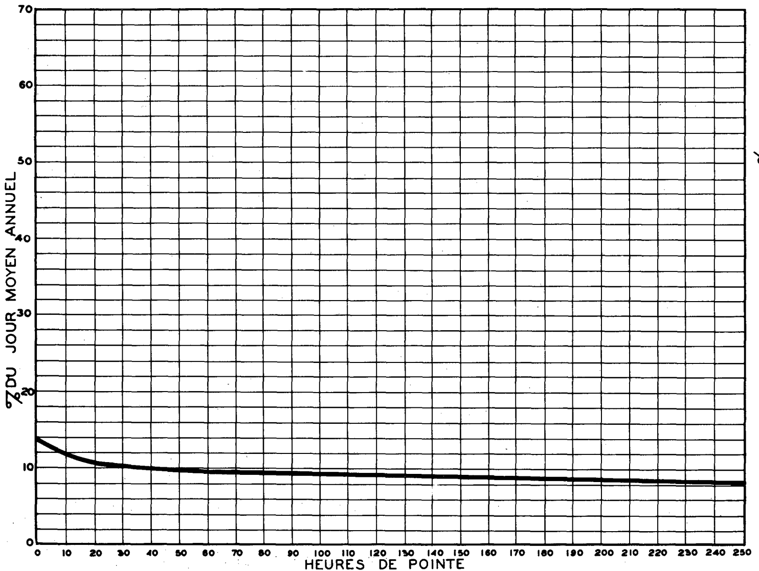
RELATION ENTRE LES HEURES DE POINTE ET LE JOUR MOYEN ANNUEL STATION: STE-ANNE DE RISTIGOUCHE ROUTE N° R-S-202
