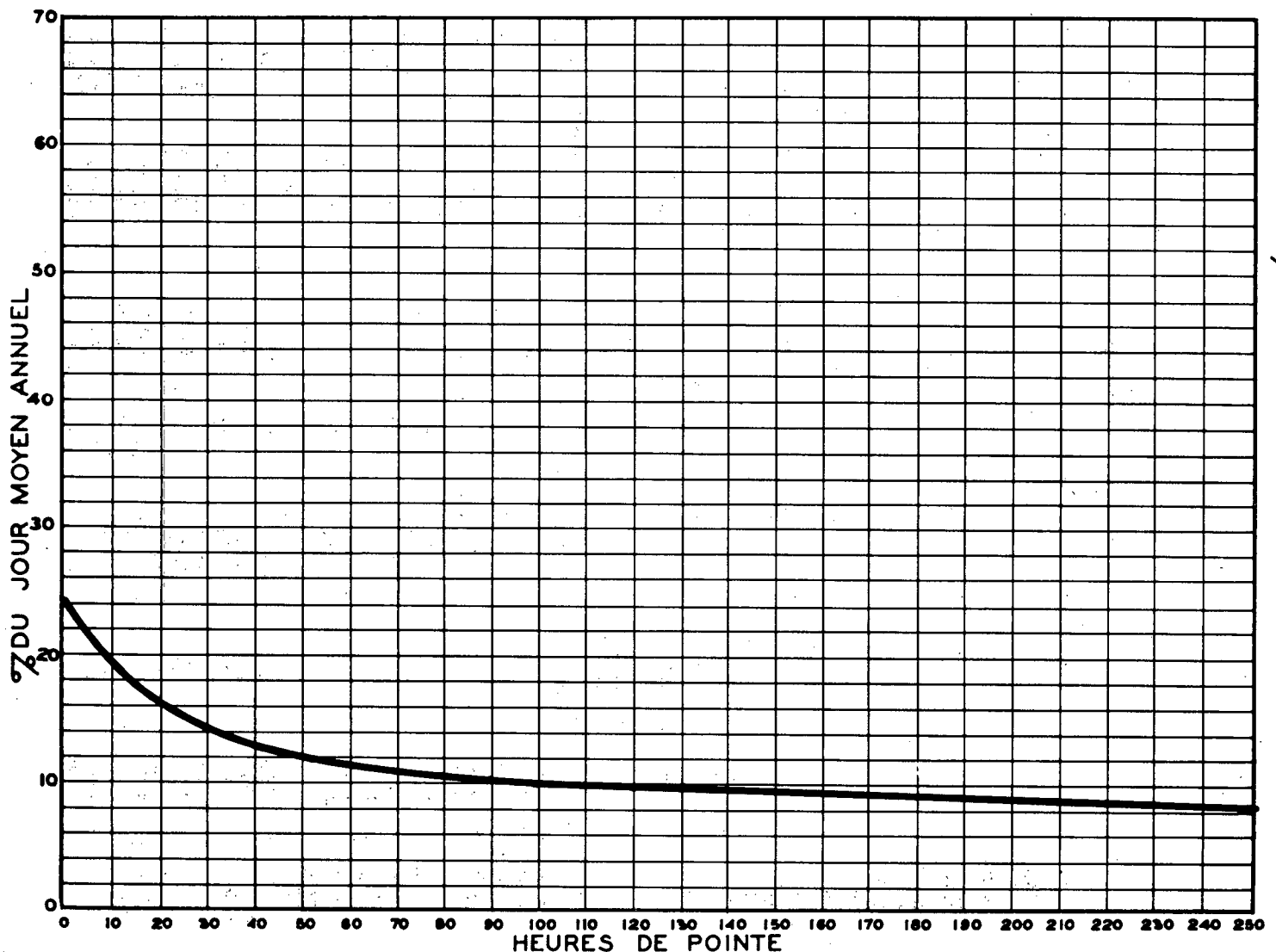
RELATION ENTRE LES HEURES DE POINTE ET LE JOUR MOYEN ANNUEL STATION: ST-GEORGES ROUTE N° 23-3-6
