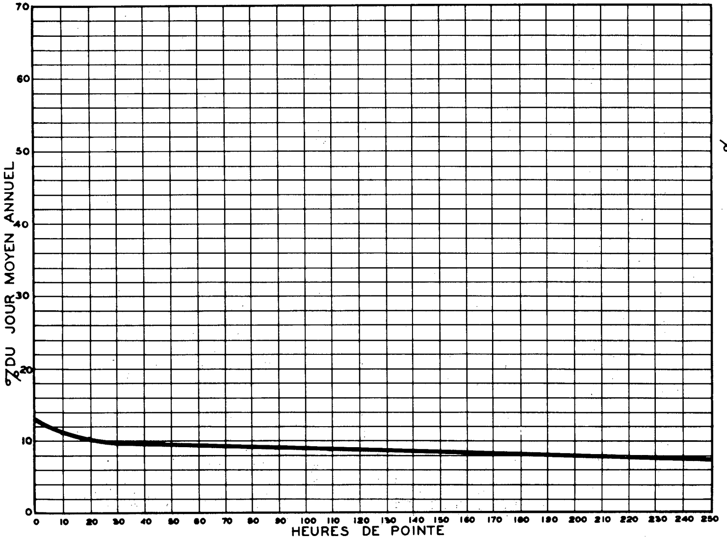
RELATION ENTRE LES HEURES DE POINTE ET LE JOUR MOYEN ANNUEL — STATION: SHERBROOKE ROUTE N° 1-3-4 (A.V.D.)
