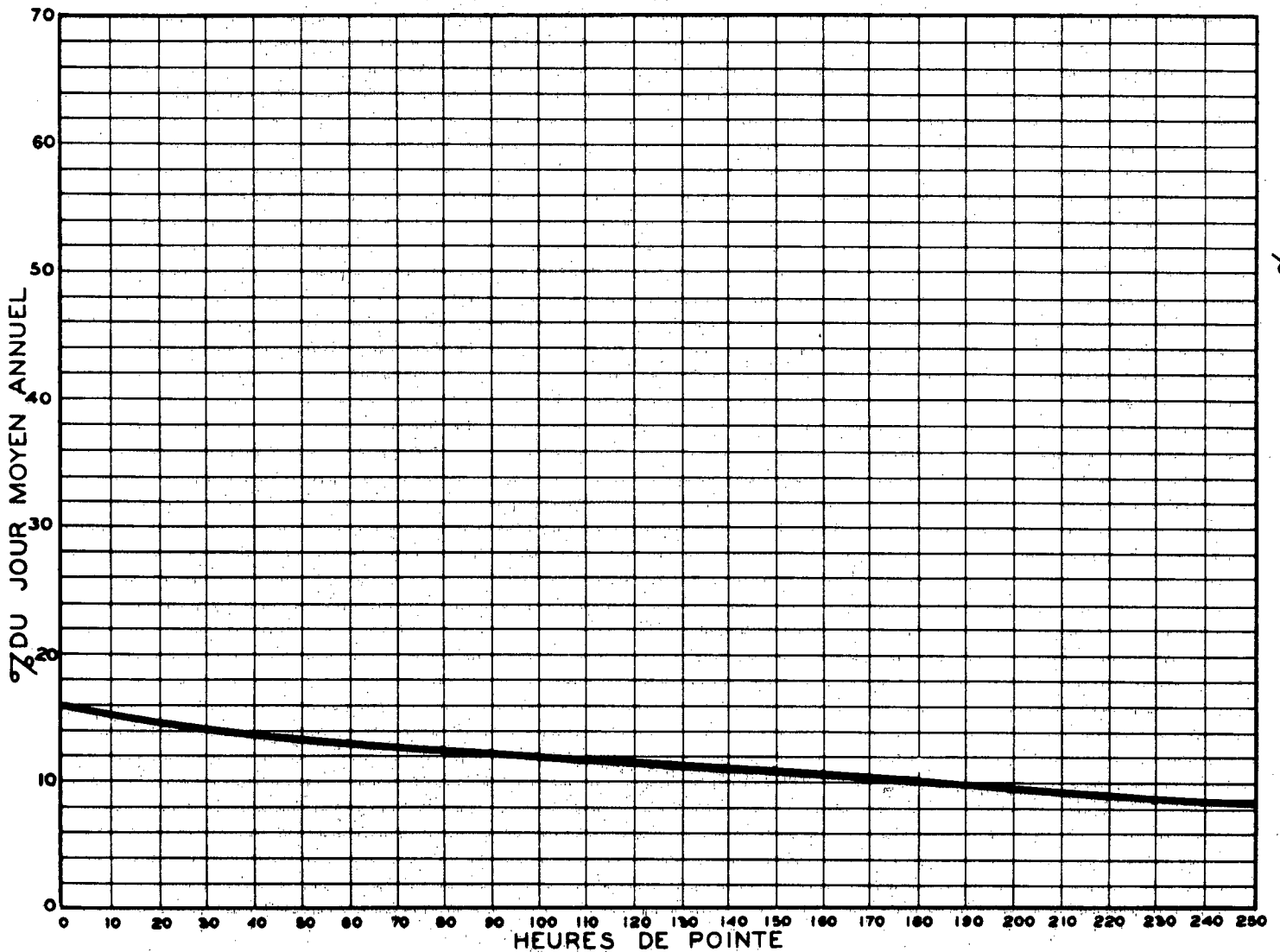
RELATION ENTRE LES HEURES DE POINTE ET LE JOUR MOYEN ANNUEL — STATION: POINTE-AUX-TREMBLES ROUTE N° 2-4-55 (EST)
