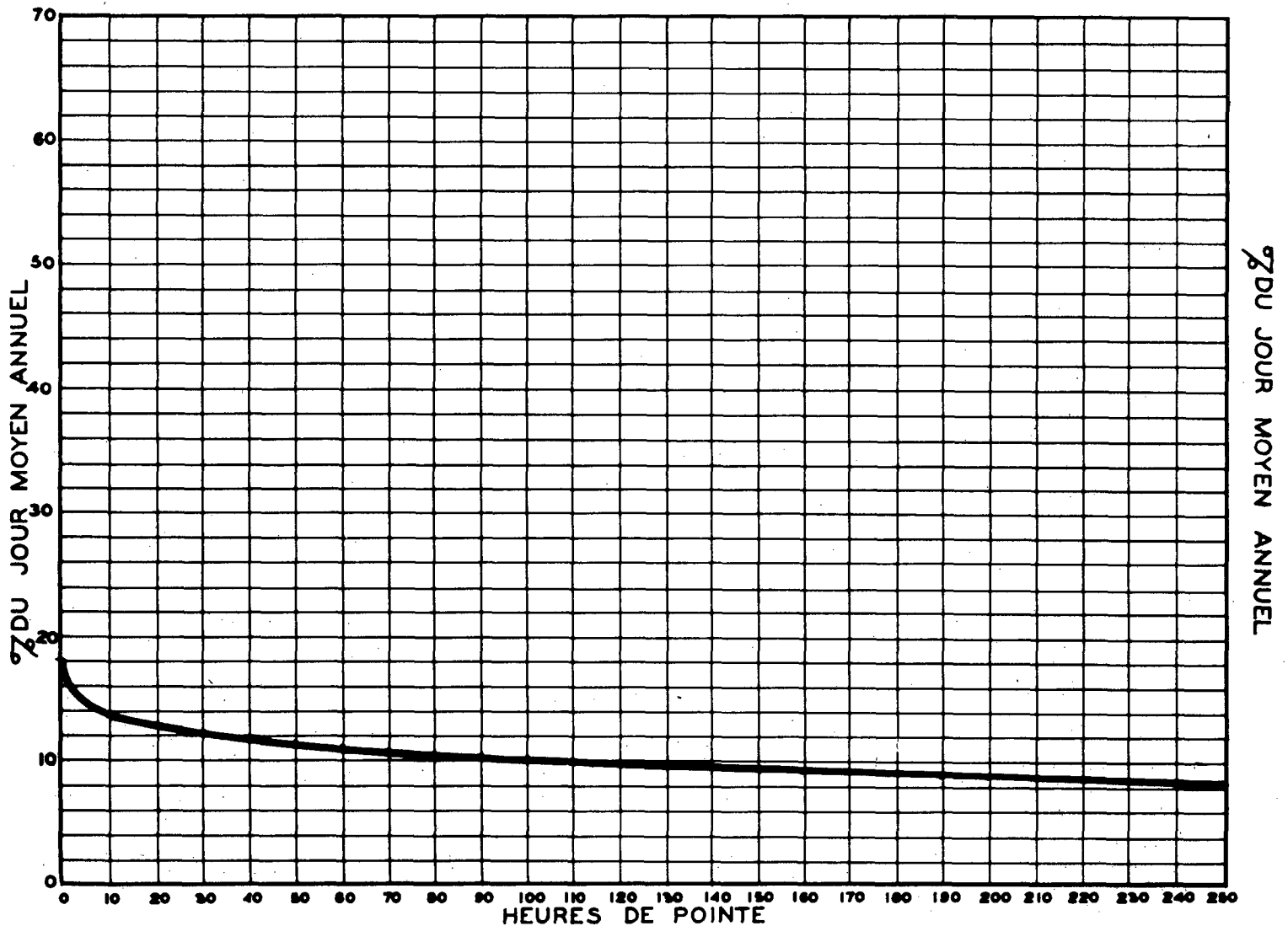
RELATION ENTRE LES HEURES DE POINTE ET LE JOUR MOYEN ANNUEL STATION: ST-LAMBERT ROUTE N° 1-1-2
