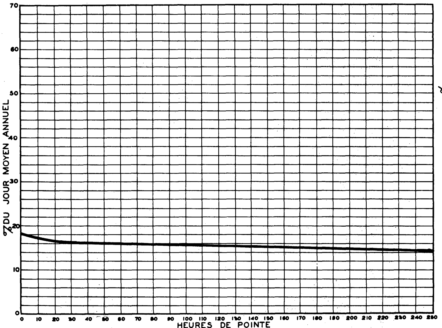
RELATION ENTRE LES HEURES DE POINTE ET LE JOUR MOYEN ANNUEL — STATION: ST-LAMBERT PONT VICTORIA — ROUTE N° 7-9-82 (SUD)
