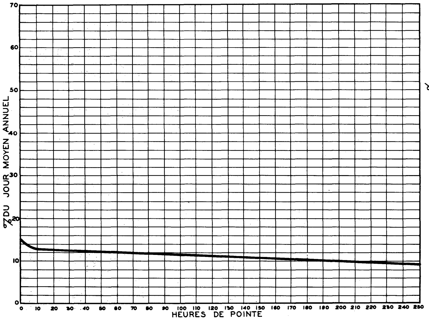
RELATION ENTRE LES HEURES DE POINTE ET LE JOUR MOYEN ANNUEL — STATION: LAVAL PONT LACHAPELLE ROUTE N° 11-4-81 (OUEST)
