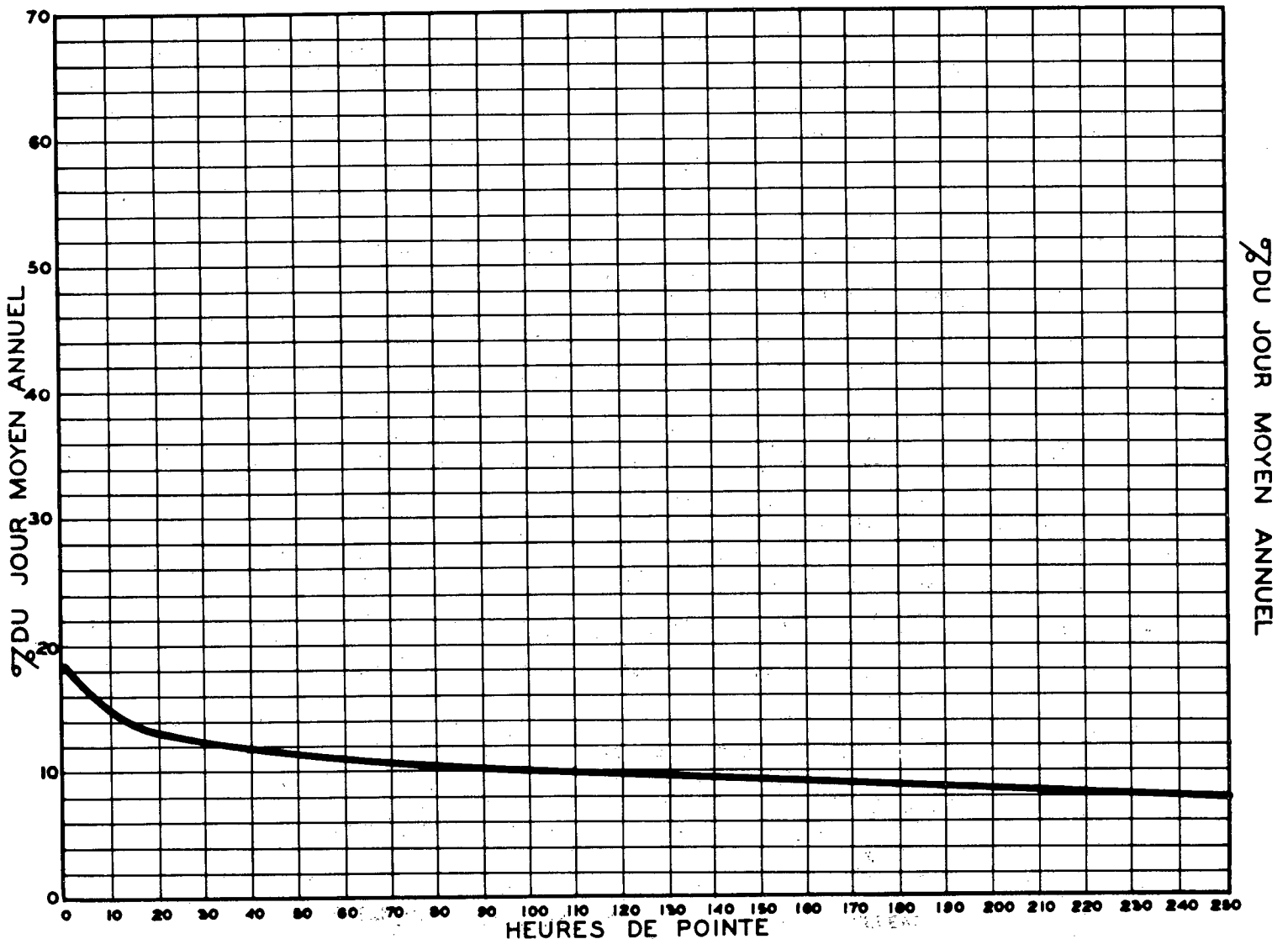
RELATION ENTRE LES HEURES DE POINTE ET LE JOUR MOYEN ANNUEL STATION: ST-NICOLAS ROUTE N° 20-1-11 (2 VOIES)
