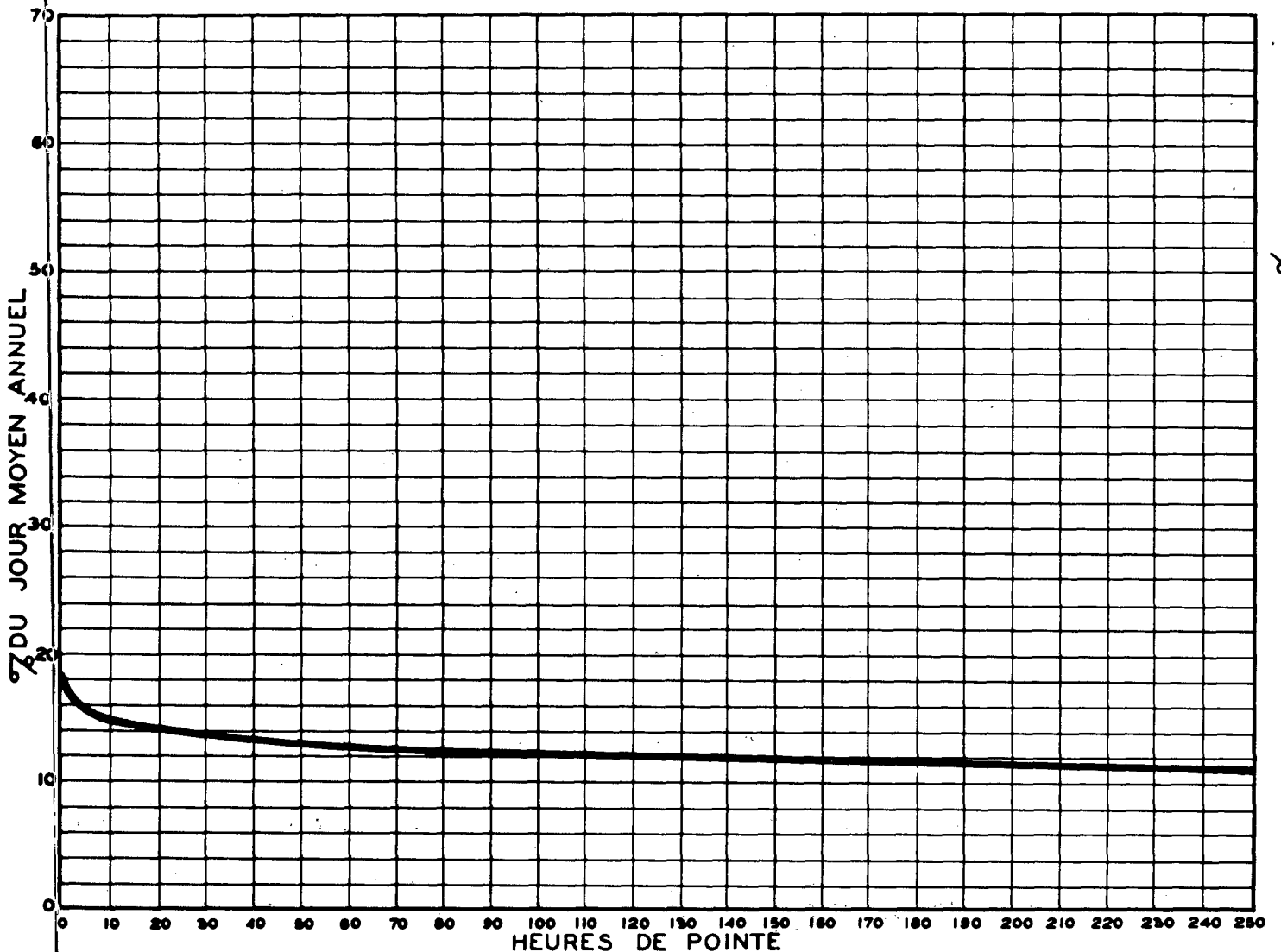
RELATION ENTRE LES HEURES DE POINTE ET LE JOUR MOYEN ANNUEL — STATION: ANQUI ROUTE N° 6-2-1
