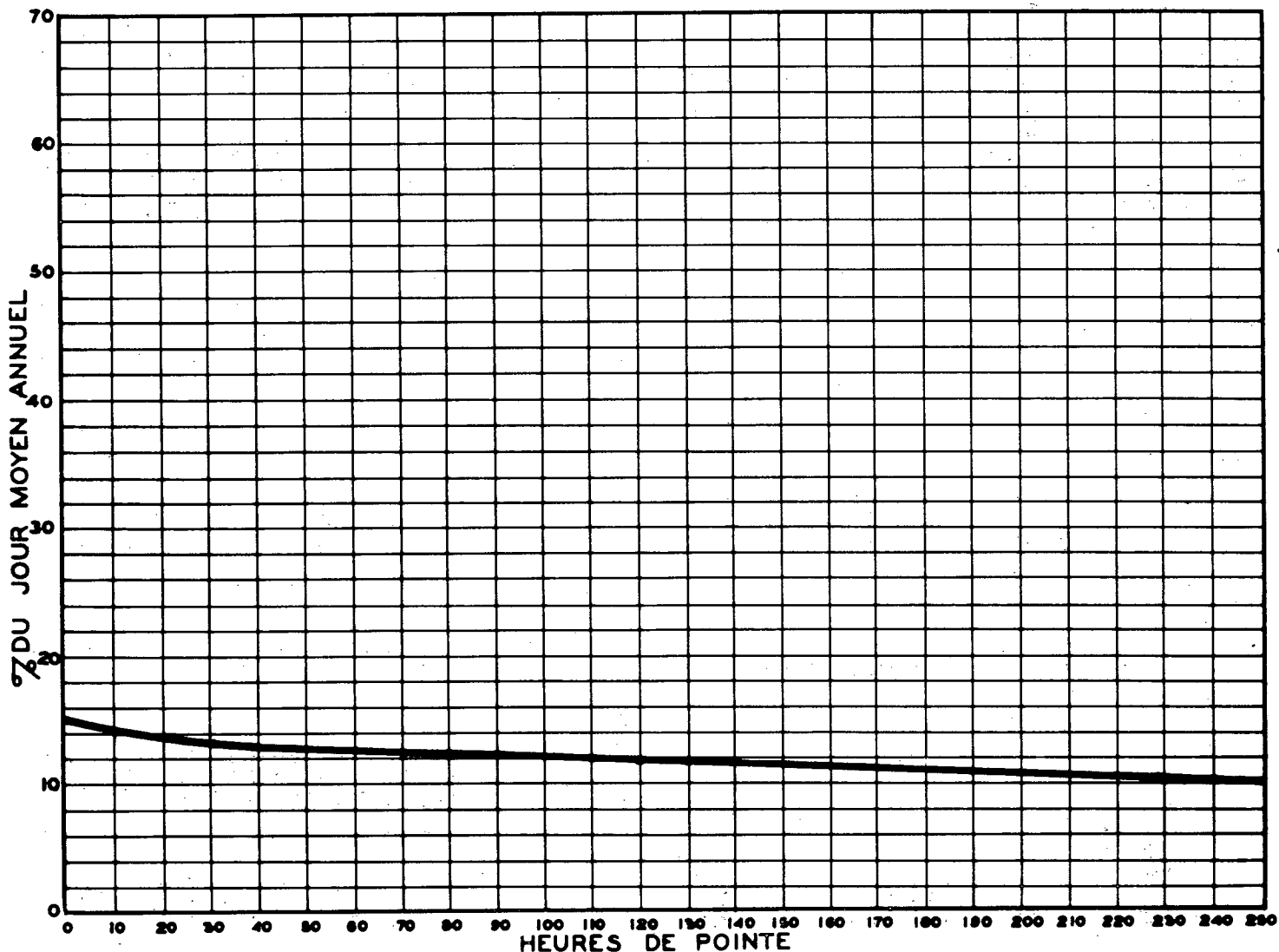
RELATION ENTRE LES HEURES DE POINTE ET LE JOUR MOYEN ANNUEL — STATION: ILE PERROT PONT GALIPEAULT ROUTE N° 2-4-54 (NORD)
