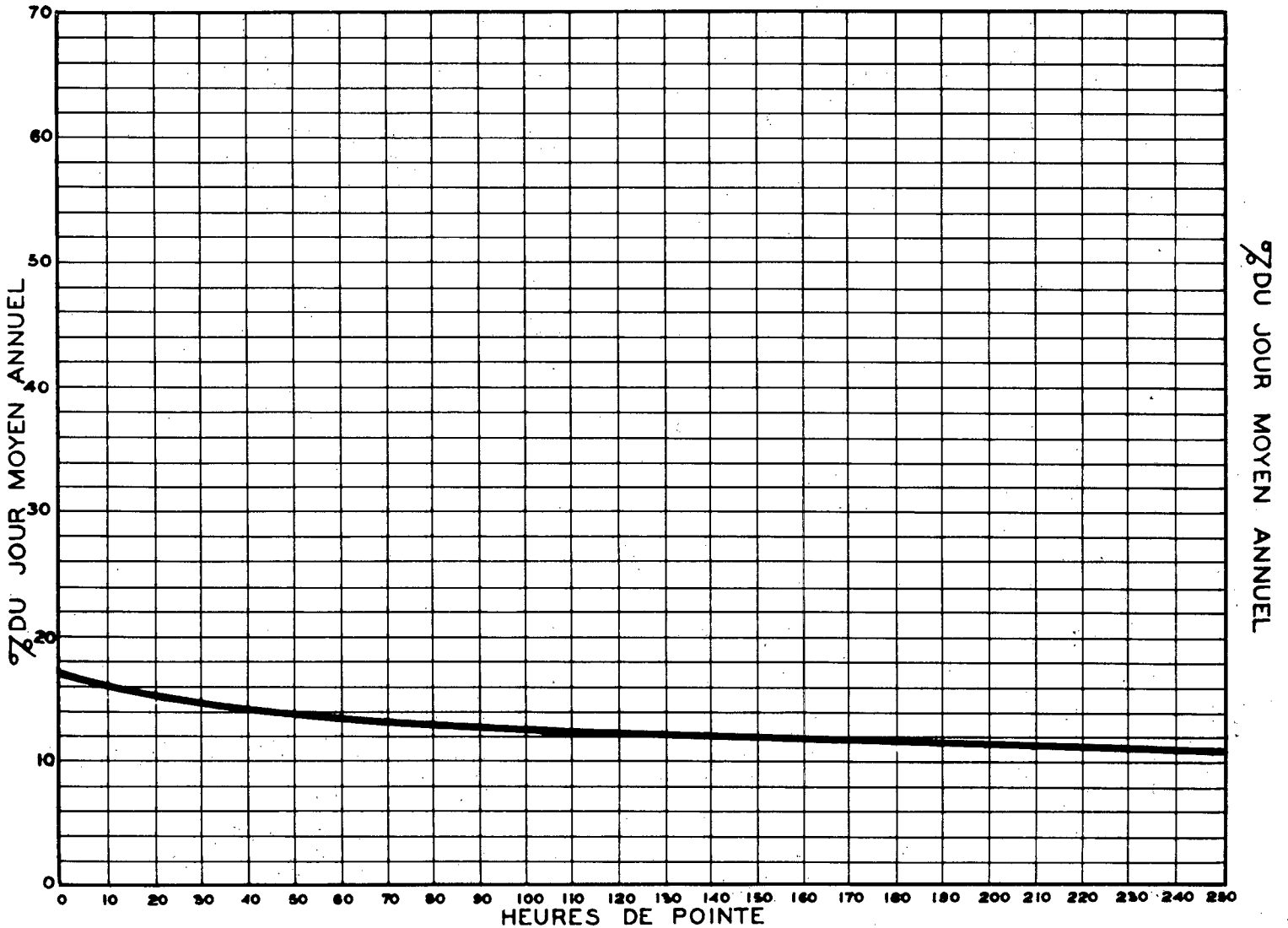
RELATION ENTRE LES HEURES DE POINTE ET LE JOUR MOYEN ANNUEL — STATION: ANCIENNE-LORETTE — ROUTE N° 2-1-7 (2 VOIES)
