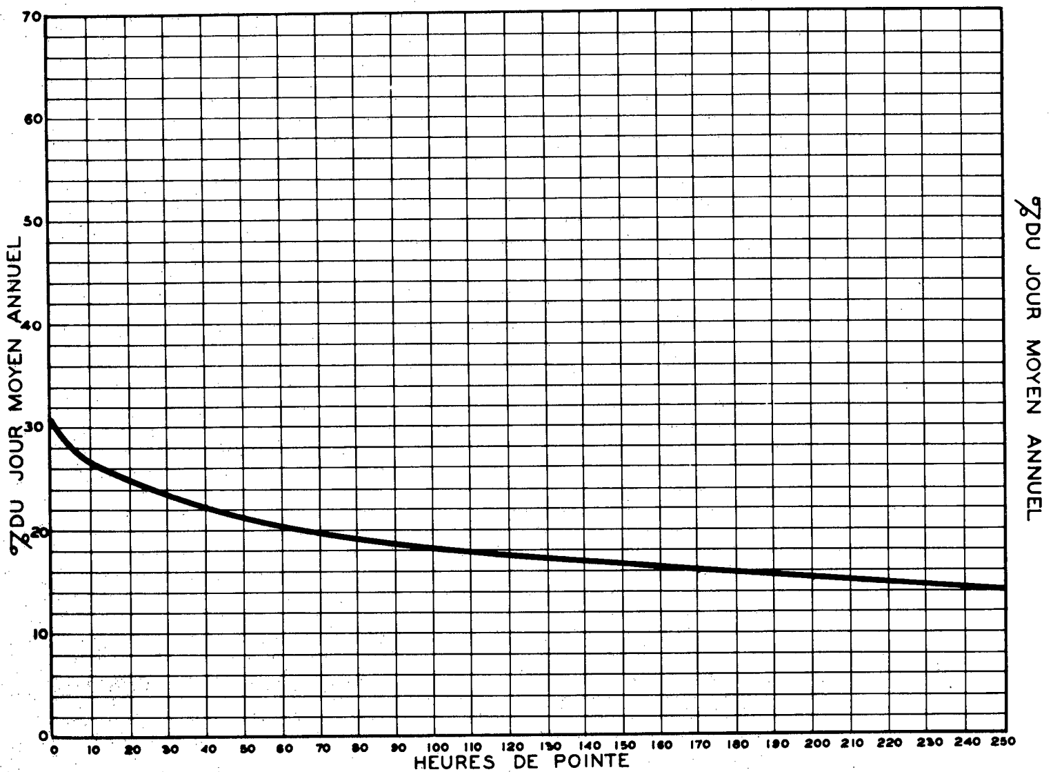
RELATION ENTRE LES HEURES DE POINTE ET LE JOUR MOYEN ANNUEL STATION: VILLEROY (HALTE ROUTIERE) NORD ROUTE N° R-S-303
