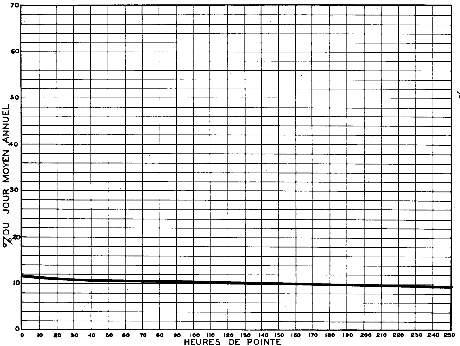
RELATION ENTRE LES HEURES DE POINTE ET LE JOUR MOYEN ANNUEL — STATION: SILLERY (BOUL. LAURIER) — ROUTE N° R-S-169 —
