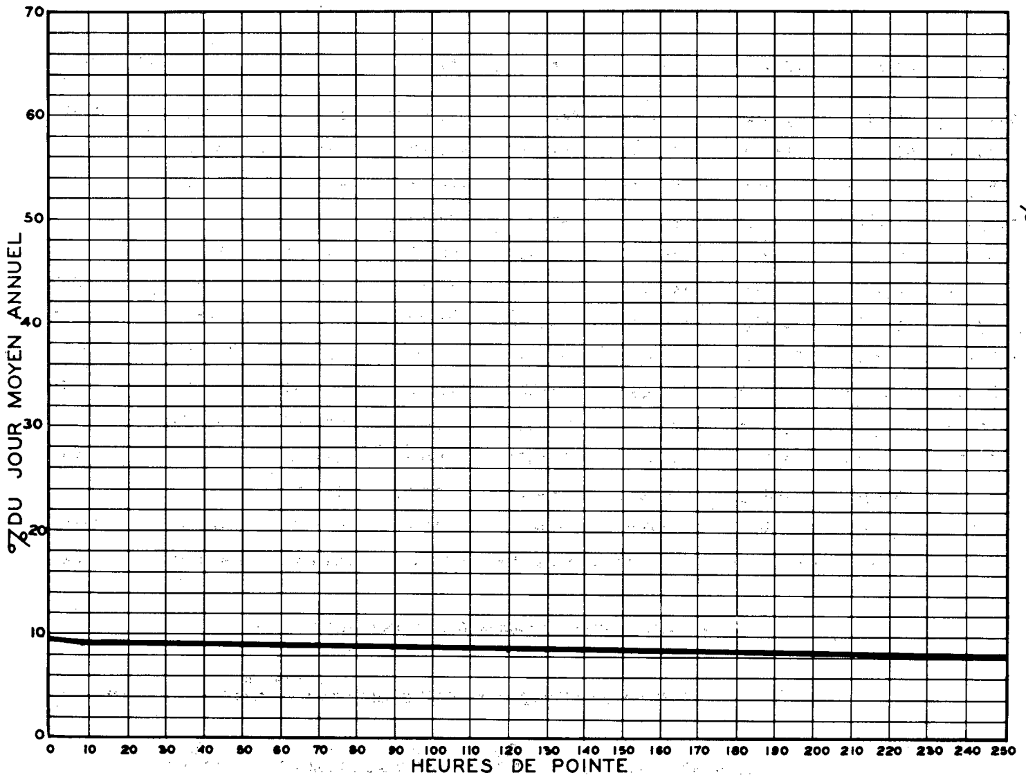
RELATION ENTRE LES HEURES DE POINTE ET LE JOUR MOYEN ANNUEL — STATION: MONTREAL BOUL. DECARIE ROUTE N° 15-4-50 (EST)
