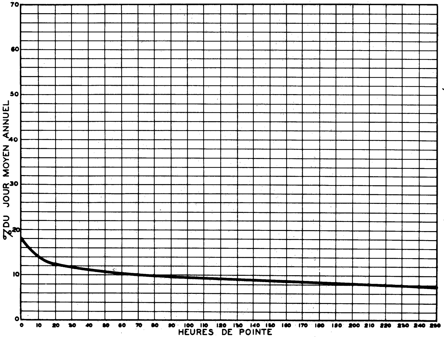
RELATION ENTRE LES HEURES DE POINTE ET LE JOUR MOYEN ANNUEL — STATION: ST-NICOLAS ROUTE N°20-1-11 (SUD)
