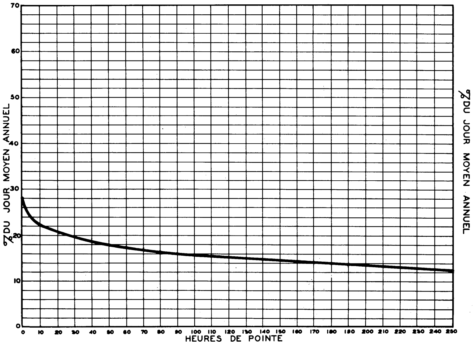
RELATION ENTRE LES HEURES DE POINTE ET LE JOUR MOYEN ANNUEL STATION: STE-ROSE-DU-DEGELIS ROUTE N° 2-2-4
