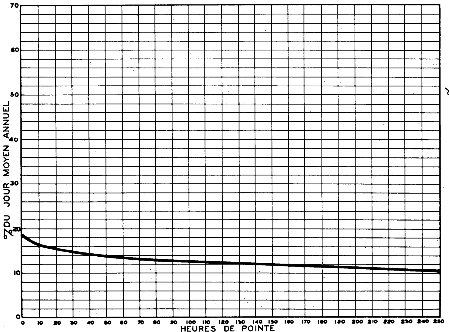
RELATION ENTRE LES HEURES DE POINTE ET LE JOUR MOYEN ANNUEL — STATION: MAGOG ROUTE N° 1-3-4 (NORD)
