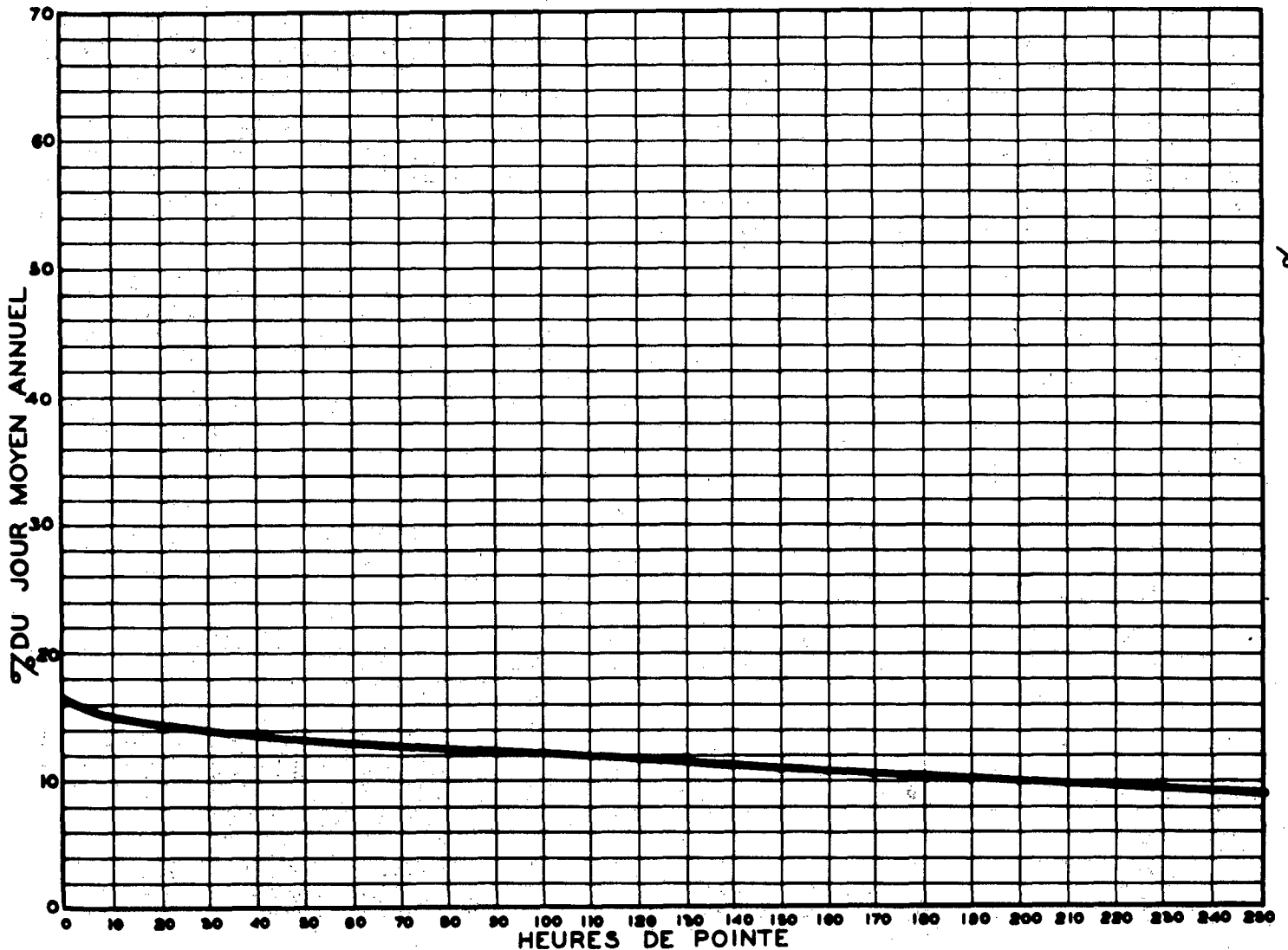
RELATION ENTRE LES HEURES DE POINTE ET LE JOUR MOYEN ANNUEL — STATION: ILE PERROT PONT GALIPEAULT — ROUTE N° 2-4-54 (SUD)
