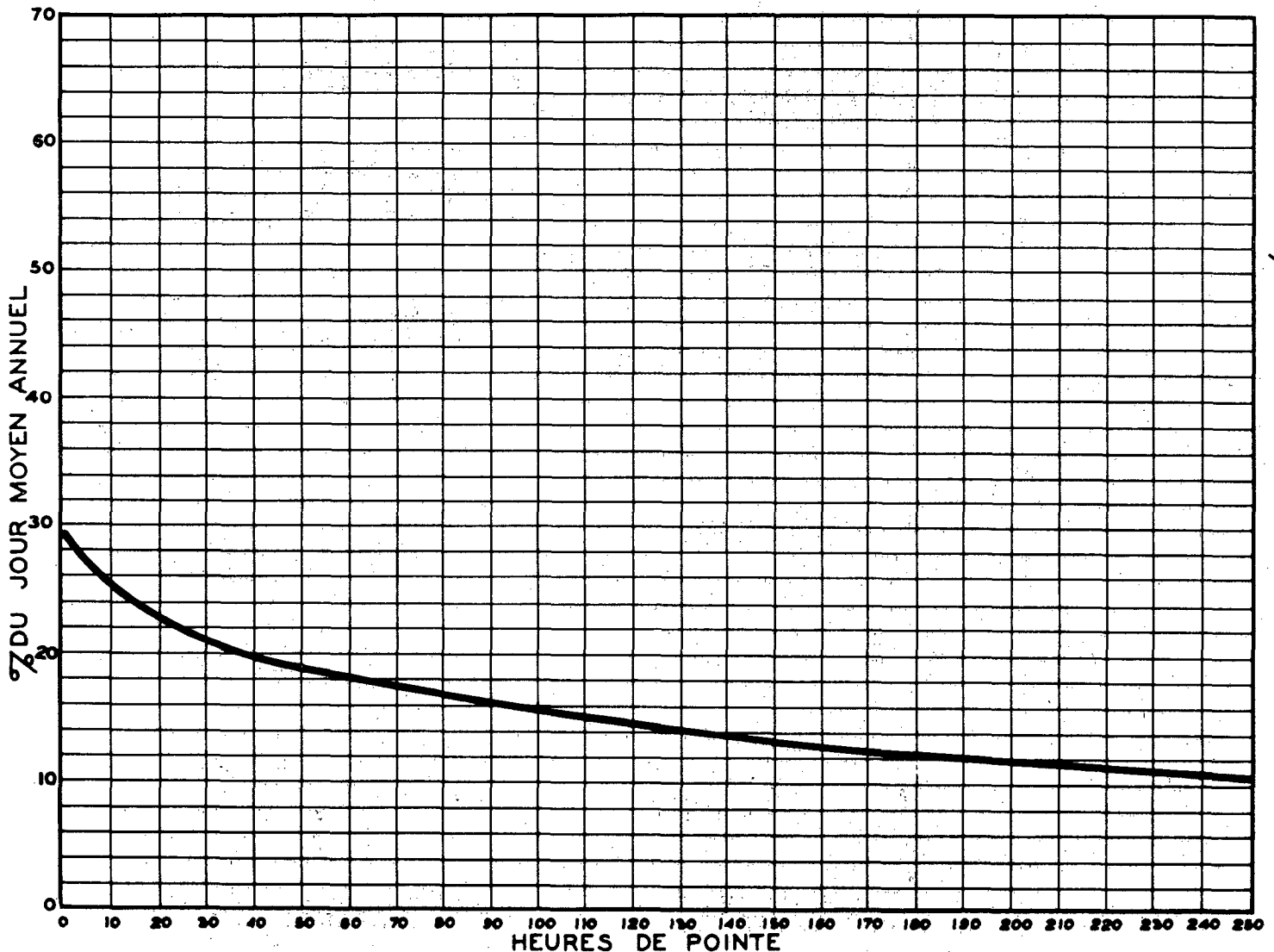
RELATION ENTRE LES HEURES DE POINTE ET LE JOUR MOYEN ANNUEL — STATION: VAUDREUIL ROUTE N° 40-4-89 (SUD)
