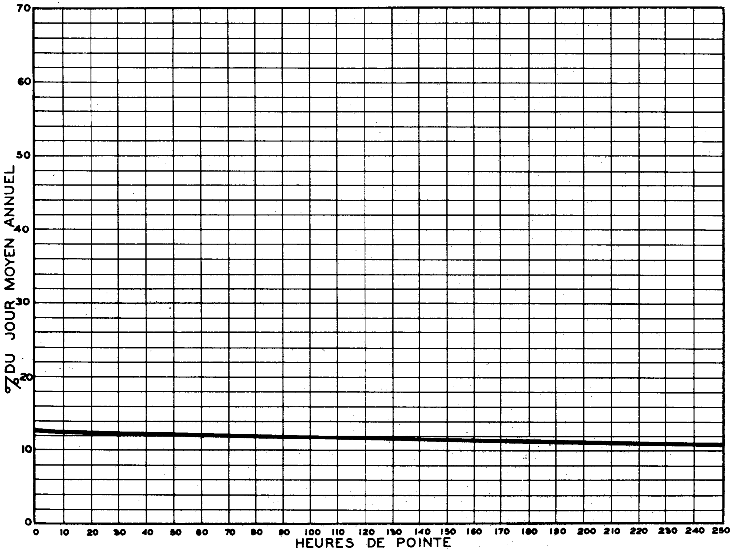
RELATION ENTRE LES HEURES DE POINTE ET LE JOUR MOYEN ANNUEL — STATION: LAVAL ROUTE N°11-4-80 (EST)
