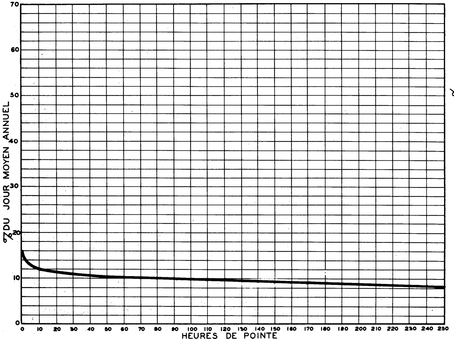
RELATION ENTRE LES HEURES DE POINTE ET LE JOUR MOYEN ANNUEL — STATION: ST-LAURENT DE MATAPEDIA ROUTE N° R-S-203
