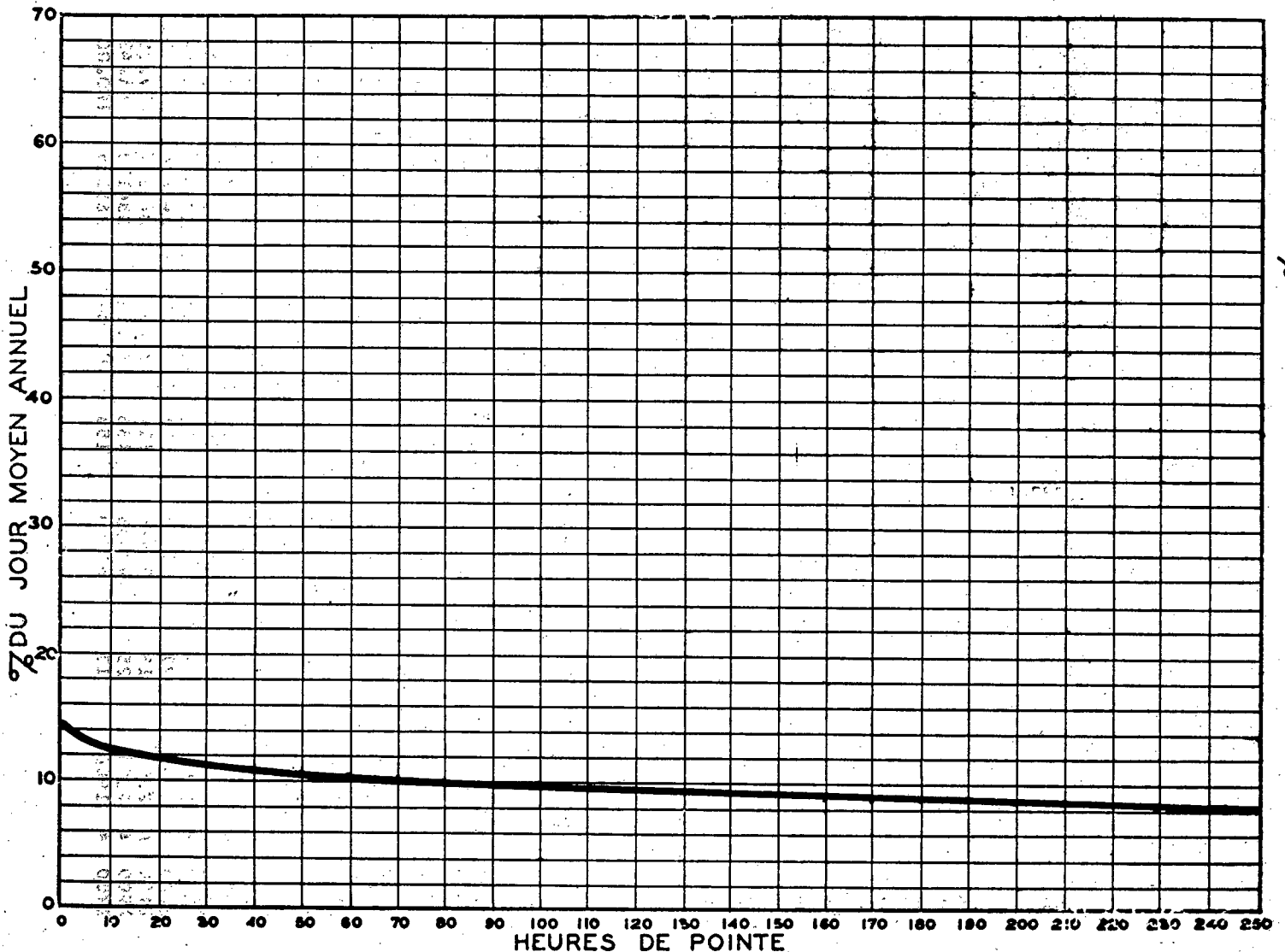
RELATION ENTRE LES HEURES DE POINTE ET LE JOUR MOYEN ANNUEL STATION: STE-EULALIE ROUTE N° 34-8-1
