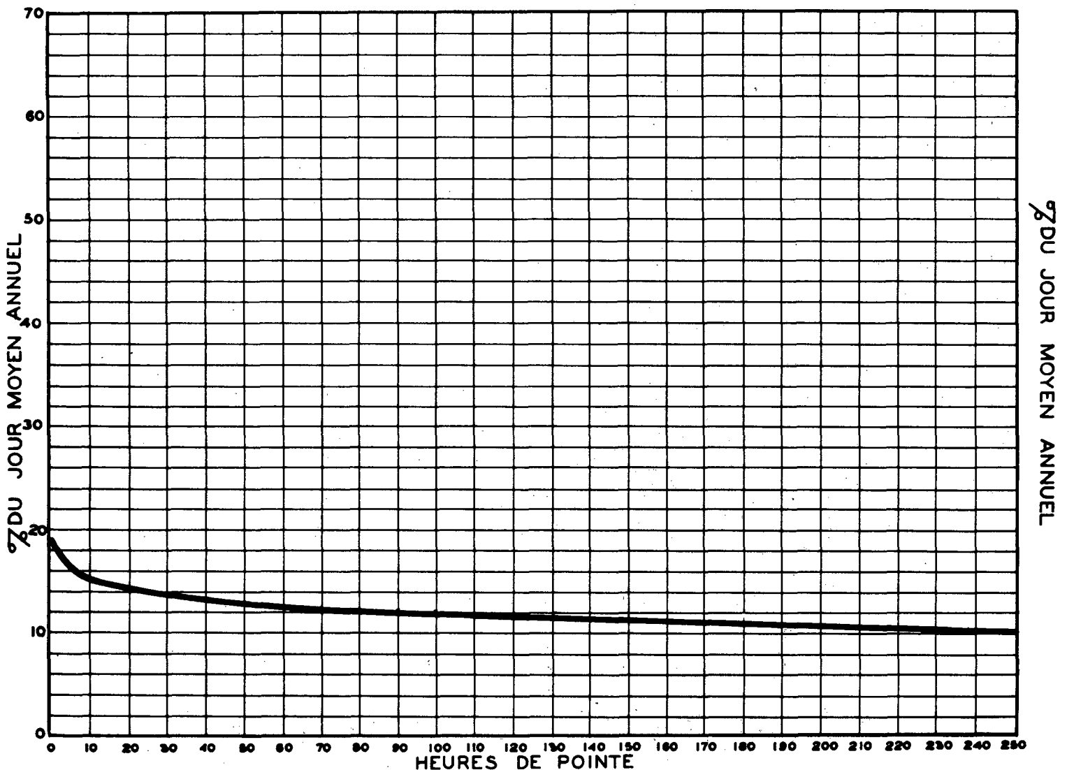
RELATION ENTRE LES HEURES DE POINTE ET LE JOUR MOYEN ANNUEL STATION: ST-LUC ROUTE N° 7-9-84
