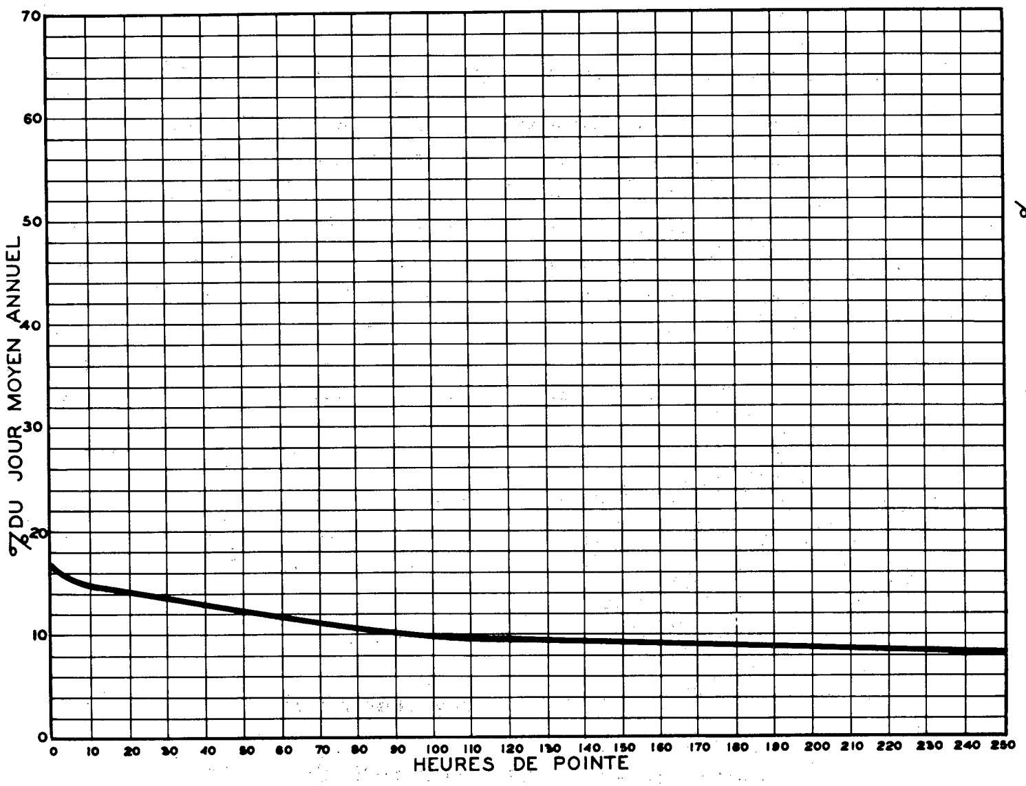
RELATION ENTRE LES HEURES DE POINTE ET LE JOUR MOYEN ANNUEL STATION: TERREBONNE ROUTE N° 25-4-51
