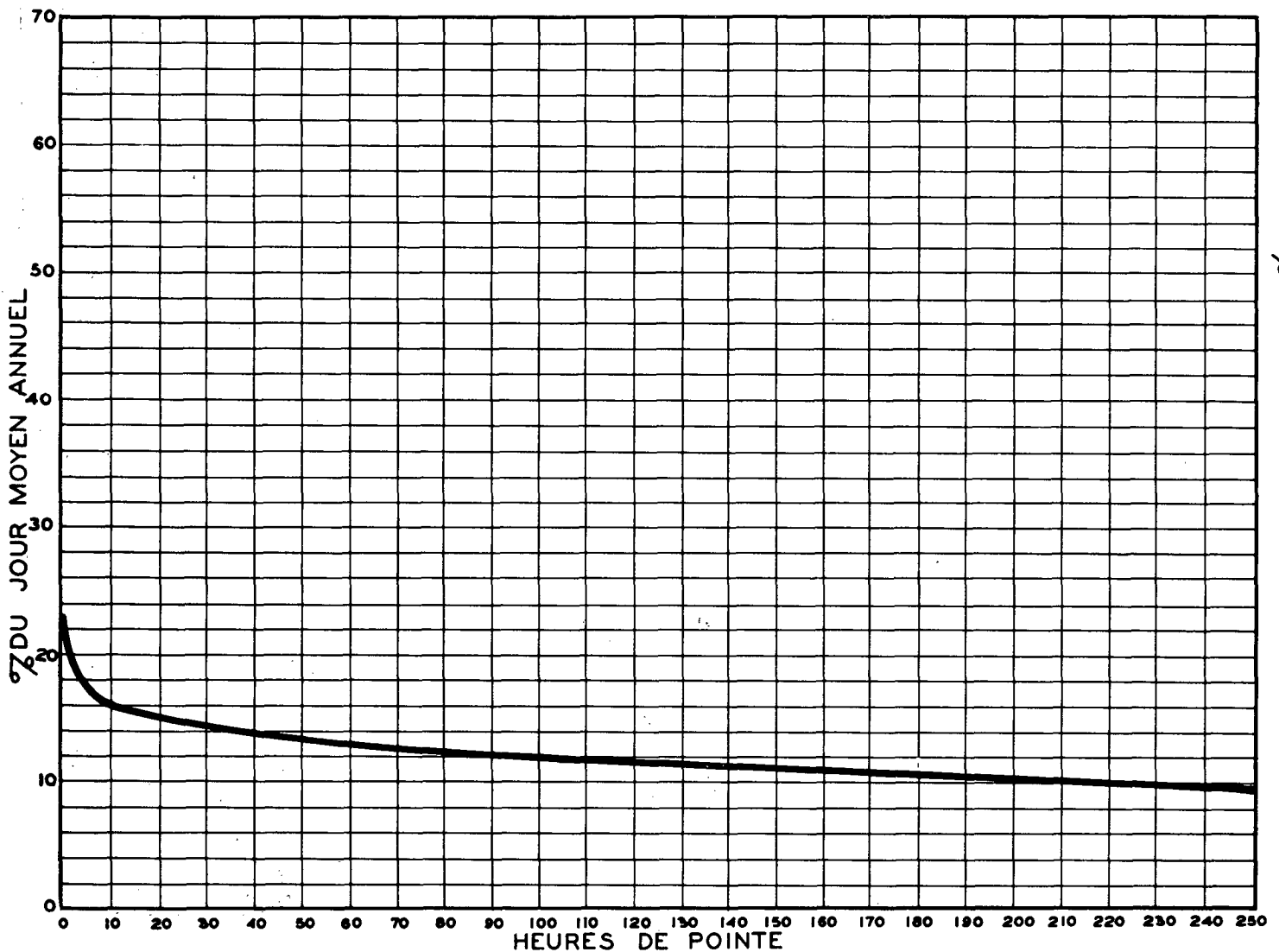
RELATION ENTRE LES HEURES DE POINTE ET LE JOUR MOYEN ANNUEL STATION: ST-GREGOIRE (PONT DE TROIS-RIVIERES) OUESTROUTE N° R-S-815
