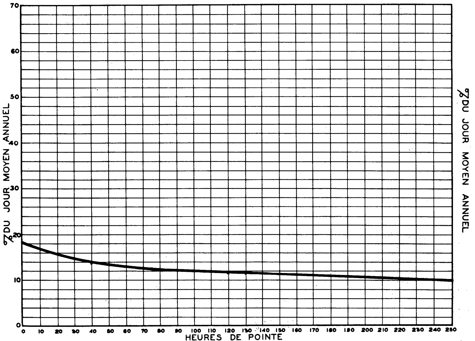
RELATION ENTRE LES HEURES DE POINTE ET LE JOUR MOYEN ANNUEL STATION: ANCIENNE-LORETTE ROUTE N° 2-1-7 (NORD)
