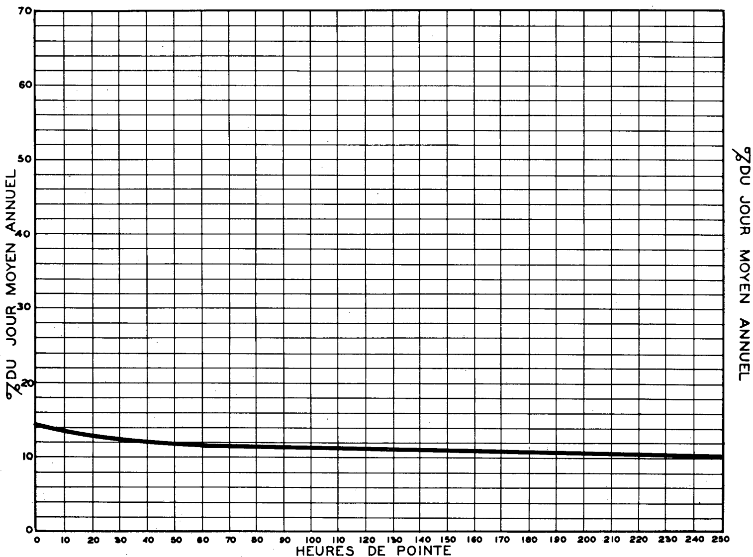
RELATION ENTRE LES HEURES DE POINTE ET LE JOUR MOYEN ANNUEL STATION: CHARLESBOURG-OUEST (BOUL. P. BERTRAND) ROUTE N° R-S-178
