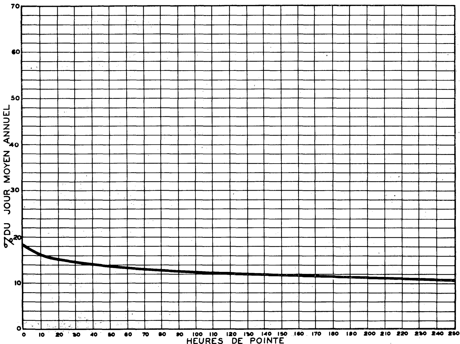
RELATION ENTRE LES HEURES DE POINTE ET LE JOUR MOYEN ANNUEL — STATION: VAUDREUIL ROUTE N° 40-4-89 (2 VOIES)
