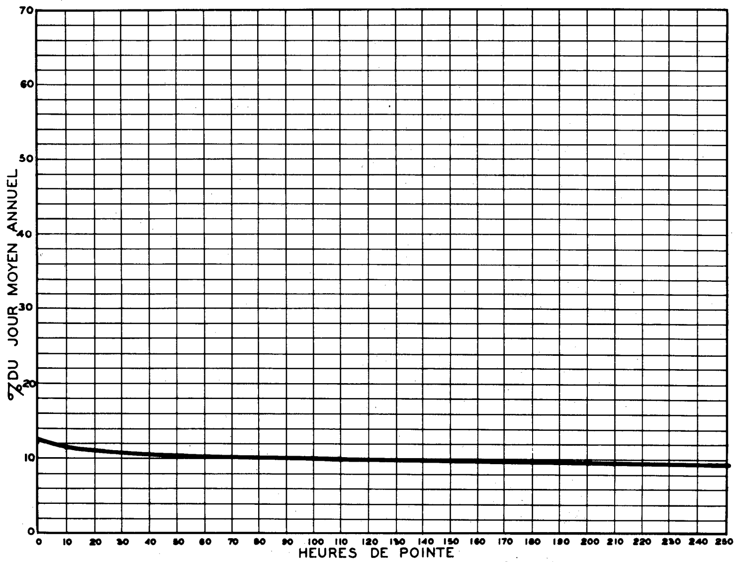
RELATION ENTRE LES HEURES DE POINTE ET LE JOUR MOYEN ANNUEL — STATION: BOUCHERVILLE ROUTE N° 20-9-81 (2 VOIES)
