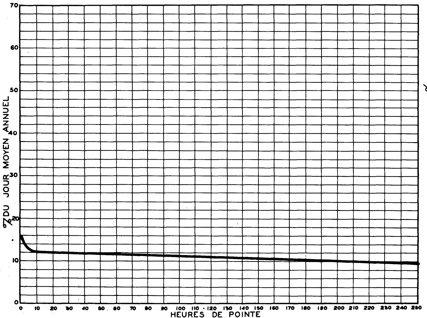
RELATION ENTRE LES HEURES DE POINTE ET LE JOUR MOYEN ANNUEL STATION: LAVAL PONT LACHAPELLE ROUTE N° 11-4-81 (EST)
