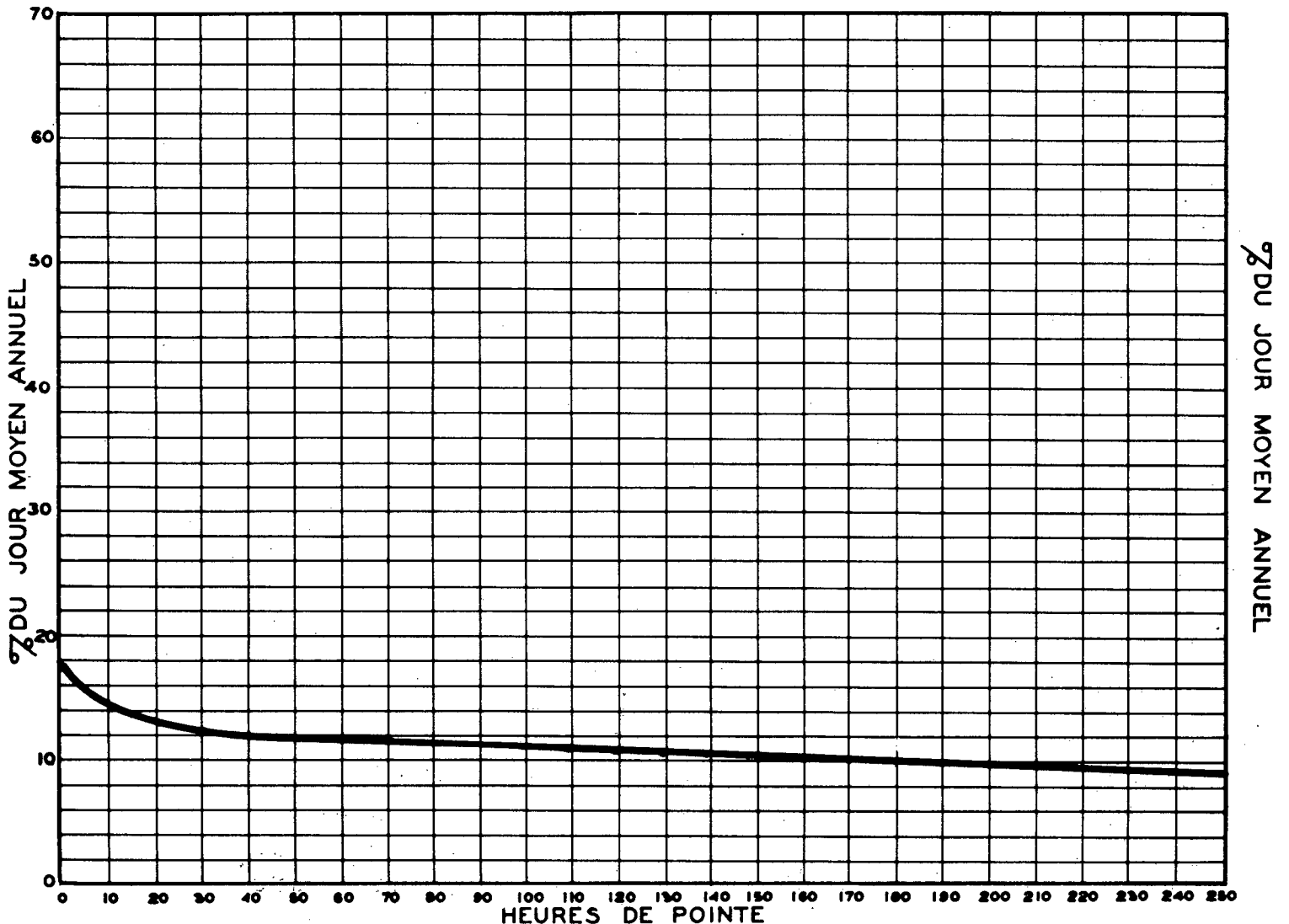
RELATION ENTRE LES HEURES DE POINTE ET LE JOUR MOYEN ANNUEL STATION: ST-TIMOTHEE ROUTE N° 3-4-57
