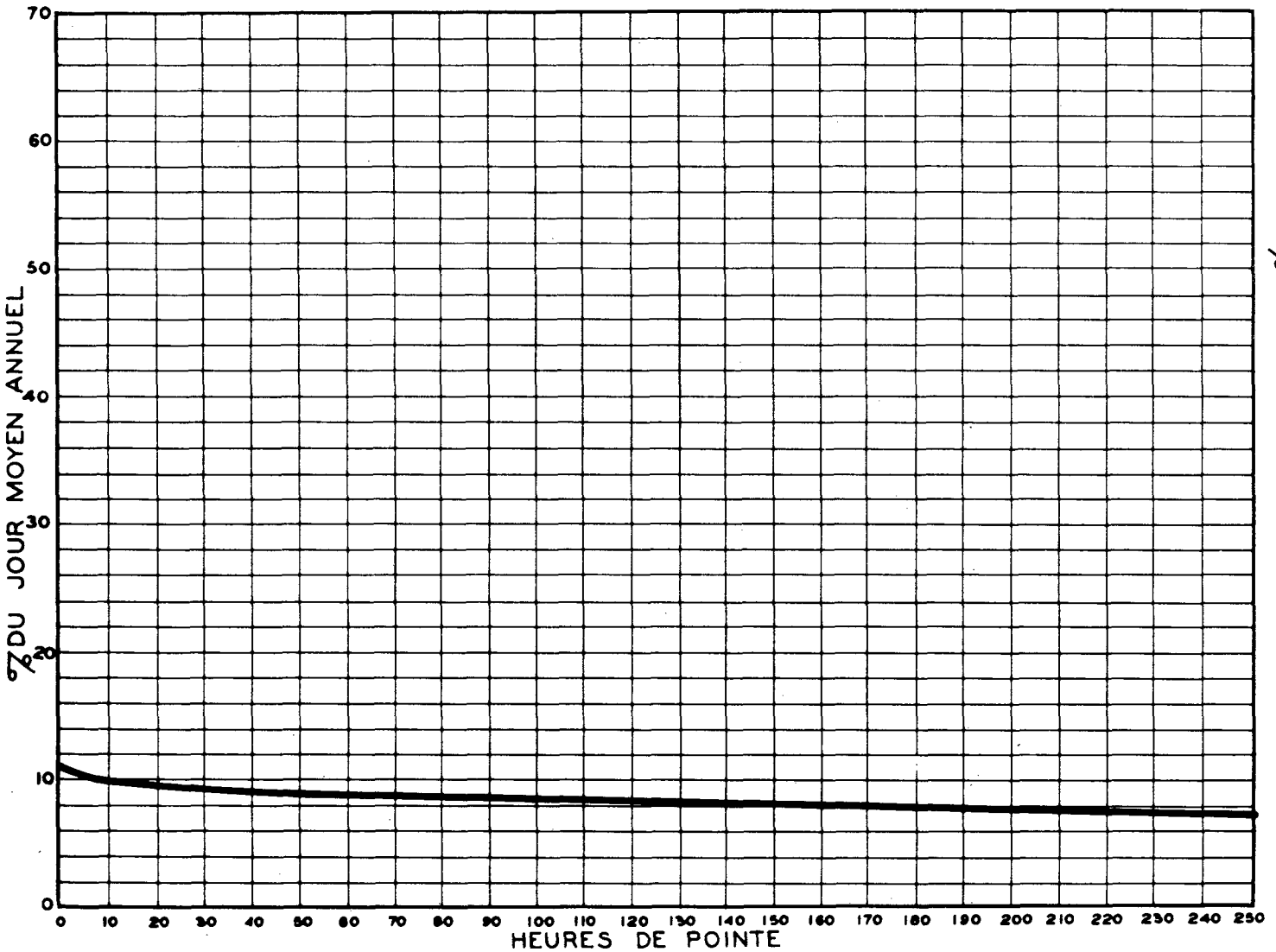
RELATION ENTRE LES HEURES DE POINTE ET LE JOUR MOYEN ANNUEL STATION: SHERBROOKE ROUTE N° 5-22-3-12 (OUEST)
