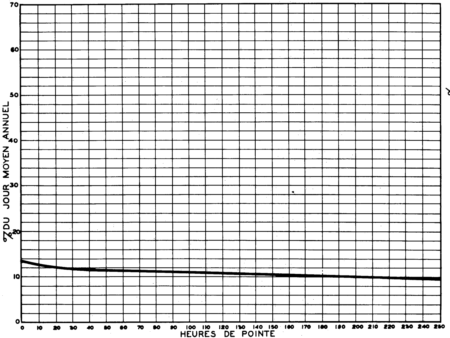
RELATION ENTRE LES HEURES DE POINTE ET LE JOUR MOYEN ANNUEL — STATION: BOUCHERVILLE ROUTE N° 20-9-81 (SUD)
