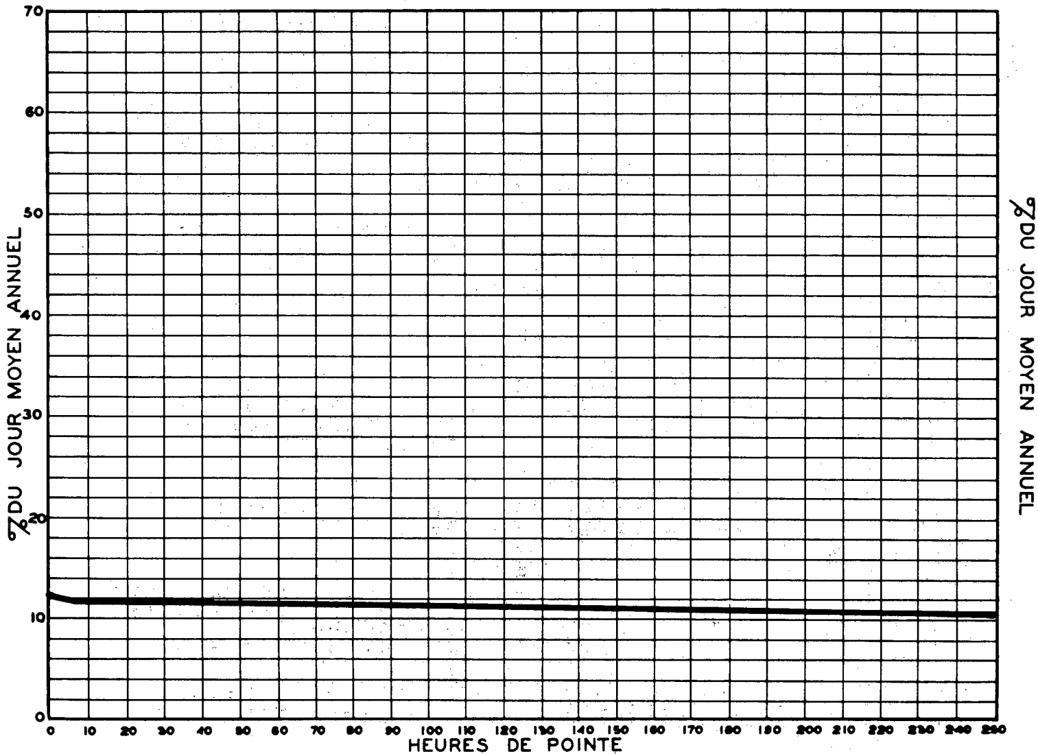
RELATION ENTRE LES HEURES DE POINTE ET LE JOUR MOYEN ANNUEL — STATION: ST-NICOLAS ROUTE N°2-9-1-6 (QUEST)
