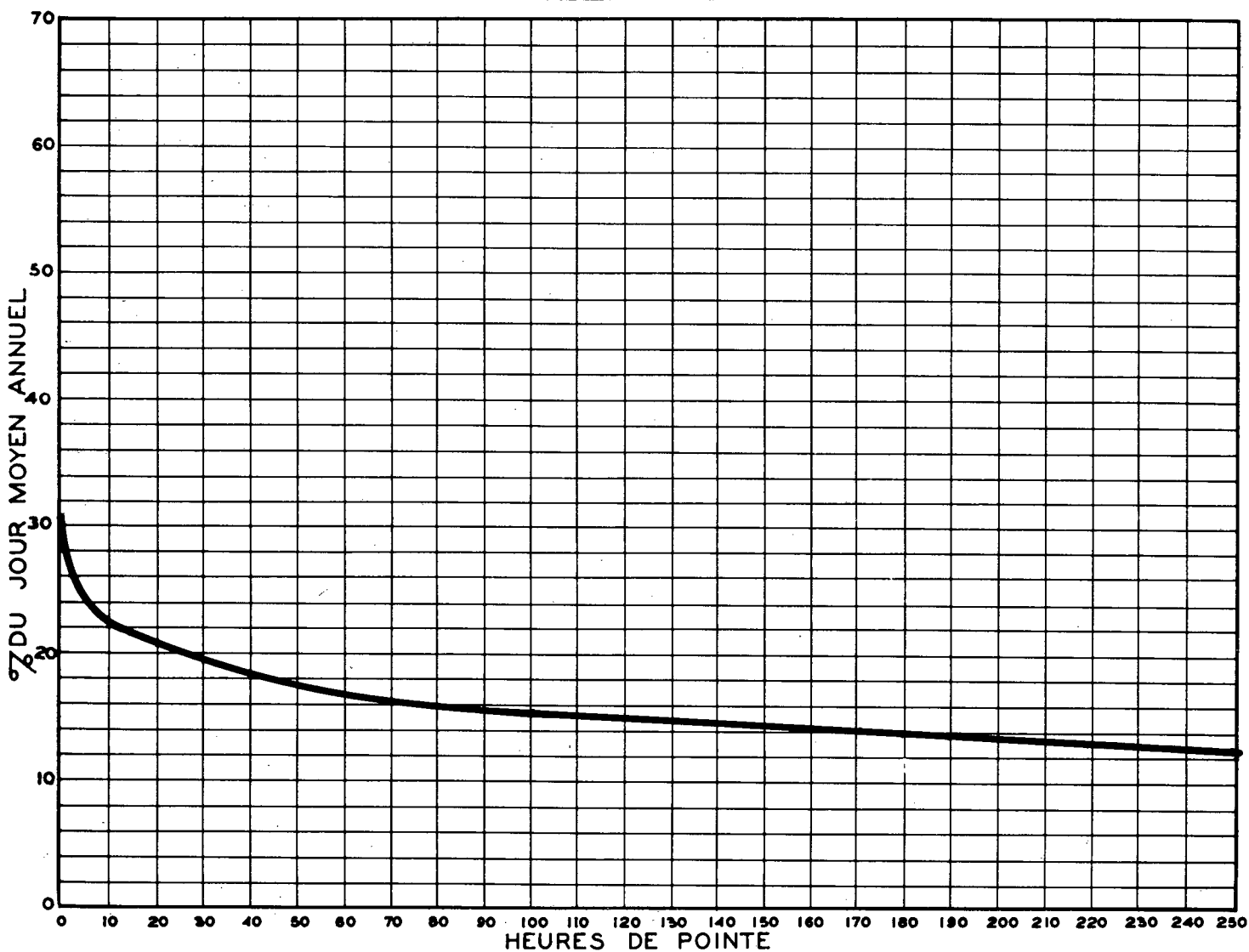
RELATION ENTRE LES HEURES DE POINTE ET LE JOUR MOYEN ANNUEL — STATION: MONTMORENCY ROUTE N° R-S-120
