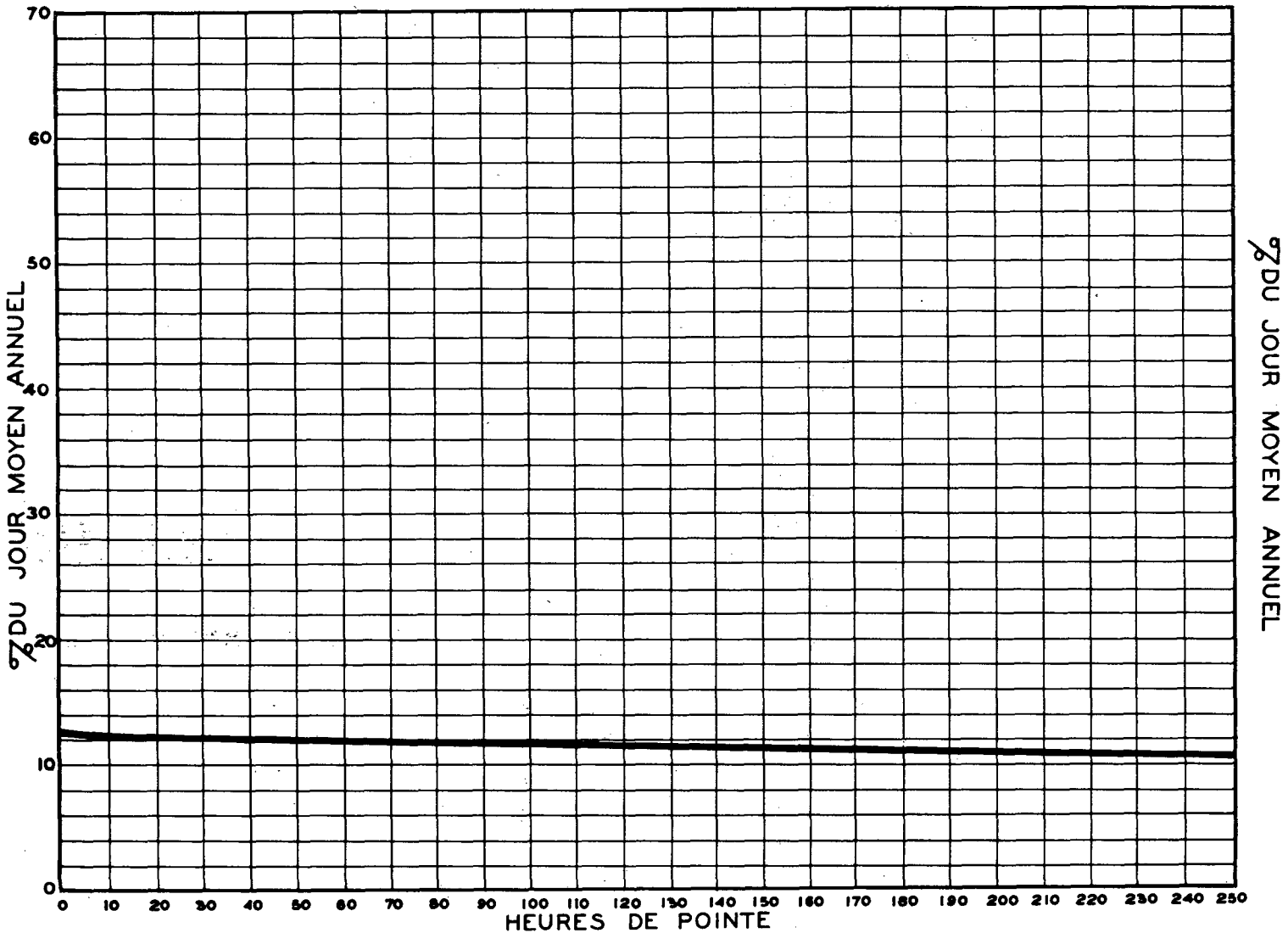
RELATION ENTRE LES HEURES DE POINTE ET LE JOUR MOYEN ANNUEL — STATION: LAVAL ROUTE N° 11-4-80 (OUEST)
