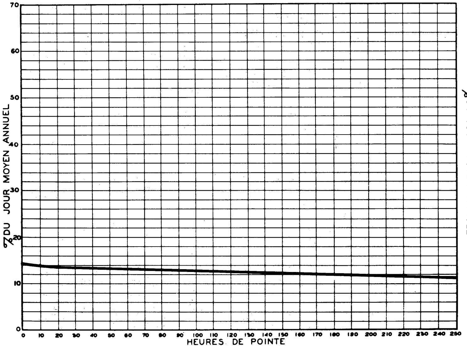
RELATION ENTRE LES HEURES DE POINTE ET LE JOUR MOYEN ANNUEL — STATION: LONGUEUIL PONT JACQUES CARTIER ROUTE N° 9-9-50 NORD
