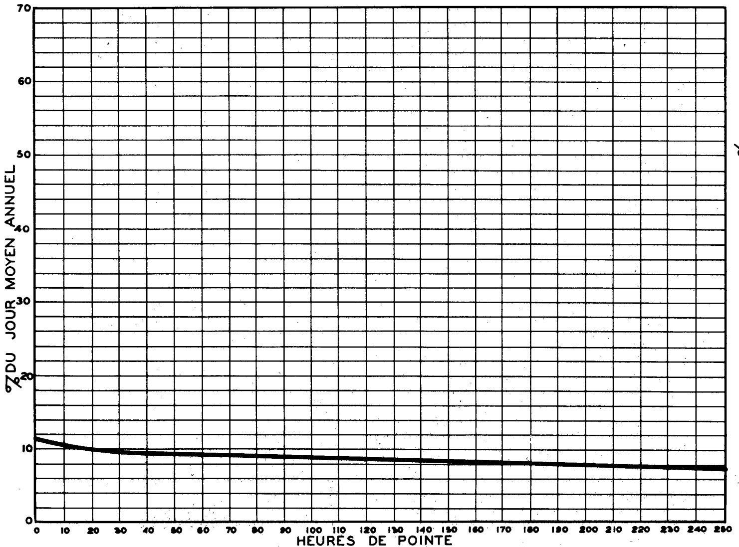
RELATION ENTRE LES HEURES DE POINTE ET LE JOUR MOYEN ANNUEL — STATION: SHERBROOKE ROUTE N° 1-3-4 (NORD)
