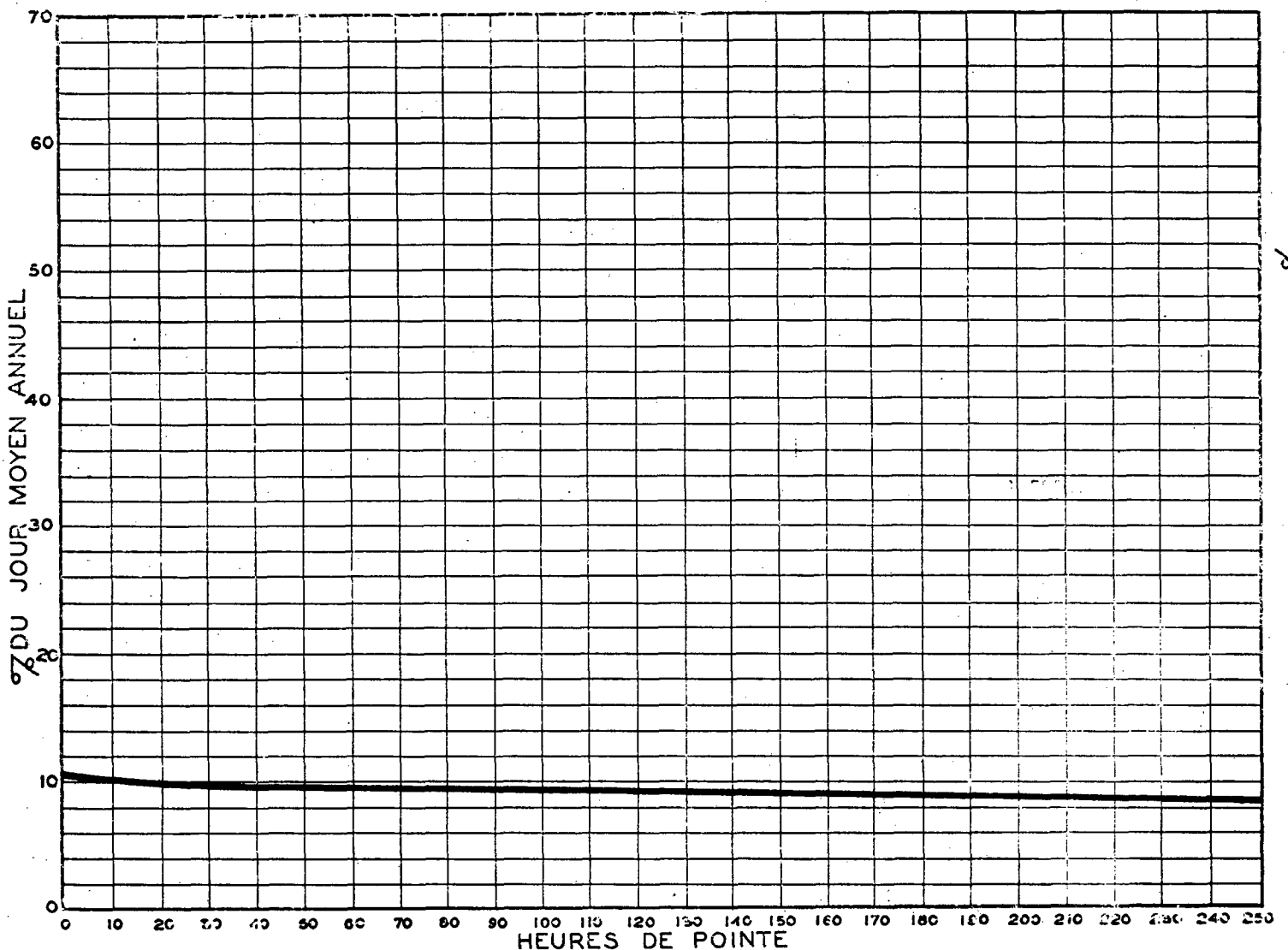
RELATION ENTRE LES HEURES DE POINTE ET LE JOUR MOYEN ANNUEL STATION: ST-LEONARD ROUTE N° 40-4-86 (NORD)
