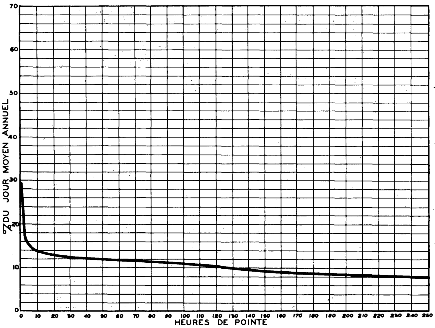
RELATION ENTRE LES HEURES DE POINTE ET LE JOUR MOYEN ANNUEL — STATION: STE-CLOTHILDE-DE-HORTON ROUTE N° 20-8-3
