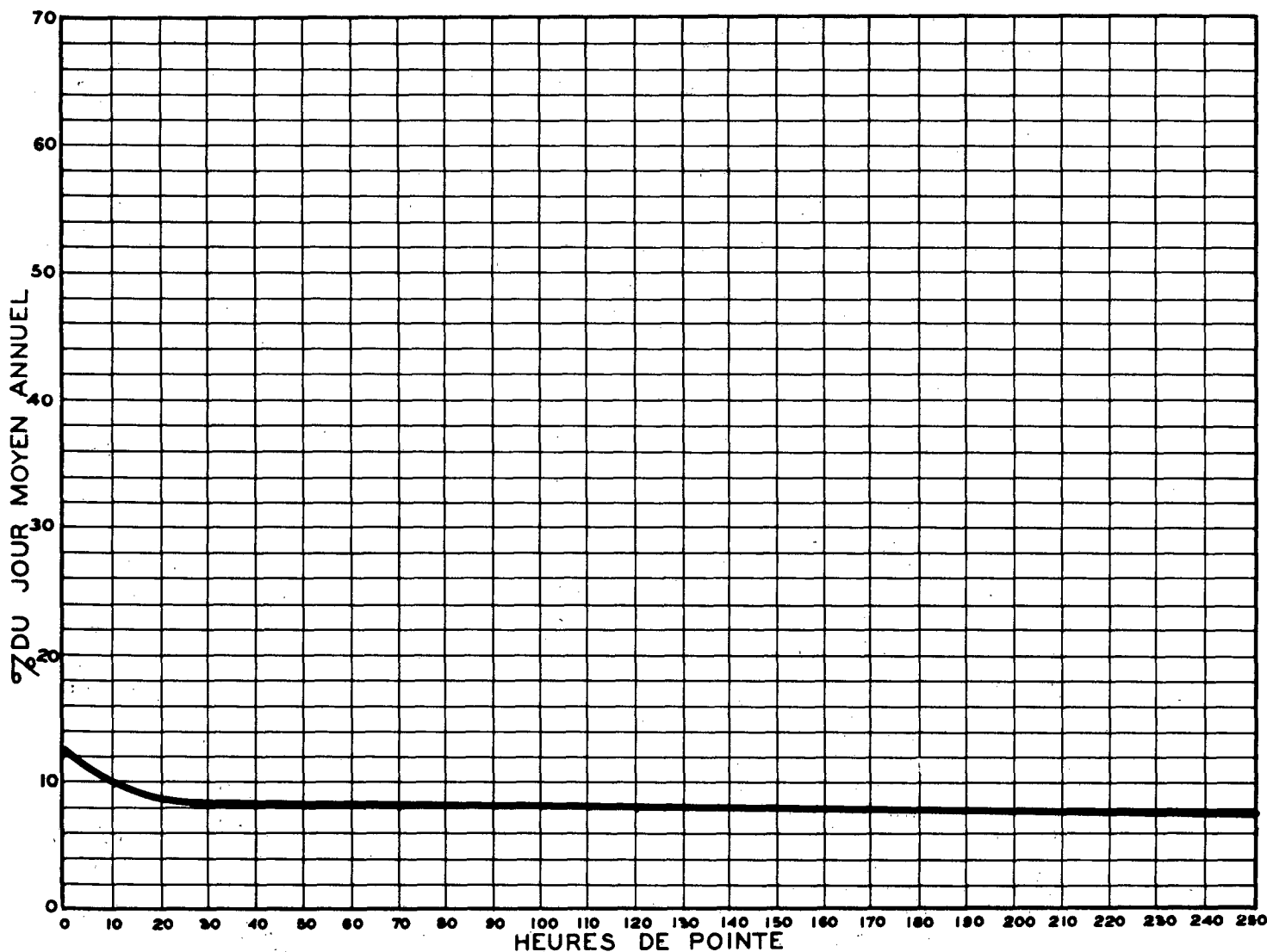
RELATION ENTRE LES HEURES DE POINTE ET LE JOUR MOYEN ANNUEL STATION: LAVAL PONT LACHAPELLE ROUTE N° 11-4-81 (2 VOIES)
