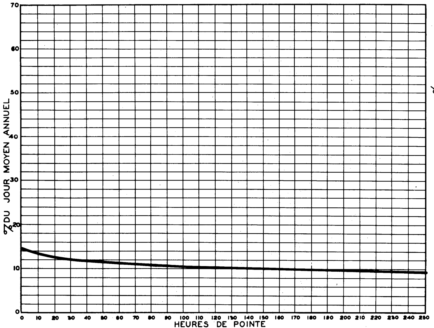
RELATION ENTRE LES HEURES DE POINTE ET LE JOUR MOYEN ANNUEL — STATION: BOUCHERVILLE ROUTE N° 20-9-81 (NORD)
