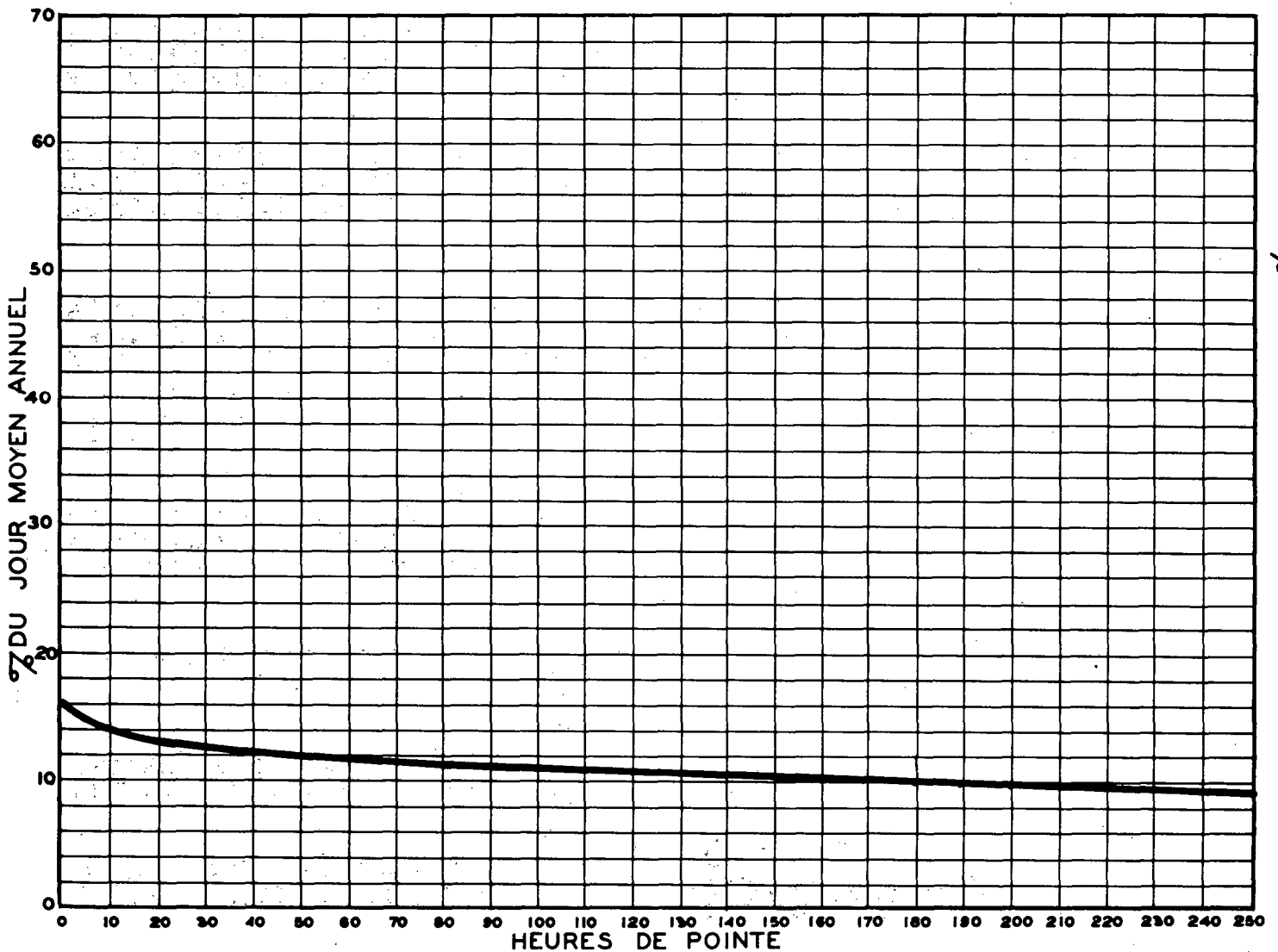
RELATION ENTRE LES HEURES DE POINTE ET LE JOUR MOYEN ANNUEL STATION: LINIÈRE ROUTE N° 23-3-1
