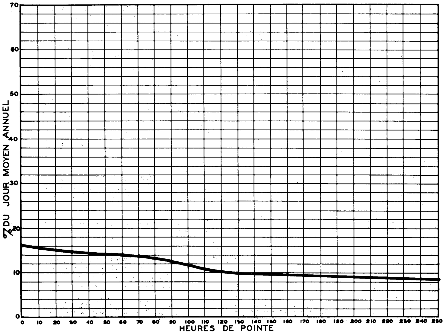
RELATION ENTRE LES HEURES DE POINTE ET LE JOUR MOYEN ANNUEL — STATION: POINTE-AUX-TREMBLES ROUTE N° 2-4-85 (OUEST)
