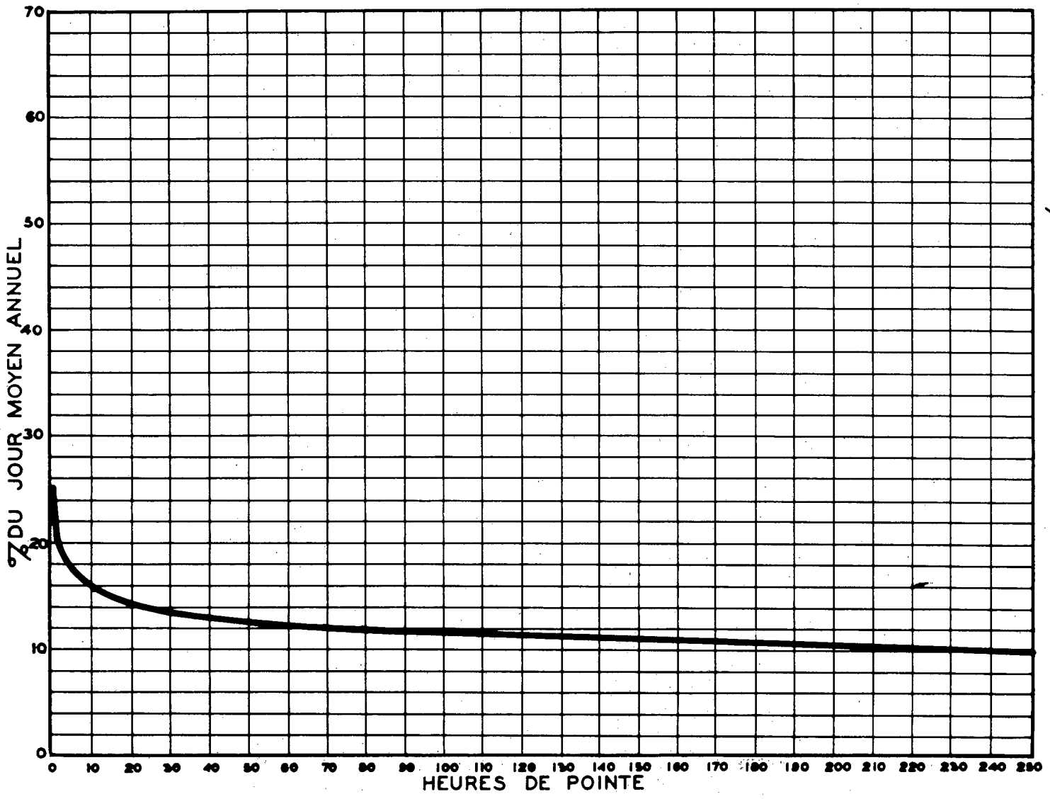
RELATION ENTRE LES HEURES DE POINTE ET LE JOUR MOYEN ANNUEL — STATION: VILLEROY ROUTE N° 20-3-1 (NORD)
