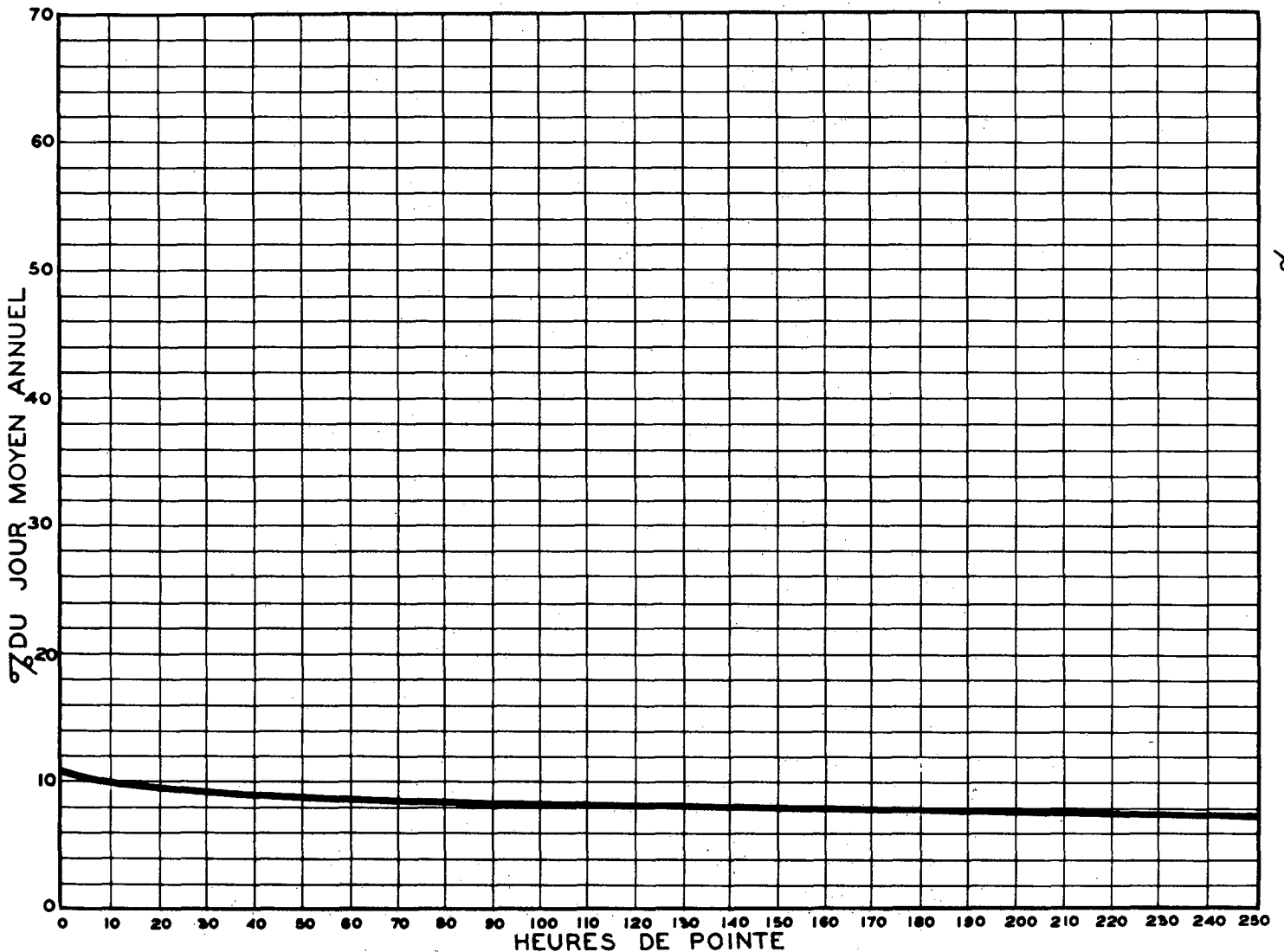
RELATION ENTRE LES HEURES DE POINTE ET LE JOUR MOYEN ANNUEL — STATION: SHERBROOKE ROUTE N° 5-22-3-12 (EST)
