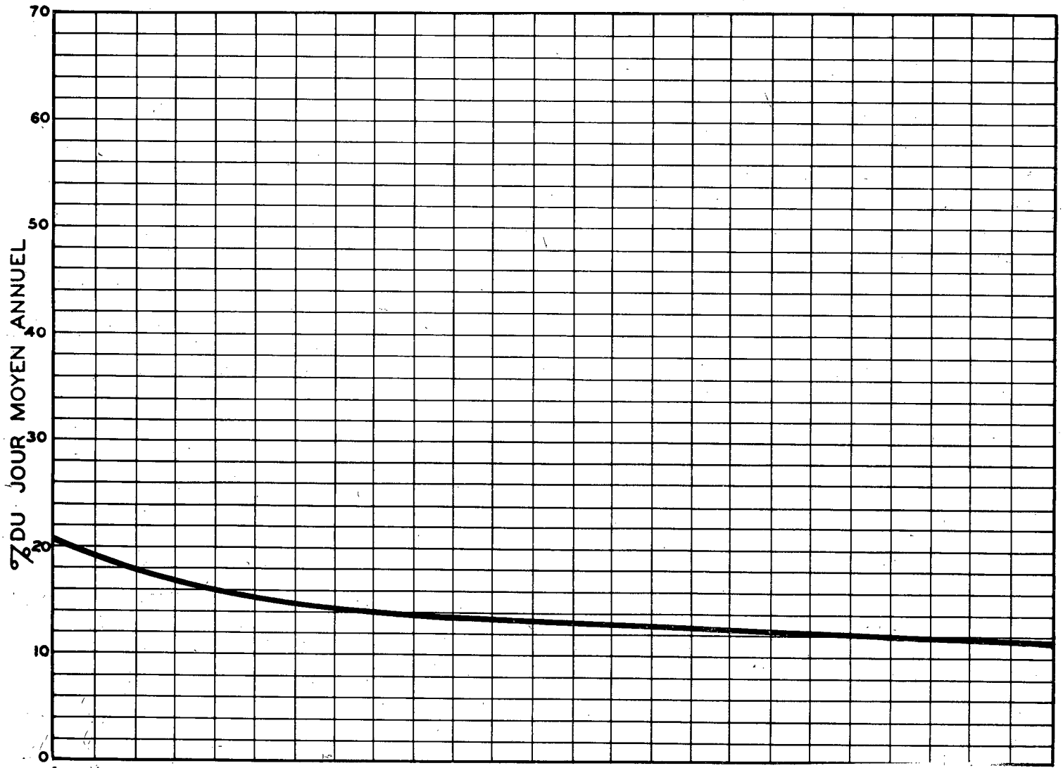
RELATION ENTRE LES HEURES DE POINTE ET LE JOUR MOYEN ANNUEL STATION: BATISCAN ROUTE N° 2-10-9
