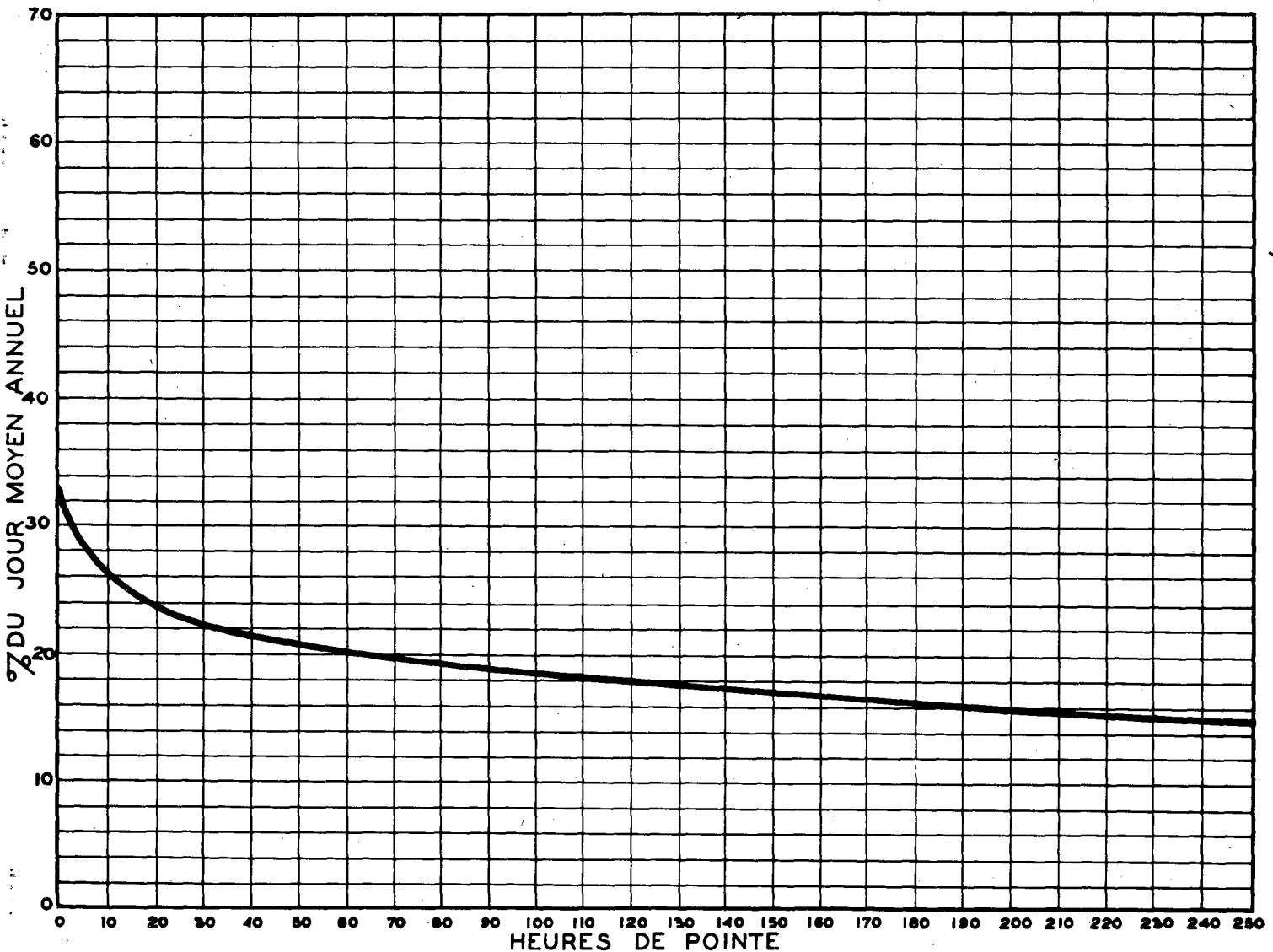
RELATION ENTRE LES HEURES DE POINTE ET LE JOUR MOYEN ANNUEL STATION: ST-MATHIEU-DE-DIXVILLE ROUTE N° 22-3-4
