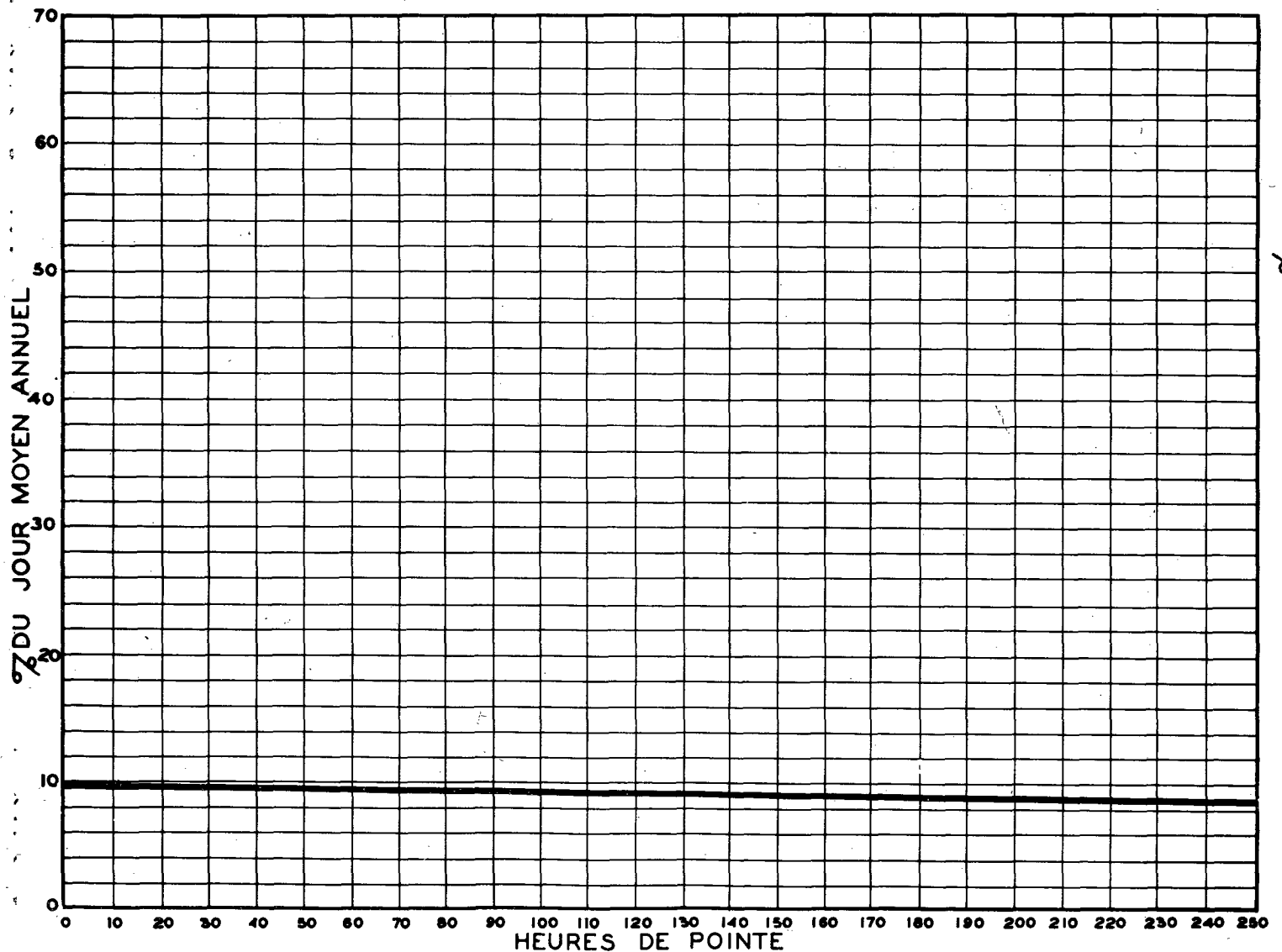
RELATION ENTRE LES HEURES DE POINTE ET LE JOUR MOYEN ANNUEL STATION: MONTREAL 2 voies BOUL. DECARIE ROUTE N°15-4-50
