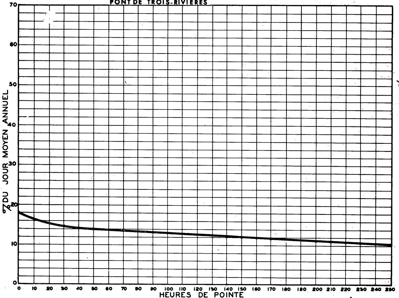
RELATION ENTRE LES HEURES DE POINTE ET LE JOUR MOYEN ANNUEL STATION: ST-GREGOIRE 2 voies PONT DE TROIS-RIVIERES ROUTE N° 8-15
