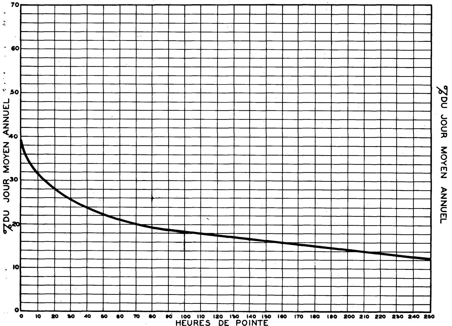
RELATION ENTRE LES HEURES DE POINTE ET LE JOUR MOYEN ANNUEL STATION: ST-MARC ROUTE N° 47-9-51
