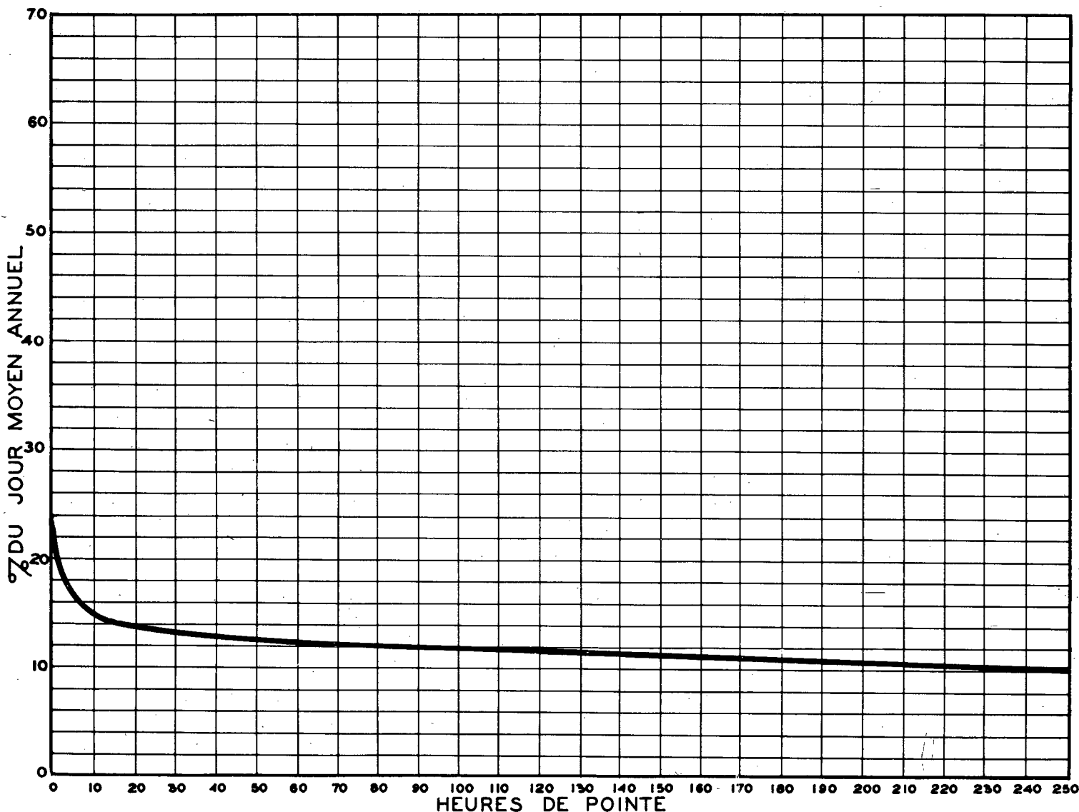
RÉLATION ENTRE LES HEURES DE POINTE ET LE JOUR MOYEN ANNUEL — STATION: MAGOG voie sud ROUTE N° 1-3-3
