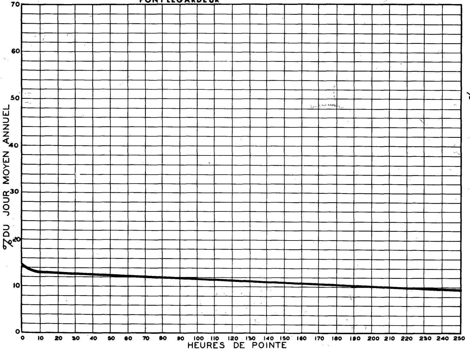
RELATION ENTRE LES HEURES DE POINTE ET LE JOUR MOYEN ANNUEL STATION: POINTE-AUX-TREMBLES voie est ROUTE N° 2-4-85 PONT LE GARDEUR
