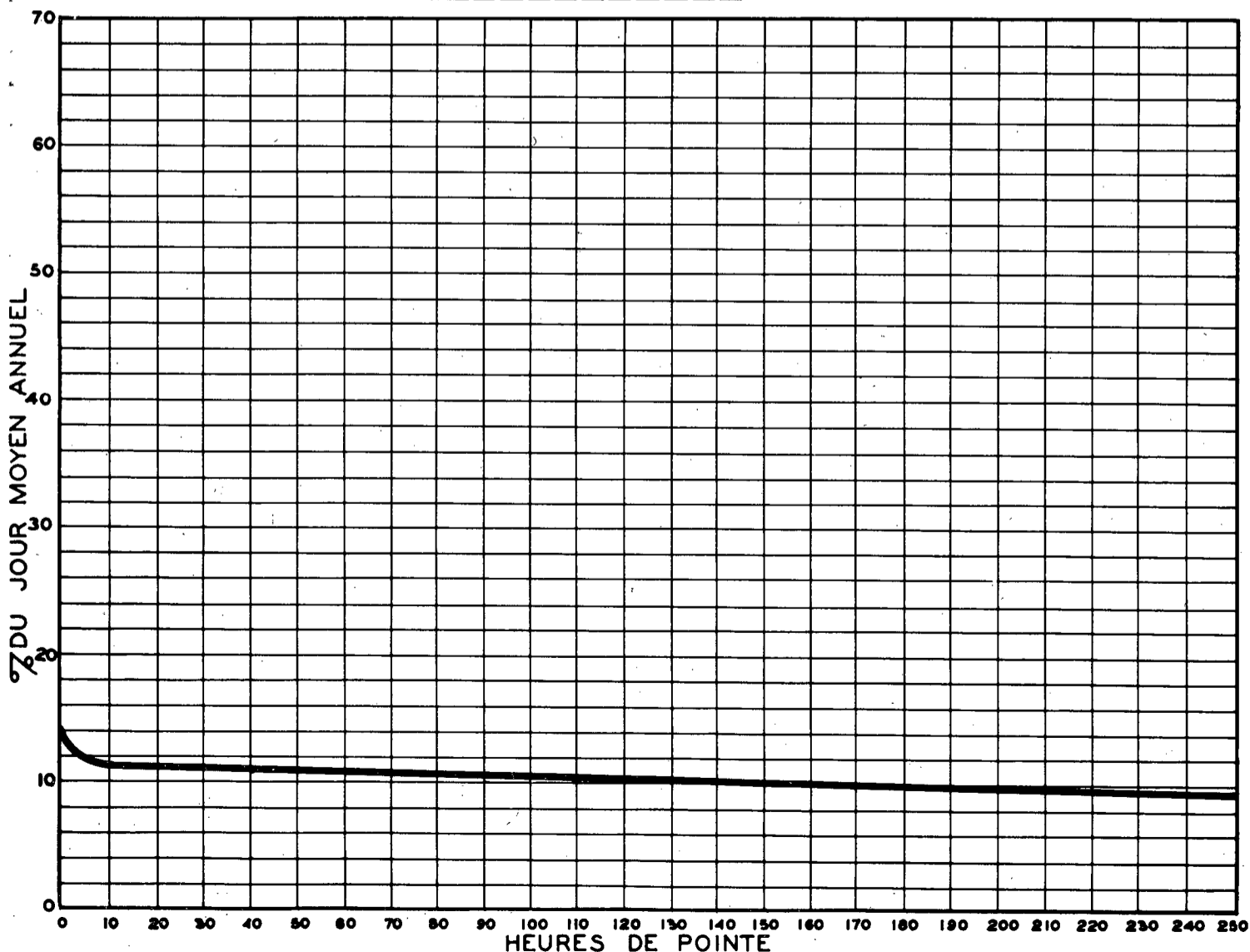
RELATION ENTRE LES HEURES DE POINTE ET LE JOUR MOYEN ANNUEL STATION: SILLERY BOUL. LAURIER ROUTE N° 1-69
