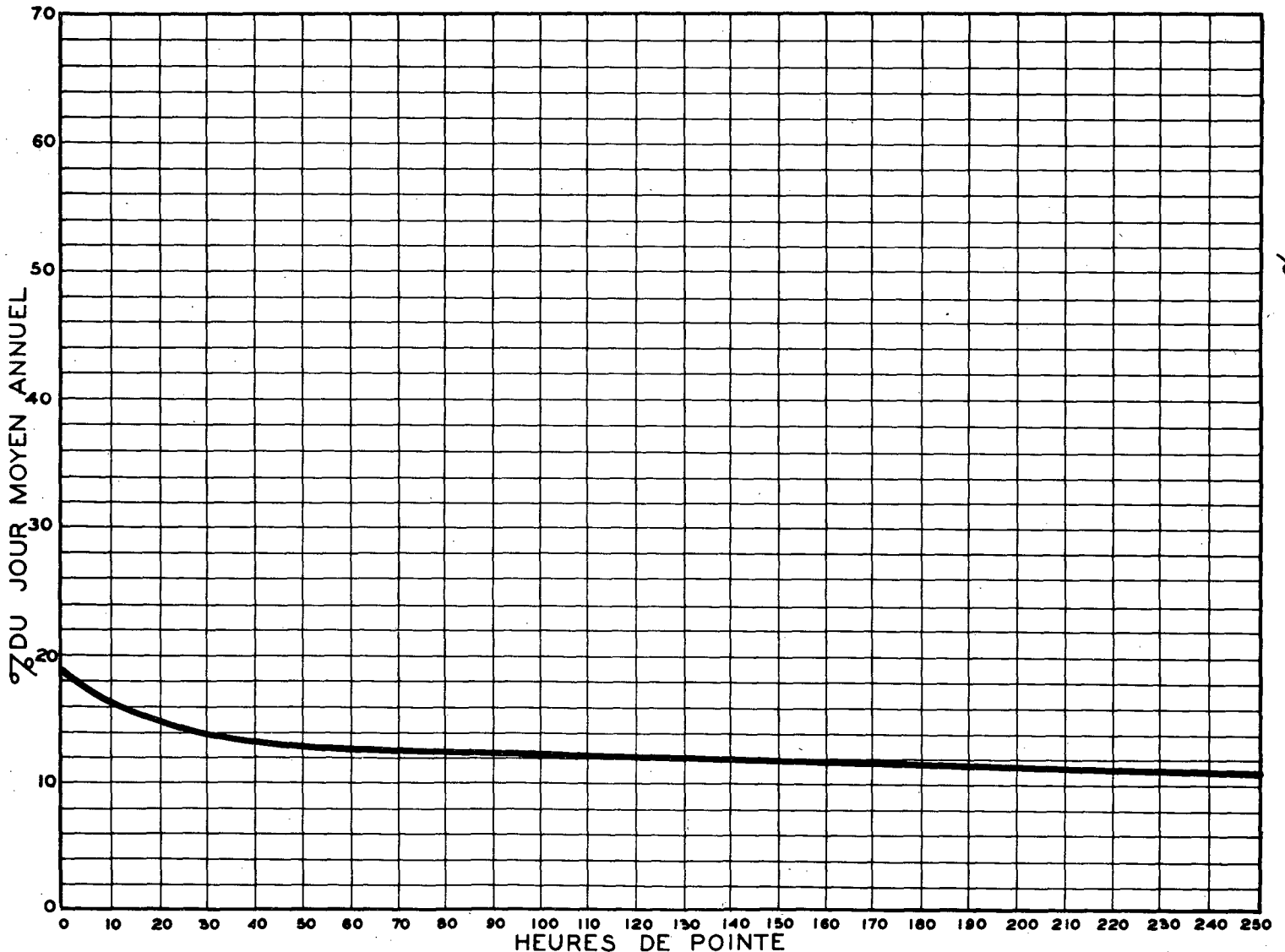
RELATION ENTRE LES HEURES DE POINTE ET LE JOUR MOYEN ANNUEL STATION: ST-NICOLAS 2 voies RTE TRANS-CANADIENNE ROUTE N°20-1-11
