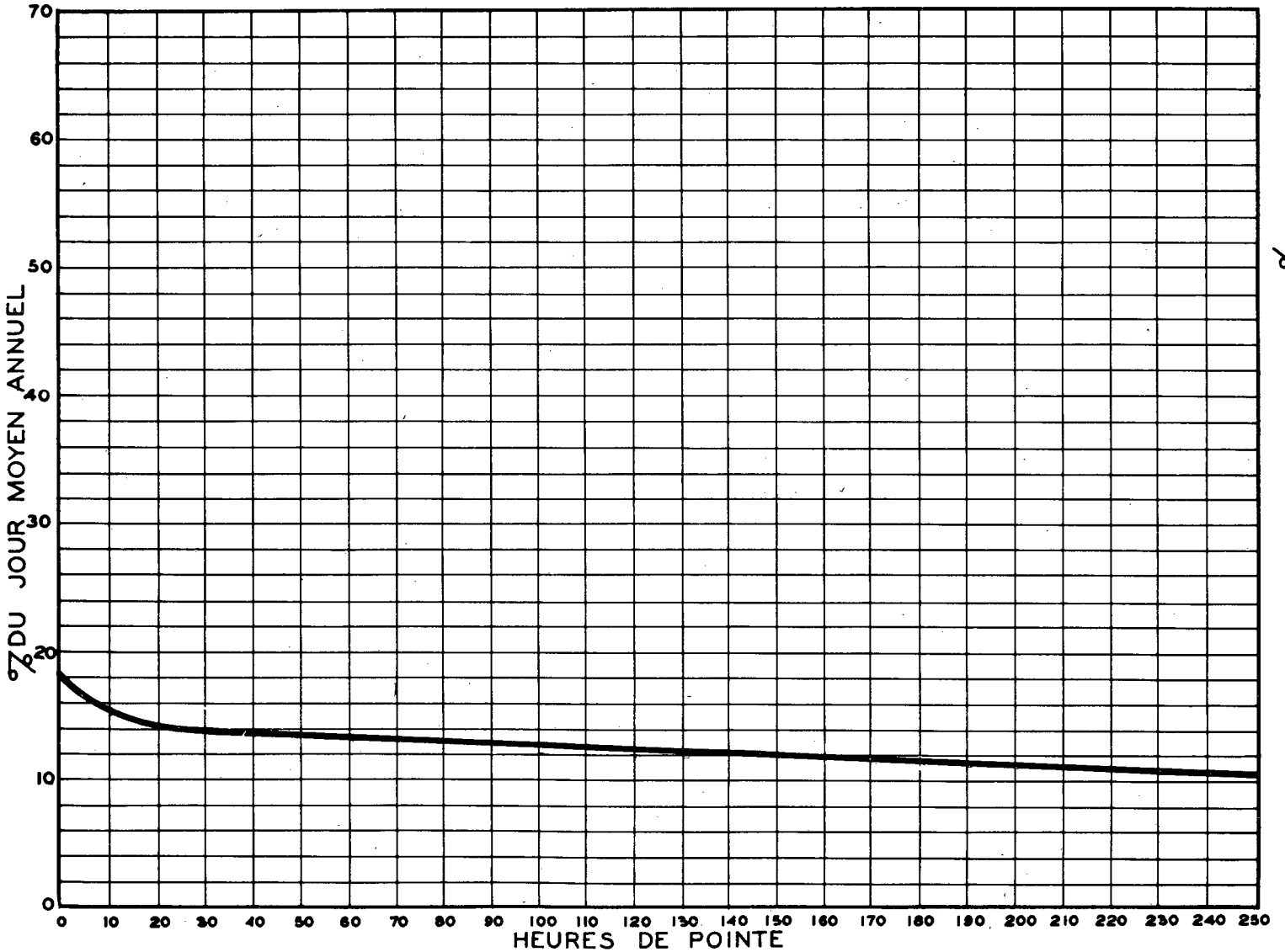
RELATION ENTRE LES HEURES DE POINTE ET LE JOUR MOYEN ANNUEL — STATION: AMQUI ROUTE N°6-2-3
