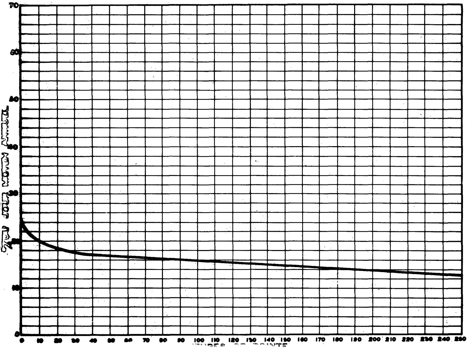
RELATION ENTRE LES HEURES DE POINTE ET LE JOUR MOYEN ANNUEL — STATION: POINTE-FORTUNE ——— ROUTE N° 40-4-91 ———
