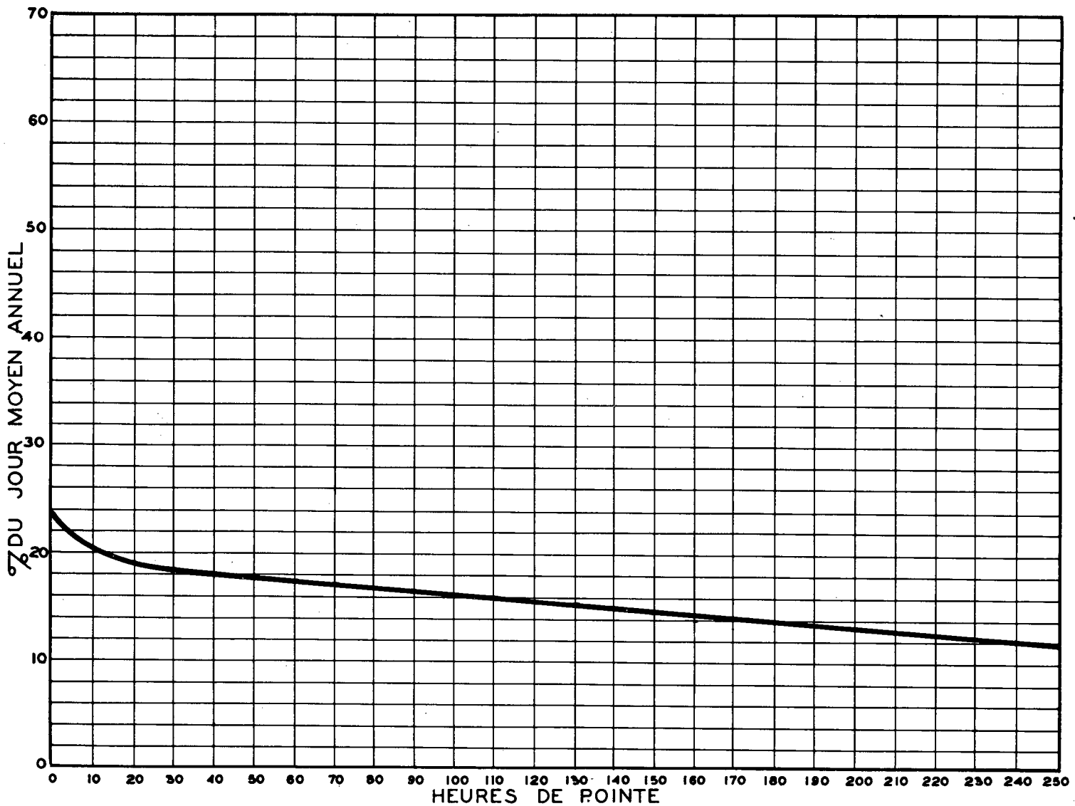
RELATION ENTRE LES HEURES DE POINTE ET LE JOUR MOYEN ANNUEL STATION: WATERLOO ROUTE No 1-8-4
