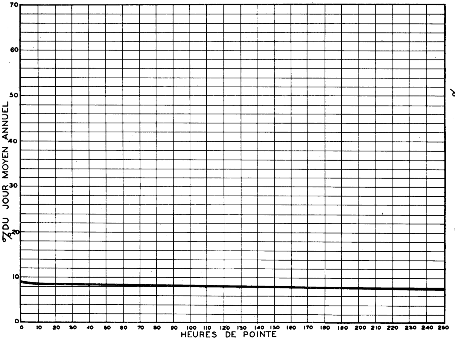
RELATION ENTRE LES HEURES DE POINTE ET LE JOUR MOYEN ANNUEL STATION: ST-LAURENT voie sud ROUTE N° 40-4-87
