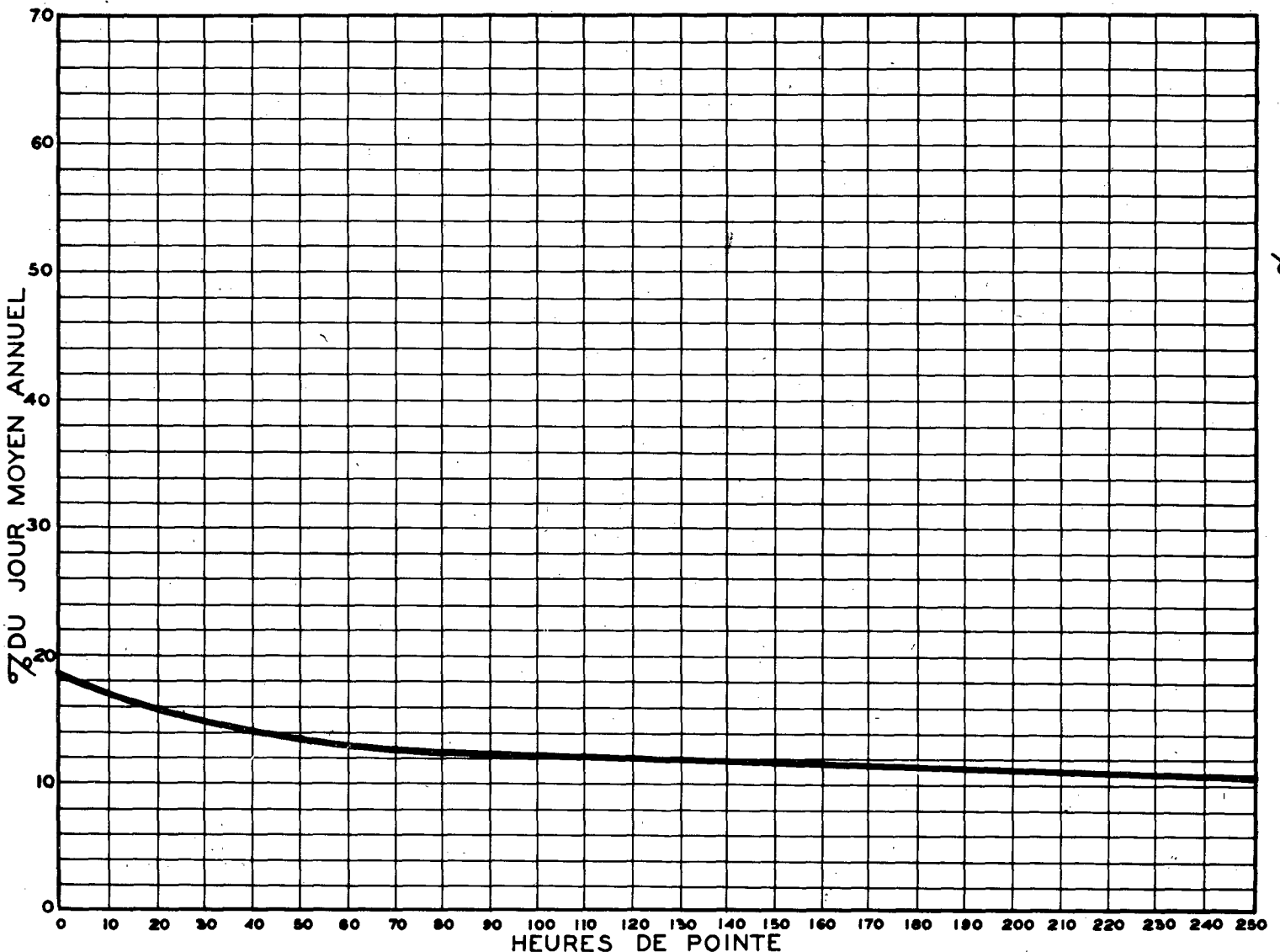
RELATION ENTRE LES HEURES DE POINTE ET LE JOUR MOYEN ANNUEL STATION: LESSISVILLE ROUTE N° 49-3-7
