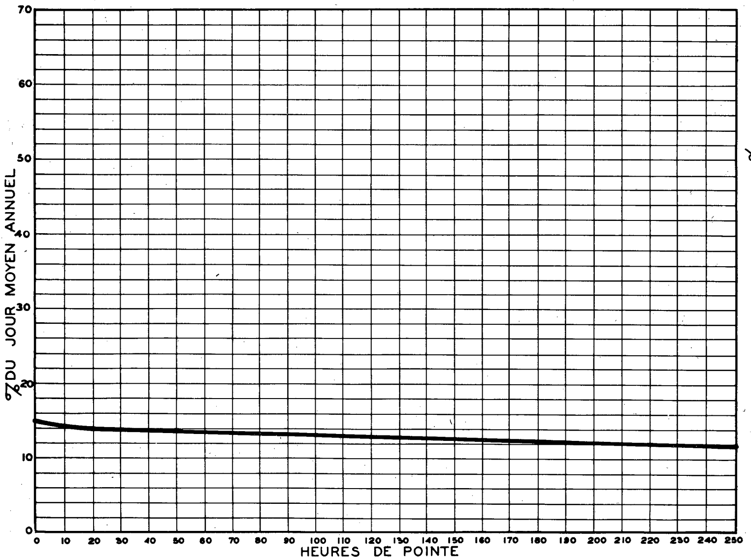
RELATION ENTRE LES HEURES DE POINTE ET LE JOUR MOYEN ANNUEL STATION: LONGUEUIL voie sud PONT JACQUES-CARTIER ROUTE N° 9-9-80
