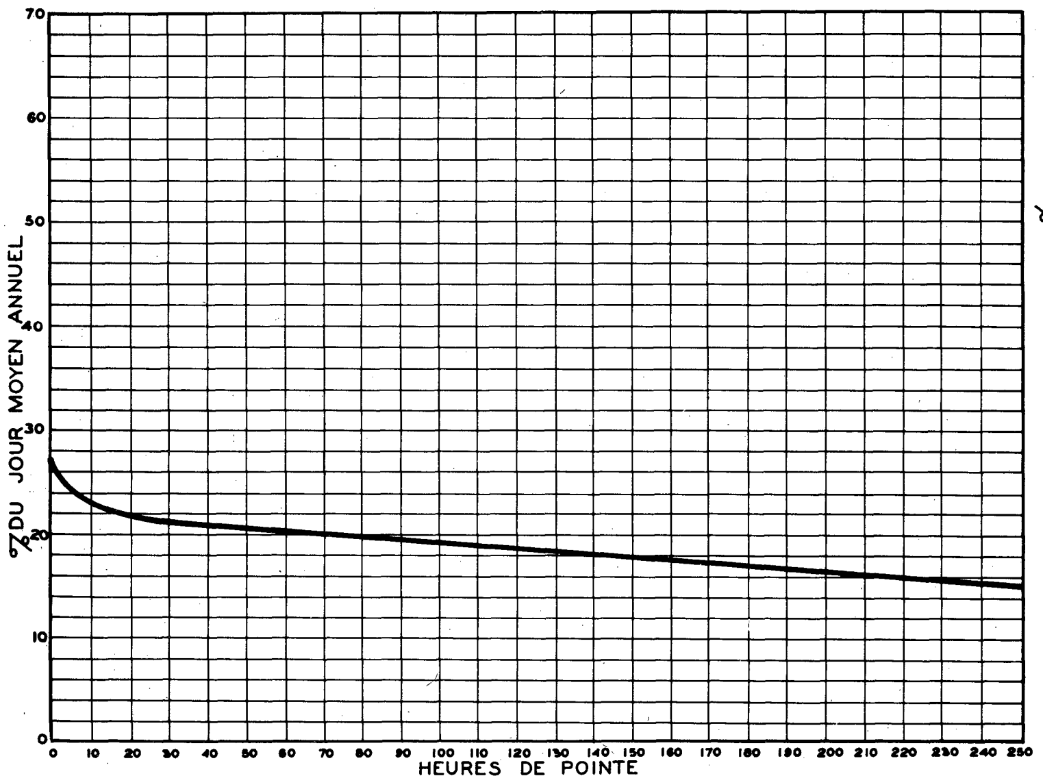
RELATION ENTRE LES HEURES DE POINTE ET LE JOUR MOYEN ANNUEL — STATION: ST-MATHIEU ROUTE N° 15-9-85
