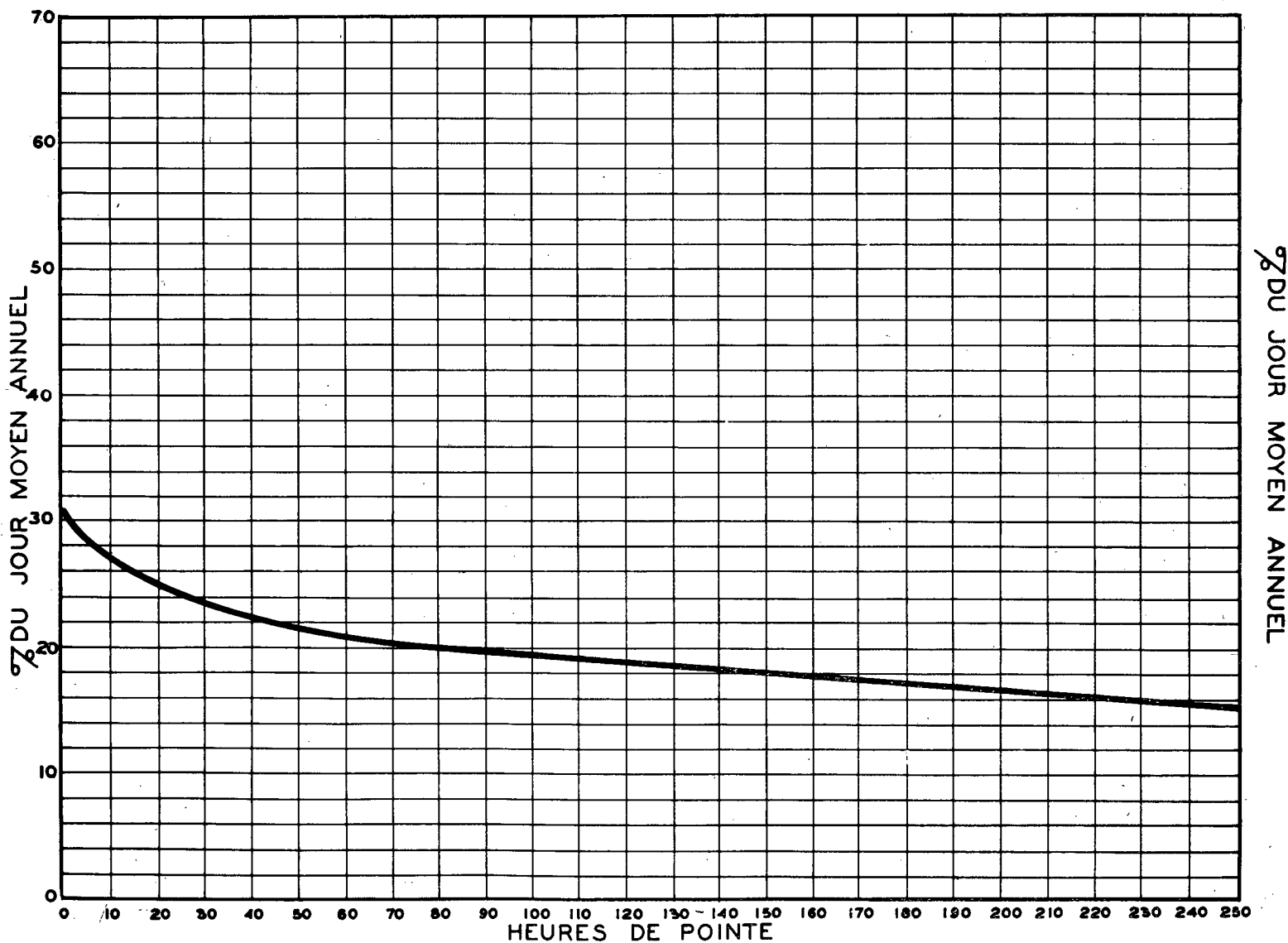
RELATION ENTRE LES HEURES DE POINTE ET LE JOUR MOYEN ANNUEL STATION: STE-FELICITE ROUTE N° 6-2-1
