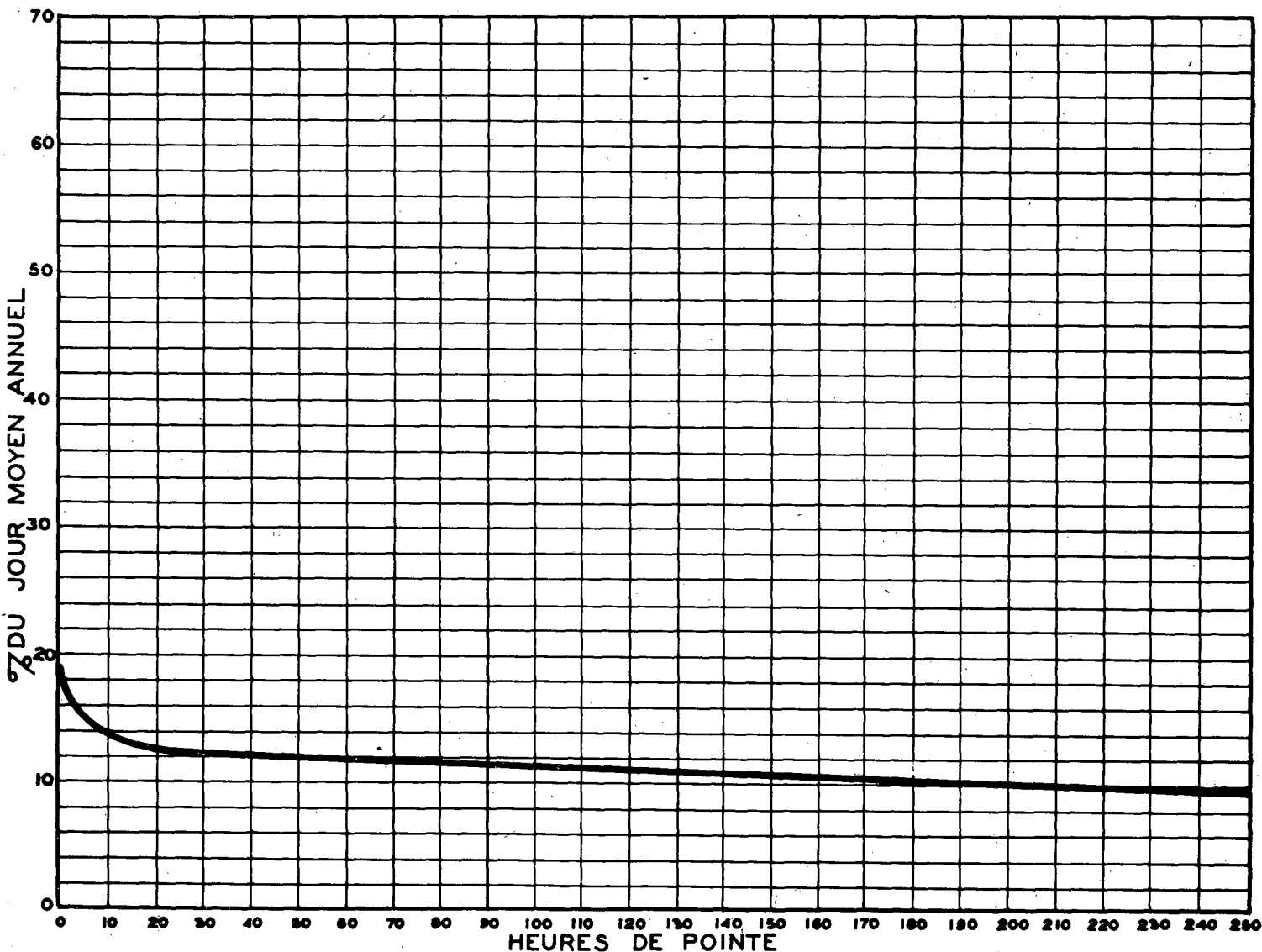
RELATION ENTRE LES HEURES DE POINTE ET LE JOUR MOYEN ANNUEL STATION: N.D. DE LA PROVIDENCE ROUTE N° 23-3-16
