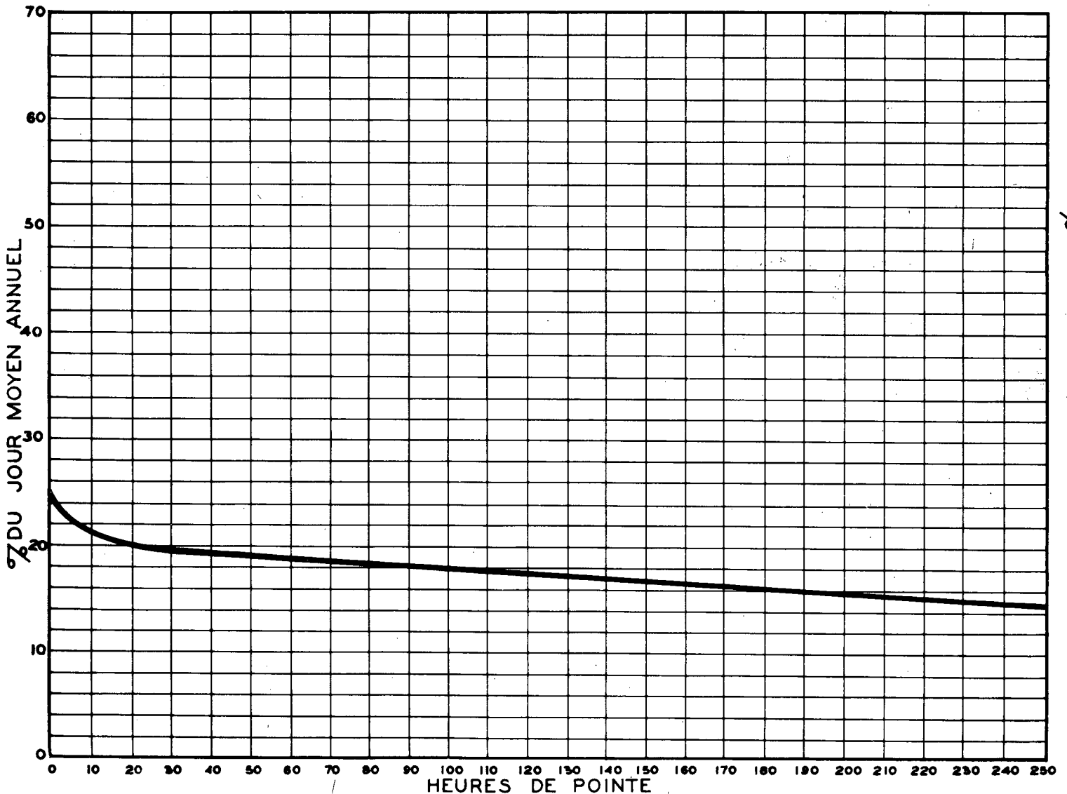
RELATION ENTRE LES HEURES DE POINTE ET LE JOUR MOYEN ANNUEL STATION: STE-ADELE ROUTE N° 11-5-65
