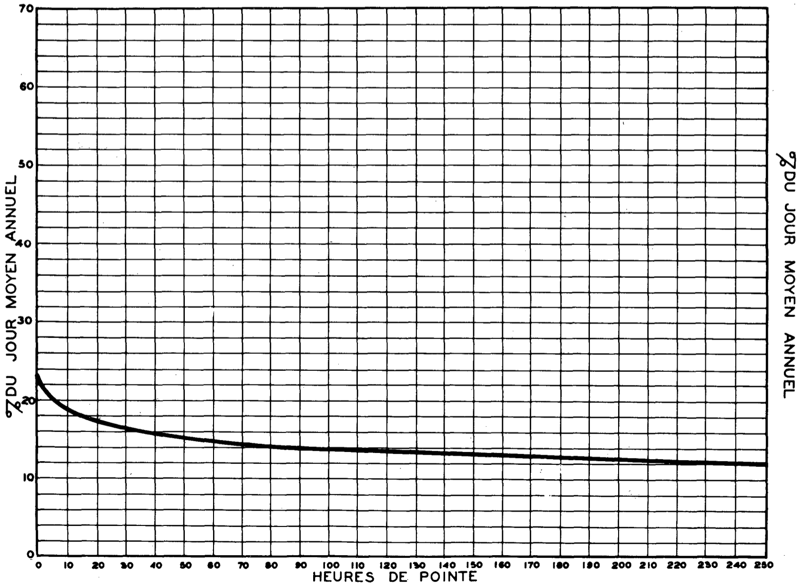
RELATION ENTRE LES HEURES DE POINTE ET LE JOUR MOYEN ANNUEL — STATION: STE-LUCE ROUTE N°10-2-1
