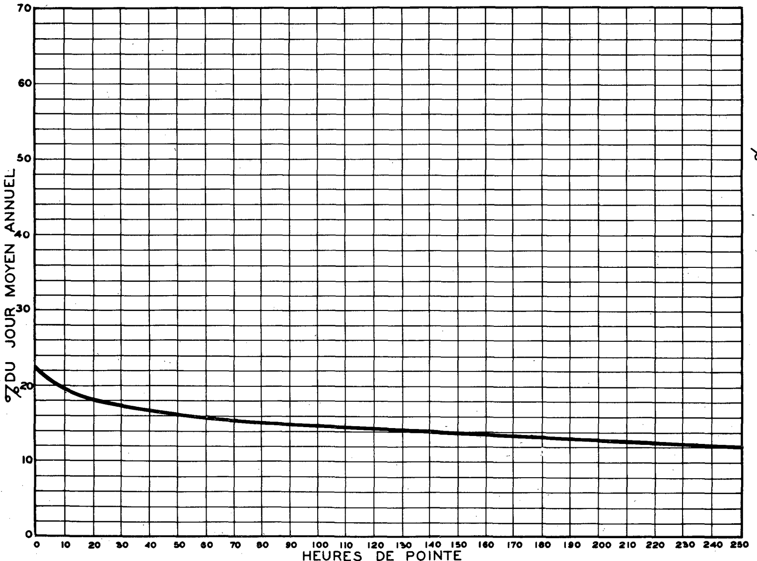
RELATION ENTRE LES HEURES DE POINTE ET LE JOUR MOYEN ANNUEL STATION: SABREVOIS ROUTE N° 7-9-64
