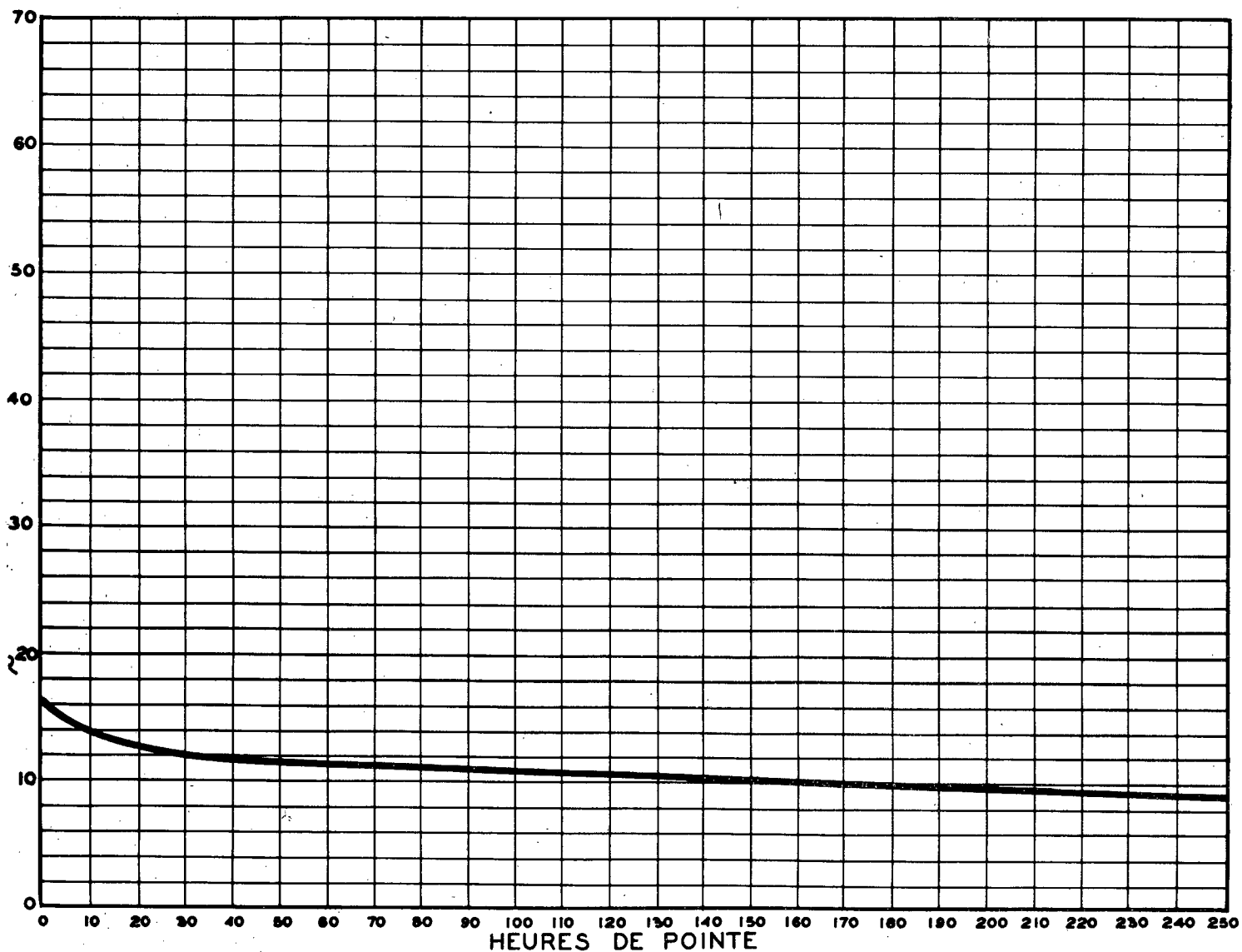
RELATION ENTRE LES HEURES DE POINTE ET LE JOUR MOYEN ANNUEL — STATION: TRACY ROUTE N° 3-8-59
