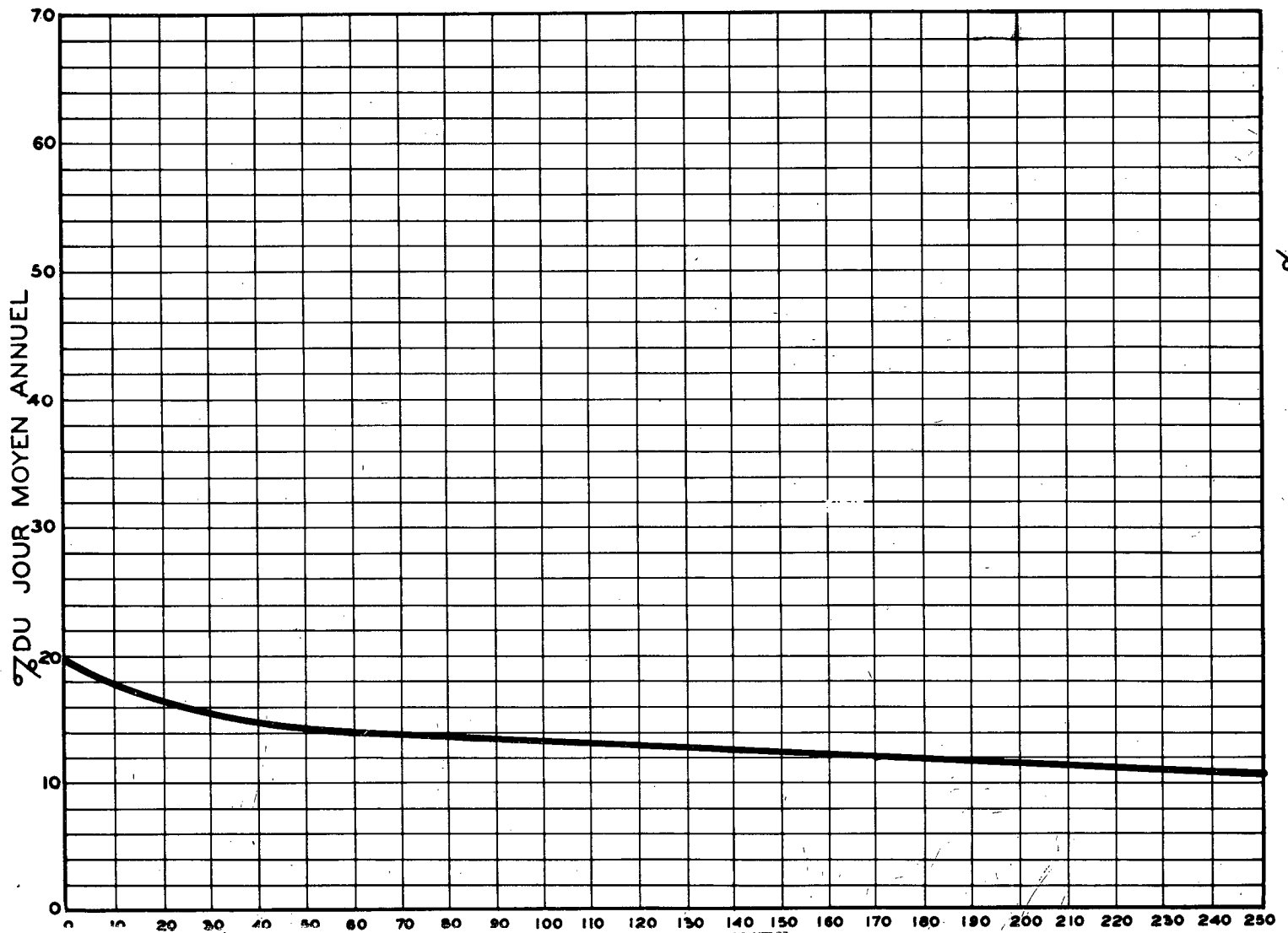
RELATION ENTRE LES HEURES DE POINTE ET LE JOUR MOYEN ANNUEL STATION: ST-GREGOIRE voie est PONT DE TROIS-RIVIERES ROUTE N° 8-15
