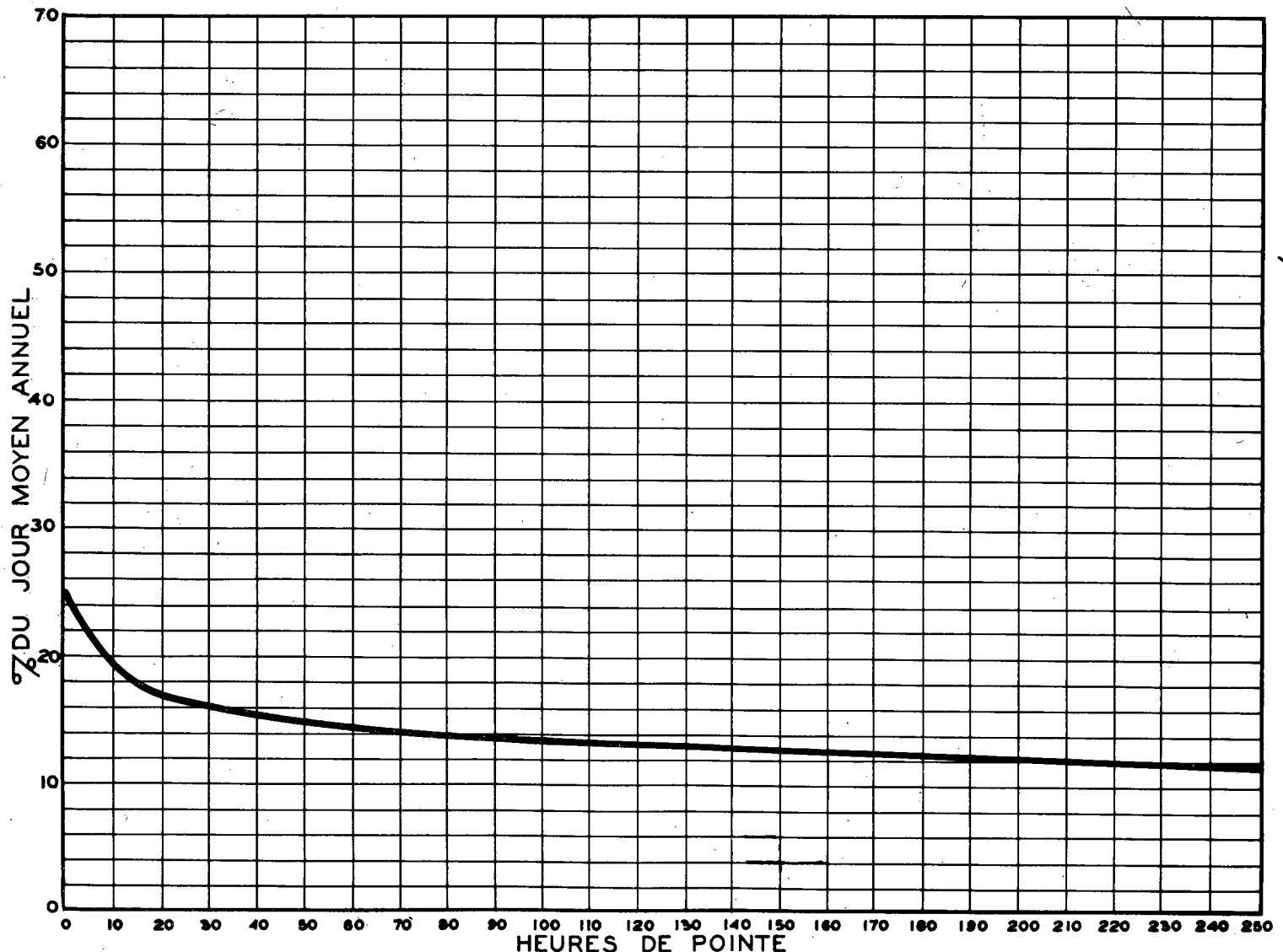
RELATION ENTRE LES HEURES DE POINTE ET LE JOUR MOYEN ANNUEL STATION: ST-LEONARD RTE TRANS-CANADIENNE ROUTE N°20-8-1
