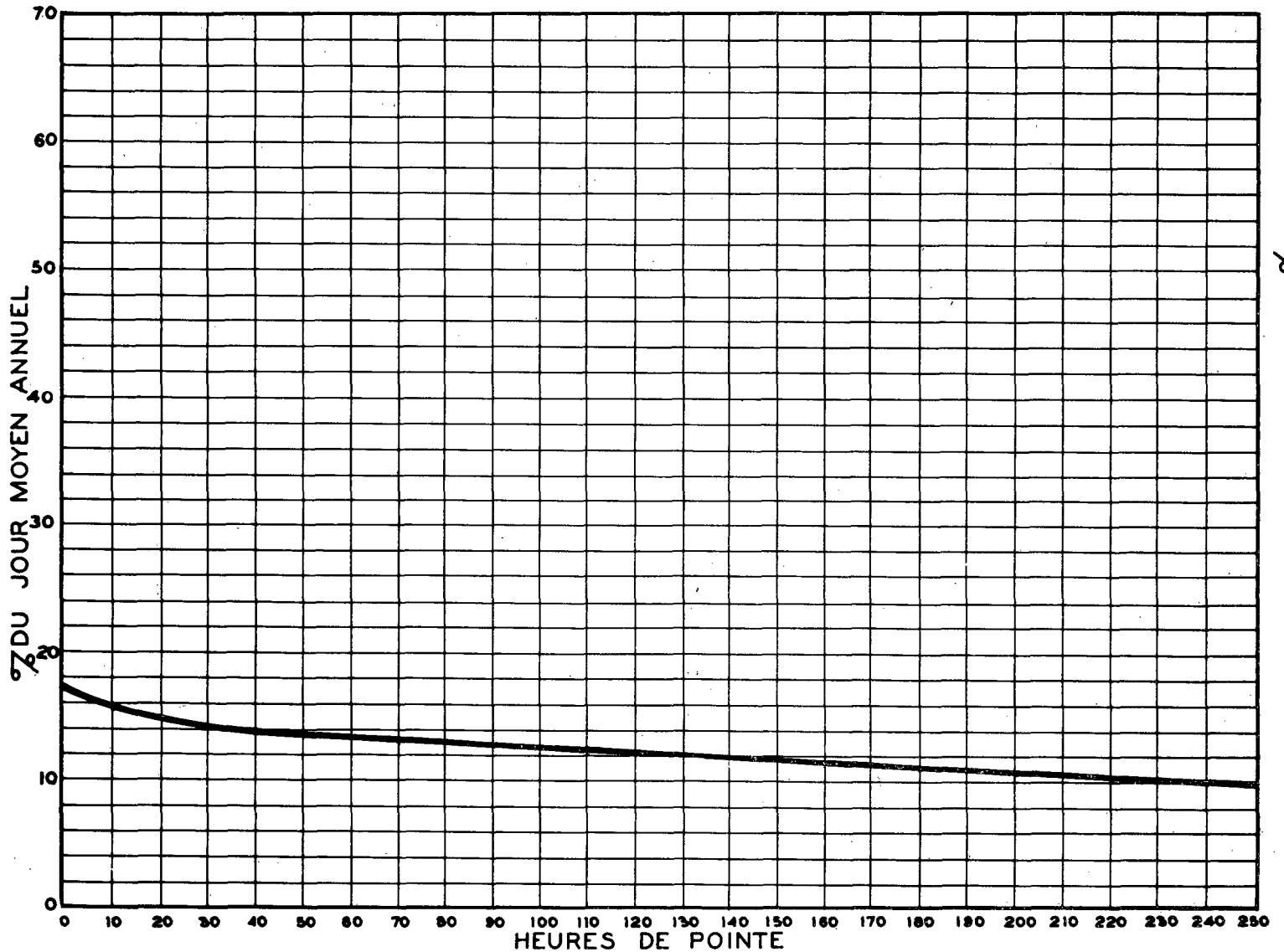
RELATION ENTRE LES HEURES DE POINTÉ ET LE JOUR MOYEN ANNUEL — STATION: WARWICK ROUTE N° 5-8-2
