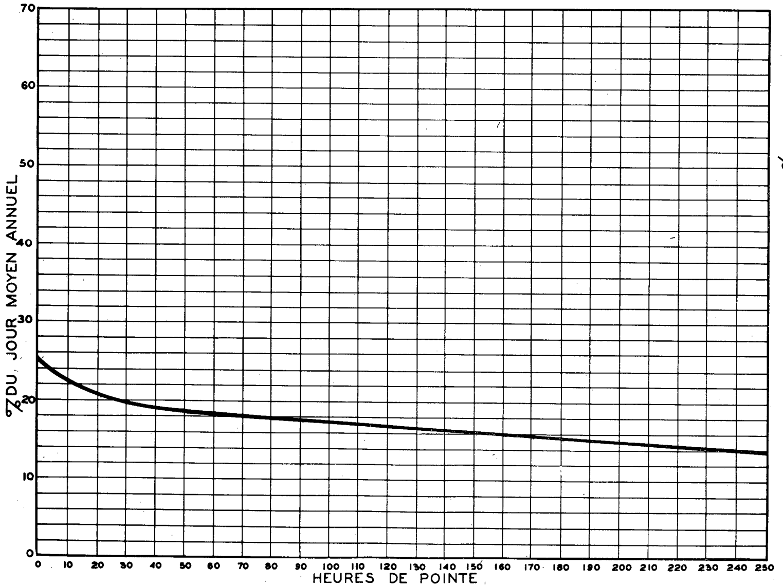
RELATION ENTRE LES HEURES DE POINTE ET LE JOUR MOYEN ANNUEL STATION: ROCK-ISLAND 2 voies ROUTE N° 5-3-12-2
