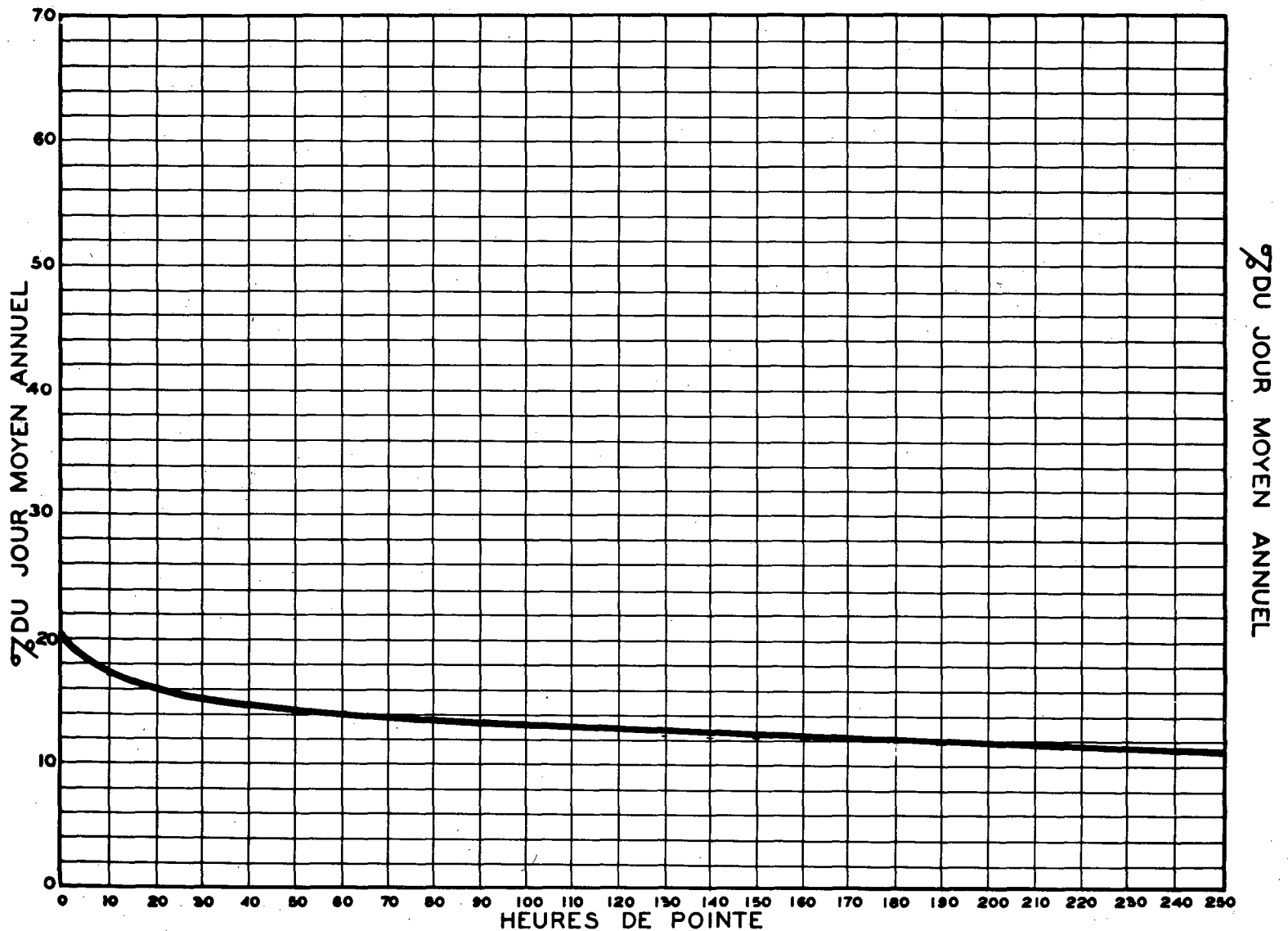
RELATION ENTRE LES HEURES DE POINTE ET LE JOUR MOYEN ANNUEL STATION: ST-PIERRE D'ESCOURT ROUTE N° 51-2-2
