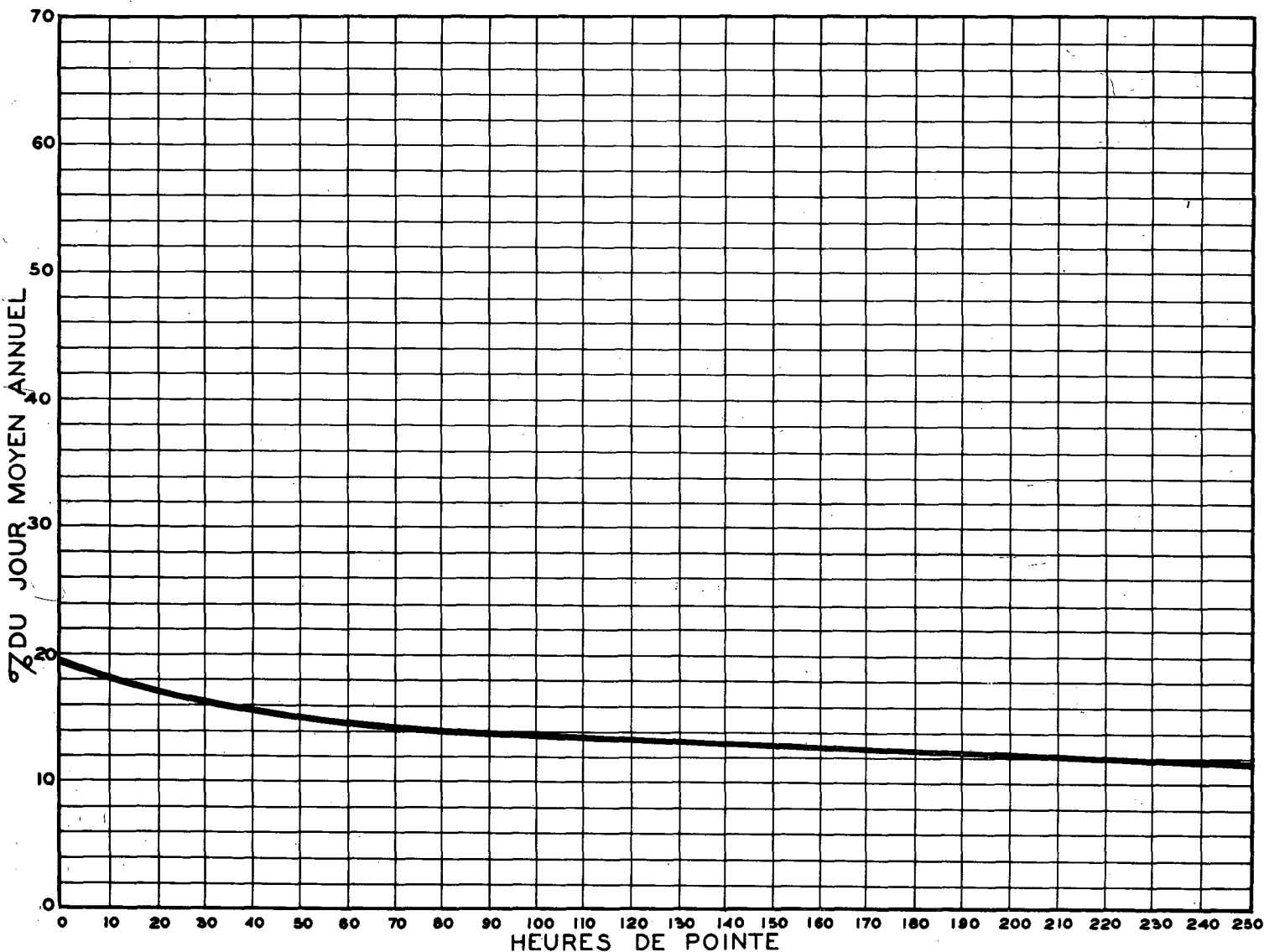
RELATION ENTRE LES HEURES DE POINTE ET LE JOUR MOYEN ANNUEL STATION: DESCHAMBAULT ROUTE No 2-1-8
