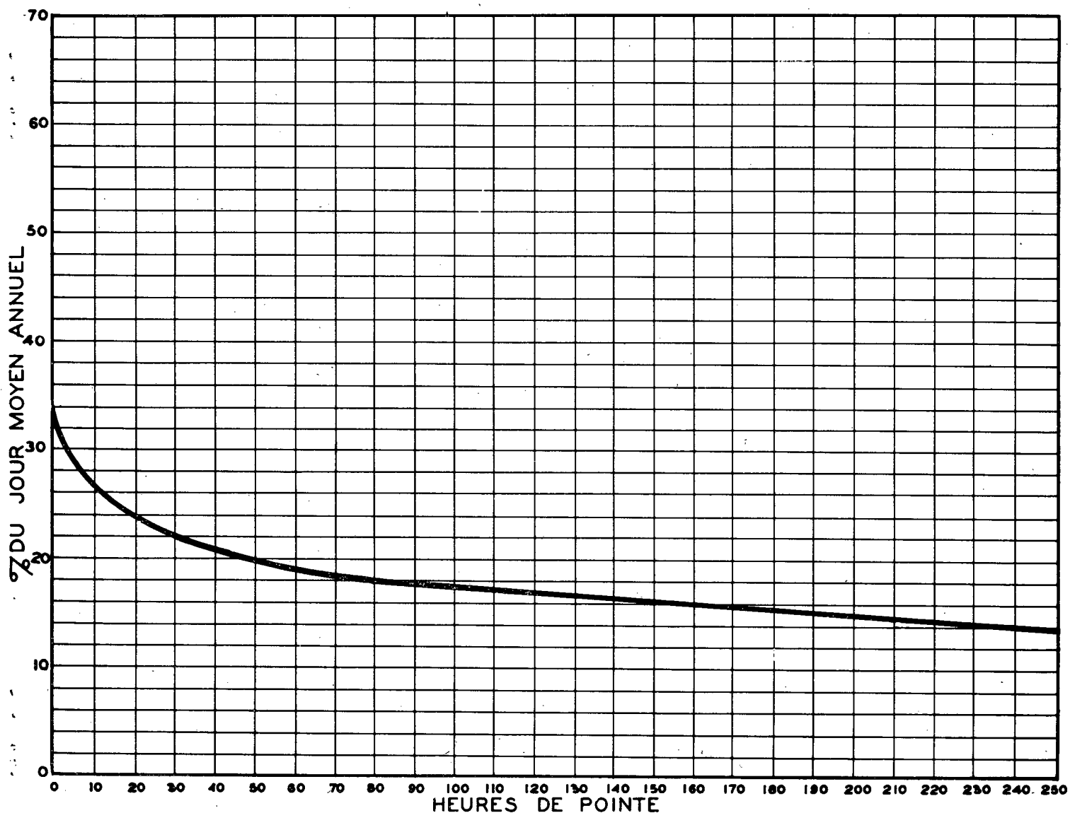
RELATION ENTRE LES HEURES DE POINTE ET LE JOUR MOYEN ANNUEL — STATION: MONTMORENCY PONT DE L'ILE D'ORLEANS ROUTE N° 1-20 —
