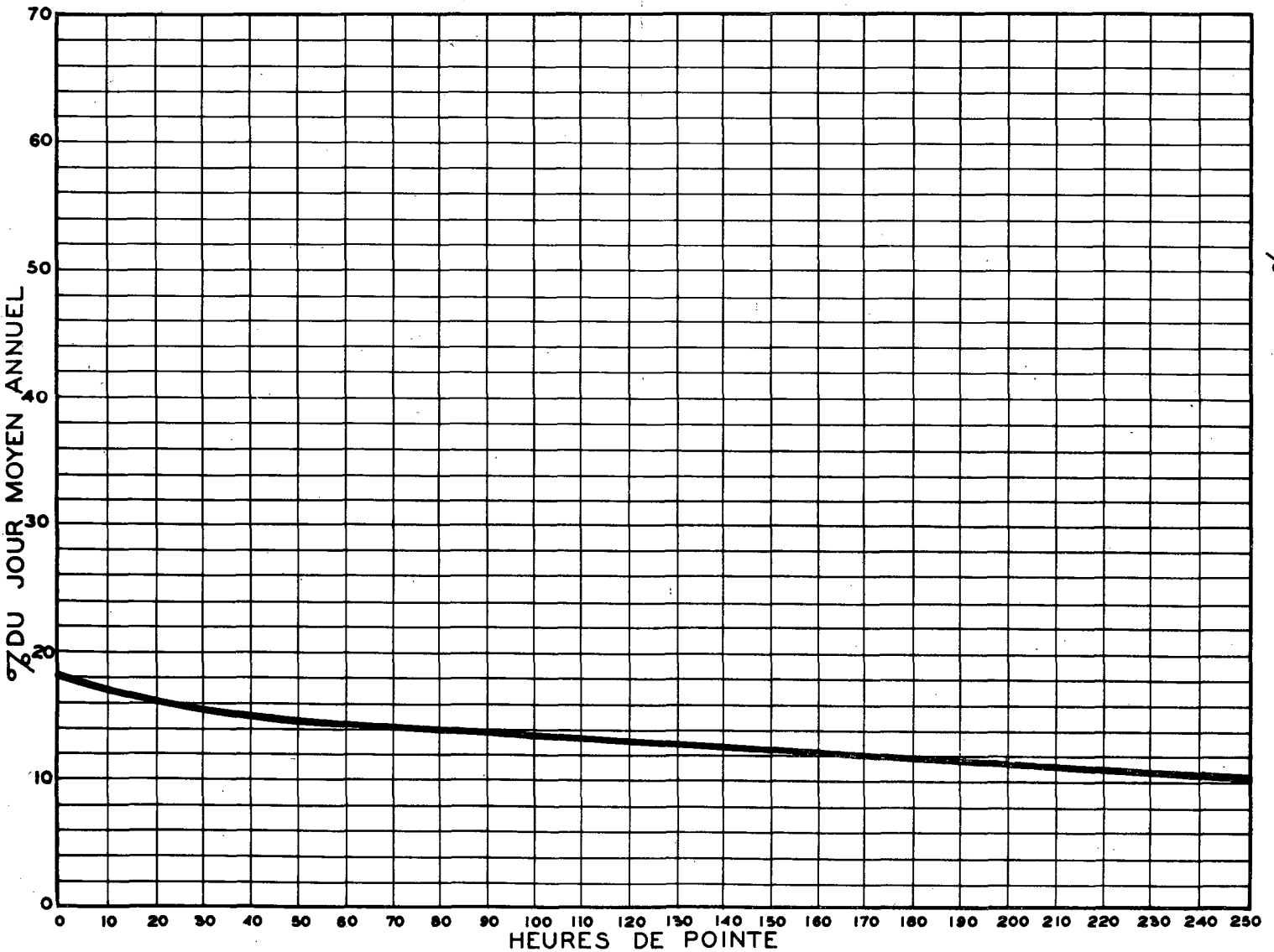
RELATION ENTRE LES HEURES DE POINTE ET LE JOUR MOYEN ANNUEL STATION: ST-SULPICE ROUTE N° 2-10-52
