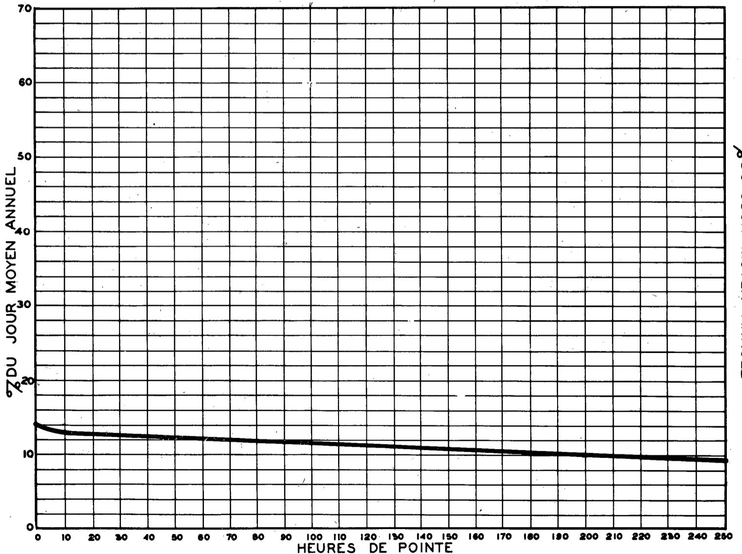
RELATION ENTRE LES HEURES DE POINTE ET LE JOUR MOYEN ANNUEL STATION: CHARLESBOURG BOUL. PIERRE BERTRAND ROUTE N° 78
