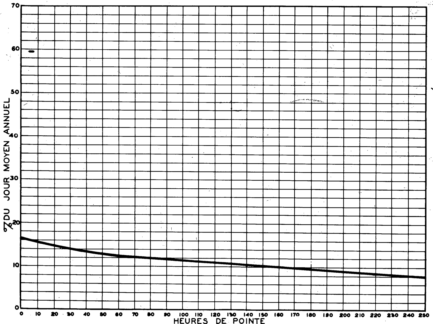
RELATION ENTRE LES HEURES DE POINTE ET LE JOUR MOYEN ANNUEL — STATION: MONTREAL-NORD voie ouest PONTPIEIX ROUTE N° 18-25-4-51
