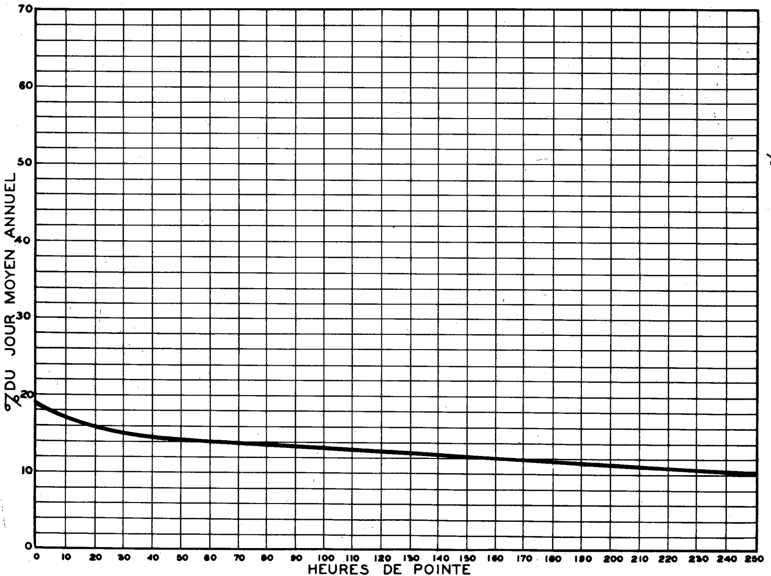
RELATION ENTRE LES HEURES DE POINTE ET LE JOUR MOYEN ANNUEL STATION: ST-BRUNO ROUTE N°16-7-3
