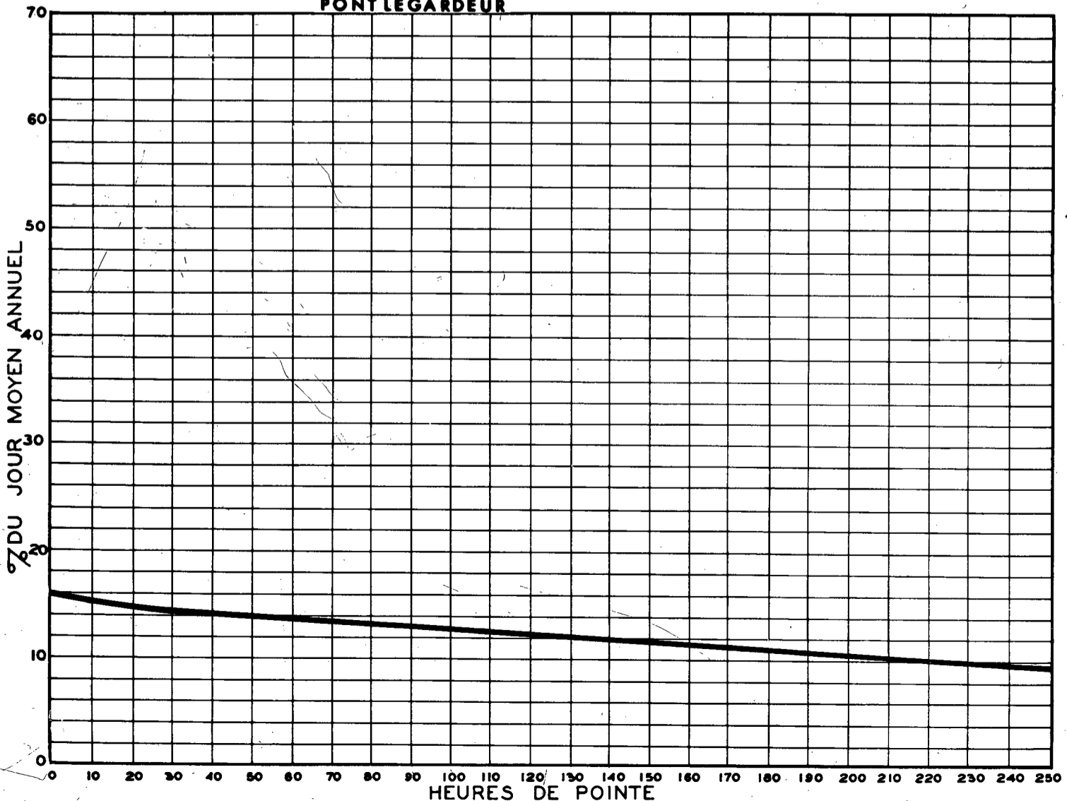
RELATION ENTRE LES HEURES DE POINTE ET LE JOUR MOYEN ANNUEL STATION: POINTE-AUX-TREMBLES voie ouest ROUTE N° 2-4-85 PONT LE GARDEUR
