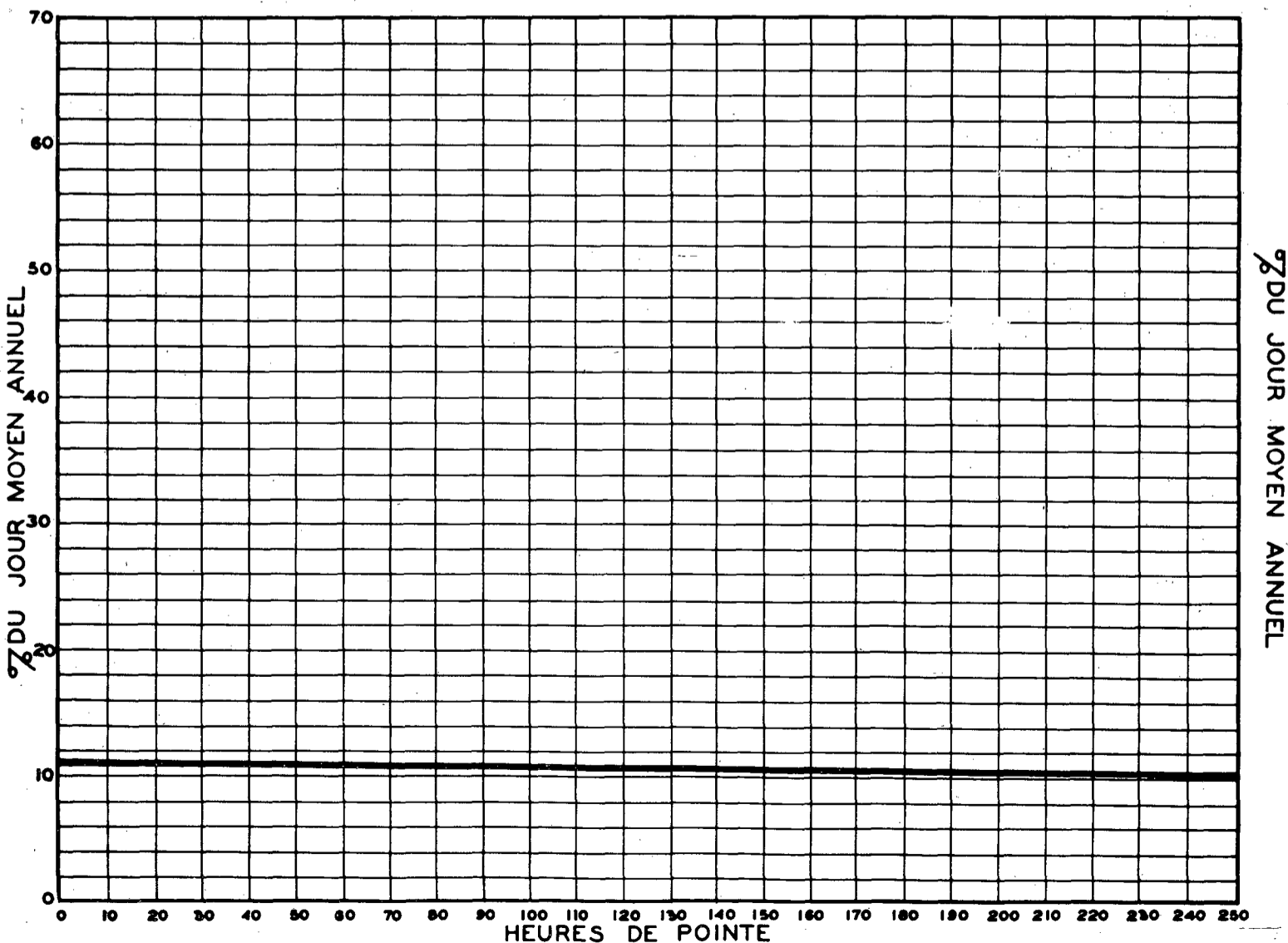
RELATION ENTRE LES HEURES DE POINTE ET LE JOUR MOYEN ANNUEL STATION: MONTREAL voie est. BOUL. DECARIE ROUTE N° 15-4-50
