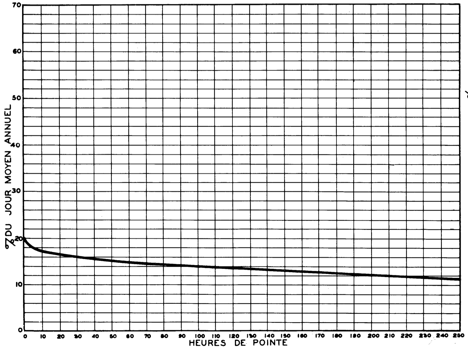
RELATION ENTRE LES HEURES DE POINTE ET LE JOUR MOYEN ANNUEL — STATION: ST-JANVIER ——— ROUTE N°11-5-63 ———
