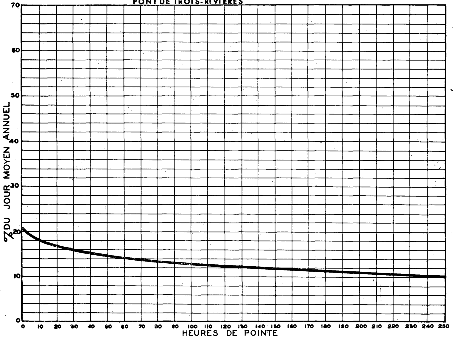
RELATION ENTRE LES HEURES DE POINTE ET LE JOUR MOYEN ANNUEL STATION: ST-GREGOIRE voie ouest PONT DE TROIS-RIVIERES ROUTE N° 8-15
