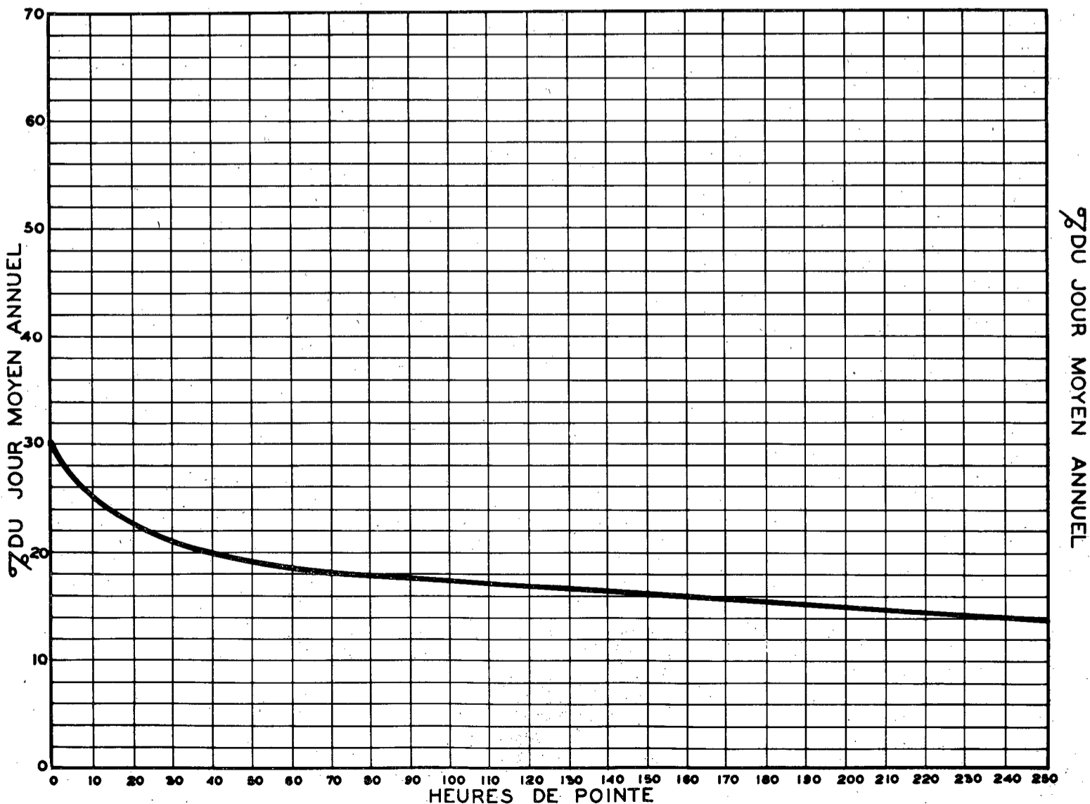
RELATION ENTRE LES HEURES DE POINTE ET LE JOUR MOYEN ANNUEL STATION: RIVIERE BEAUDETTE ROUTE N°20-4-90
