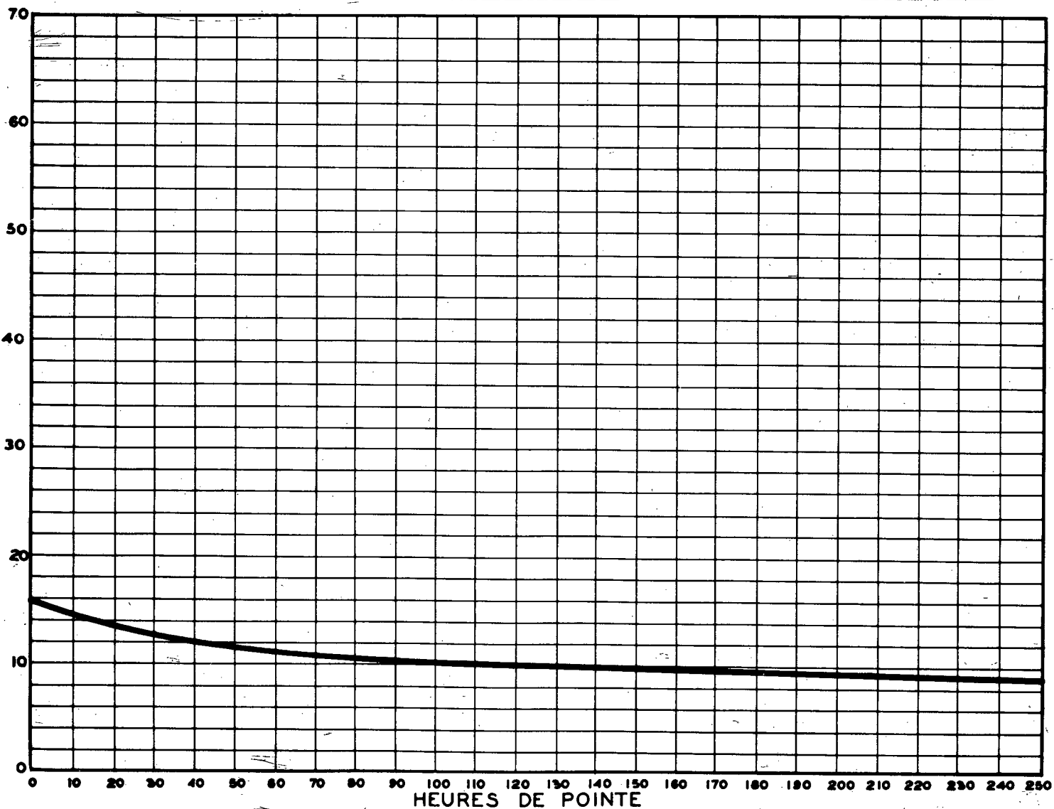
RELATION ENTRE LES HEURES DE POINTE ET LE JOUR MOYEN ANNUEL STATION: DOUVILLE ROUTE N° 9-8-65
