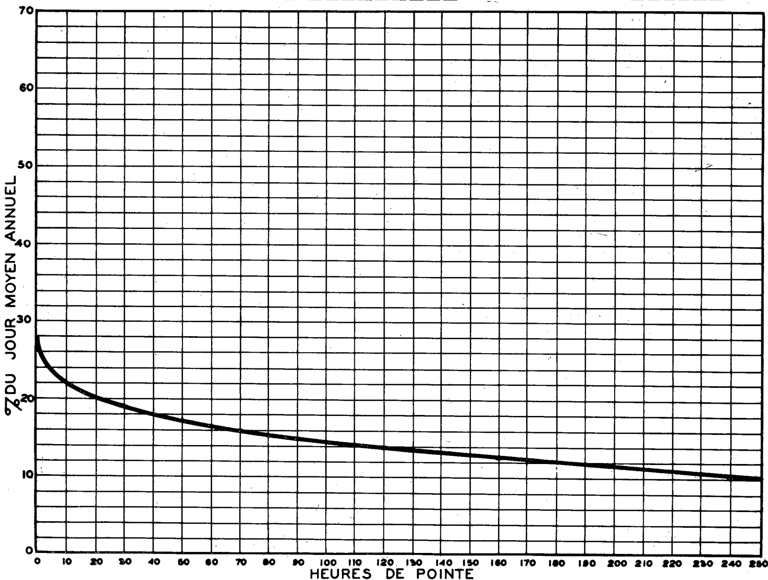
RELATION ENTRE LES HEURES DE POINTE ET LE JOUR MOYEN ANNUEL — STATION: N.D. DES LAURENTIDES — — — — — ROUTE N° 54-1-17 — — — — —
