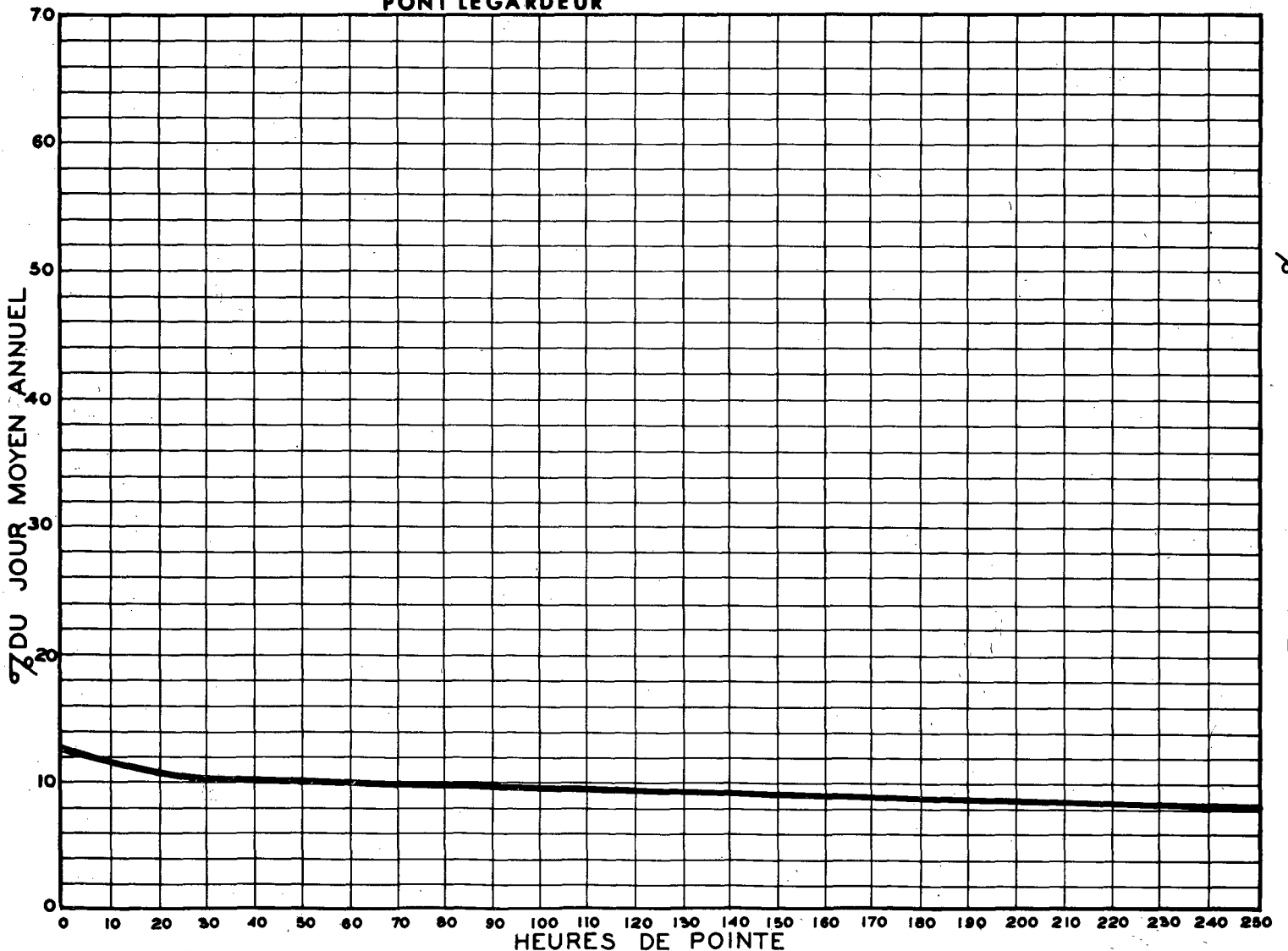
RELATION ENTRE LES HEURES DE POINTE ET LE JOUR MOYEN ANNUEL STATION: POINTE-AUX-TREMBLES 2voies ROUTE N° 2-4-85 PONT LE GARDEUR
