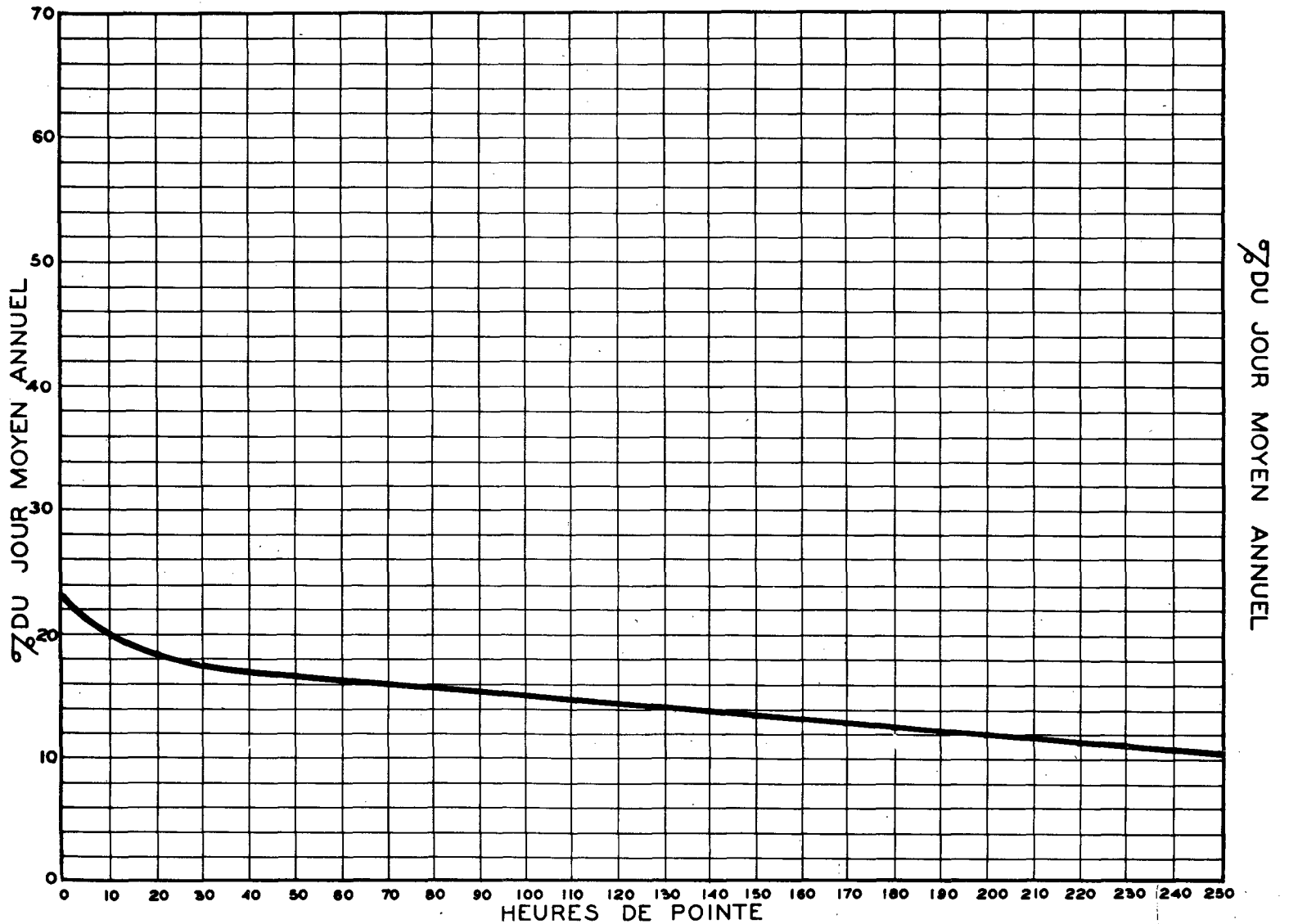
RELATION ENTRE LES HEURES DE POINTE ET LE JOUR MOYEN ANNUEL STATION: ROUEMONT ROUTE N° 1-8-80
