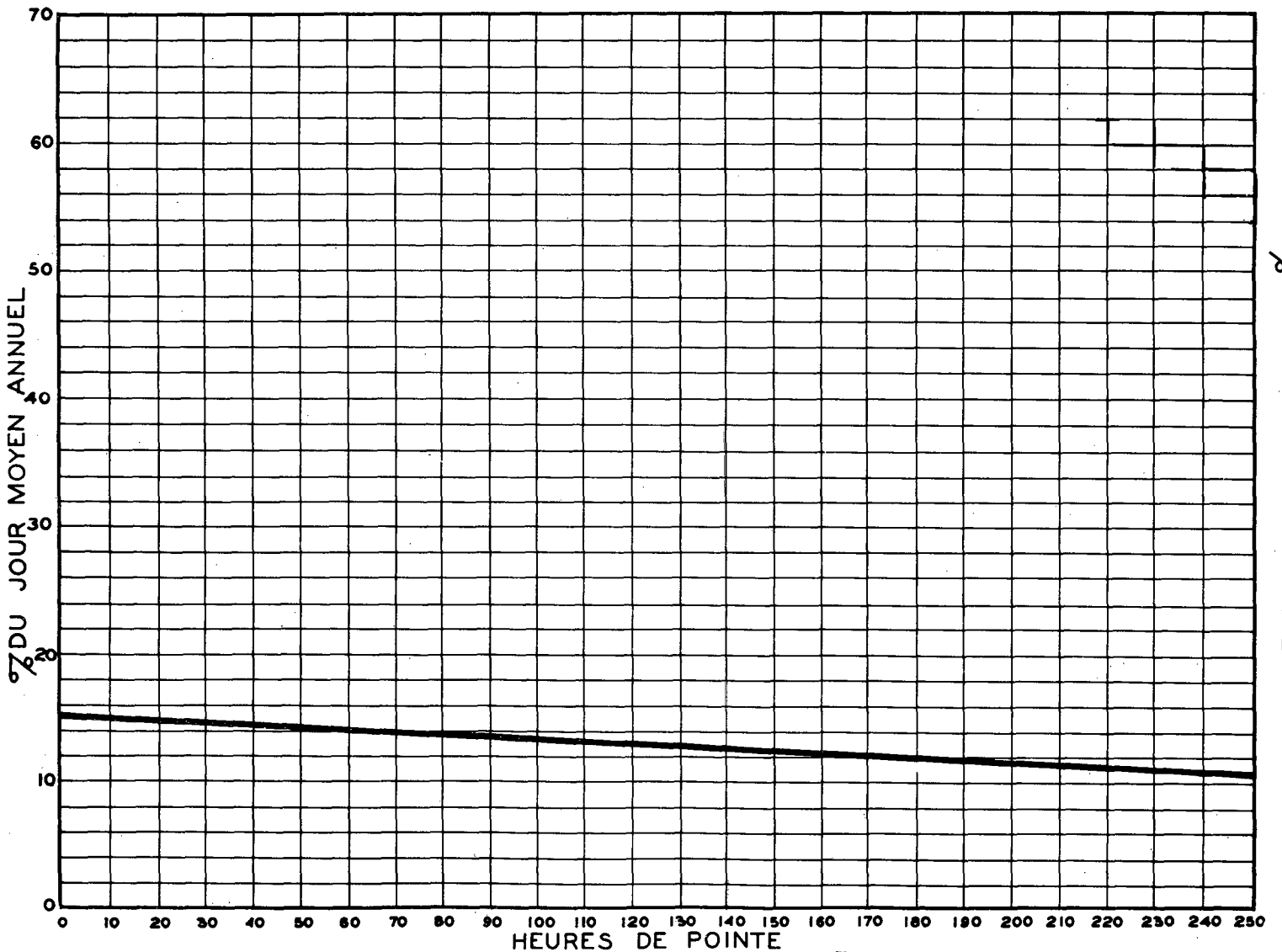
RELATION ENTRE LES HEURES DE POINTE ET LE JOUR MOYEN ANNUEL STATION: ILE PERROT voie sud — PONT GALIPEAULT ROUTE N° 2-4-54 —
