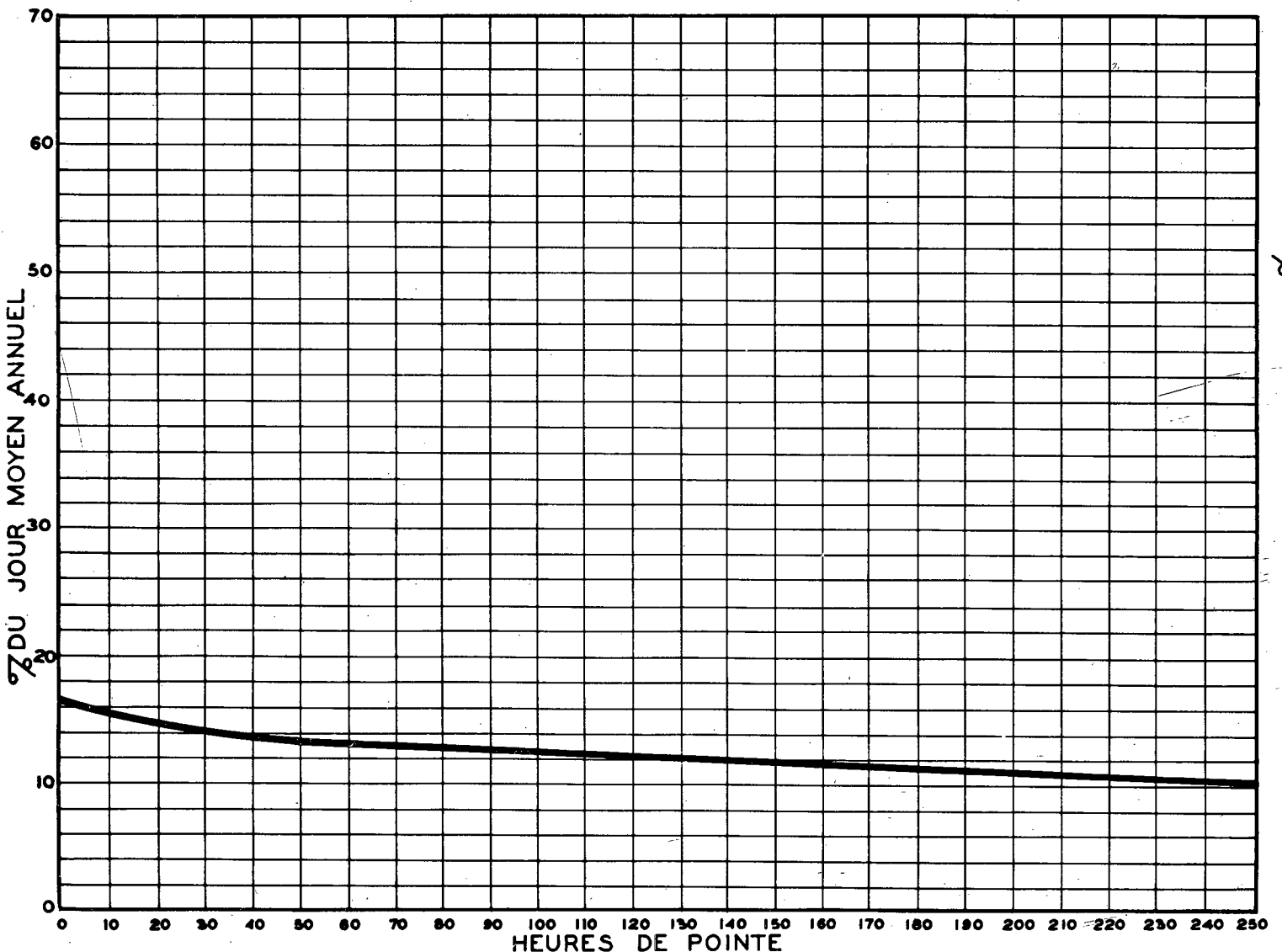
RELATION ENTRE LES HEURES DE POINTE ET LE JOUR MOYEN ANNUEL STATION: POINTE DU LAC ROUTE N° 2-10-54
