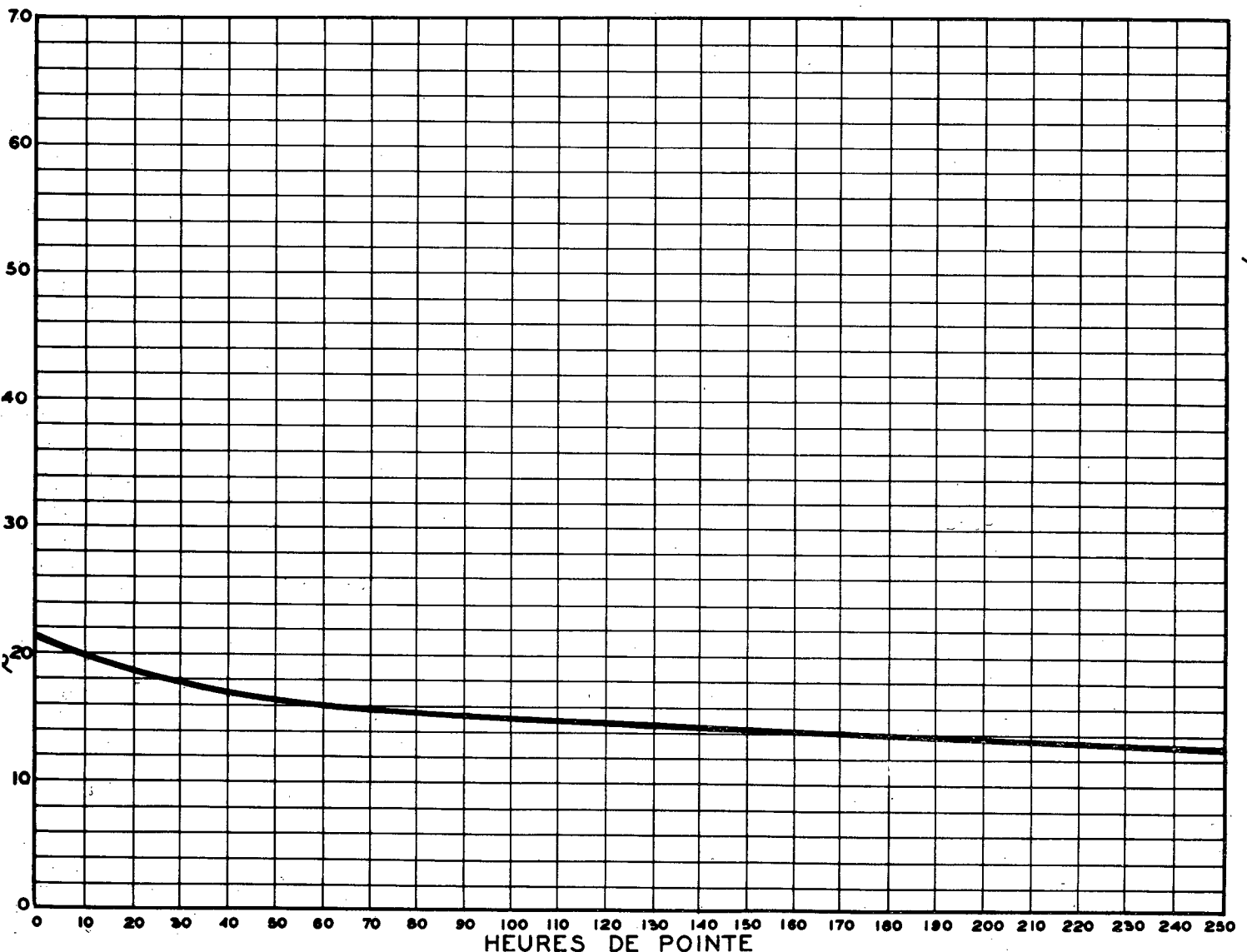
RELATION ENTRE LES HEURES DE POINTE ET LE JOUR MOYEN ANNUEL — STATION: STANSTEAD EST ROUTE N° 5-3-9
