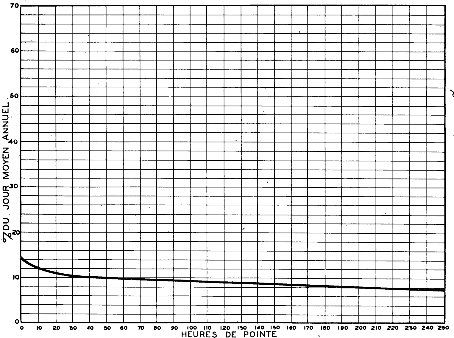
RELATION ENTRE LES HEURES DE POINTE ET LE JOUR MOYEN ANNUEL STATION: LAVAL PONT ST-EUSTACHE ROUTE N° 8-4-55
