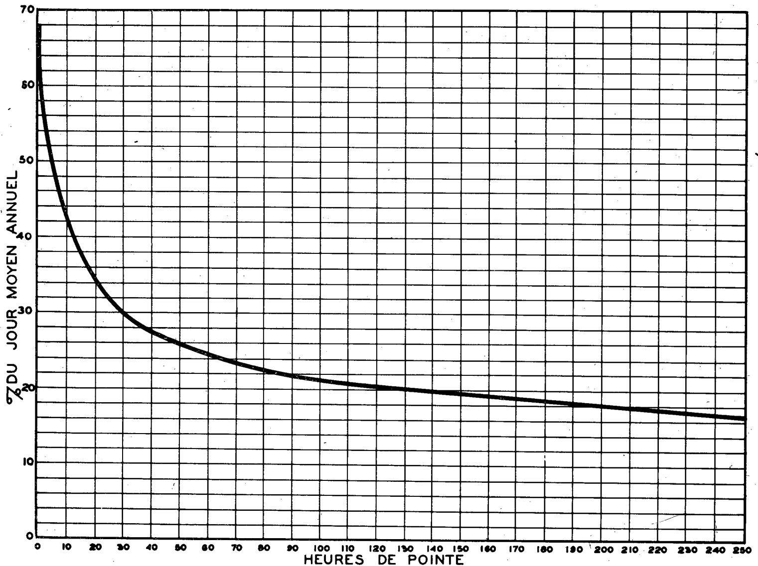
RELATION ENTRE LES HEURES DE POINTE ET LE JOUR MOYEN ANNUEL — STATION: ST-JEAN-BOSCO ——— ROUTE N° 19-10-4 ———
