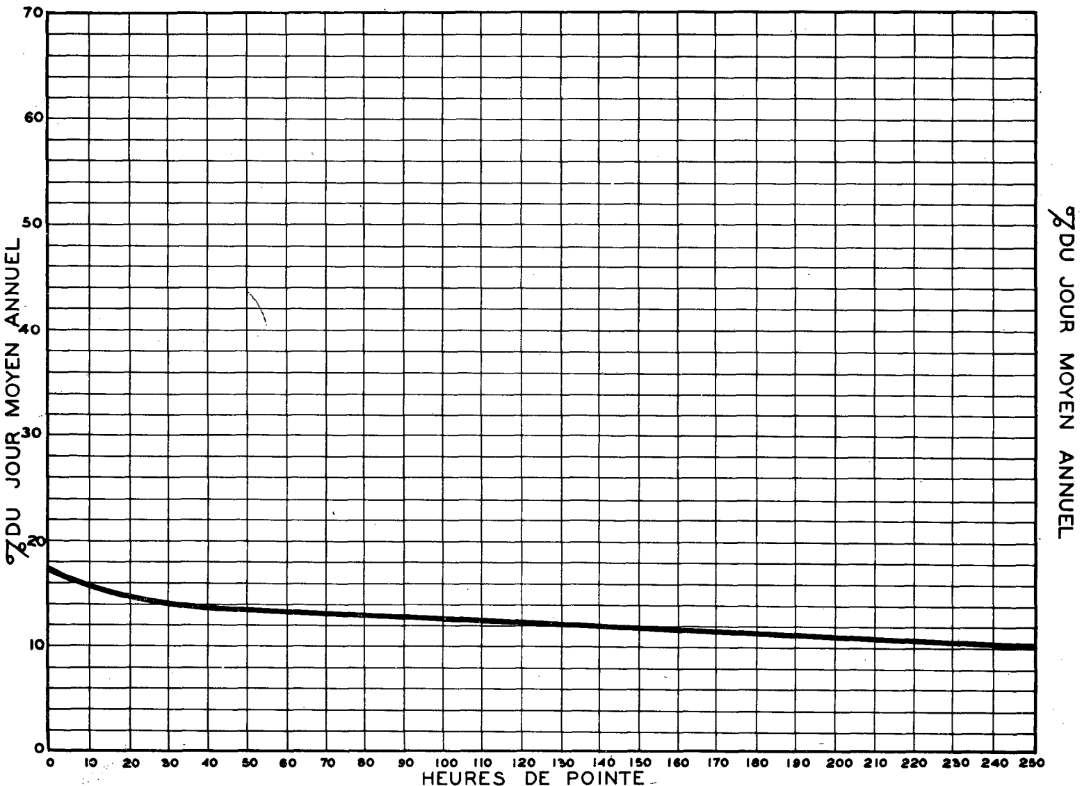
RELATION ENTRE LES HEURES DE POINTE ET LE JOUR MOYEN ANNUEL — STATION ST-GREGOIRE ROUTE N° 3-8-5
