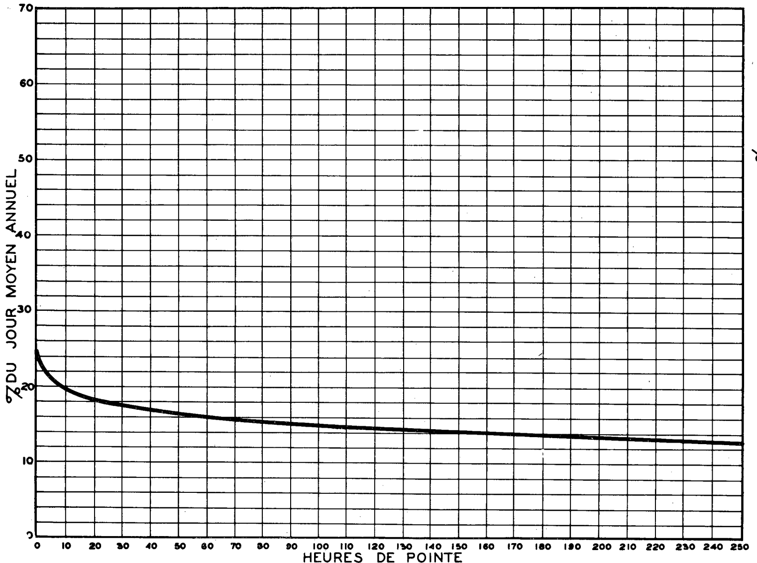
RELATION ENTRE LES HEURES DE POINTE ET LE JOUR MOYEN ANNUÉL STATION: AYLMER ROUTE N° 8-5-59
