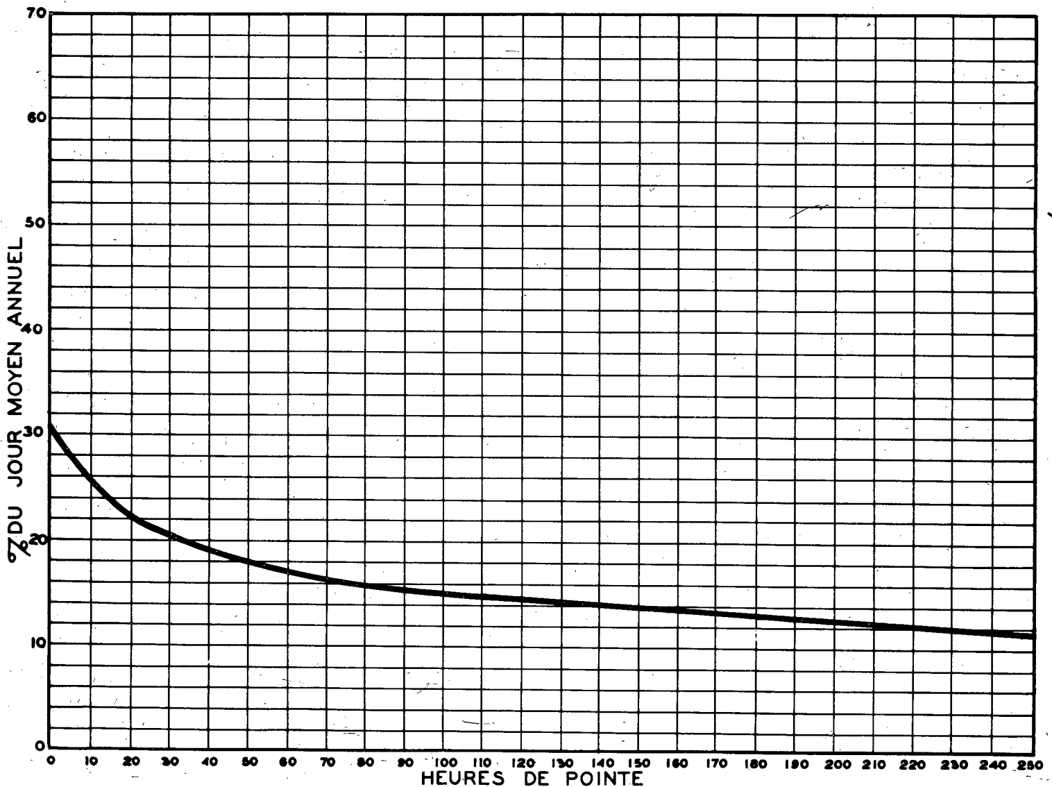
RELATION ENTRE LES HEURES DE POINTE ET LE JOUR MOYEN ANNUEL STATION: GRANDES-PILES ROUTE N° 19-10-14
