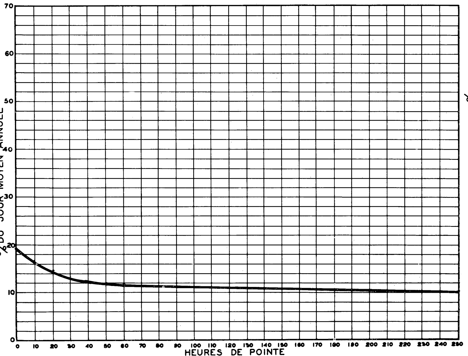
RELATION ENTRE LES HEURES DE POINTE ET LE JOUR MOYEN ANNUEL — STATION: PONT LE GARDEUR POINTE AUX TREMBLES ROUTE N° 2-4-85 VOIE EST
