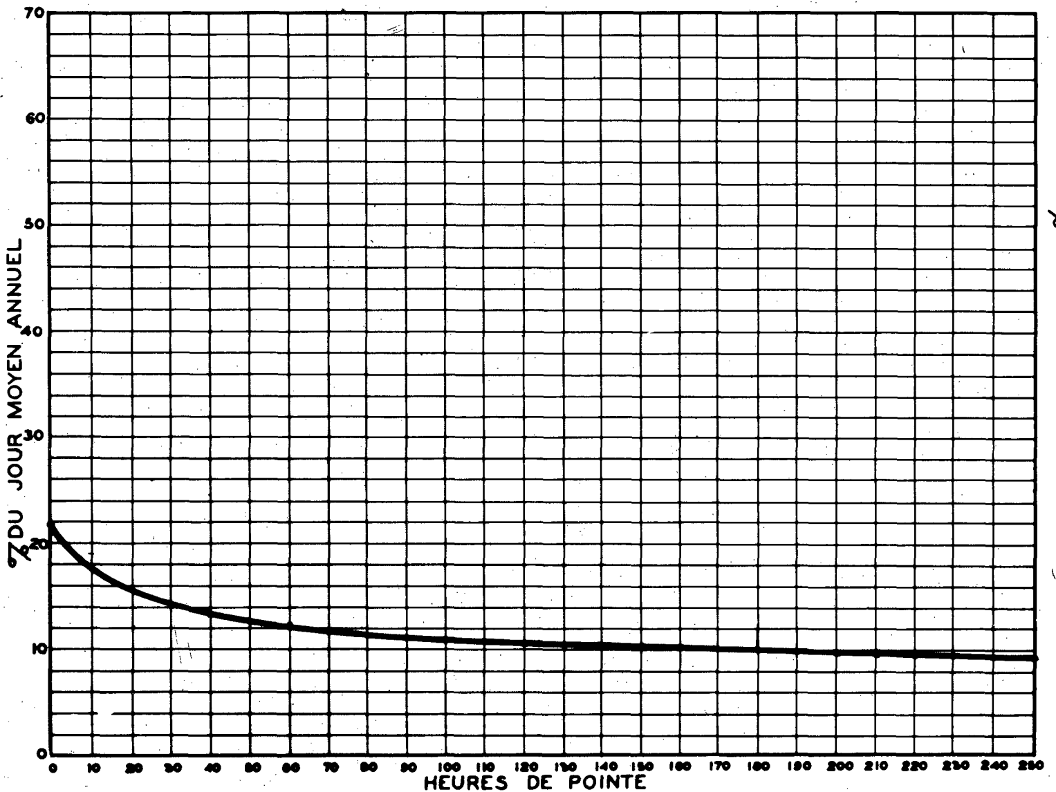
RELATION ENTRE LES HEURES DE POINTE ET LE JOUR MOYEN ANNUEL — STATION: SAINT-NICOLAS voie nord ROUTE No 9-1-11
