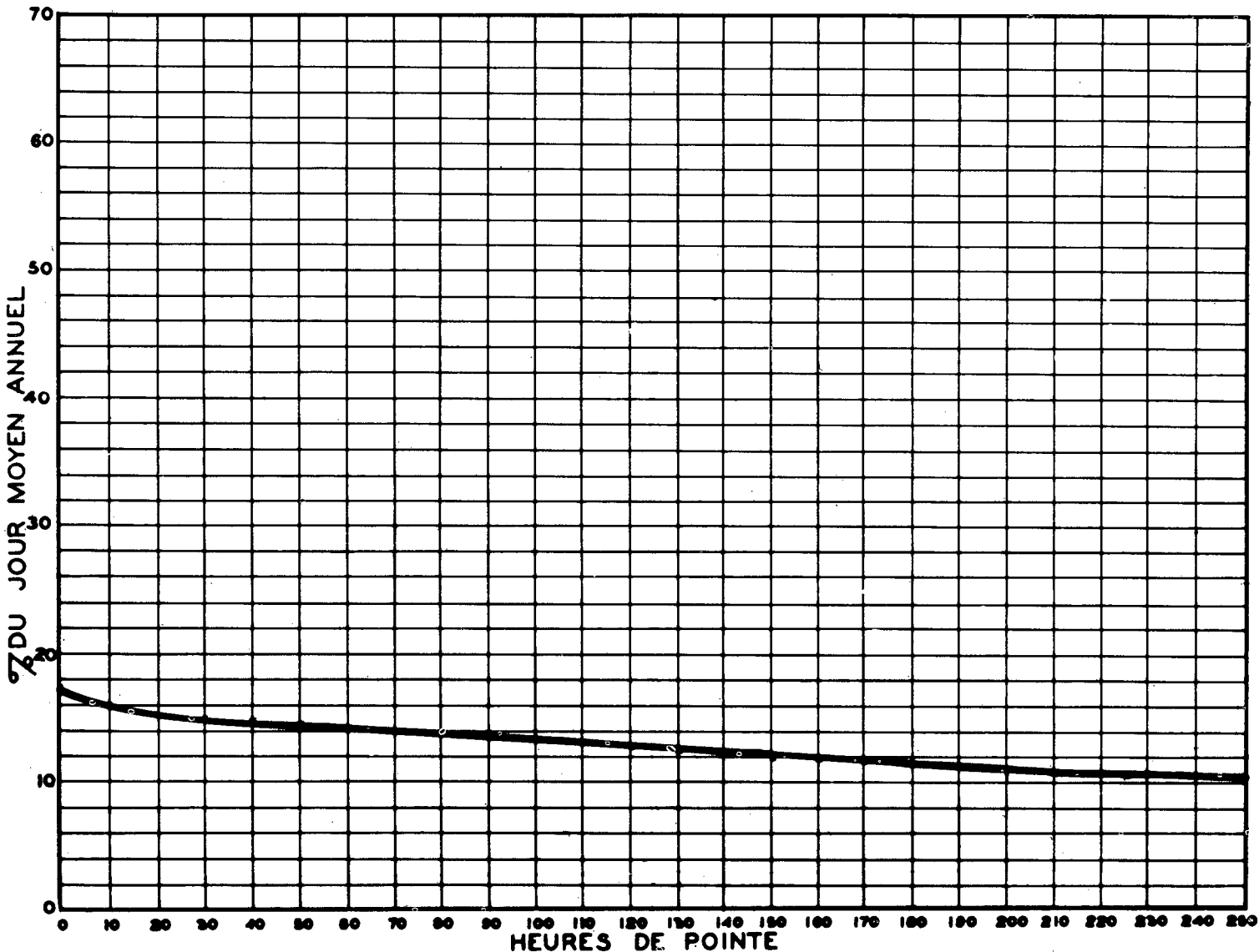
RELATION ENTRE LES HEURES DE POINTE ET LE JOUR MOYEN ANNUEL — STATION: ST-LUC ROUTE No 7-9-84
