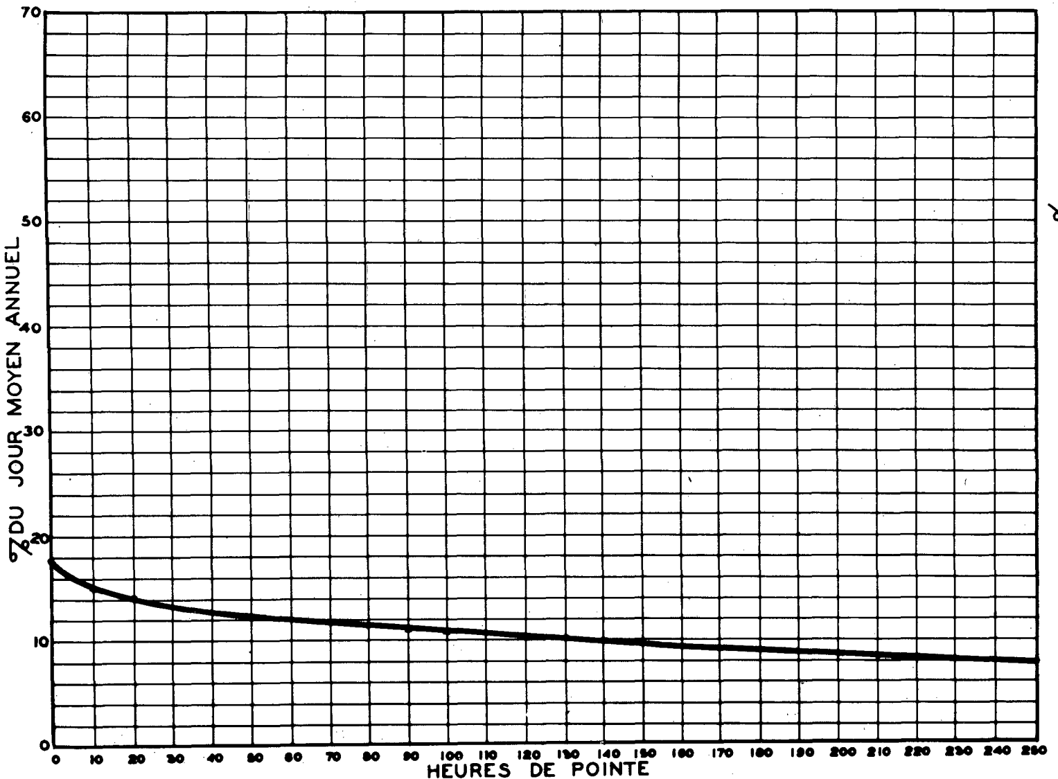
RELATION ENTRE LES HEURES DE POINTE ET LE JOUR MOYEN ANNUEL STATION: ST-JEROME ROUTE N° 54-7-3
