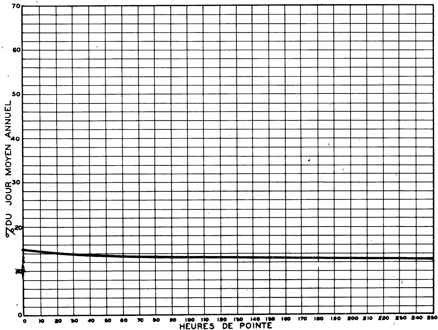
RELATION ENTRE LES HEURES DE POINTE ET LE JOUR MOYEN ANNUEL STATION: ST-LAMBERT voie nord. ROUTE N° 7-9-82
