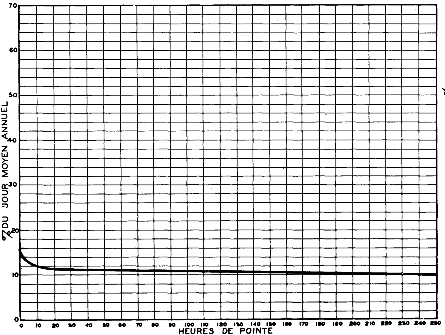
RELATION ENTRE LES HEURES DE POINTE ET LE JOUR MOYEN ANNUEL STATION: POINTE CLAIRE ROUTE N° 40-4-4R
