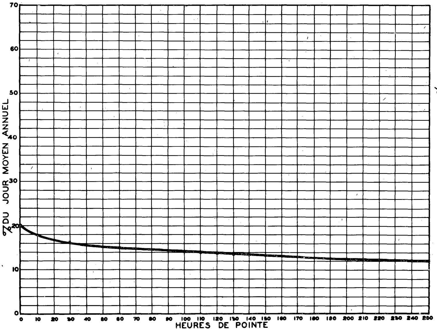
RELATION ENTRE LES HEURES DE POINTE ET LE JOUR MOYEN ANNUEL STATION: BOISCHATTEL ROUTE N°15-1-12
