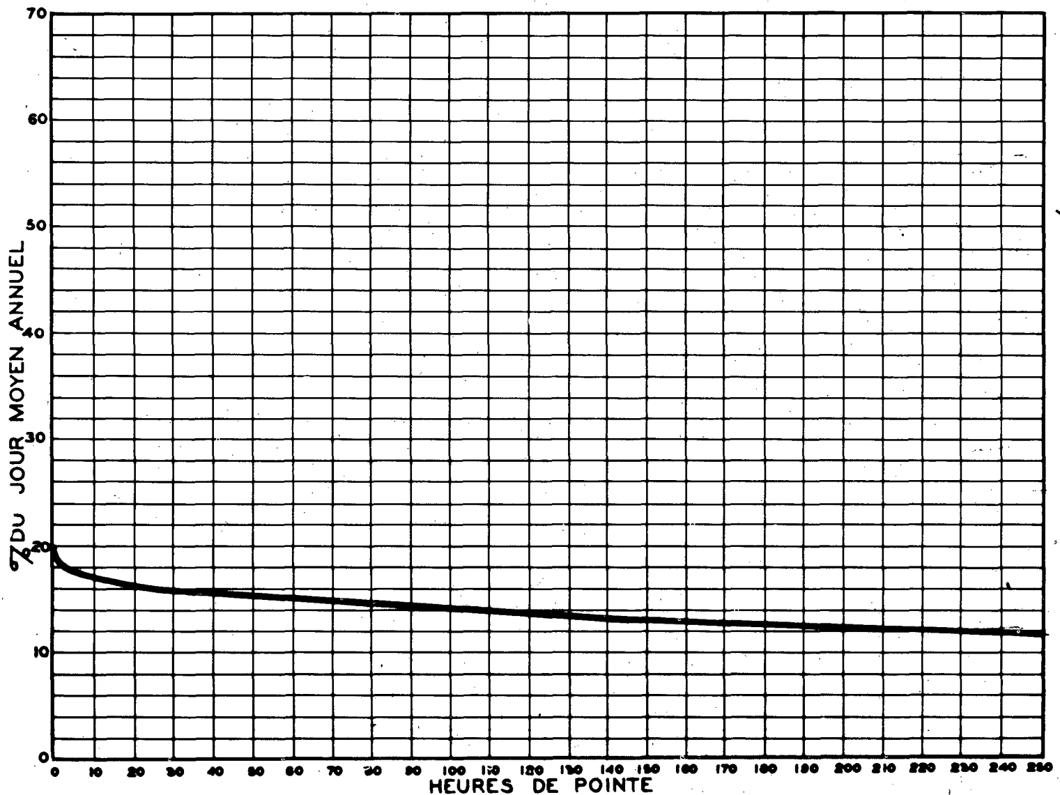
RELATION ENTRE LES HEURES DE POINTE ET LE JOUR MOYEN ANNUEL — STATION: ST-JANVIER ROUTE N°11-4-63
