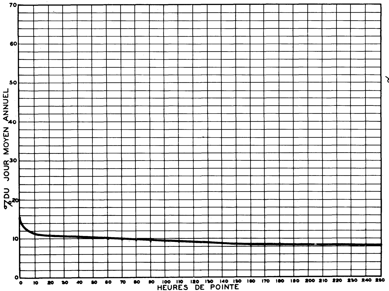
RELATION ENTRE LES HEURES DE POINTE ET LE JOUR MOYEN ANNUEL STATION: LAVAL ROUTE N° 8-4-55
