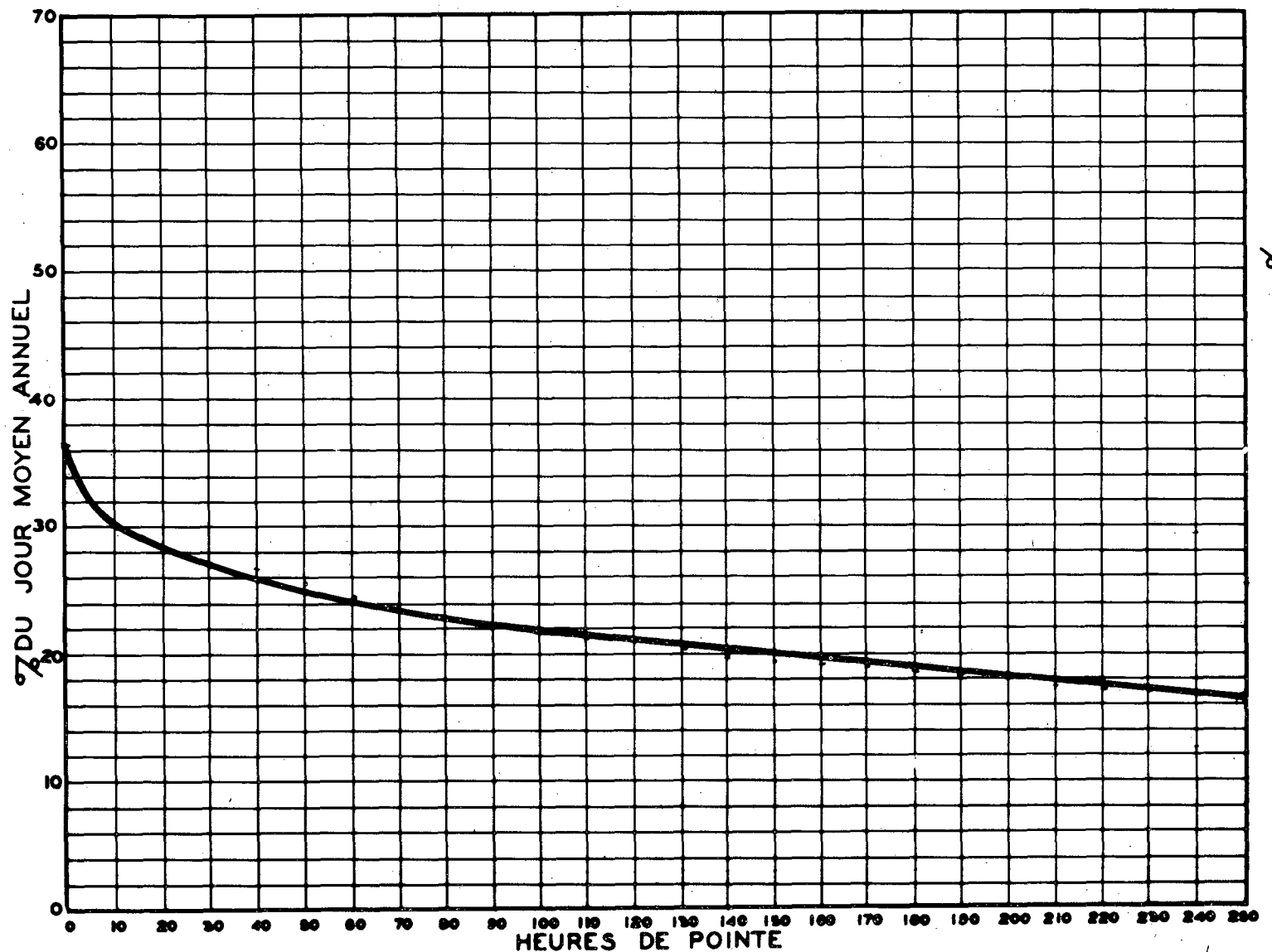
RELATION ENTRE LES HEURES DE POINTE ET LE JOUR MOYEN ANNUEL STATION: RIV. BEAUDETTE ROUTE N° 2-4-55
