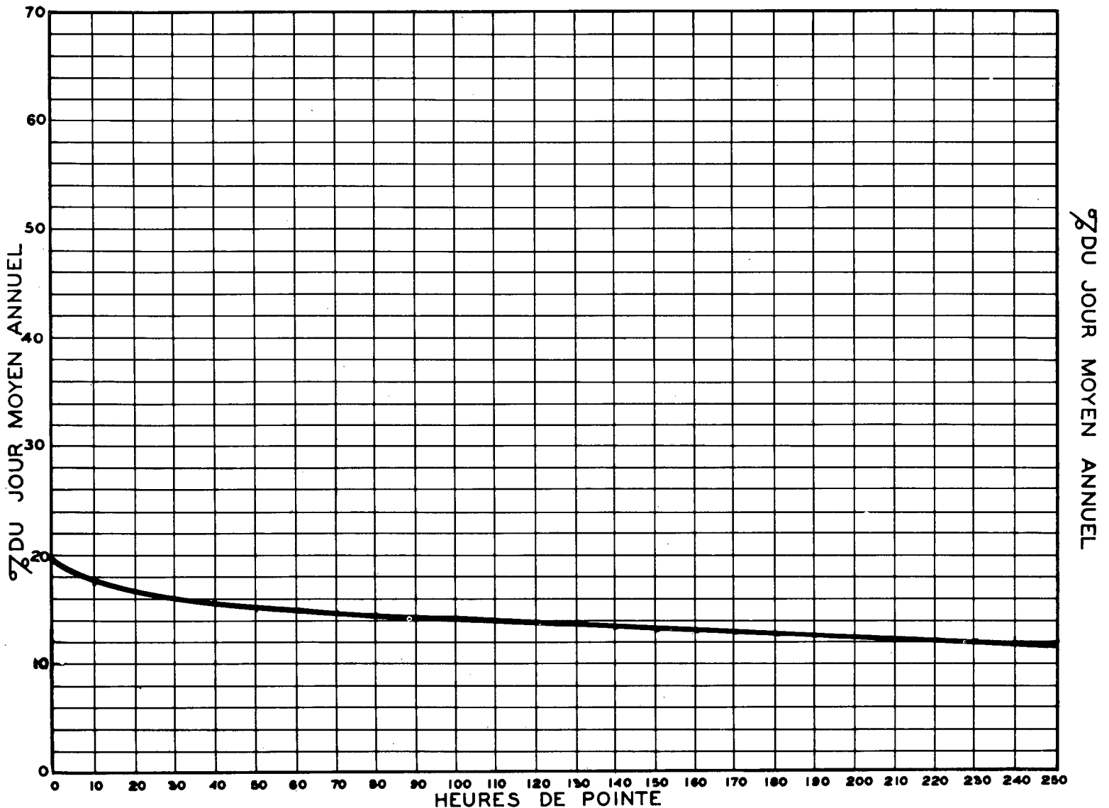
RELATION ENTRE LES HEURES DE POINTE ET LE JOUR MOYEN ANNUEL STATION: ANC-LORETTE ROUTE N° 2-1-7
