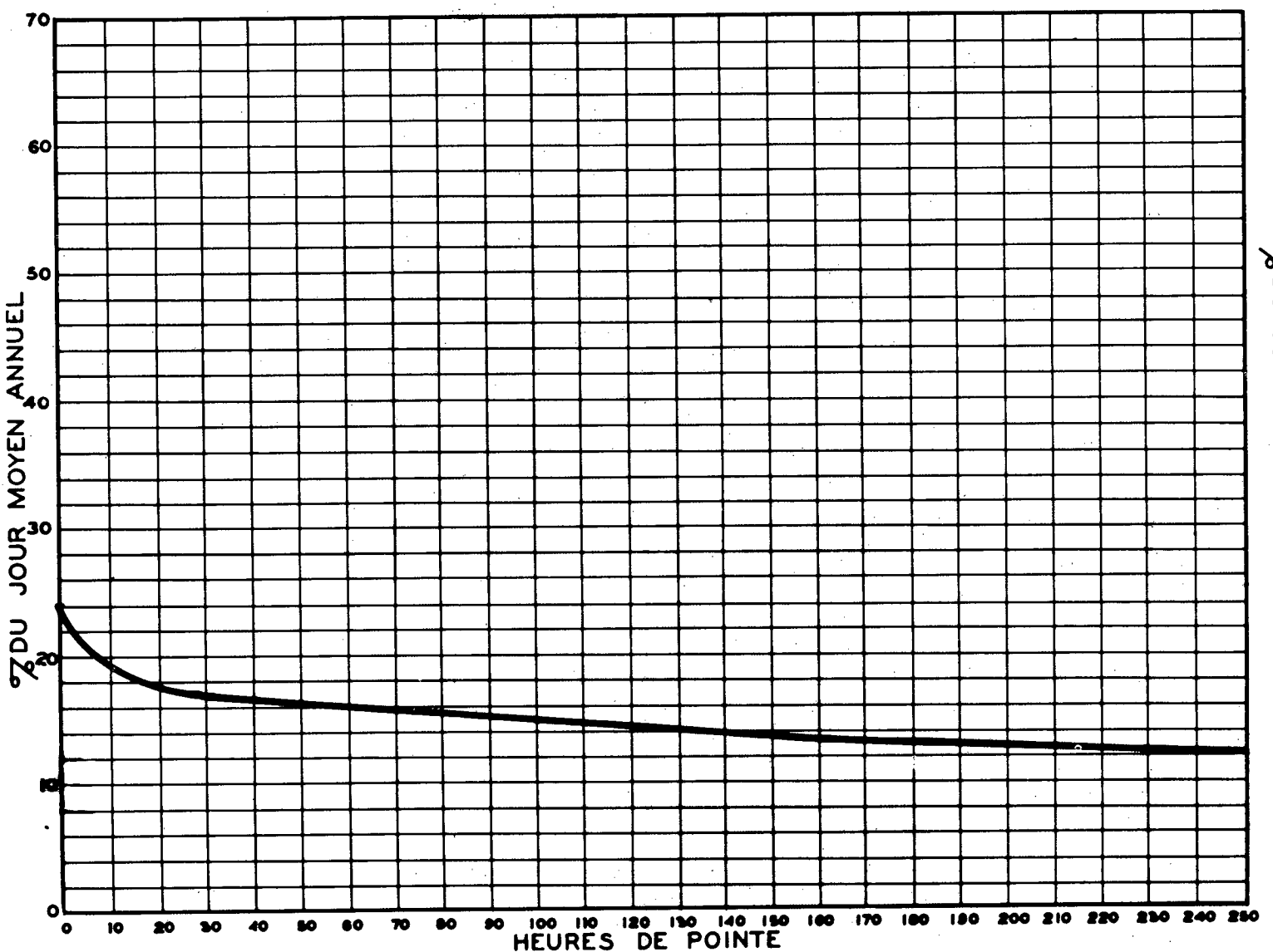
RELATION ENTRE LES HEURES DE POINTE ET LE JOUR MOYEN ANNUEL STATION: ROCK-ISLAND ROUTE N° 5-3-12
