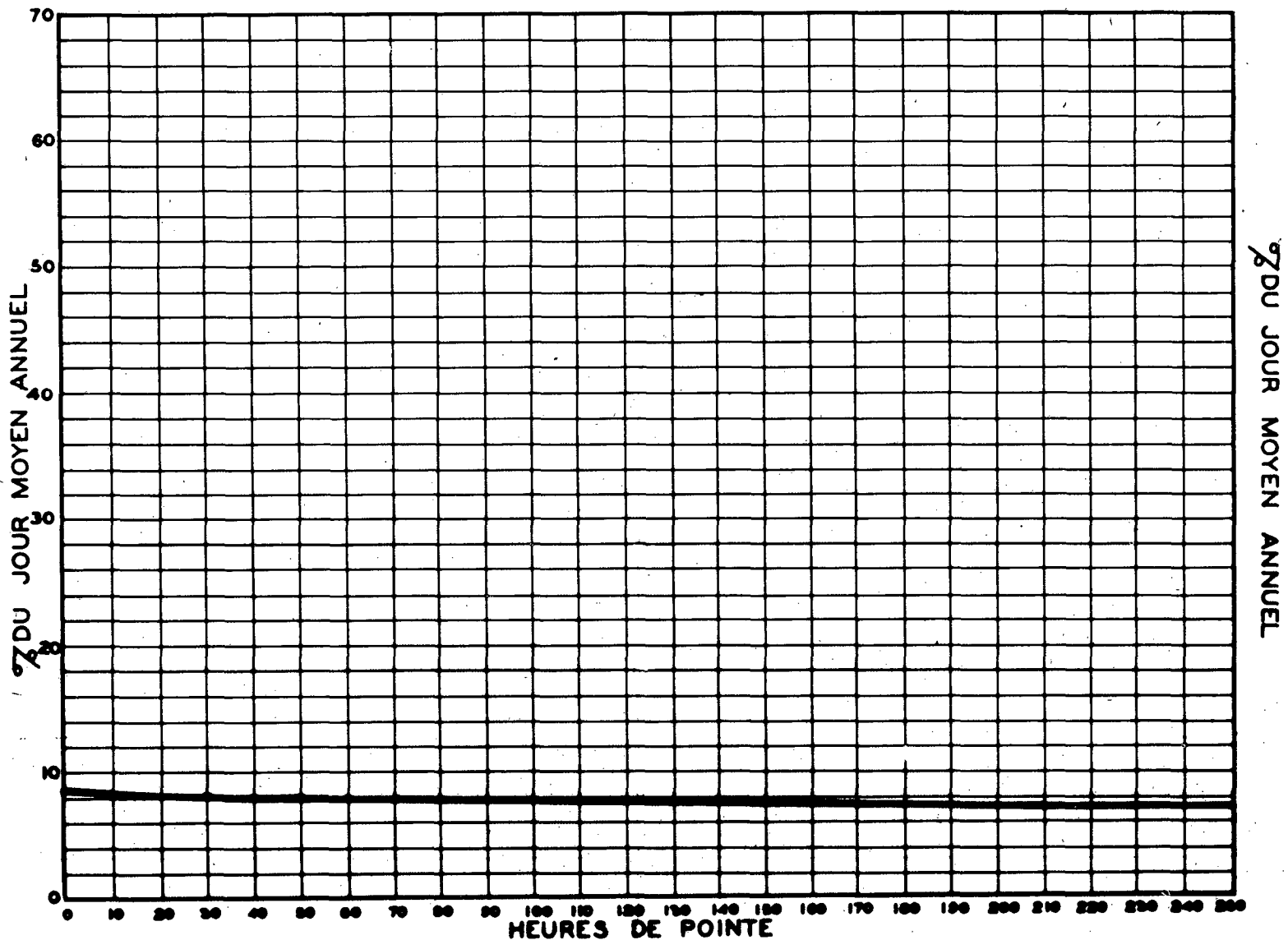
RELATION ENTRE LES HEURES DE POINTE ET LE JOUR MOYEN ANNUEL — STATION: MONTREAL (BOUL. DECARIE) 2VOIES ROUTE N°15-4-50 —
