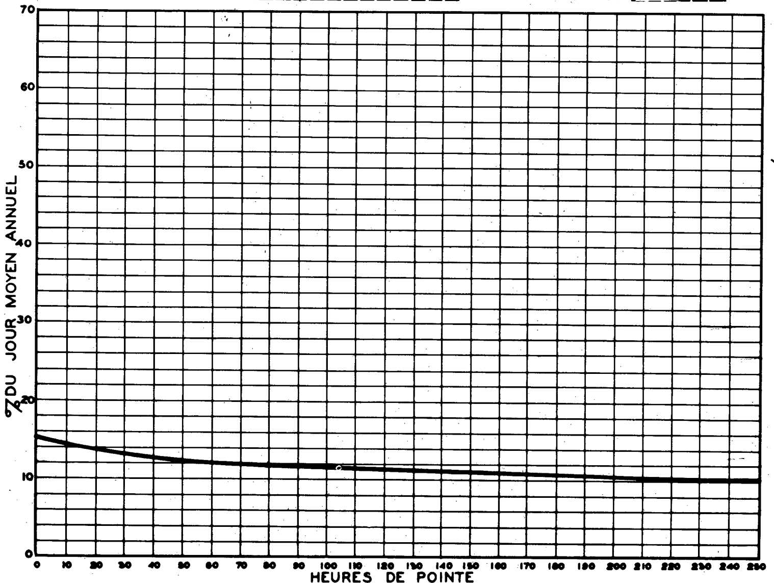
RELATION ENTRE LES HEURES DE POINTE ET LE JOUR MOYEN ANNUEL STATION: BOUCHERVILLE (PONT TUNEL) VOIE NORD ROUTE N°20-9-81
