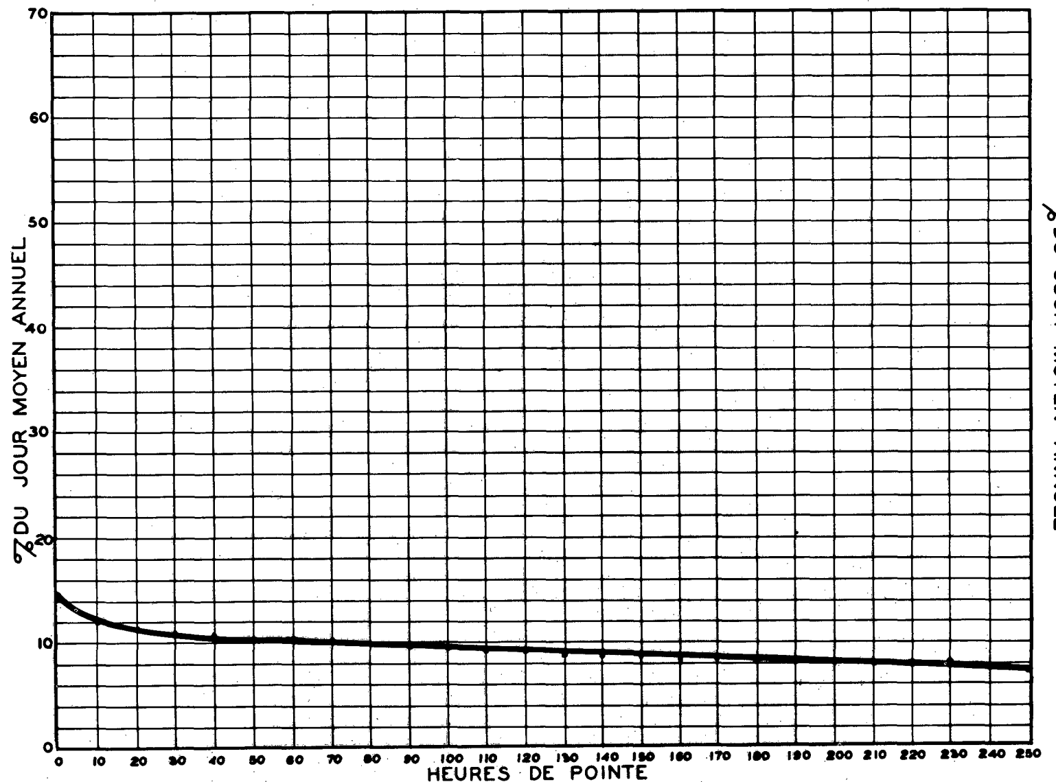
RELATION ENTRE LES HEURES DE POINTE ET LE JOUR MOYEN ANNUEL STATION: _____ TACHE _____ ROUTE N.R.S. 702 _____
