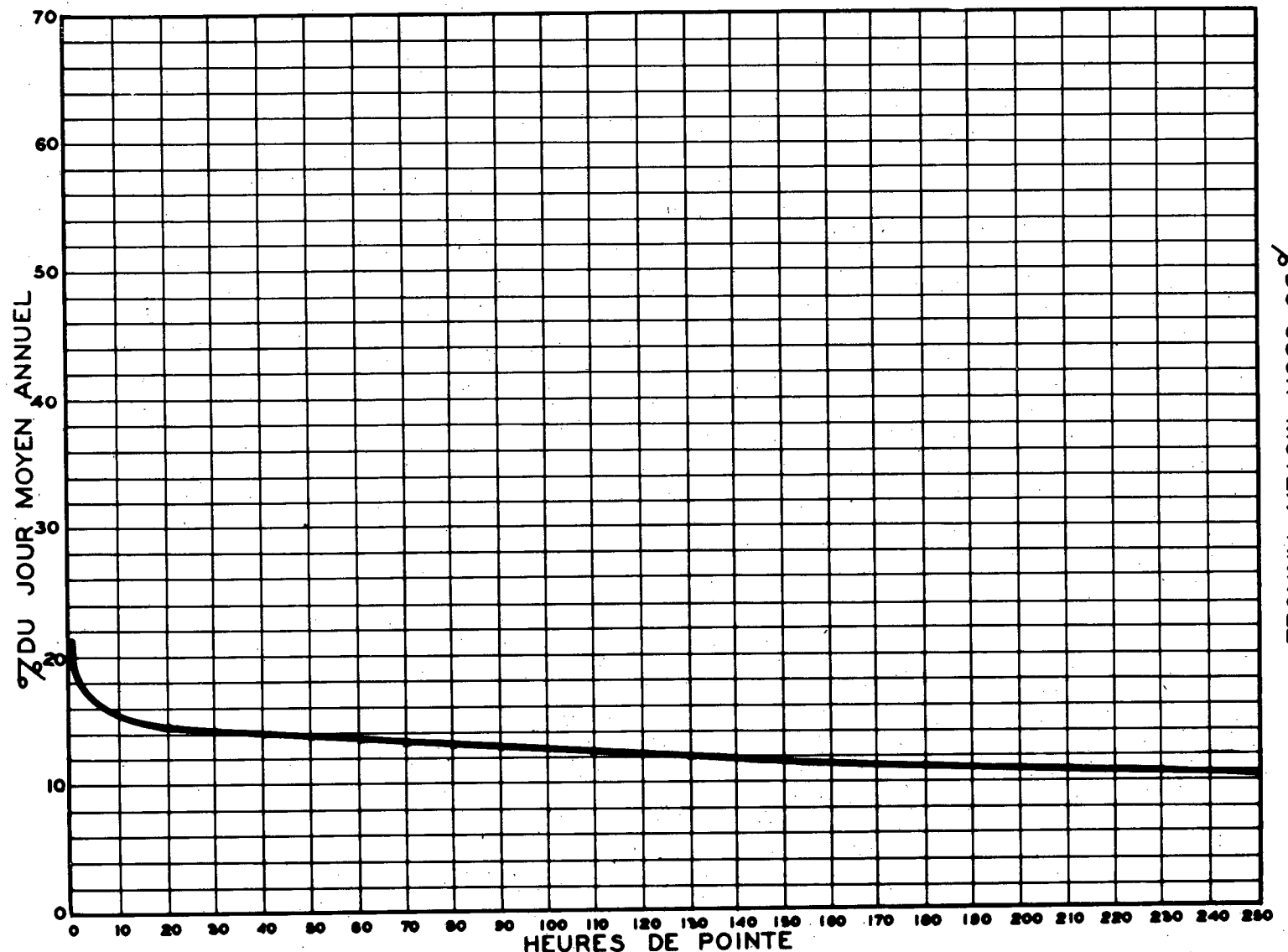
RELATION ENTRE LES HEURES DE POINTE ET LE JOUR MOYEN ANNUEL STATION: ST-ALBERT ROUTE No 20-8-14
