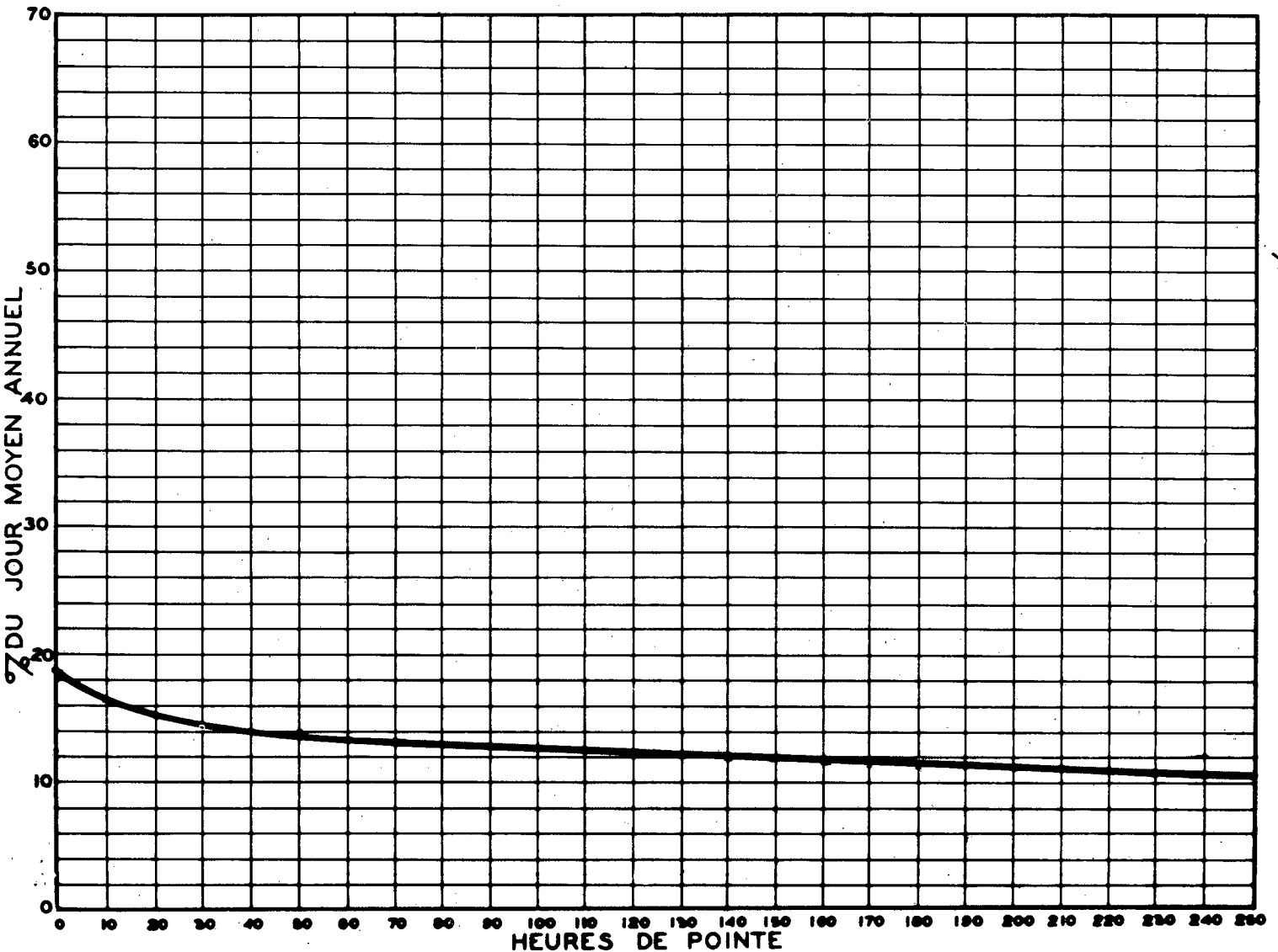
RELATION ENTRE LES HEURES DE POINTE ET LE JOUR MOYEN ANNUEL — STATION: ST-HENRI TAILLON ROUTE N° 55-7-2
