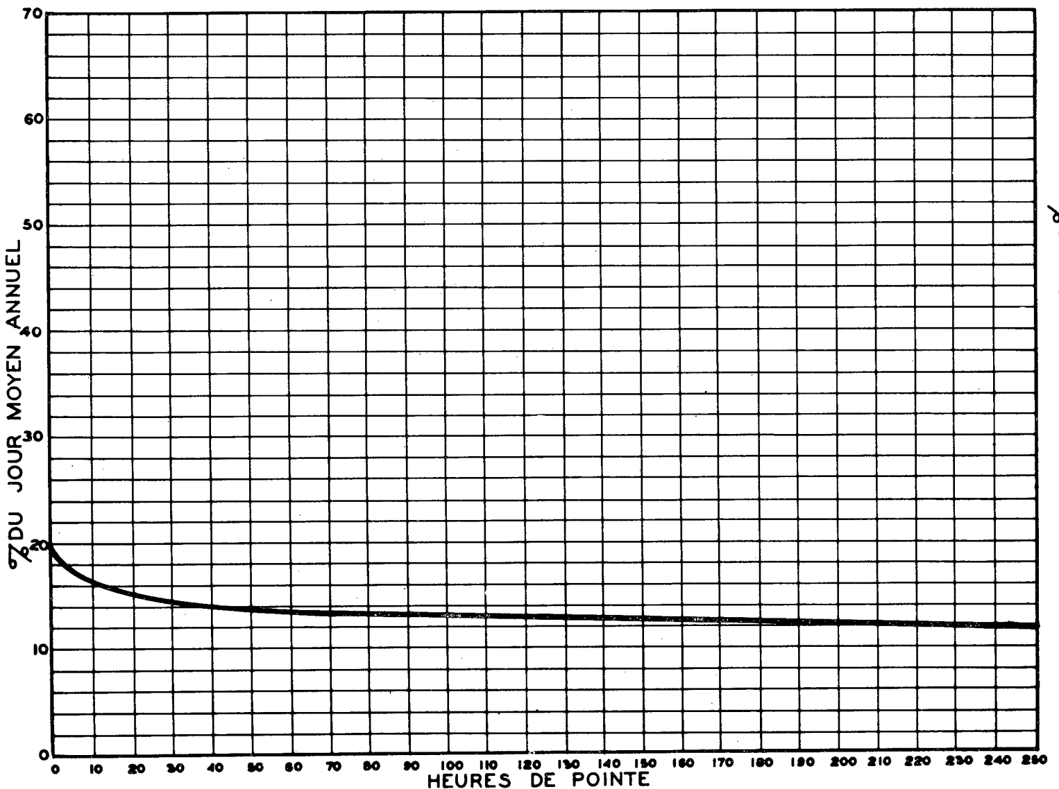
RELATION ENTRE LES HEURES DE POINTE ET LE JOUR MOYEN ANNUEL — STATION: PONT LE GARDEUR PONT AUX TREMBLES ROUTE N° 2-4-85 VOIE OUEST
