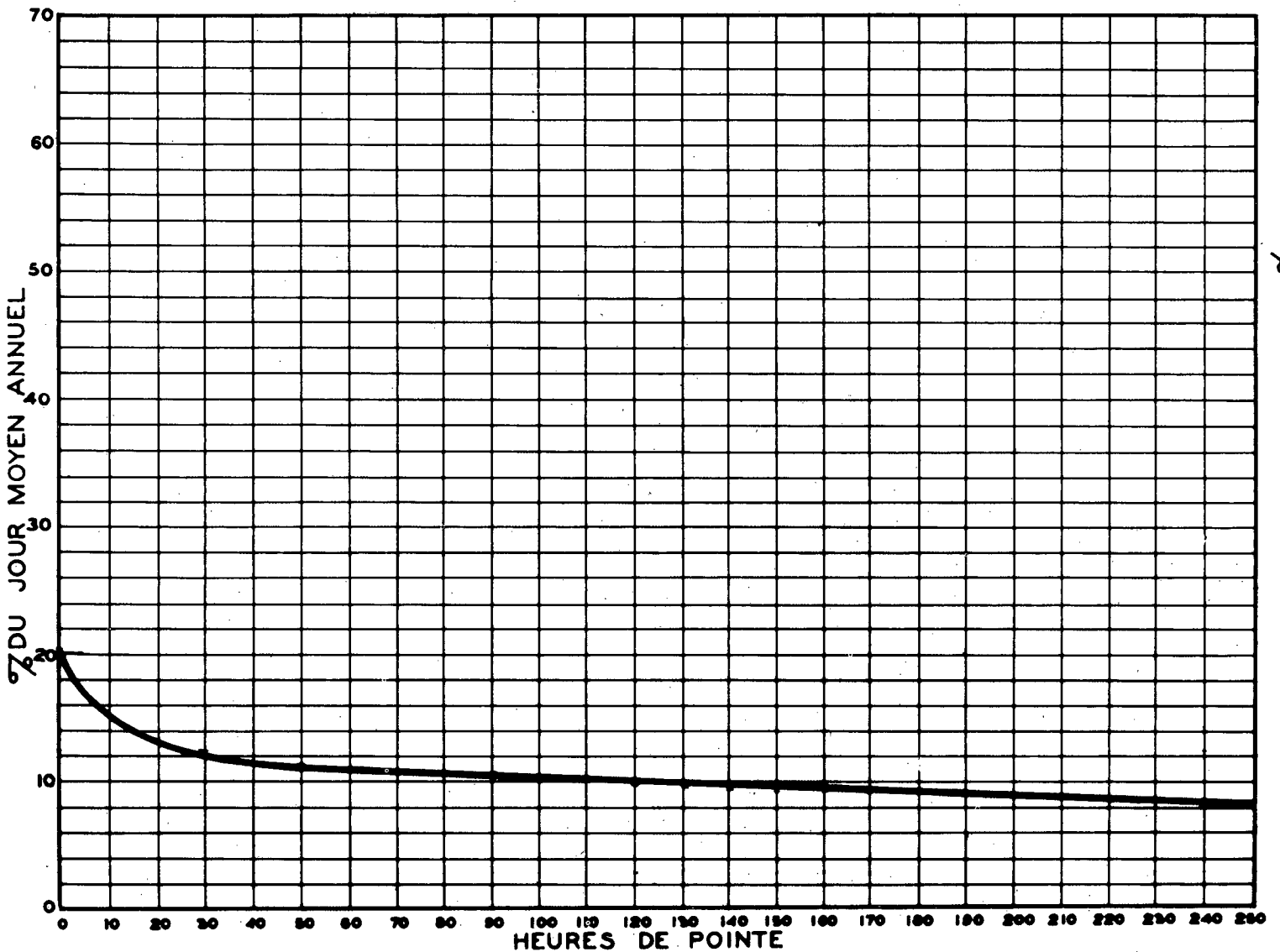
RELATION ENTRE LES HEURES DE POINTE ET LE JOUR MOYEN ANNUEL STATION: N.D. D'HEBERVILLE ROUTE N° 54-7-4
