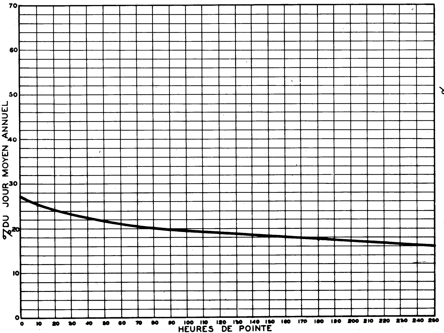
RELATION ENTRE LES HEURES DE POINTE ET LE JOUR MOYEN ANNUEL — STATION: ST-AGATHE ROUTE No 11-5-66
