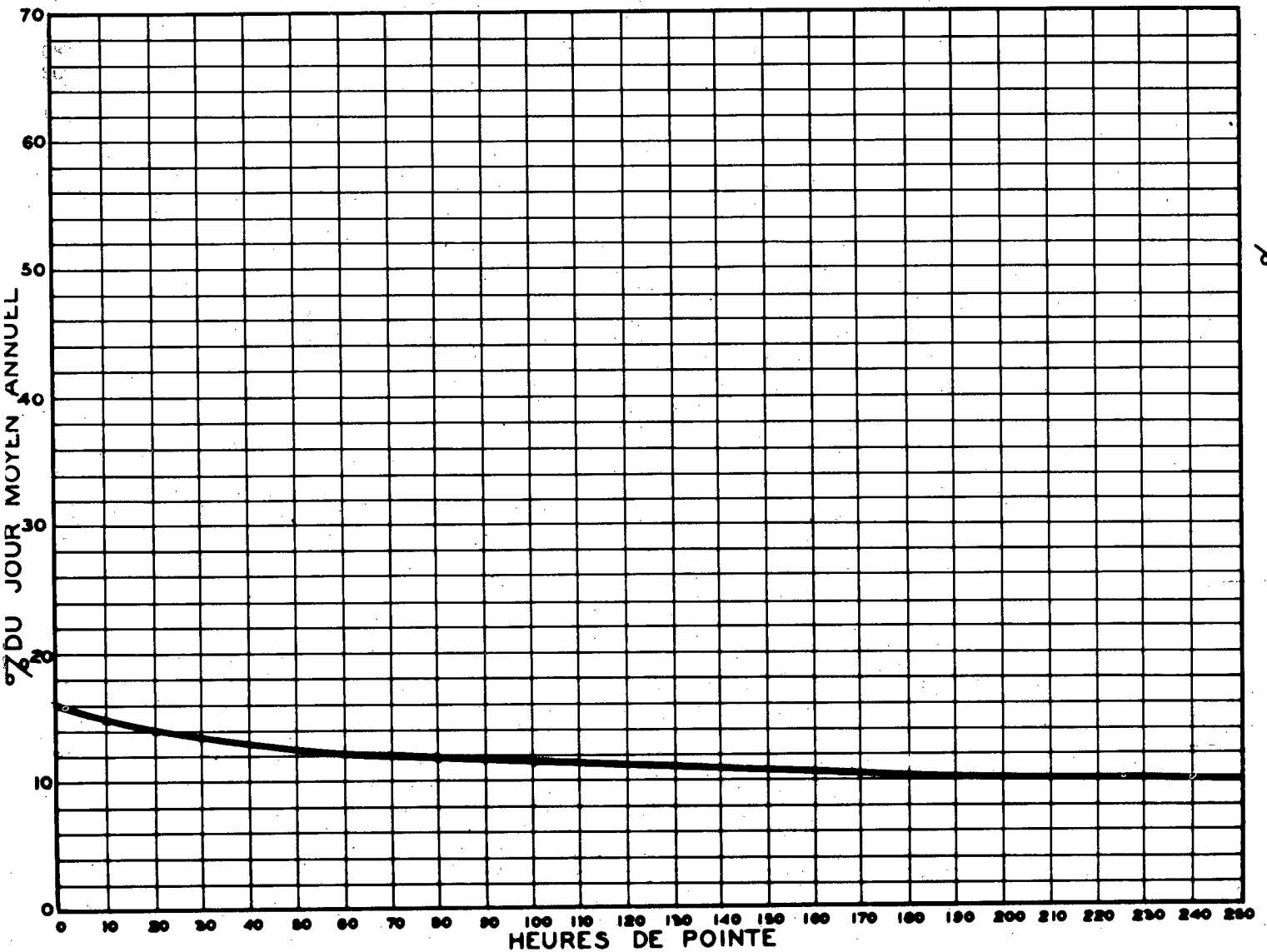
RELATION ENTRE LES HEURES DE POINTE ET LE JOUR MOYEN ANNUEL STATION: BOUCHERVILLE (PONT TUNEL) VOIE SUD ROUTE No 20-9-81
