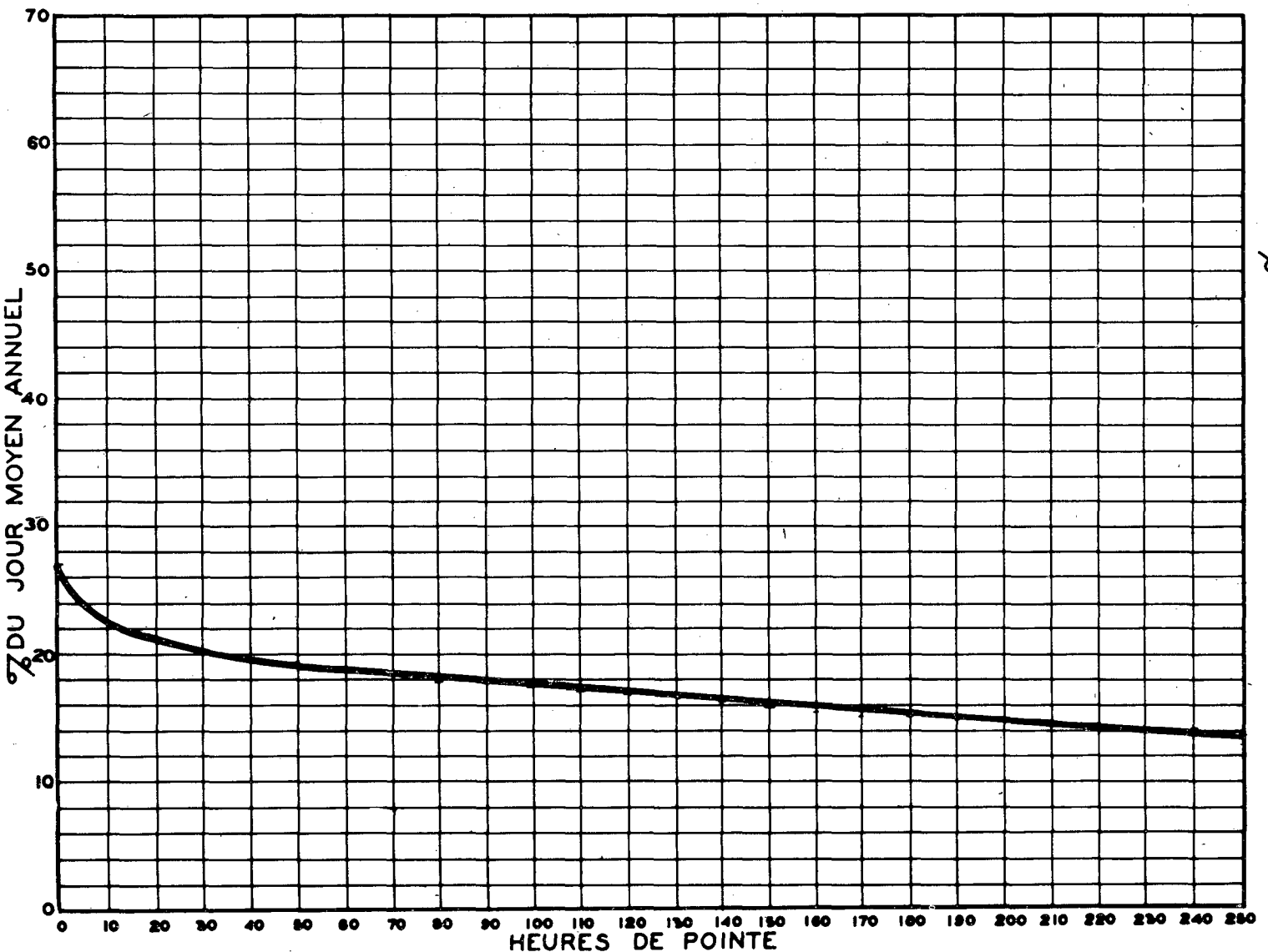
RELATION ENTRE LES HEURES DE POINTE ET LE JOUR MOYEN ANNUEL — STATION: ST-JOACHIM ROUTE N° 15-4-13
