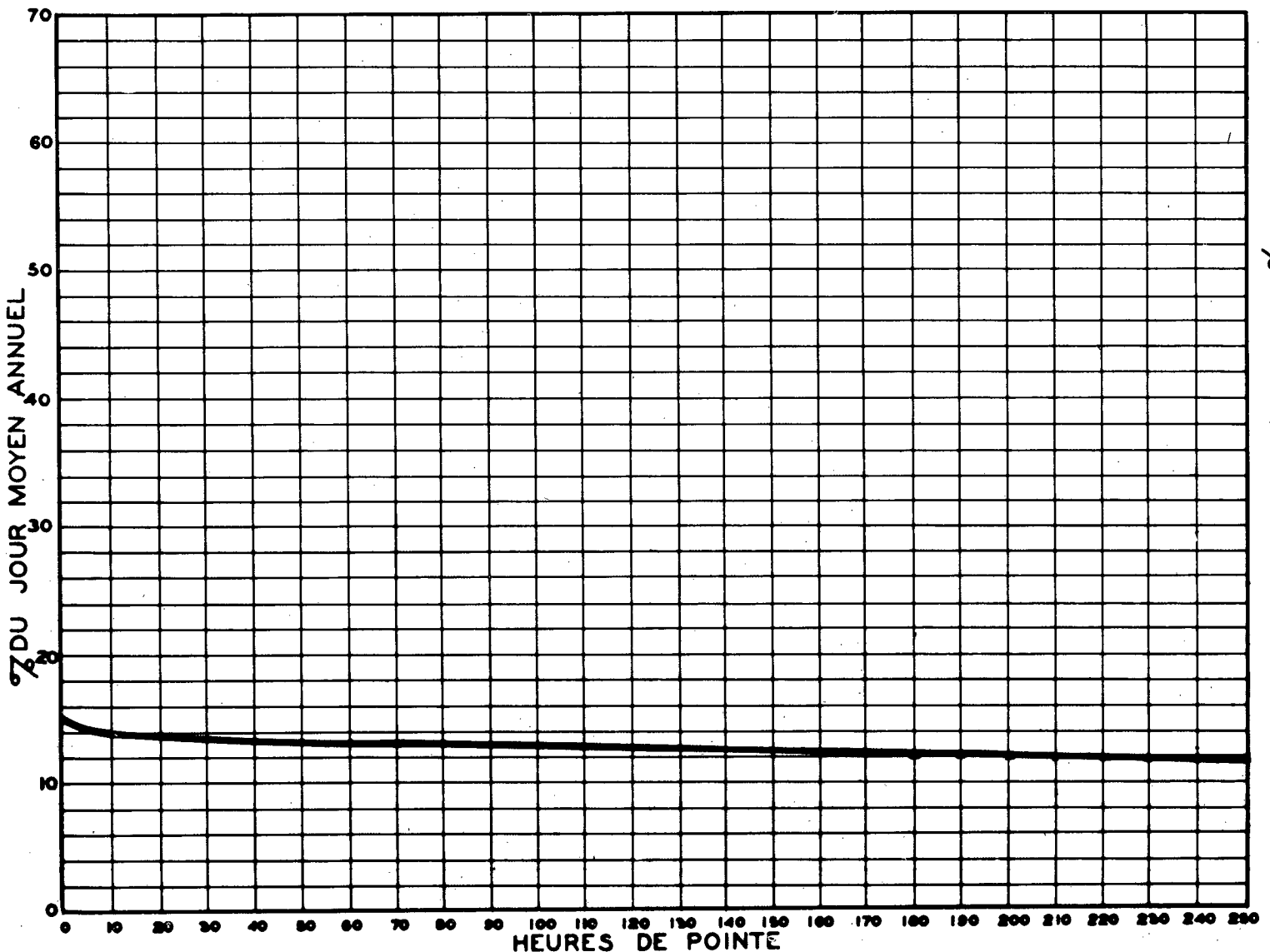
RELATION ENTRE LES HEURES DE POINTE ET LE JOUR MOYEN ANNUEL — STATION LONGUEUIL ROUTE N° VOIE SUD 9-9-80
