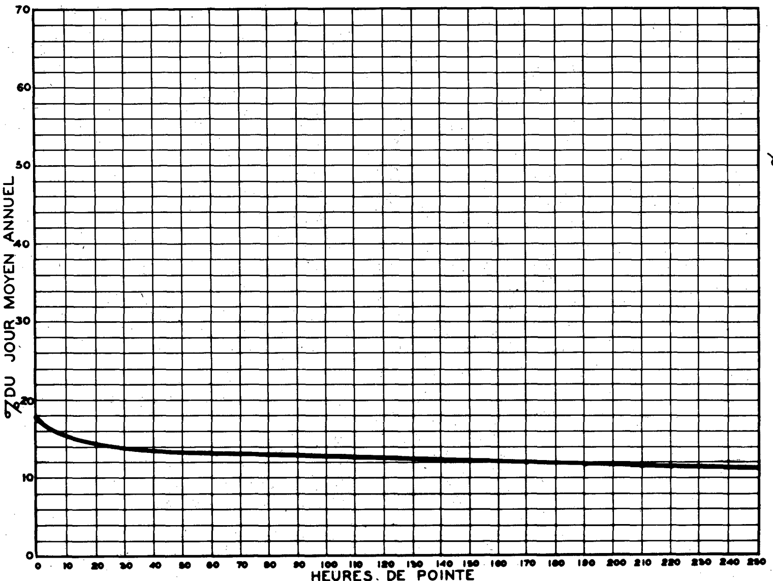
RELATION ENTRE LES HEURES DE POINTE ET LE JOUR MOYEN ANNUEL STATION: ST-NICOLAS 2 voies ROUTE N° 9-1-11
