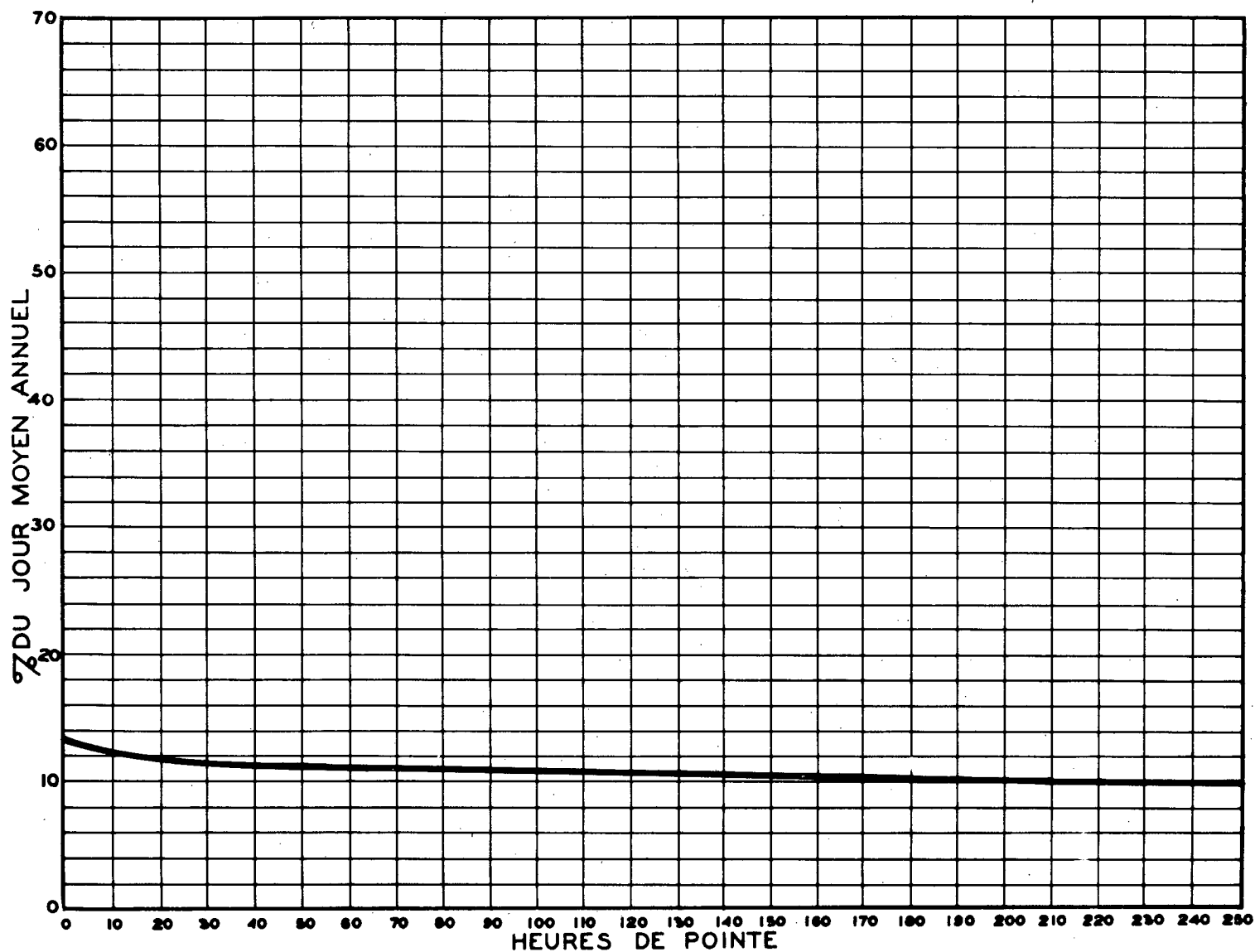
RELATION ENTRE LES HEURES DE POINTE ET LE JOUR MOYEN ANNUEL — STATION: BOUCHERVILLE (PONT TUNNEL) 2 VOIES ROUTE N° 20-9-81
