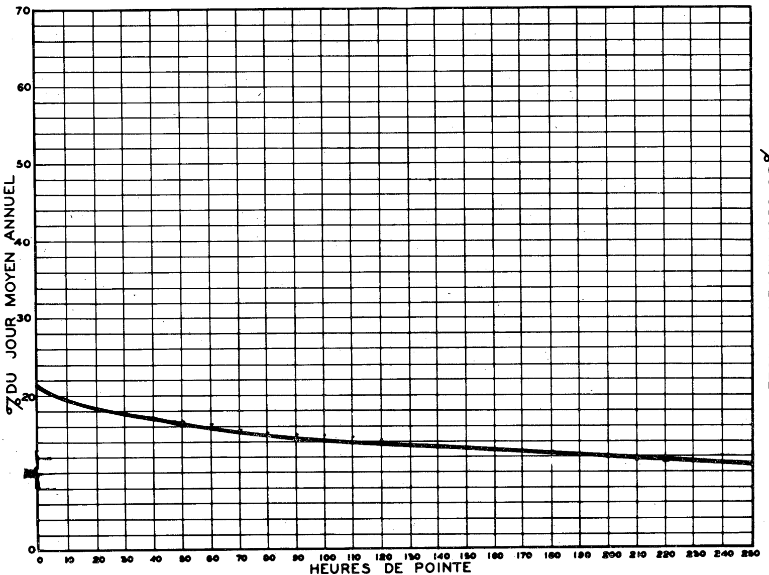
RELATION ENTRE LES HEURES DE POINTE ET LE JOUR MOYEN ANNUEL — STATION: ST-GREGOIRE ROUTE No 3-8-5
