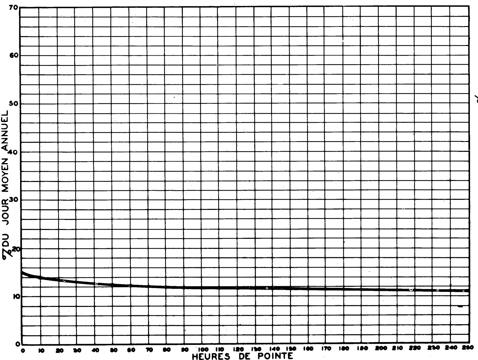
RELATION ENTRE LES HEURES DE POINTE ET LE JOUR MOYEN ANNUEL — STATION: LONGUEUIL ROUTE N° VOIE NORD 9-9-80
