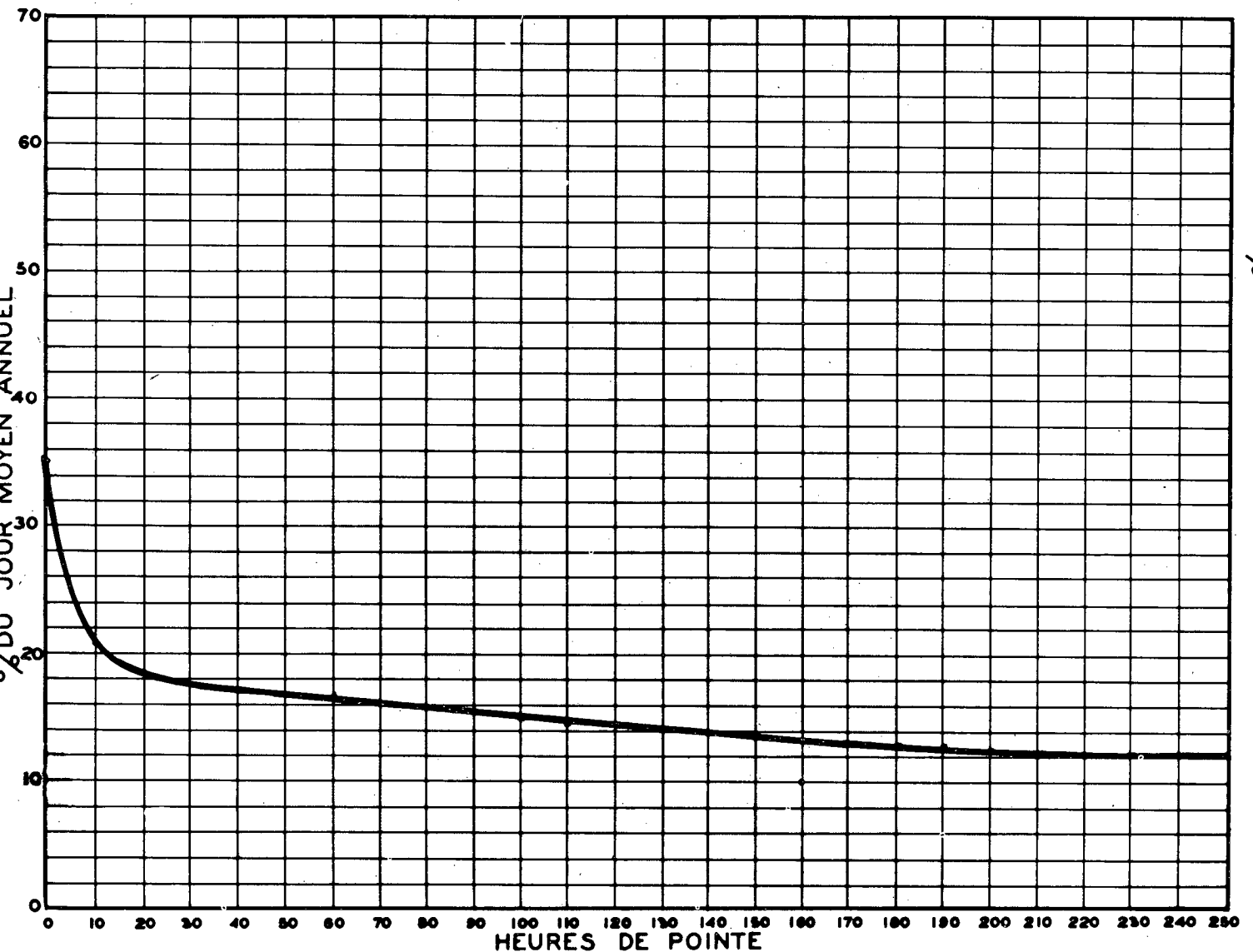
RELATION ENTRE LES HEURES DE POINTE ET LE JOUR MOYEN ANNUEL STATION: BATISCAN ROUTE N° 2-1-9
