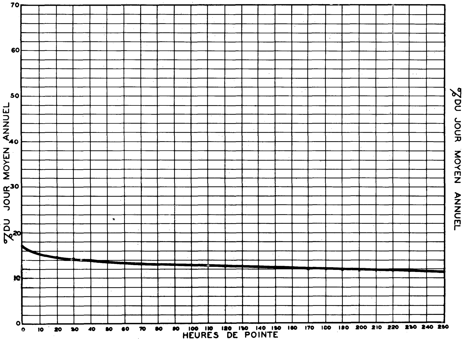
RELATION ENTRE LES HEURES DE POINTE ET LE JOUR MOYEN ANNUEL — STATION: ST-PATRICE ROUTE No 10-2-2,
