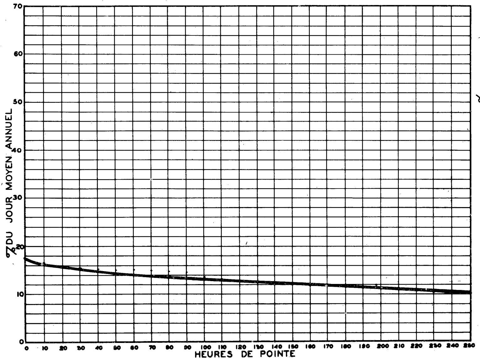
RELATION ENTRE LES HEURES DE POINTE ET LE JOUR MOYEN ANNUEL STATION: LA SALLE VOIE EST ROUTE N° 4-4-83
