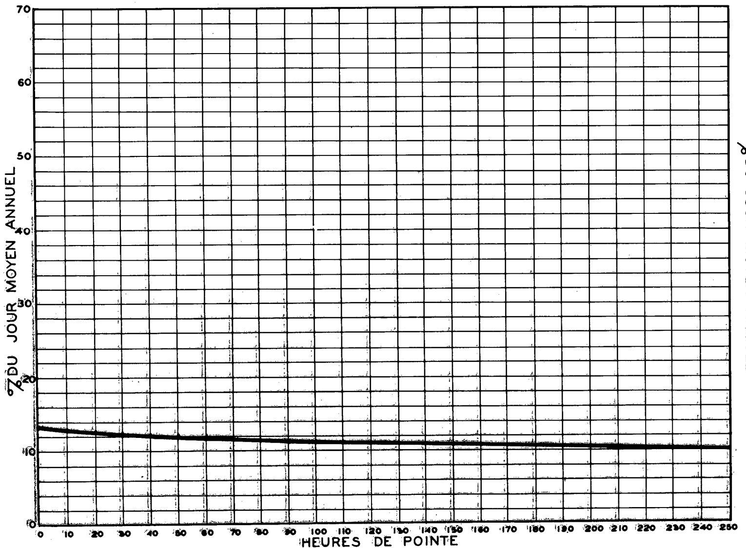
RELATION ENTRE LES HEURES DE POINTE ET LE JOUR MOYEN ANNUEL STATION: CHARLESBOURG ROUTE N° R.S.178
