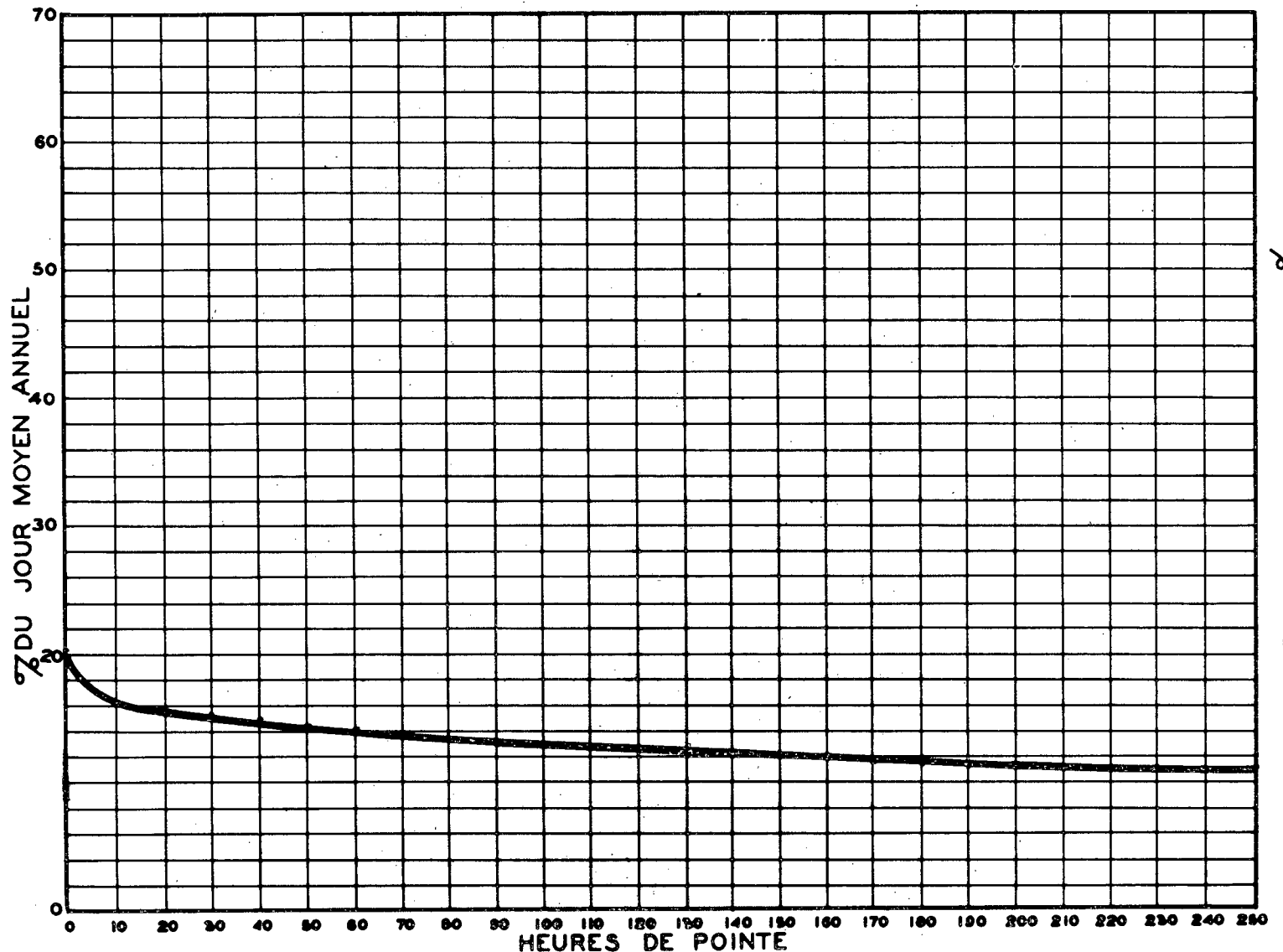
RELATION ENTRE LES HEURES DE POINTE ET LE JOUR MOYEN ANNUEL STATION: SAINT-ETIENNE ROUTE N° 5-117
