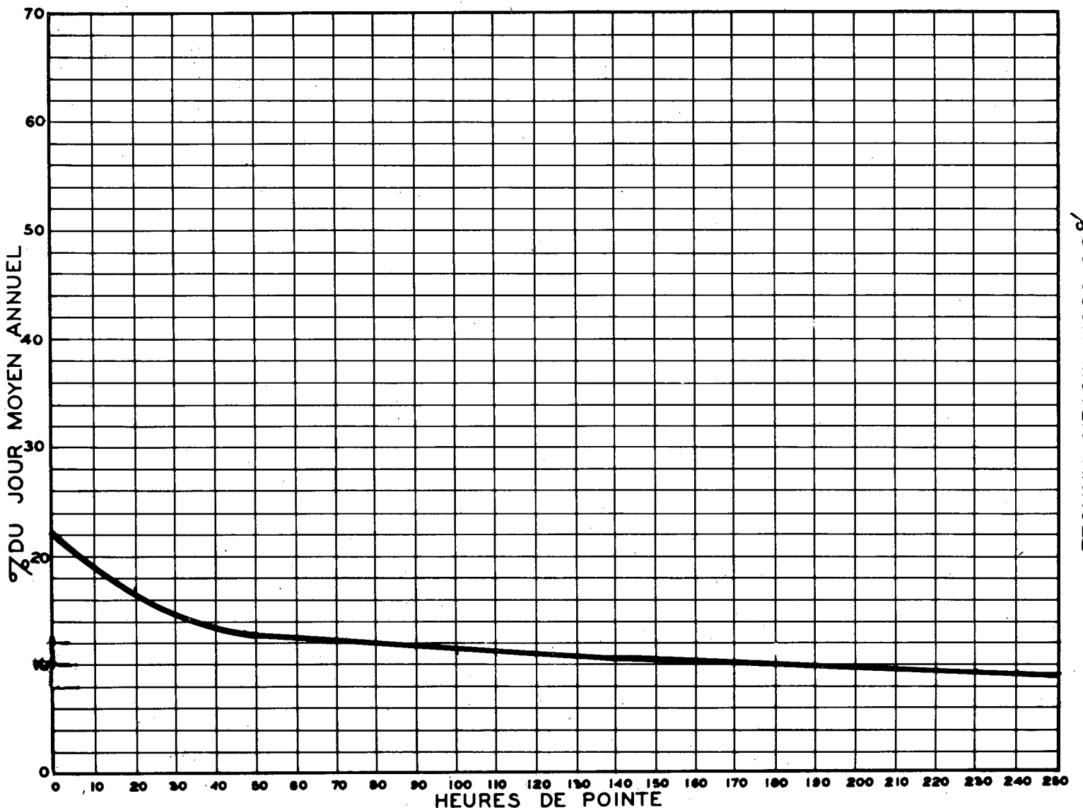
RELATION ENTRE LES HEURES DE POINTE ET LE JOUR MOYEN ANNUEL STATION: STE-ROSE-DU-DEGELEE ROUTE N° 2-2-4
