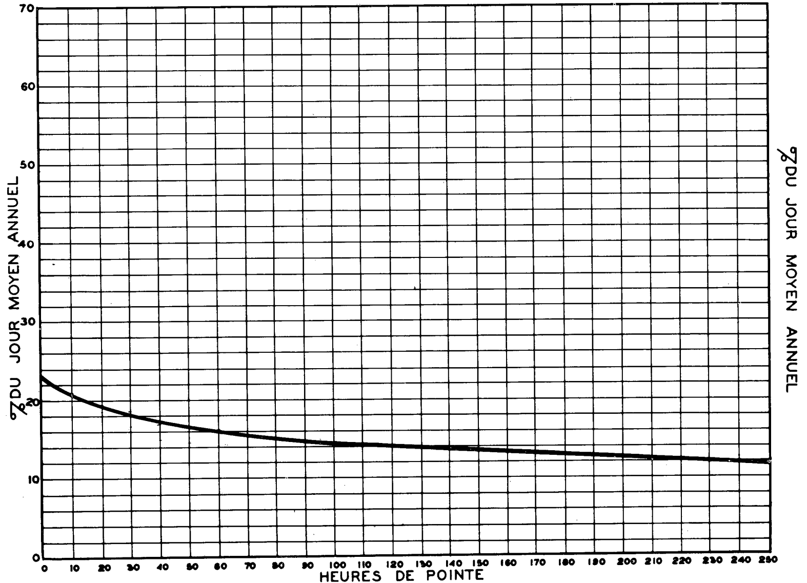
RELATION ENTRE LES HEURES DE POINTE ET LE JOUR MOYEN ANNUEL STATION: MASSON ROUTE N° 8-5-58
