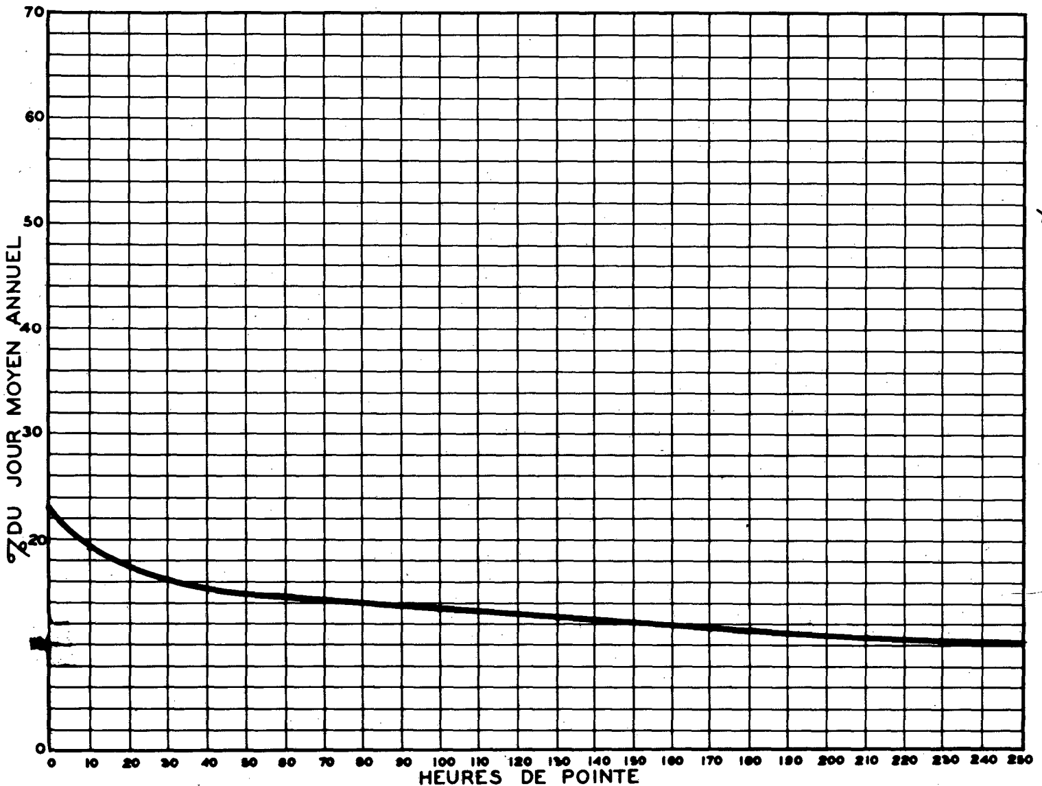
RELATION ENTRE LES HEURES DE POINTE ET LE JOUR MOYEN ANNUEL — STATION: ST-FREDERIC ROUTE No 1-3-1
