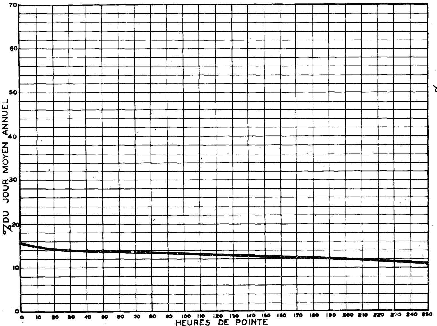
RELATION ENTRE LES HEURES DE POINTE ET LE JOUR MOYEN ANNUEL STATION: LASALLE VOIE OUEST ROUTE N° 4-4-83
