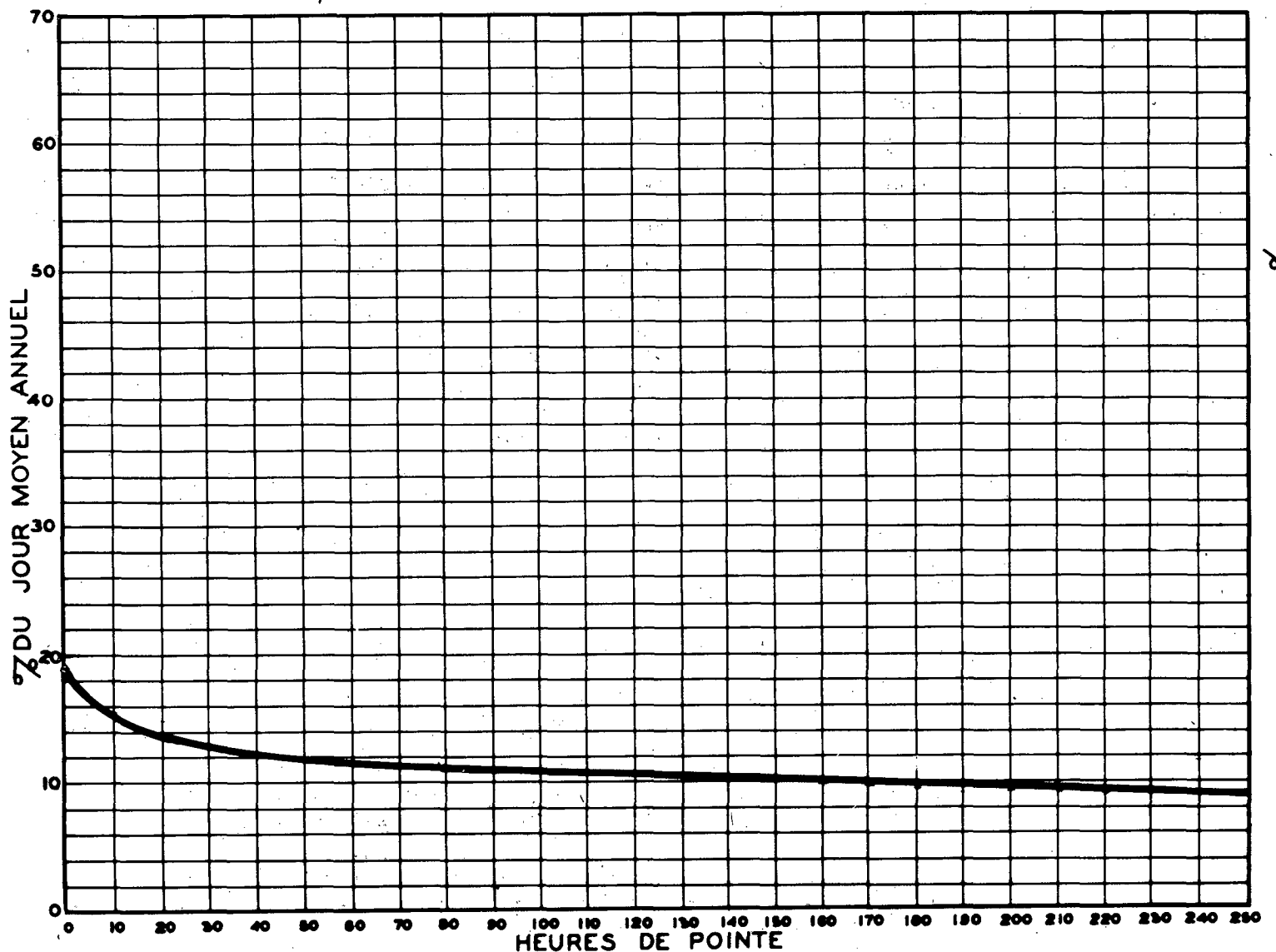
RELATION ENTRE LES HEURES DE POINTE ET LE JOUR MOYEN ANNUEL STATION: SAINT-NICOLAS VOIE SUD ROUTE N° 9-1-11
