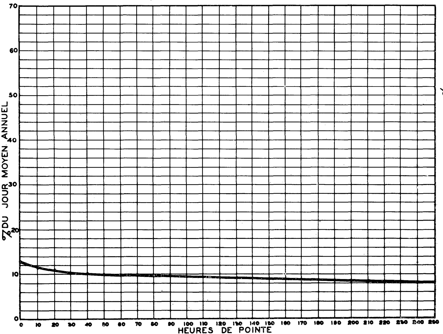
RELATION ENTRE LES HEURES DE POINTE ET LE JOUR MOYEN ANNUEL — STATION: PONT LE GARDEUR POINTE AUX TREMBLES ROUTE N° 2-4-85 2 VOIES
