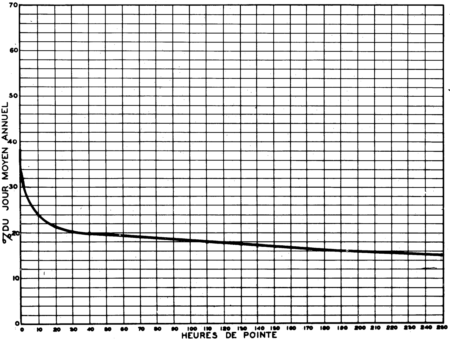
RELATION ENTRE LES HEURES DE POINTE ET LE JOUR MOYEN ANNUEL STATION: ST-ADELE ROUTE N° 11-4-65
