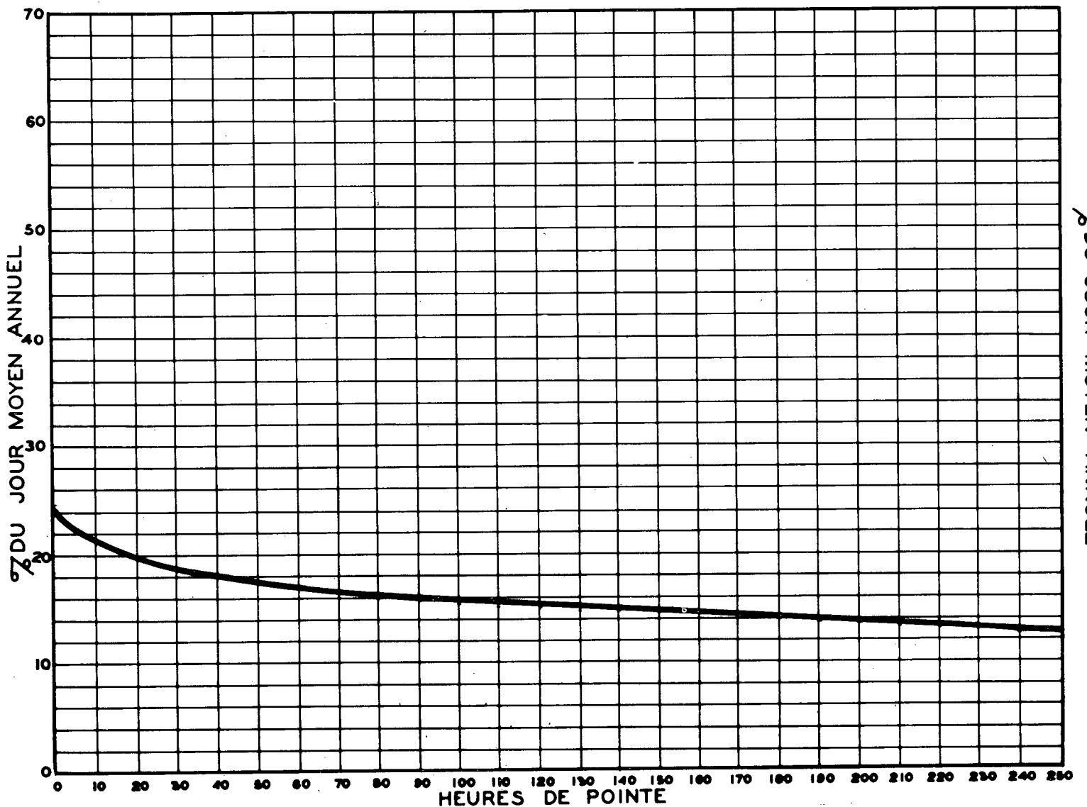
RELATION ENTRE LES HEURES DE POINTE ET LE JOUR MOYEN ANNUEL STATION: AYLMER ROUTE N° 8-5-59
