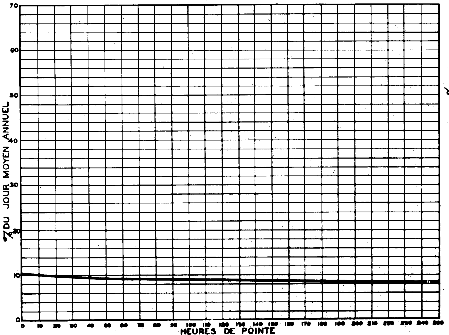
RELATION ENTRE LES HEURES DE POINTE ET LE JOUR MOYEN ANNUEL — STATION MONTREAL (BOUL. DECARIE) ROUTE N° VOIE OUEST 15-4-50
