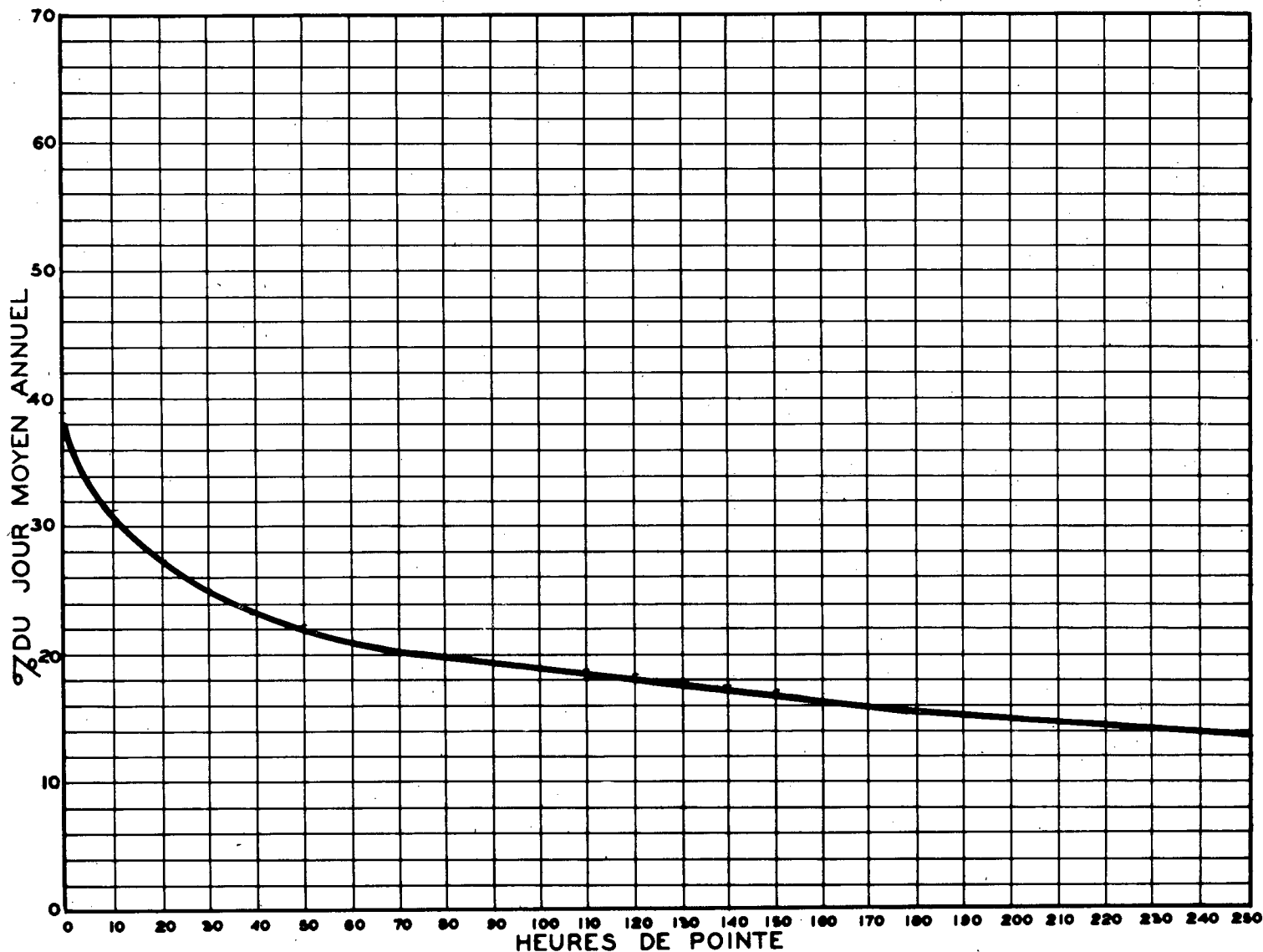
RELATION ENTRE LES HEURES DE POINTE ET LE JOUR MOYEN ANNUEL STATION: GRANDS-PILES ROUTE N°19-1-14
