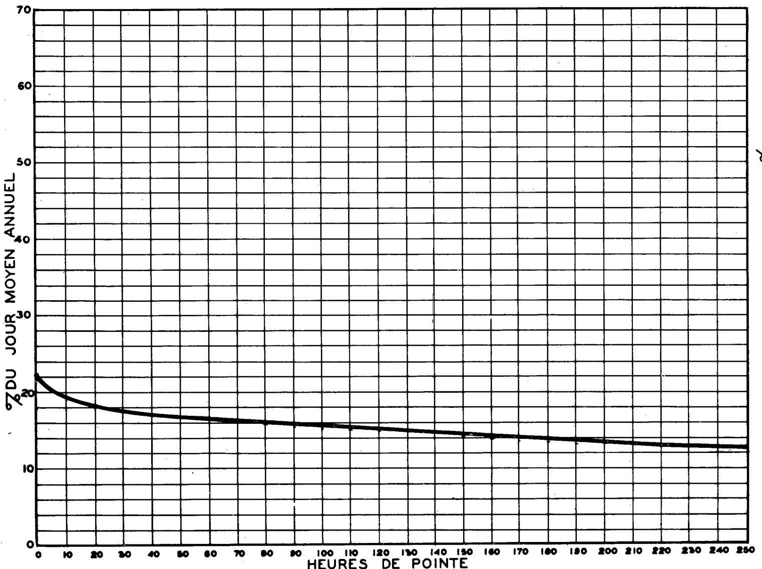
RELATION ENTRE LES HEURES DE POINTE ET LE JOUR MOYEN ANNUEL — STATION: SABREVOIS 2voies ROUTE N° 7-9-64
