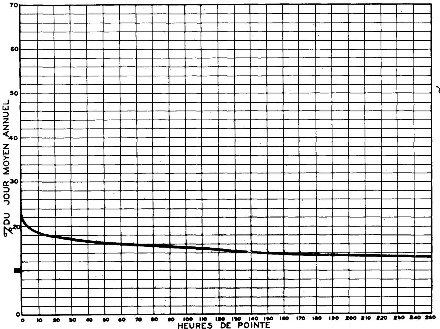
RELATION ENTRE LES HEURES DE POINTE ET LE JOUR MOYEN ANNUEL — STATION: STANSTEAD ROUTE N° 5-3-9
