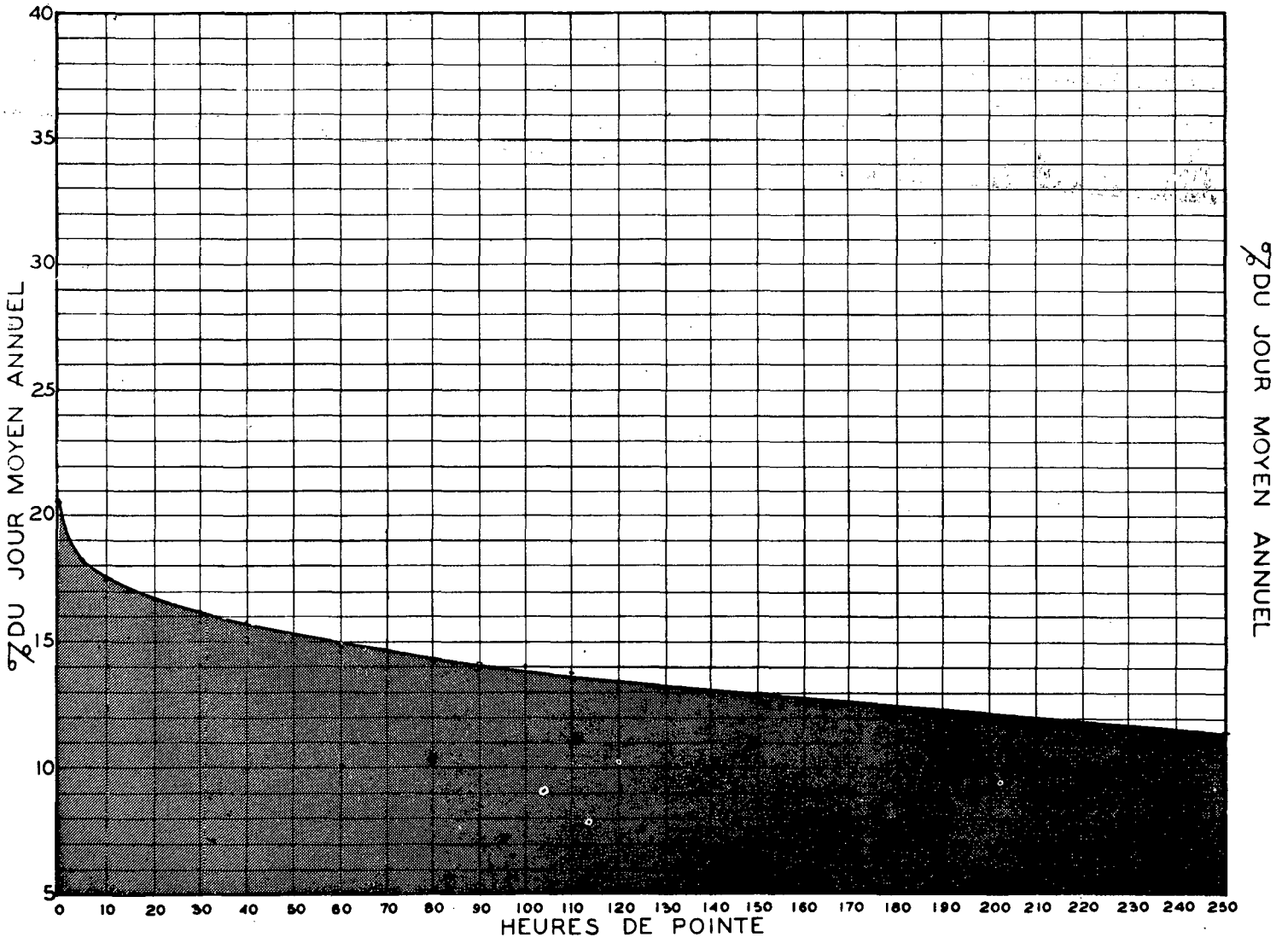
RELATION ENTRE LES HEURES DE POINTE ET LE JOUR MOYEN ANNUEL STATION ANCIENNE LORETTE ROUTE N° 2
