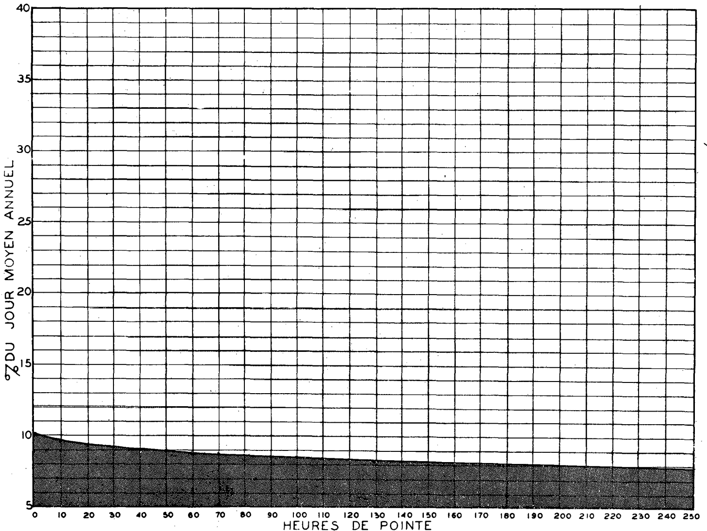
RELATION ENTRE LES HEURES DE POINTE ET LE JOUR MOYEN ANNUEL STATION: ST-HUBERT 2 VOIES ROUTE N° 9
