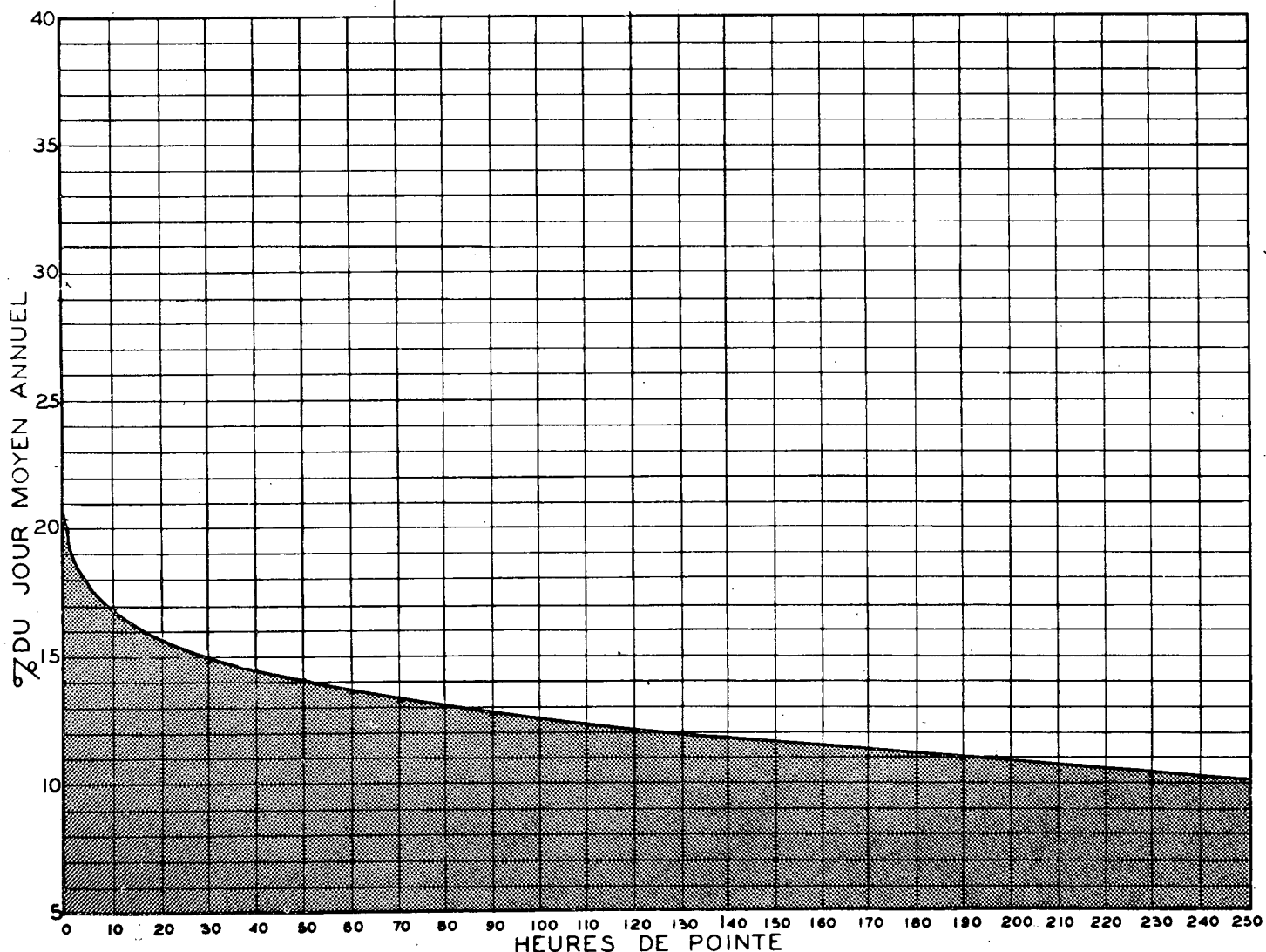
RELATION ENTRE LES HEURES DE POINTE ET LE JOUR MOYEN ANNUEL STATION: POINTE DU LAC ROUTE N° 2
