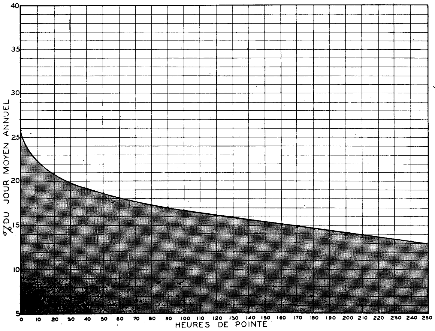
RELATION ENTRE LES HEURES DE POINTE ET LE JOUR MOYEN ANNUEL STATION: ST-JOACHIM ROUTE N° 15
