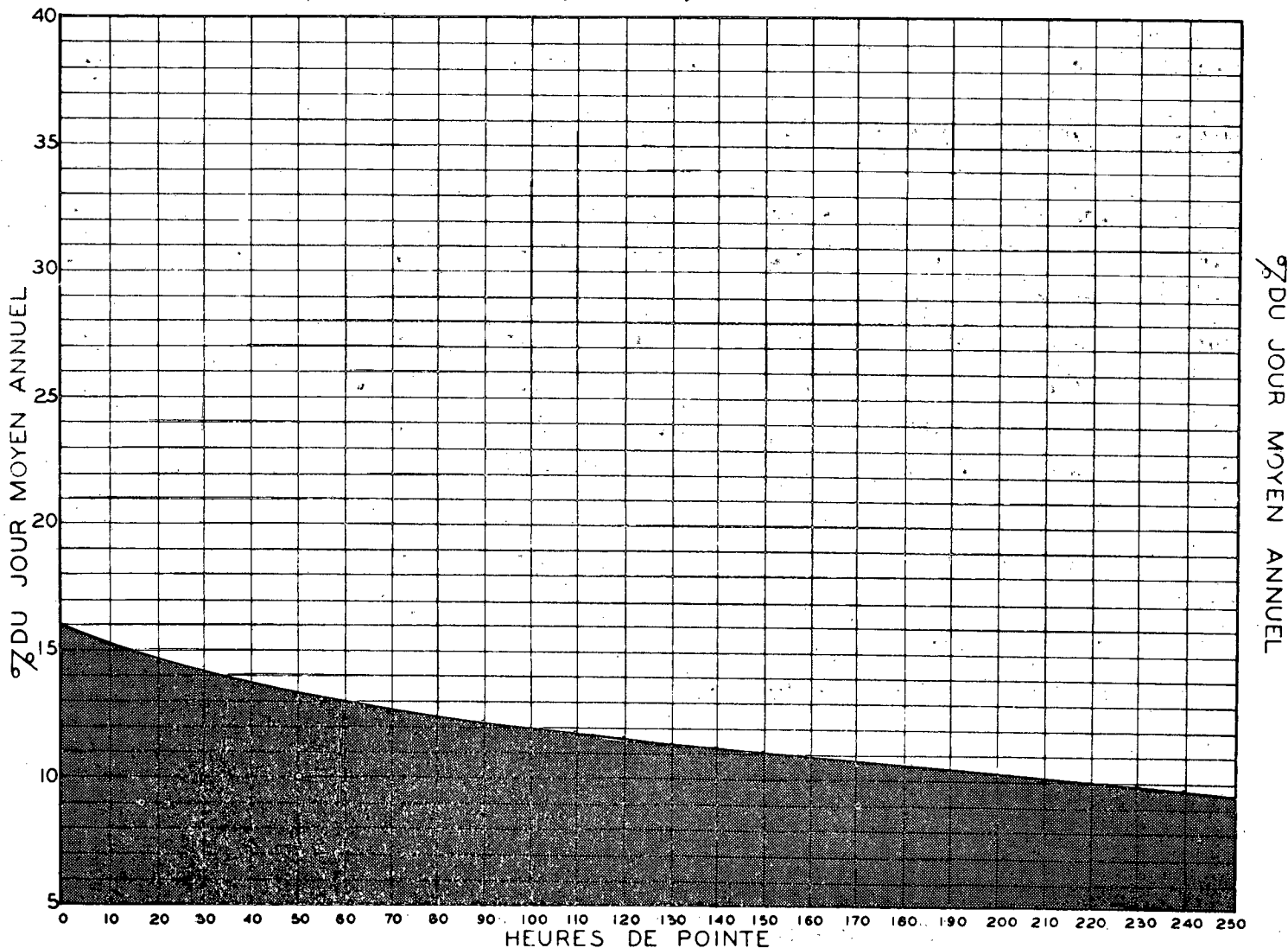
RELATION ENTRE LES HEURES DE POINTE ET LE JOUR MOYEN ANNUEL — STATION: PREVILLE (VOIE EST) — ROUTE N° 3 —
