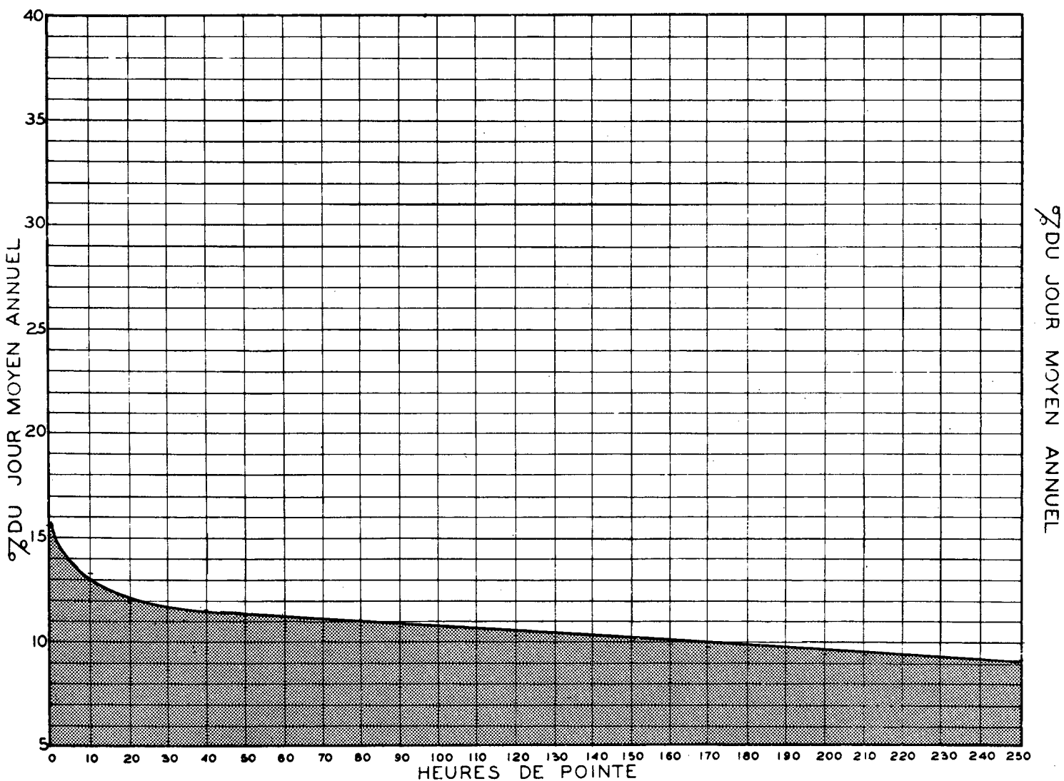
RELATION ENTRE LES HEURES DE POINTE ET LE JOUR MOYEN ANNUEL STATION: STE - HÉLÈNE (2 VOIES) ROUTE N° 9
