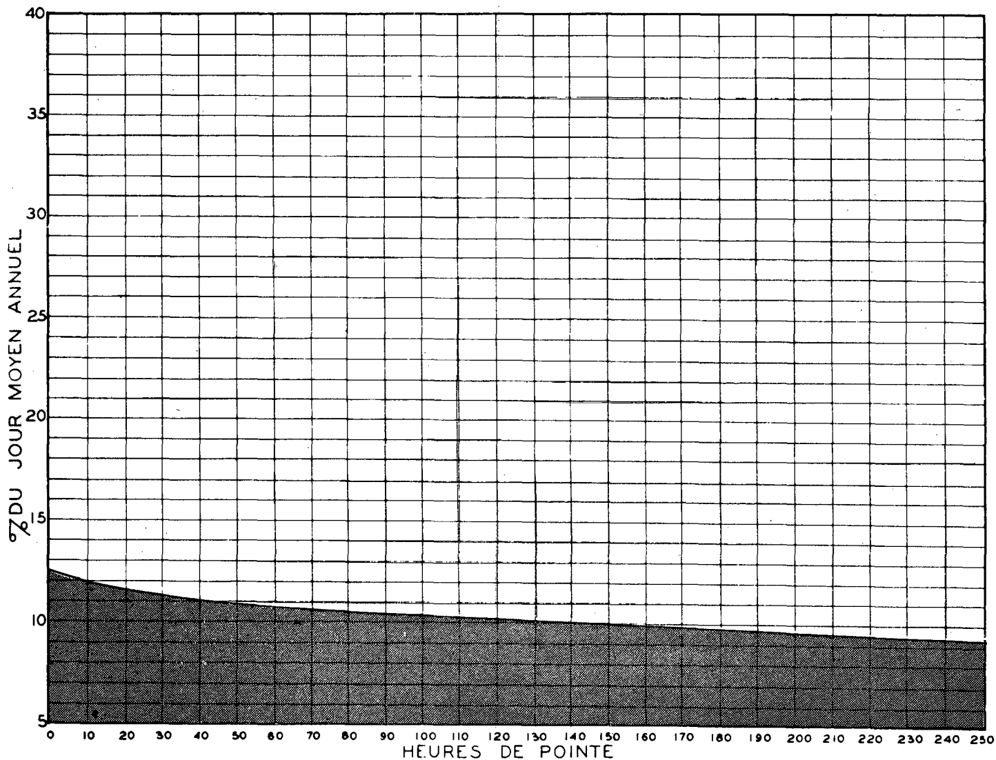
RELATION ENTRE LES HEURES DE POINTE ET LE JOUR MOYEN ANNUEL — STATION: LONGUEUIL (VOIE OUEST) ROUTE N° 3
