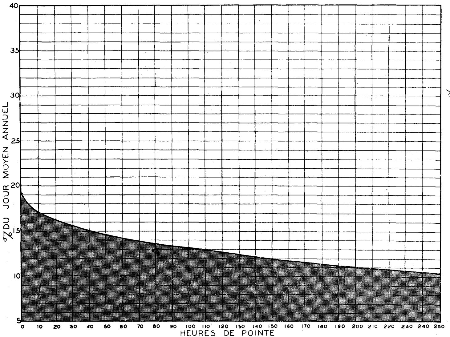
RELATION ENTRE LES HEURES DE POINTE ET LE JOUR MOYEN ANNUEL STATION: STE - ETIENNE ROUTE N° 5
