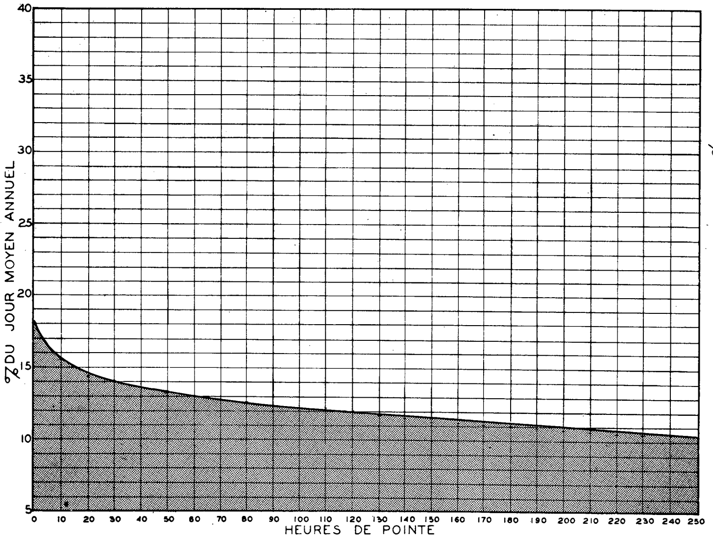
RELATION ENTRE LES HEURES DE POINTE ET LE JOUR MOYEN ANNUEL STATION: BERTHIERVILLE ROUTE N° 2
