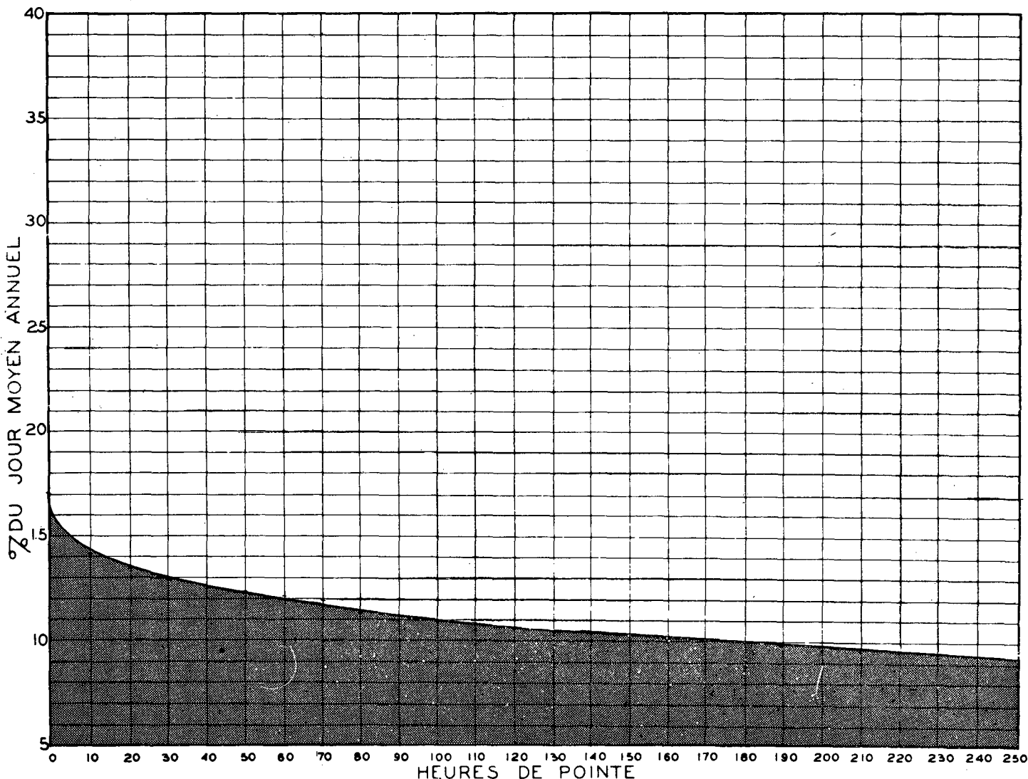
RELATION ENTRE LES HEURES DE POINTE ET LE JOUR MOYEN ANNUEL STATION: ST-REDEMPTEUR 2VOIES ROUTE N° 5
