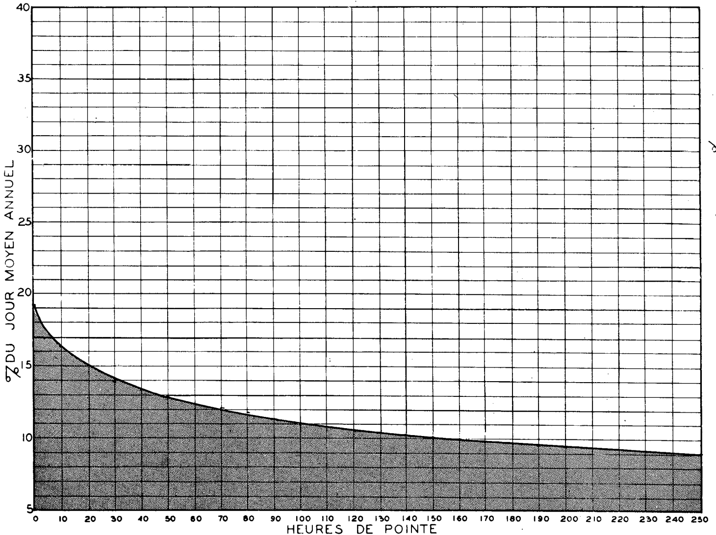
RELATION ENTRE LES HEURES DE POINTE ET LE JOUR MOYEN ANNUEL STATION: COURVILLE ( 2 VOIES) ROUTE N° 15
