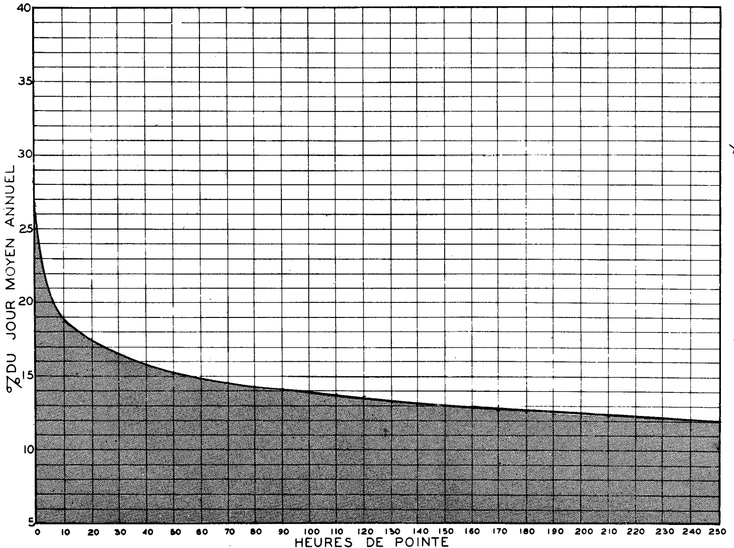
RELATION ENTRE LES HEURES DE POINTE ET LE JOUR MOYEN ANNUEL — STATION: ST-LEONARD ROUTE N° 9
