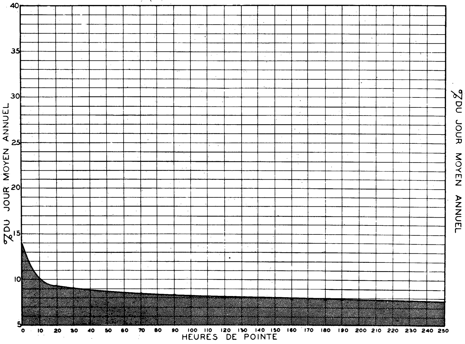
RELATION ENTRE LES HEURES DE POINTE ET LE JOUR MOYEN ANNUEL STATION: LAPRAIRIE 2 VOIES ROUTE N° 9
