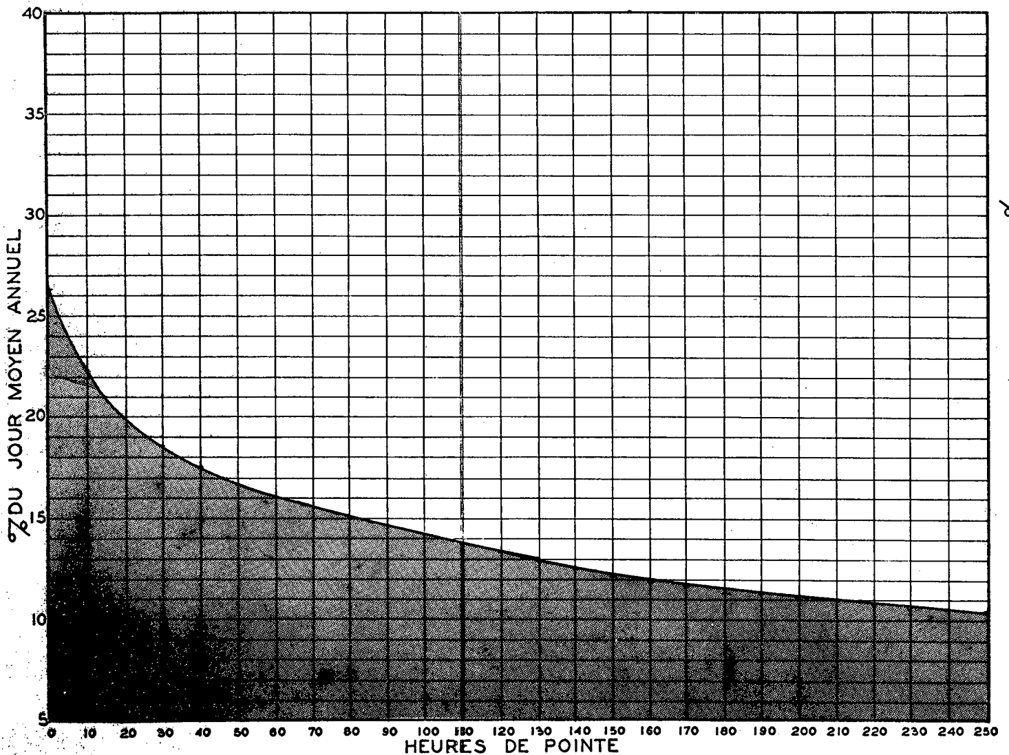
RELATION ENTRE LES HEURES DE POINTE ET LE JOUR MOYEN ANNUEL STATION: N.D. DES LAURENTIDES ROUTE N° 54
