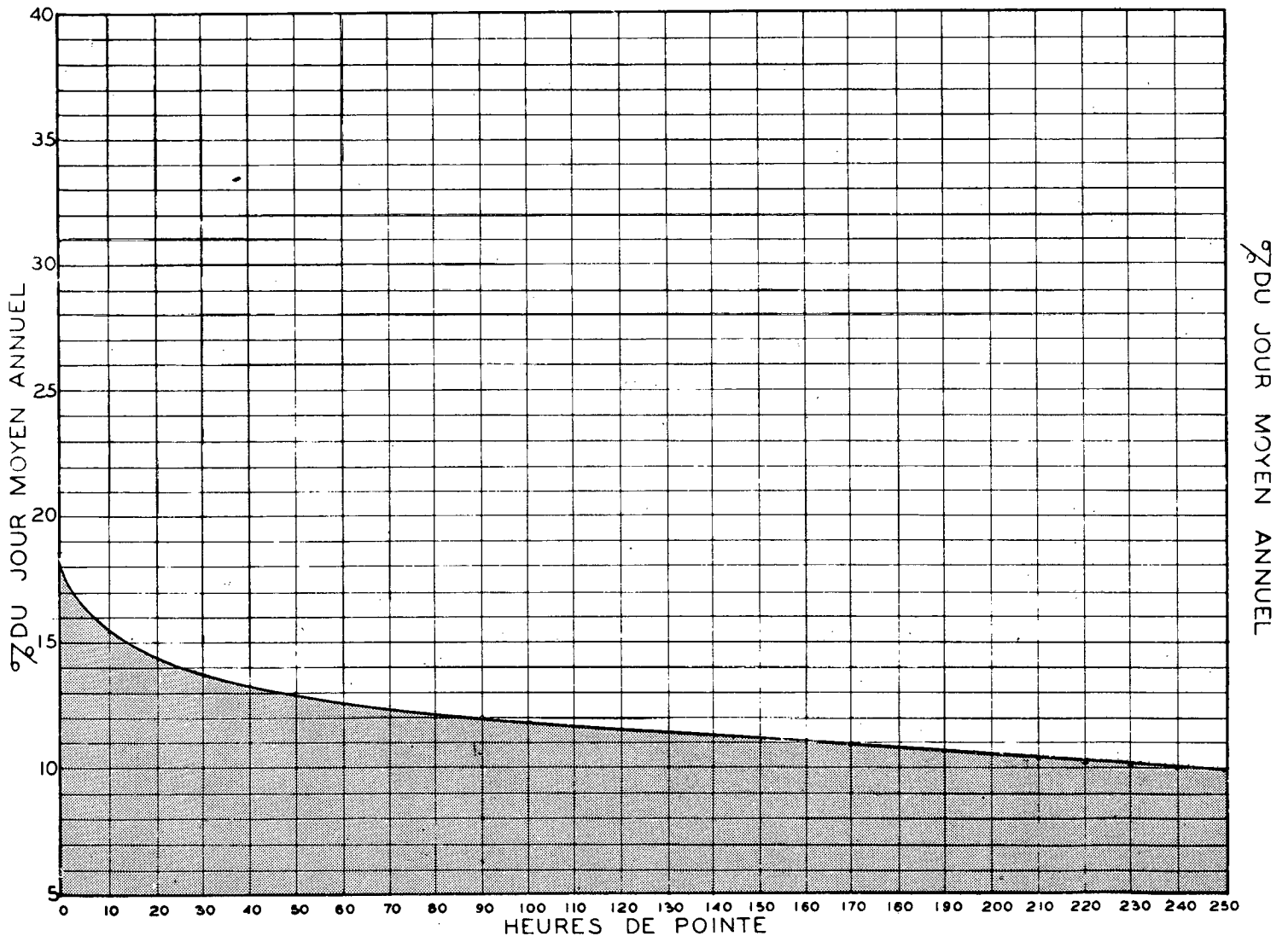
RELATION ENTRE LES HEURES DE POINTE ET LE JOUR MOYEN ANNUEL STATION: STE ANNE DE LA POCATIÈRE ROUTE N° 2
