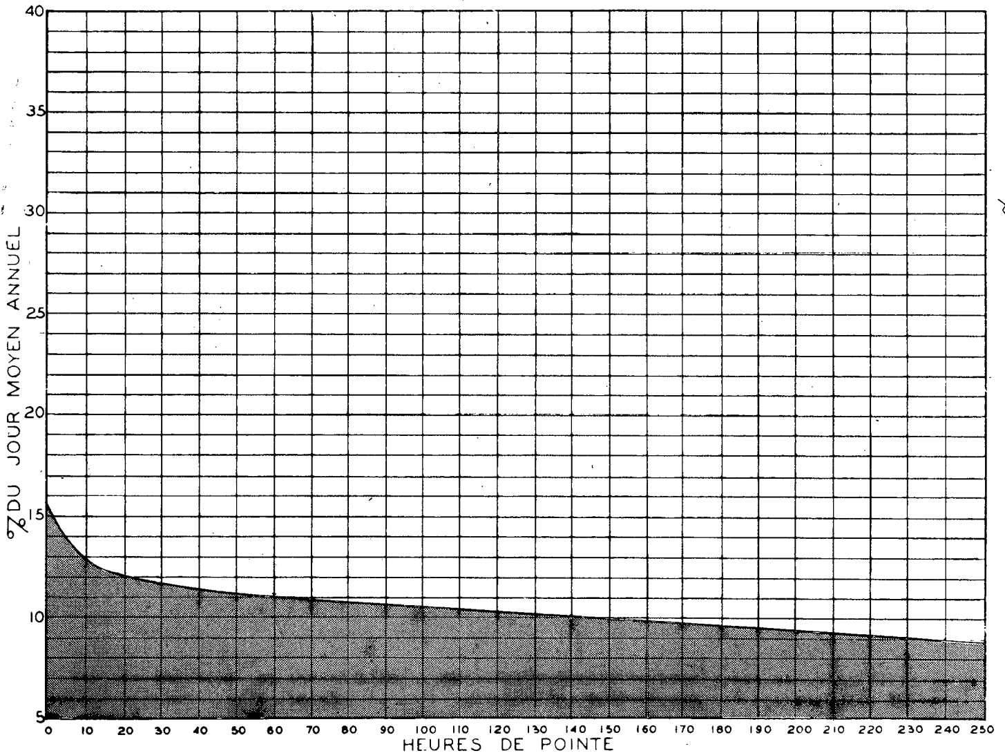
RELATION ENTRE LES HEURES DE POINTE ET LE JOUR MOYEN ANNUEL STATION: POINTE-CLAIRE (VOIE SUD) ROUTE N° 2
