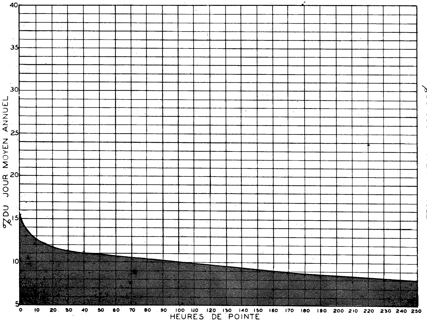
RELATION ENTRE LES HEURES DE POINTE ET LE JOUR MOYEN ANNUEL STATION: ST-LOUIS DE PINTENDRE (2 VOIES) ROUTE N° 23
