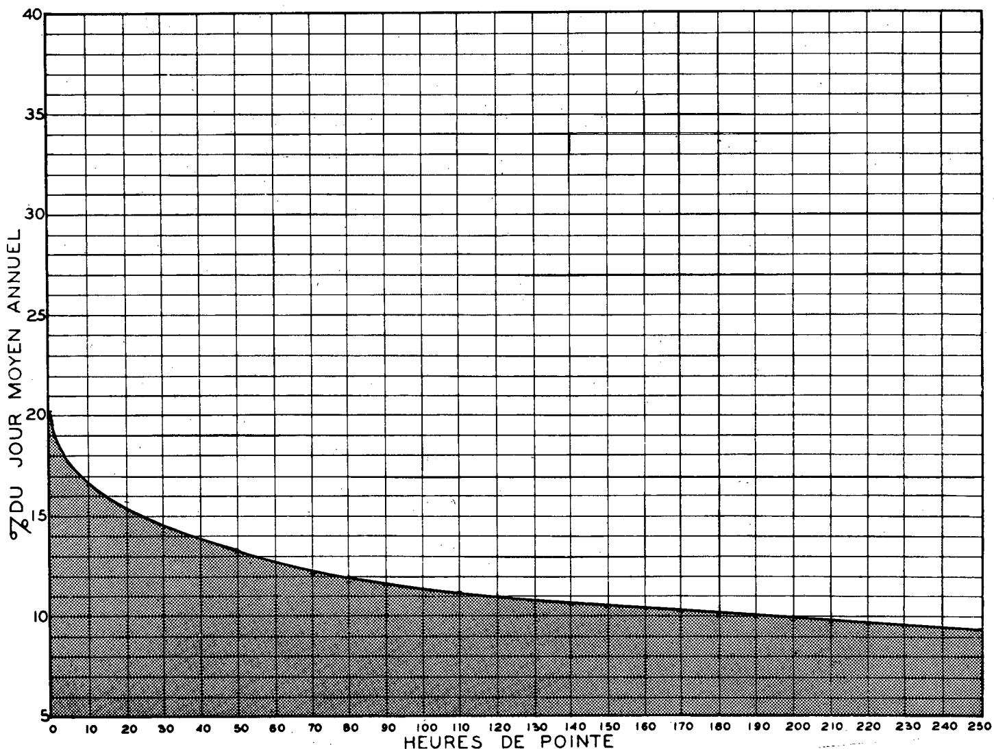
RELATION ENTRE LES HEURES DE POINTE ET LE JOUR MOYEN ANNUEL STATION: STE-HÉLÈNE (VOIE SUD) ROUTE N° 9
