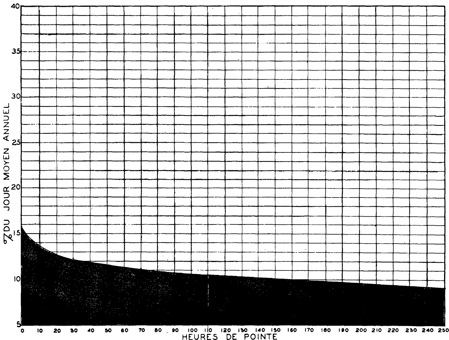
RELATION ENTRE LES HEURES DE POINTE ET LE JOUR MOYEN ANNUEL STATION: LAUZON ROUTE N° 2
