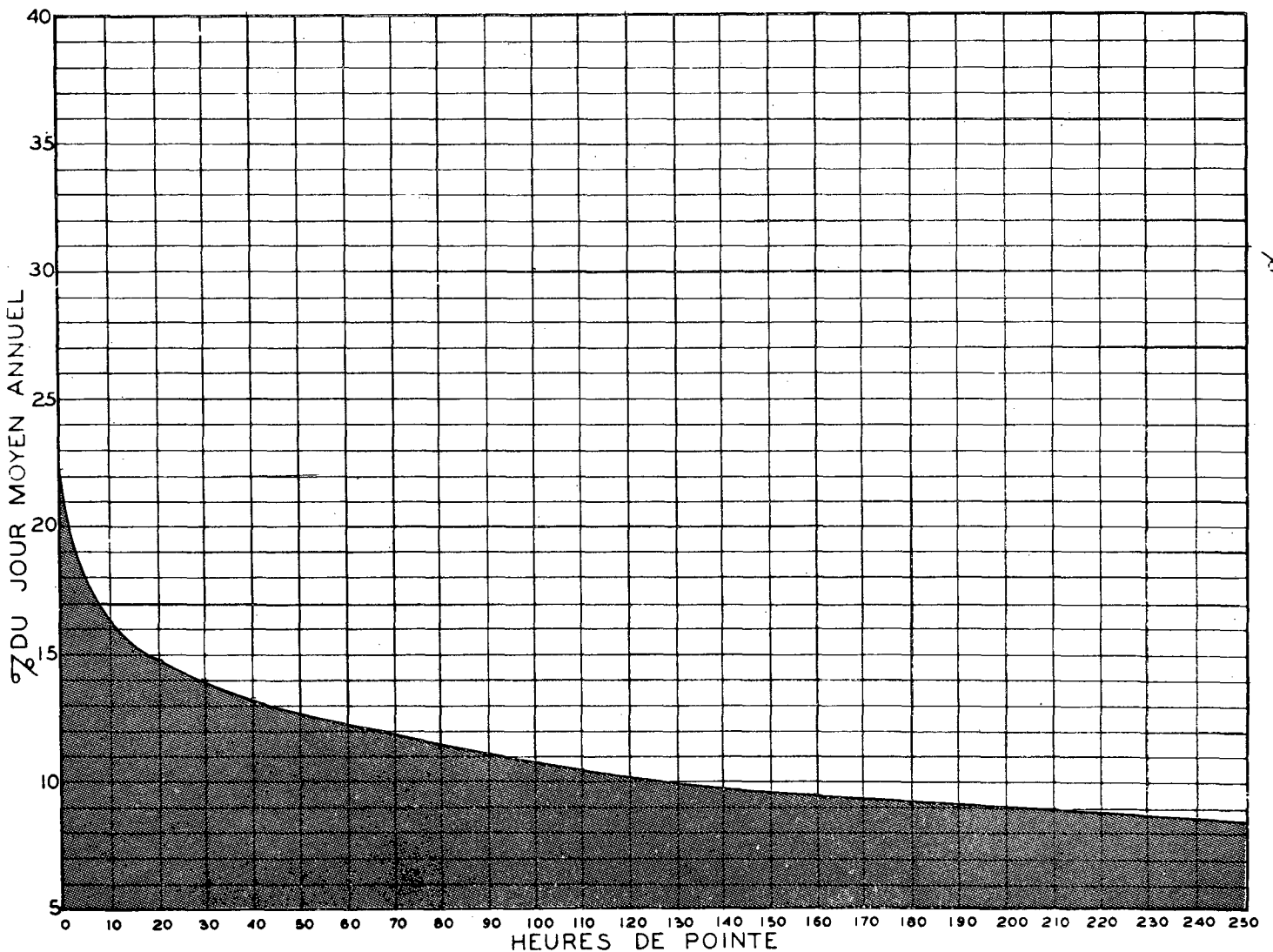
RELATION ENTRE LES HEURES DE POINTE ET LE JOUR MOYEN ANNUEL — STATION: ST-NICOLAS (VOIE EST) ROUTE N° 9
