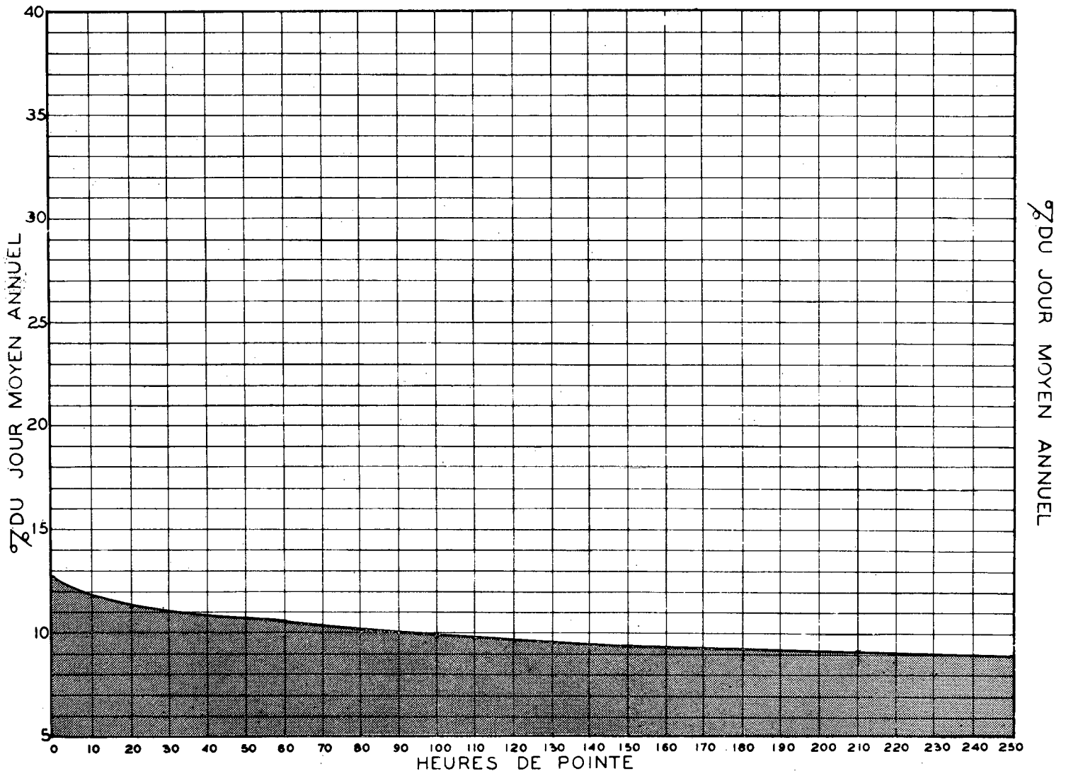
RELATION ENTRE LES HEURES DE POINTE ET LE JOUR MOYEN ANNUEL — STATION: VARENNE ----- ROUTE N° 3 -----
