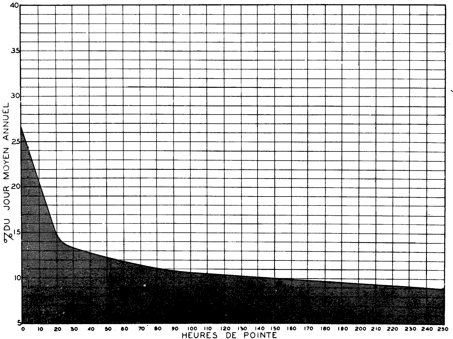
RELATION ENTRE LES HEURES DE POINTE ET LE JOUR MOYEN ANNUEL STATION: ST-NICOLAS (VOIE OUEST) ROUTE N° 9
