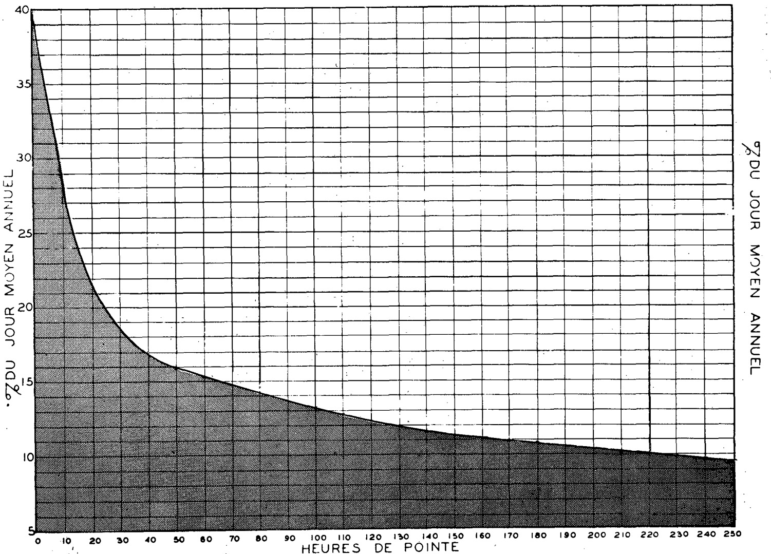
RELATION ENTRE LES HEURES DE POINTE ET LE JOUR MOYEN ANNUEL STATION: LAC BEAUPORT ROUTE N° BOUL. LAURENTIEN
