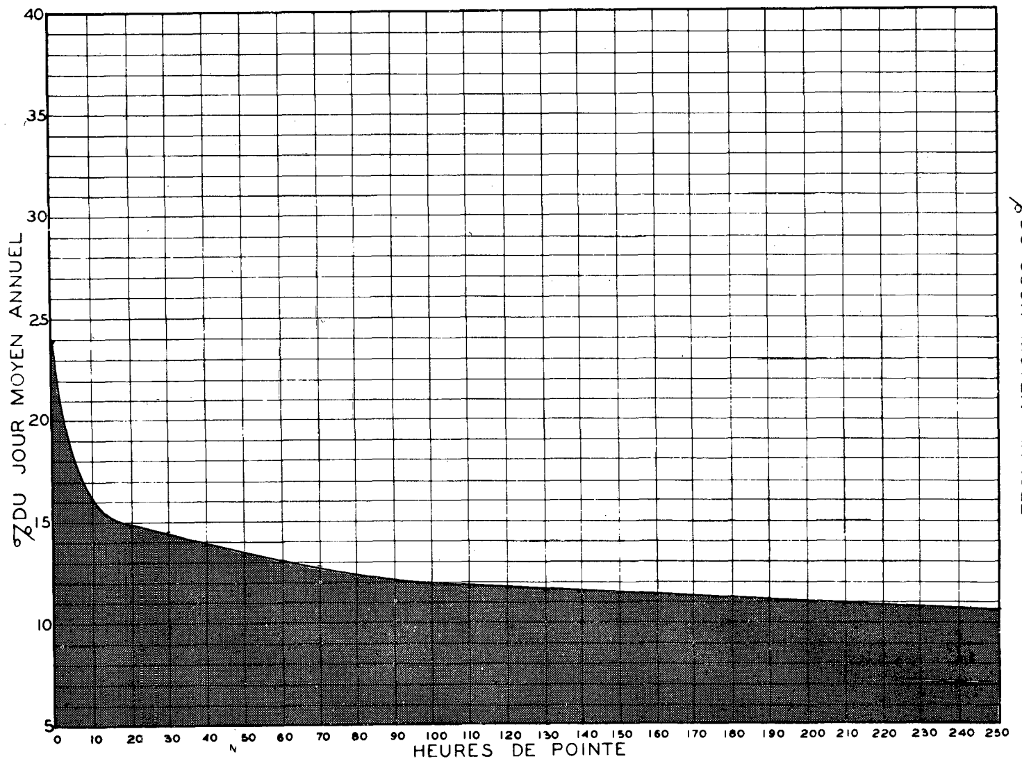
RELATION ENTRE LES HEURES DE POINTE ET LE JOUR MOYEN ANNUEL STATION: PREVILLE (VOIE OUEST) ROUTE N° 3
