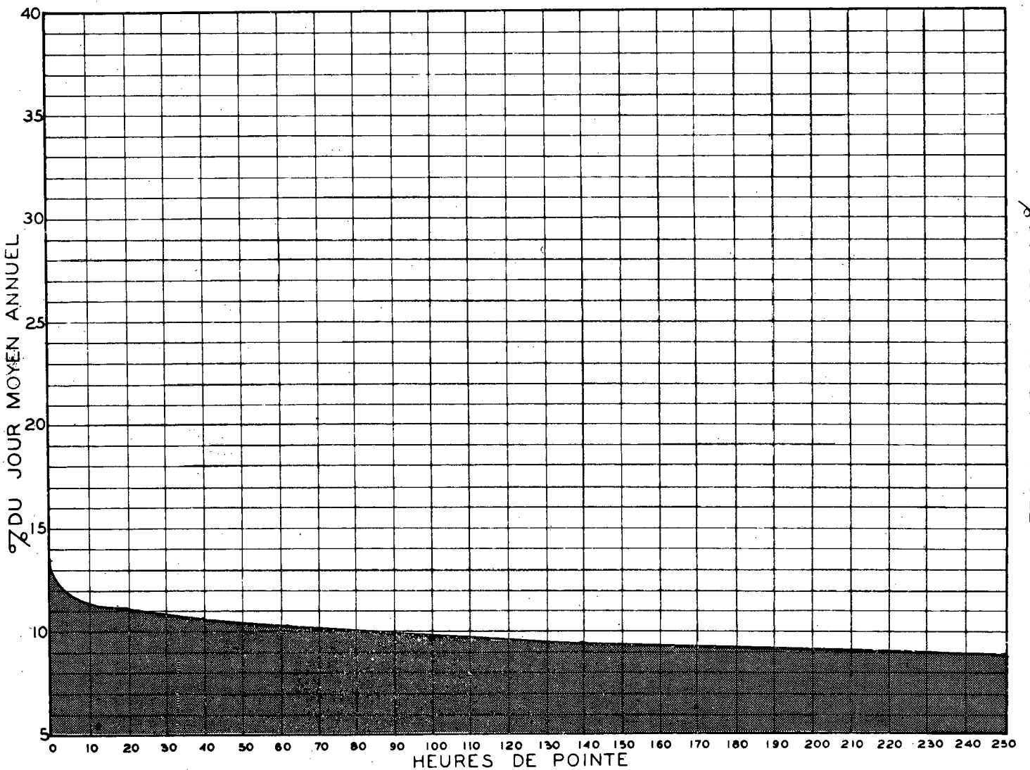
RELATION ENTRE LES HEURES DE POINTE ET LE JOUR MOYEN ANNUEL STATION: LAPRAIRIE 2 VOIES ROUTE N° 3
