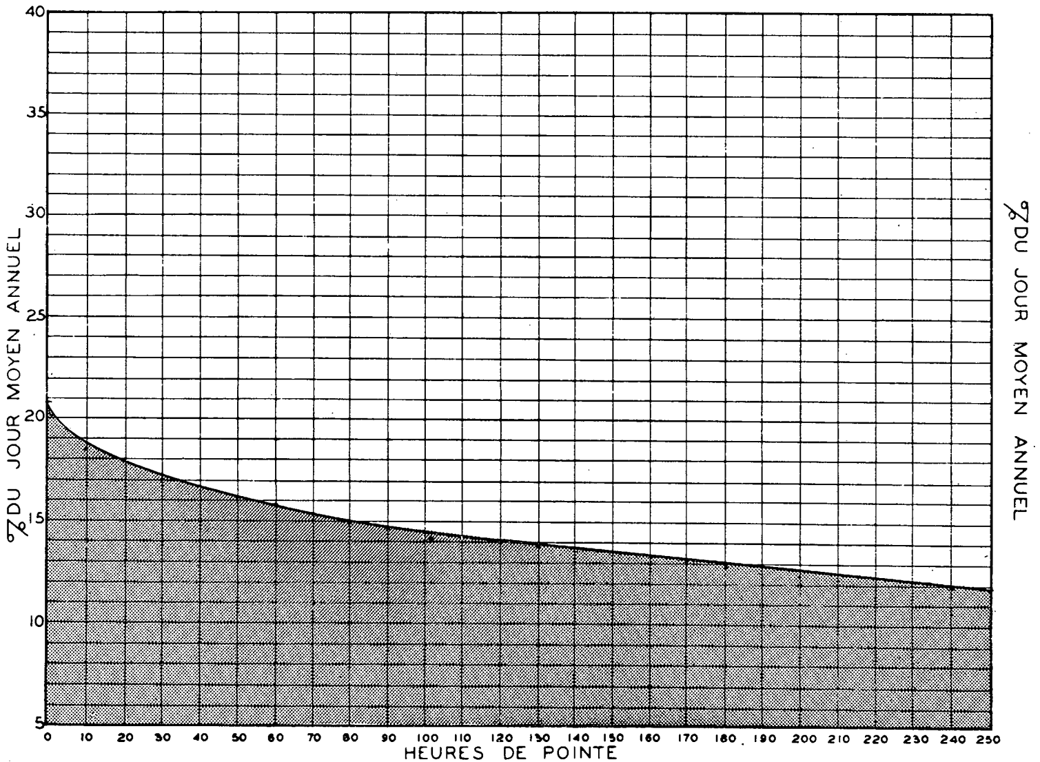
RELATION ENTRE LES HEURES DE POINTE ET LE JOUR MOYEN ANNUEL — STATION: RIVIERE BEAUDETTE — ROUTE N° 2 —
