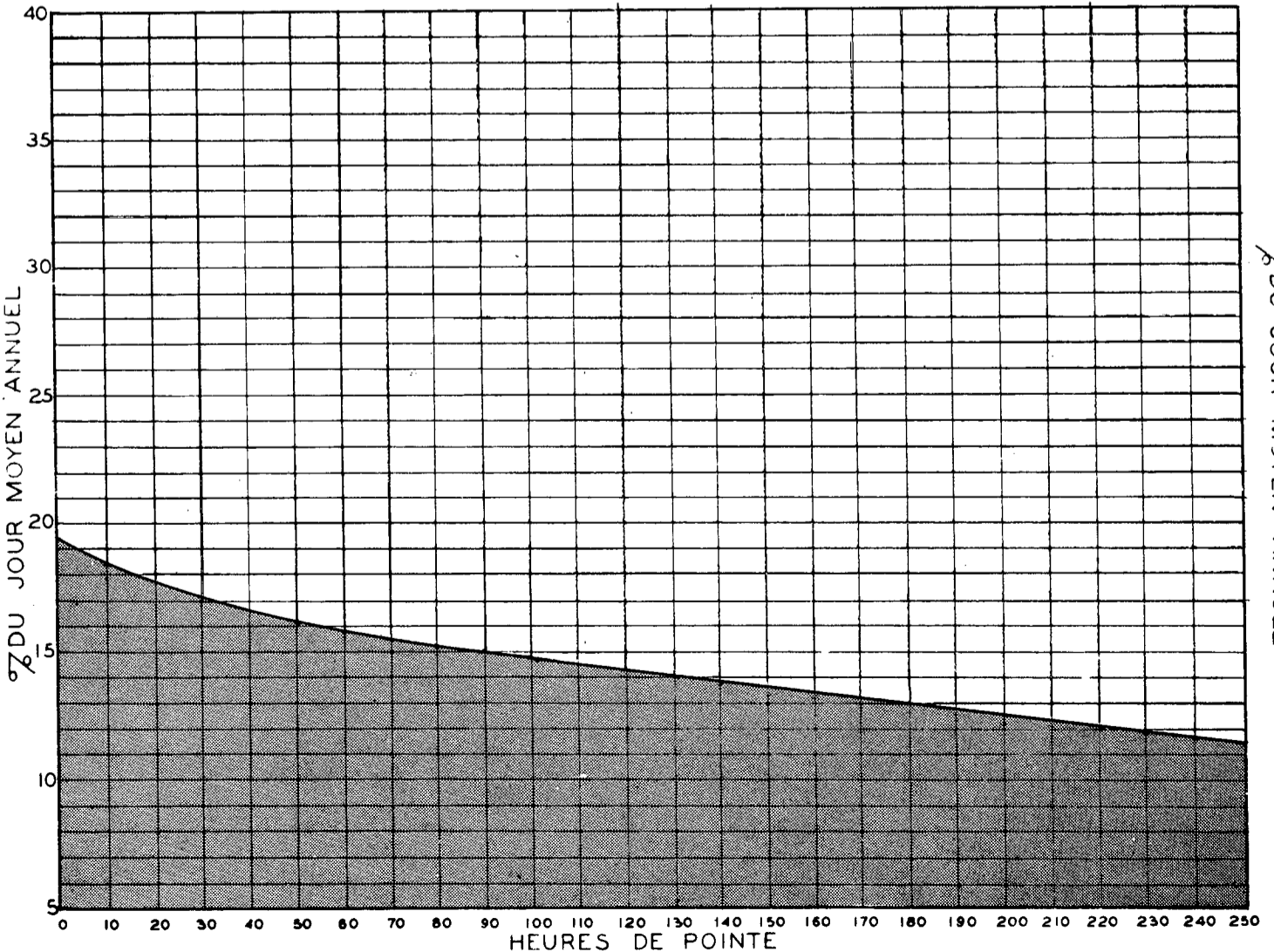
RELATION ENTRE LES HEURES DE POINTE ET LE JOUR MOYEN ANNUEL STATION: BOISCHATEL ROUTE N 15
