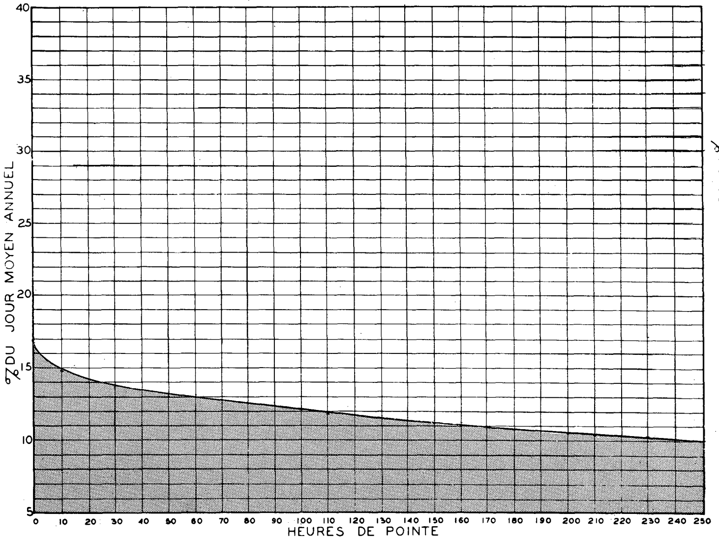
RELATION ENTRE LES HEURES DE POINTE ET LE JOUR MOYEN ANNUEL — STATION TERREBONNE — 2 VOIES — ROUTE N° 18 —
