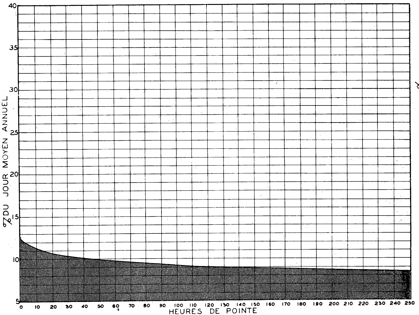
RELATION ENTRE LES HEURES DE POINTE ET LE JOUR MOYEN ANNUEL STATION: POINTE CLAIRE 2 VOIES ROUTE N° 2
