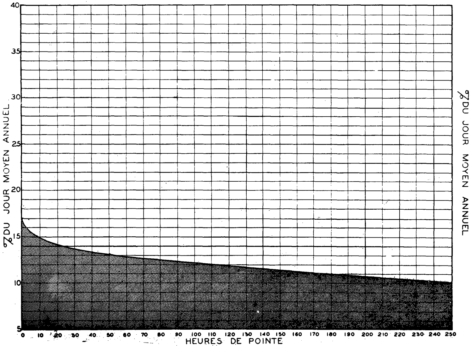
RELATION ENTRE LES HEURES DE POINTE ET LE JOUR MOYEN ANNUEL STATION: ST-BERNARD ROUTE N° 1
