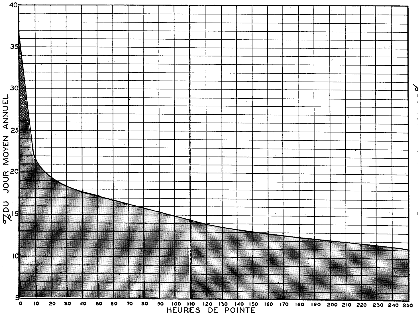
RELATION ENTRE LES HEURES DE POINTE ET LE JOUR MOYEN ANNUEL STATION: STORNOWAY ROUTE N° 34
