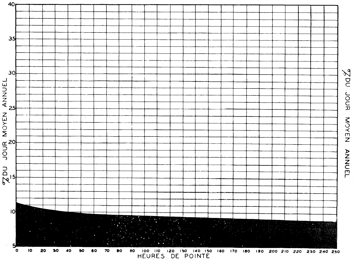
RELATION ENTRE LES HEURES DE POINTE ET LE JOUR MOYEN ANNUEL STATION: LONGUEUIL 2 VOIES ROUTE N° 3
