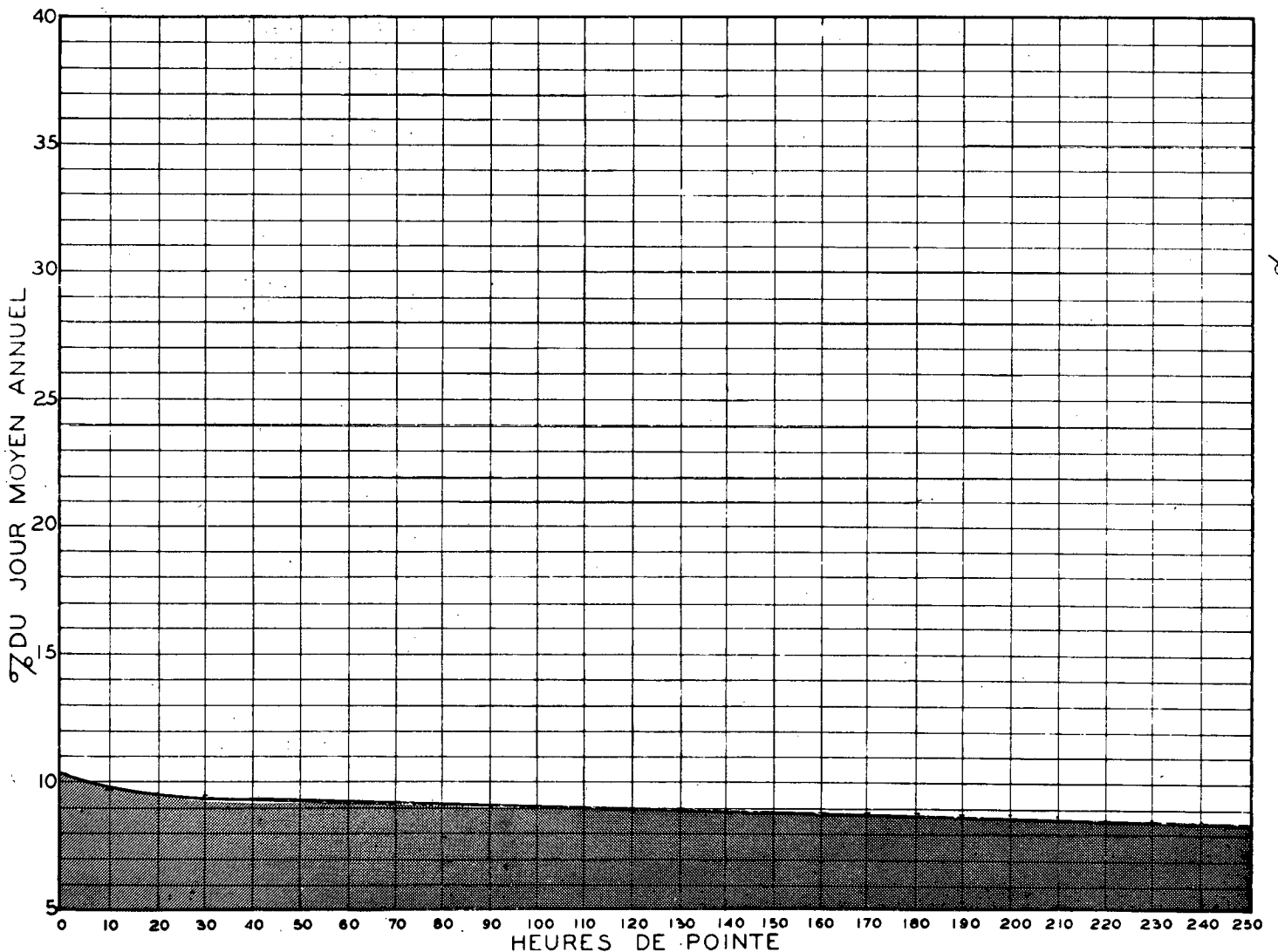
RELATION ENTRE LES HEURES DE POINTE ET LE JOUR MOYEN ANNUEL STATION: PONT SAMSON ROUTE N° R. S.
