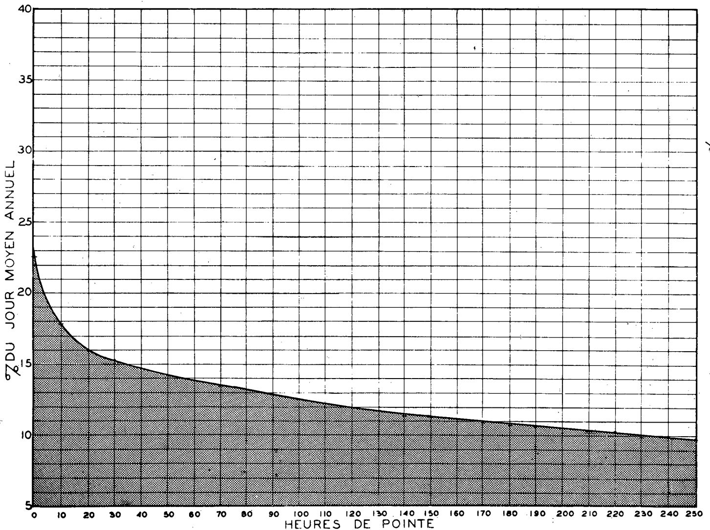
RELATION ENTRE LES HEURES DE POINTE ET LE JOUR MOYEN ANNUEL STATION: ST-JEAN CHRYSOSTOME ROUTE N°
