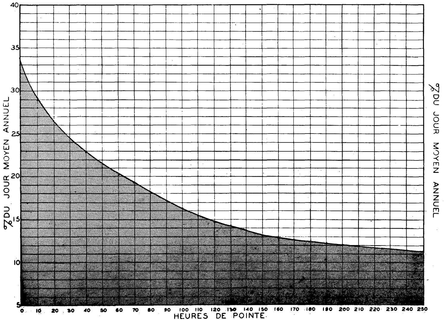
RELATION ENTRE LES HEURES DE POINTE ET LE JOUR MOYEN ANNUEL STATION: ANCIENNE LORETTE ROUTE N° R. S.
