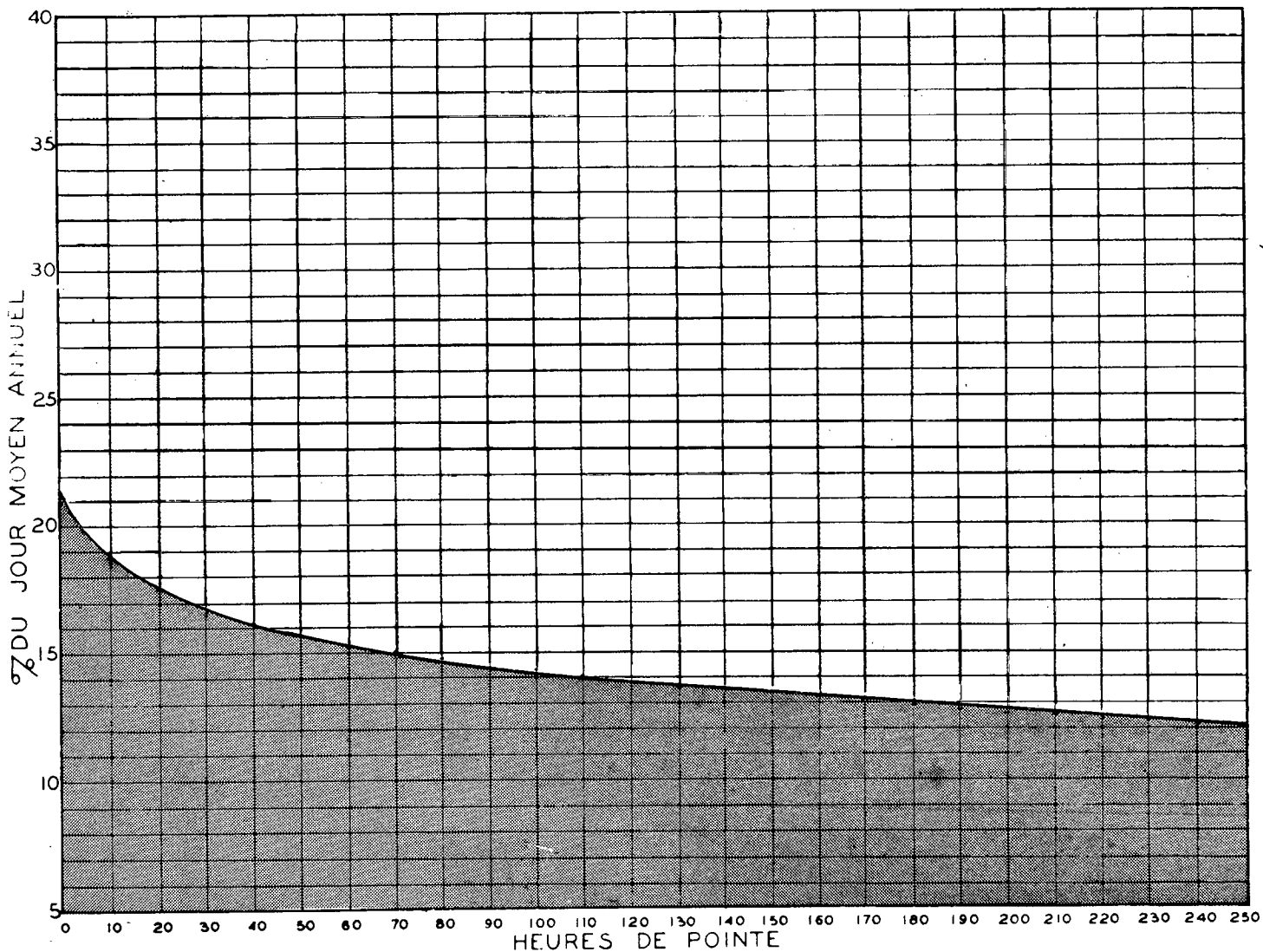
RELATION ENTRE LES HEURES DE POINTE ET LE JOUR MOYEN ANNUEL — STATION: BERTHIER ROUTE N° 2
