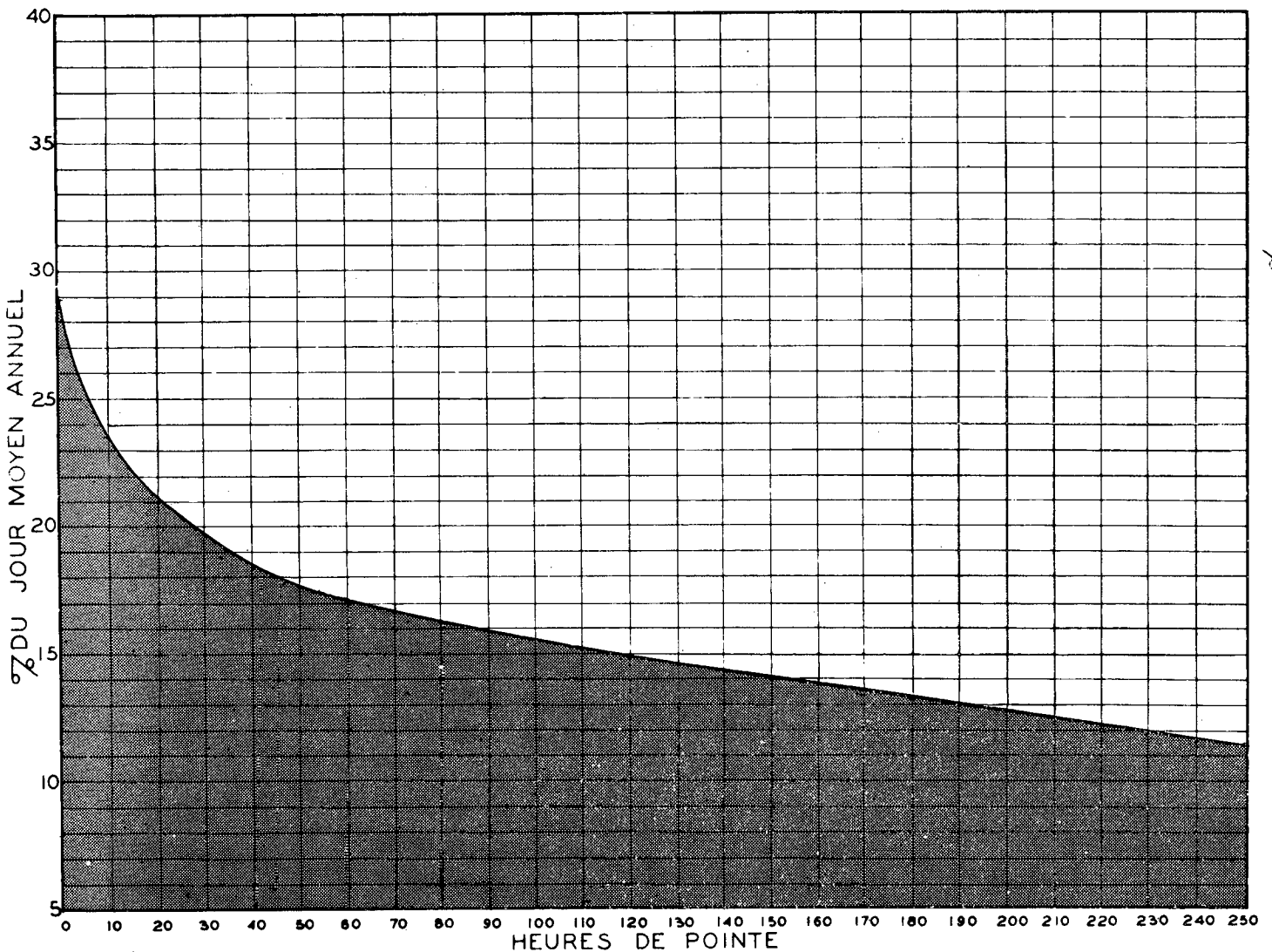
RELATION ENTRE LES HEURES DE POINTE ET LE JOUR MOYEN ANNUEL STATION: ST-JEAN (VOIE NORD) ROUTE N° 7
