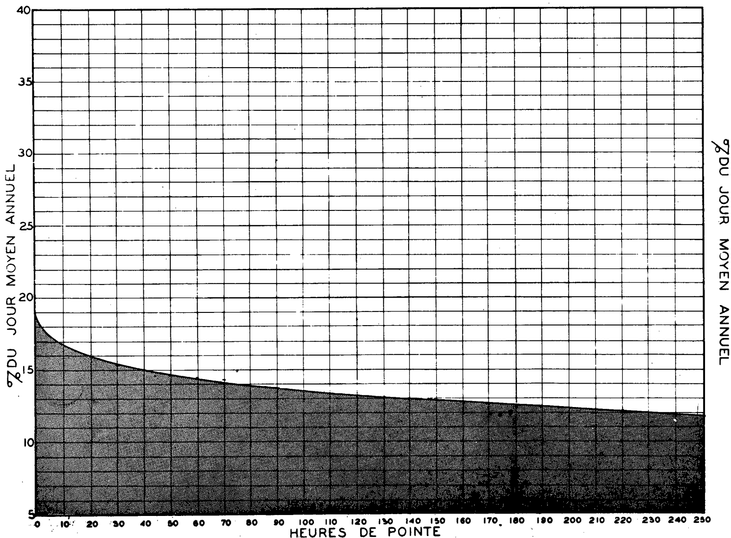
RELATION ENTRE LES HEURES DE POINTE ET LE JOUR MOYEN ANNUEL STATION: POINTE FORTUNE ROUTE N° 17
