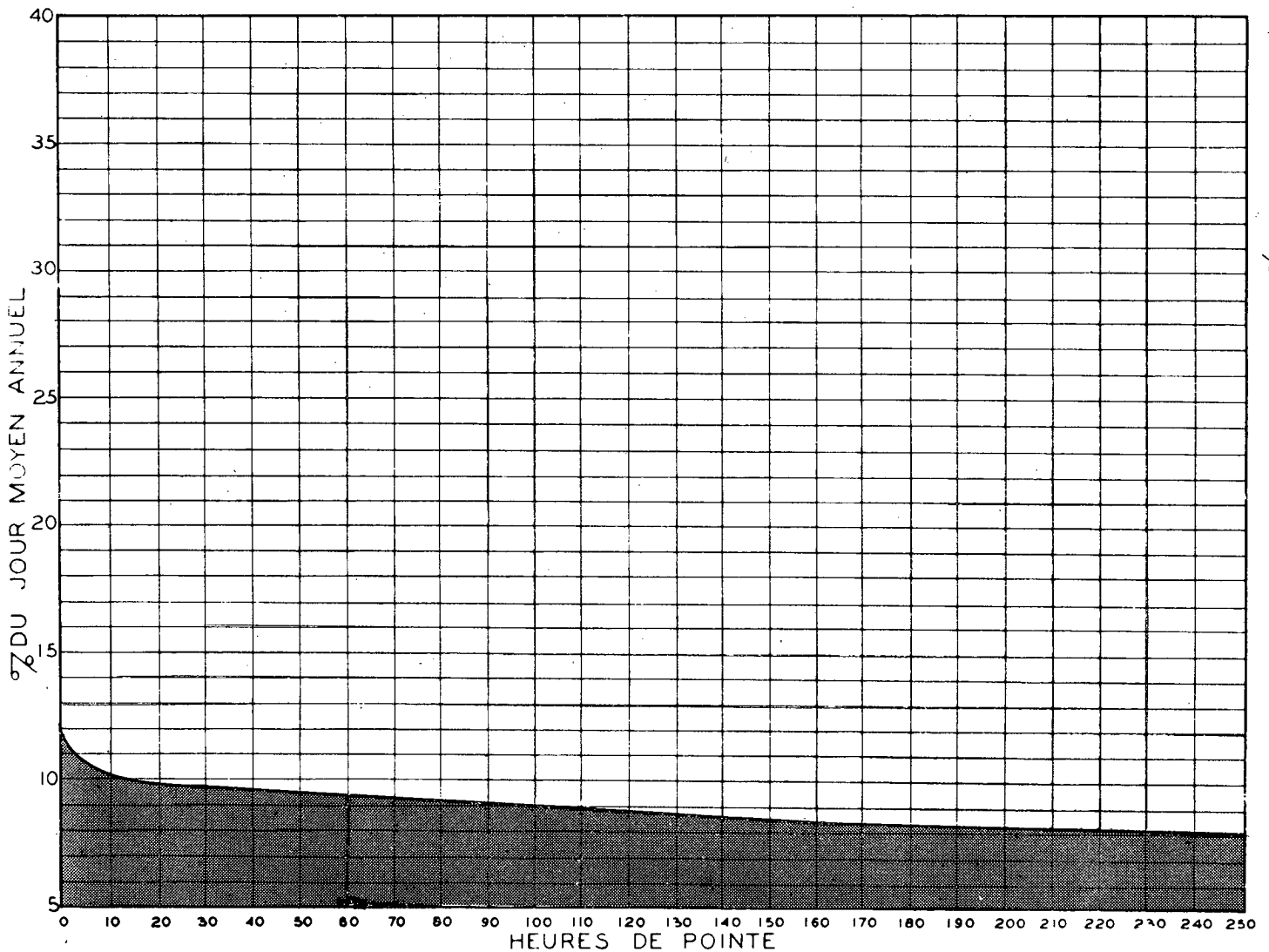
RELATION ENTRE LES HEURES DE POINTE ET LE JOUR MOYEN ANNUEL STATION: BOUCHERVILLE ROUTE N° 3
