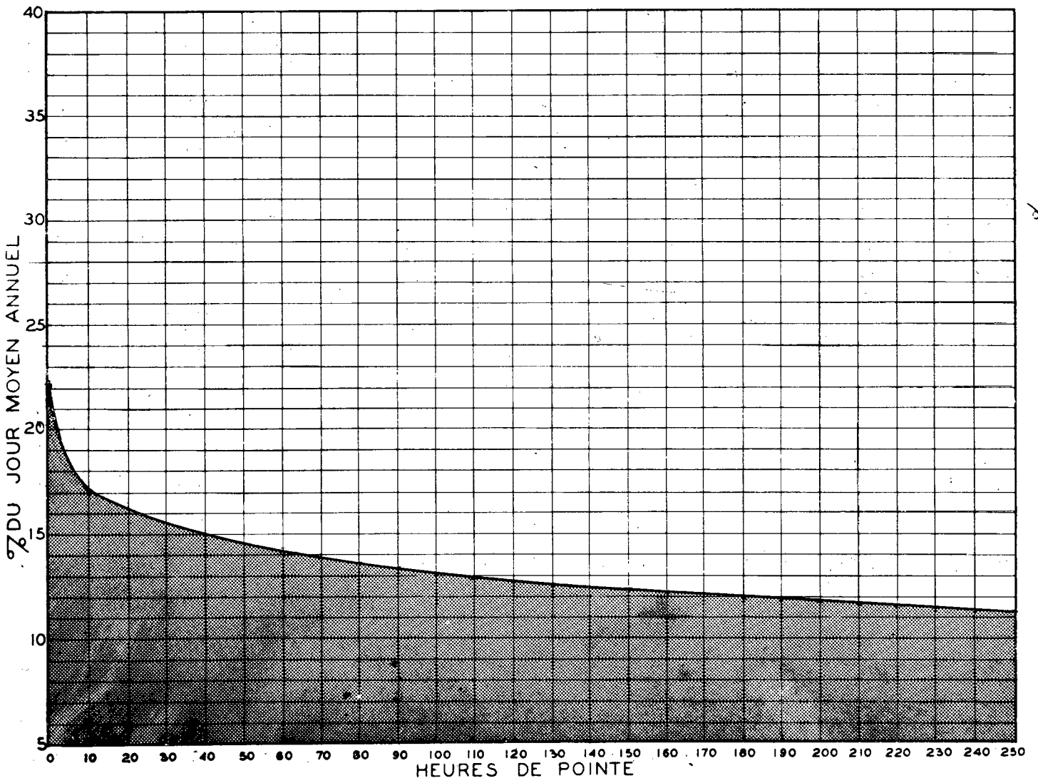
RELATION ENTRE LES HEURES DE POINTE ET LE JOUR MOYEN ANNUEL STATION: ARMSTRONG (2 VOIES) ROUTE N° 23
