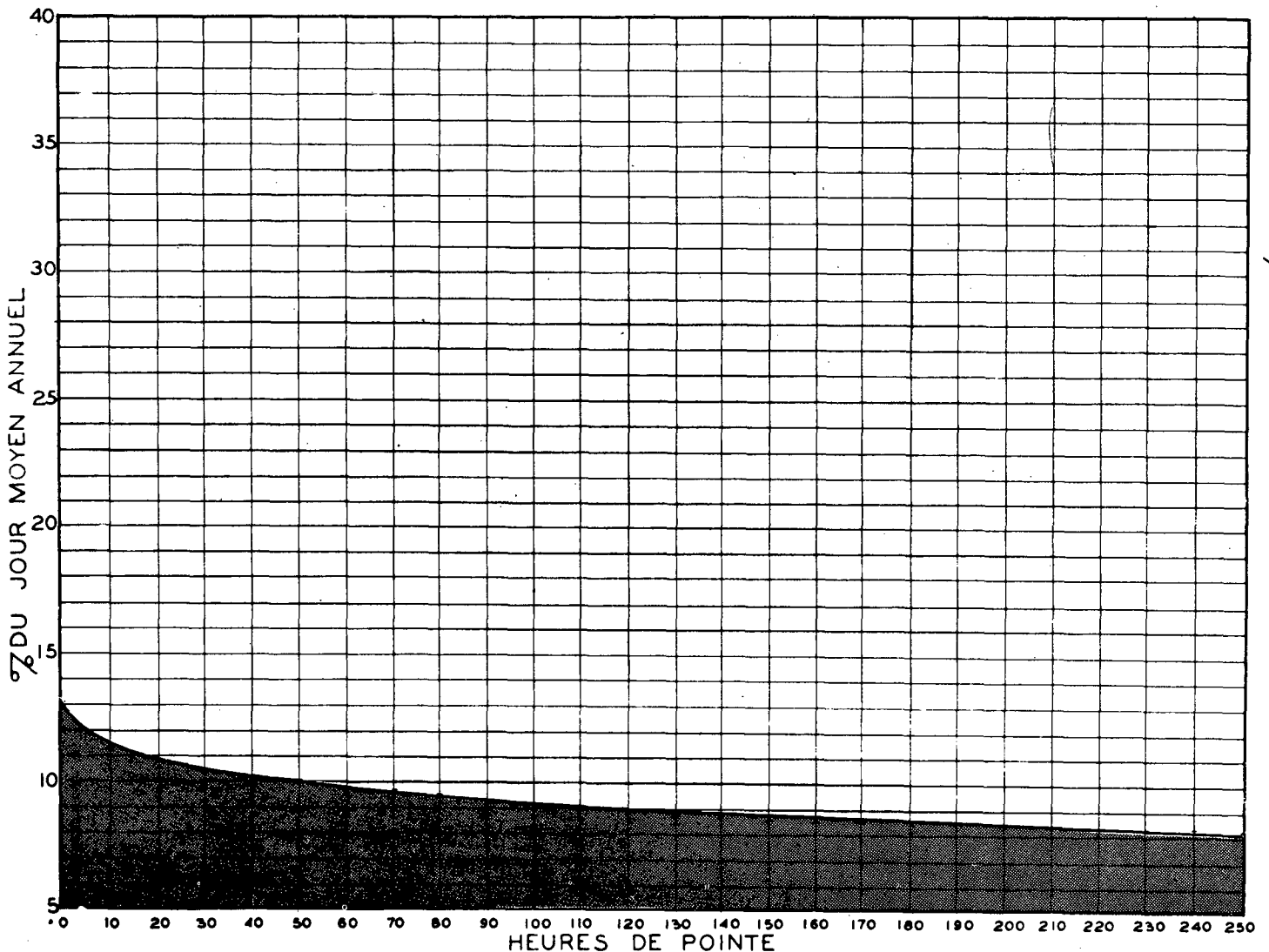
RELATION ENTRE LES HEURES DE POINTE ET LE JOUR MOYEN ANNUEL STATION: LAPRAIRIE (VOIE EST) ROUTE N° 9
