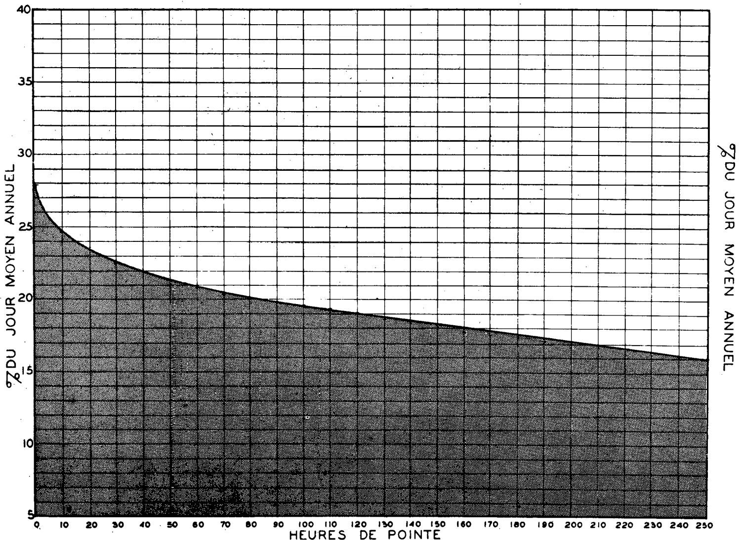
RELATION ENTRE LES HEURES DE POINTE ET LE JOUR MOYEN ANNUEL — STATION: ST - AGATHE ROUTE N° 11
