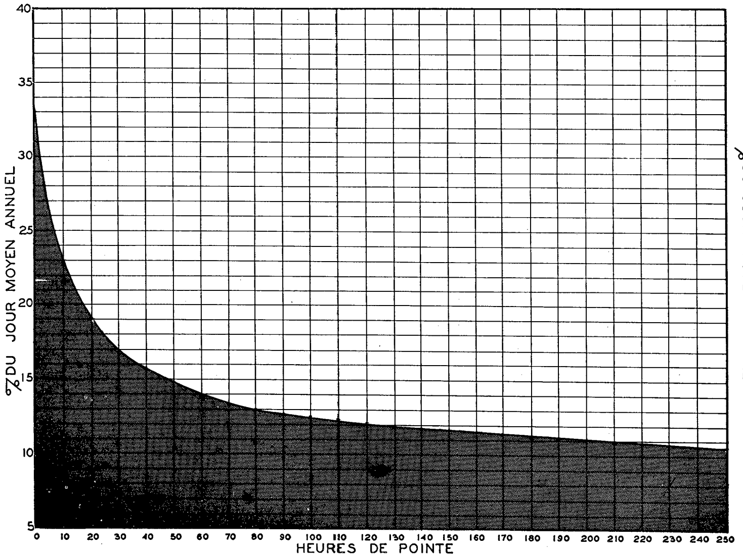
RELATION ENTRE LES HEURES DE POINTE ET LE JOUR MOYEN ANNUEL STATION: STE-ROSE ROUTE N° 24
