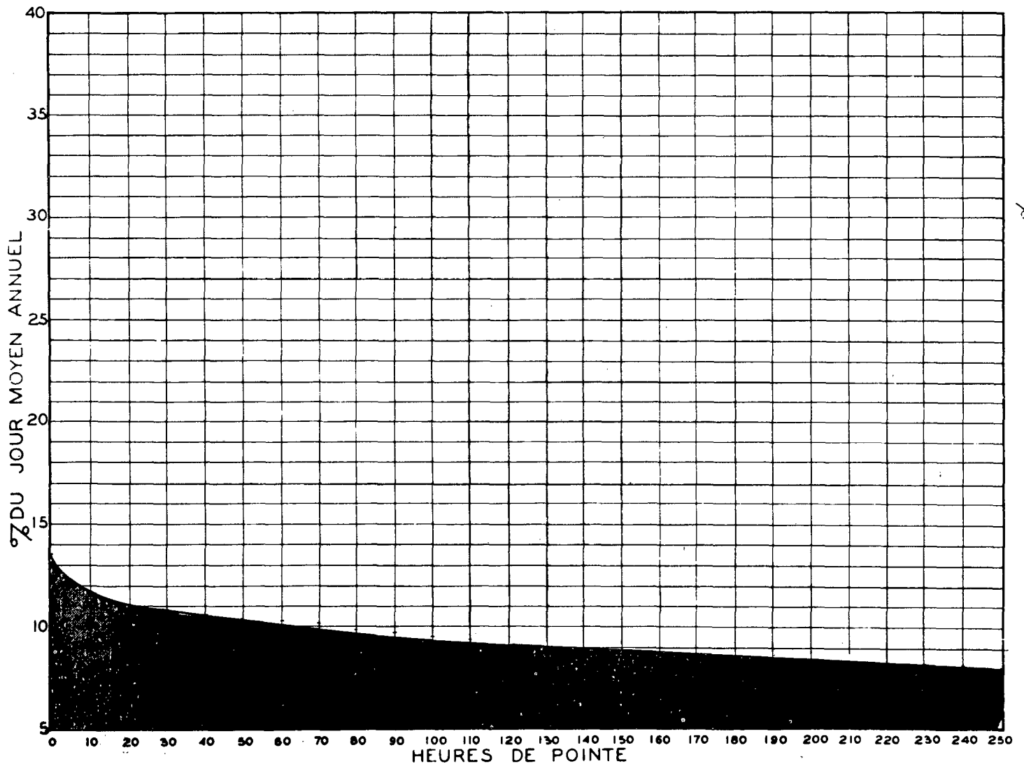
RELATION ENTRE LES HEURES DE POINTE ET LE JOUR MOYEN ANNUEL STATION: CHAMBLY ROUTE N° L
