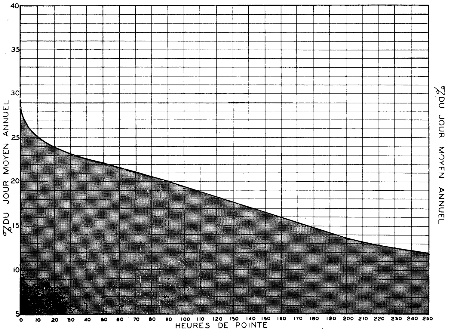
RELATION ENTRE LES HEURES DE POINTE ET LE JOUR MOYEN ANNUEL STATION: TERREBONNE (VOIE OUEST) ROUTE N° 18
