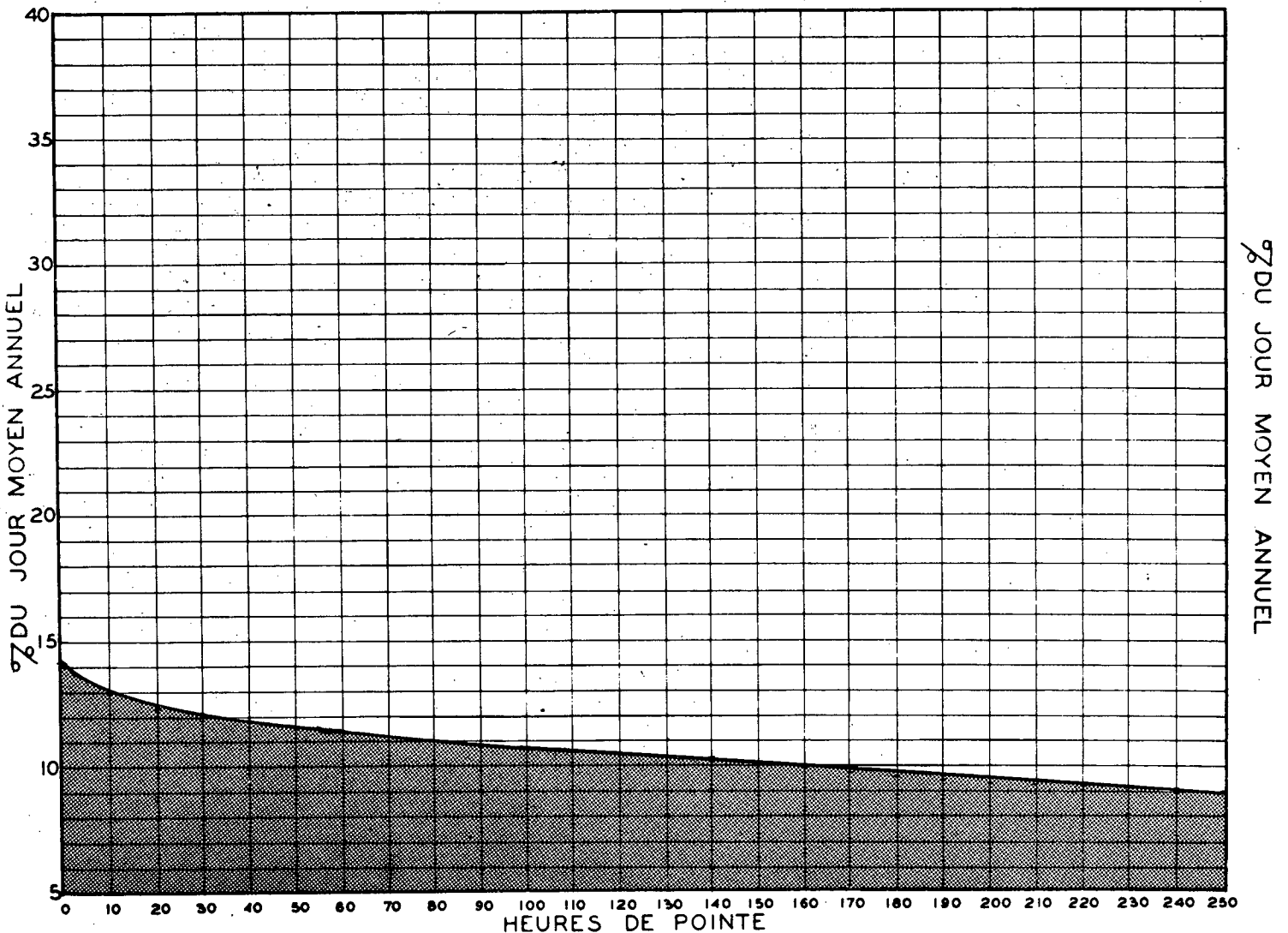
RELATION ENTRE LES HEURES DE POINTE ET LE JOUR MOYEN ANNUEL STATION: GREENFIELD PARK (VOIE EST) ROUTE N° 9
