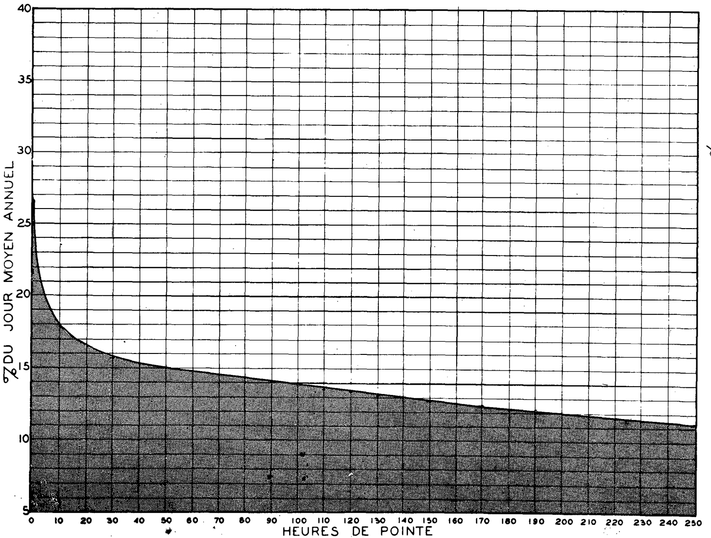
RELATION ENTRE LES HEURES DE POINTE ET LE JOUR MOYEN ANNUEL STATION: ST-LEONARD ROUTE N° 13
