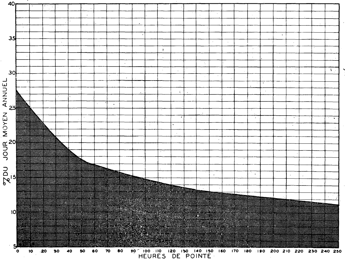
RELATION ENTRE LES HEURES DE POINTE ET LE JOUR MOYEN ANNUEL STATION: ST-JEAN (VOIE SUD) ROUTE N° 7
