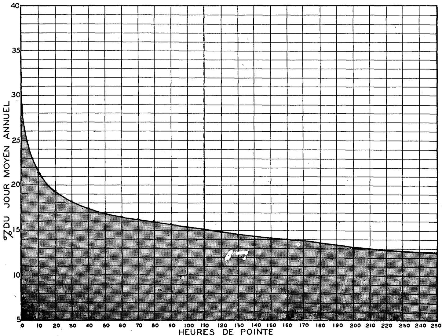
RELATION ENTRE LES HEURES DE POINTE ET LE JOUR MOYEN ANNUEL STATION: STORNOWAY ROUTE N° 28
