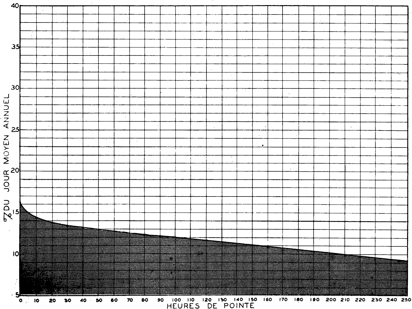
RELATION ENTRE LES HEURES DE POINTE ET LE JOUR MOYEN ANNUEL STATION: BOIS DES FILLION (2 VOIES) ROUTE N° 65
