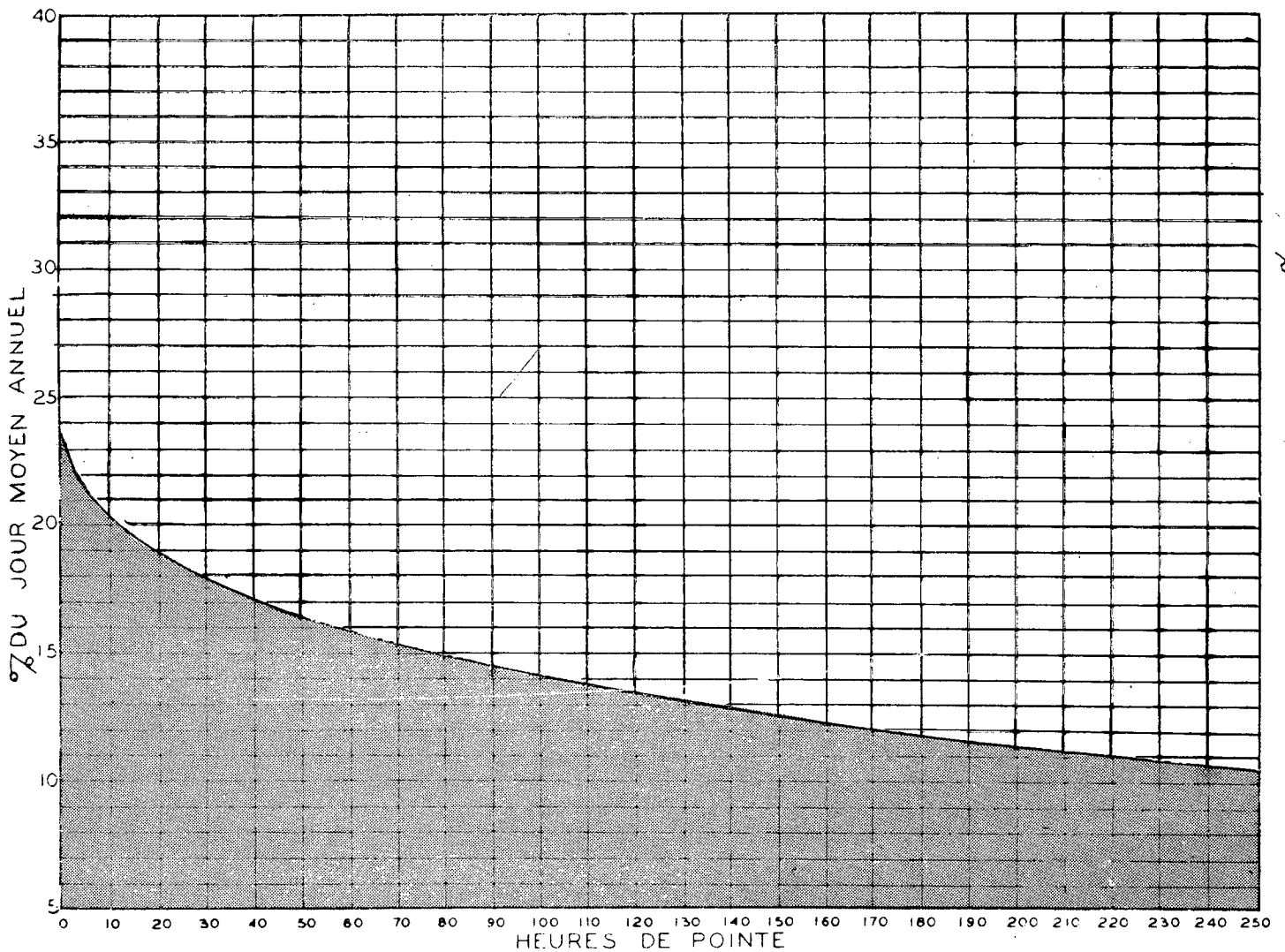
RELATION ENTRE LES HEURES DE POINTE ET LE JOUR MOYEN ANNUEL STATION: ANCIENNE LORETTE ROUTE N° RANG DES MINES
