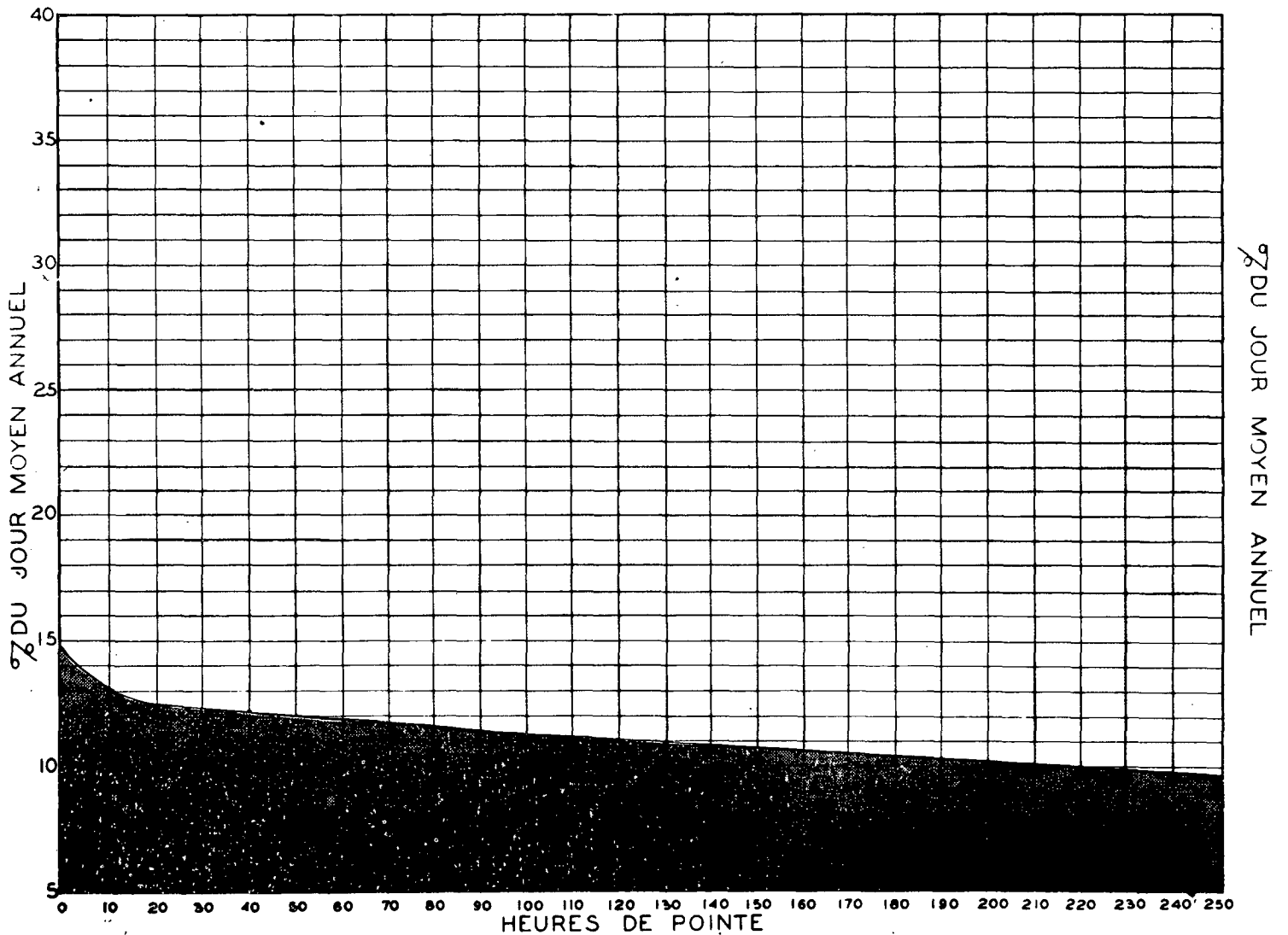
RELATION ENTRE LES HEURES DE POINTE ET LE JOUR MOYEN ANNUEL STATION: REPENTIGNY ROUTE N° 2
