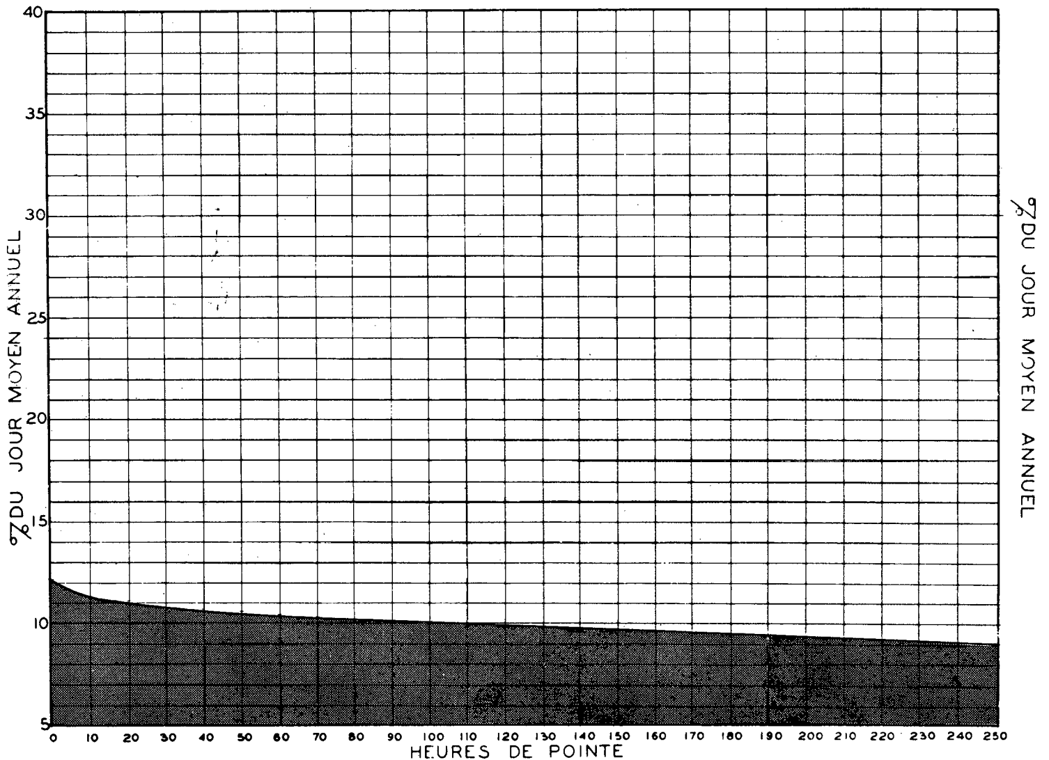
RELATION ENTRE LES HEURES DE POINTE ET LE JOUR MOYEN ANNUEL STATION: LONGUEUIL (VOIE EST) ROUTE N° 3
