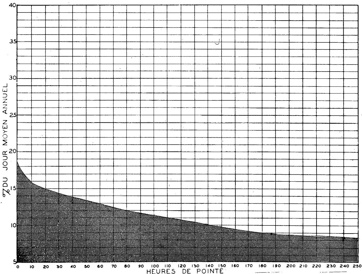
RELATION ENTRE LES HEURES DE POINTE ET LE JOUR MOYEN ANNUEL STATION: GRANBY ROUTE N° 1
