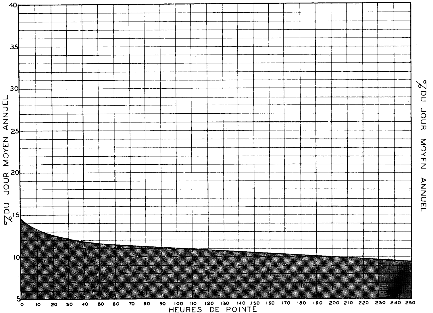
RELATION ENTRE LES HEURES DE POINTE ET LE JOUR MOYEN ANNUEL STATION: LAPRAIRIE (VOIE OUEST) ROUTE N° 3
