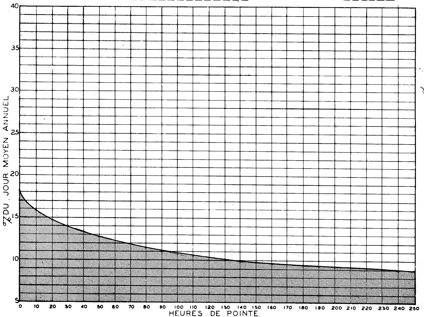
RELATION ENTRE LES HEURES DE POINTE ET LE JOUR MOYEN ANNUEL STATION NEUFCHATEL ROUTE N° R. S.
