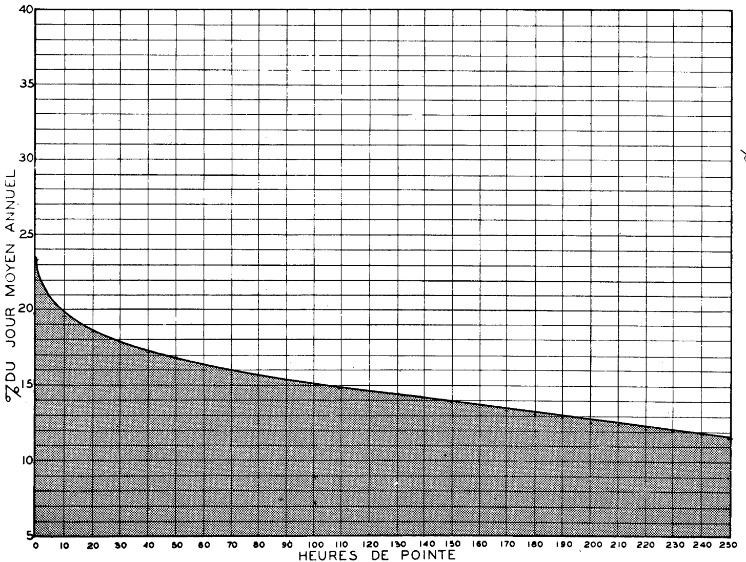
RELATION ENTRE LES HEURES DE POINTE ET LE JOUR MOYEN ANNUEL STATION: TERREBONNE (VOIE EST) ROUTE N° 18
