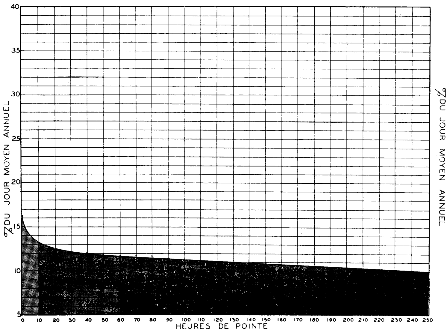
RELATION ENTRE LES HEURES DE POINTE ET LE JOUR MOYEN ANNUEL STATION: PREVILLE 2 VOIES ROUTE N° 3
