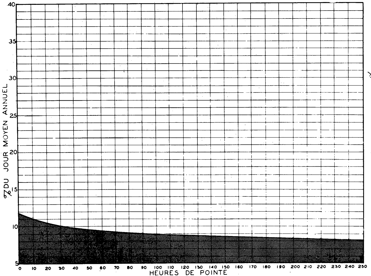
RELATION ENTRE LES HEURES DE POINTE ET LE JOUR MOYEN ANNUEL STATION: STE-CATHERINE 2 VOIES ROUTE N° 9
