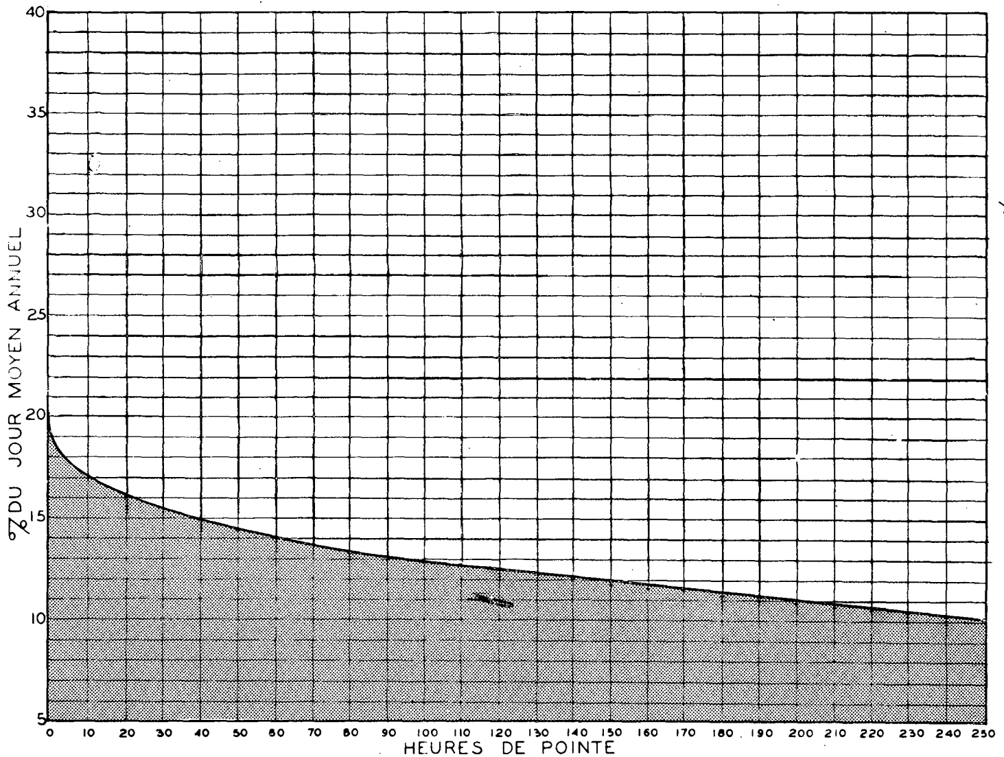
RELATION ENTRE LES HEURES DE POINTE ET LE JOUR MOYEN ANNUEL STATION MAGOG (2 VOIES) ROUTE N° 1
