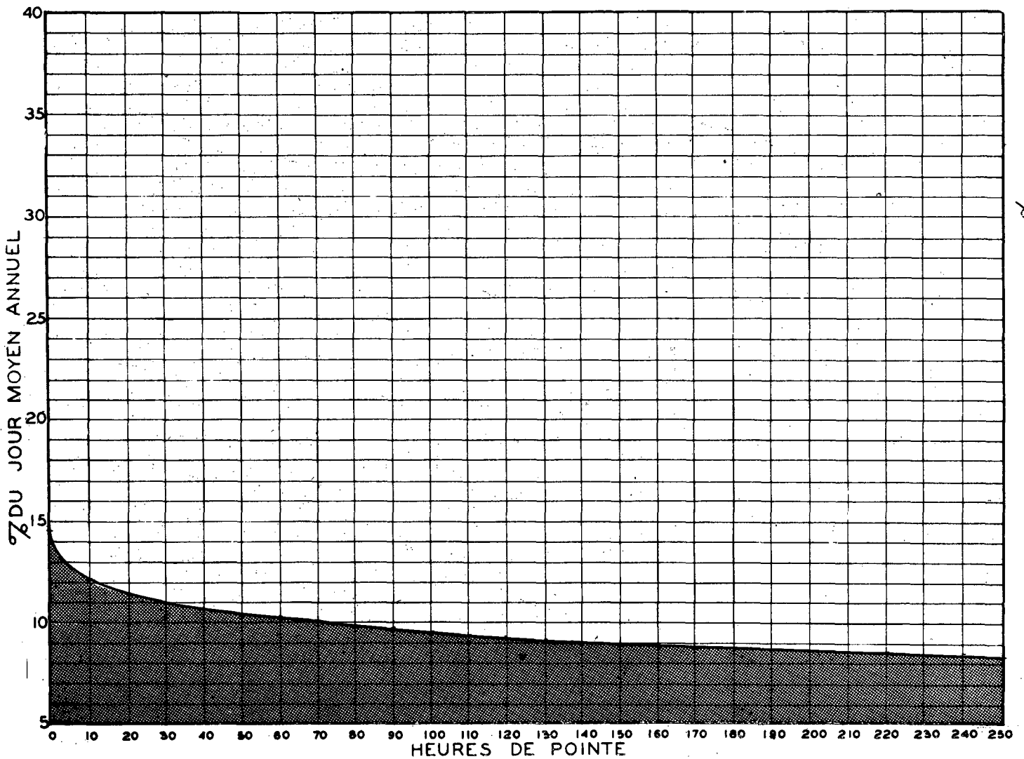
RELATION ENTRE LES HEURES DE POINTE ET LE JOUR MOYEN ANNUEL STATION: CHARNY (RTE DU SAULT) ROUTE N° _____
