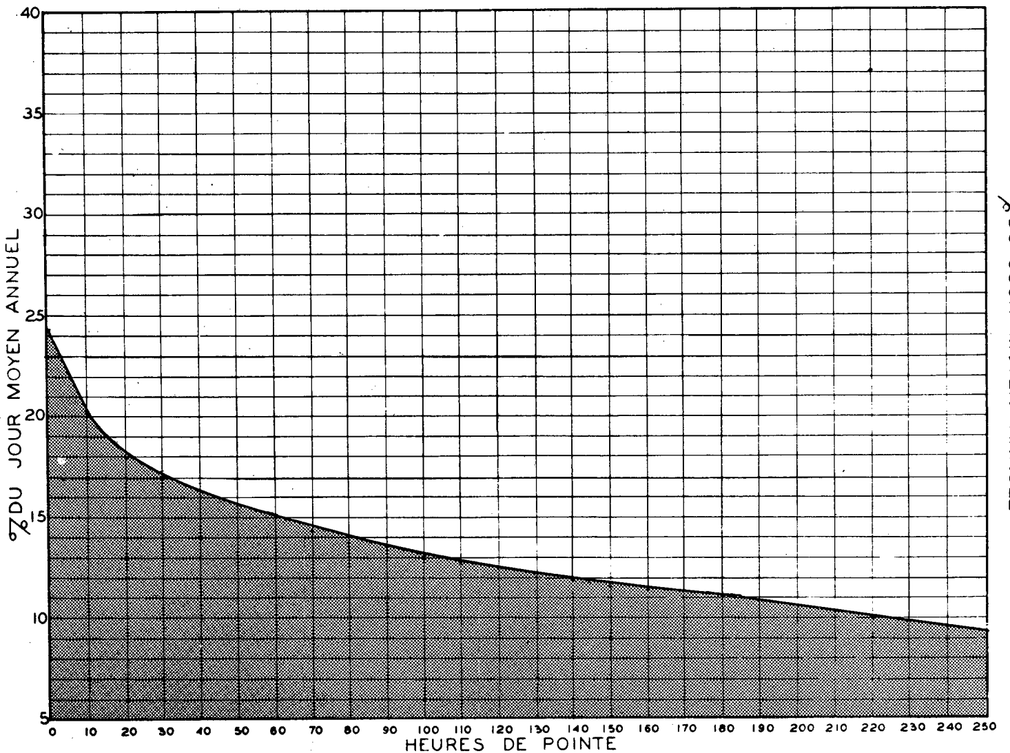
RELATION ENTRE LES HEURES DE POINTE ET LE JOUR MOYEN ANNUEL STATION: STE - HÉLÈNE (VOIE NORD) ROUTE N° 9
