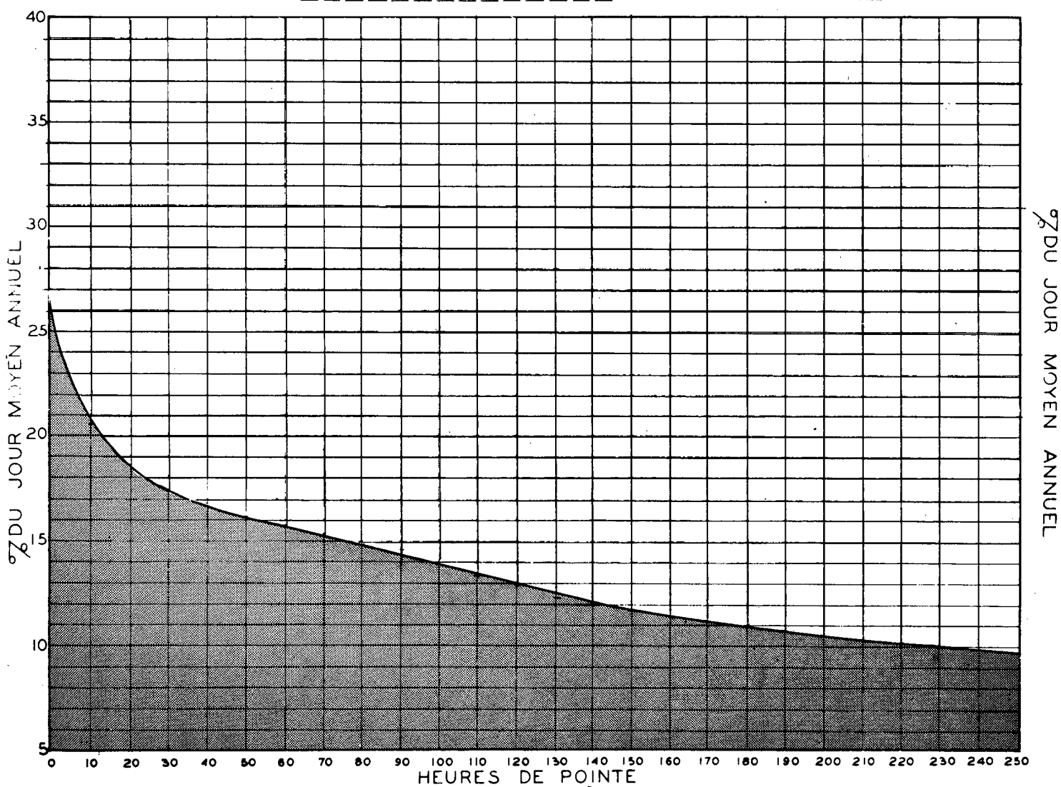
RELATION ENTRE LES HEURES DE POINTE ET LE JOUR MOYEN ANNUEL STATION N.D. DES LAURENTIDES (2 VOIES) ROUTE N° 54
