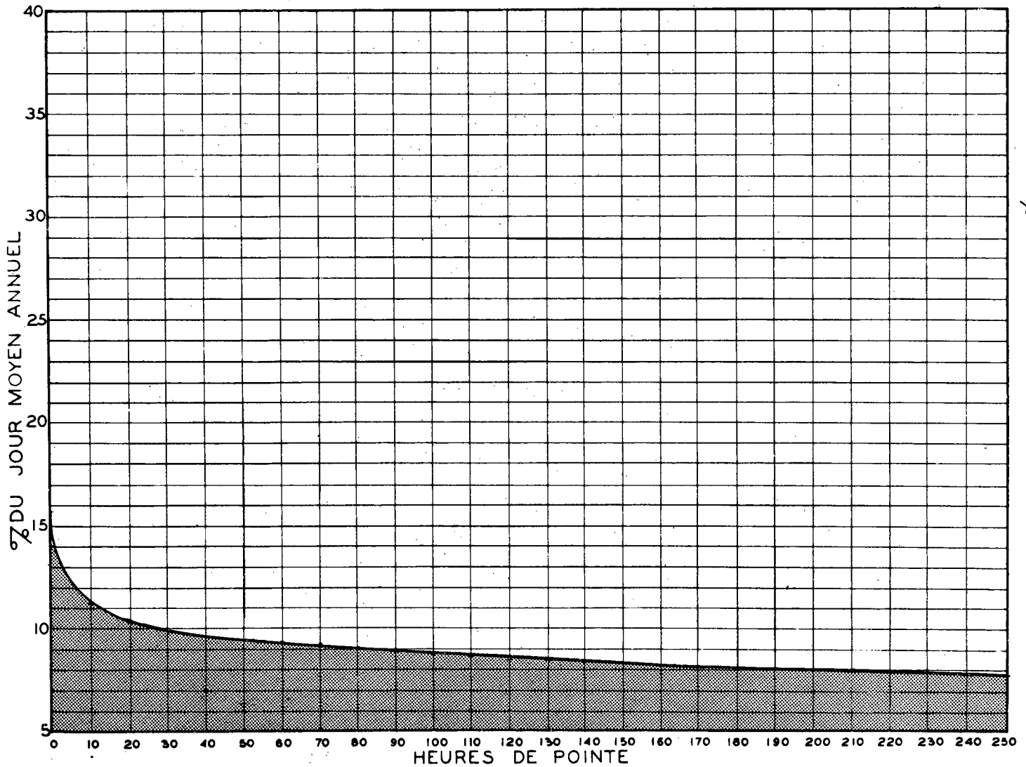
RELATION ENTRE LES HEURES DE POINTE ET LE JOUR MOYEN ANNUEL STATION: LAPRAIRIE (VOIE OUEST) ROUTE N° 9
