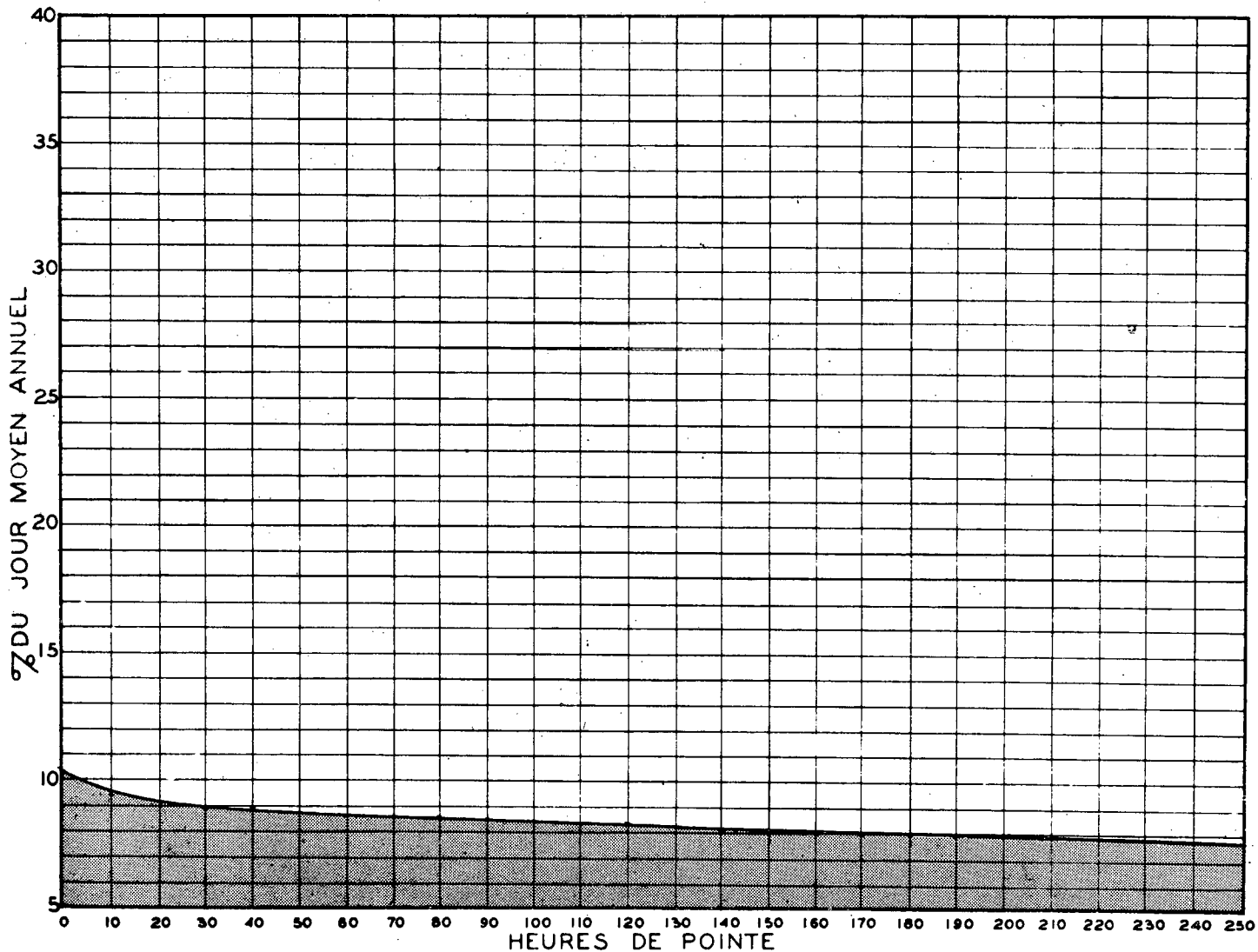
RELATION ENTRE LES HEURES DE POINTE ET LE JOUR MOYEN ANNUEL STATION: GREENFIELD PARK 2VOIES ROUTE N° 9
