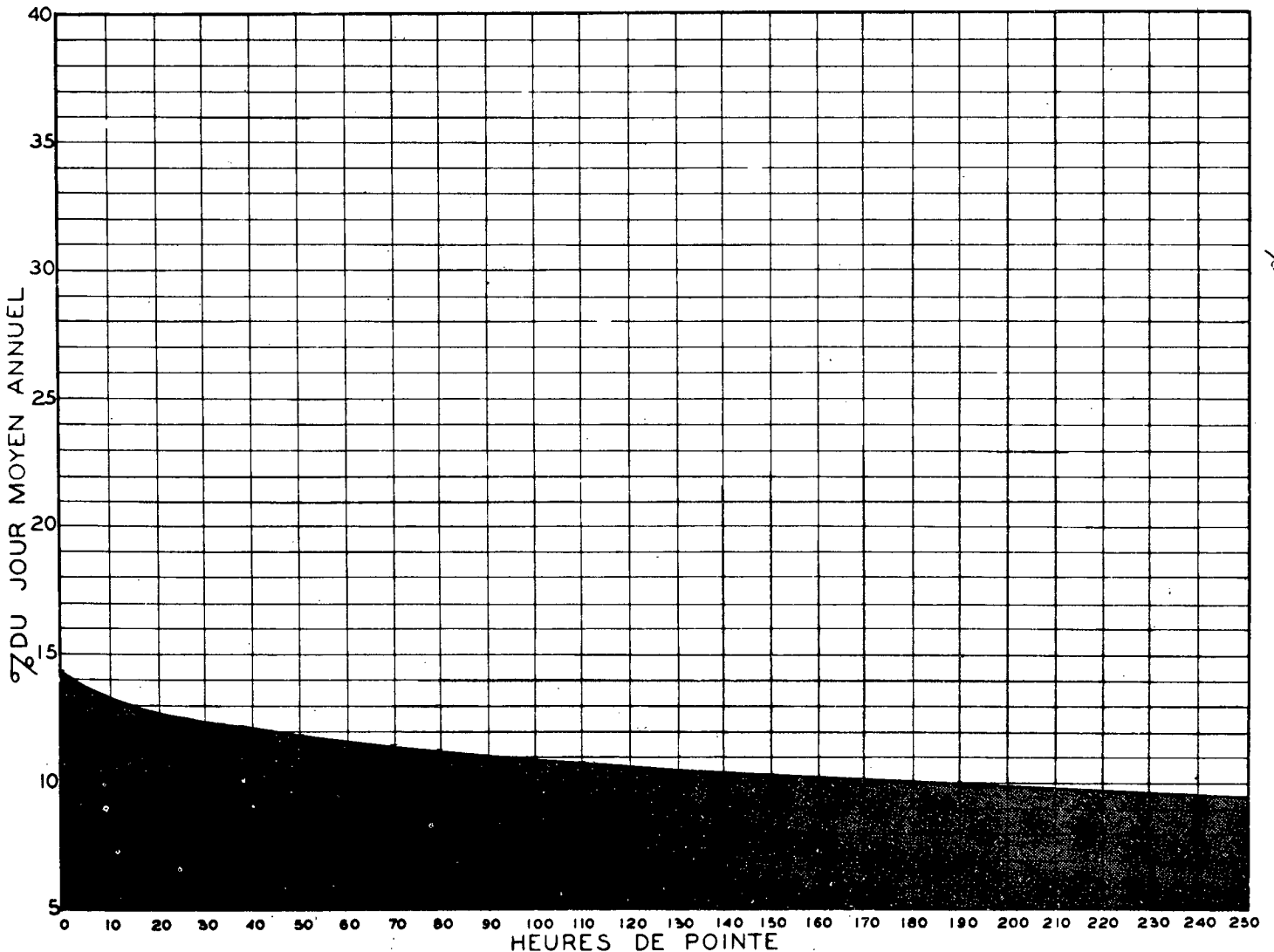
RELATION ENTRE LES HEURES DE POINTE ET LE JOUR MOYEN ANNUEL STATION: ST-HUBERT (VOIE NORD) ROUTE N° 9
