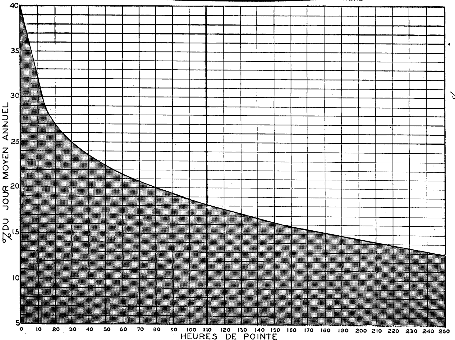
RELATION ENTRE LES HEURES DE POINTE ET LE JOUR MOYEN ANNUEL STATION: GRANDES-PILES ROUTE N°
