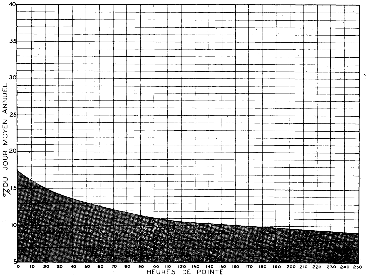
RELATION ENTRE LES HEURES DE POINTE ET LE JOUR MOYEN ANNUEL STATION: LAPRAIRIE (VOIE EST) ROUTE N° 3
