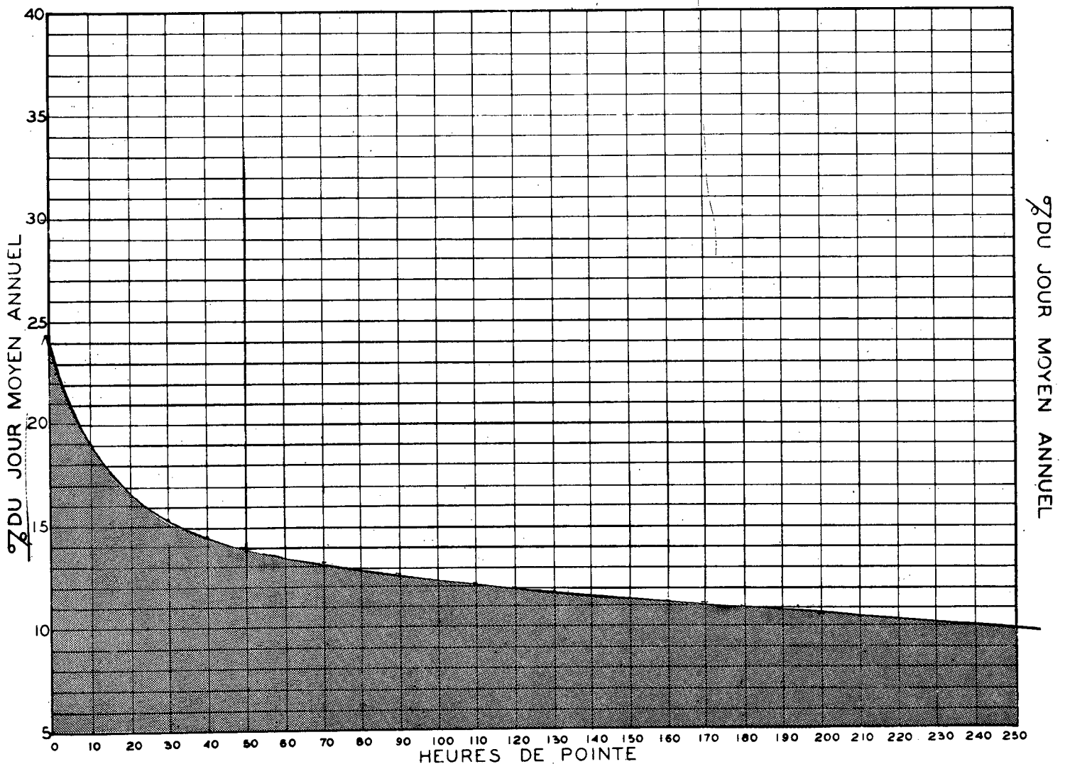
RELATION ENTRE LES HEURES DE POINTE ET LE JOUR MOYEN ANNUEL STATION: ANCIENNE LORETTE ROUTE N° AÉROPORT
