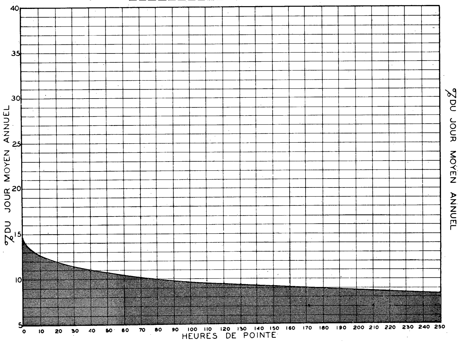
RELATION ENTRE LES HEURES DE POINTE ET LE JOUR MOYEN ANNUEL STATION: ST-NICOLAS ROUTE N° 3
