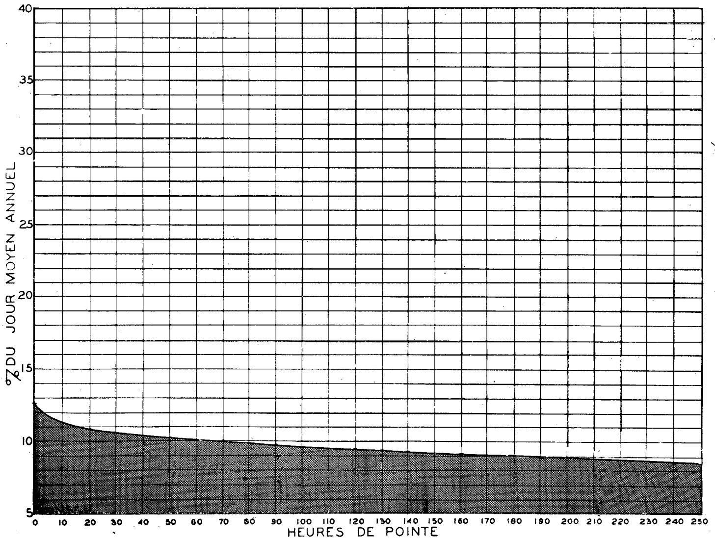
RELATION ENTRE LES HEURES DE POINTE ET LE JOUR MOYEN ANNUEL — STATION CHARLEMAGNE ROUTE N° 48
