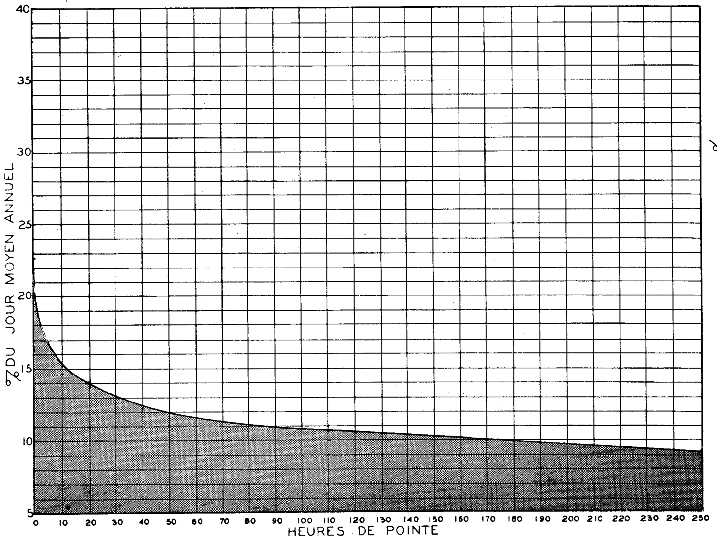
RELATION ENTRE LES HEURES DE POINTE ET LE JOUR MOYEN ANNUEL STATION: POINTE-CLAIRE (VOIE NORD) ROUTE N° 2
