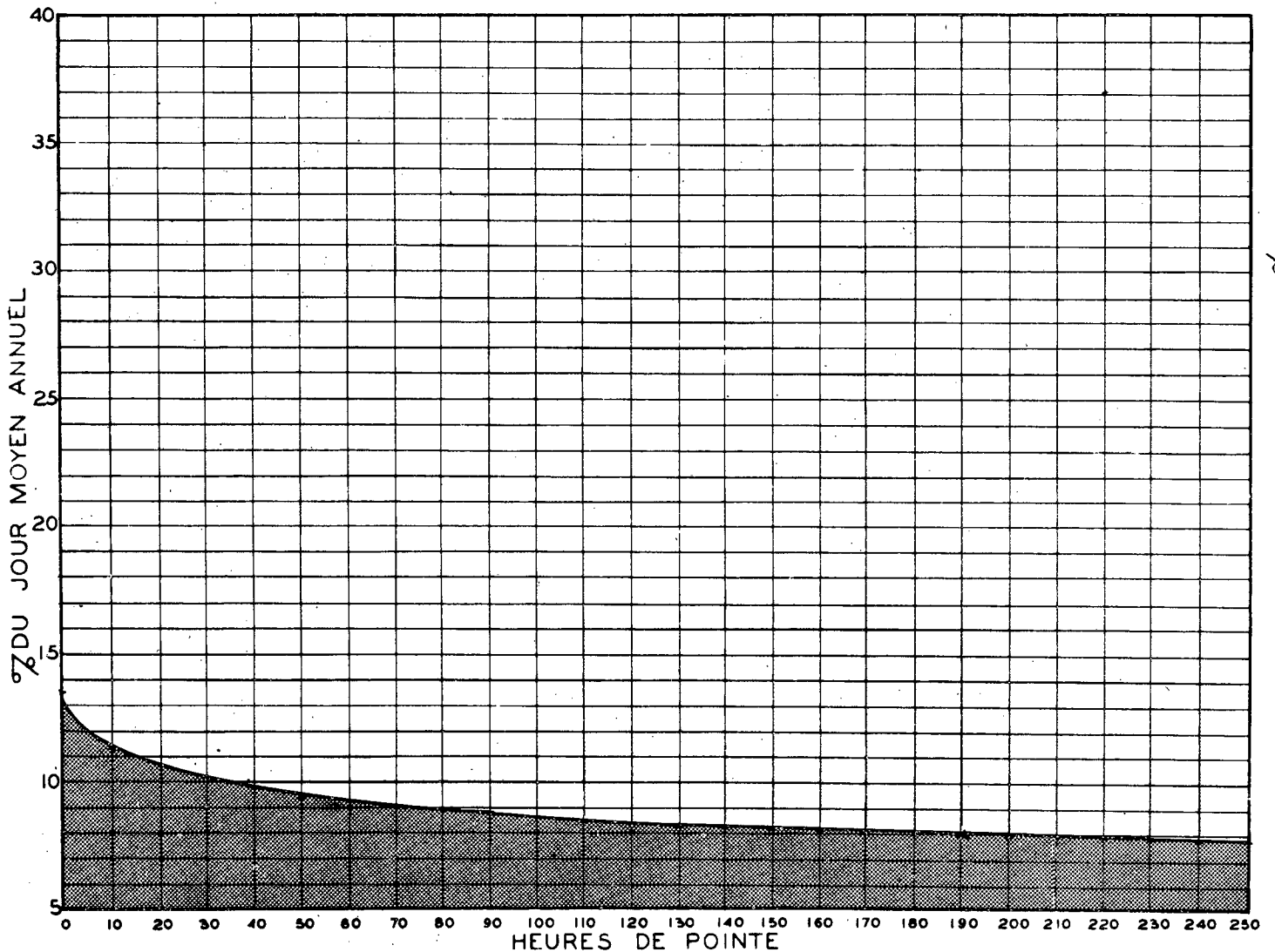
RELATION ENTRE LES HEURES DE POINTE ET LE JOUR MOYEN ANNUEL STATION: GREENFIELD PARK (VOIE OUEST) ROUTE N° 9
