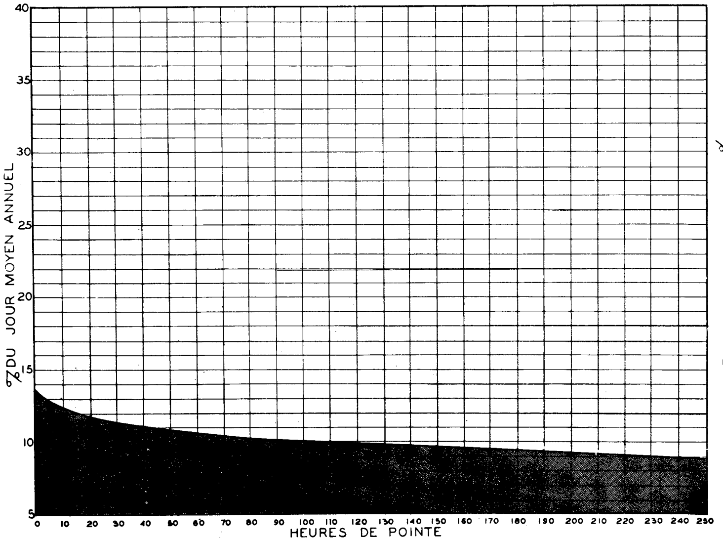
RELATION ENTRE LES HEURES DE POINTE ET LE JOUR MOYEN ANNUEL STATION: ST-HUBERT (VOIE SUD) ROUTE N° 9
