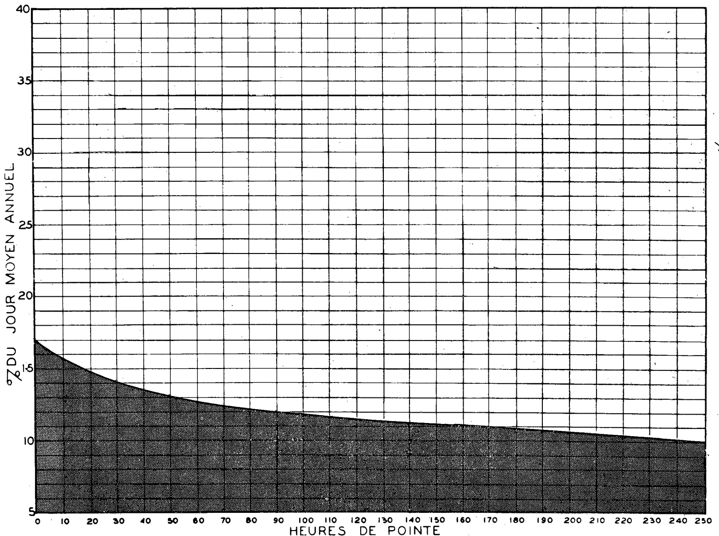
RELATION ENTRE LES HEURES DE POINTE ET LE JOUR MOYEN ANNUEL STATION: ST-JEAN (2 VOIES) ROUTE N° 7
