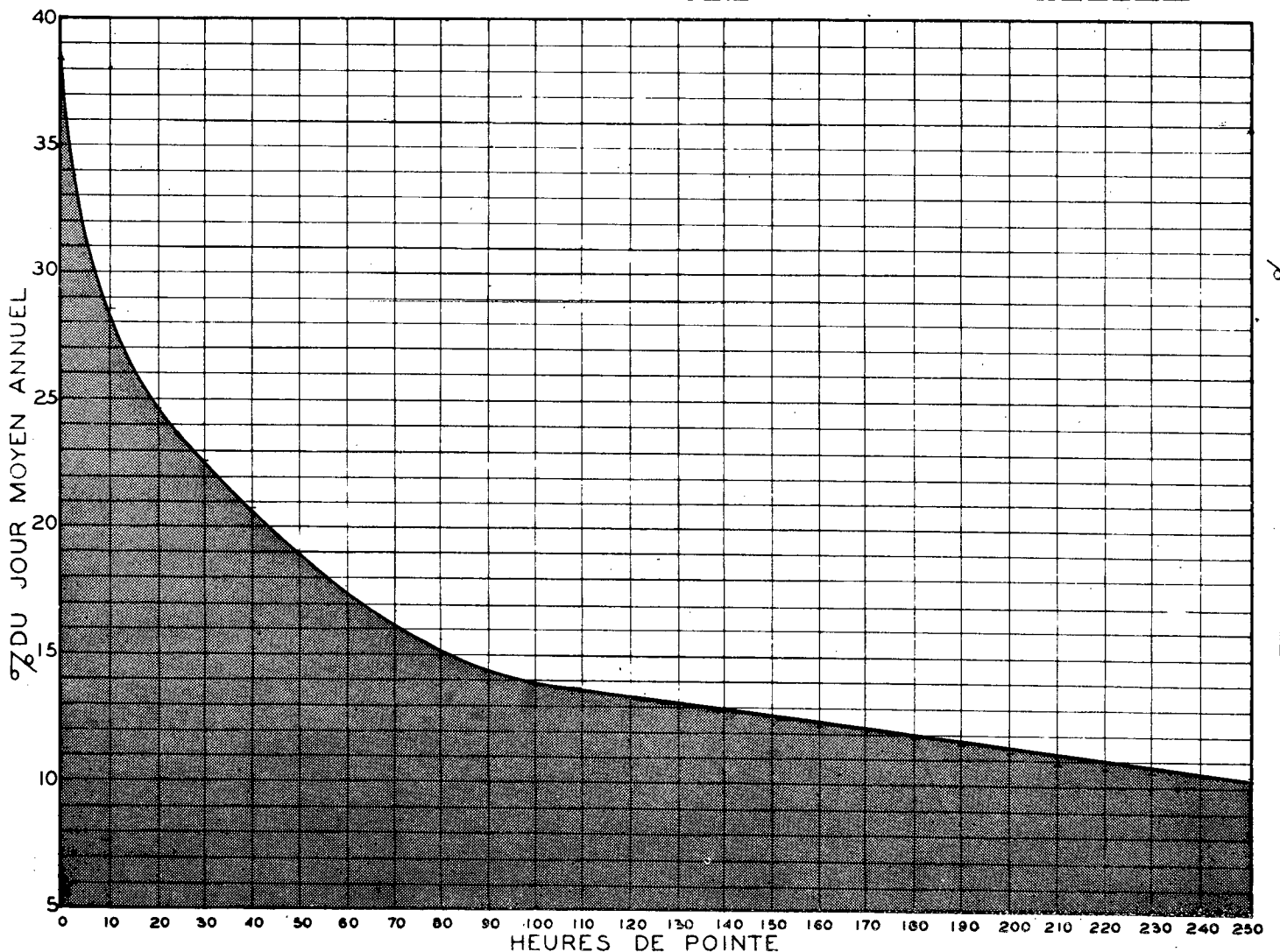
RELATION ENTRE LES HEURES DE POINTE ET LE JOUR MOYEN ANNUEL STATION: LAVAL (RUE ST-JEAN BAPTISTE) ROUTE N° _____
