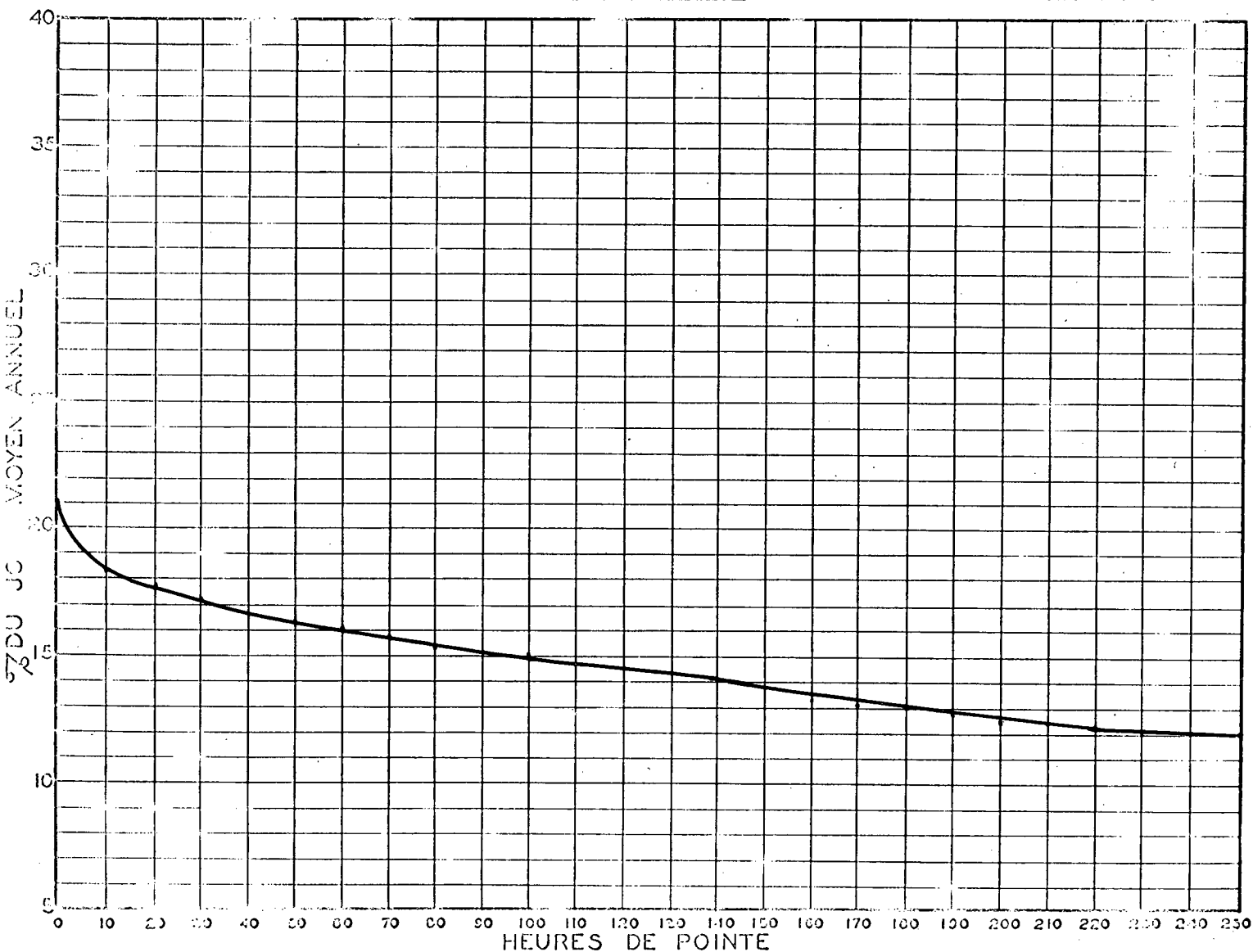
RELATION ENTRE LES HEURES DE POINTE ET LE JOUR MOYEN ANNUEL STATION: ANC. LORETTE ROUTE N° 2
