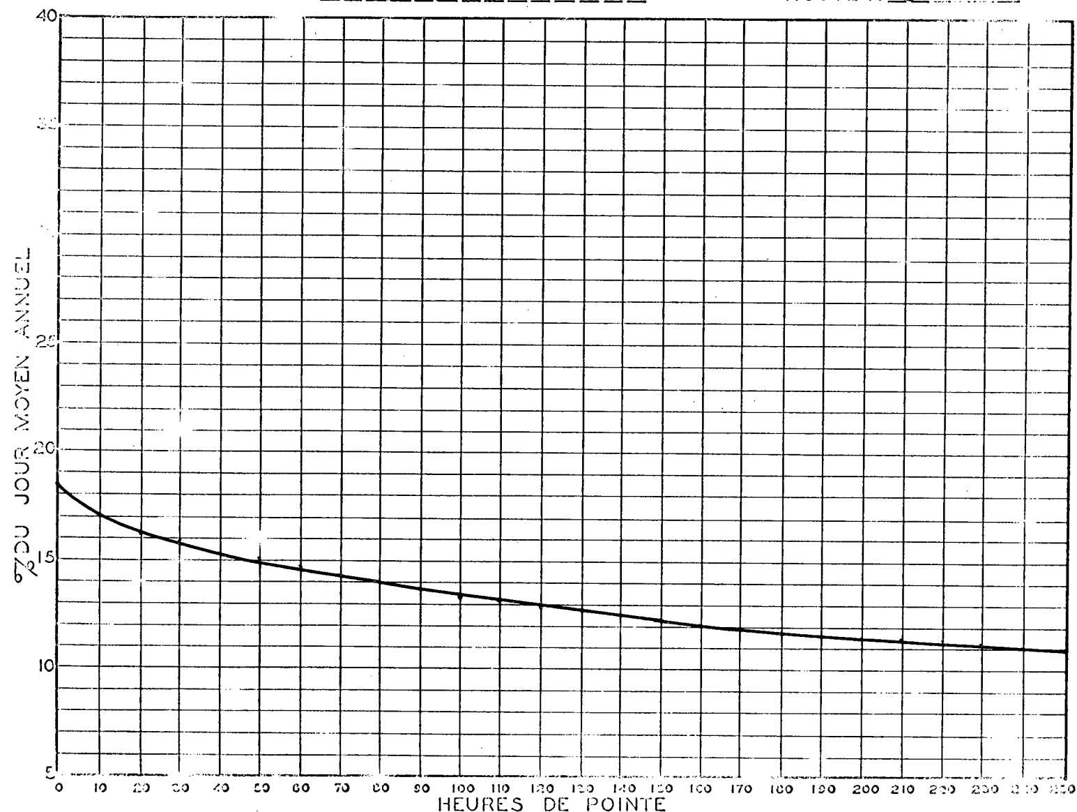
RELATION ENTRE LES HEURES DE POINTE ET LE JOUR MOYEN ANNUEL STATION: WARWICK ROUTE N° 5
