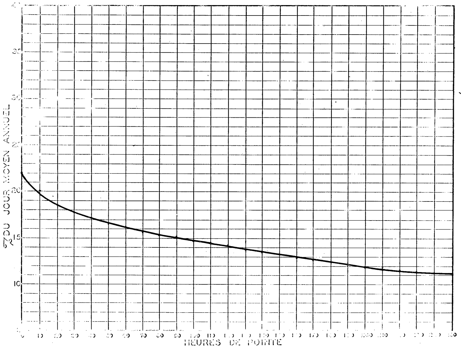
RELATION ENTRE LES HEURES DE POINTE ET LE JOUR MOYEN ANNUEL STATION: ST-BRUNO ROUTE N°16
