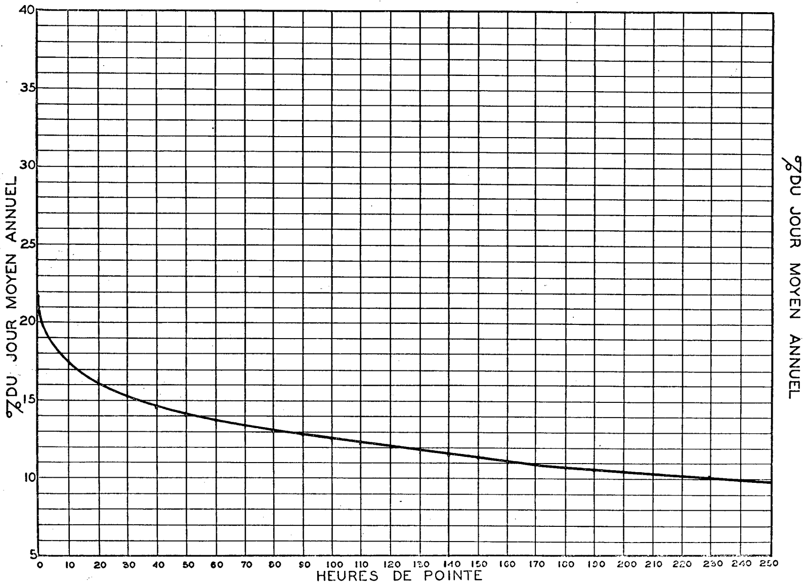
RELATION ENTRE LES HEURES DE POINTE ET LE JOUR MOYEN ANNUEL STATION: ST-EUSTACHE ROUTE N° 8
