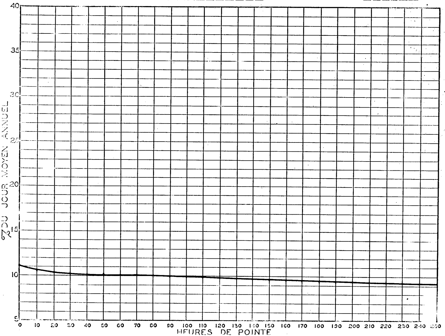
RELATION ENTRE LES HEURES DE POINTE ET LE JOUR MOYEN ANNUEL STATION: ST-NICOLAS 2 VOIES ROUTE N° 2-9
