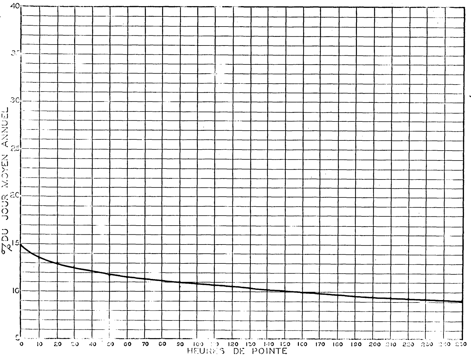
RELATION ENTRE LES HEURES DE POINTE ET LE JOUR MOYEN ANNUEL STATION: VARENNES ROUTE N° 3
