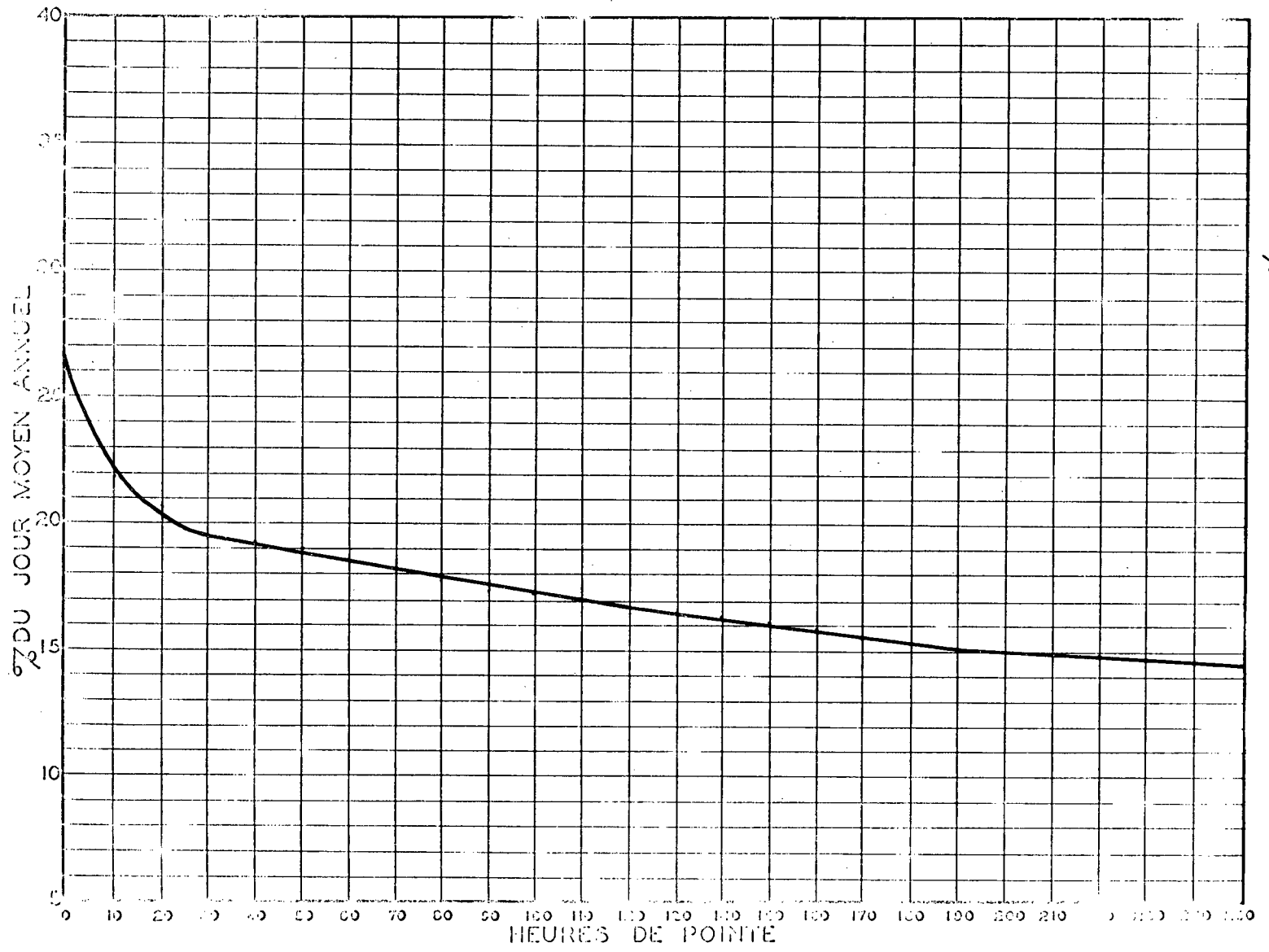
RELATION ENTRE LES HEURES DE POINTE ET LE JOUR MOYEN ANNUEL STATION: DOUGLASTOWN ROUTE N° 6
