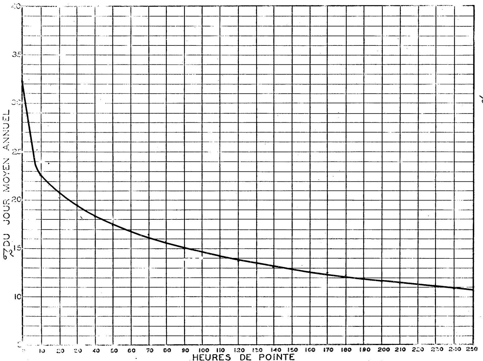
RELATION ENTRE LES HEURES DE POINTE ET LE JOUR MOYEN ANNUEL STATION: CHAMBORD ROUTE N° 55
