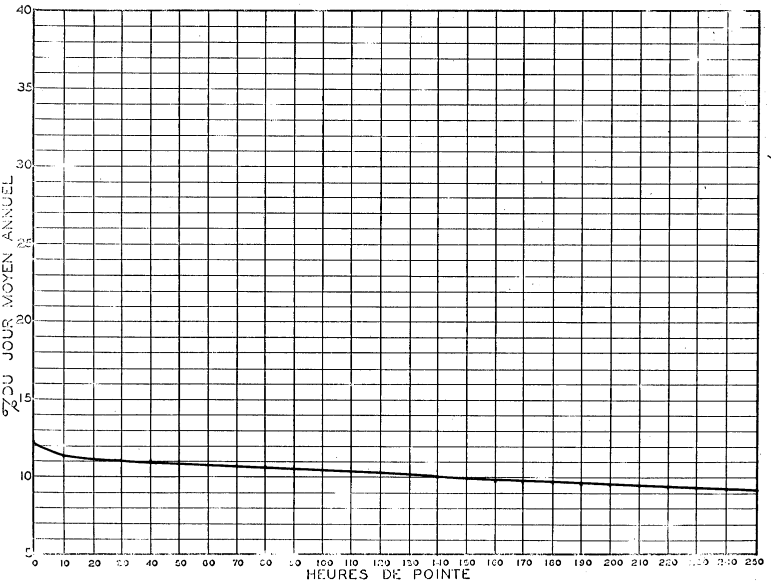
RELATION ENTRE LES HEURES DE POINTE ET LE JOUR MOYEN ANNUEL STATION: ST-NICOLAS VOIE EST ROUTE N° 2-9
