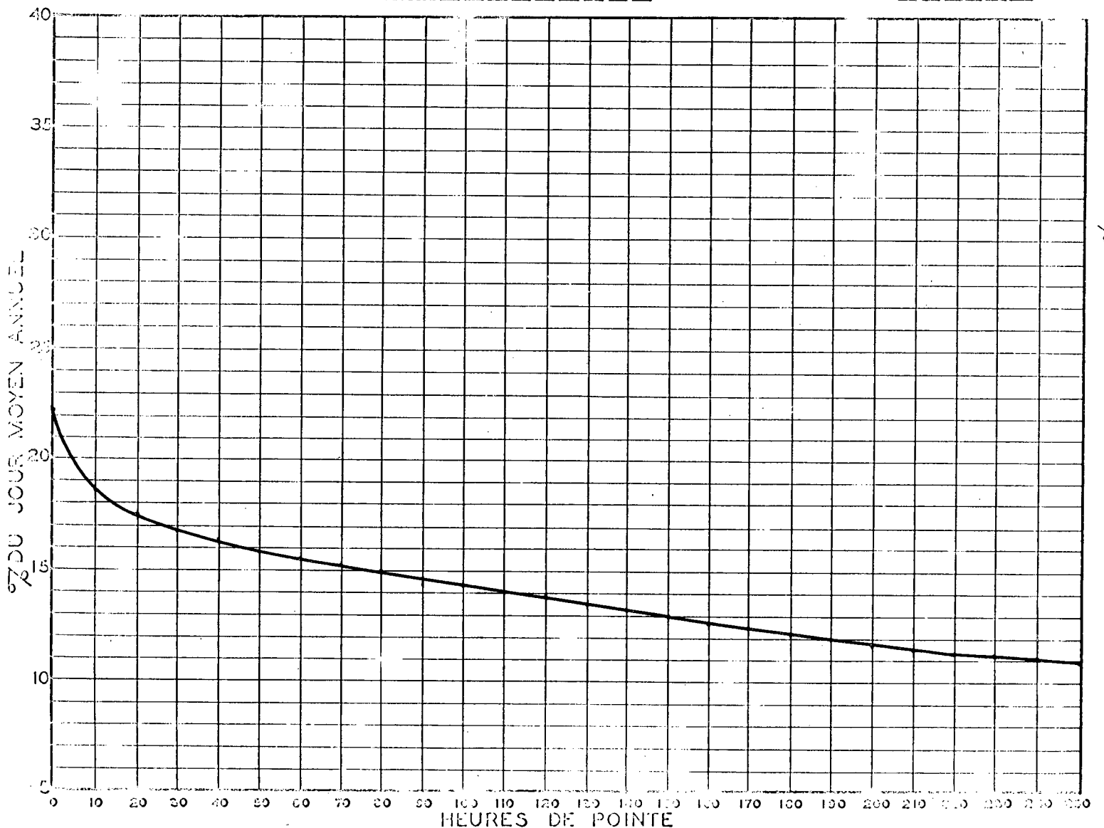
RELATION ENTRE LES HEURES DE POINTE ET LE JOUR MOYEN ANNUEL STATION: ST-FRÉDÉRIC ROUTE N° 1
