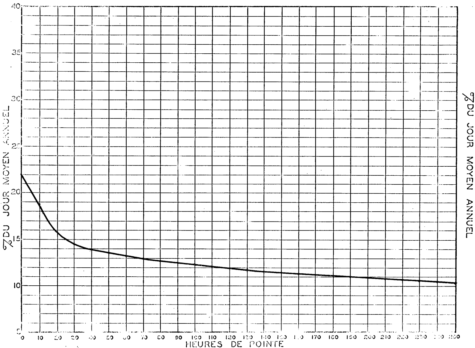
RELATION ENTRE LES HEURES DE POINTE ET LE JOUR MOYEN ANNUEL STATION: ST-BERNARD ROUTE N° J
