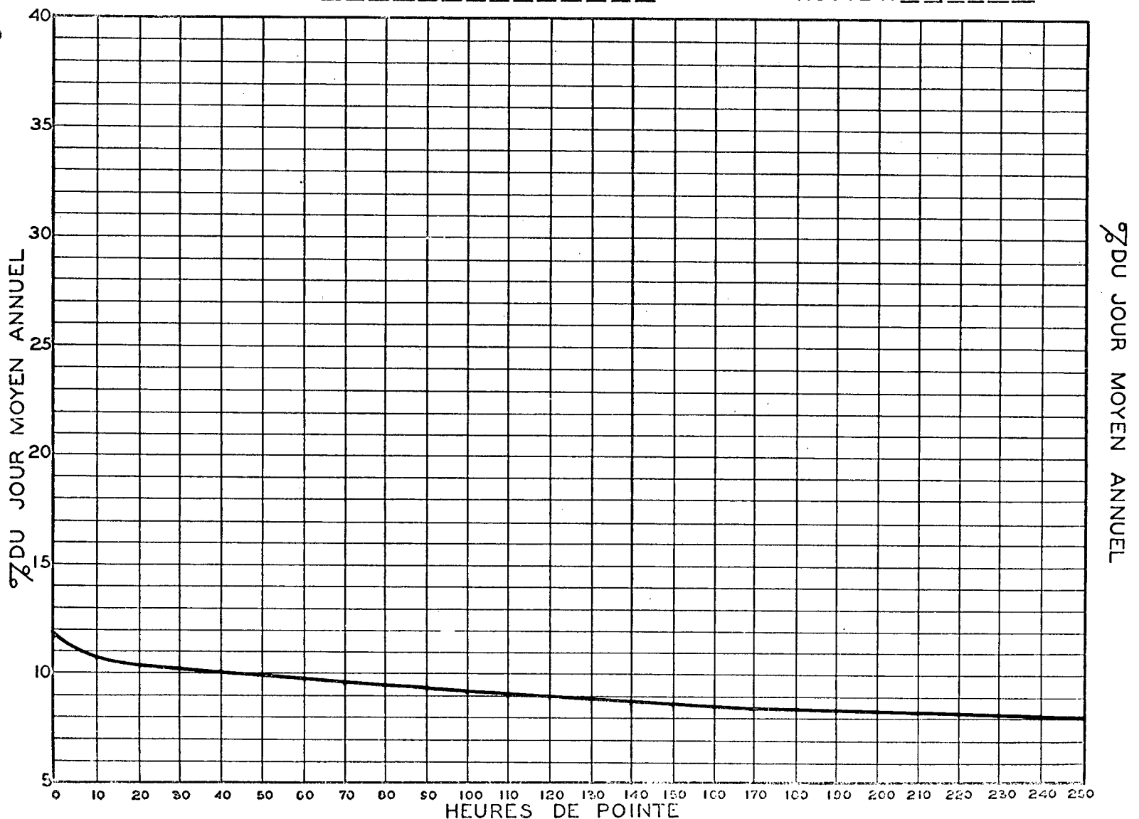
RELATION ENTRE LES HEURES DE POINTE ET LE JOUR MOYEN ANNUEL STATION: STE-PHILOMÈNE ROUTE N° 4
