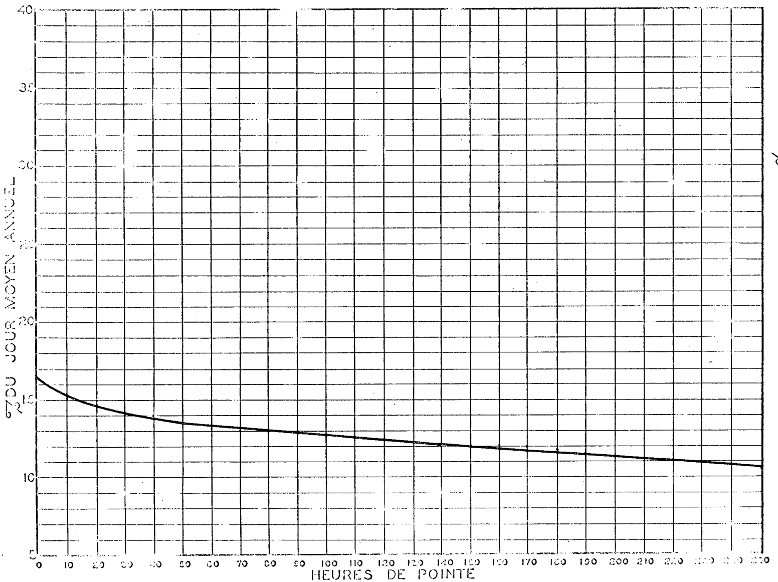
RELATION ENTRE LES HEURES DE POINTE ET LE JOUR MOYEN ANNUEL STATION: WINDSOR ROUTE N° 5-22
