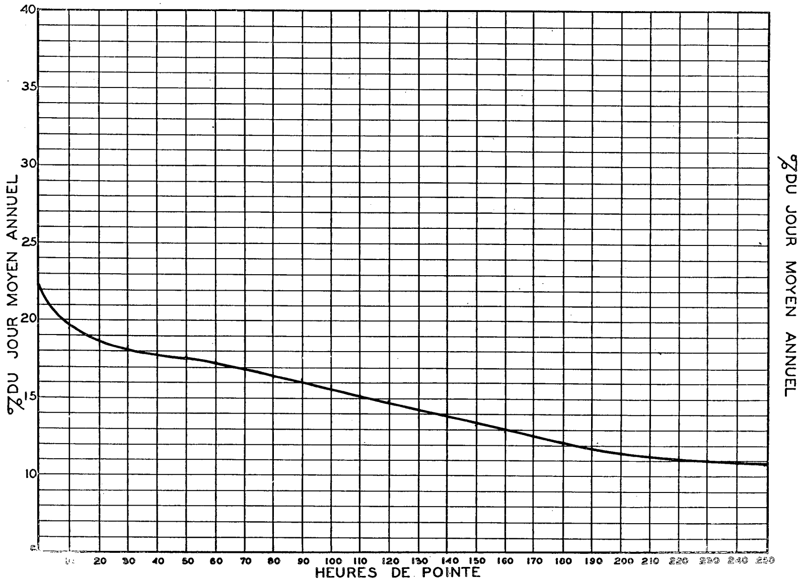
RELATION ENTRE LES HEURES DE POINTE ET LE JOUR MOYEN ANNUEL STATION: STE-MARTHE ROUTE N° 29
