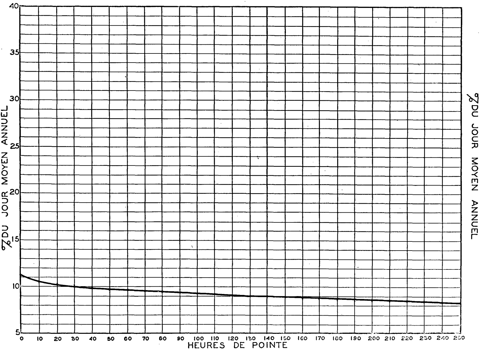
RELATION ENTRE LES HEURES DE POINTE ET LE JOUR MOYEN ANNUEL STATION: LÉRY ROUTE N° 3
