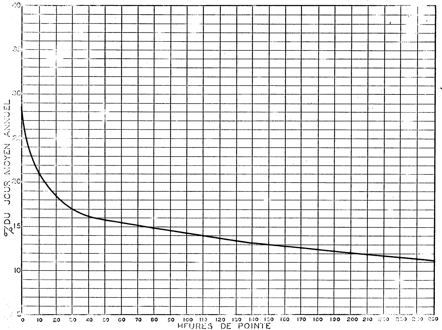
RELATION ENTRE LES HEURES DE POINTE ET LE JOUR MOYEN ANNUEL STATION: MAGOG VOIE NORD ROUTE N° 1
