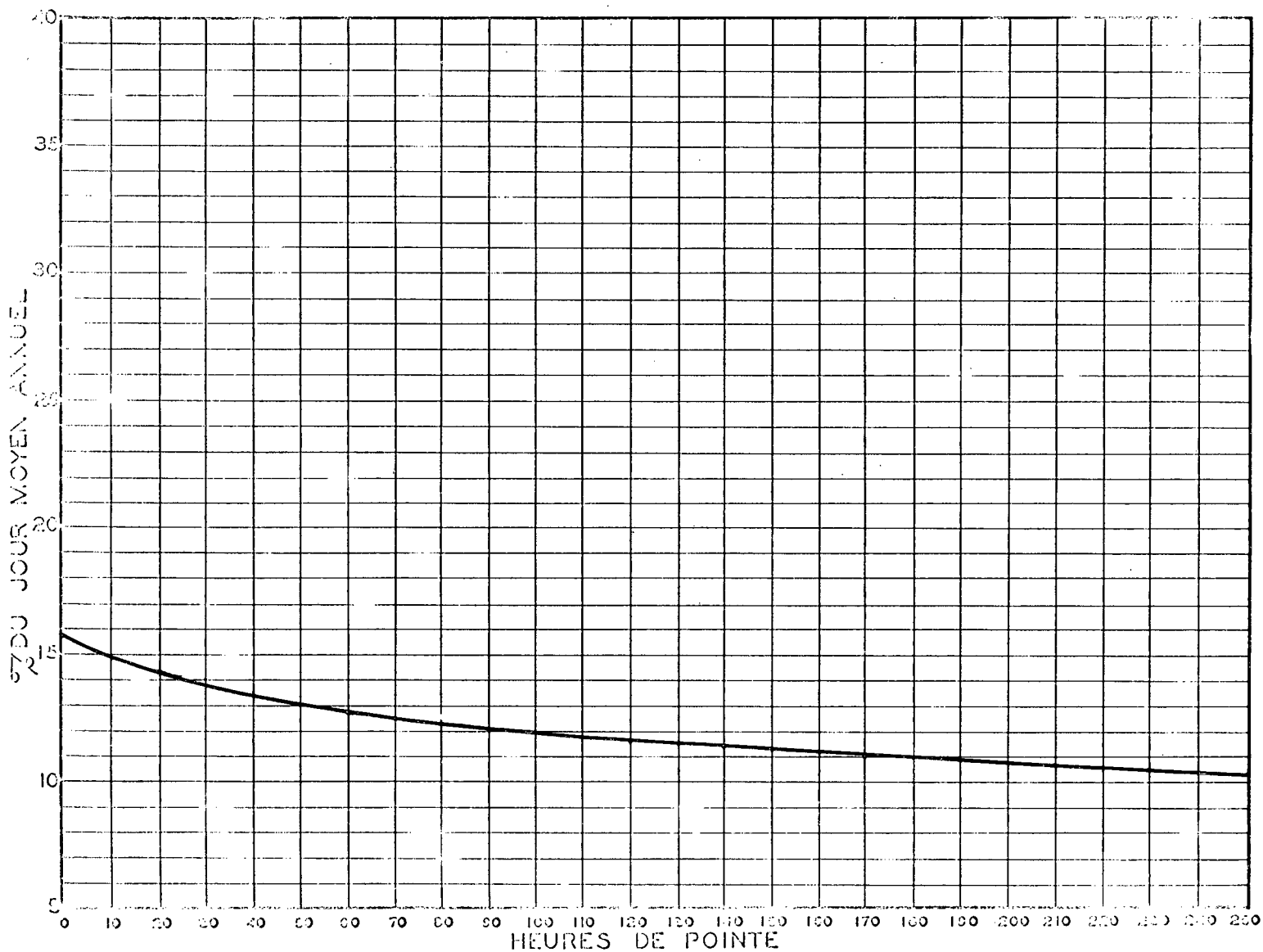
RELATION ENTRE LES HEURES DE POINTE ET LE JOUR MOYEN ANNUEL STATION: LENNOXVILLE ROUTE N° 5-22
