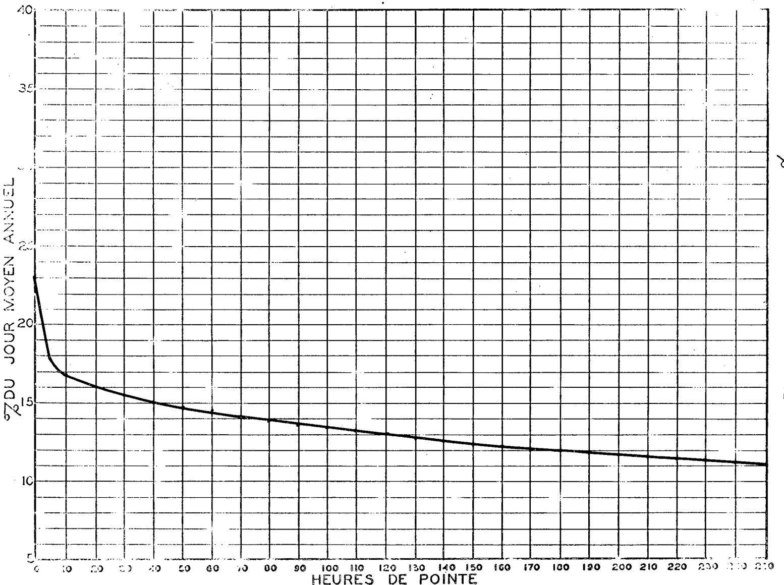
RELATION ENTRE LES HEURES DE POINTE ET LE JOUR MOYEN ANNUEL STATION: ST-HENRI-DE-TAILLON ROUTE N° 55
