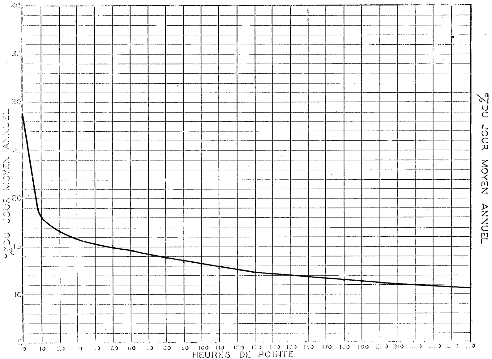
RELATION ENTRE LES HEURES DE POINTE ET LE JOUR MOYEN ANNUEL STATION: ST-ÉTIENNE ROUTE N° 5
