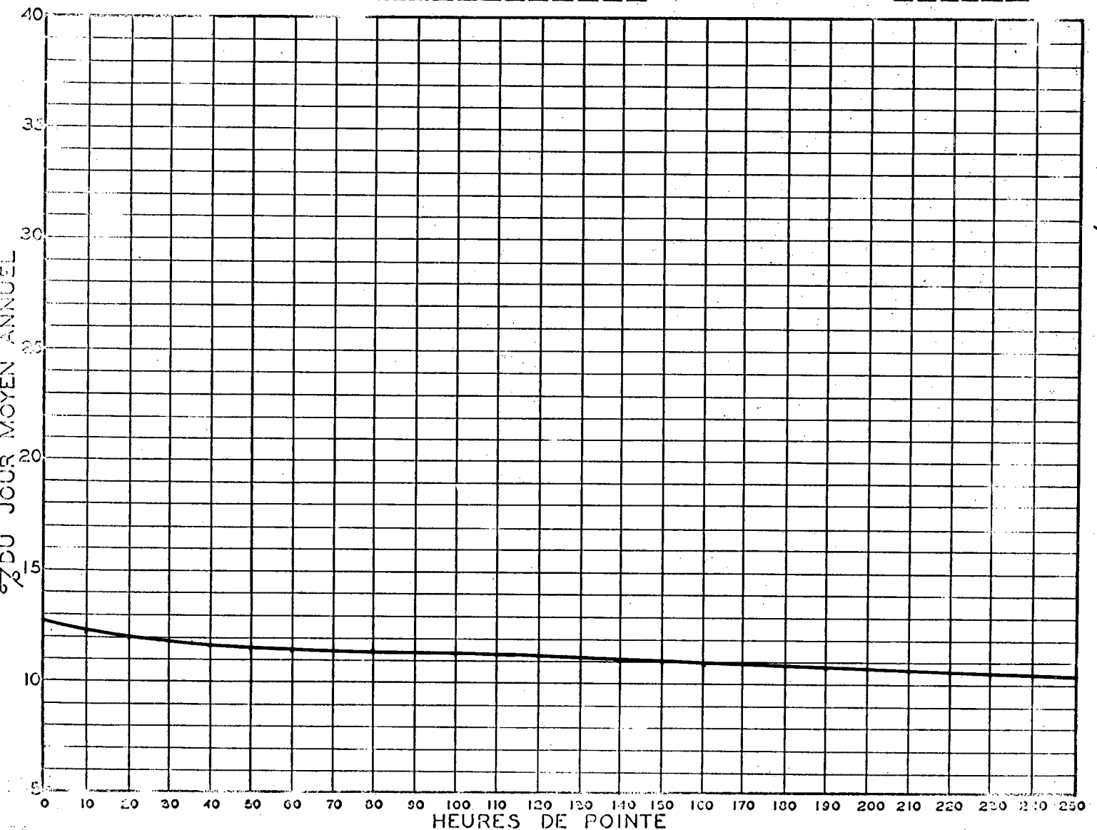
RELATION ENTRE LES HEURES DE POINTE ET LE JOUR MOYEN ANNUEL STATION: ST-NICOLAS VOIE OUEST ROUTE N° 2-9
