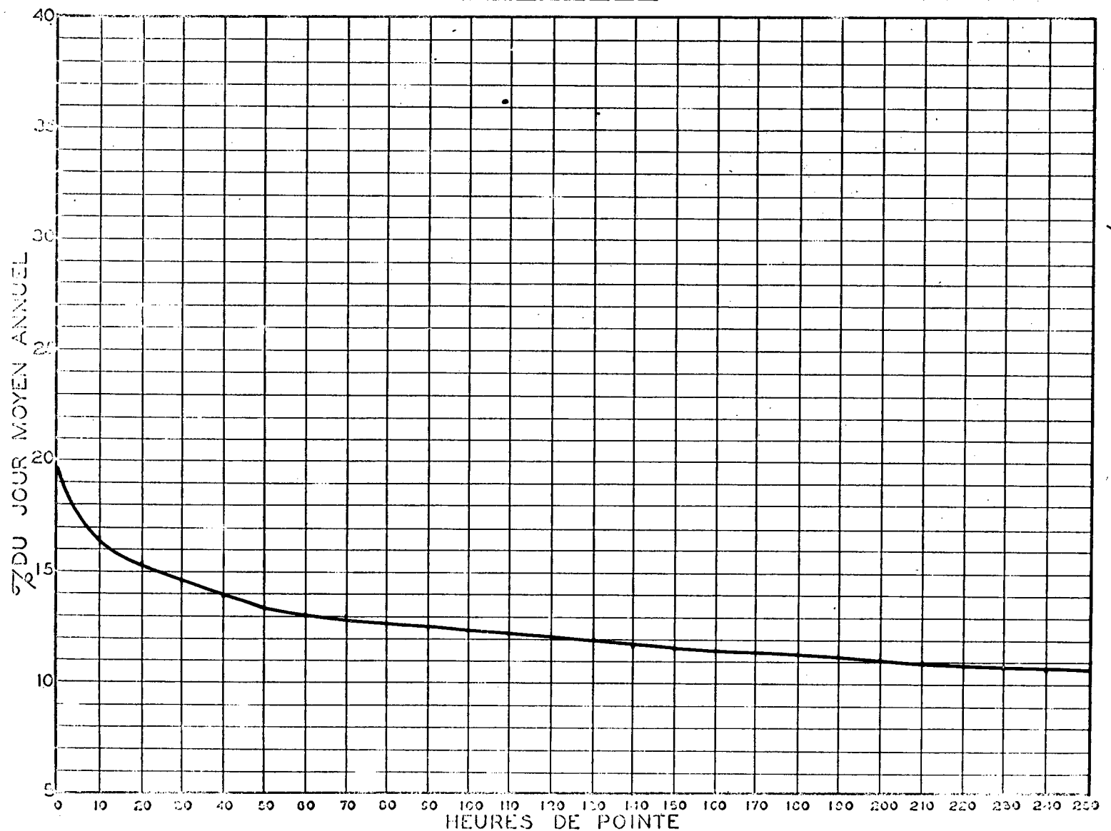
RELATION ENTRE LES HEURES DE POINTE ET LE JOUR MOYEN ANNUEL STATION: BERTHIER (MONTRÉAL) ROUTE N° 2
