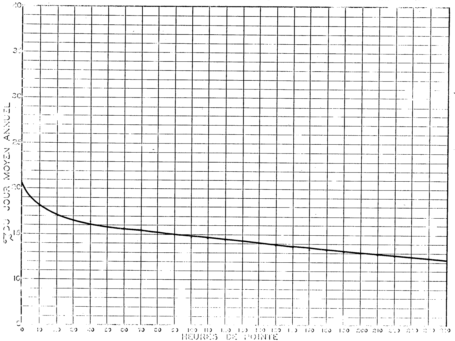
RELATION ENTRE LES HEURES DE POINTE ET LE JOUR MOYEN ANNUEL STATION: ST-JANVIER ROUTE N° 11
