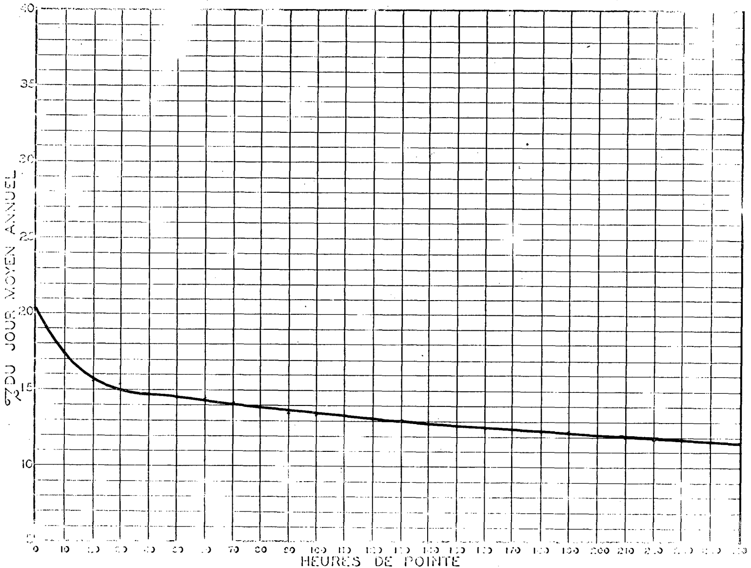
RELATION ENTRE LES HEURES DE POINTE ET LE JOUR MOYEN ANNUEL STATION: PTE FORTUNE ROUTE N°17
