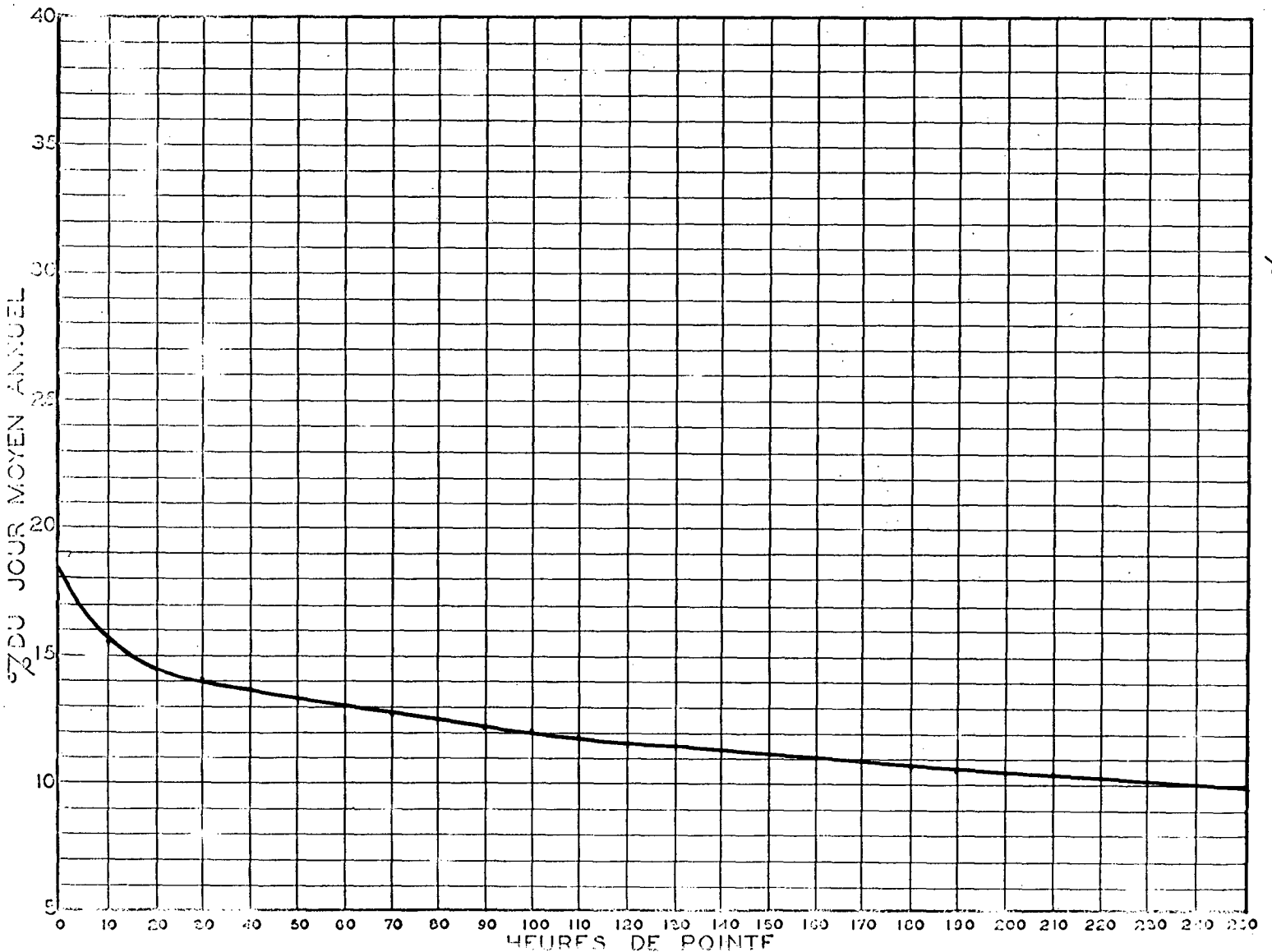
RELATION ENTRE LES HEURES DE POINTE ET LE JOUR MOYEN ANNUEL STATION: ST-GREGOIRE ROUTE N° 3
