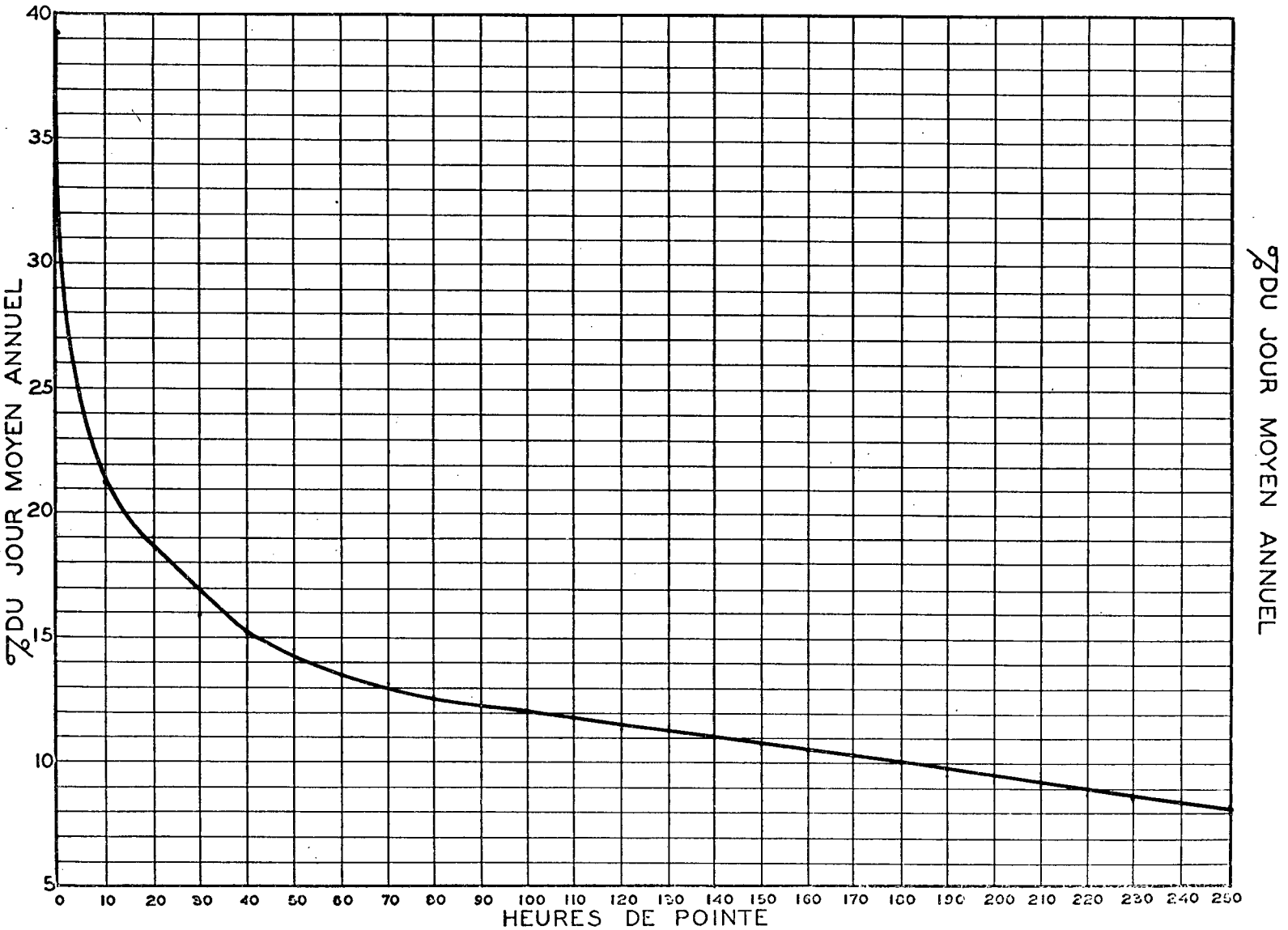
RELATION ENTRE LES HEURES DE POINTE ET LE JOUR MOYEN ANNUEL STATION: SABREVOIS ROUTE N° 7
