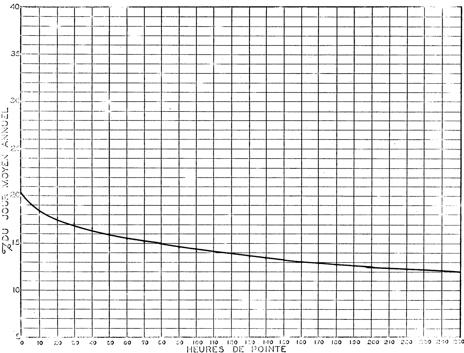
RELATION ENTRE LES HEURES DE POINTE ET LE JOUR MOYEN ANNUEL STATION: BERTHIER ROUTE N° 2
