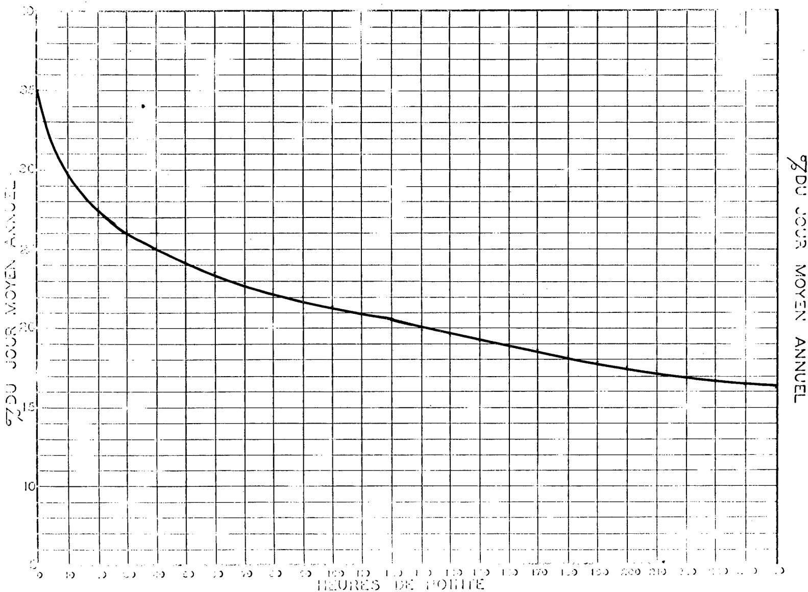
RELATION ENTRE LES HEURES DE POINTE ET LE JOUR MOYEN ANNUEL STATION: STE-AGATHE ROUTE N° 11
