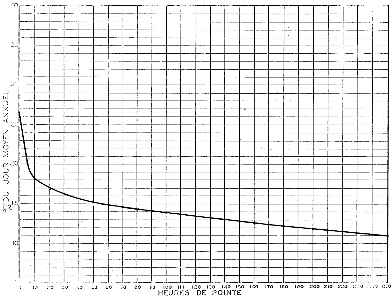
RELATION ENTRE LES HEURES DE POINTE ET LE JOUR MOYEN ANNUEL STATION: PLESSISVILLE ROUTE N° 49
