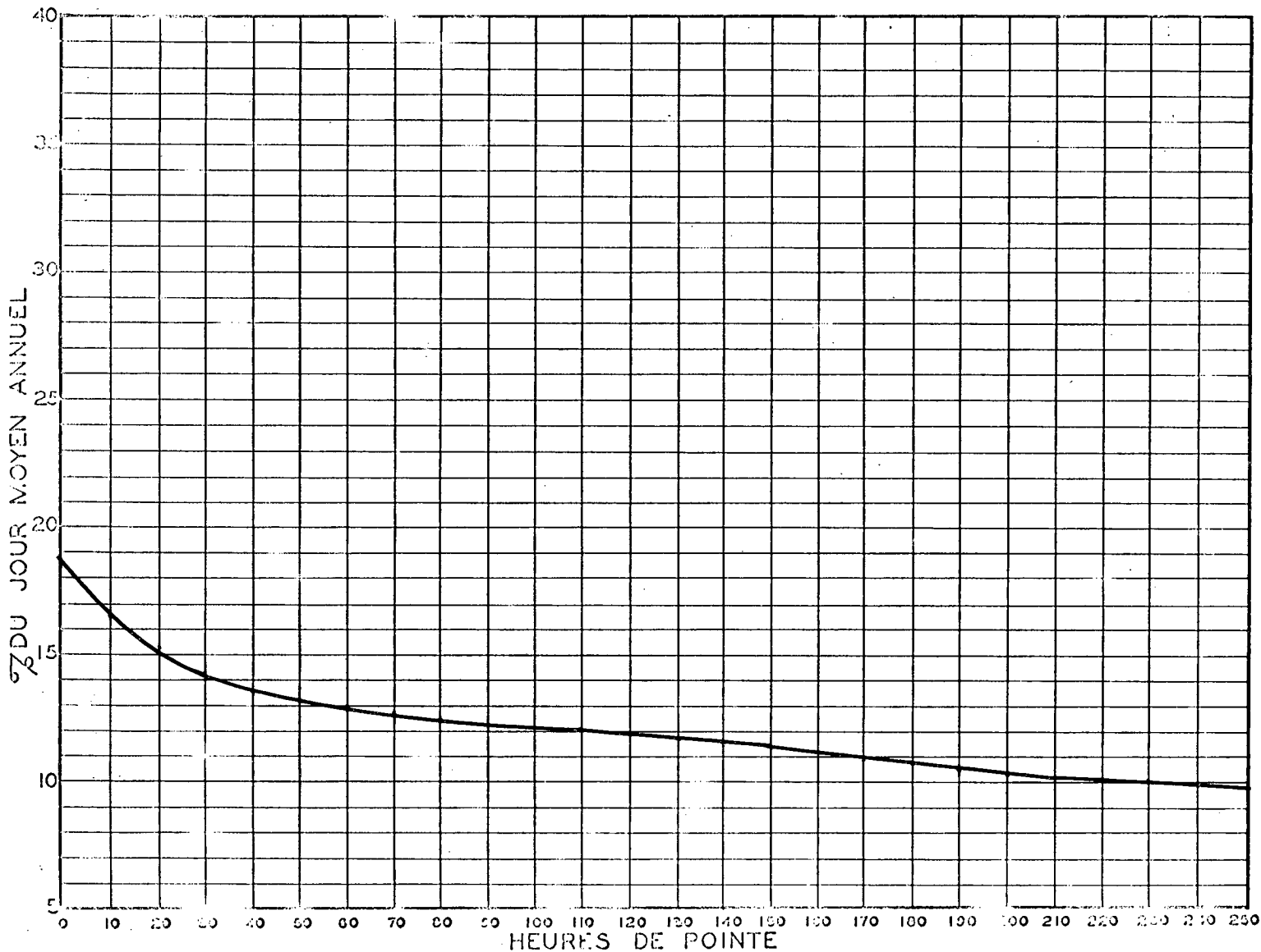
RELATION ENTRE LES HEURES DE POINTE ET LE JOUR MOYEN ANNUEL STATION: ST-TIMOTHÉE ROUTE N° 3
