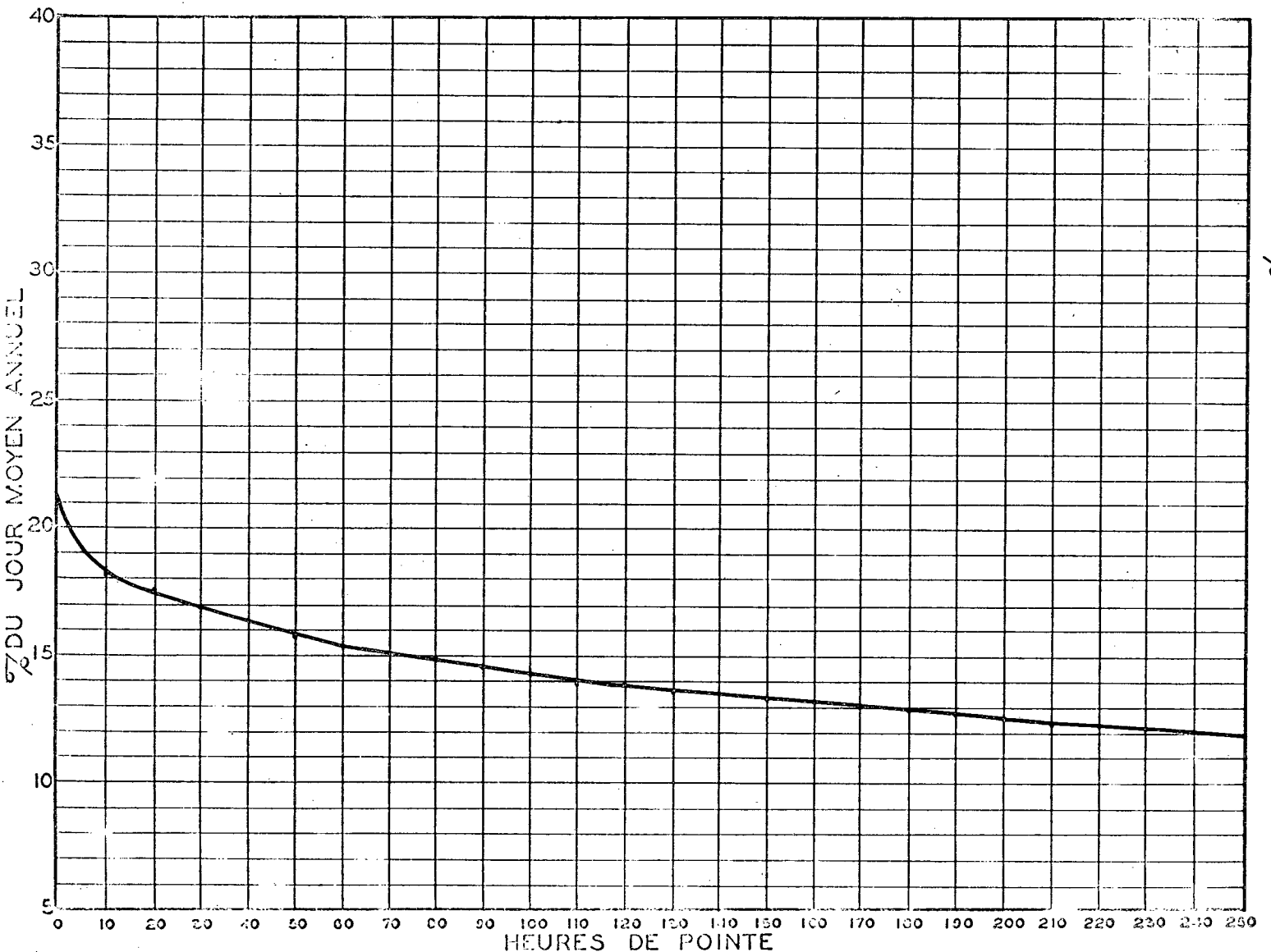
RELATION ENTRE LES HEURES DE POINTE ET LE JOUR MOYEN ANNUEL STATION: DUDSWELL ROUTE N° 1
