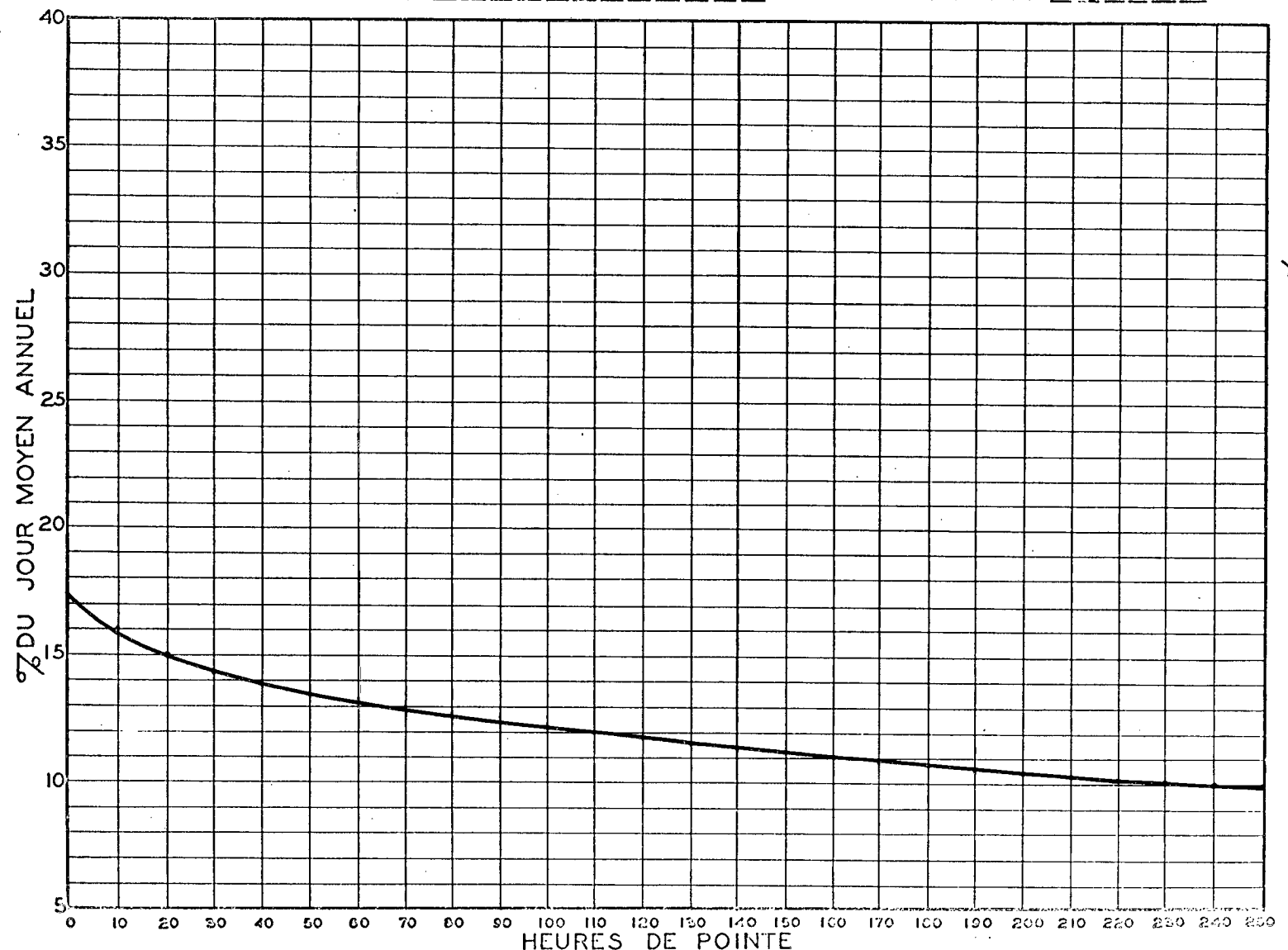
RELATION ENTRE LES HEURES DE POINTE ET LE JOUR MOYEN ANNUEL STATION: STE-CÉCILE ROUTE N° 3
