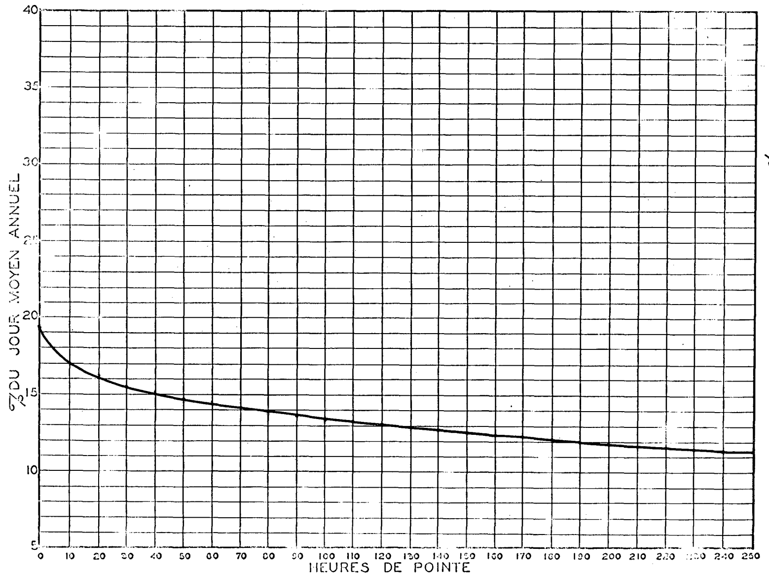
RELATION ENTRE LES HEURES DE POINTE ET LE JOUR MOYEN ANNUEL STATION: DESCHAMBAULT ROUTE N° 2
