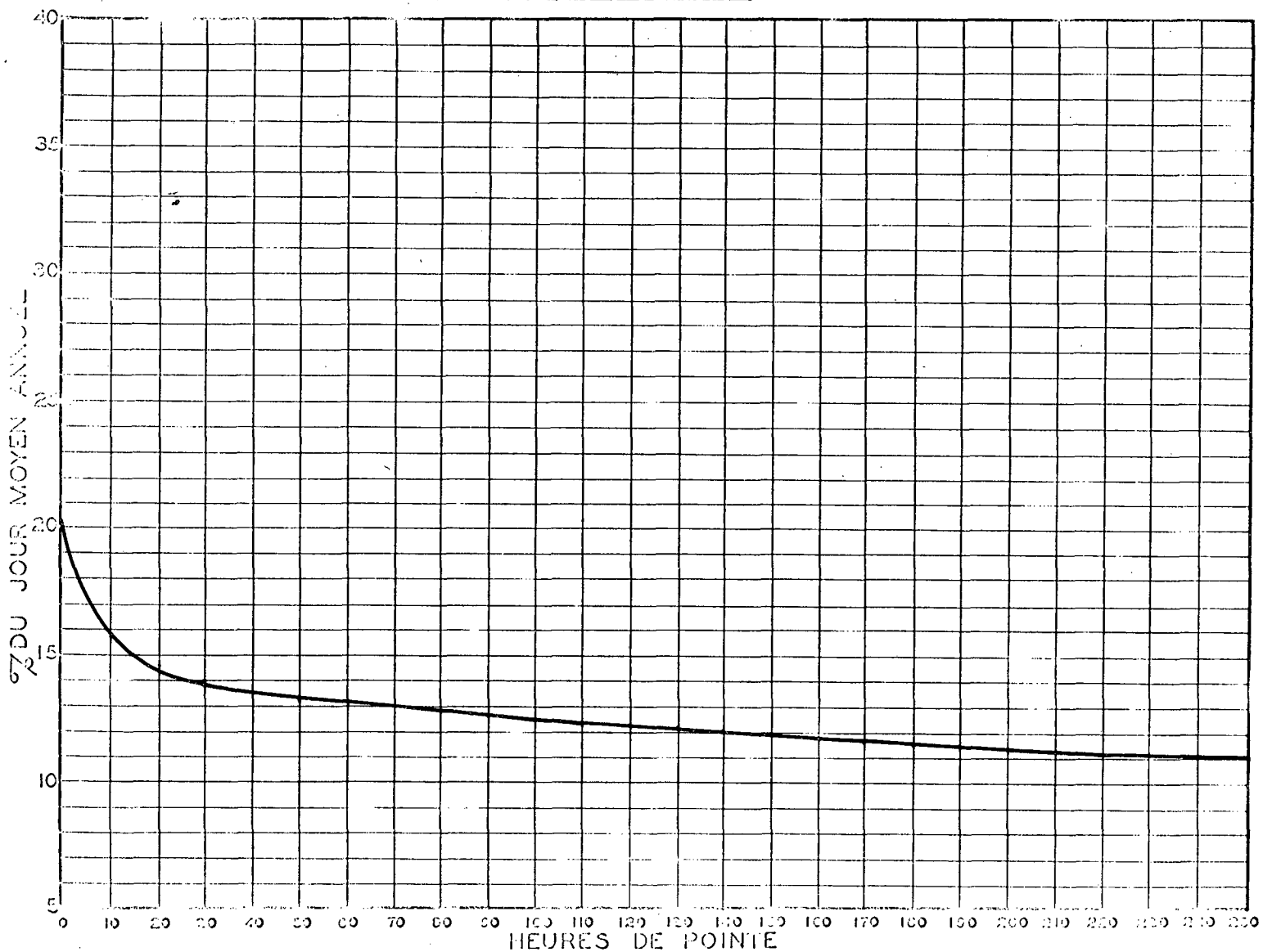
RELATION ENTRE LES HEURES DE POINTE ET LE JOUR MOYEN ANNUEL STATION: AMQUI ROUTE N°6
