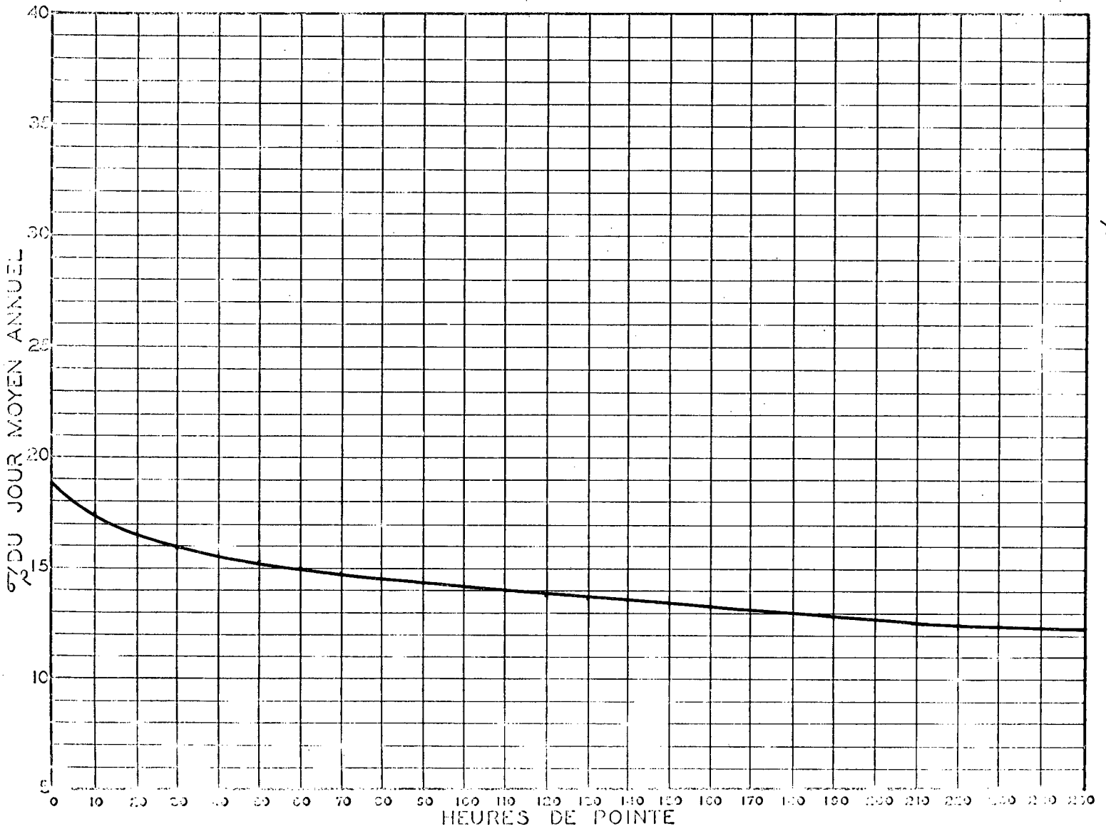
RELATION ENTRE LES HEURES DE POINTE ET LE JOUR MOYEN ANNUEL STATION: STANSTEAD EST ROUTE N° 5
