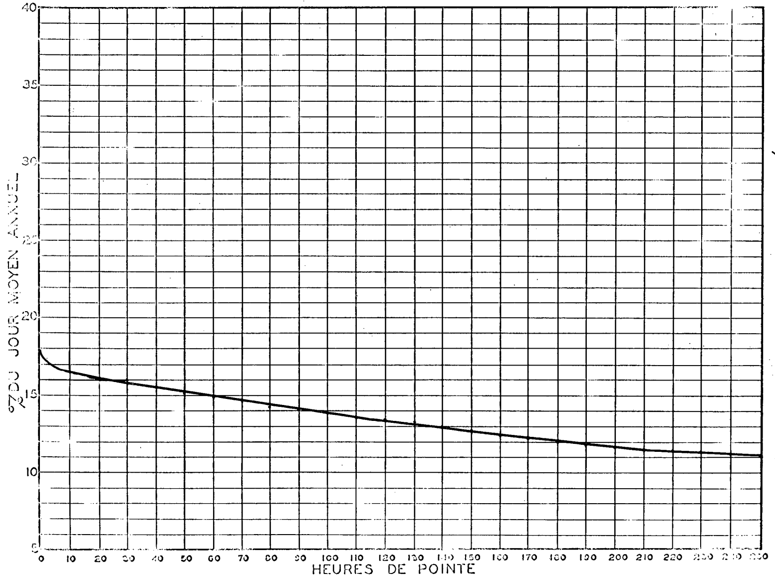
RELATION ENTRE LES HEURES DE POINTE ET LE JOUR MOYEN ANNUEL STATION: WATERLOO ROUTE N° 1
