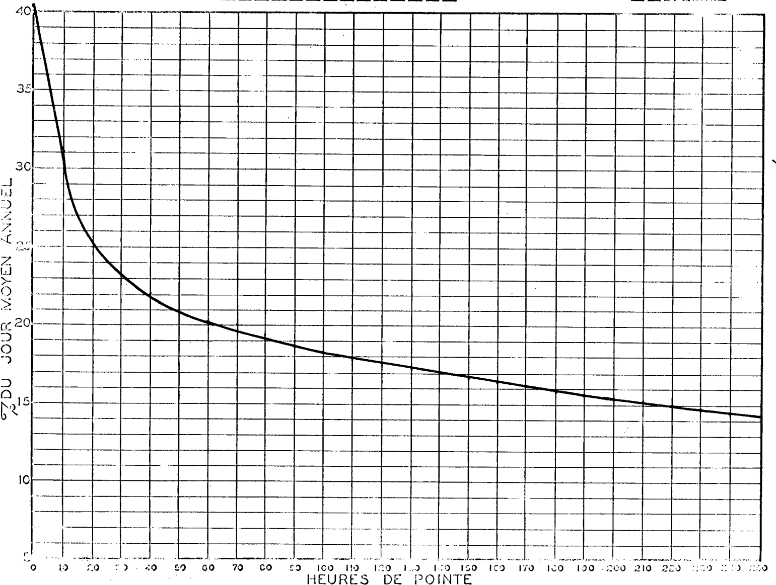
RELATION ENTRE LES HEURES DE POINTE ET LE JOUR MOYEN ANNUEL. STATION: AYLMEU ROUTE N° 8
