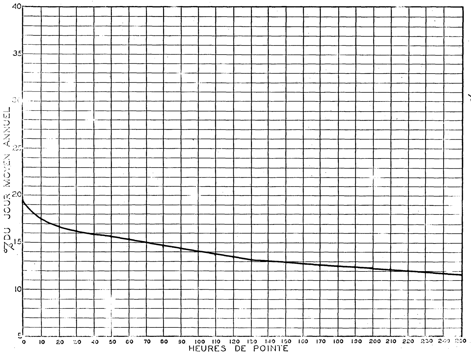
RELATION ENTRE LES HEURES DE POINTE ET LE JOUR MOYEN ANNUEL STATION: RIV. BEAUDETTE ROUTE N° 2
