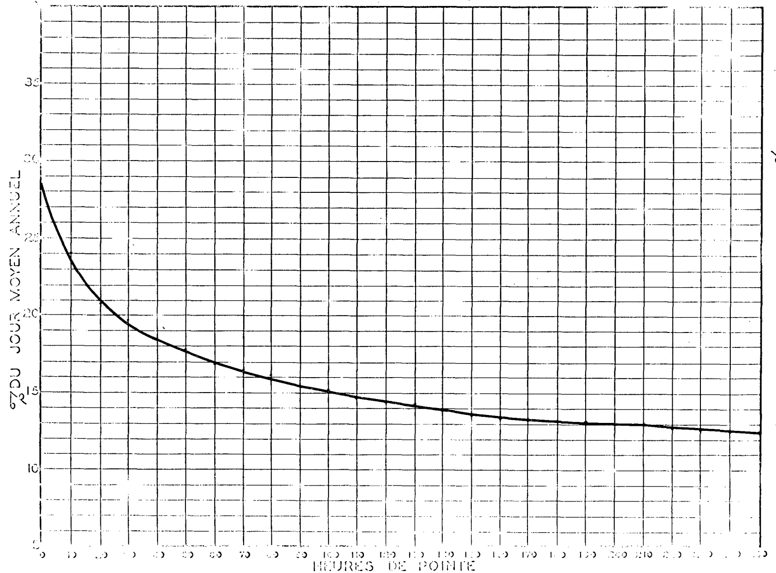
RELATION ENTRE LES HEURES DE POINTE ET LE JOUR MOYEN ANNUEL STATION: STE - LUCE ROUTE N°10
