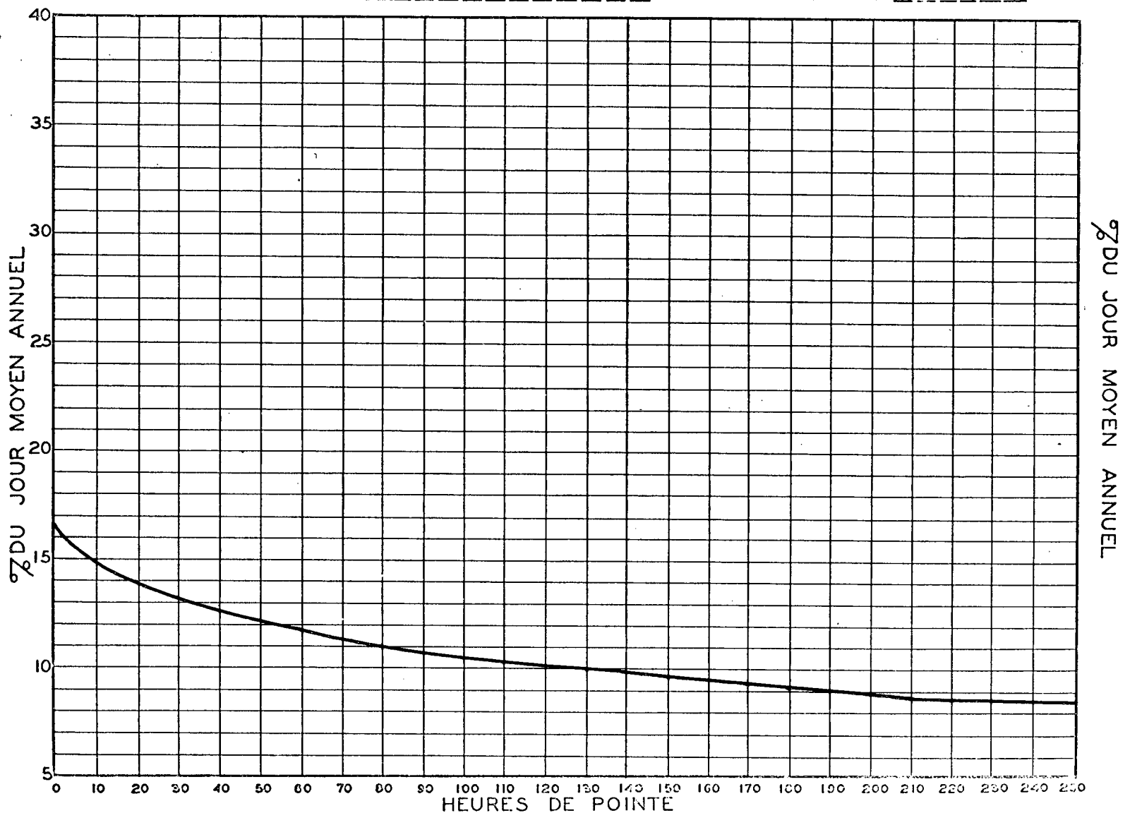
RELATION ENTRE LES HEURES DE POINTE ET LE JOUR MOYEN ANNUEL STATION: VALLEYFIELD ROUTE N° 3
