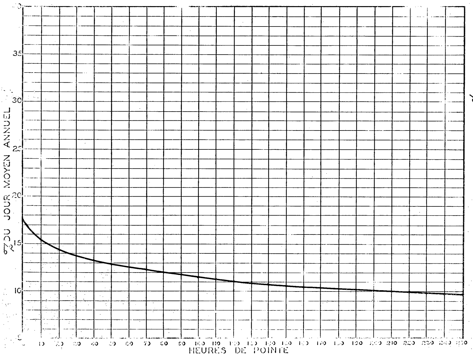
RELATION ENTRE LES HEURES DE POINTE ET LE JOUR MOYEN ANNUEL STATION: N.D-DE-LA-PROVIDENCE ROUTE N° 23
