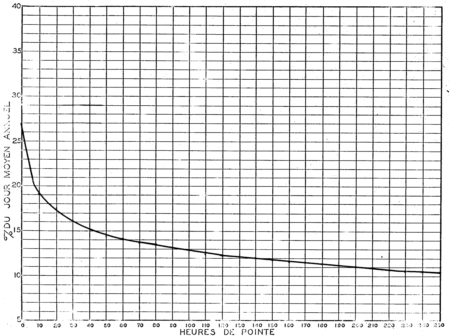
RELATION ENTRE LES HEURES DE POINTE ET LE JOUR MOYEN ANNUEL STATION: MAGOG VOIE SUD ROUTE N° 1
