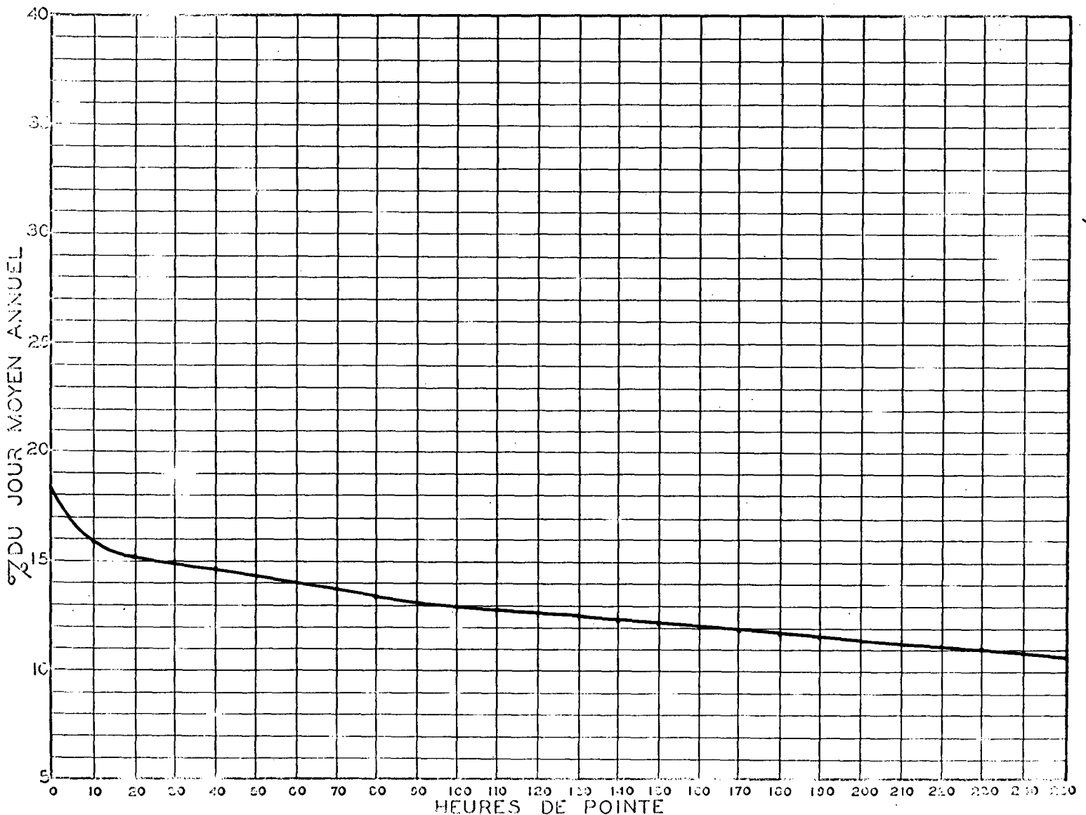
RELATION ENTRE LES HEURES DE POINTE ET LE JOUR MOYEN ANNUEL STATION: YAMASKA ROUTE N° 3
