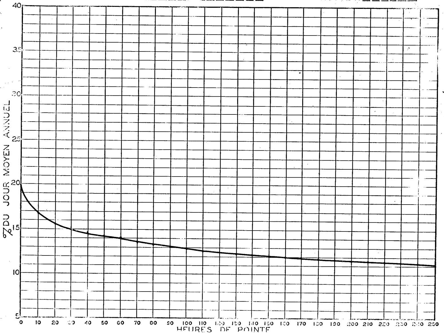
RELATION ENTRE LES HEURES DE POINTE ET LE JOUR MOYEN ANNUEL STATION: ST-ANTONIN ROUTE N° 2
