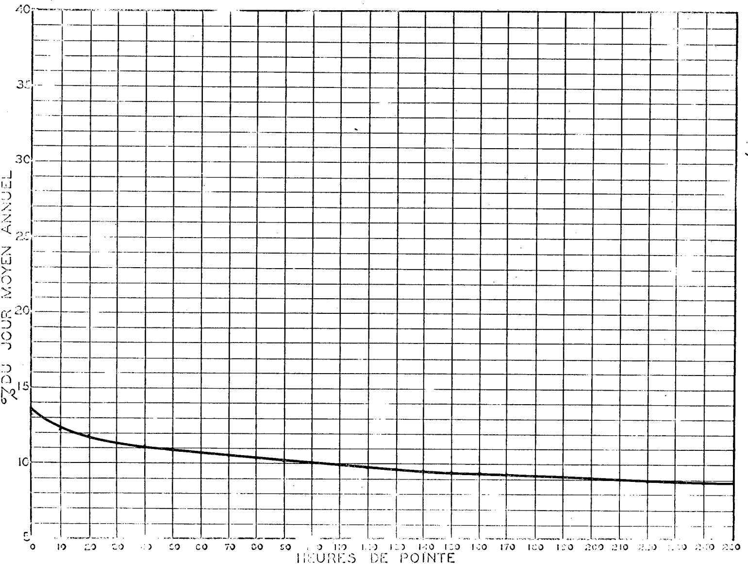
RELATION ENTRE LES HEURES DE POINTE ET LE JOUR MOYEN ANNUEL STATION: ST-HYACINTHE ROUTE N° 9
