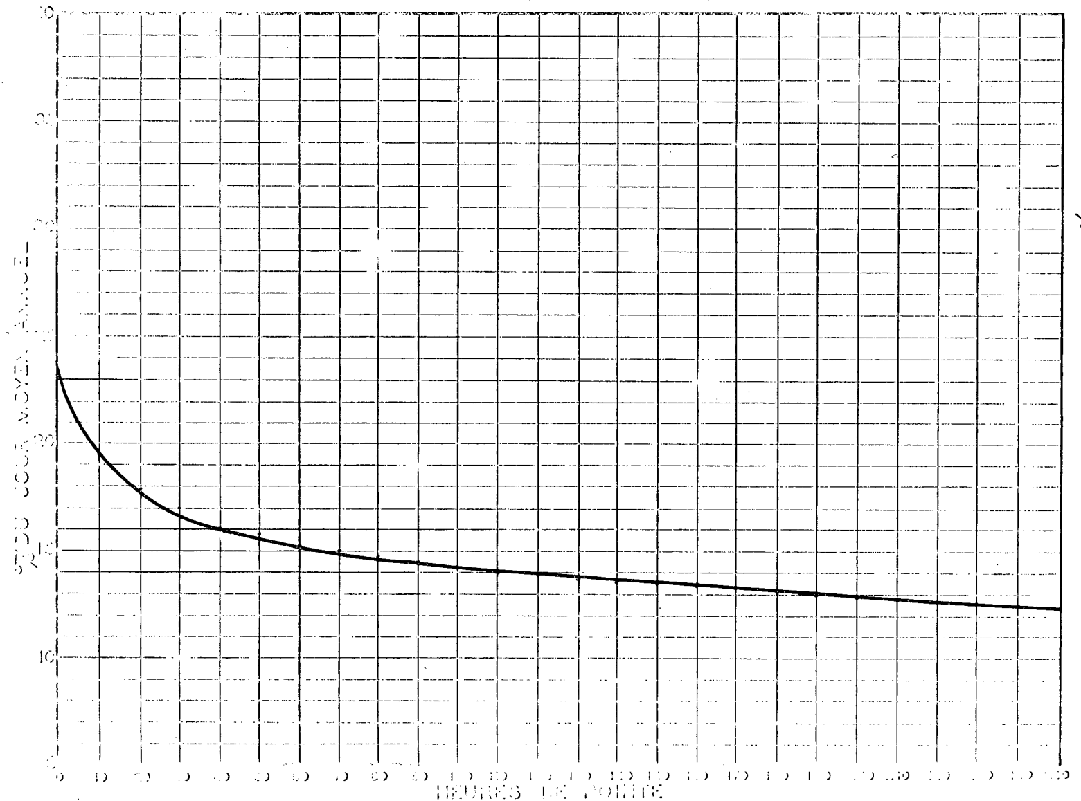
RELATION ENTRE LES HEURES DE POINTE ET LE JOUR MOYEN ANNUEL STATION: ST-PATRICE ROUTE N° 10
