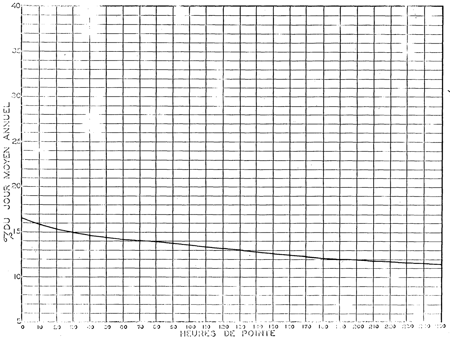
RELATION ENTRE LES HEURES DE POINTE ET LE JOUR MOYEN ANNUEL STATION: ST-SULPICE ROUTE N° 2
