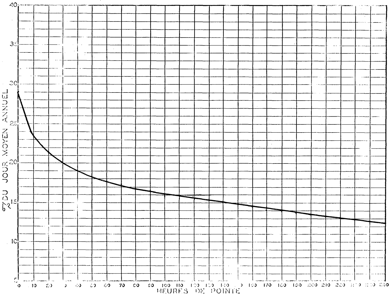
RELATION ENTRE LES HEURES DE POINTE ET LE JOUR MOYEN ANNUEL STATION: ST-HERMAS ROUTE N° 8
