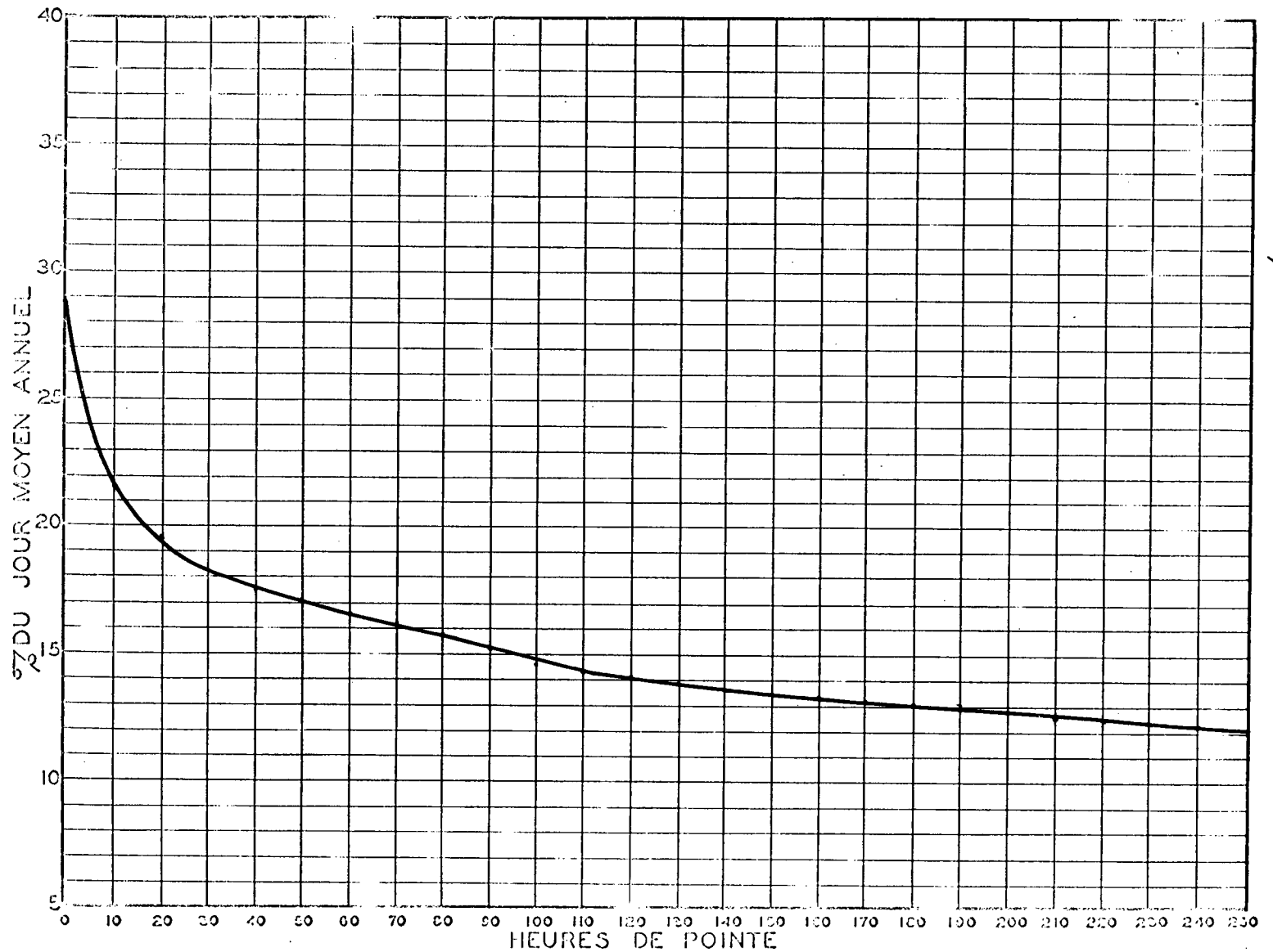
RELATION ENTRE LES HEURES DE POINTE ET LE JOUR MOYEN ANNUEL STATION: BATISCAN ROUTE N° 2
