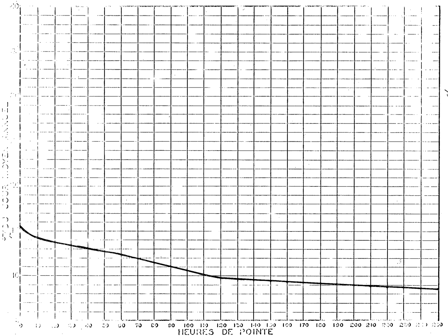
RELATION ENTRE LES HEURES DE POINTE ET LE JOUR MOYEN ANNUEL STATION: PONT SCOTT ROUTE 12
