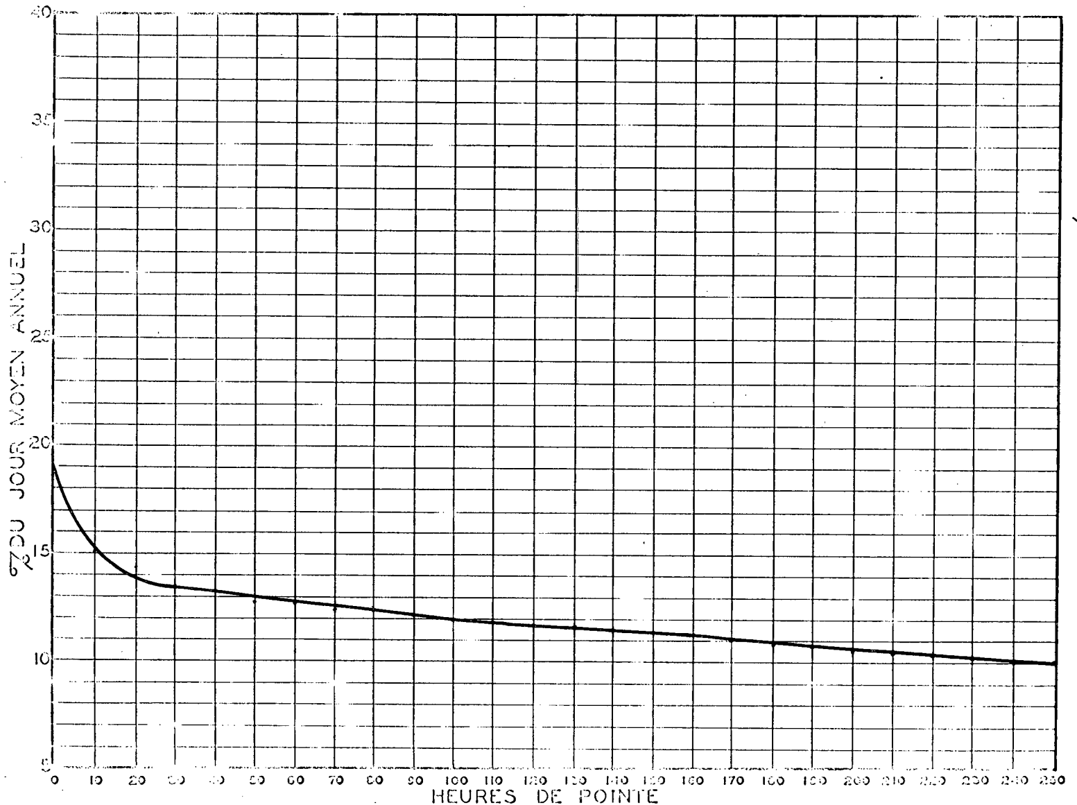
RELATION ENTRE LES HEURES DE POINTE ET LE JOUR MOYEN ANNUEL STATION: MASSON ROUTE N° 8
