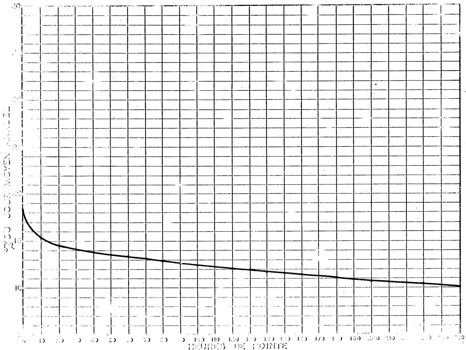
RELATION ENTRE LES HEURES DE POINTE ET LE JOUR MOYEN ANNUEL STATION: ST-ALBERT ROUTE N° 20
