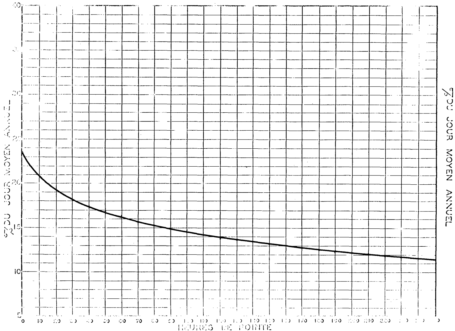
RELATION ENTRE LES HEURES DE POINTE ET LE JOUR MOYEN ANNUEL STATION: HULL ROUTE N° 11
