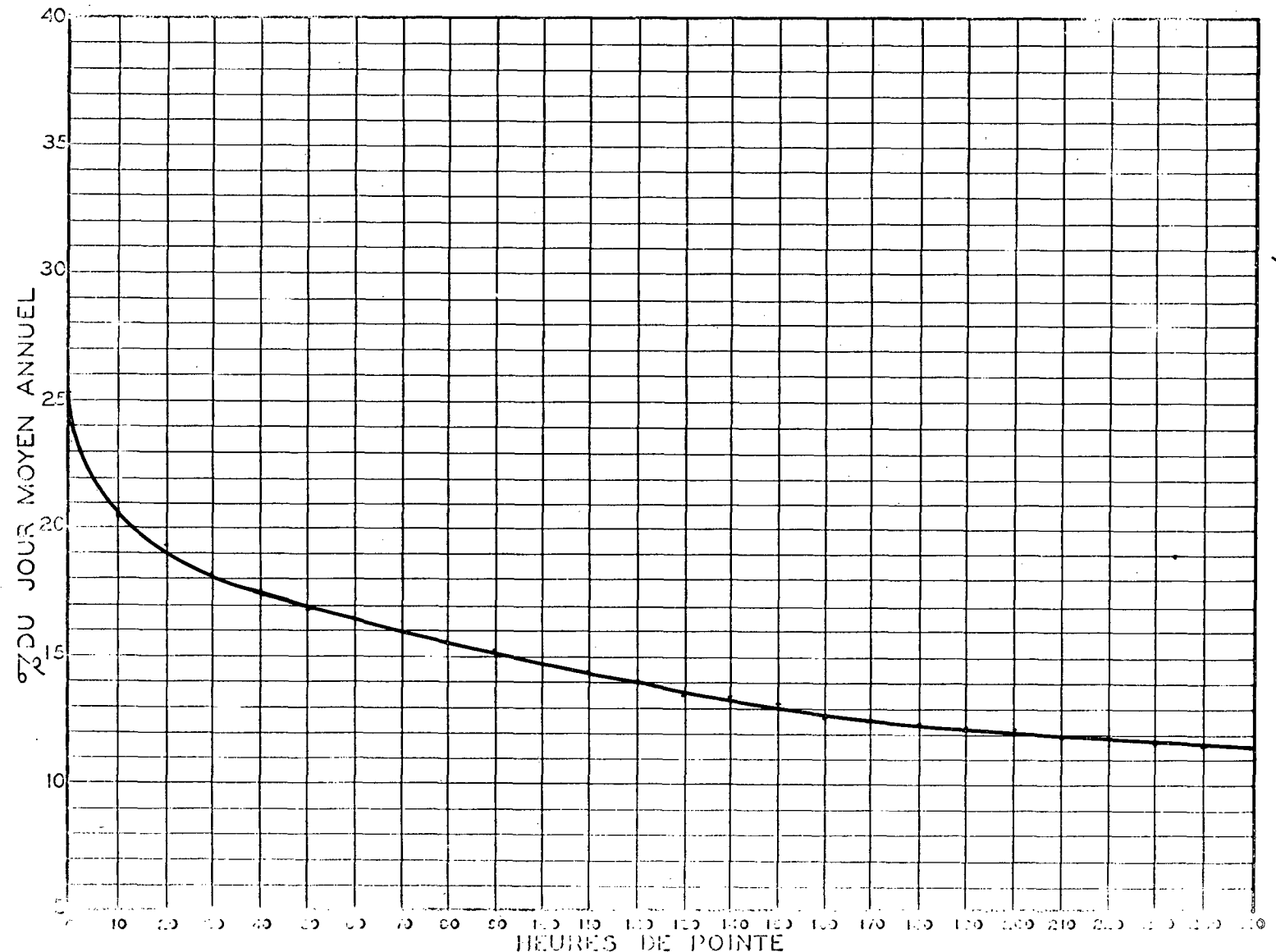
RELATION ENTRE LES HEURES DE POINTE ET LE JOUR MOYEN ANNUEL STATION: ST-ISIDORE ROUTE N° 23
