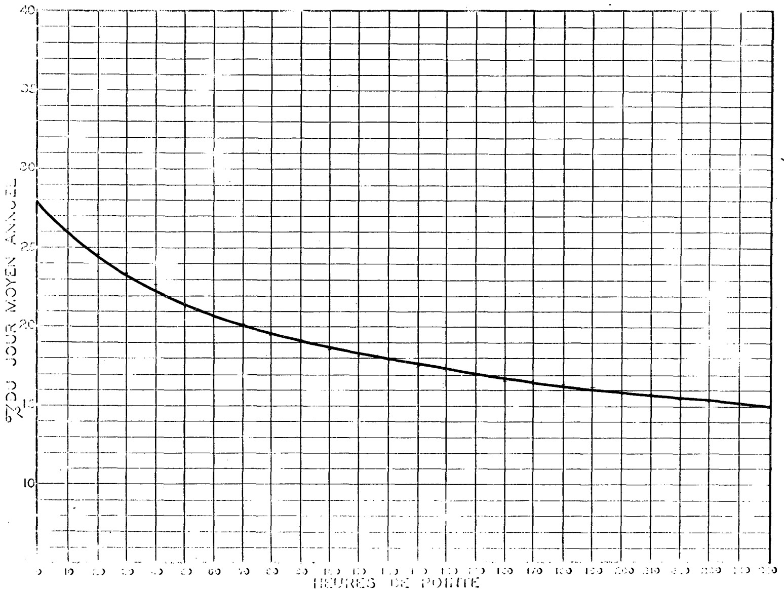
RELATION ENTRE LES HEURES DE POINTE ET LE JOUR MOYEN ANNUEL STATION: TERREBONNE ROUTE N°18
