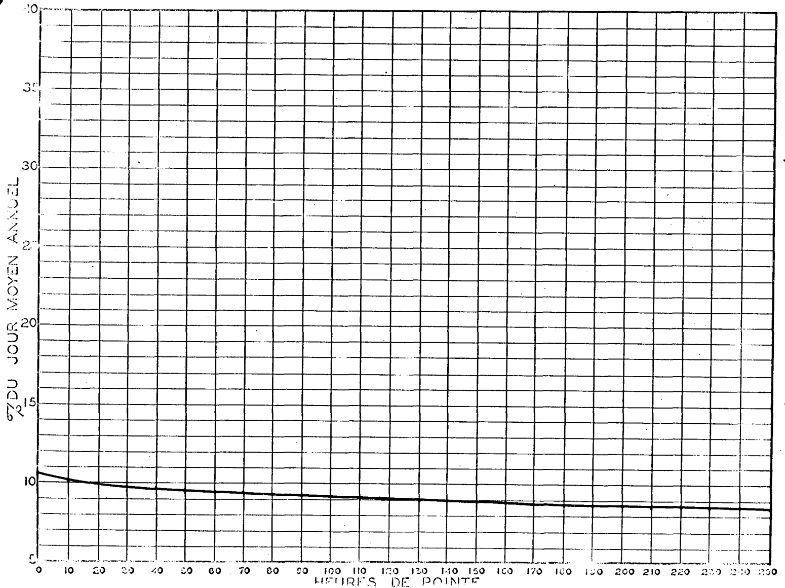
RELATION ENTRE LES HEURES DE POINTE ET LE JOUR MOYEN ANNUEL STATION: ST-ROMUALD ROUTE N° 2
