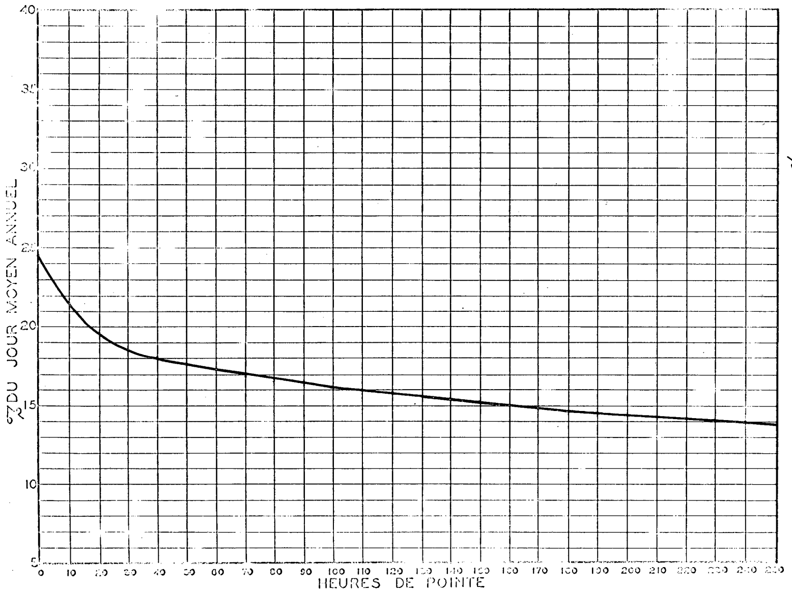
RELATION ENTRE LES HEURES DE POINTE ET LE JOUR MOYEN ANNUEL STATION: STE-FÉLICITÉ ROUTE N° 6
