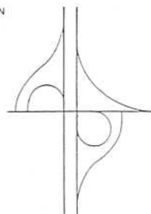
PARCLO A-3
