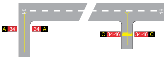
Figure 5.14 – Exemples de panneaux d'identification de piste
