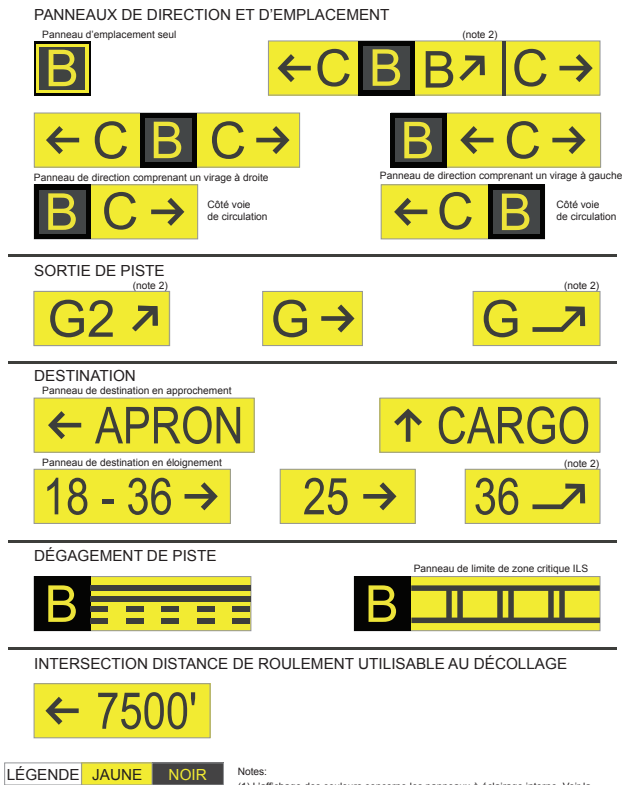
Figure 5.13 – Panneaux d'indication
