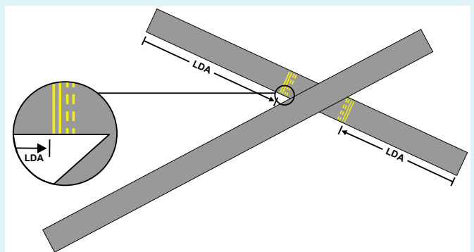
Figure 4.7 — Distance utilisable à l'atterrissage et lignes d'attente pour le LAHSO
