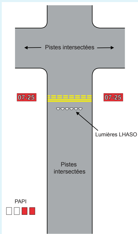
Figure 4.8 — Configuration des aides visuelles pour le LAHSO
