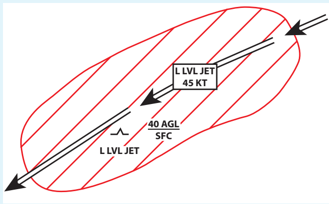
Figure 4.5i) – LLJ et turbulence
