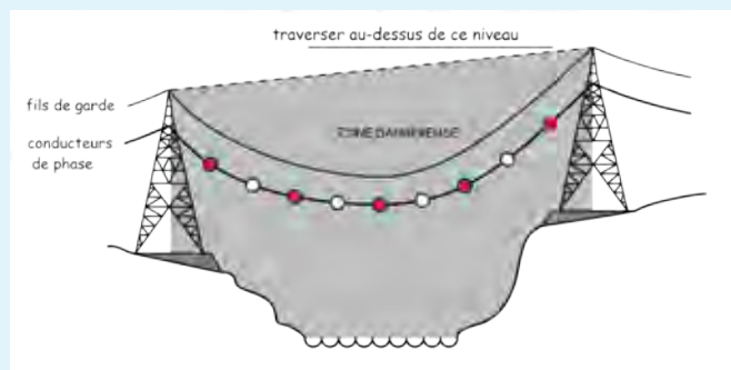
Figure 2.4 — Survoler les caténares
