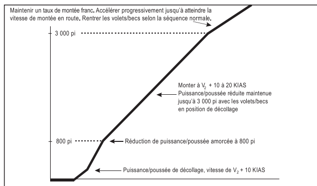
Figure 7.1 – Critère pour procédure d'atténuation du bruit (NADP 1)
