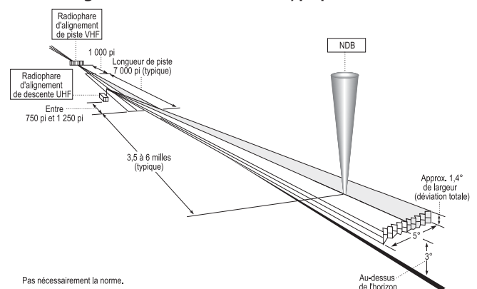
Figure 4.2 – Installation typique d'un ILS
