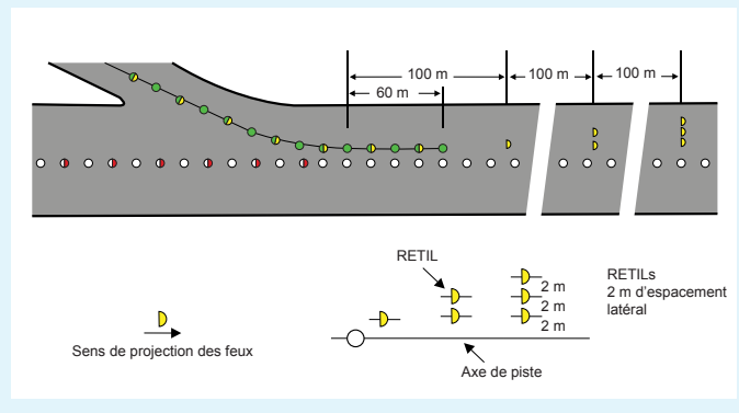
Figure 7.14 – Feux de voie de sortie rapide
