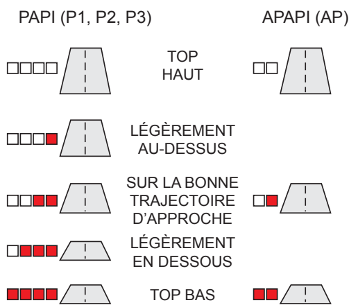
Figure 7.7 – Indications de PAPI et d'APAPI
