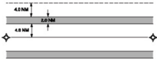
Figure 2.7b) – Coupe transversale d'une route RNAV fixe
