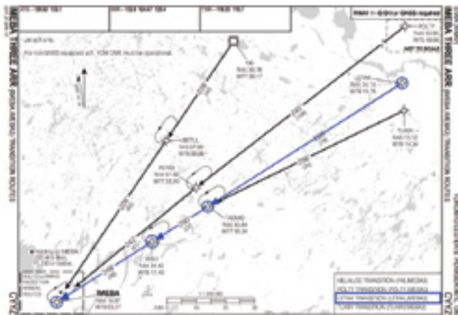
Figure 9.2 Exemple d'une transition en route sur la procédure d'arrivée IMEBA THREE ARR de CYYZ
