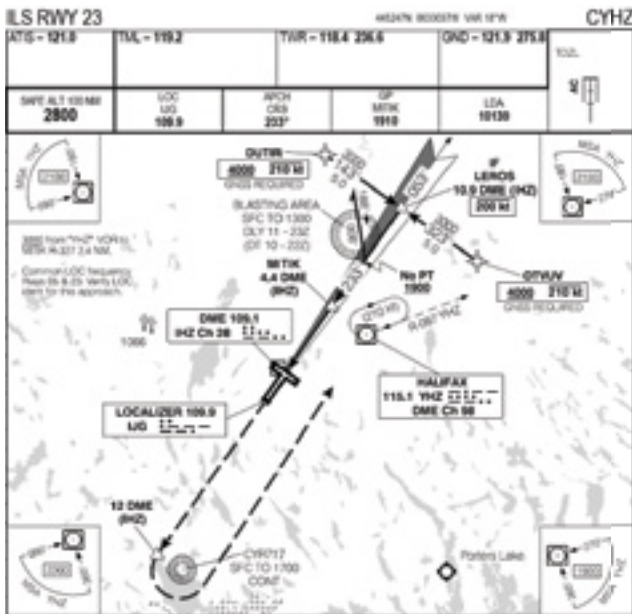
Figure 9.5 – Transitions d'un IAWP à gauche et à droite vers un IWP à CYHZ, RNAV (GNSS) Z piste 23
