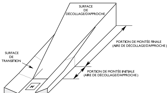
Figure 4.2 – Surfaces et aires de décollage/d'approche d'un hélicoptère
