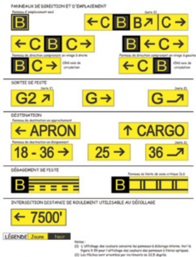
Figure 5.13 – Panneaux d'indication
