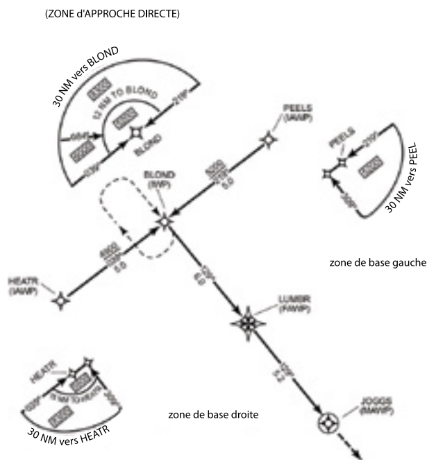
Figure 9.1 – Approche standard en "T" avec illustration de la TAA
