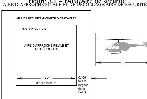
Figure 3.1 – FATO/Aire de sécurité
