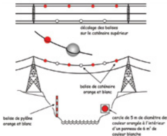
Figure 6.4 – Balises de câbles aériens
