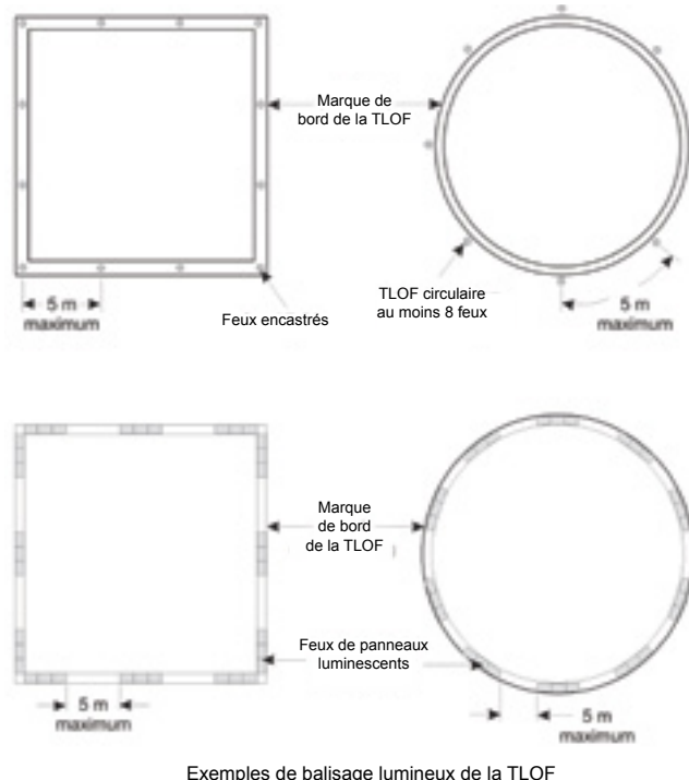
Figure 7.15 – Exemples de balisage lumineux de la TLOF
