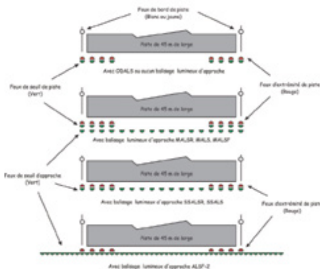
Figure 7.11 – Feux de seuil et d'extrémité de piste
