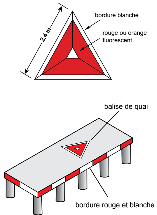
Figure 5.3 – Balises d'identification de quai pour hydravions
