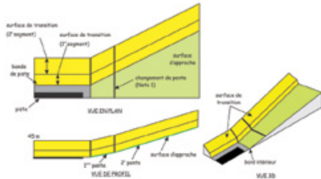
Figure 4.1 – Exemple de surfaces de limitation d'obstacle
