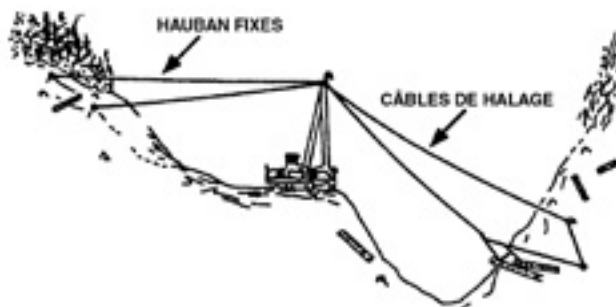
Figure 2.4 – Pylône articulé
