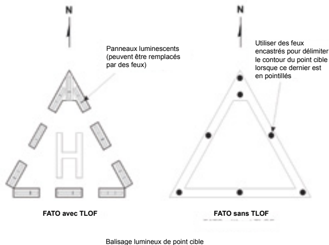
Balisage lumineux de point cible
