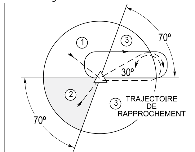
Figure 10.2 – Secteurs d'entrée
