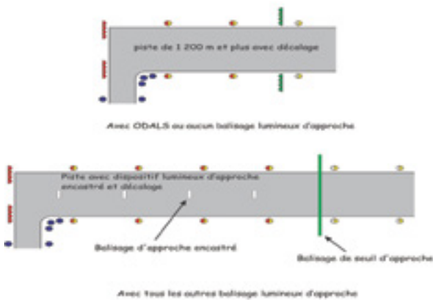
Figure 7.12 – Balisage lumineux du seuil de piste décalé
