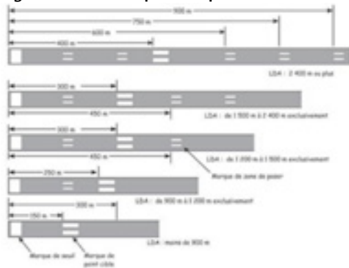
Figure 5.4 – Marques de point cible et TDZ
