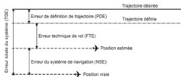
Figure 6.1 – Erreurs de navigation latérale
