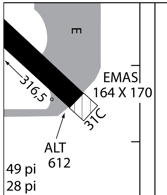
Représentation d'un EMAS sur une carte d'aérodrome
