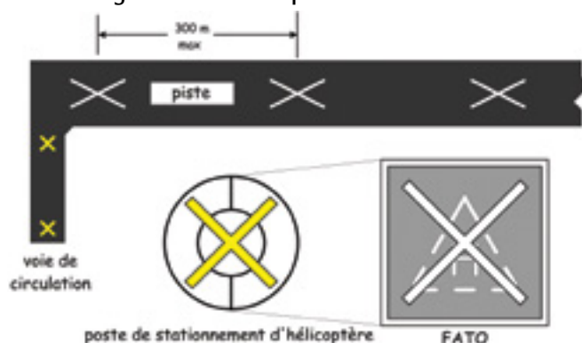
Figure 5.11 – Marques de zone fermée
