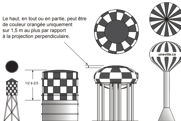
Figure 6.1 – Marques utilisées pour les réservoirs
