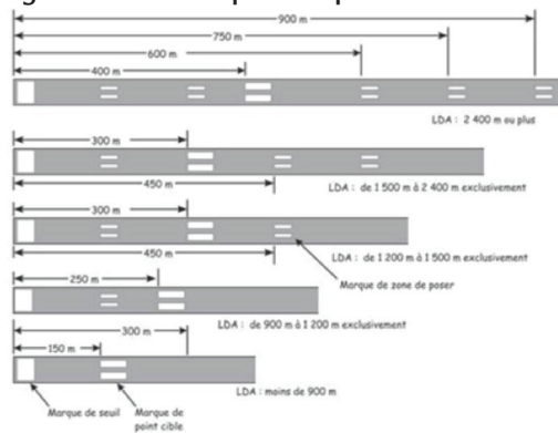
Figure 5.4 – Marques de point cible et TDZ
