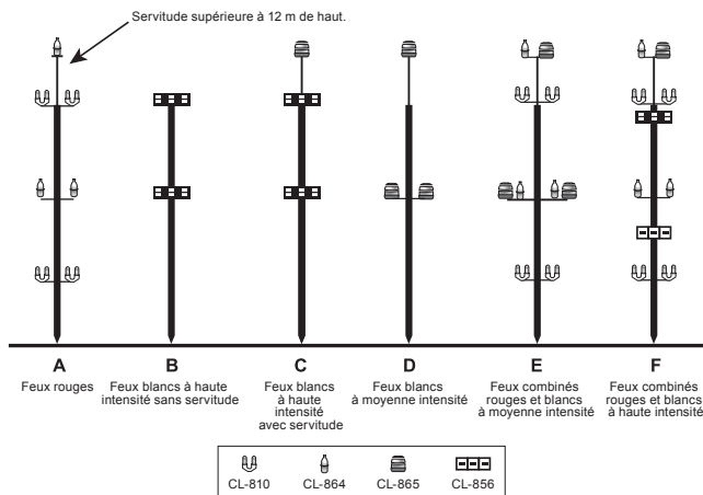
Figure 6.3 – Éclairage des tours et antennes
