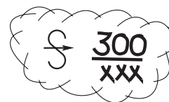
Figure 12.2g) – Tempêtes de sable ou de poussière sur une grande étendue
