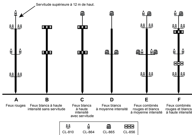
Figure 6.3 – Éclairage de charpentes
