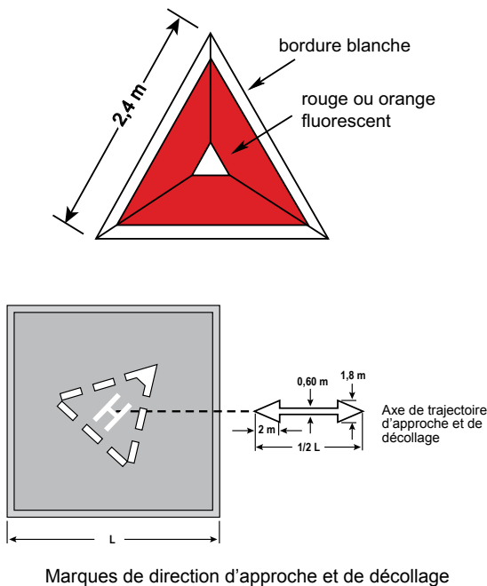
Marques de direction d'approche et de décollage
