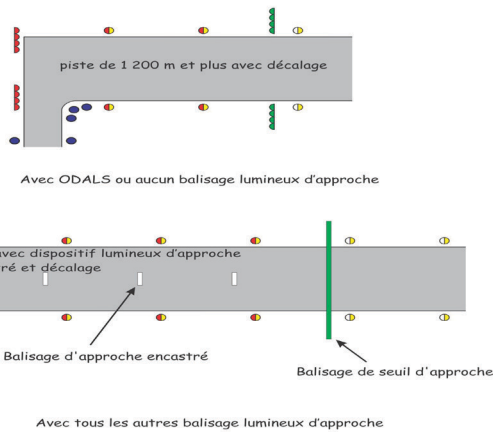
Figure 7.12 – Décalage du balisage lumineux du seuil de piste
