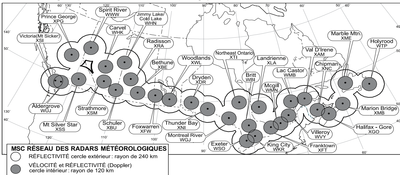
Figure 1.1 – Réseau des radars météorologiques d'Environnement Canada et du MDN
