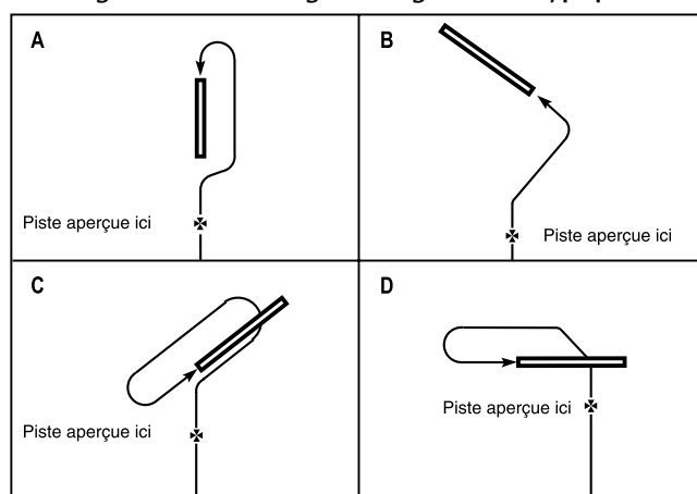
Figure 9.10 – Virages d'alignement typiques
