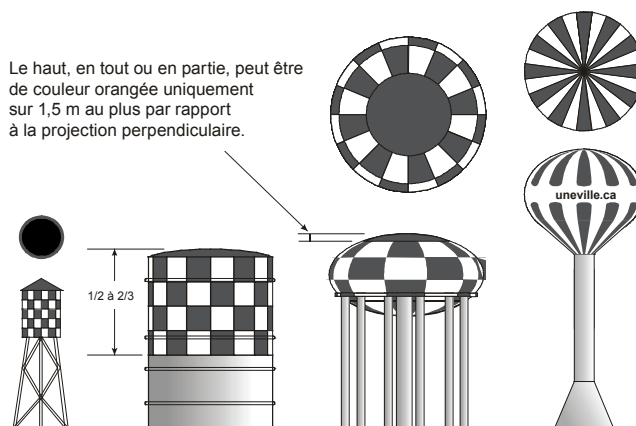
Figure 6.1 – Marques utilisées pour les réservoirs
