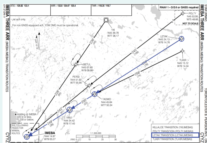
Figure 9.2 Exemple d'une transition en route sur la procédure d'arrivée IMEBA THREE ARR de CYYZ
