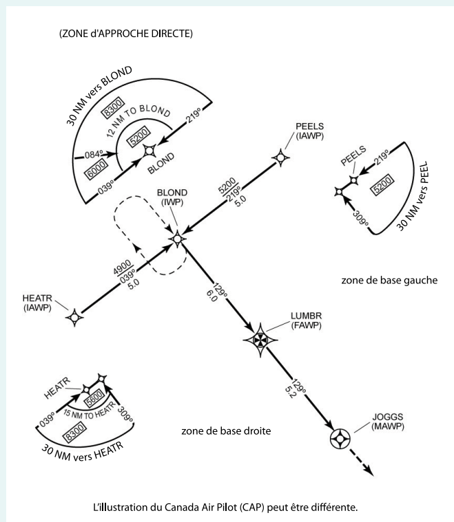
Figure 9.1 – Approche standard en "T" avec illustration de la TAA
