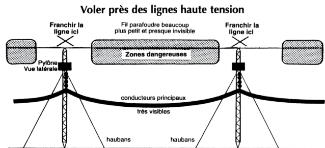
Figure 2.3 – Voler près des lignes haute tension
