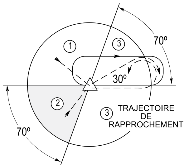
Figure 10.2 – Secteurs d'entrée
