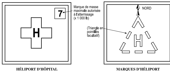
Figure 5.9 – Marques d'hélicoptères
