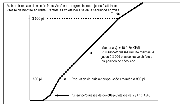
Figure 7.1 – Critère pour procédure d'atténuation du bruit (NADP 1)
