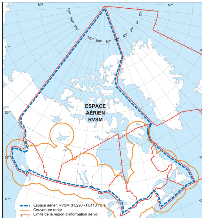
Figure 11.1 – Espace aérien RVSM et espace aérien de transition RVSM
