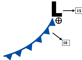
Figure 4.4b) – Éléments synoptiques
