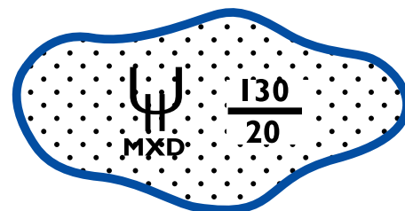
Figure 4.5b) – Givrage
