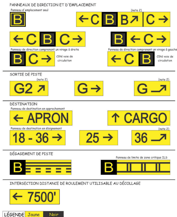
Figure 5.14 – Panneaux d'indication
