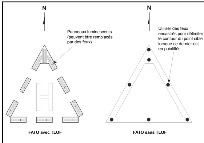
Figure 7.16 – Balisage lumineux de la FATO et du point cible
