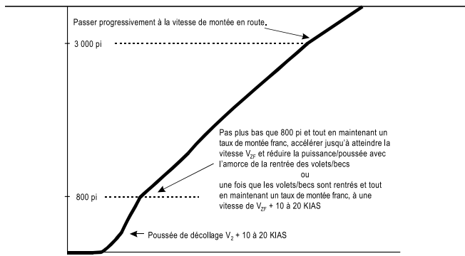
Figure 7.2 – Critère pour procédure d'atténuation du bruit (NADP 2)
