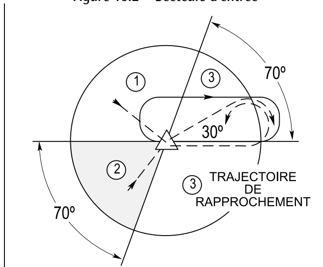
Figure 10.2 – Secteurs d'entrée
