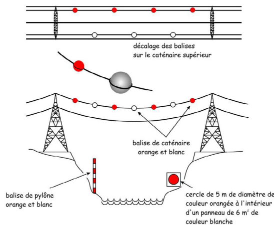
Figure 6.4 - Balise de câbles aériens
