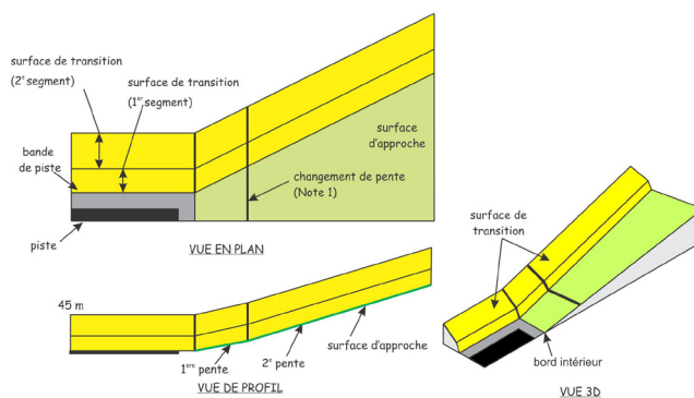
Figure 4.1 – Exemple de surfaces de limitation d'obstacle
