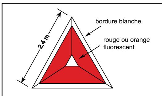
Figure 5.3 - Marques d'identification de quai pour hydravions
