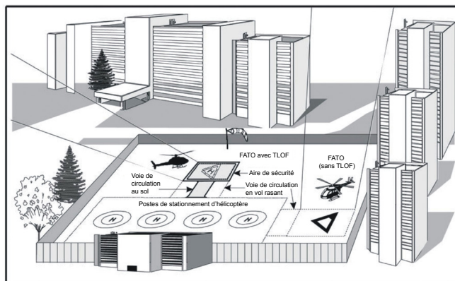
Figure 3.2 – Disposition générale d'un hélicopt
