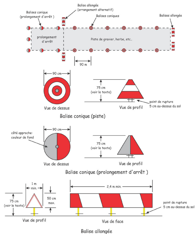
Figure 5.1 – Exemples de balises coniques et de balise allongée
