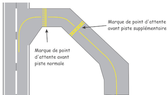
Figure 5.7 – Marques de point d'attente avant piste
