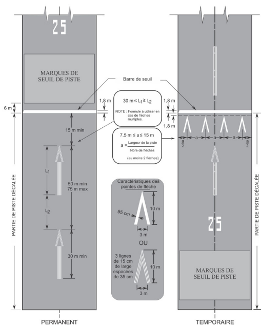
Figure 5.5 – Marques de seuil décalé
