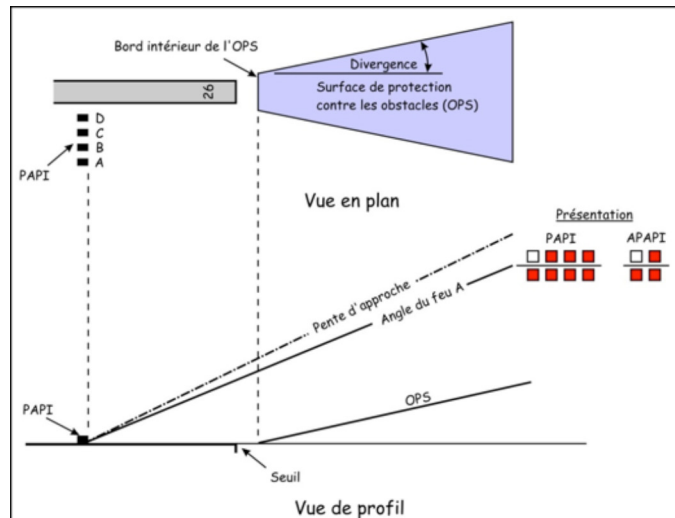
Figure 7.9 – OPS de PAPI/d'APAPI
