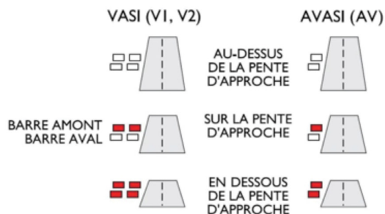
Figure 7.6 – Indications de VASI et d'AVASI
