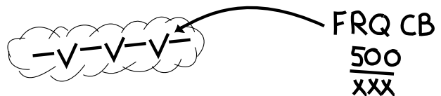
Figure 12.2f) – Lignes de grains forts
