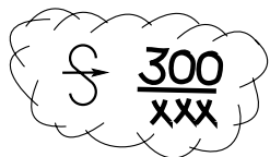
Figure 12.2g) – Tempêtes de sable ou de poussière sur une grande étendue
