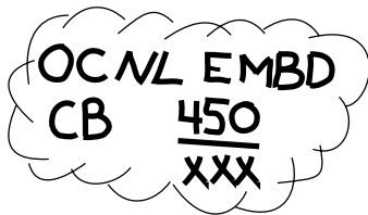
Figure 12.2b) – Hauteur des nuages
