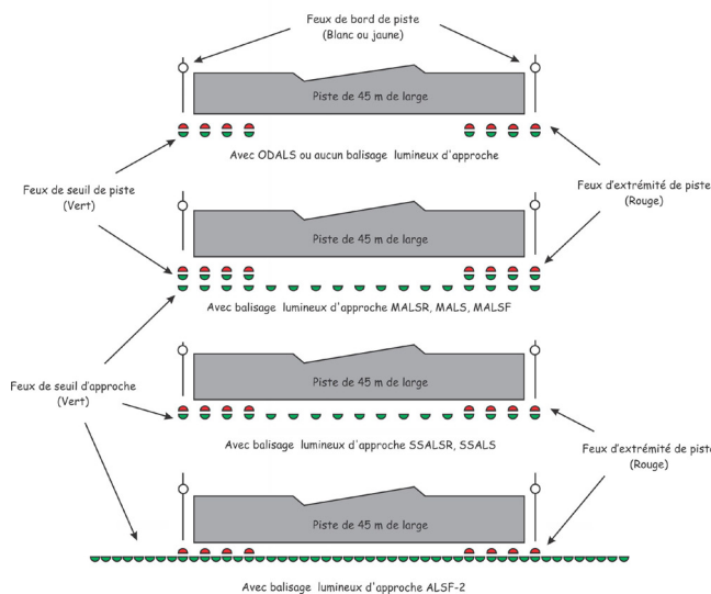
Figure 7.11 – Feux de seuil d'extrémité de piste
