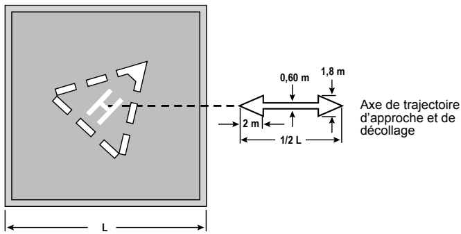
Figure 5.11 – Marques de direction d'approche et de décollage
