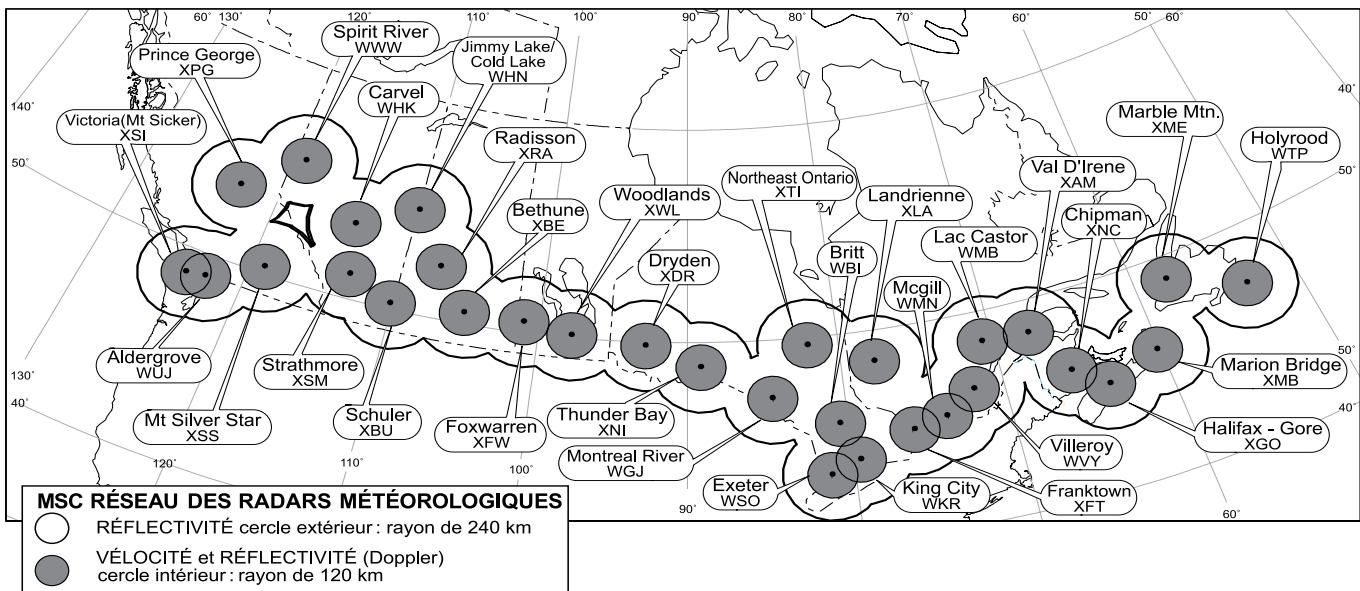
Figure 1.3 – Réseau des radars météorologiques d'Environnement Canada et du MDN
