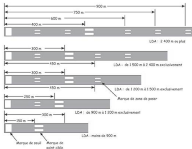
Figure 5.4 - Marques de point cible et TDZ
