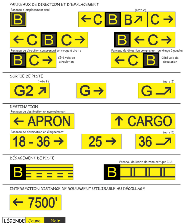
Figure 5.14 – Panneaux d'indication
