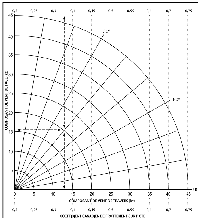
Figure 1.1 – Limites de vent de travers en fonction du CRFI
