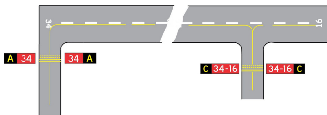
Figure 5.15 – Exemples de panneaux d'identification de piste
