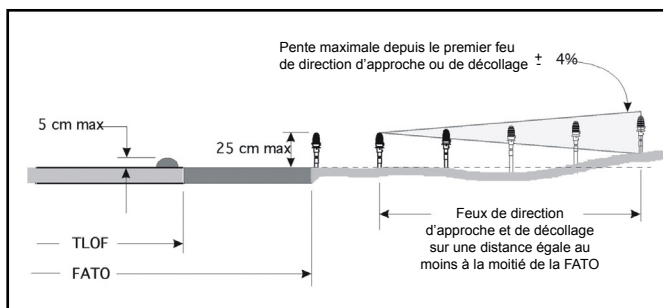
Figure 7.17 – Hauteur maximale de montage des feux de la TLOF, de la FATO et de direction d'approche ou de décollage
