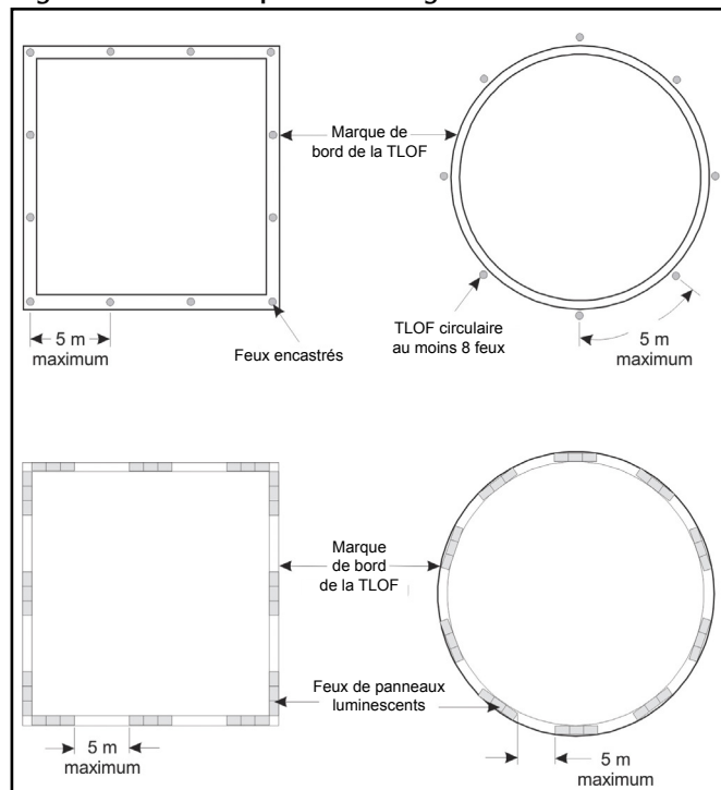
Figure 7.15 – Exemple de balisage lumineux de la TLOF
