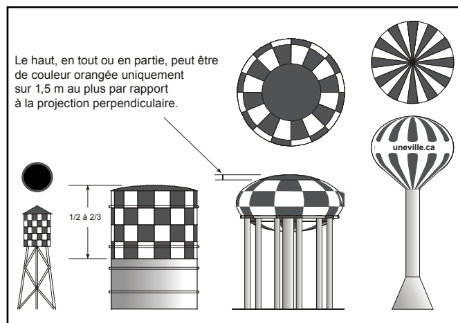
Figure 6.1 – Marques utilisées pour les réservoirs
