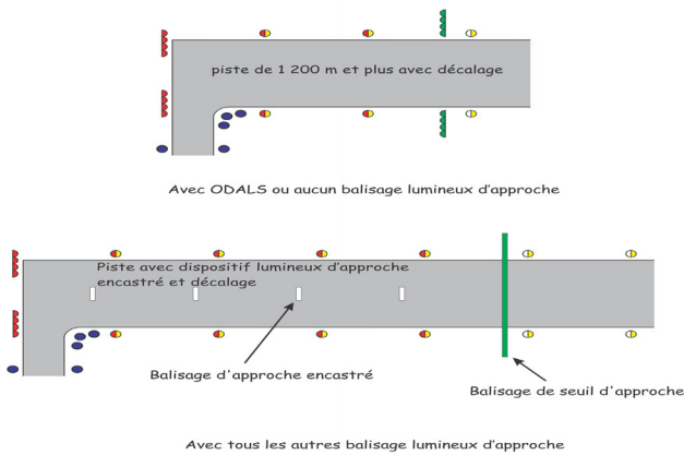
Figure 7.12 – Décalage du balisage lumineux du seuil de piste
