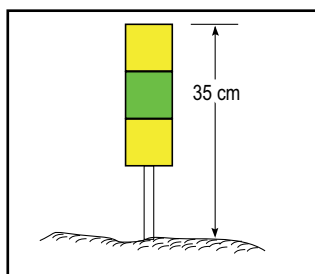
Figure 5.2 - Balise de bord de voie de circulation en vol rasant
