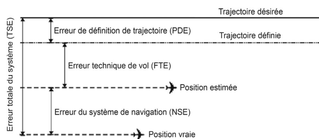
Figure 6.1 – Erreurs de navigation latérale
