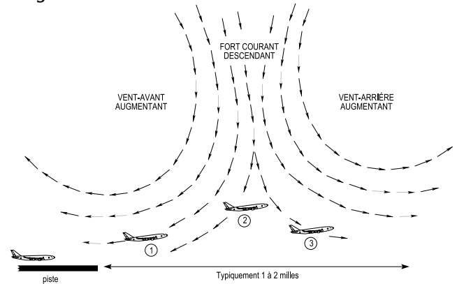
Figure 2.6 – Cisaillement du vent à basse altitude
