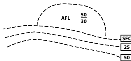
Figure 4.5g) – Niveau de congélation
