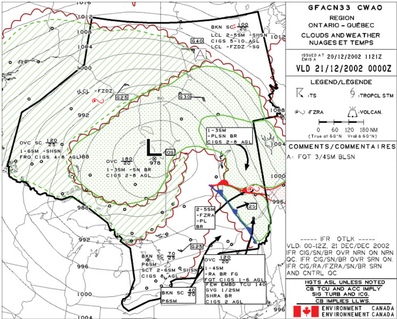
Figure 4.4a) – Exemple de carte des nuages et du temps de la GFA
