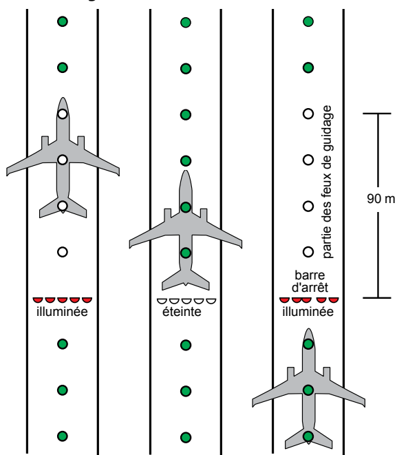
Figure 7.14 – Feux de barre d'arrêt
