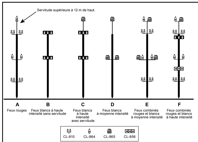
Figure 6.3 - Éclairage de charpentes
