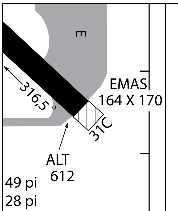
Figure 9.2 – Représentation d'un EMAS sur une carte d'aérodrome
