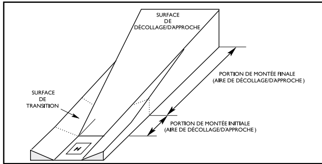
Figure 4.2 – Surfaces et aires de décollage/d’approche d’un hélicoptère
