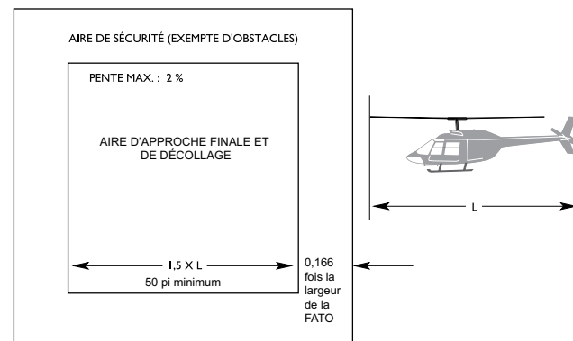
Figure 3.1 – Aire d'approche finale et de décollage/Aire de sécurité
