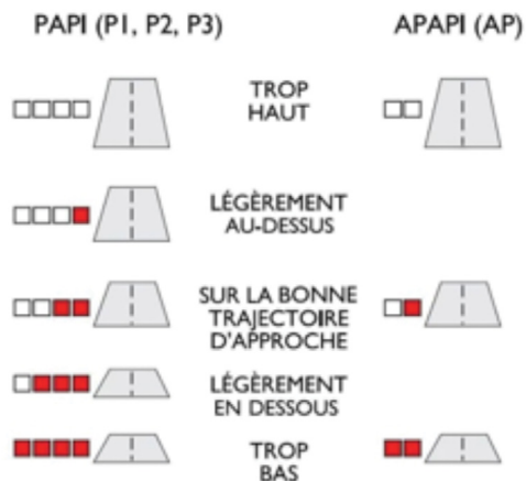
Figure 7.7 – Indications de PAPI et d'APAPI
