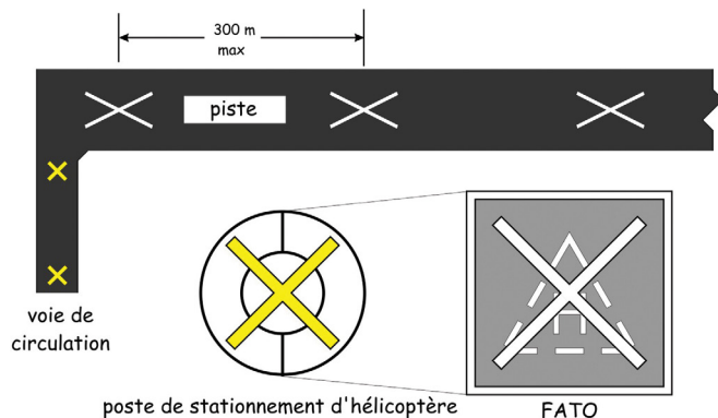
Figure 5.12 – Marques de zone fermée
