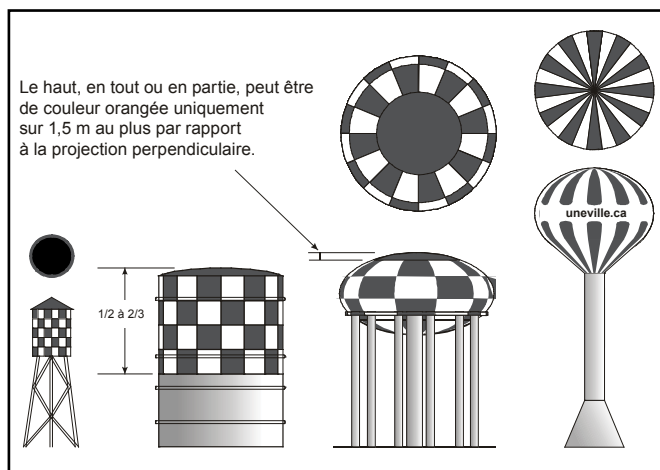
Figure 6.1 – Marques utilisées pour les réservoirs
