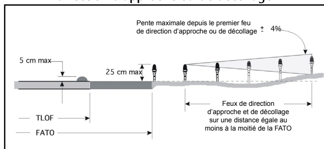
Figure 7.17 – Hauteur maximale de montage des feux de la TLOF, de la FATO et de direction d'approche ou de décollage
