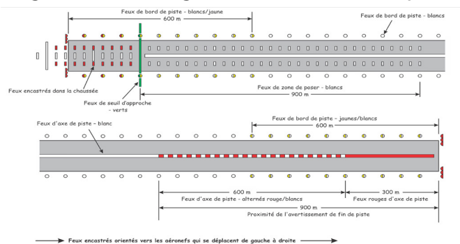
Figure 7.13 – Balisage lumineux de la zone de poser
