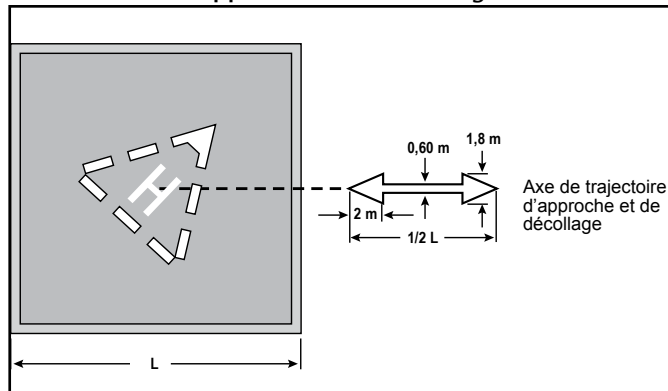
Figure 5.11 – Marques de direction d'approche et de décollage
