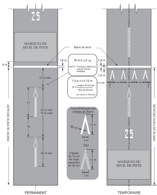
Figure 5.5 – Marques de seuil décalé
