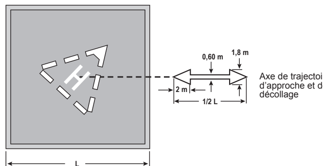
Marques de direction d'approche et de décollage
