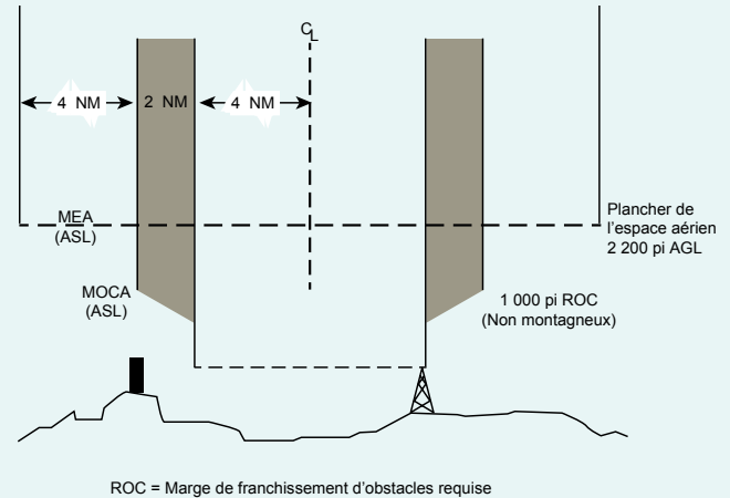
Figure 2.7b) – Coupe transversale d'une route RNAV fixe
