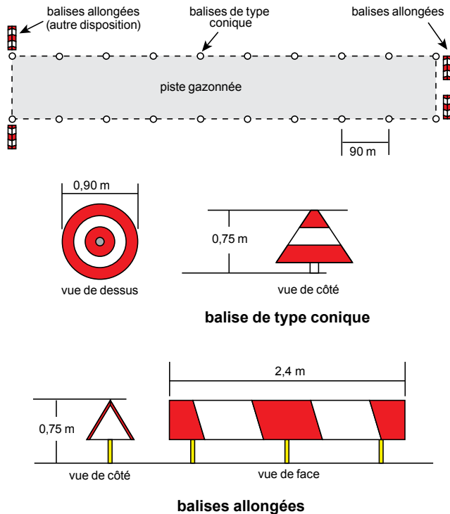
Exemples de balises de type conique et de balises allongées
