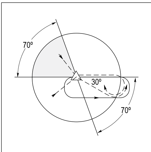
Figure 10.3 – Entrée dans un circuit non classique
