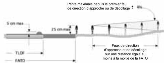
Hauteur maximale de montage des feux de la TLOF, de la FATO et de direction d'approche ou de décollage
