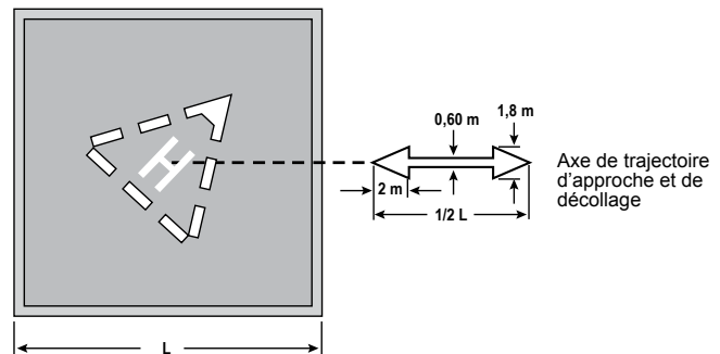
Marques de direction d'approche et de décollage
