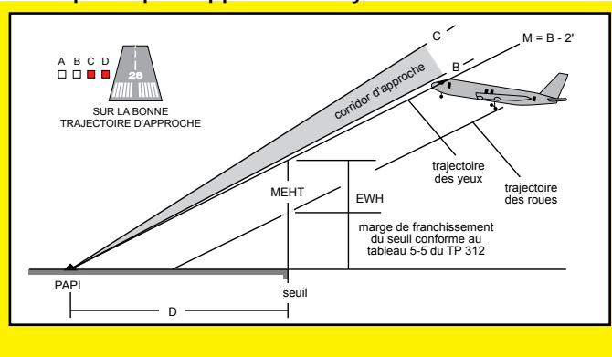
Figure 7-1 PAPI - Trajectoire des yeux du pilote par rapport à la trajectoire des roues
