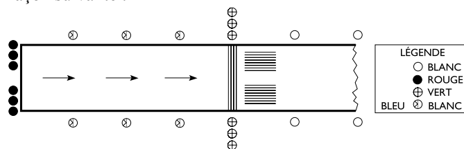
BALISAGE LUMINEUX DU SEUIL DÉCALÉ DE PISTE
