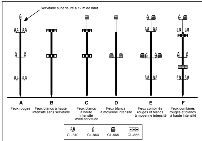
Figure 6.4.2 : Éclairage de charpentés
