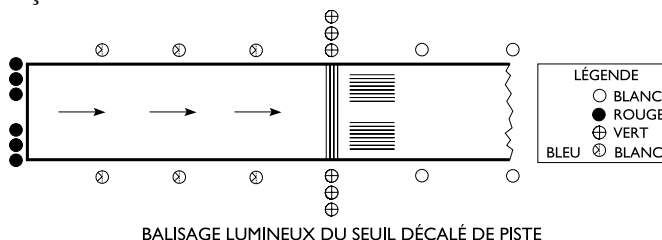
BALISAGE LUMINEUX DU SEUIL DÉCALÉ DE PISTE
