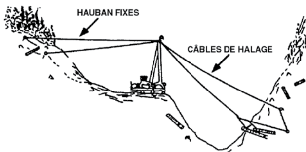
Figure 2.1 - Pylône articulé
