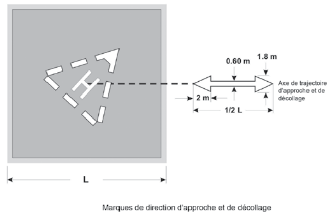
Marques de direction d'approche et de décollage
