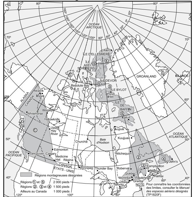
Figure 2.10 – Régions désignées montagneuses du Canada
