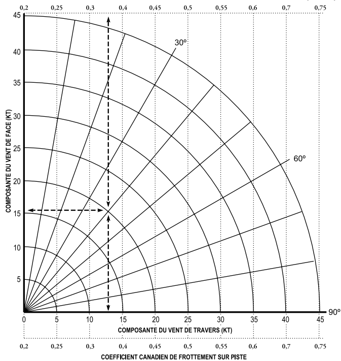
TABEAU 3 LIMITES DE VENT DE TRAVERS EN FONCTION DU COEFFICIENT CANADIEN DE FROTTEMENT SUR PISTE (CRFI)
