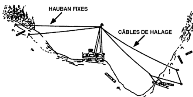
Figure 2.1 - Pylône articulé
