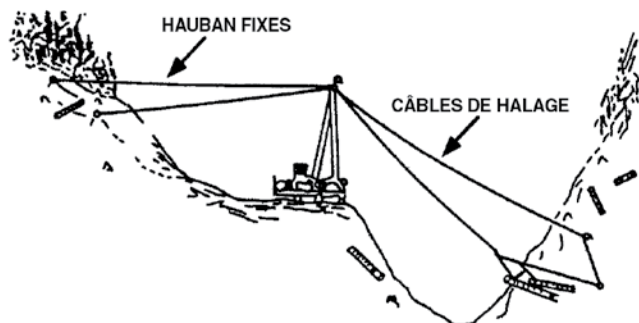
Figure 2.1 - Pylône articulé
