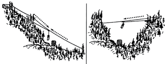
Figure 2.2 - Pont roulant sur câble aérien
