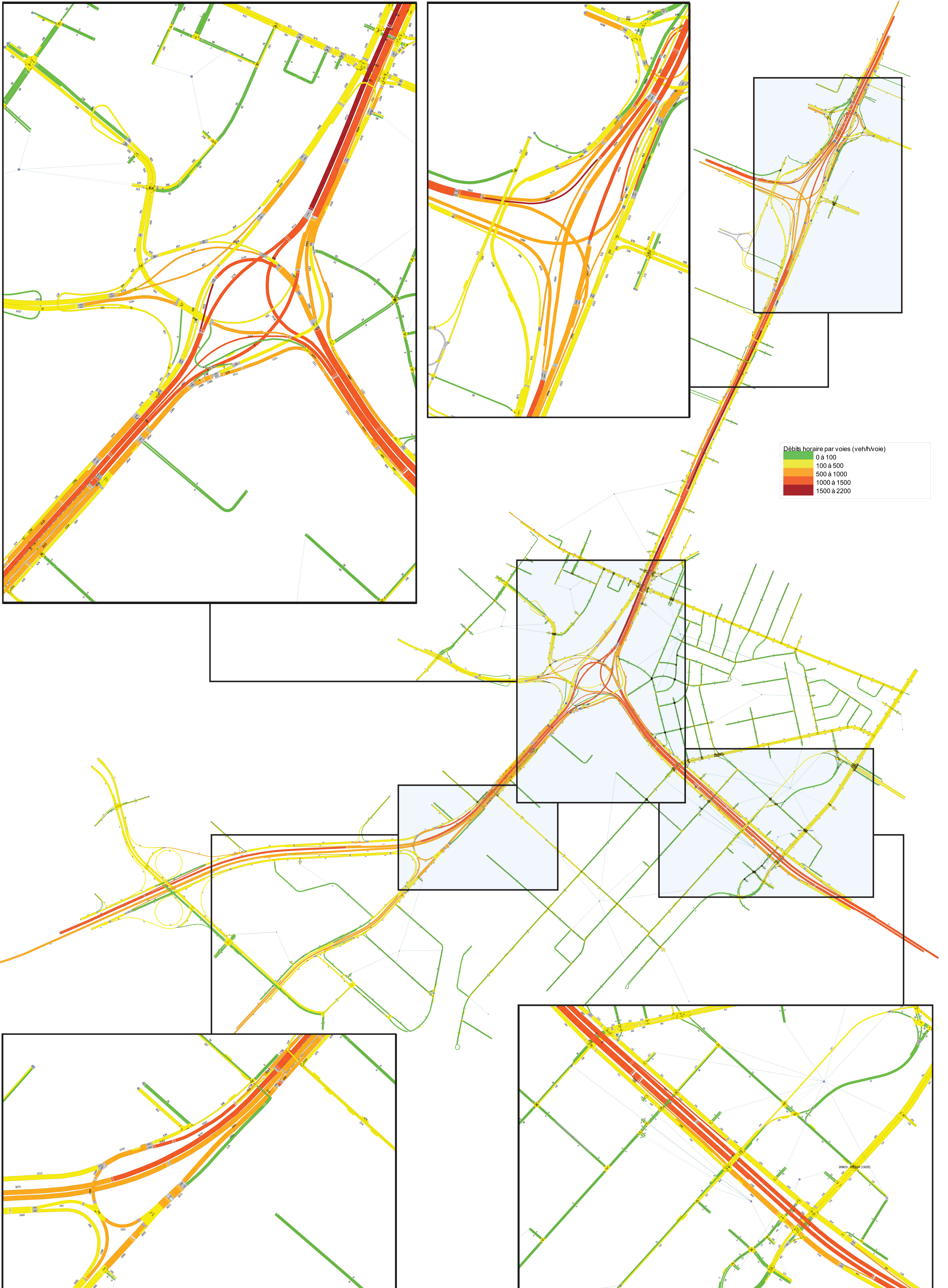
Figure C-2.1 DEBITS DE CIRCULATION ACTUELS – HEURE DE POINTE PM
