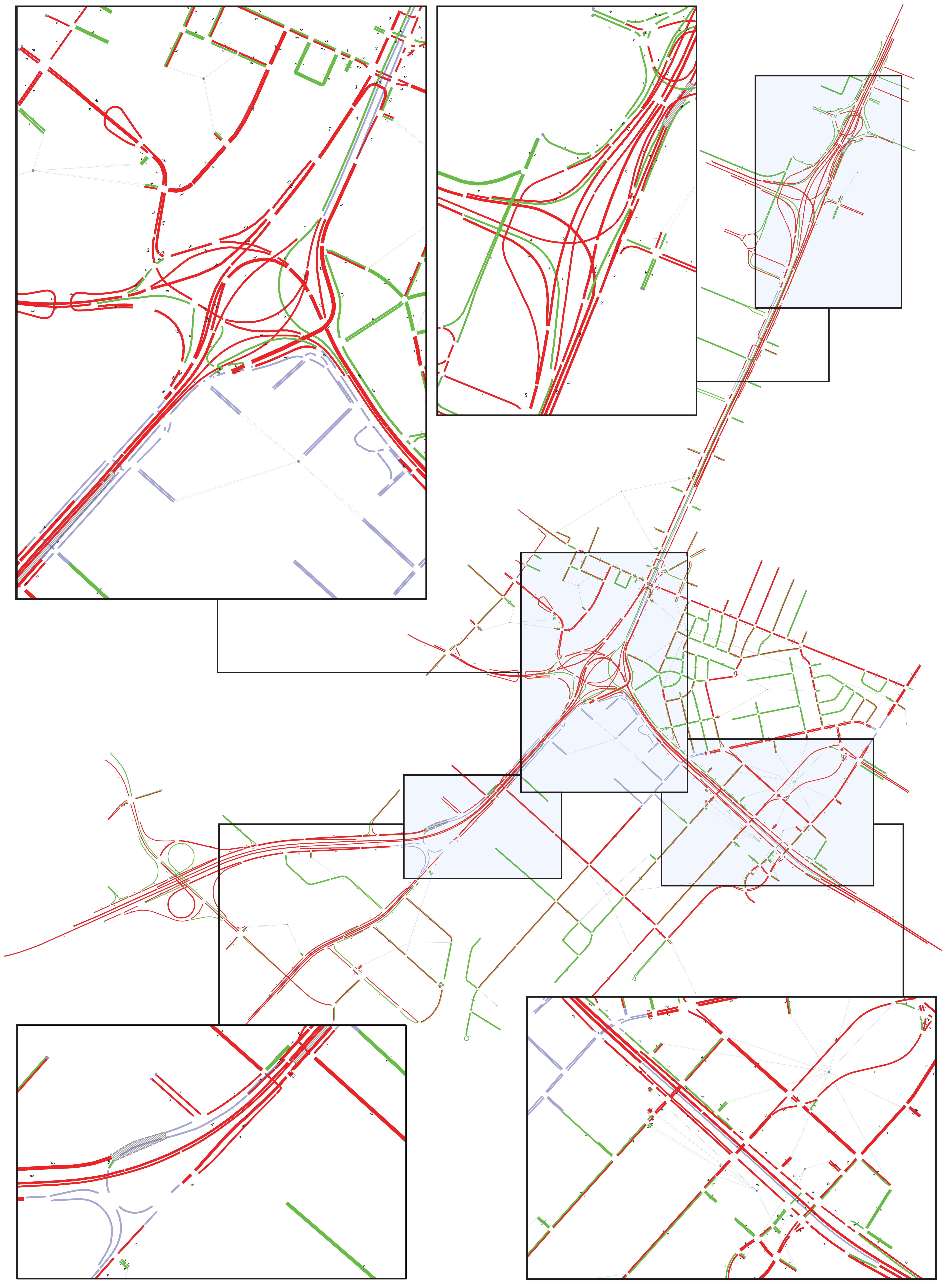
Figure C-2.5 DÉBITS DE CIRCULATION AJOUTÉS - SCÉNARIO 1 - HEURE DE POINTE PM
