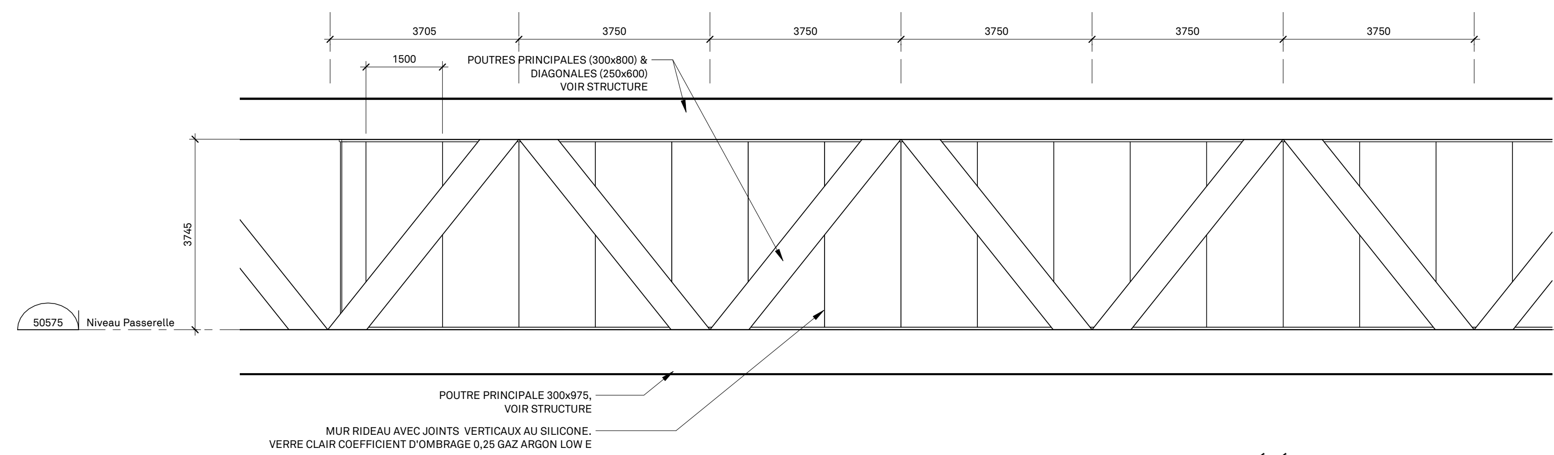
ÉLÉVATION TYPE MUR RIDEAU PASSERELLE 1 ÉCHELLE : 1:75 A251
