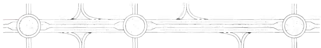
Fig. 10 — Principe d'aménagement des routes de type R à 2 x 2 voies.
