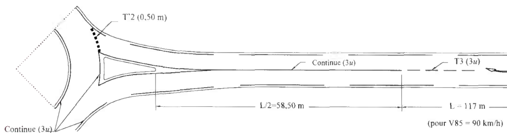
Fig. 21 — Principe d'implantation du marquage.
