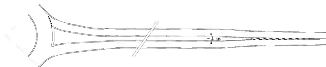
Fig. 16 — Exemple de traitement d'approche difficile par un allongement de l'îlot séparateur.
