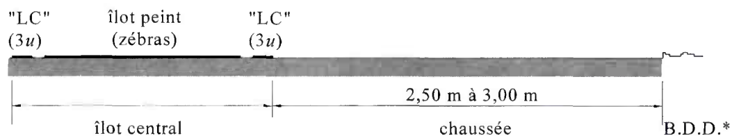
Fig. 19 — Détail de la réalisation des îlots peints pour les carrefours des routes secondaires à chaussée étroite (inférieure à 5 m).
