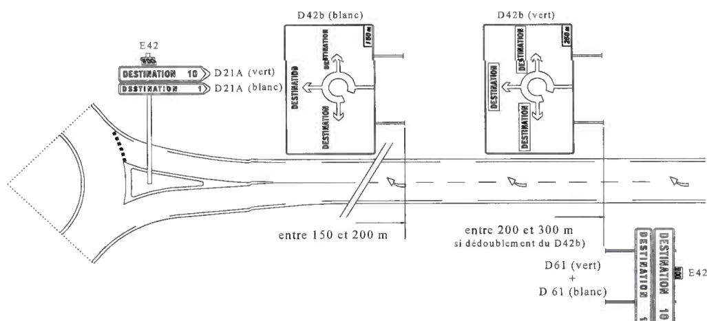
Fig. 20 — Principe d'implantation de la signalisation de direction. 23
