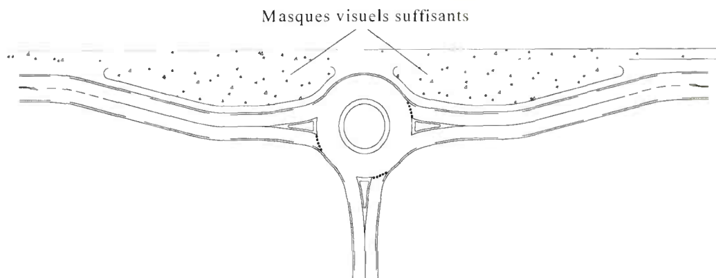
Fig. 7 — Configuration des branches d'un giratoire « en tête décalé ».
