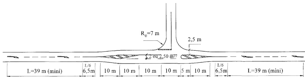
Fig. 18 — Caractéristiques minimales applicables aux aménagements de carrefours sur les routes secondaires à chaussée étroite ( inférieure à 5 m).
