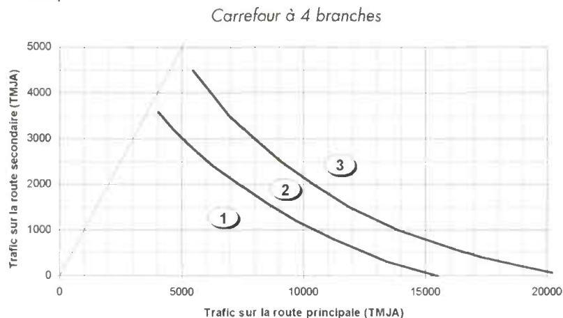
Fig. 1 — Quelques repères sur le niveau d'étude de trafic à mener (routes de rase campagne à 2 ou 3 voies).
