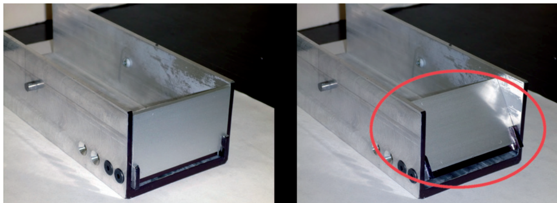
Figure 27 Montage de rétroréflexion variable
