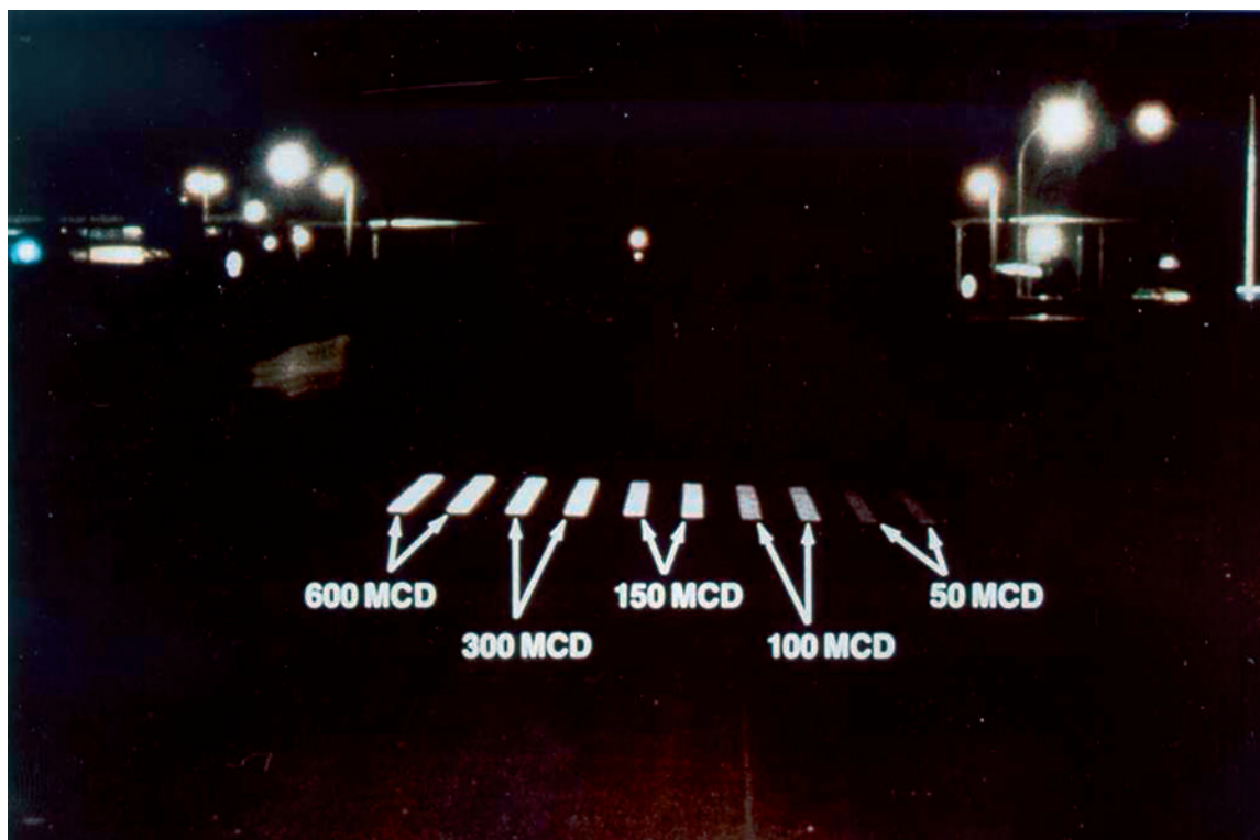
Figure 16 Détermination visuelle de la rétroréflexion (Réf. : 3M)
