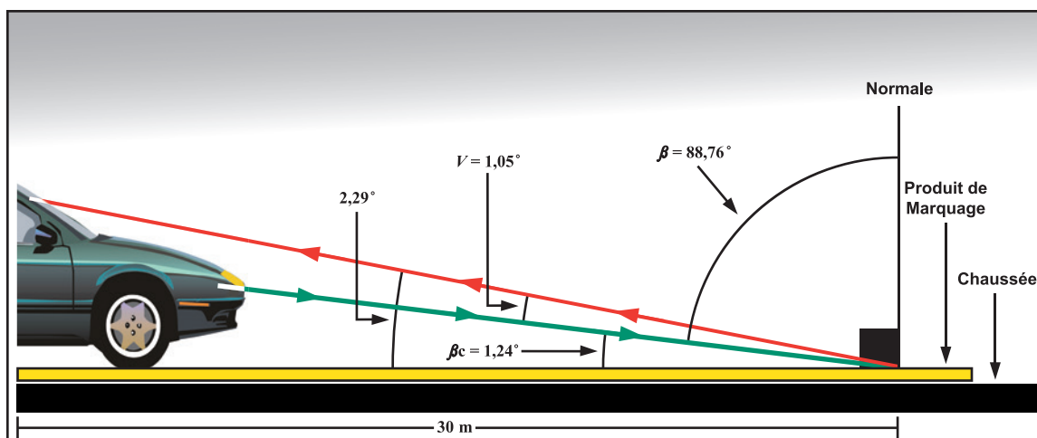
Figure 6 Géométrie de la rétro réflexion
