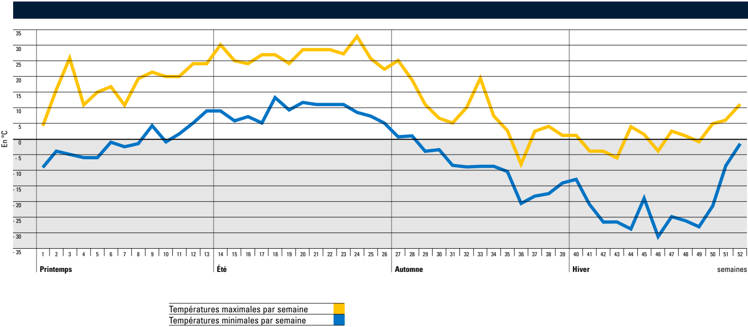
Températures minimales et maximales hebdomadaires – 1 (période du 29 mars 2002 au 28 mars 2003)
