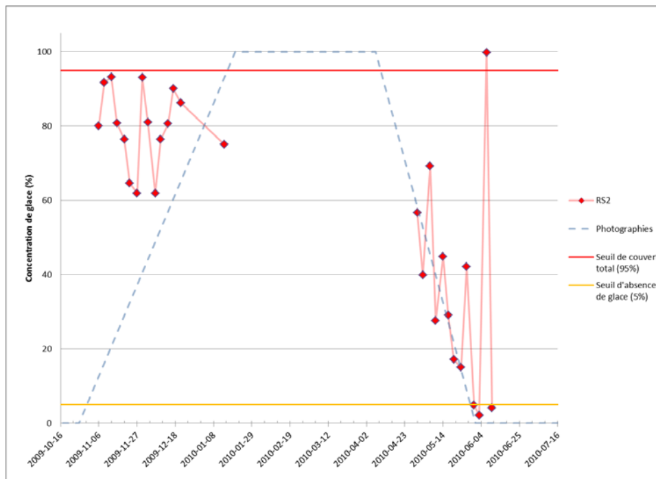
Figure 52 Concentrations de glace dans la zone d'influence autour de l'infrastructure maritime de Kuujuaq, hiver 2009-2010, selon les cartes de glace issues de RADARSAT-2 et les photos des caméras fixes.
