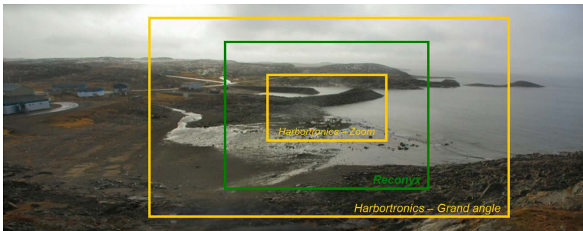
Figure 73 Comparaison des angles de champ de chacune des caméras
