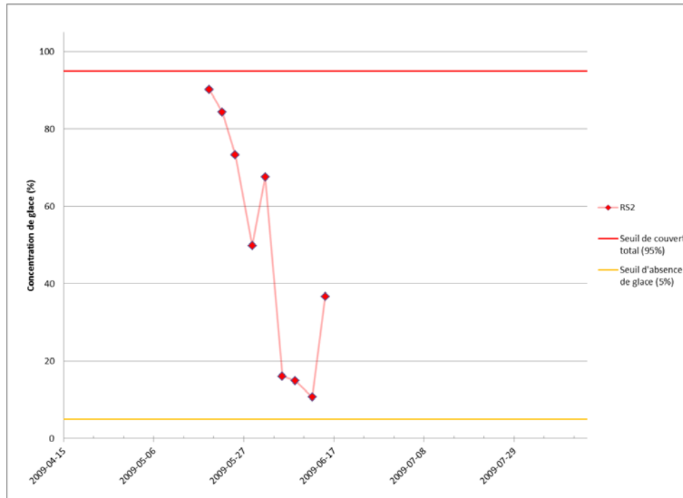
Figure 51 Concentrations de glace dans la zone d'influence autour de l'infrastructure maritime de Kuujuaq, printemps 2009, selon les cartes de glace issues de RADARSAT-2.
