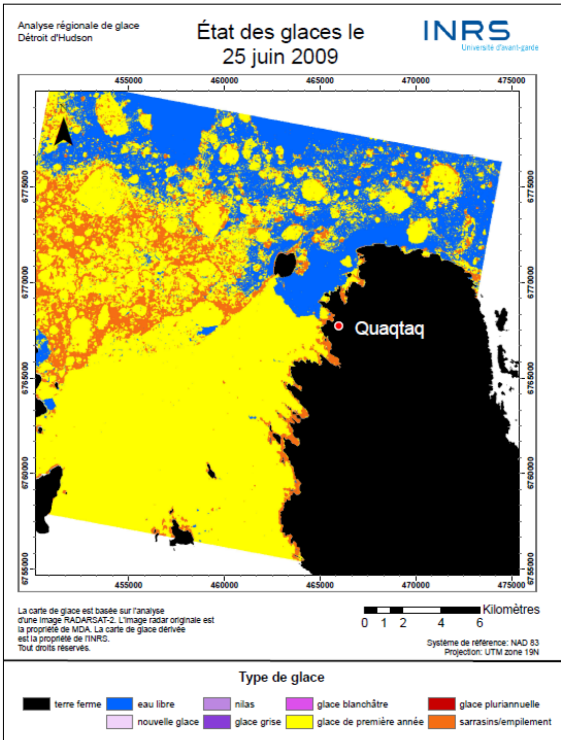
Figure 27 Carte de glace du 25 juin 2009. La banquise côtière est encore fixe dans la baie Diana alors qu'on observe de l'eau libre entre l'île Hearn et l'anse de la Mission.
