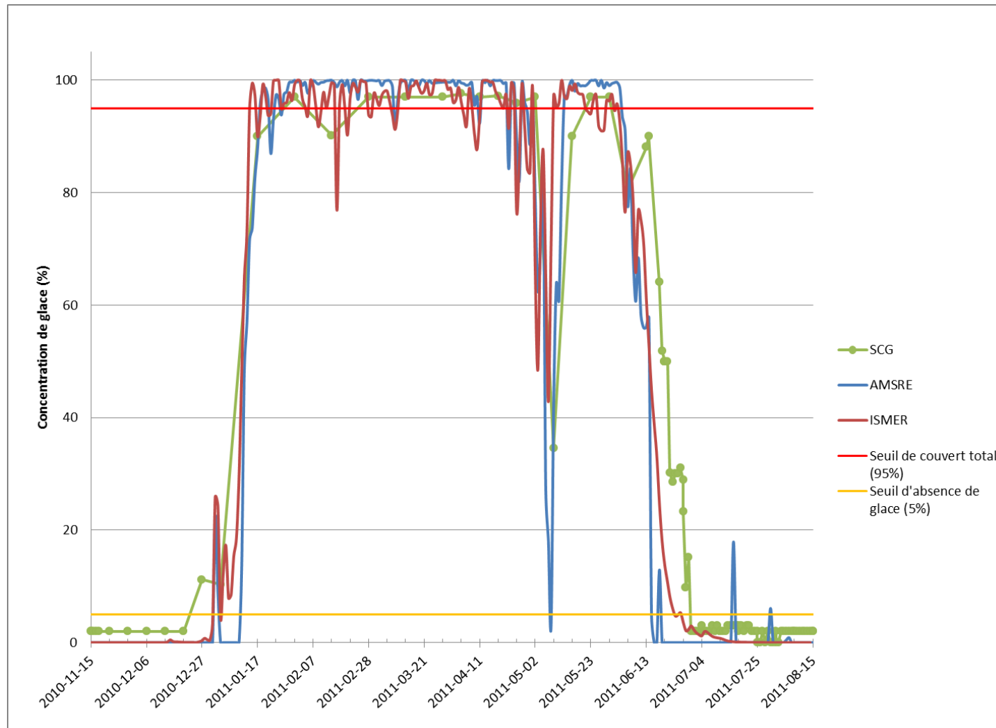
Figure 13 : Concentrations de glace dans le détroit d'Hudson, régime des glaces 2010-2011, à partir de trois différentes sources.
