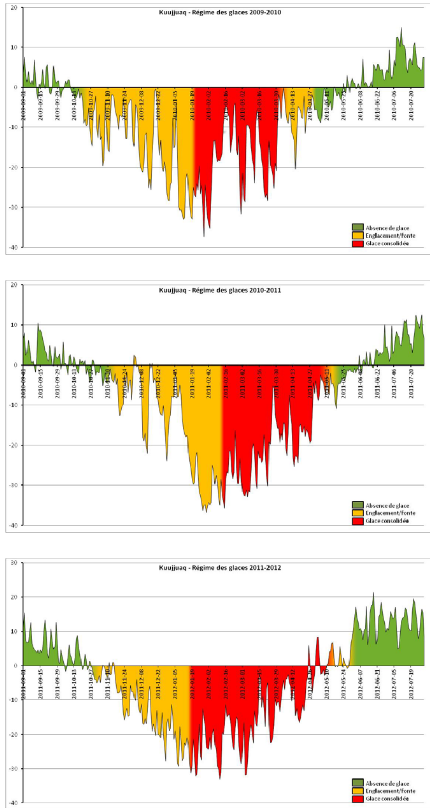
Figure 70 Description des régimes de glace 2009-2010, 2010-2011 et 2011-2012 en fonction de la température, pour la région de Kuujuaq.
