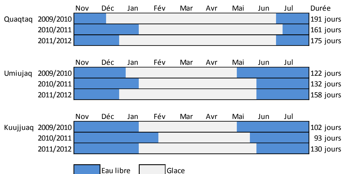
Figure 72 Période et durée en jours de la présence du couvert de glace pour les trois communautés (2009-2012)
