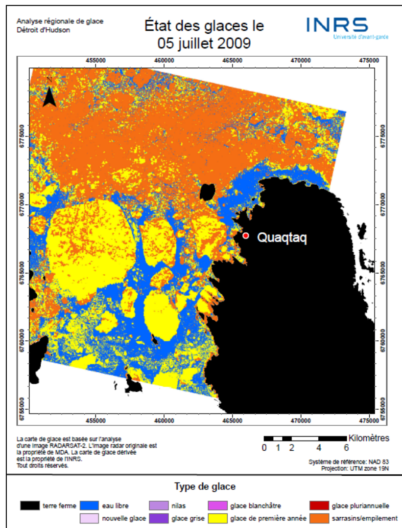
Figure 17 Carte des glaces lors de la fonte printanière 2009 dans la région de la Baie Diana, issue d'une image RADARSAT -2 en mode fin du 5 juillet 2009.
