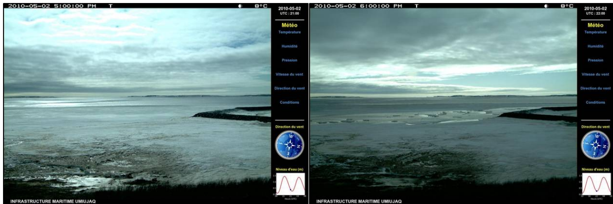
Figure 41 Décrochement de la banquise côtière en face du village d'Umiuqak le 2 mai 2010. À gauche, photo Reconyx prise à 17hrs et à droite, photo prise à 18 hrs.
