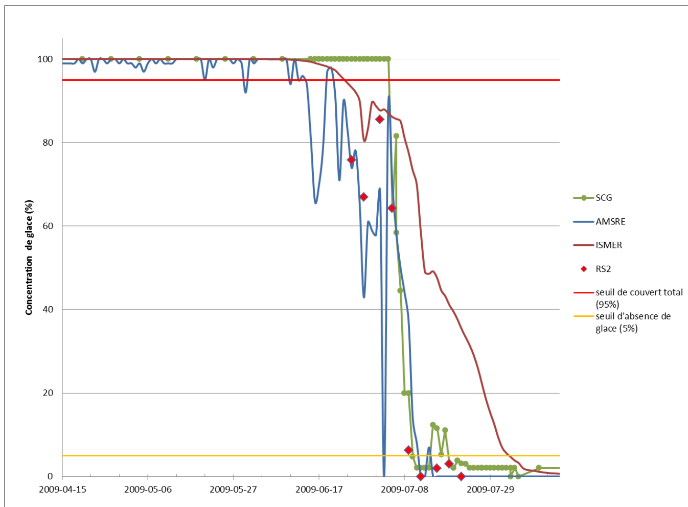
Figure 7 Concentrations de glace dans la baie Diana au printemps 2009 à partir de quatre différentes sources.
