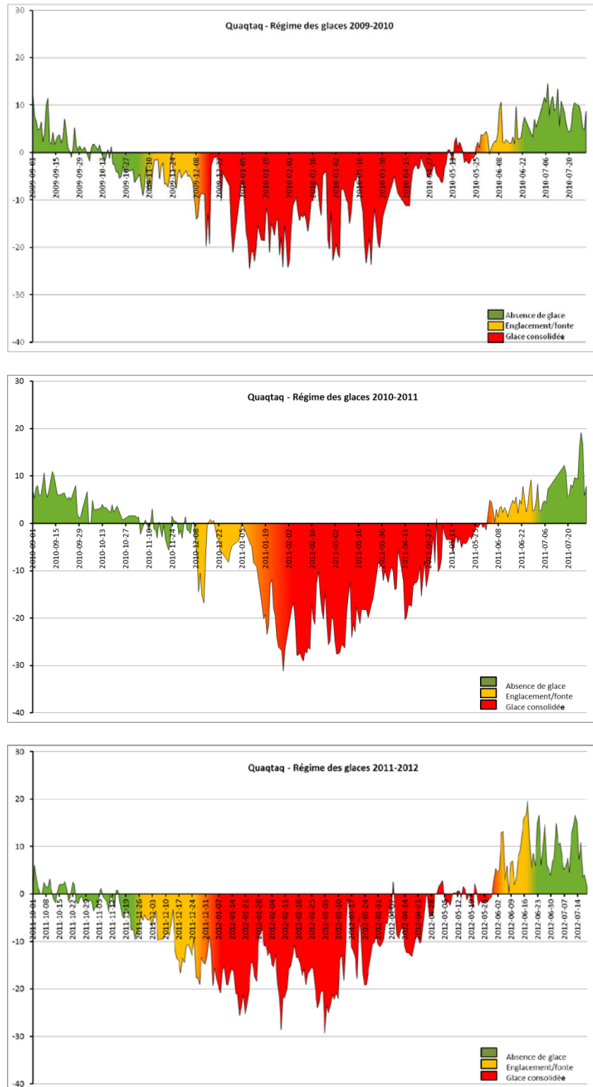
Figure 68 Description des régimes de glace en 2009-2010, 2010-2011 et 2011-2012 en fonction de la température pour la région de Quaqaq.
