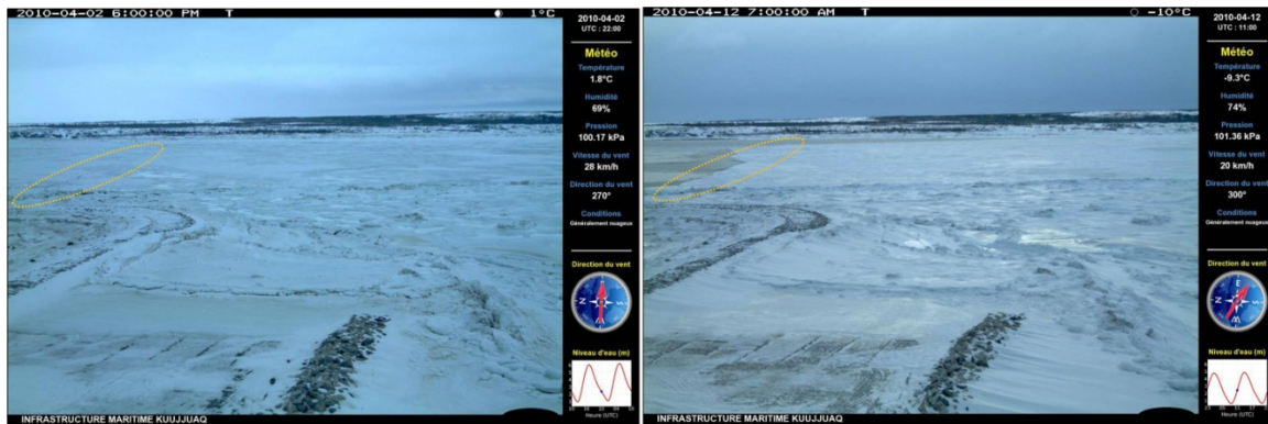
Figure 67 À gauche, apparition d'une fissure (encerclée en jaune) le 2 avril 2010. À droite, le 12 avril, migration du front de glace au niveau de cette fissure.
