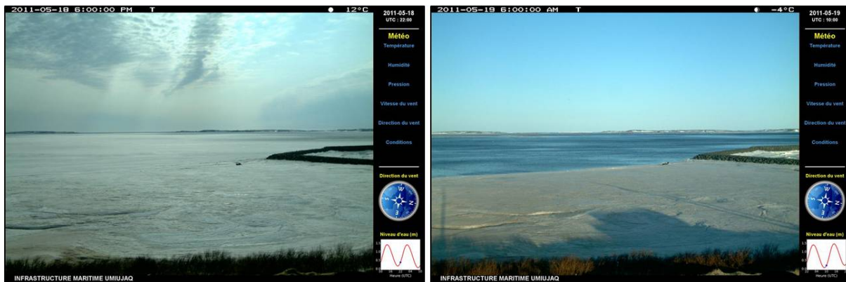
Figure 42 Évacuation de la banquise côtière en face du village d'Umiuqak au printemps 2011. À gauche, photo Reconyx du 18 mai 2011 à 17hrs et à droite, 11hrs plus tard, photo du 19 mai 2011 à 6hrs.
