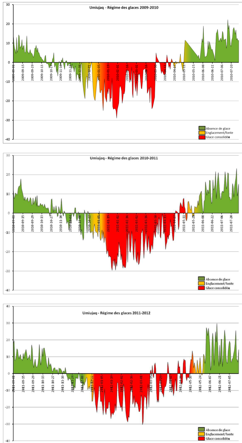
Figure 69 Description des régimes de glace en 2009-2010, 2010-2011 et 2011-2012 en fonction de la température, pour la région d'Umiujaq.
