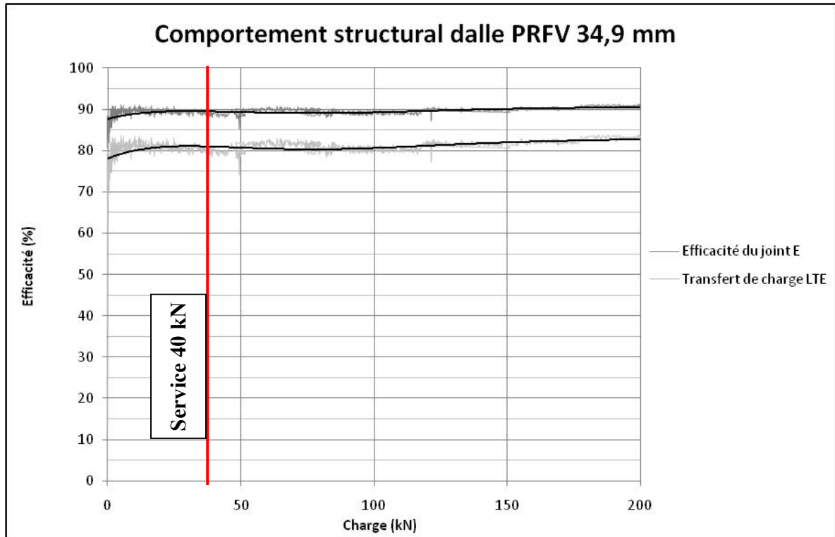
Figure 3.81 : Efficacité et transfert de charge sous chargement monotonique
