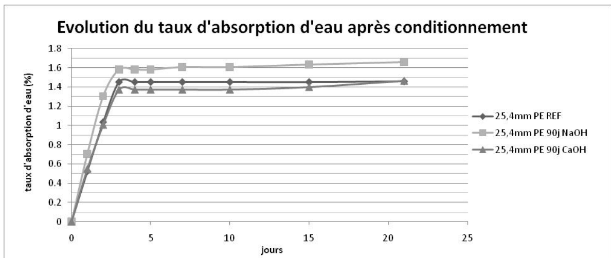
Figure 3.36 : Taux d'absorption d'eau à saturation résine polyester
