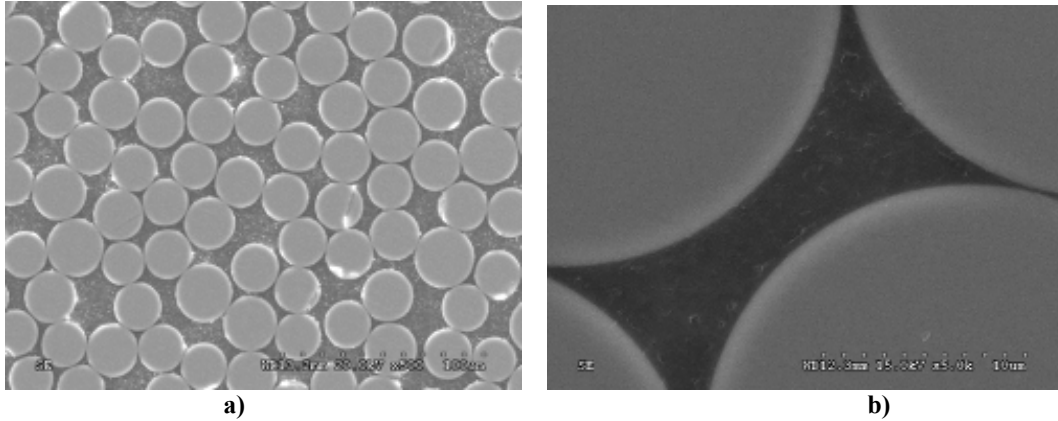
Figures 3.40 : Microscopies à l'état initial de goujon en résine polyester de diamètre 25,4 mm, grossissements de a) 500 et b) 5 000 fois
