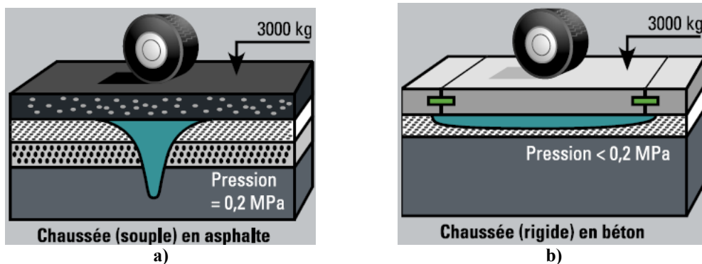
Figures 2.1 : Répartition de la charge sur des chaussées a) en asphalte, b) en béton [Ciment Québec, 2002]
