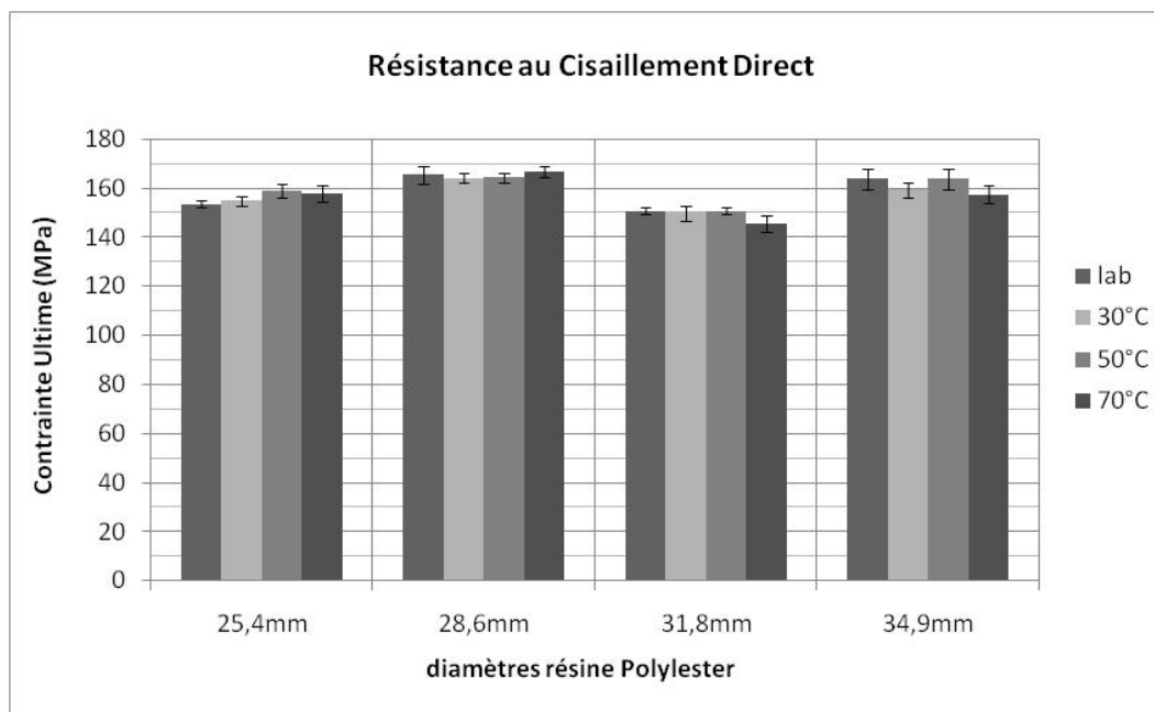
Figure 3.12 : Résistance au cisaillement direct à différentes températures (résine polyester)
