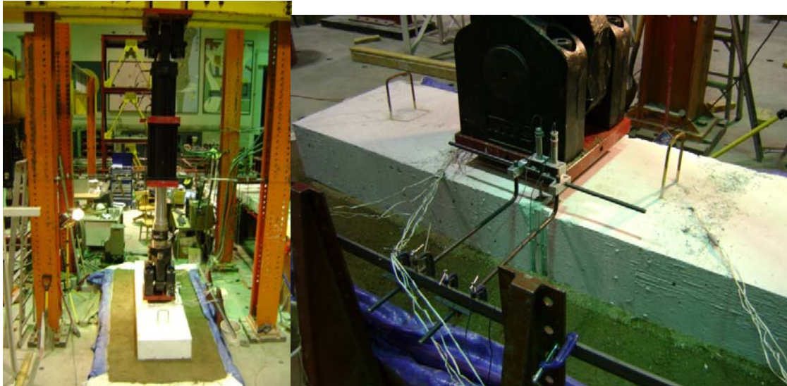
Figures 3.75 : Montage en laboratoire
