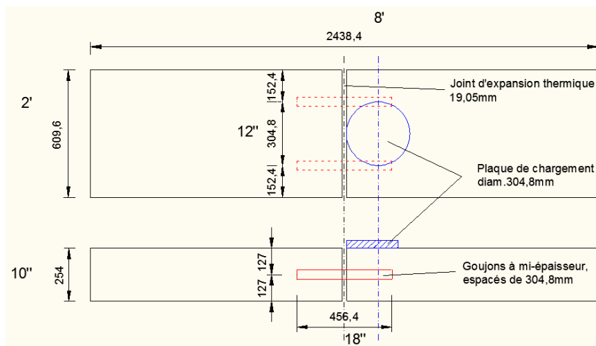
Figure 3.69 : Dimensions des spécimens de dalle testés (mm)
