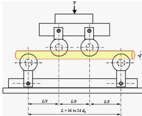
Figure 3.3 : Montage de flexion par 4 points
