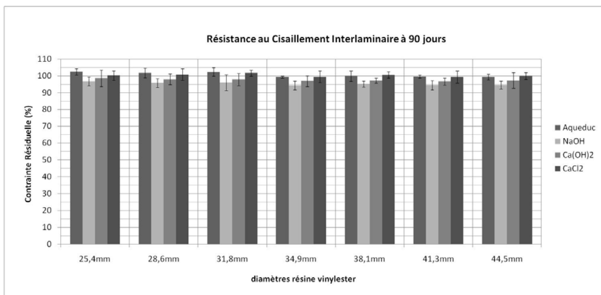
Figure 3.32 : Résistance au cisaillement interlaminaire après 90 jours de conditionnement dans différentes solutions (résine vinylester)
