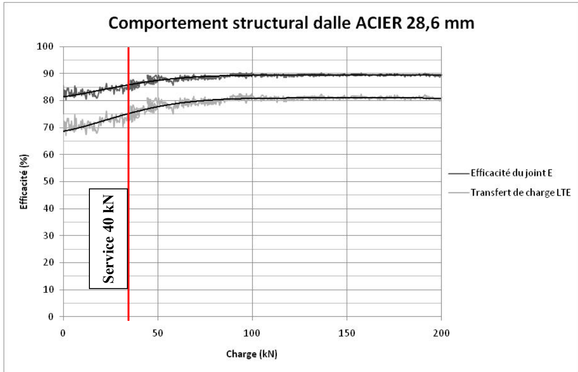
Figure 3.78 : Efficacité et transfert de charge sous chargement monotonique
