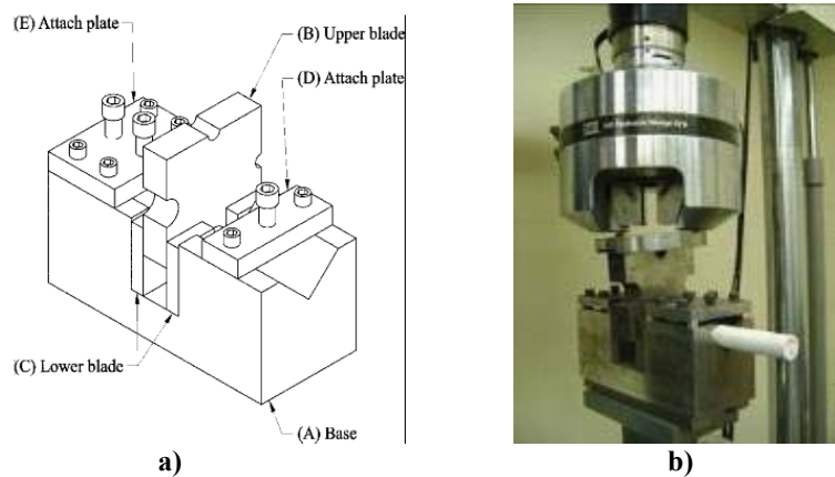
Figures 3.2 : Montage de cisaillement direct
