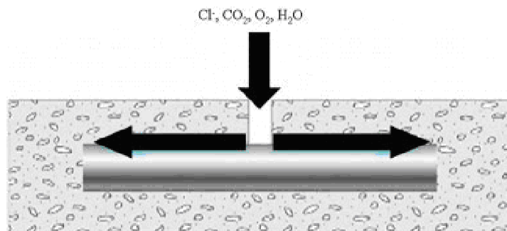
Figure 2.17 : Infiltration des ions agressifs par le joint de chaussée ou une fissure [Park et al., 2008]
