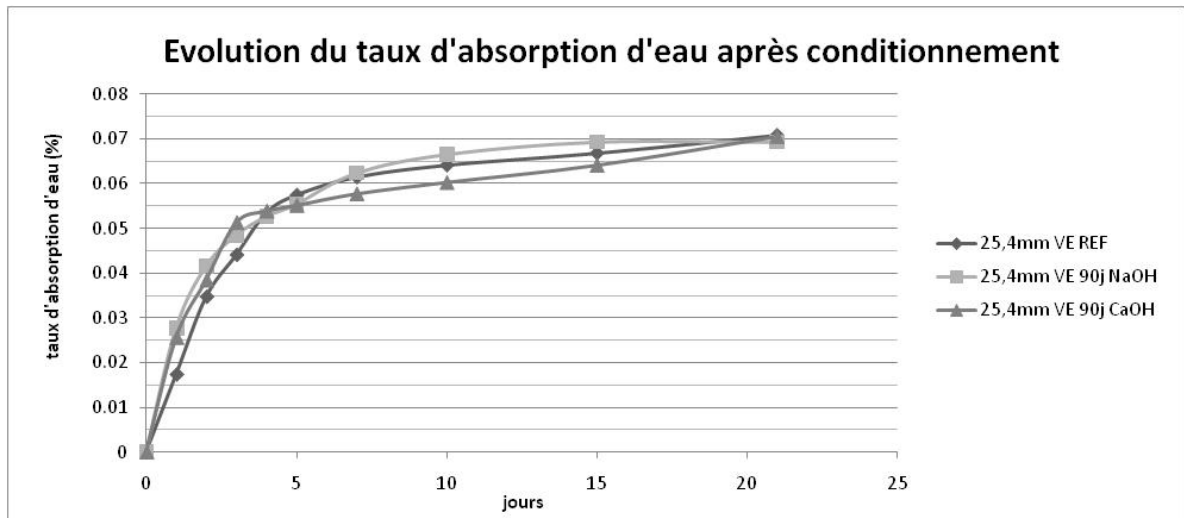
Figure 3.35 : Taux d'absorption d'eau à saturation résine vinylester
