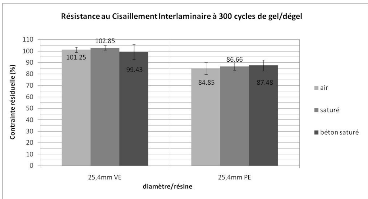
Figure 3.30 : Résistance au cisaillement interlaminaire de goujons 25,4 mm après 300 cycles de gel/dégel
