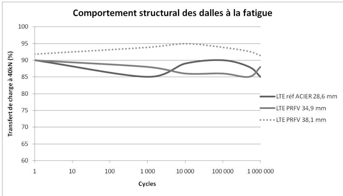
Figure 3.92 : Transfert de charge sous chargement réglementaire de 40 kN
