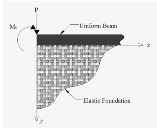
Figure 3.64 : Poutre semi-infinie sur une base élastique [Porter, 2006]
