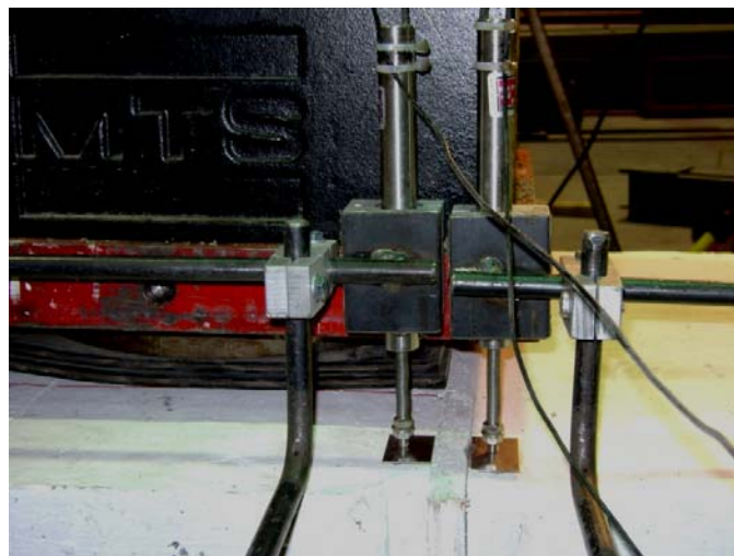
Figure 3.76 : Mesure des déflexions de chaque dalle de part et d'autre de joint (LVDT)
