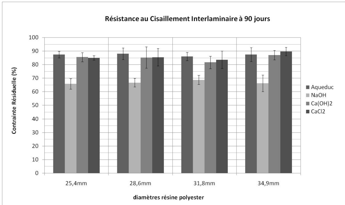
Figure 3.33 : Résistance au cisaillement interlaminaire après 90 jours de conditionnement dans différentes solutions (résine polyester)
