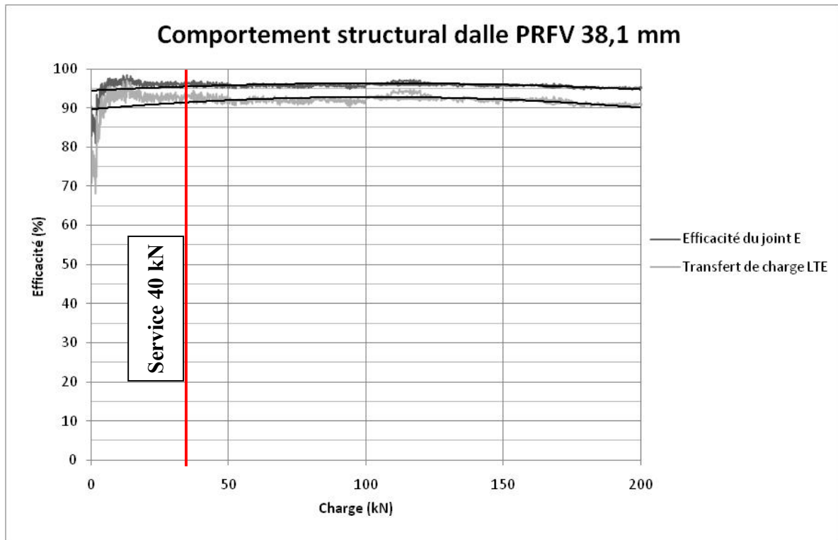
Figure 3.84 : Efficacité et transfert de charge sous chargement monotonique
