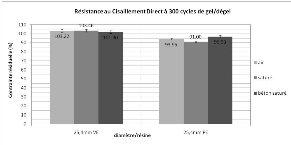
Figure 3.29 : Résistance au cisaillement direct de goujons 25,4 mm après 300 cycles de gel/dégel
