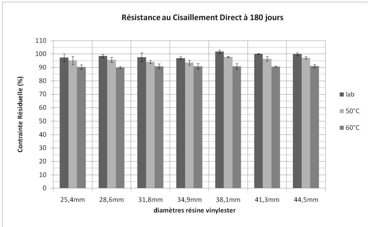
Figure 3.45 : Résistance au cisaillement direct après conditionnement (résine vinylester)
