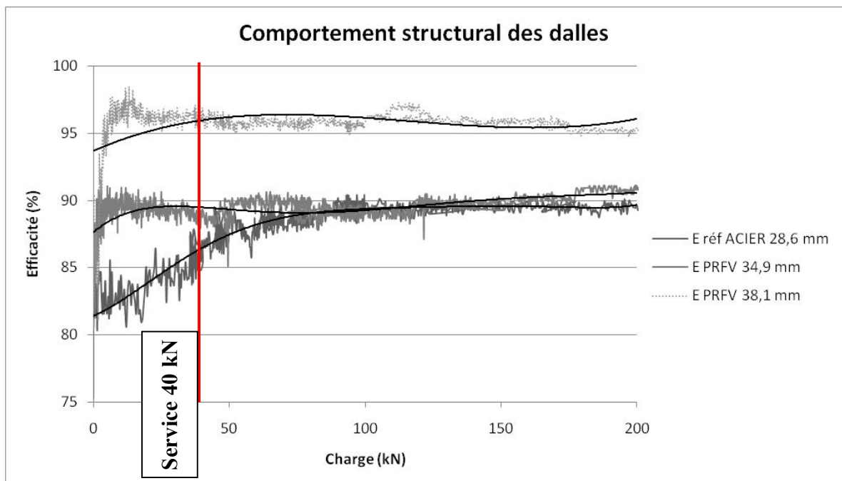
Figure 3.86 : Efficacité du joint sous chargement monotonique
