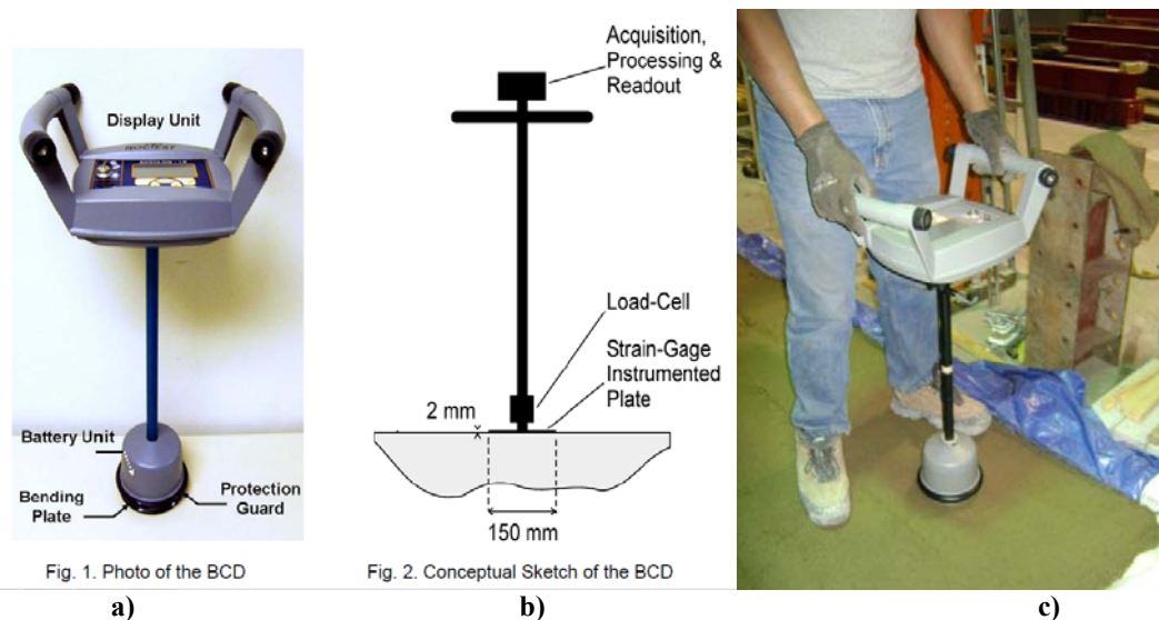
Figures 3.74 : appareil BCD de contrôle de compaction
