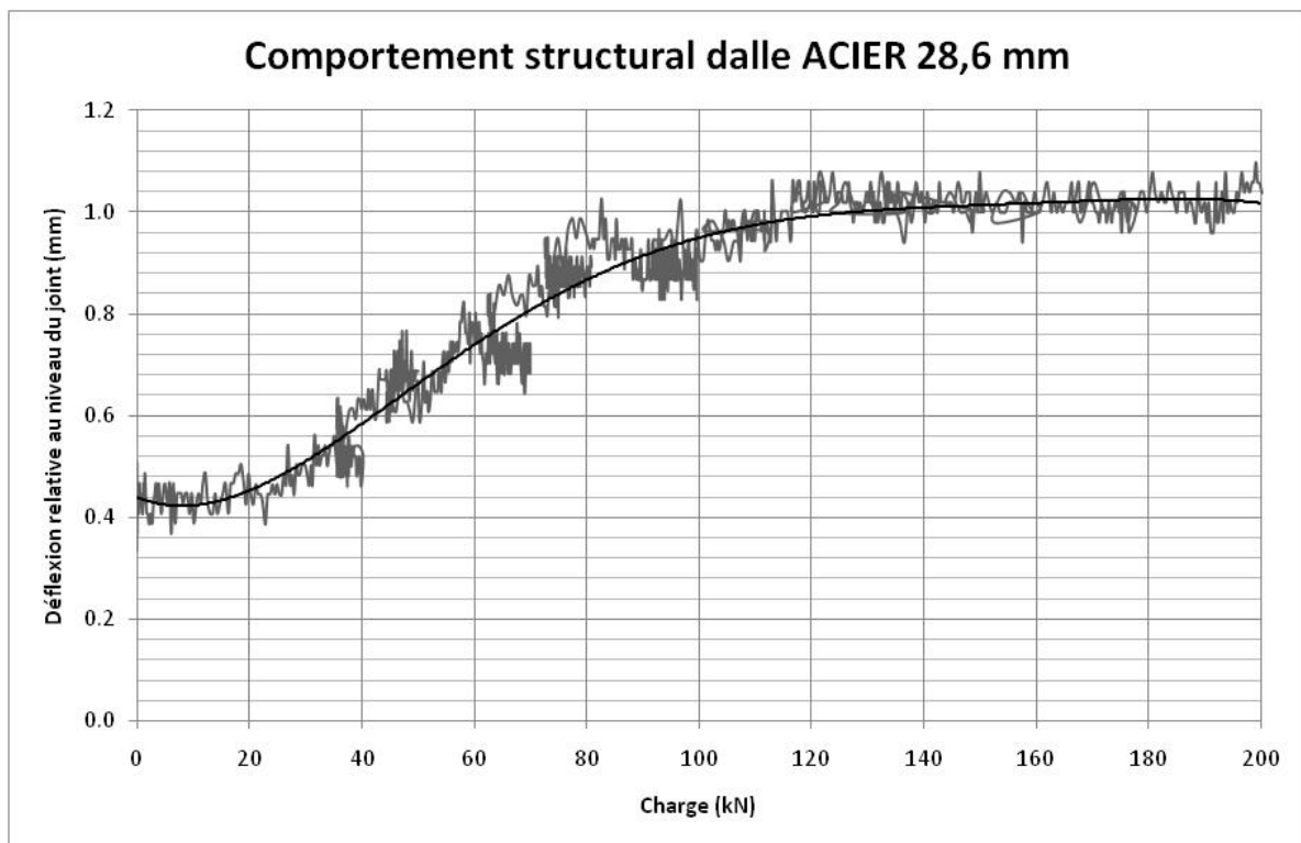
Figure 3.79 : Déflexion relative des dalles sous chargement monotonique
