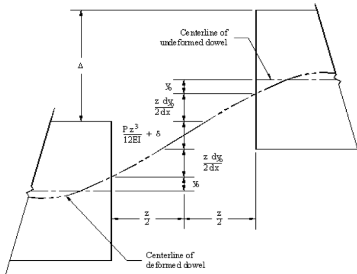
Figure 3.66 : Déflexion relative entre dalles goujonnées [Porter et al., 2006]
