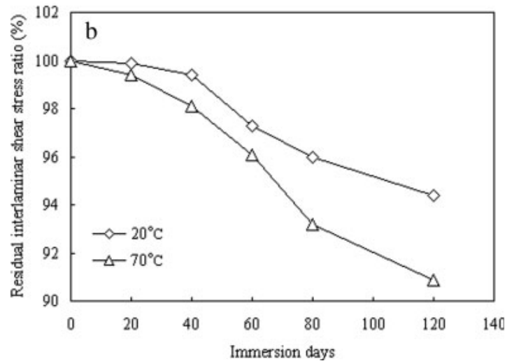
Figure 2.19 : Propriétés interlaminaires résiduelles (%) [Park et al., 2008]
