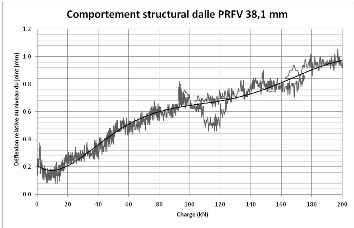
Figure 3.85 : Déflexion relative des dalles sous chargement monotonique
