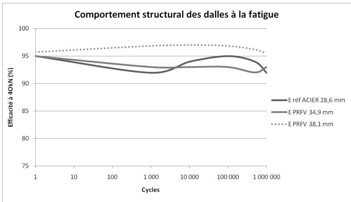
Figure 3.91 : Efficacité du joint à long terme sous chargement réglementaire de 40 kN
