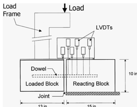
Figure 3.65 : Instrumentation de spécimens de dalles goudonnées [Porter et al., 2006]
