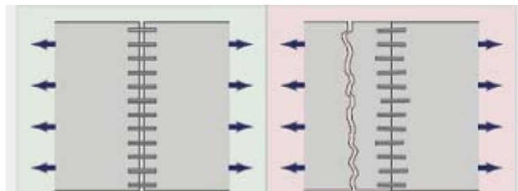
Figure 2.6 : Effet du mauvais alignement des goudons [ACPA, 2008]
