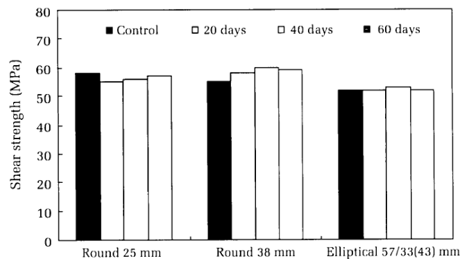
Figure 2.21 : Résistance au cisaillement en solution saline à 70°C [Won et al., 2006]
