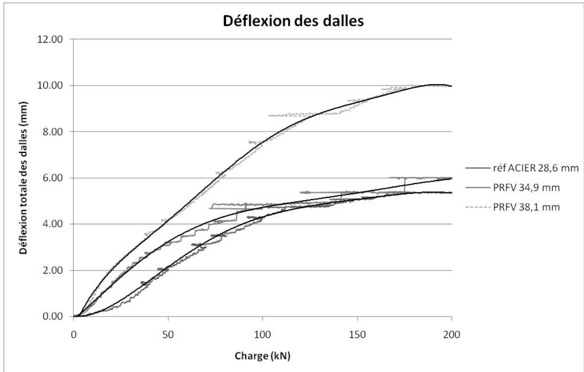
Figure 3.89 : Déflexion totale des dalles sous chargement monotonique (dalle côté chargé)
