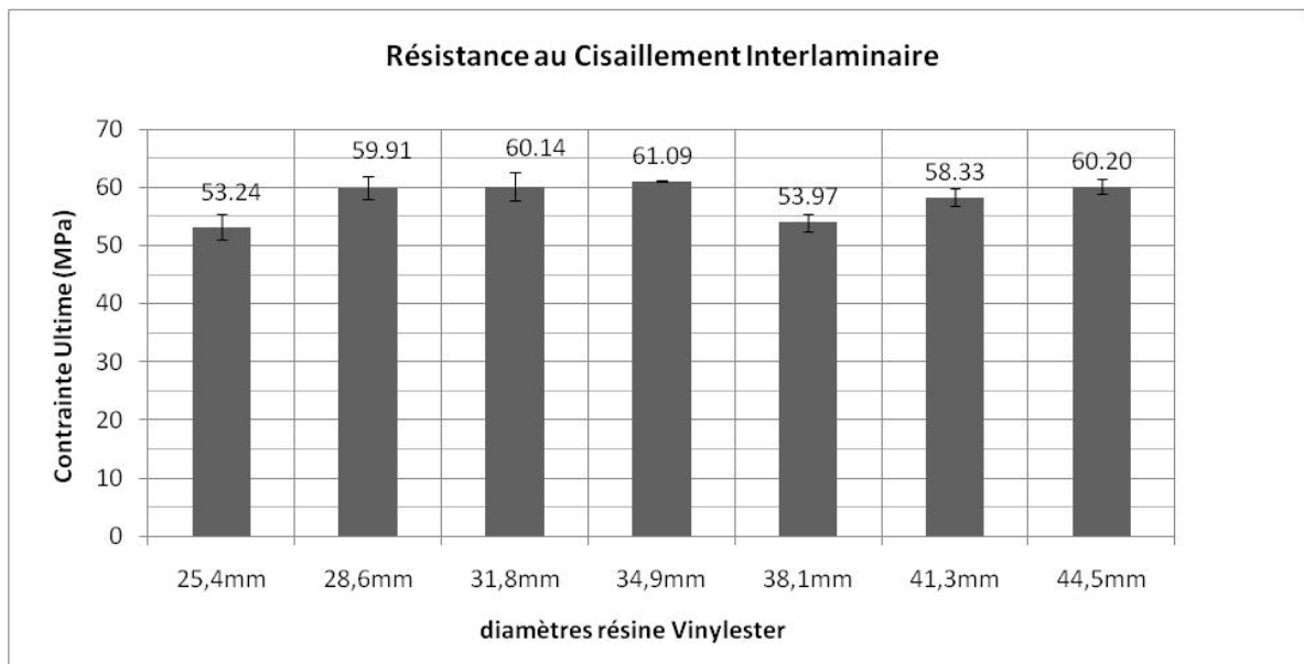
Figure 3.18 : Résistance au cisaillement interlaminaire à température ambiante (résine vinylester)
