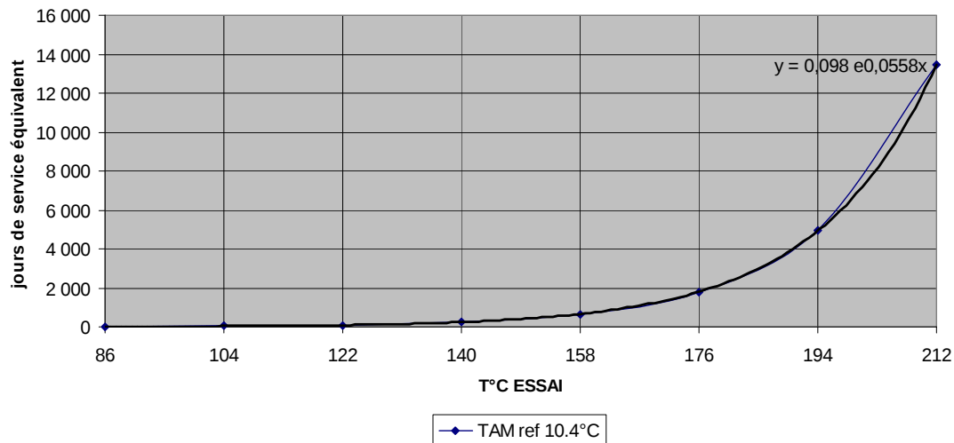
Figure 2.24 : Simulation jours de service à 10,4°C/jours d'essai en fonction de la température
