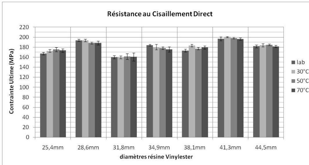
Figure 3.11 : Résistance au cisaillement direct à différentes températures (résine vinylester)
