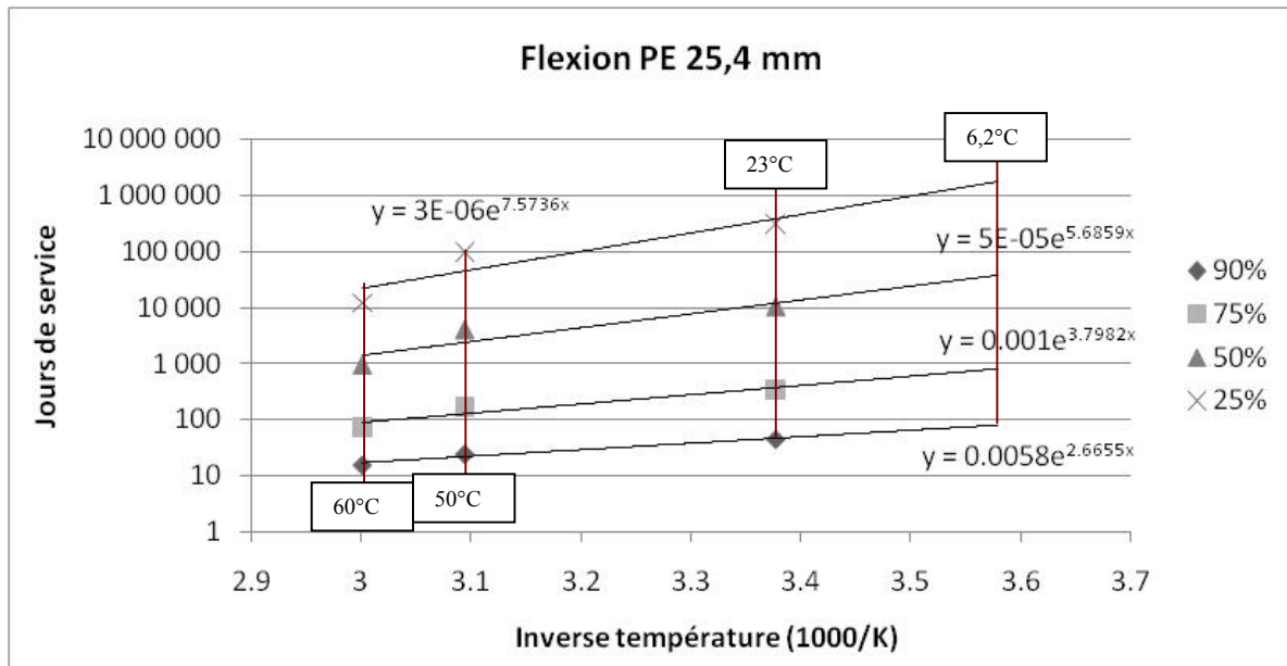
Figure 3.60 : Courbes des taux de rétention de la contrainte en flexion en fonction de la température
