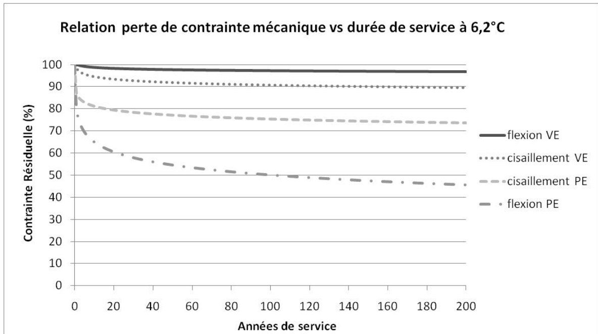
Figure 3.61 : Prédiction des propriétés mécaniques à long terme
