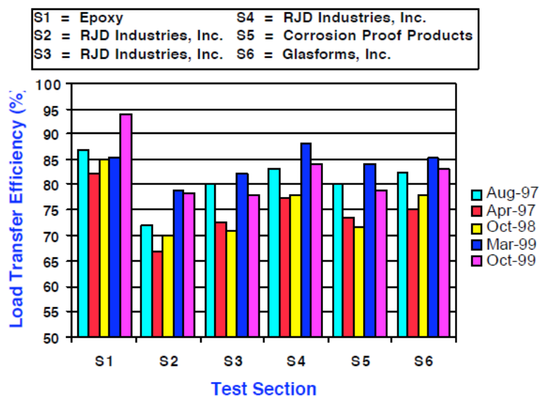
Figure 2.14 : Transferts de charge des différents goujons à différentes périodes [Smith, 2001]
