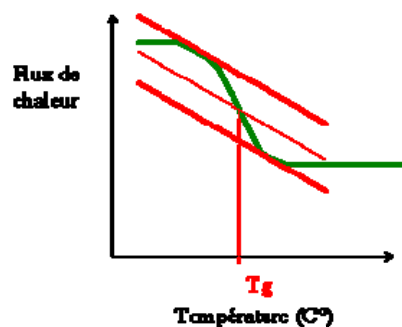
Figure 3.6 : Phase de transition vitreuse
