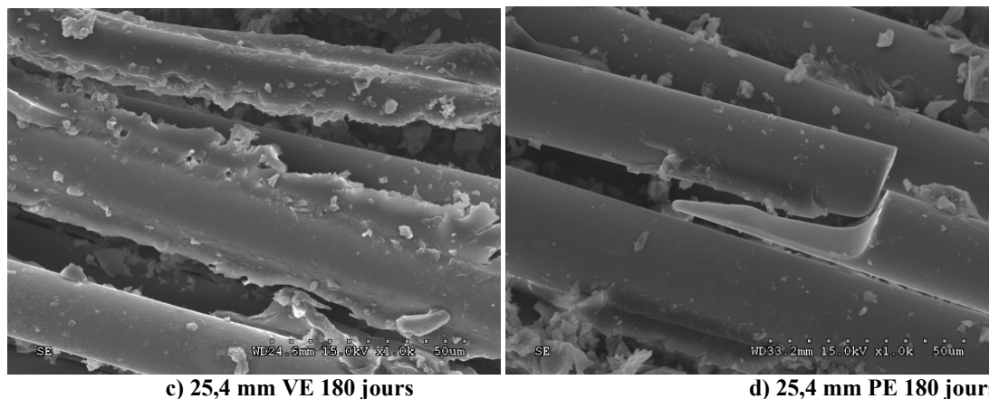
Figures 3.58 : Faciès de rupture en flexion de goujons de diamètre 25,4 mm après 180 jours à 60°C en solution alcaline (grossissement de 1 000 fois)
