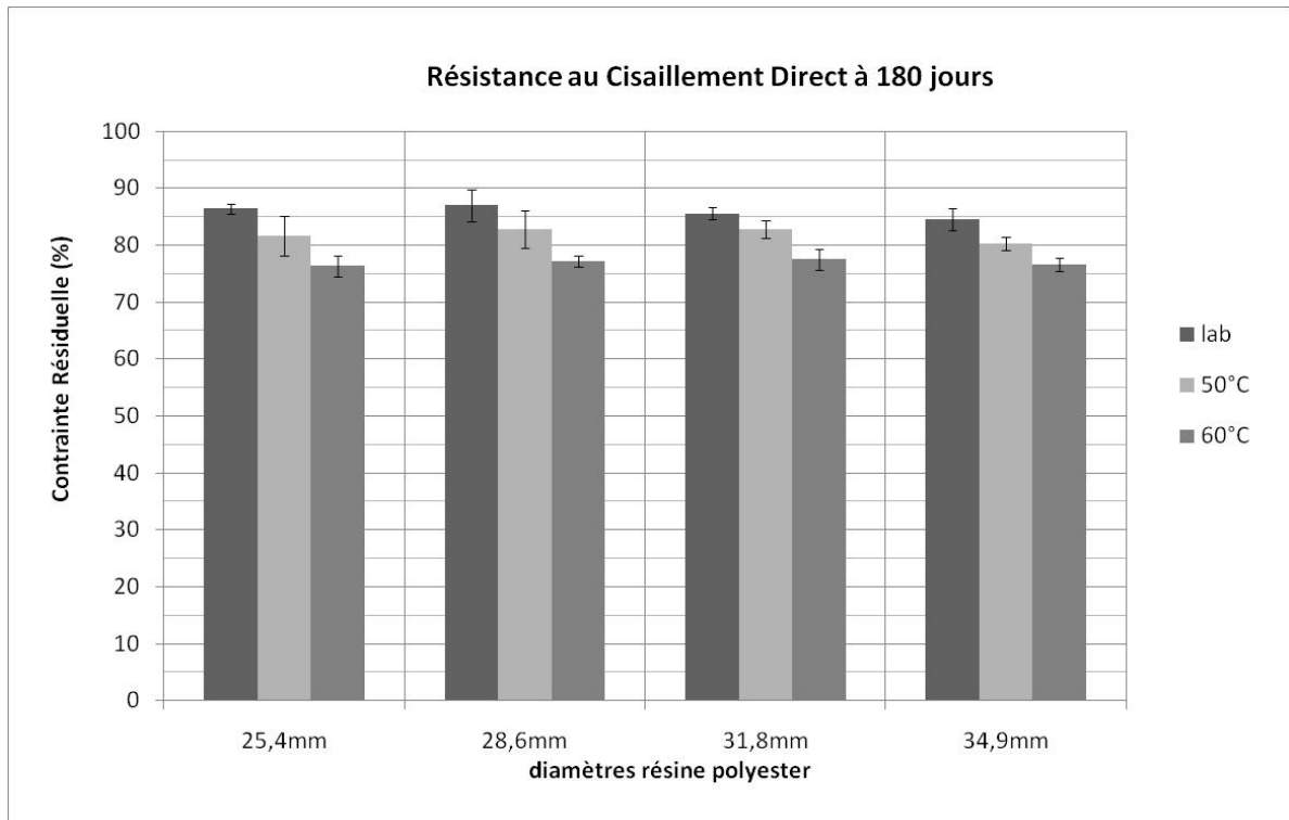
Figure 3.47 : Résistance au cisaillement direct après conditionnement (résine polyester)
