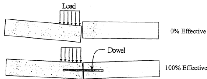
Figure 2.9 : Efficacité du joint [Eddie et al., 2001]
