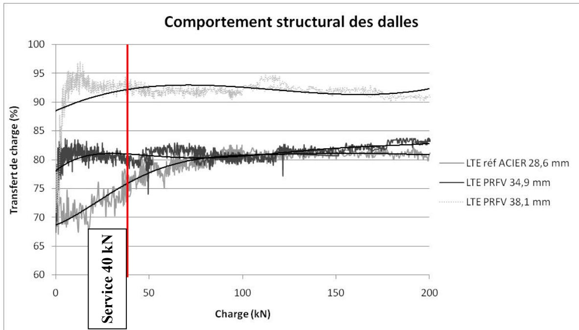
Figure 3.87 : Transfert de charge sous chargement monotonique
