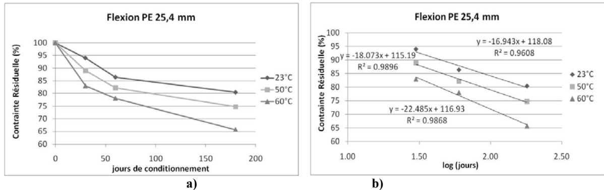
Figures 3.59 : Courbes de dégradation en fonction du temps et de la température a) échelle linéaire et b) logarithmique
