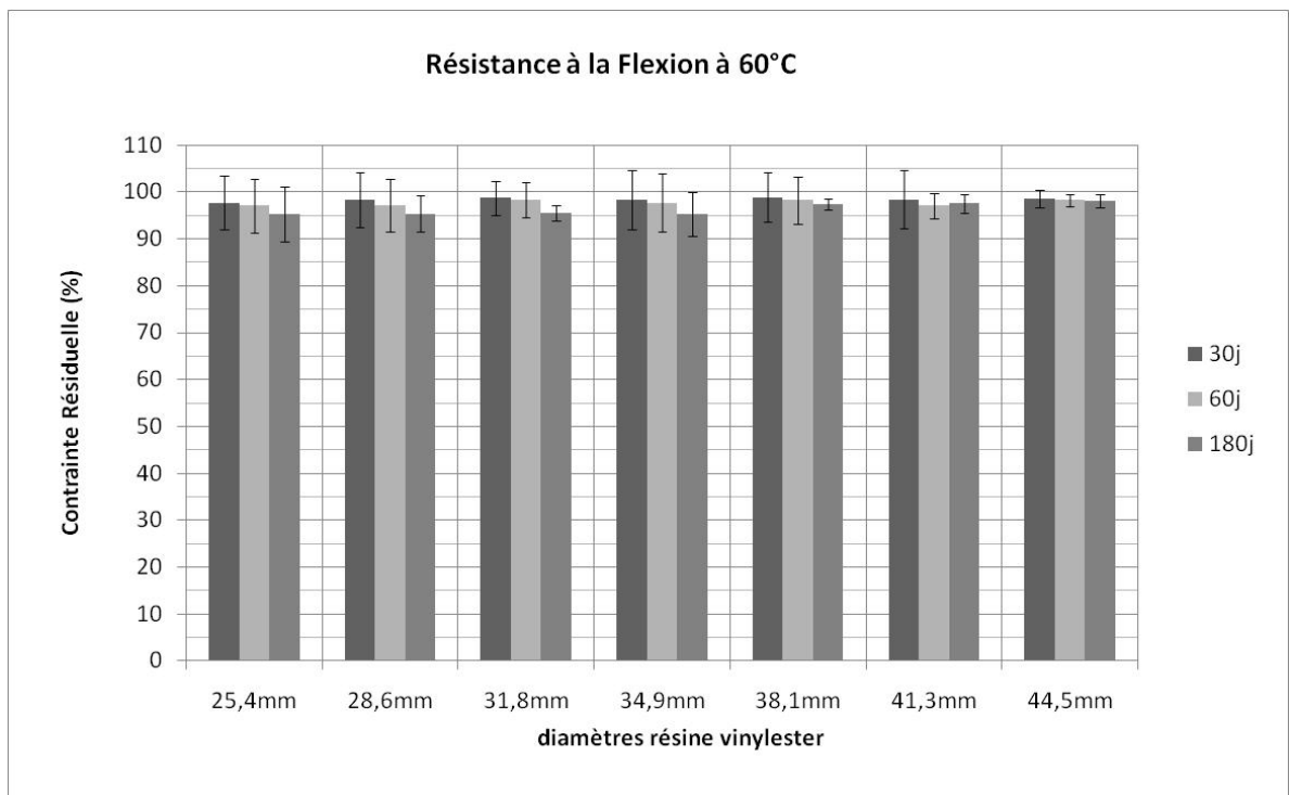
Figure 3.50 : Résistance à la flexion par 4 points après conditionnement (résine vinylester)
