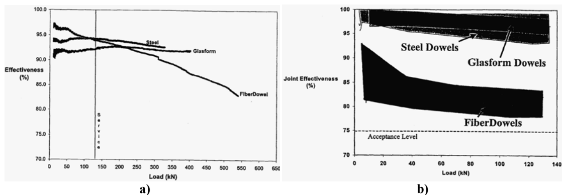
Figures 2.16 : Efficacité du joint sous chargement statique a) initial, b) jusqu'à 1 000 000 de cycles [Eddie et al., 2001]
