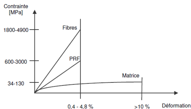
Figure 2.12 : Courbes contrainte/déformation des PRF, fibres et matrice [ISIS Design Manual #3, (2009)]
