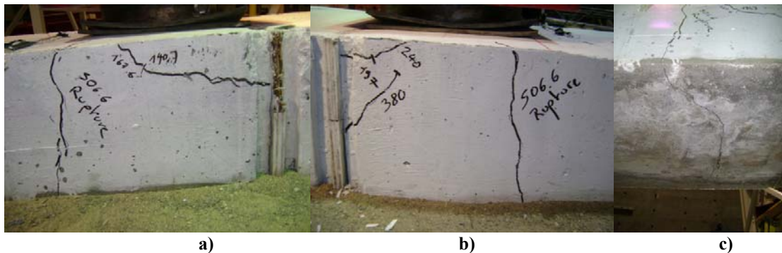
Figures 3.77 : Fissuration de la dalle côté chargé a) bord 1, b) bord 2 et c) rupture en cisaillement
