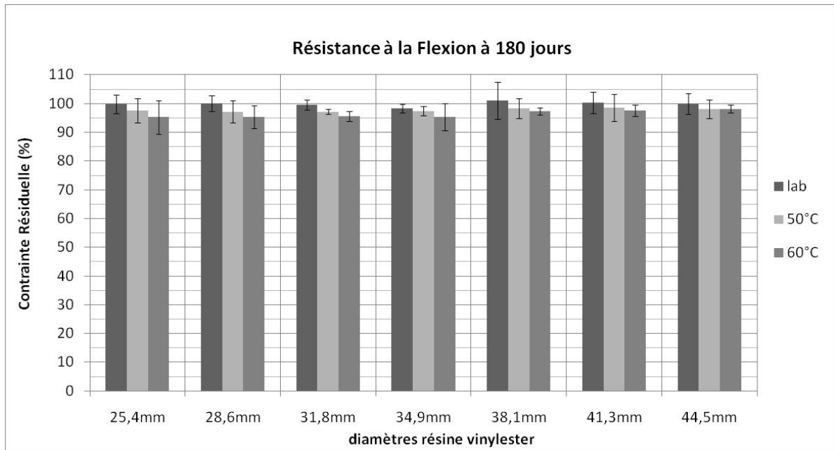
Figure 3.49 : Résistance à la flexion par 4 points après conditionnement (résine vinylester)
