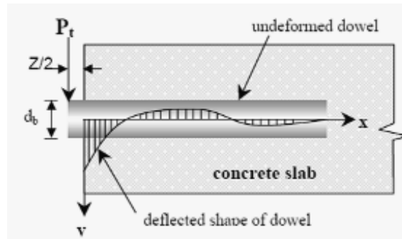
Figure 3.63 : Courbe de déflexion d'un goujon au sein du béton [Murison et al., 2002]
