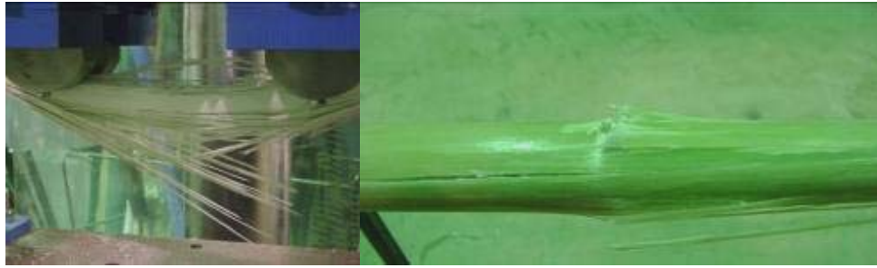
Figures 3.15 : Rupture en flexion équilibrée des goujons de PRFV
