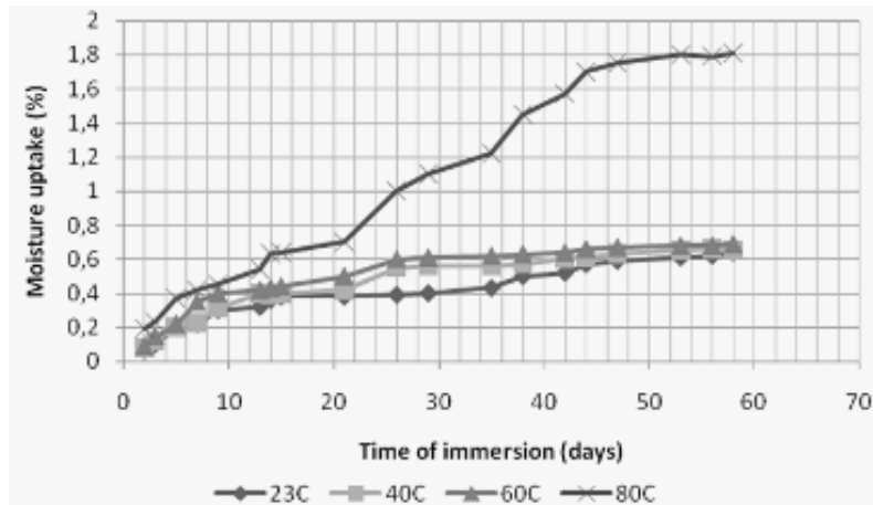
Figure 2.25 Absorption d'eau de barres de PRFV dans l'eau à différentes températures [Wang, 2005]
