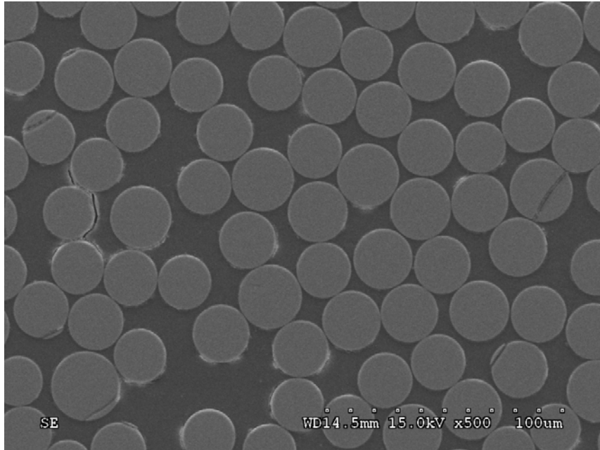
Figure 3.42 : Microscopies après 90 jours en solution de 3% NaOH de goujon en résine polyester de diamètre 25,4 mm (grossissements de 500 fois au centre de la barre)
