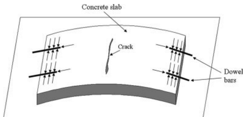
Figure 2.3 : Conséquences du verrouillage d'un joint [Park et al., 2008]
