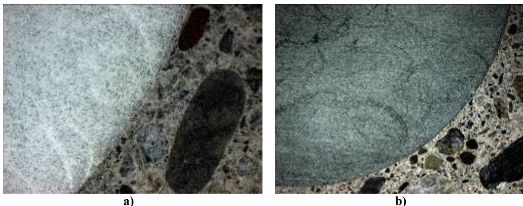
Figures 3.31 : microscopies optiques après 300 cycles de gel/dégel de goujons a) de polyester et b) de vinylester
