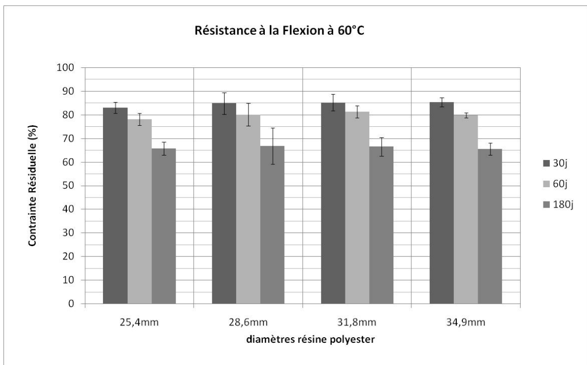
Figure 3.52 : Résistance à la flexion par 4 points après conditionnement (résine polyester)
