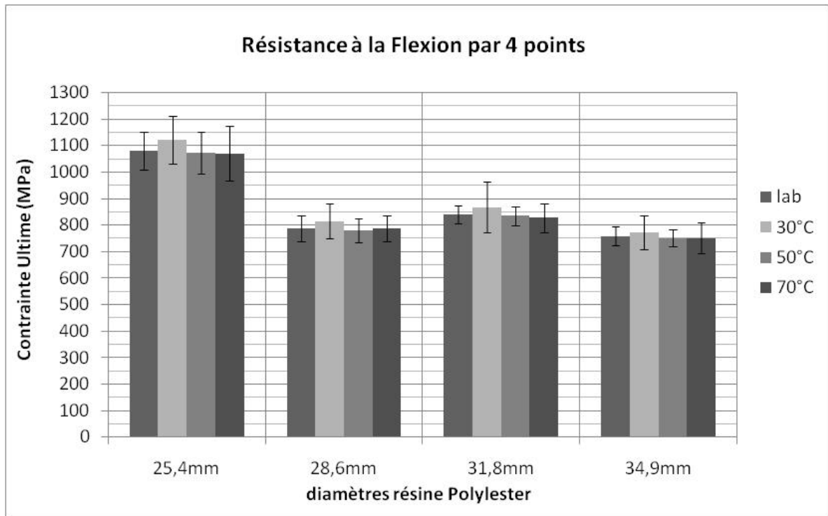
Figure 3.17 : Résistance à la flexion par 4 points à différentes températures (résine polyester)
