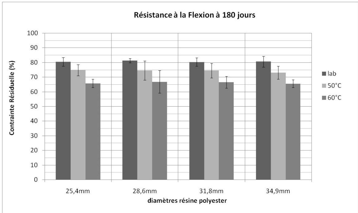
Figure 3.51 : Résistance à la flexion par 4 points après conditionnement (résine polyester)
