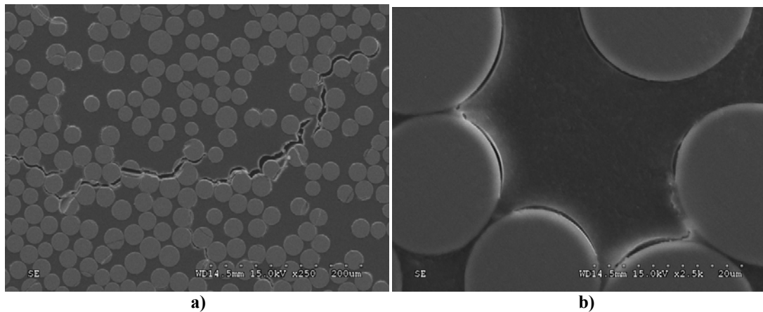
Figures 3.41 : Microscopies après 90 jours en solution de 3% NaOH de goujon en résine polyester de diamètre 25,4 mm, grossissements de a) 250 et b) 2 500 fois
