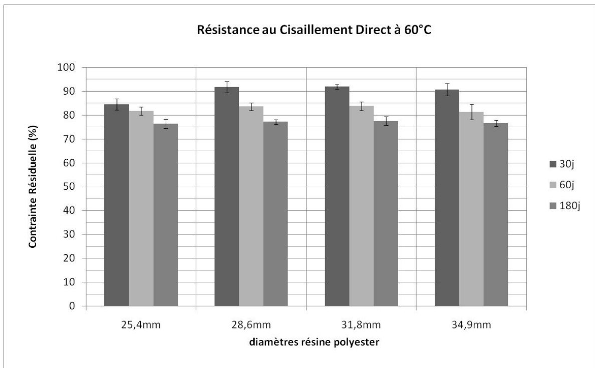
Figure 3.48 : Résistance au cisaillement direct après conditionnement (résine polyester)
