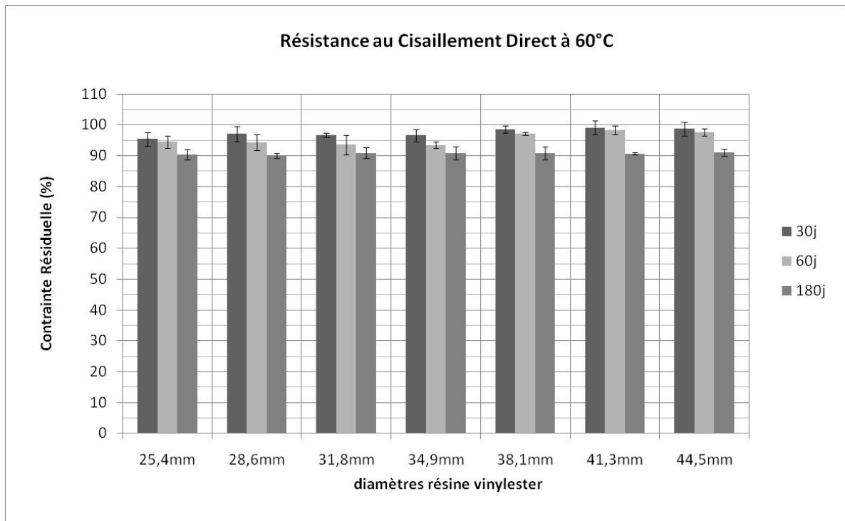
Figure 3.46 : Résistance au cisaillement direct après conditionnement (résine vinylester)
