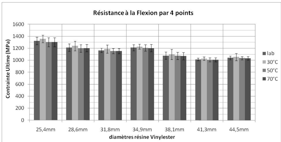
Figure 3.16 : Résistance à la flexion par 4 points à différentes températures (résine vinylester)
