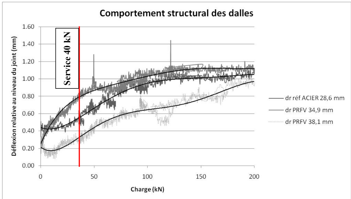
Figure 3.88 : Déflexion relative des dalles sous chargement monotonique
