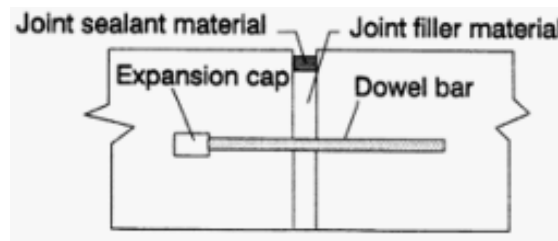
Figure 2.5 : Caractéristiques d'un joint d'expansion [FHA, 2009]
