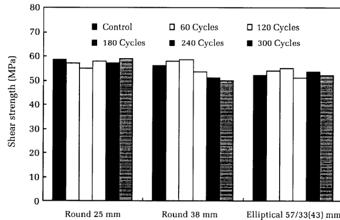
Figure 2.22 : Résistance au cisaillement interlaminaire après des cycles de gel/dégel [Won et al., 2006]
