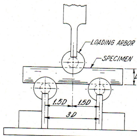
Figure 3.5 : Montage de cisaillement interlaminaire [ASTM D 4475-02]
