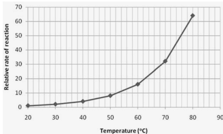
Figure 2.23 : Évolution du degré de réaction k en fonction de la température [Robert et al., 2008]
