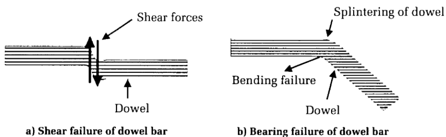
1. Figure 2.10 : Modes de fonctionnement en service des goujons [Won et al., 2006]
