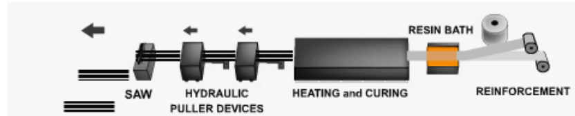
Figure 2.13 : Procédé de pultrusion [Pultrall, (2009)]
