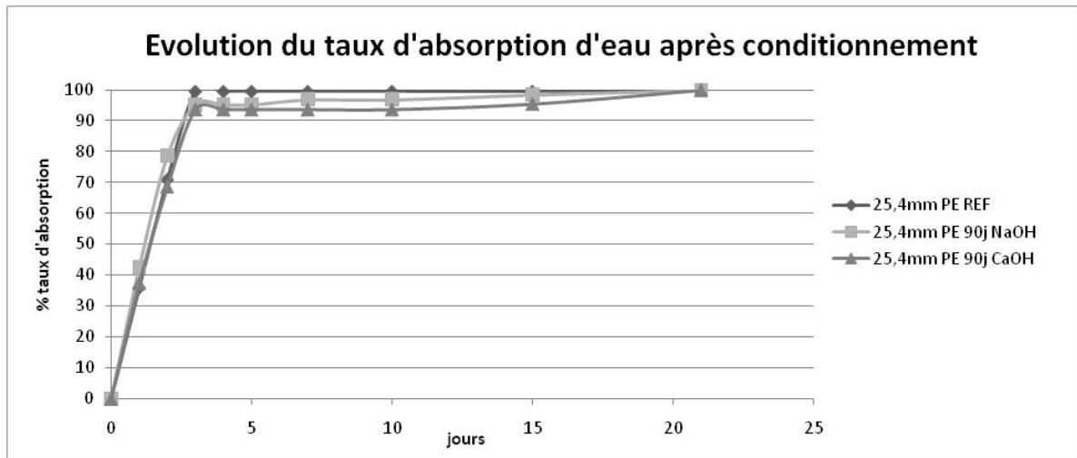
Figure 3.37 : Cinétique d'absorption résine polyester
