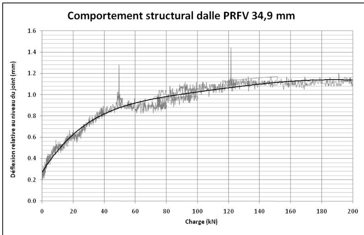
Figure 3.82 : Déflexion relative des dalles sous chargement monotonique
