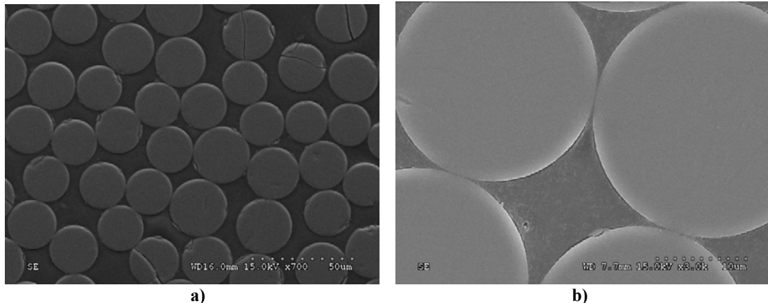
Figures 3.57 : microscopies après 180 jours d'immersion à 60°C de goujon en résine vinylester de diamètre 25,4 mm, grossissements de a) 700 et b) 3 000 fois
