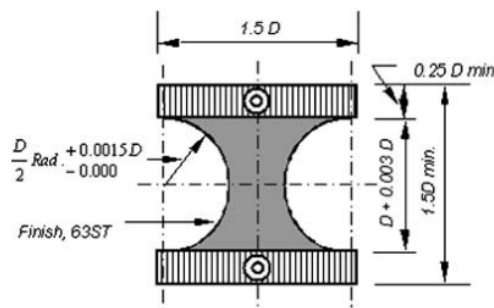
Figure 3.4 : Poulie de support et chargement
