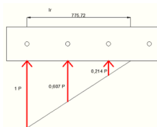
Figure 3.68 : Distribution du transfert de charge
