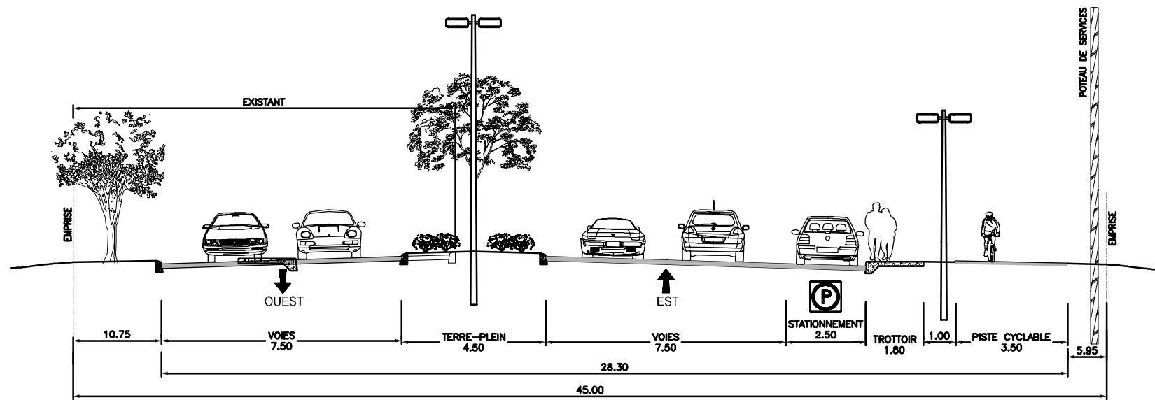
COUPE FL-A RUE FÉLIX-LECLERC AVEC PISTE CYCLABLE ET "KISS'n RIDE" POUR LA GARE
