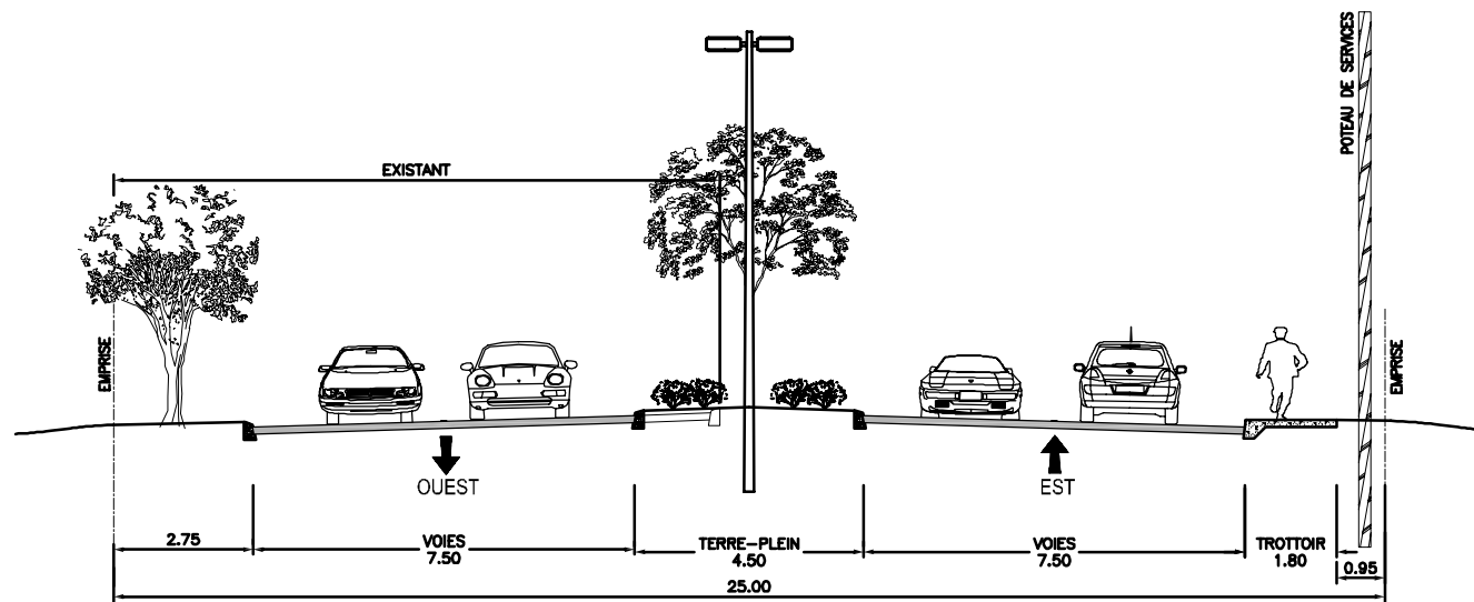
COUPE FL-B RUE FÉLIX-LECLERC SANS PISTE CYCLABLE
