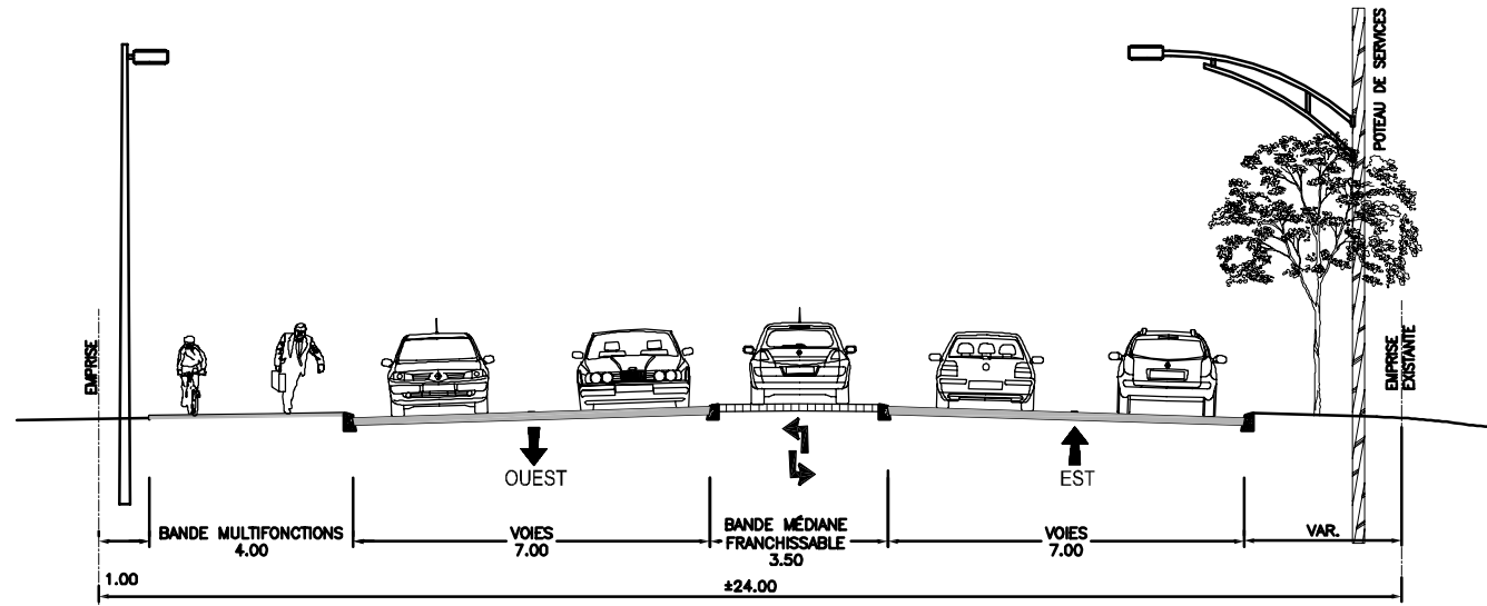
COUPE CDJ-C BOULEVARD CITÉ DES JEUNES AVEC BANDE MULTIFONCTIONS
