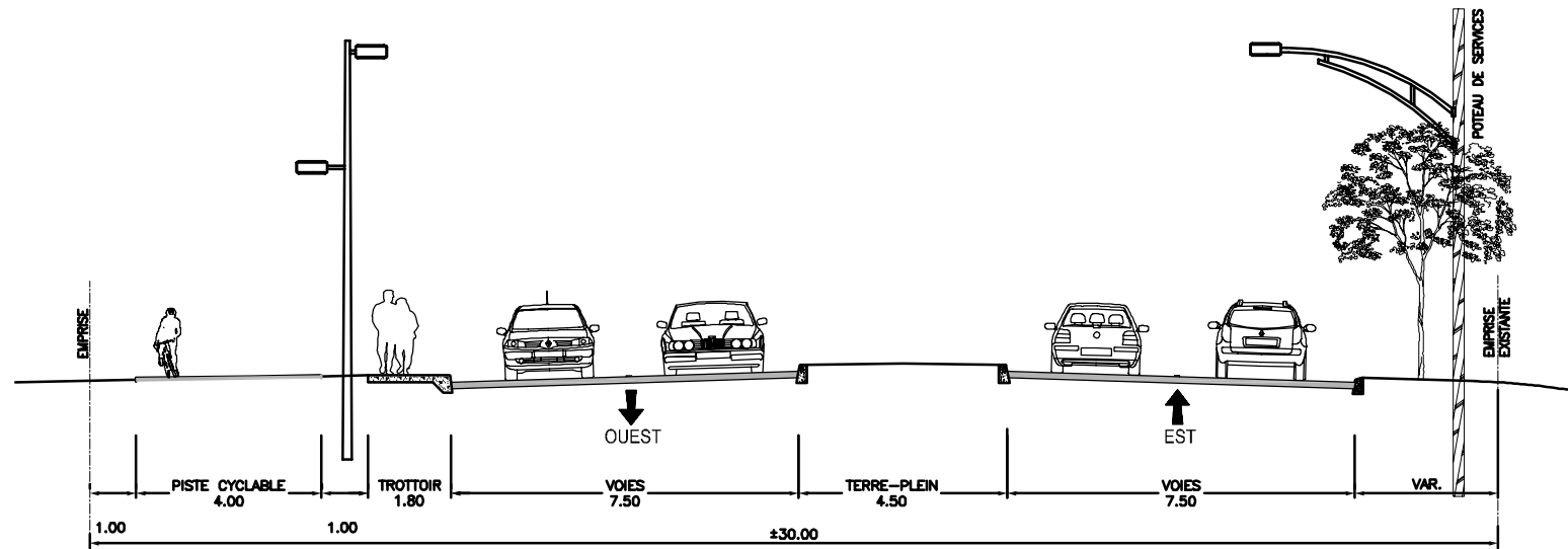
COUPE CDJ-B BOULEVARD CITÉ DES JEUNES AVEC MAIL CENTRAL SURÉLEVÉ
