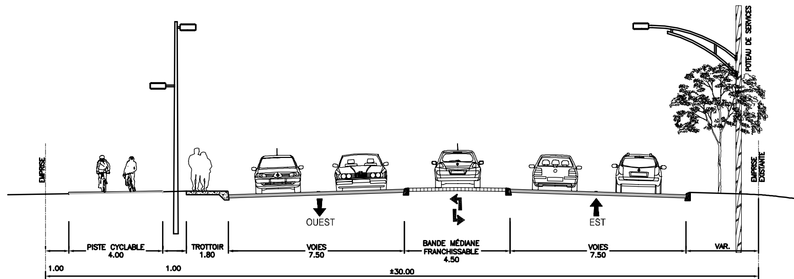
COUPE CDJ-A BOULEVARD CITÉ DES JEUNES AVEC TROTTOIR ET PISTE CYCLABLE
