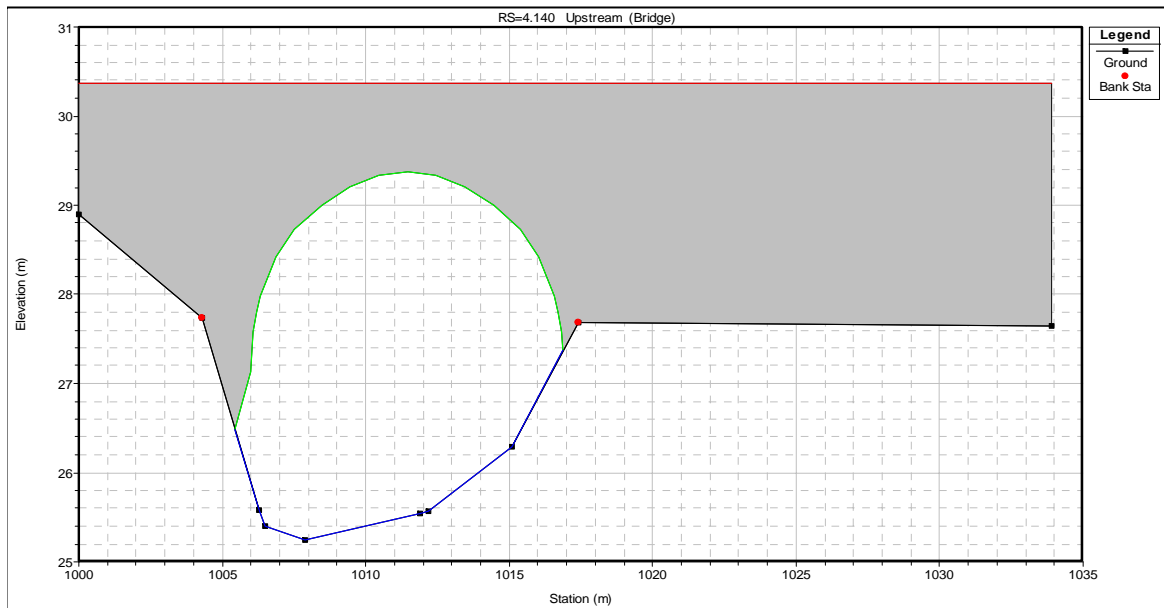
A.6(b) - Section du pont de la rue Henry-Ford
