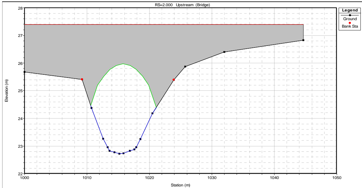
A.4(b) - Section du pont de la rue des Floralties
