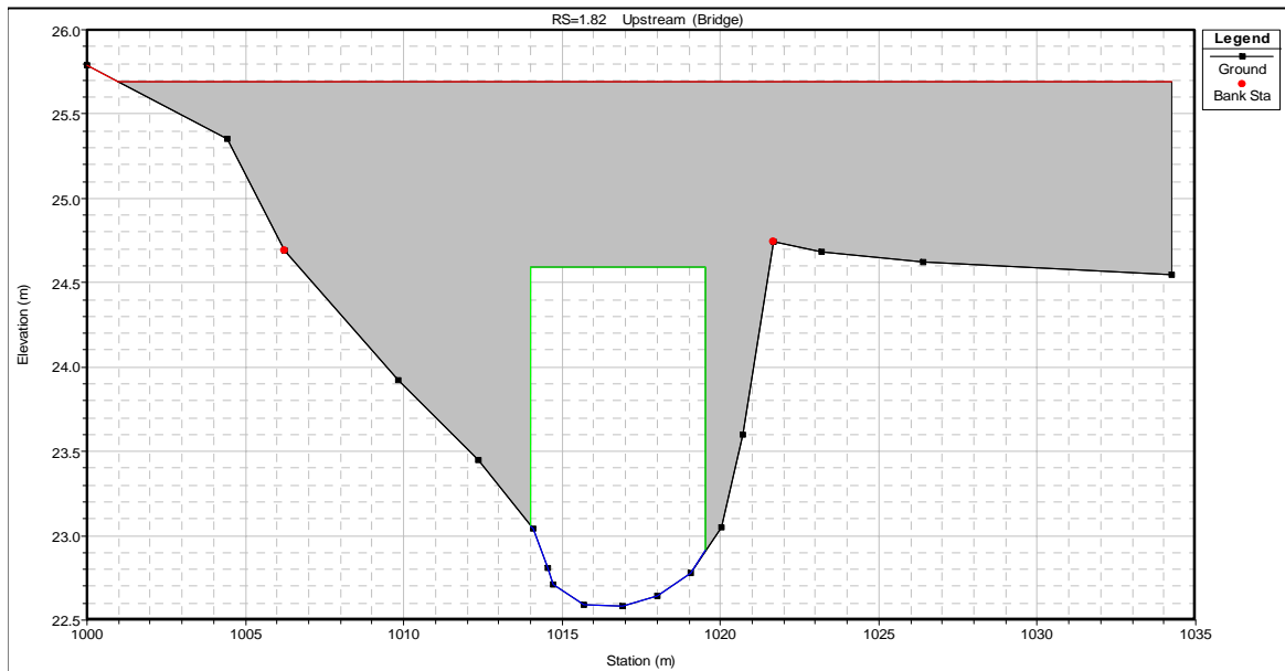
A.3(b) - Section de la traverse du chemin de fer du CP
