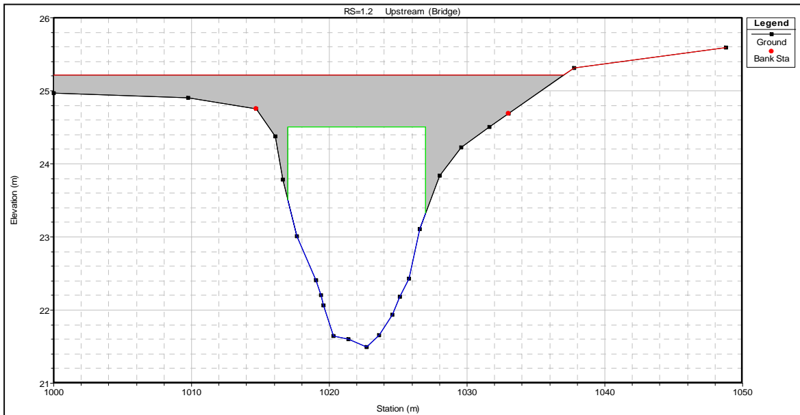
A.2(b) - Section du pont de la rue Ouimet
