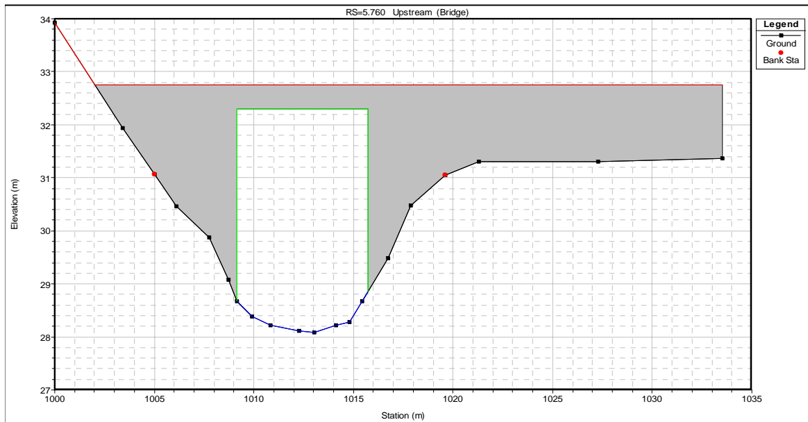
A.7(b) - Section du pont de la route Harwood
