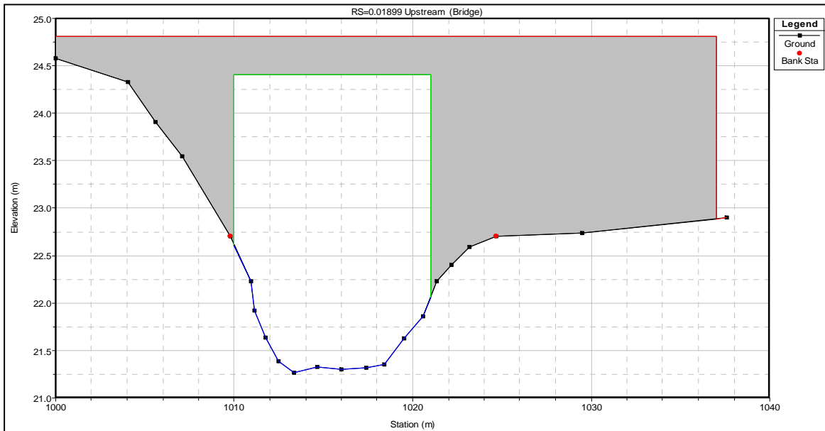
A.1(b) - Section du pont de la rue St-Charles
