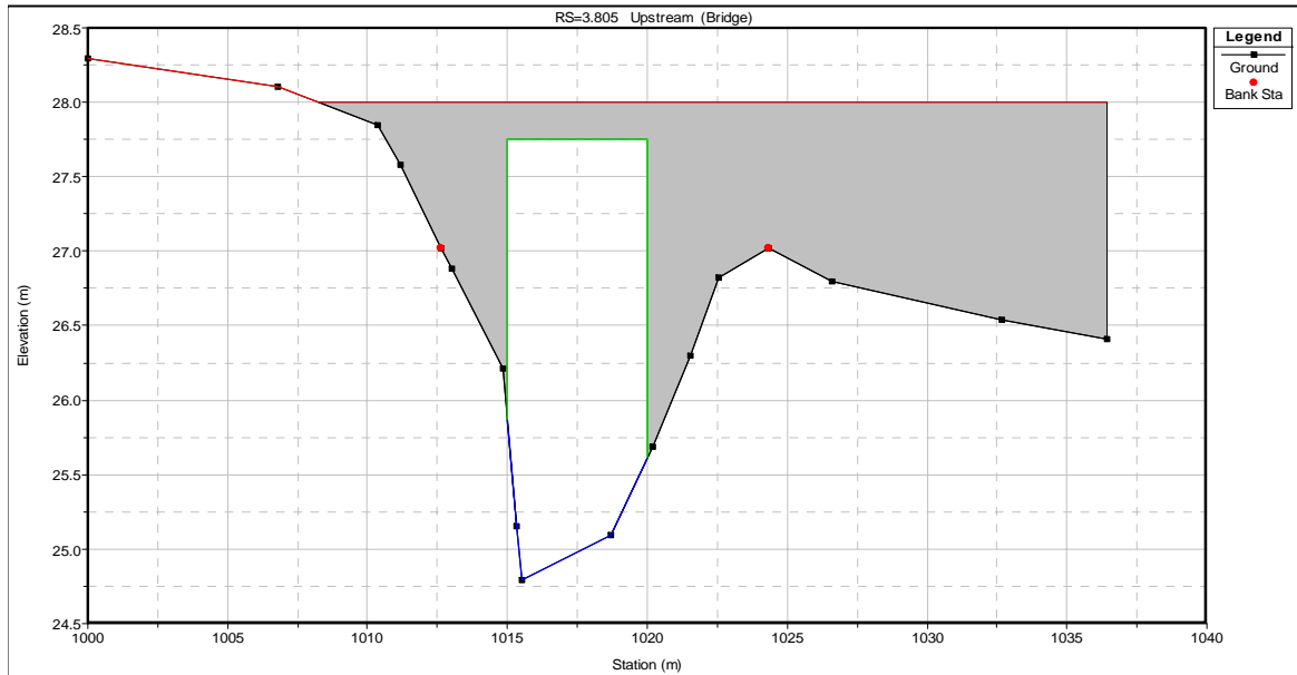
A.5(b) - Section du pont de la rue White
