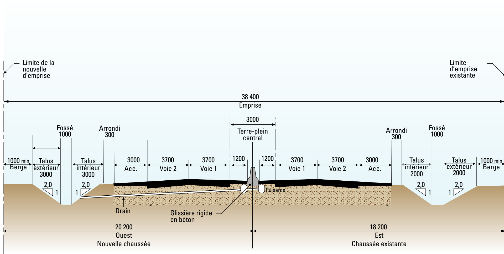
FIGURE 4.4 : Section type d'un terre-plein étroit, sans virage à gauche
