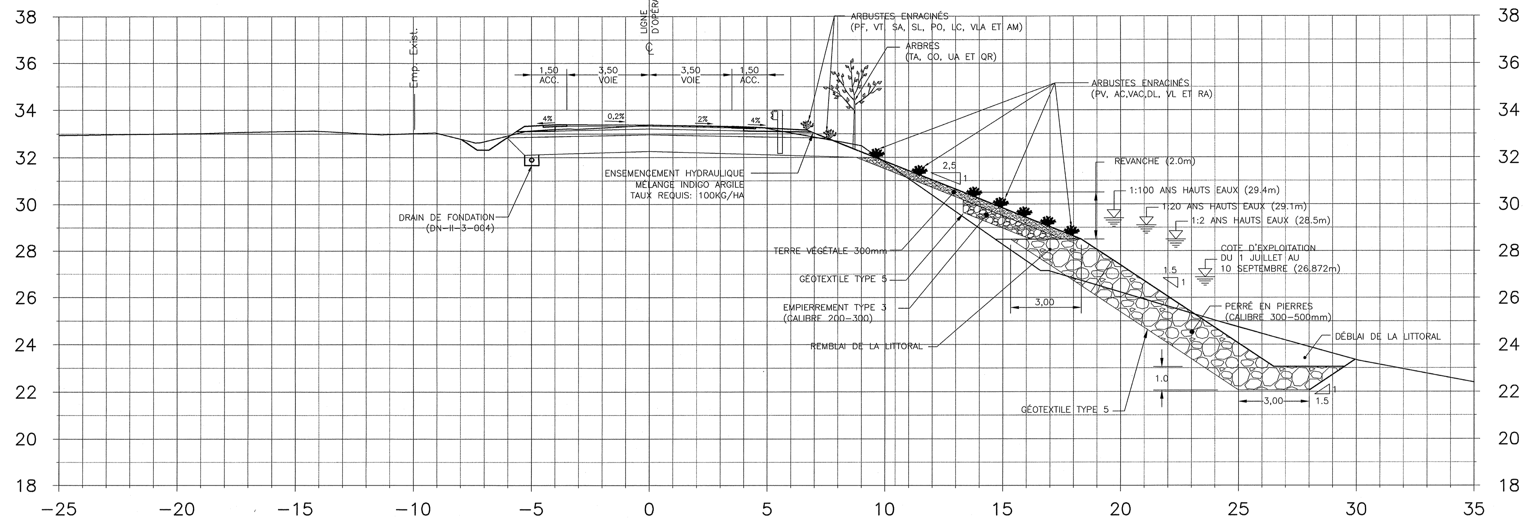
ROUTE 231 COUPE TRANSVERSALE CH. 1+620
