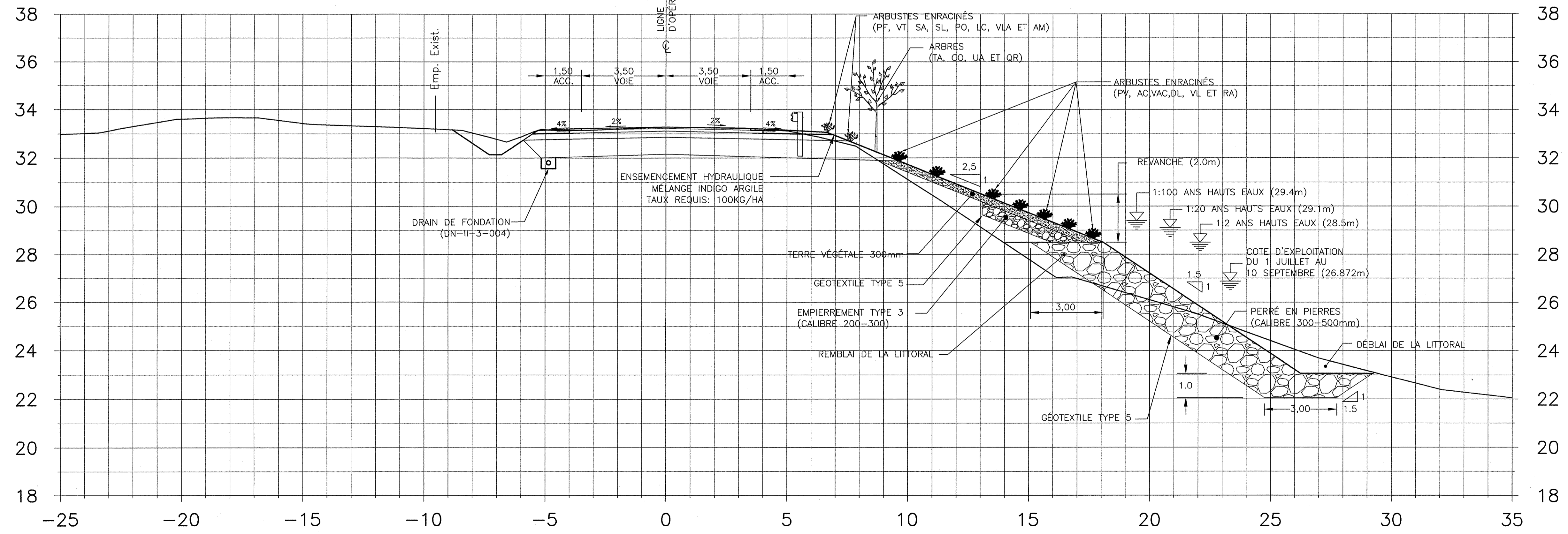
ROUTE 231 COUPE TRANSVERSALE CH. 1+660
