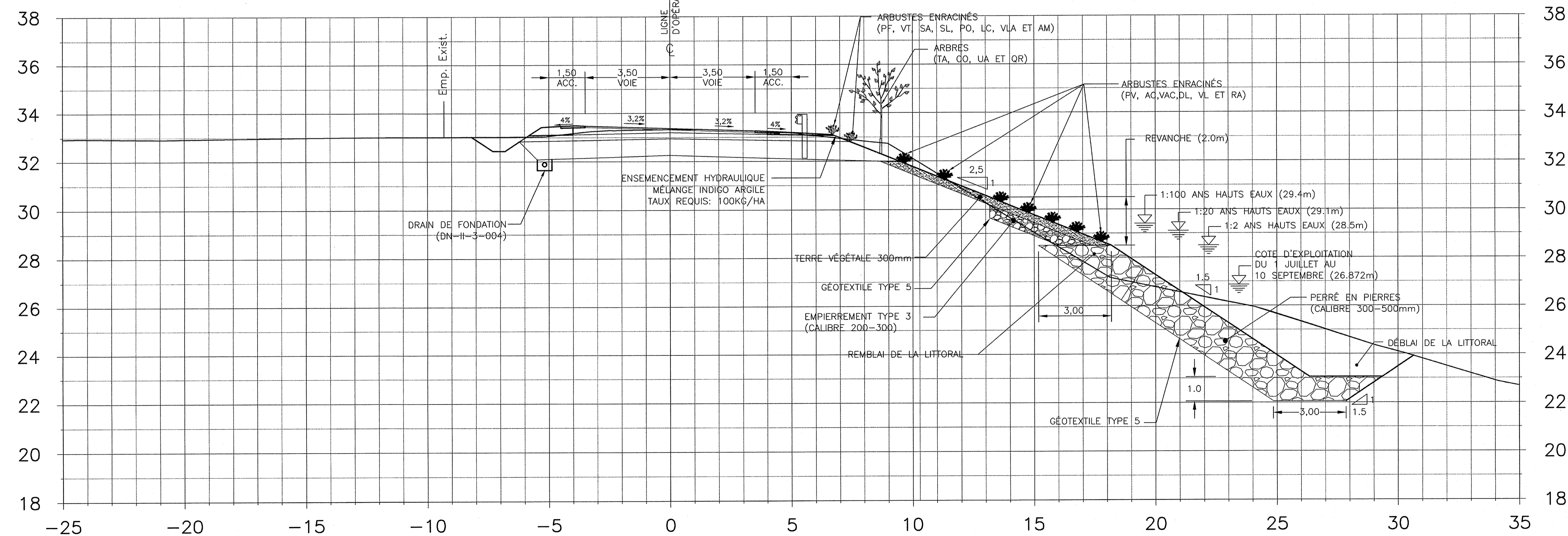
ROUTE 231 COUPE TRANSVERSALE CH. 1+500
