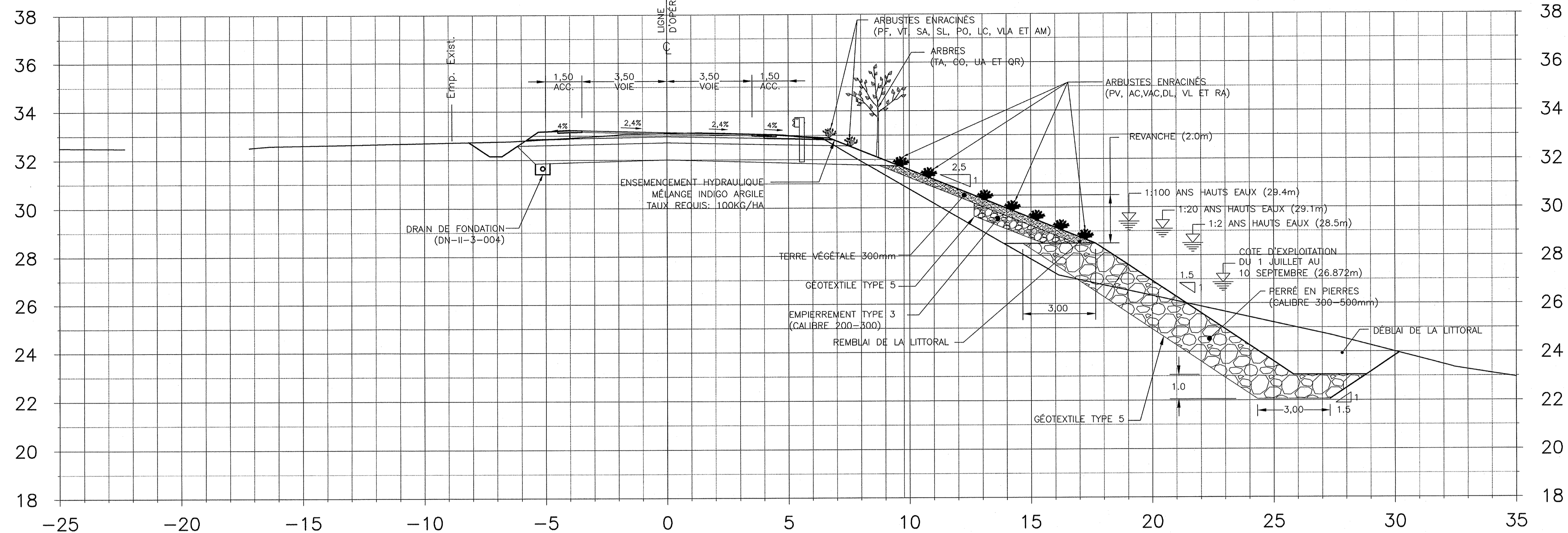
ROUTE 231 COUPE TRANSVERSALE CH. 1+460
