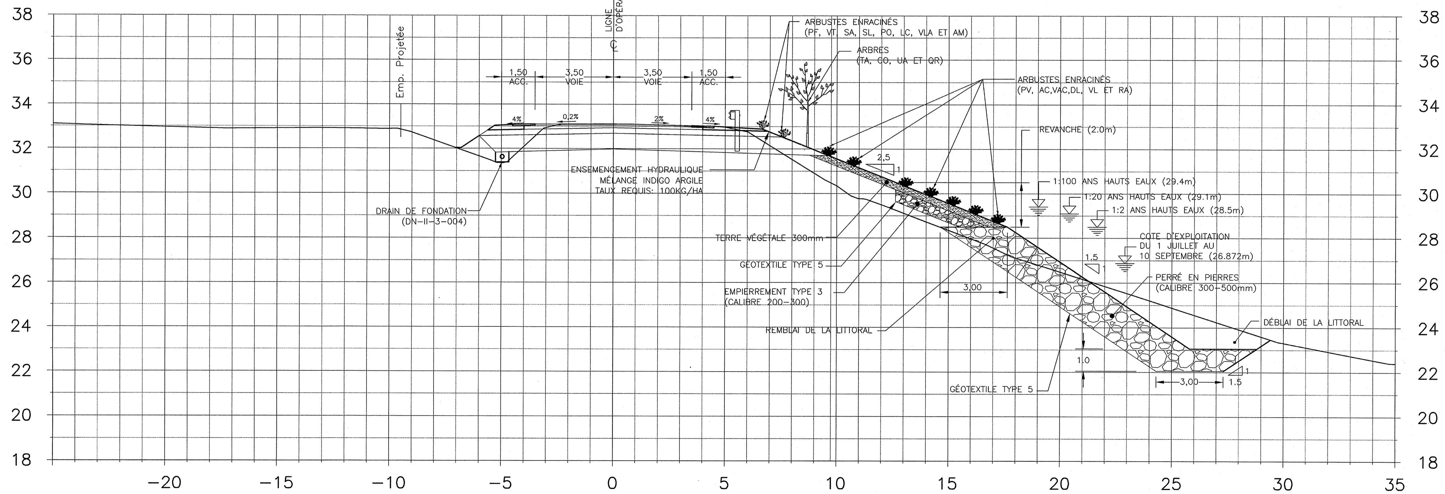
ROUTE 231 COUPE TRANSVERSALE CH. 1+420
