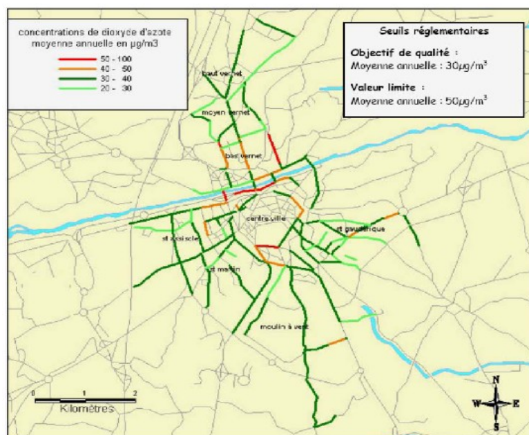
Carte des concentrations de dioxyde d'azote pour l'état initial – Évaluation environnementale du PDU de Perpignan
