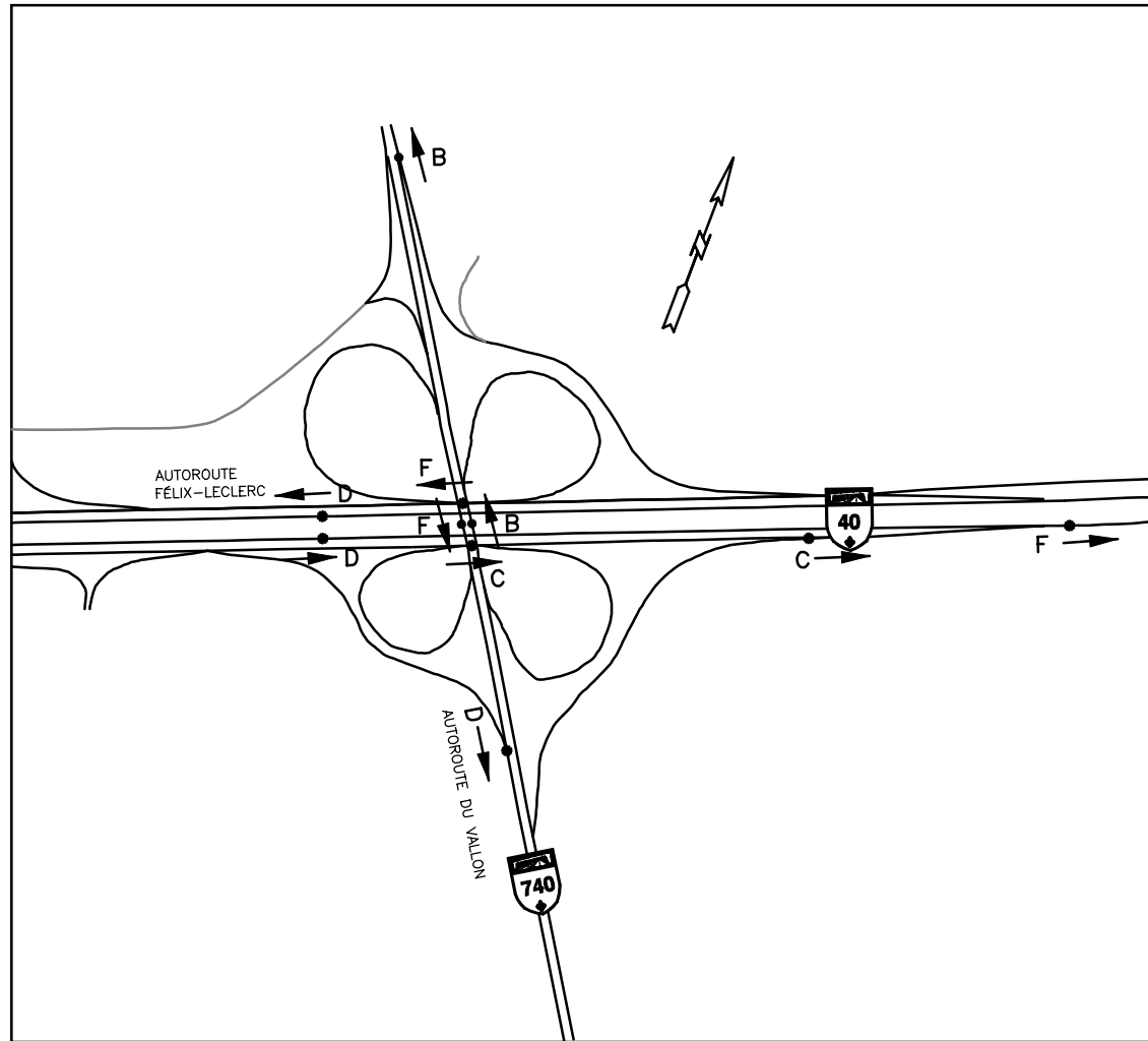
AGRANDISSEMENT ÉCHANGEUR AUTOROUTES DU VALLON (740) ET FÉLIX-LECLERC (40)
