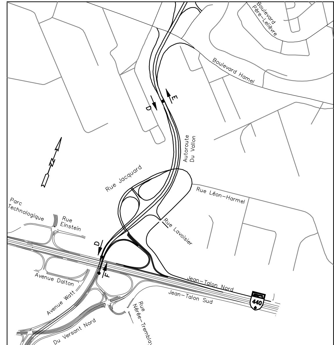
AGRANDISSEMENT ÉCHANGEUR AUTOROUTES DU VALLON (740) ET CHAREST (440)
