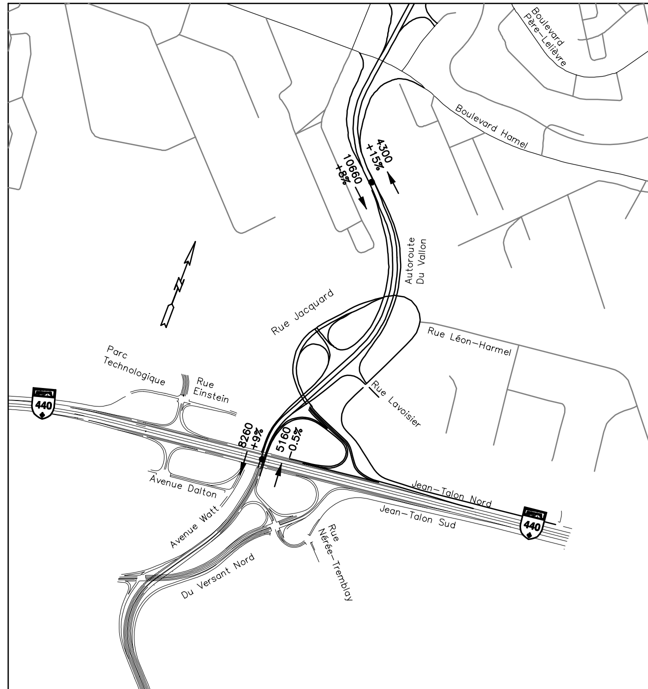
AGRANDISSEMENT ÉCHANGEUR AUTOROUTES DU VALLON (740) ET CHAREST (440)
