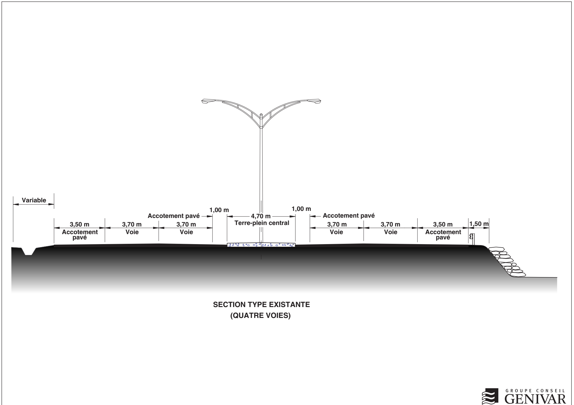
Figure 4.1 Profil en travers type du boulevard Champlain actuel.
