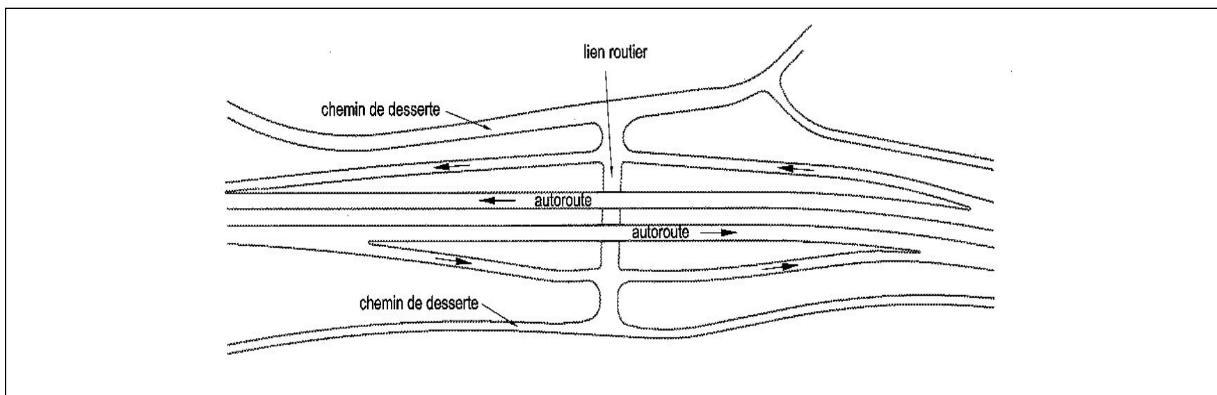
Figure 5.2 – Carrefour dénivelé de type losange
