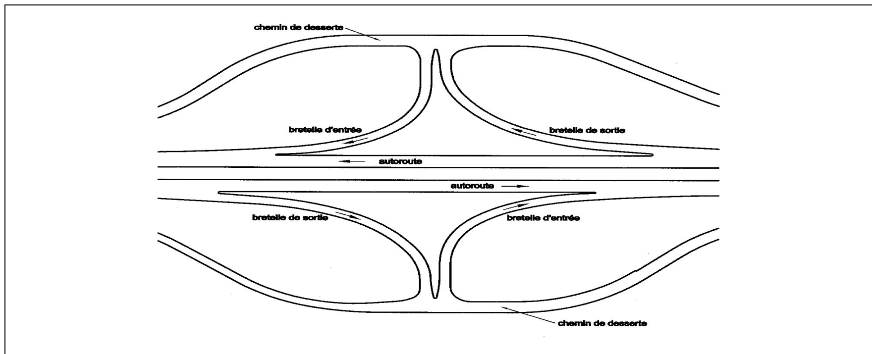
Figure 5.1 – Carrefour dénivelé de type trèfle modifié
