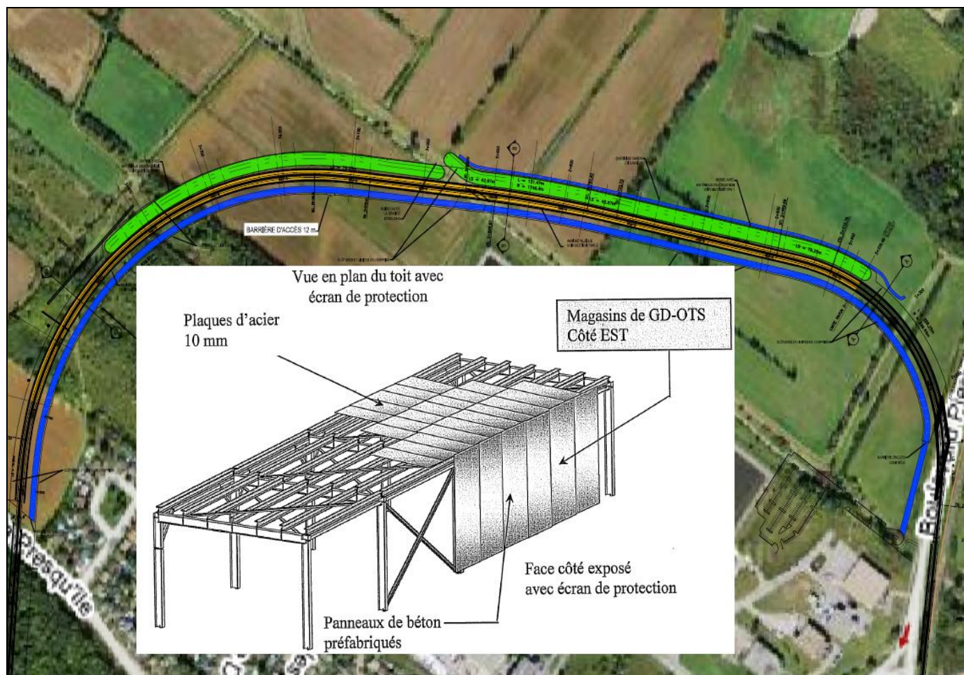
FIGURE 6 : BERME DE TERRE ET STRUCTURE MÉTALLIQUE AVEC TOIT ENVISAGÉES LE LONG DU PARCOURS DE LA VOIE FERRÉE SUR LES TERRAINS DE GENERAL DYNAMICS
