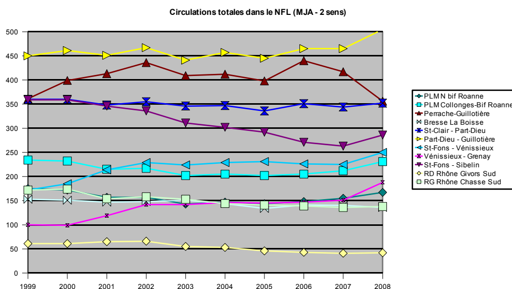
Graphique d'évolution du trafic moyen journalier annuel
