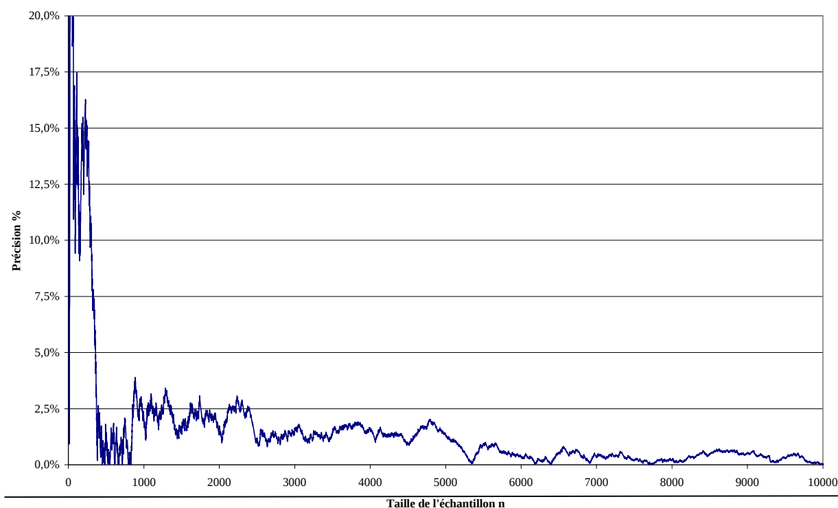
Figure 2 : variation de la précision de la mesure en fonction de la taille de l'échantillon (exemple)
