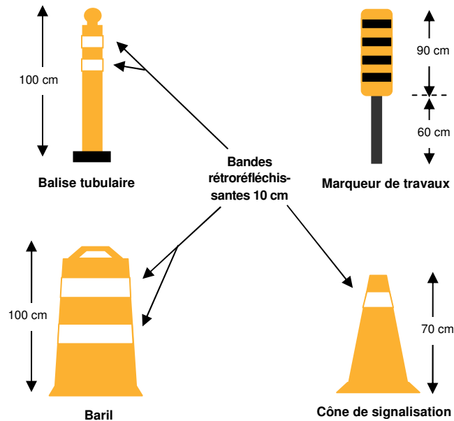
Figure 3-2 : Dispositifs de balisage
