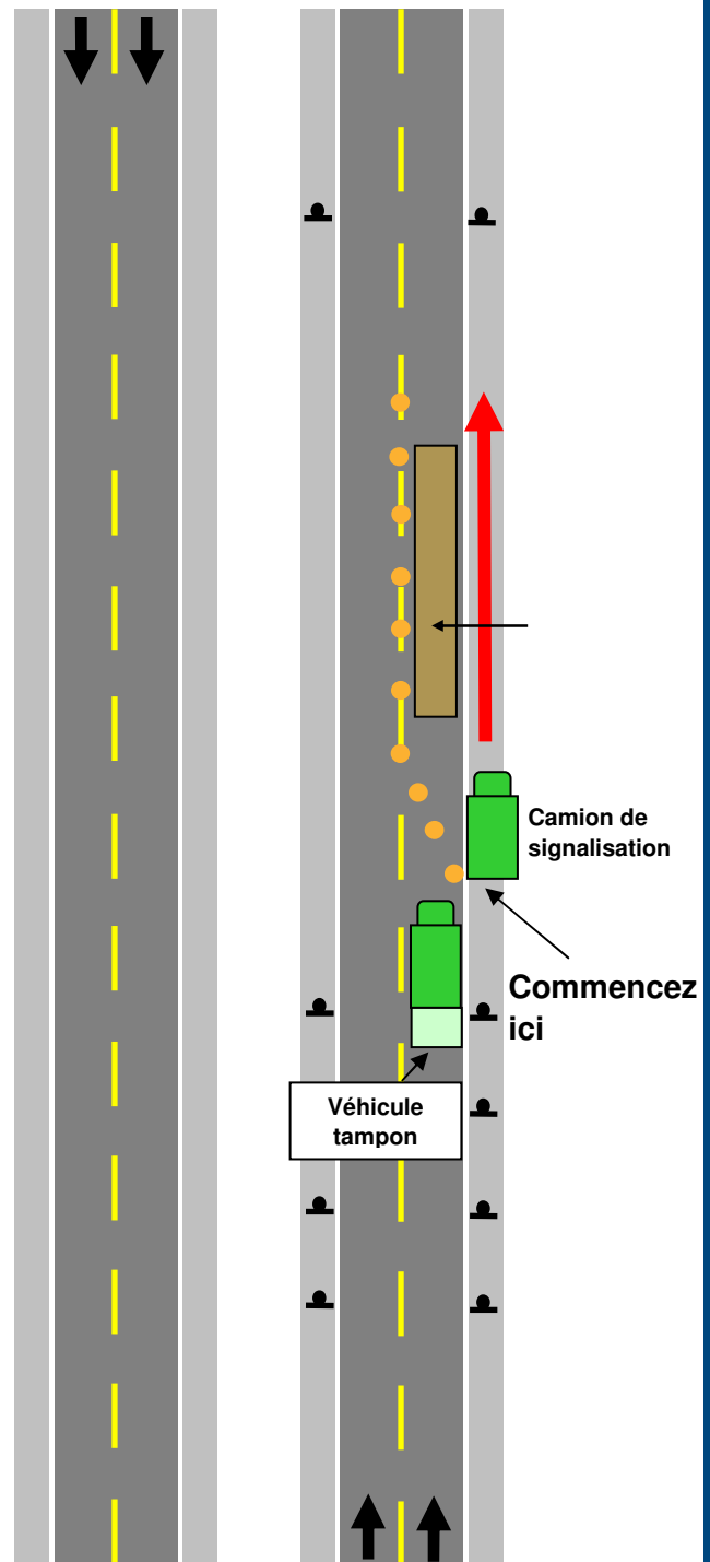
Figure 4-8 : Installation en cas de fermeture d'une voie (routes à voies multiples à chaussées séparées)
