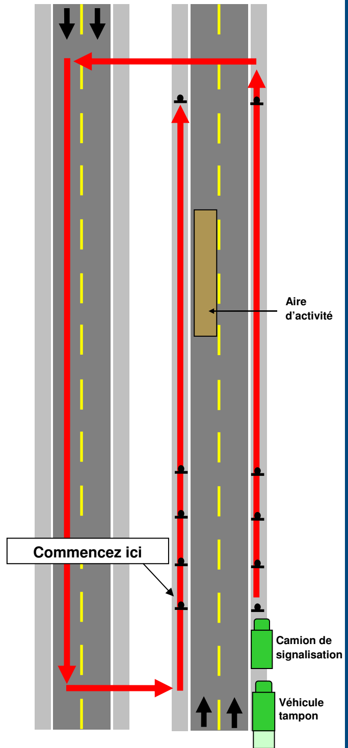
Figure 4-7 : Installation des panneaux (routes à voies multiples à chaussées séparées)
