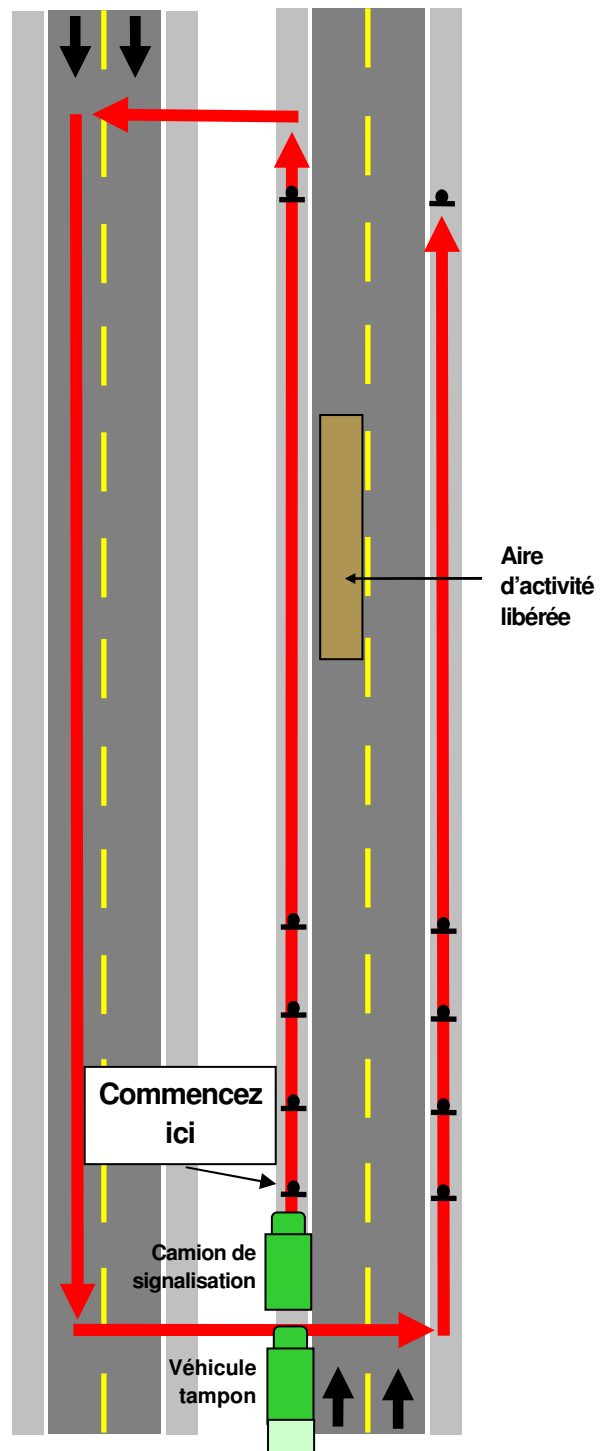
Figure 4-10 : Enlèvement des panneaux (routes à voies multiples à chaussées séparées)
