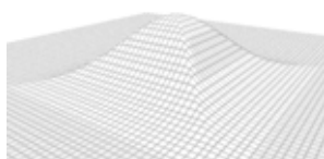
Fonction gaussienne
