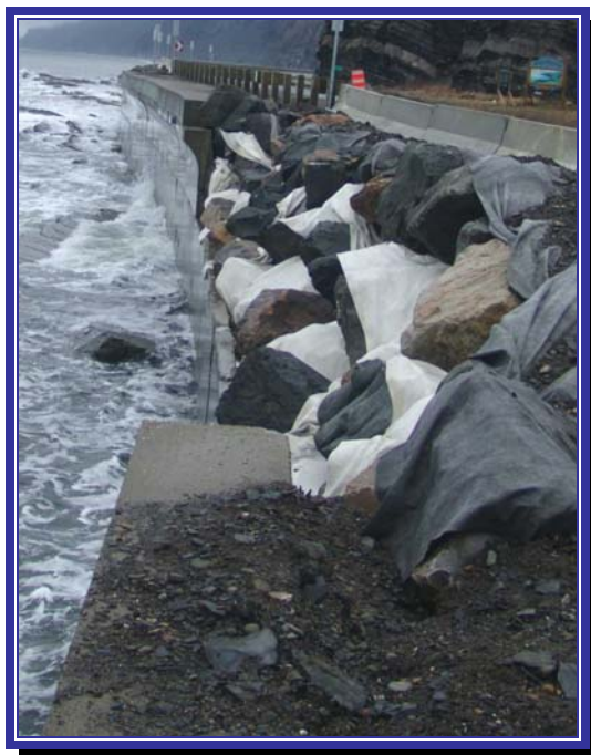
FIGURE 2 : SECTION DE 30 M DE LA PARTIE SUPÉRIEURE DU MUR À RÉPARER (LOUIS BELZILE, MAI 2008).
