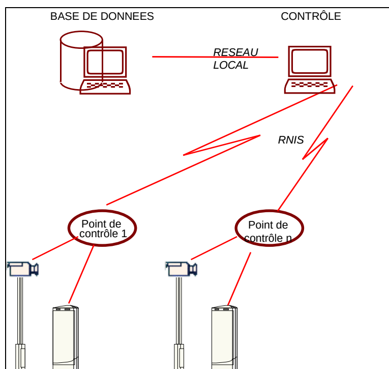
Figure 8 : Contrôle automatique basée sur un système avancé de traitement d'image (Digidock) à Barcelone
